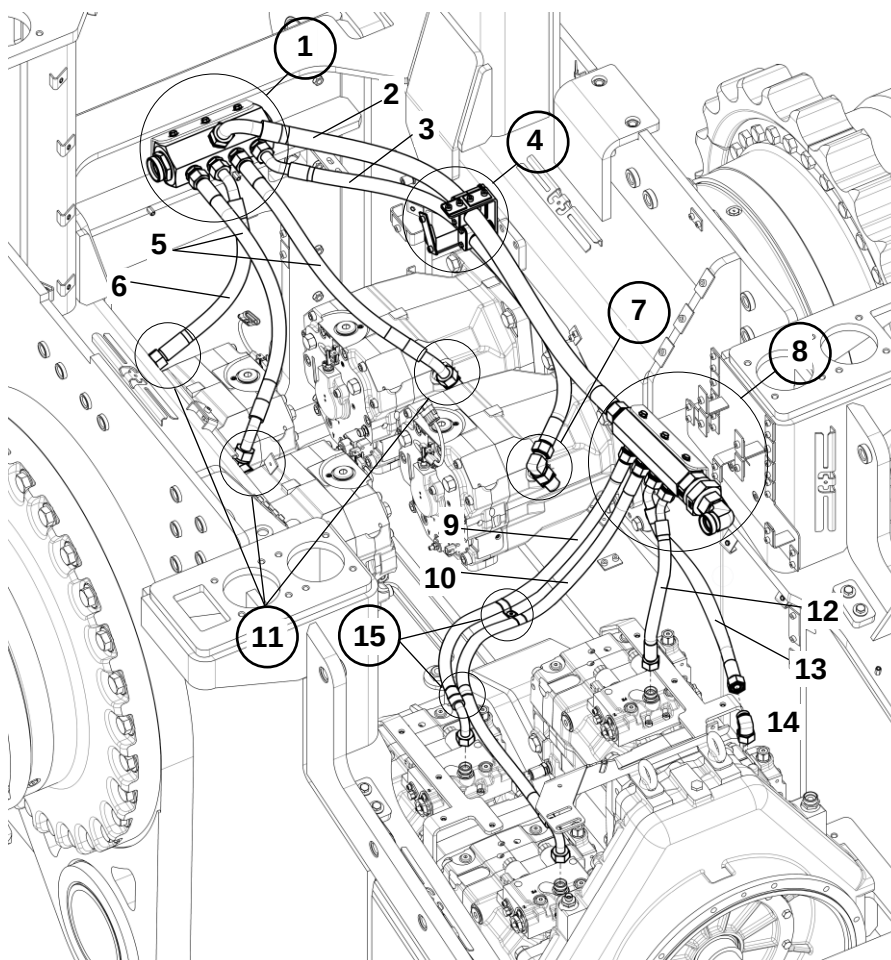
Трубопроводы гидросистемы трансмиссии
