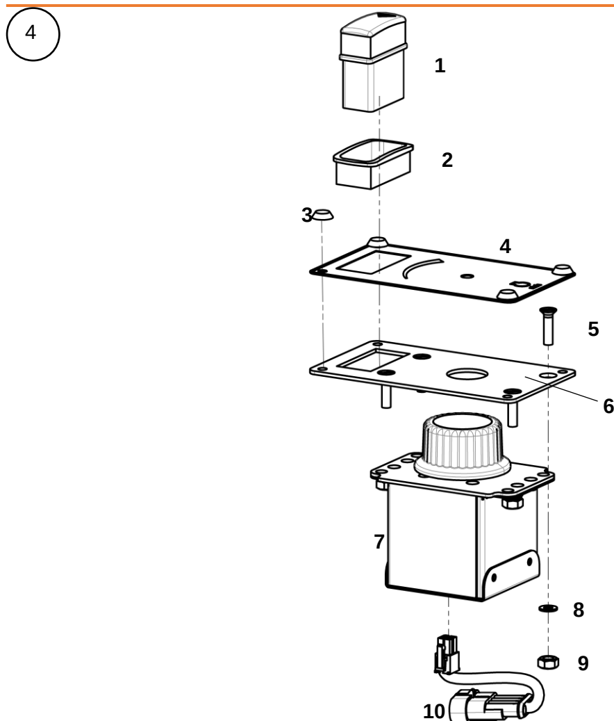
Панель управления
