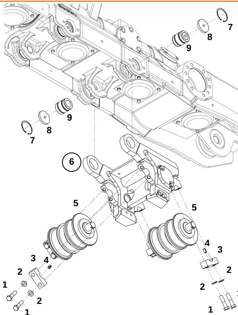
Каретка средняя в сборе
