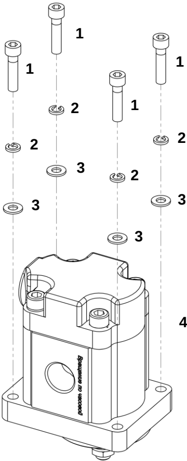
Гидромотор шестеренный
