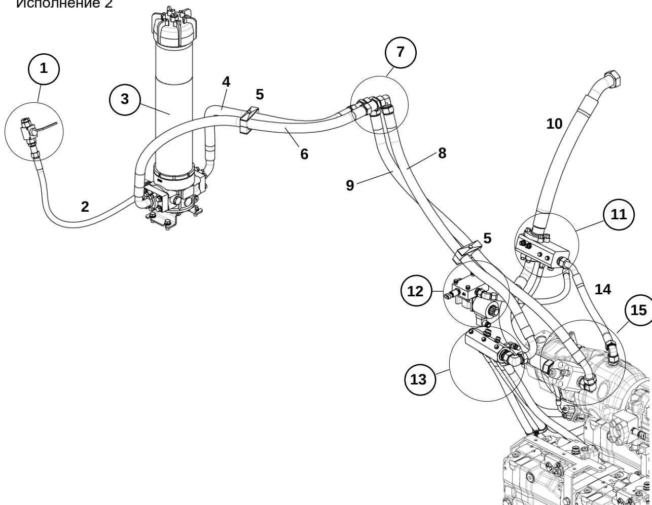
Трубопроводы гидросистемы трансмиссии
