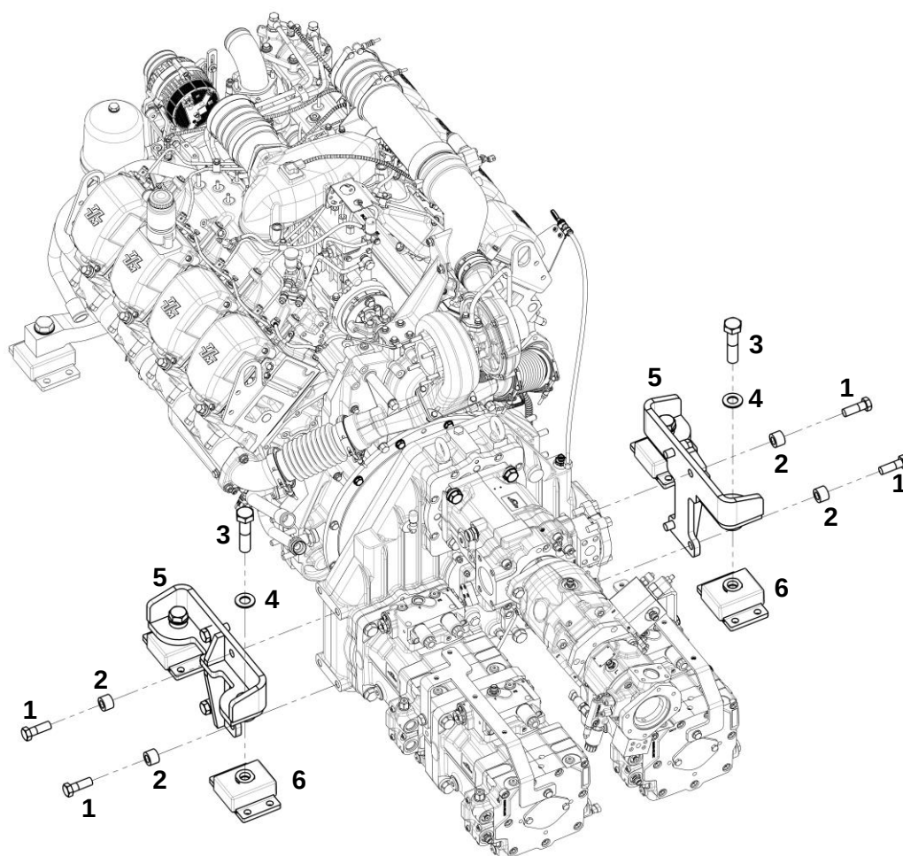
Силовой агрегат в сборе
