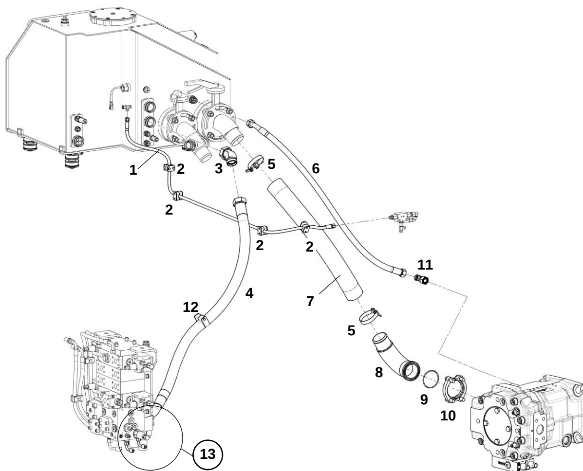
Трубопроводы гидросистемы навесного оборудования
