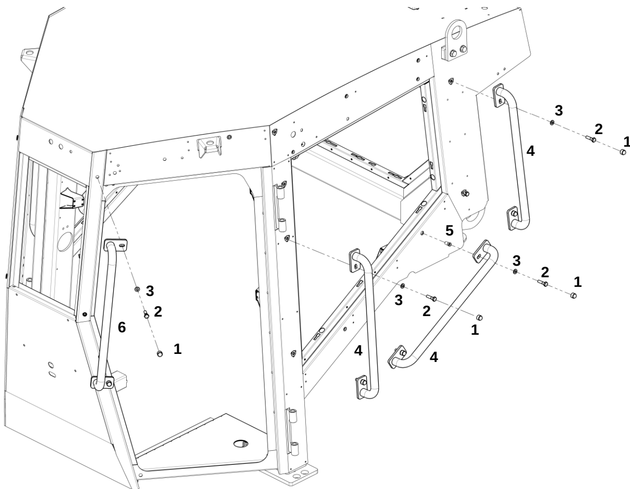
Поручни кабины слева
