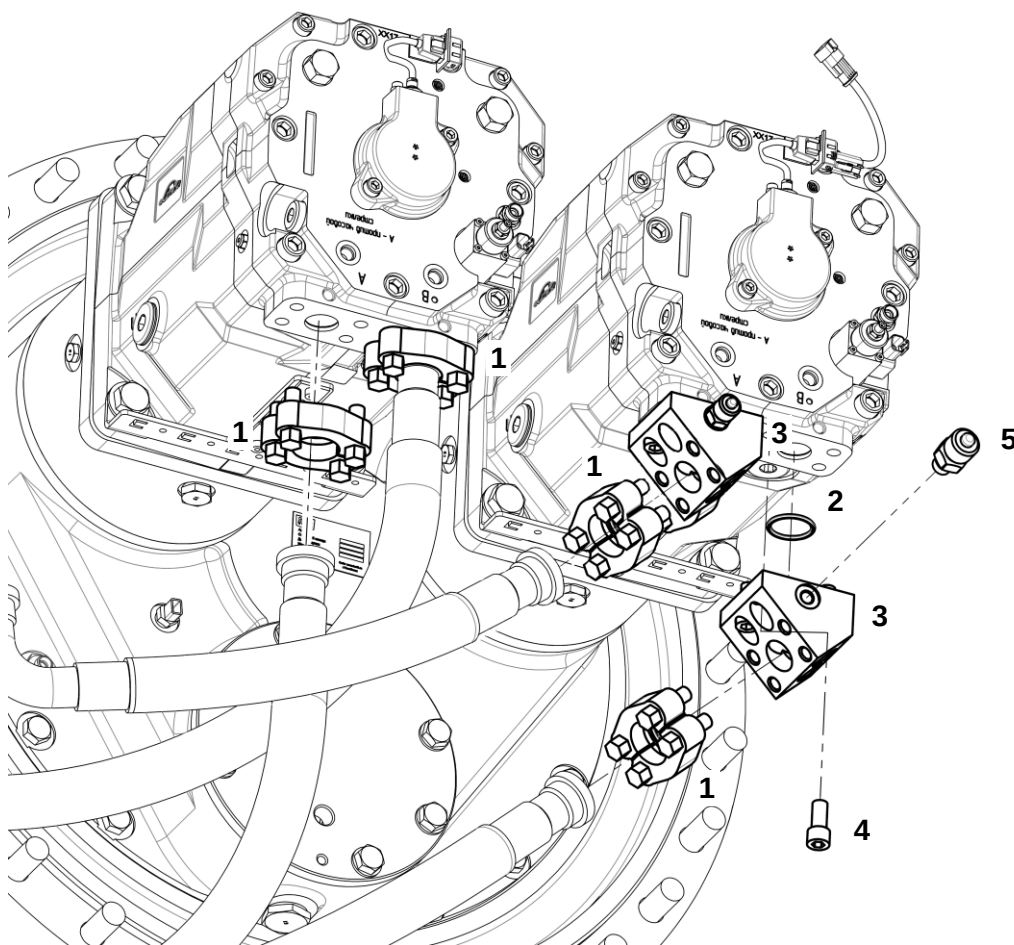
Крепление РВД к приводу хода
