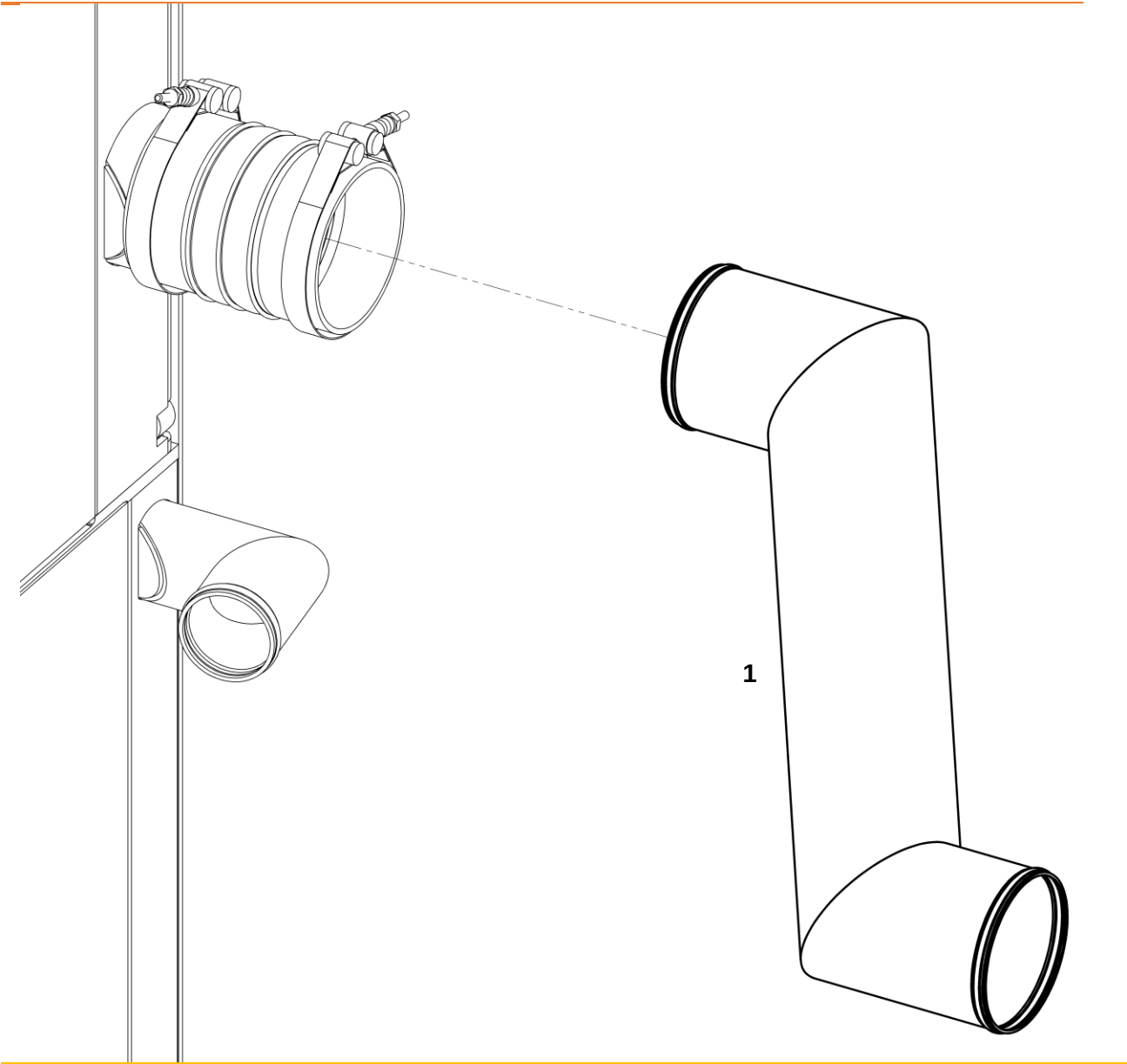
Трубопровод ОНВ
