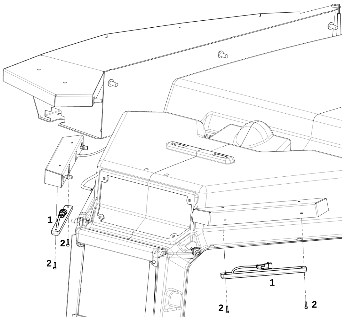
Элементы освещения кабины
