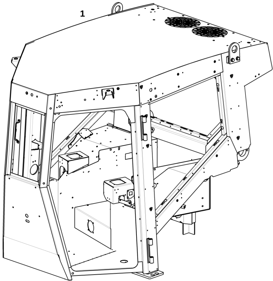
Каркас кабины
