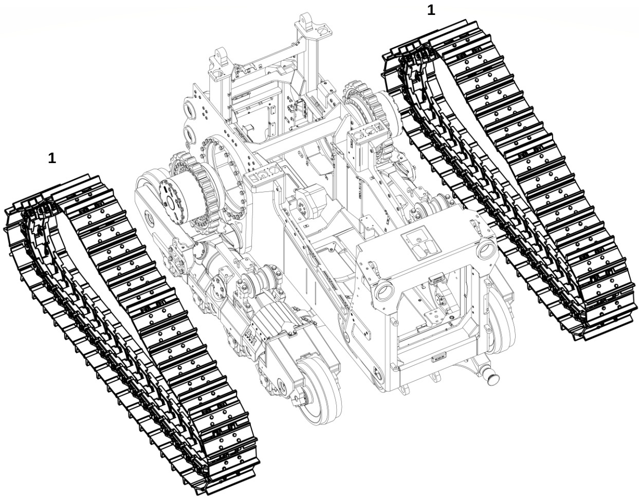
Система гусеничная
