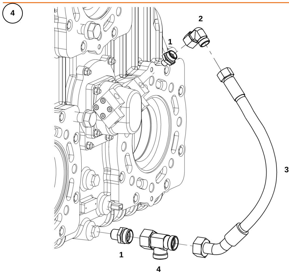
Крепление рукава к раздаточному редуктору
