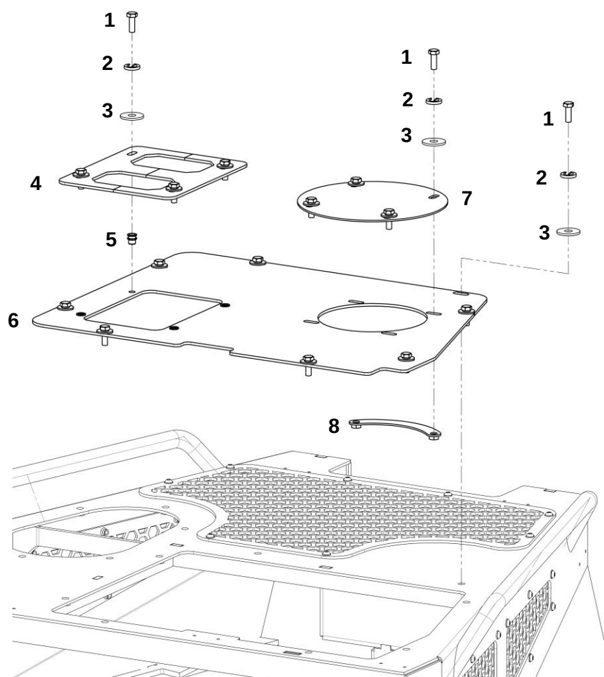
Капот в сборе
