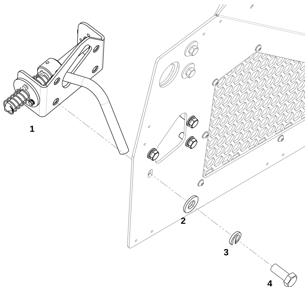
Створка в сборе
