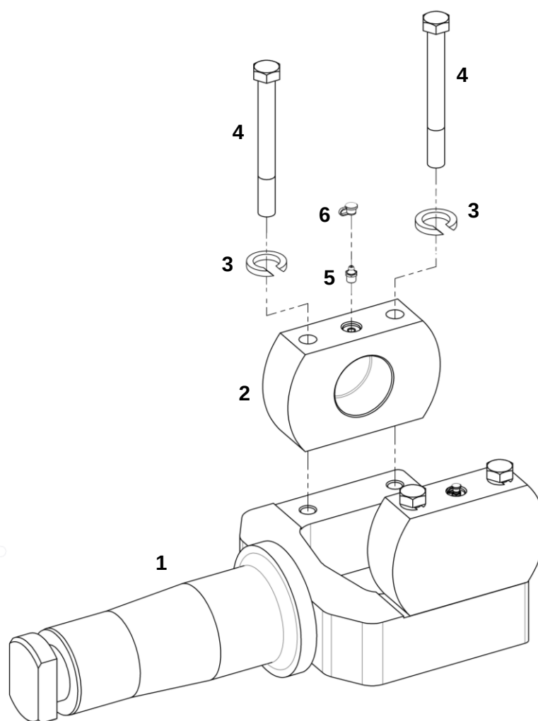
Вилка в сборе
