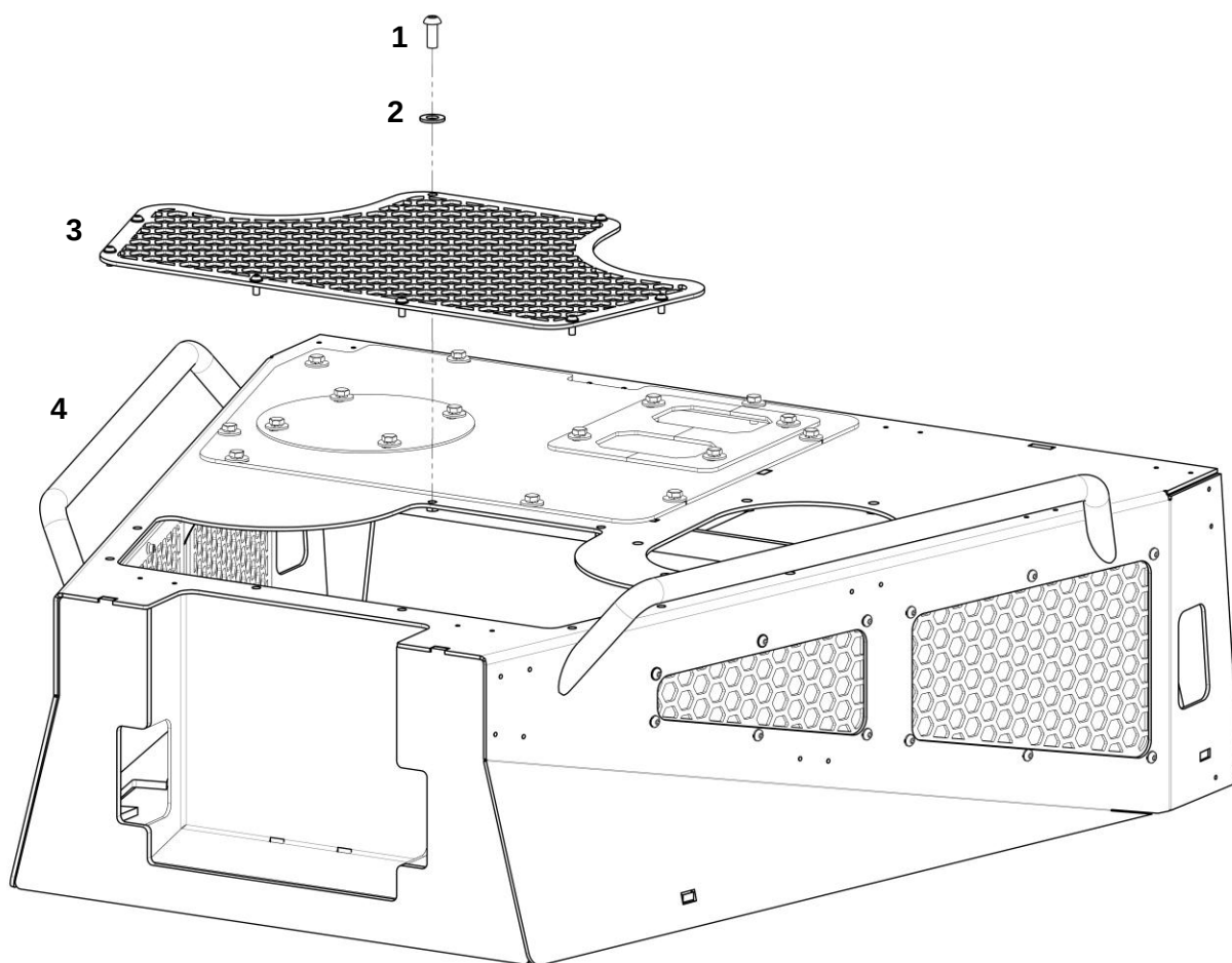
Капот в сборе
