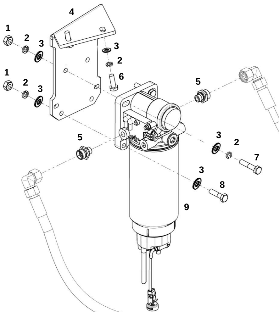
Крепление фильтра грубой очистки топлива
