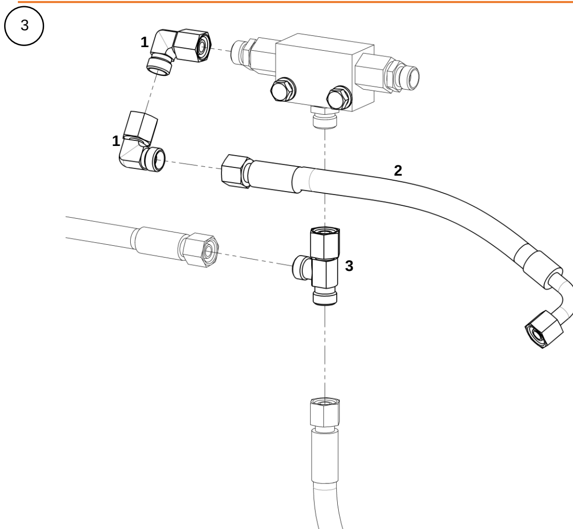
Подключение клапана ИЛИ
