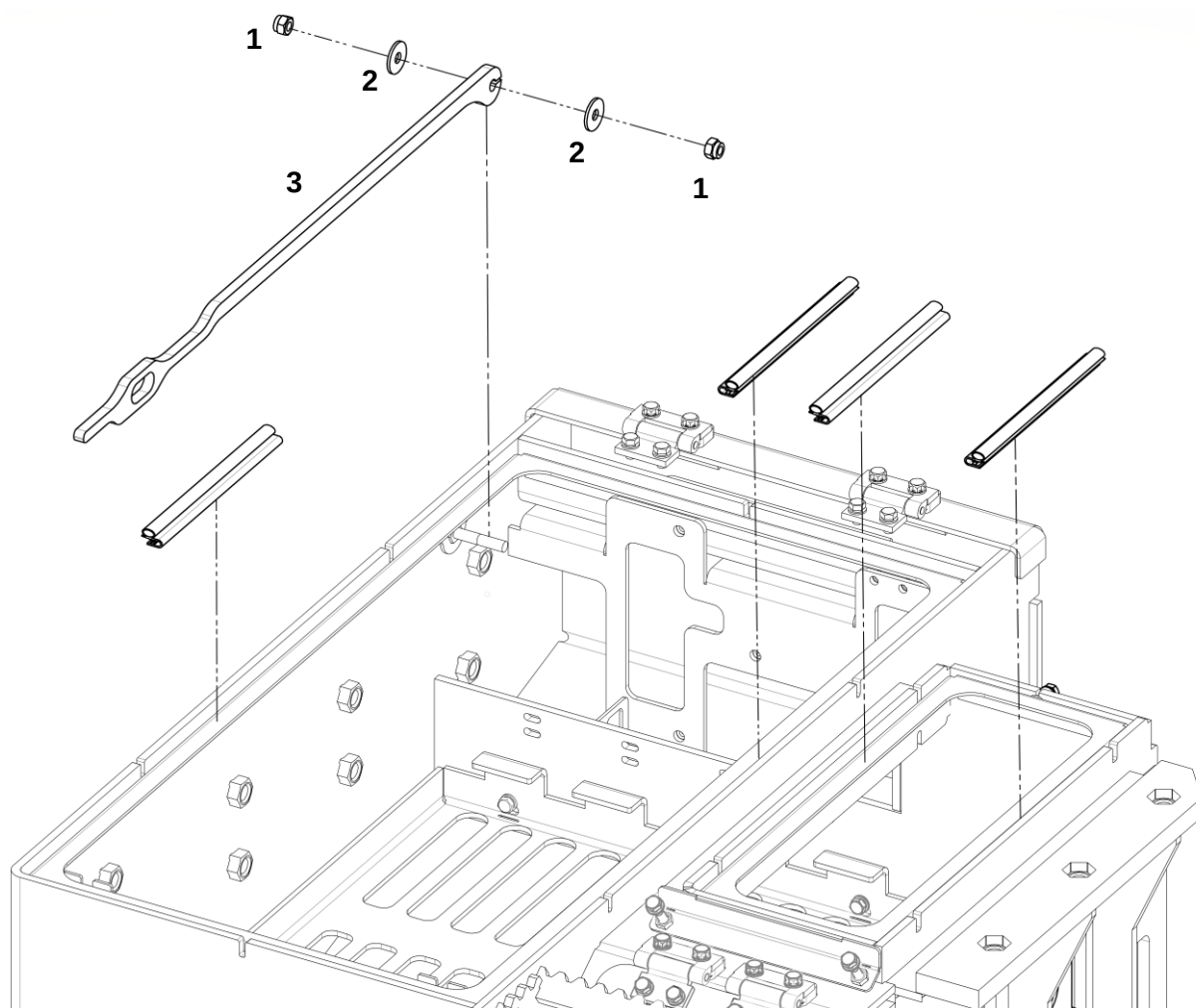
Подножка
