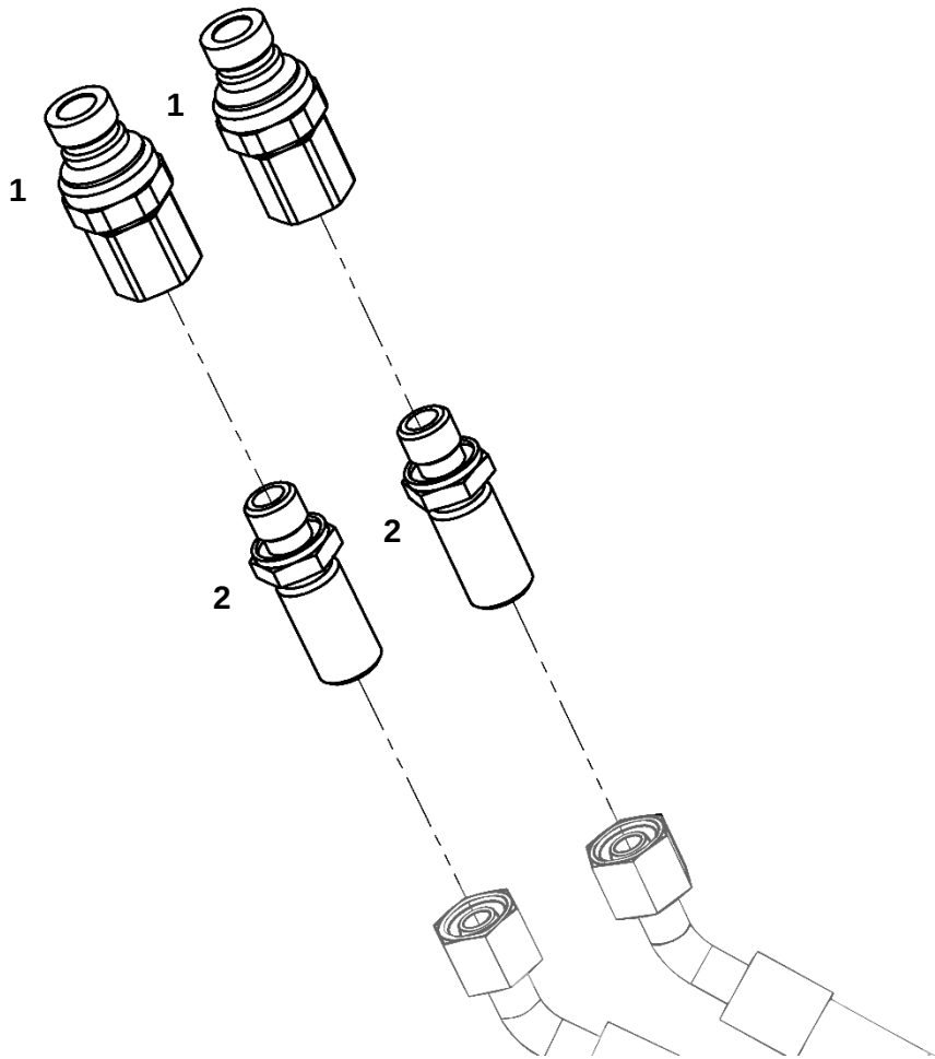
Крепление РВД к системе подъема кабины
