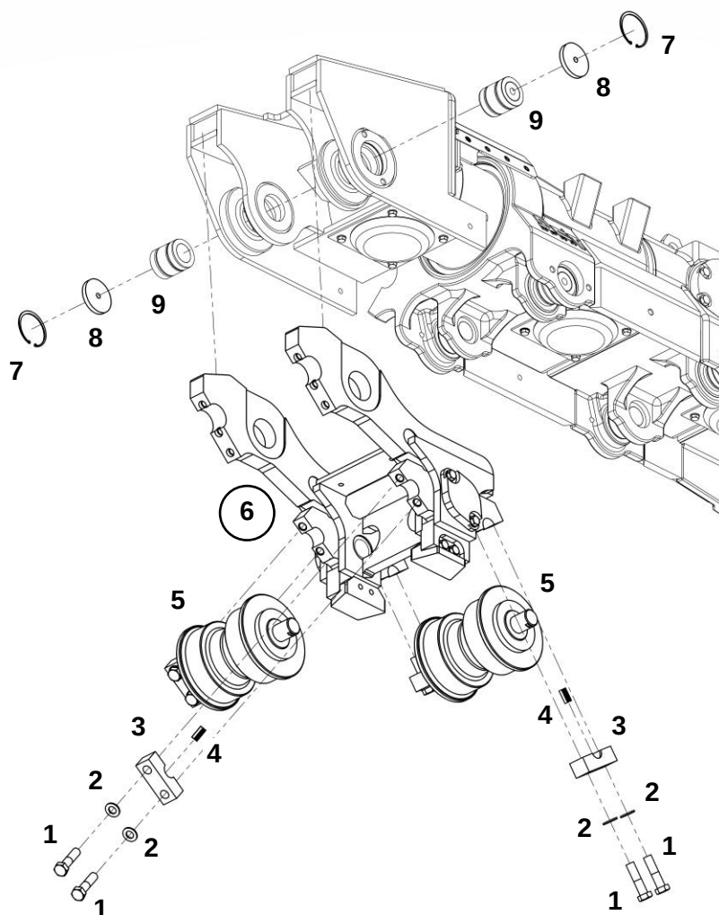
Каретка передняя в сборе
