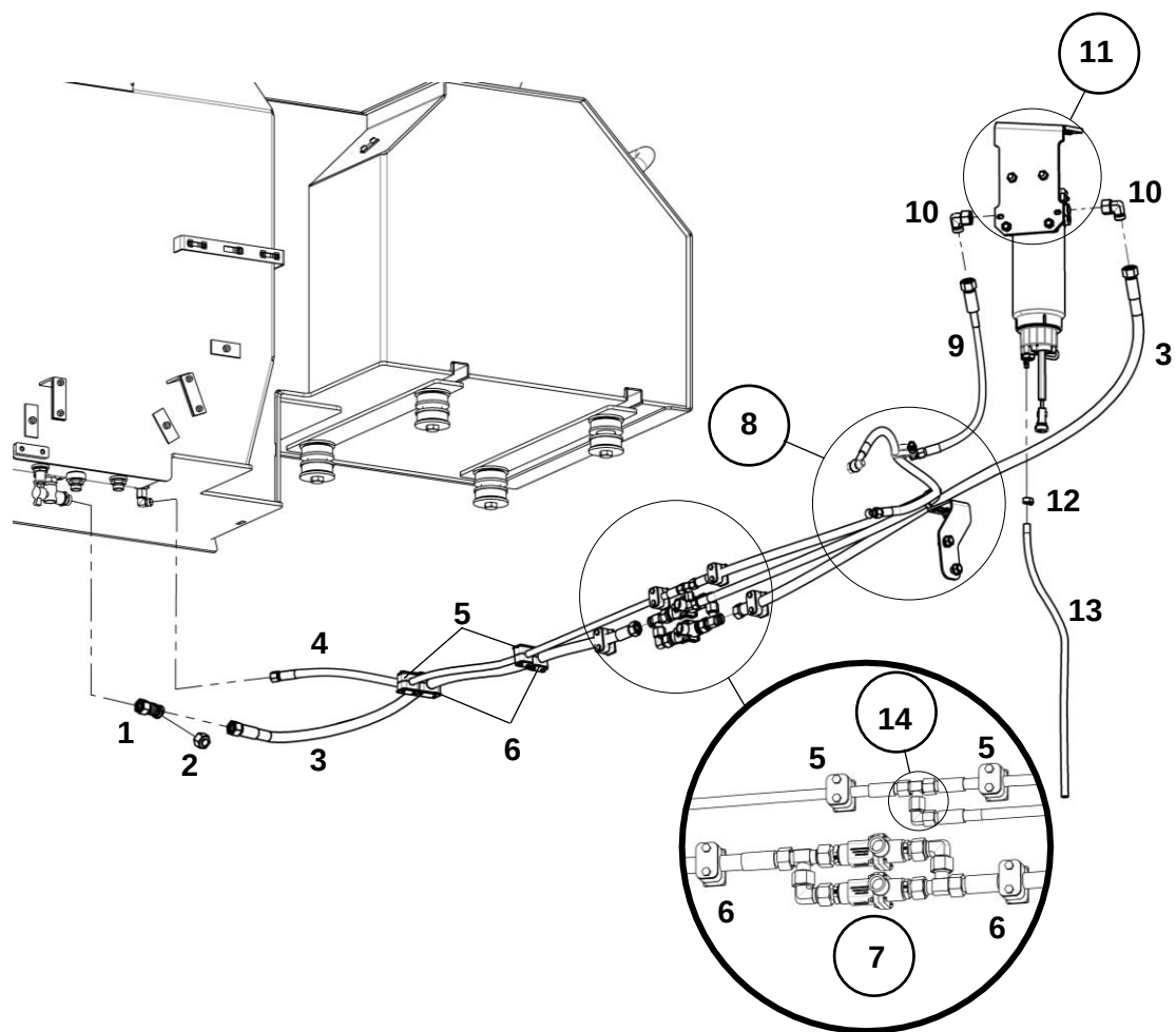
Система топливная
