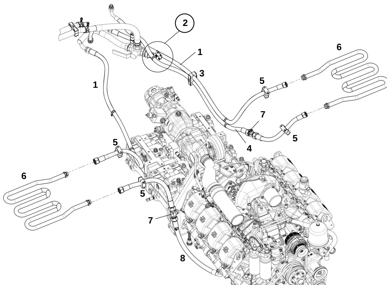
Система предпускового подогрева двигателя
