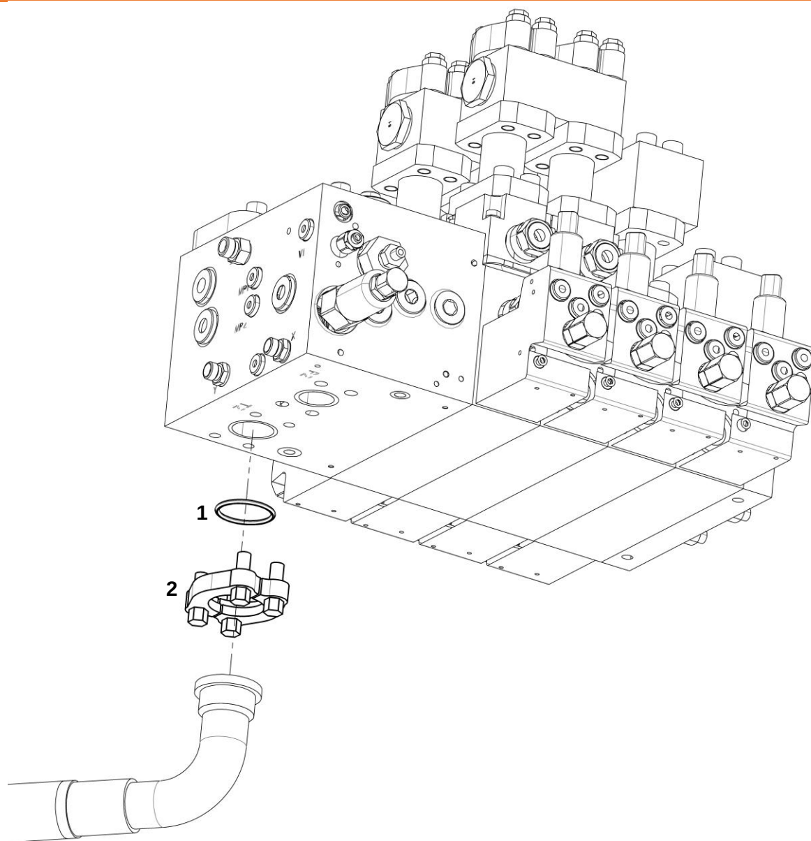
Соединение с гидрораспределителем отвала
