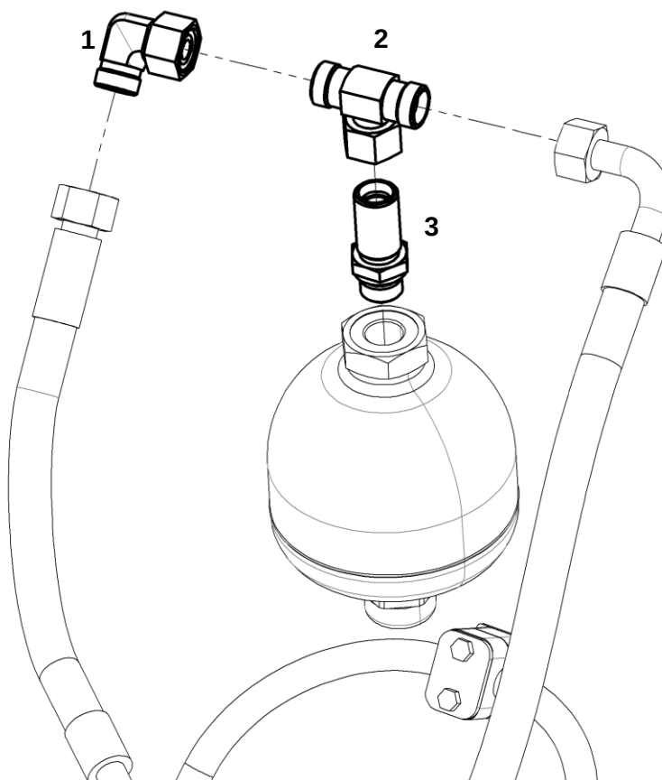
Соединение с гидроаккумулятором
