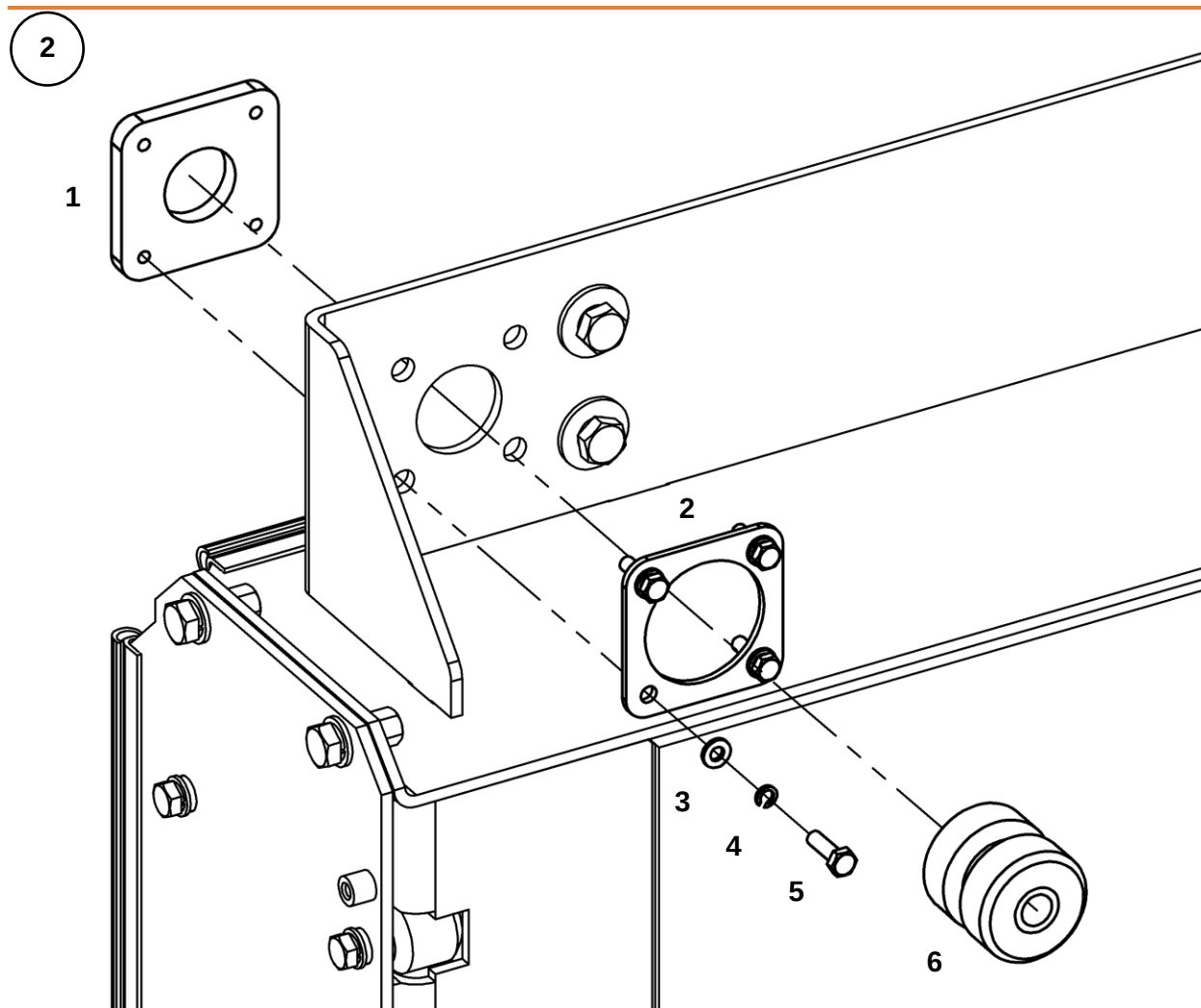
Установка виброизолятора к блоку радиатора
