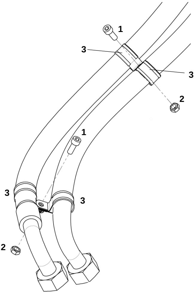
Крепление хомутов
