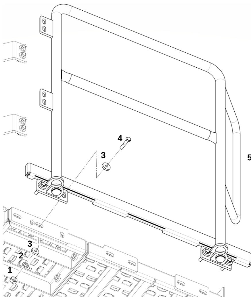
Боковые опоры в сборе
