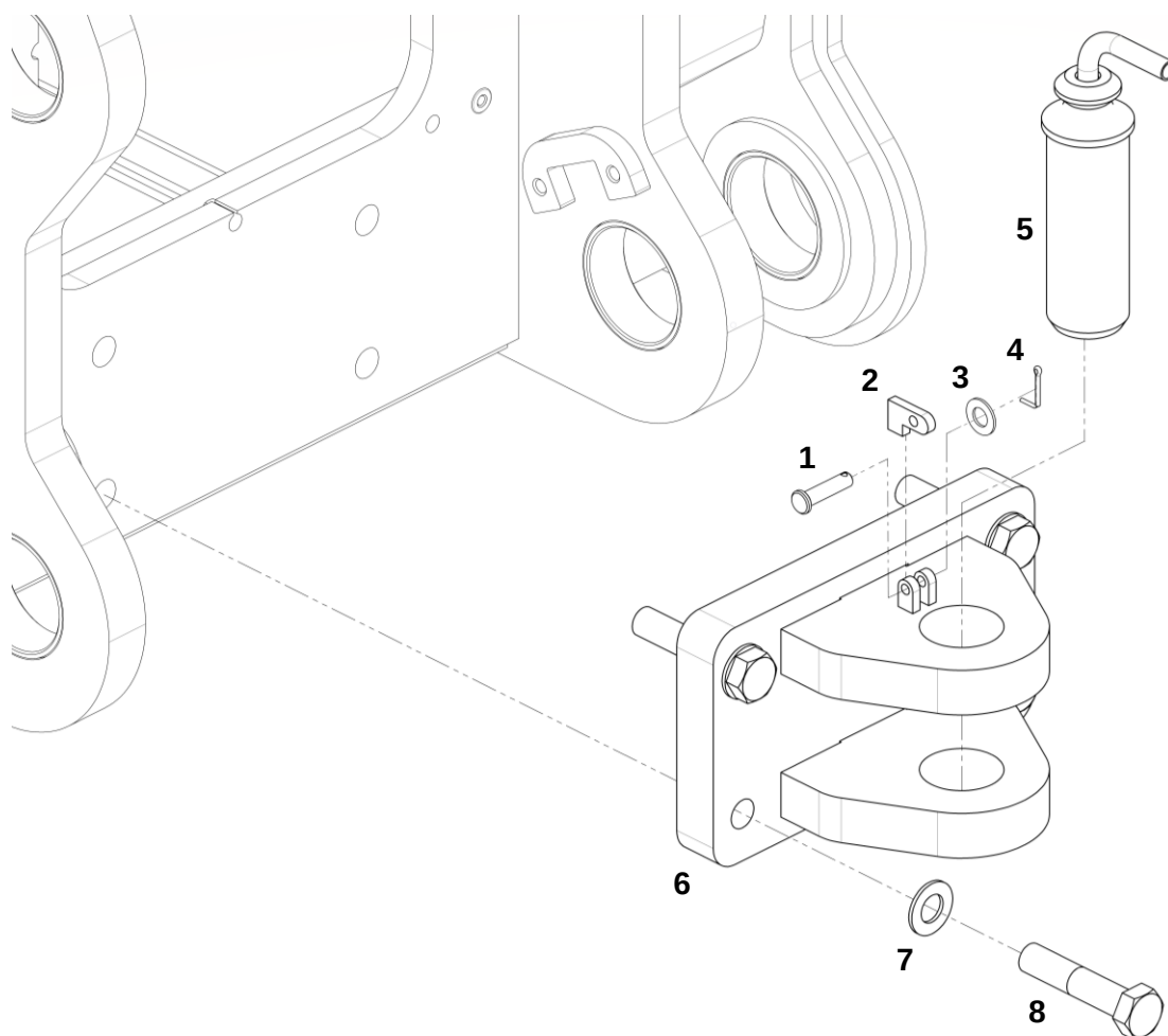
Жесткое прицепное устройство
