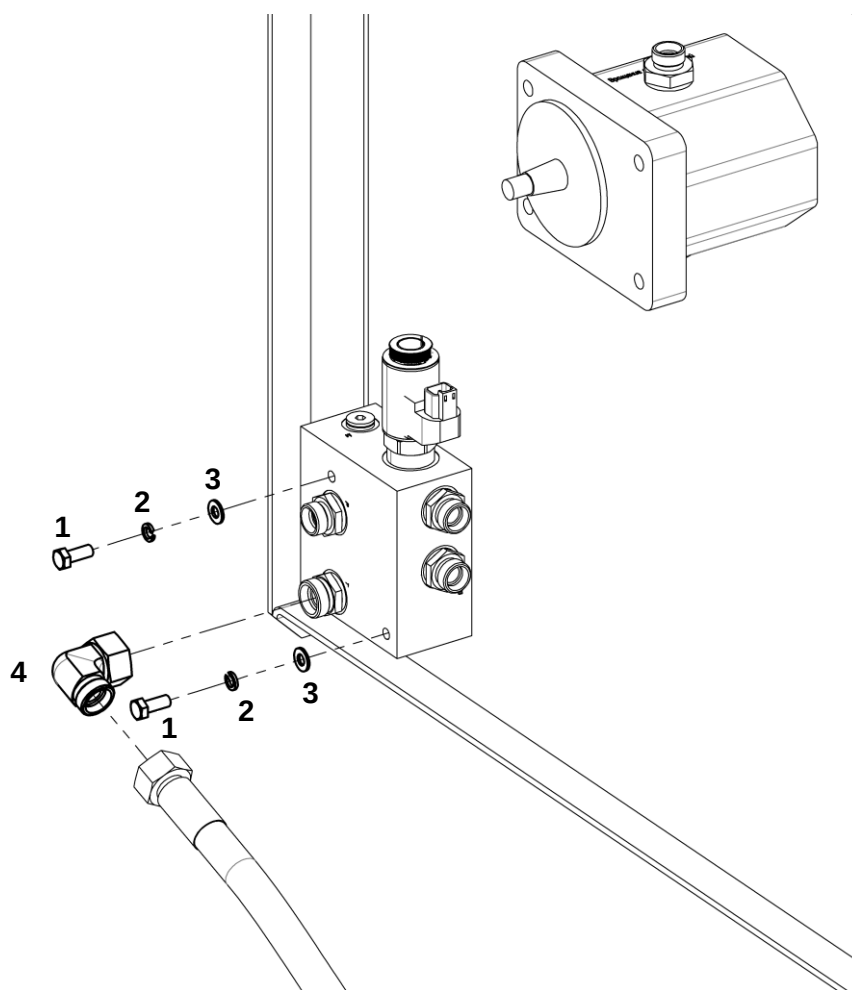
Клапанная коробка в сборе
