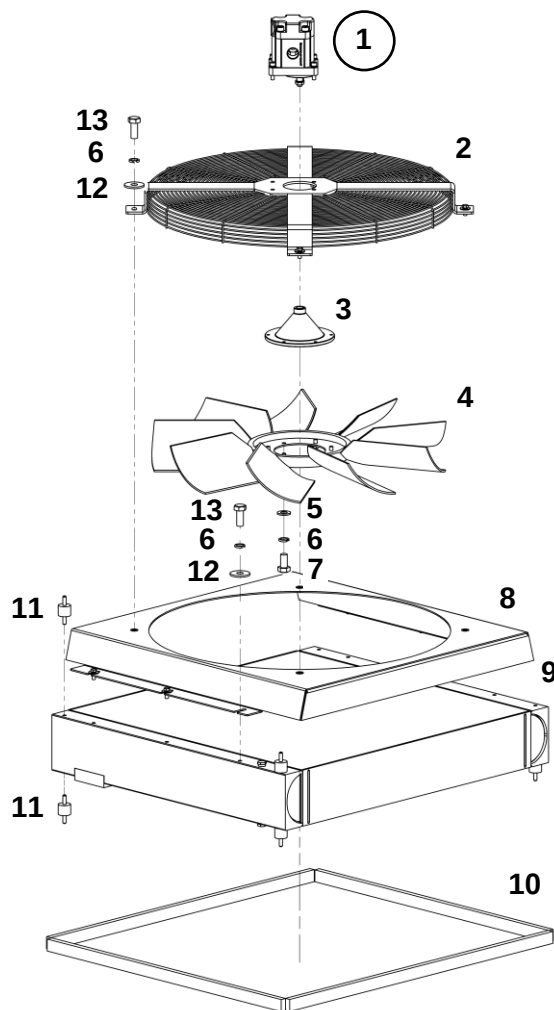
Радиатор масляный в сборе
