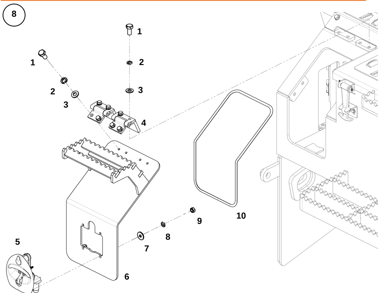
Крепление люка
