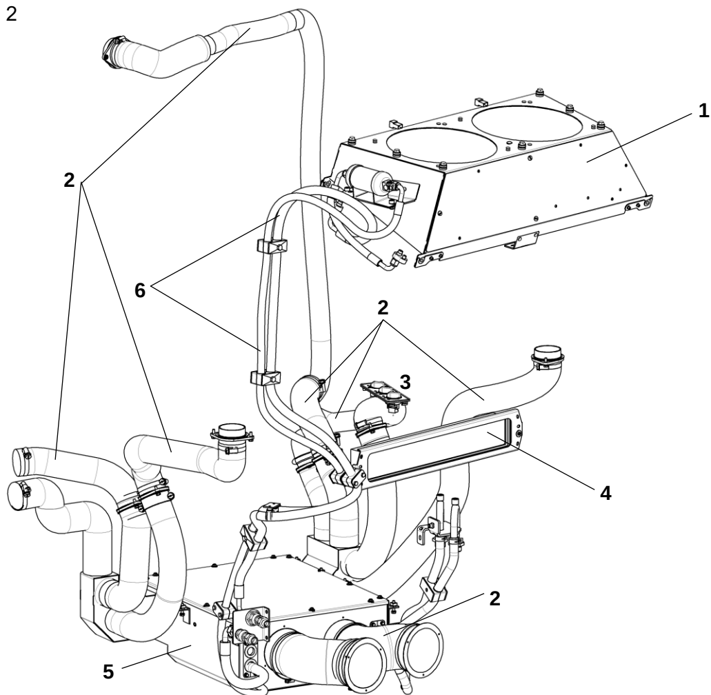
Система климатическая
