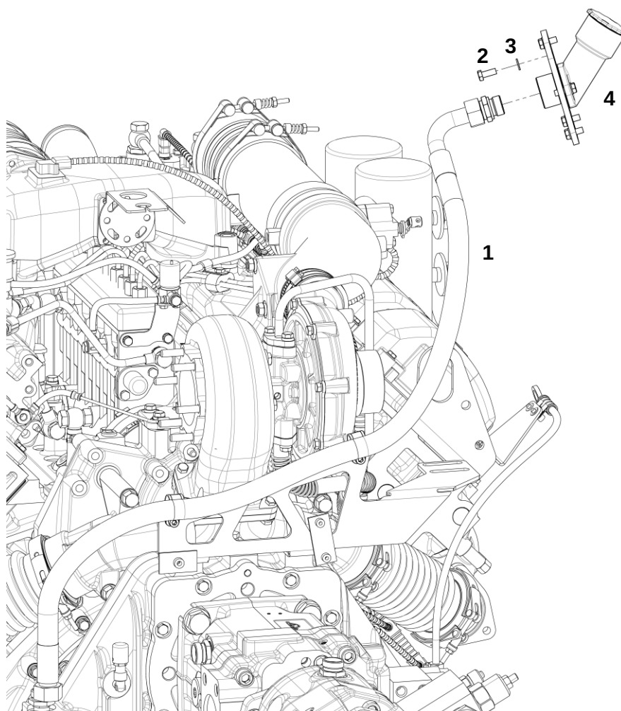
Горловина маслозаливная в сборе
