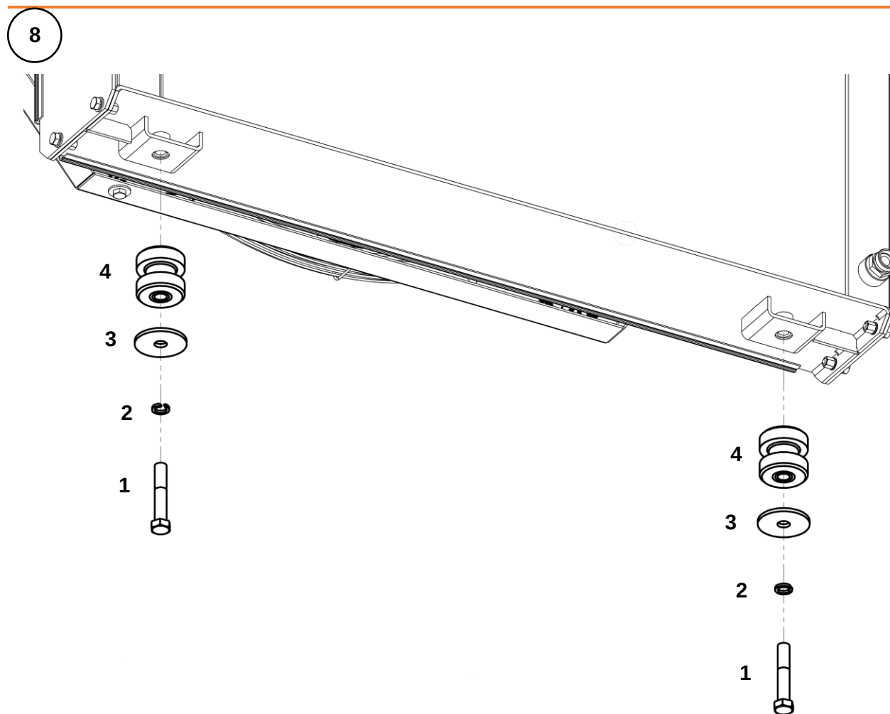
Крепление виброизолятора к блоку радиатора
