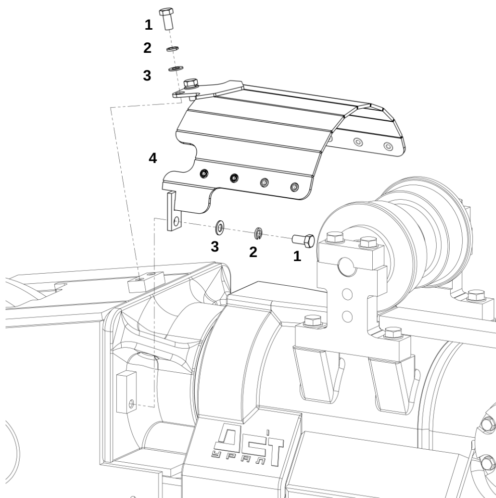
Крепление кожуха к узлу направляющего колеса в сборе
