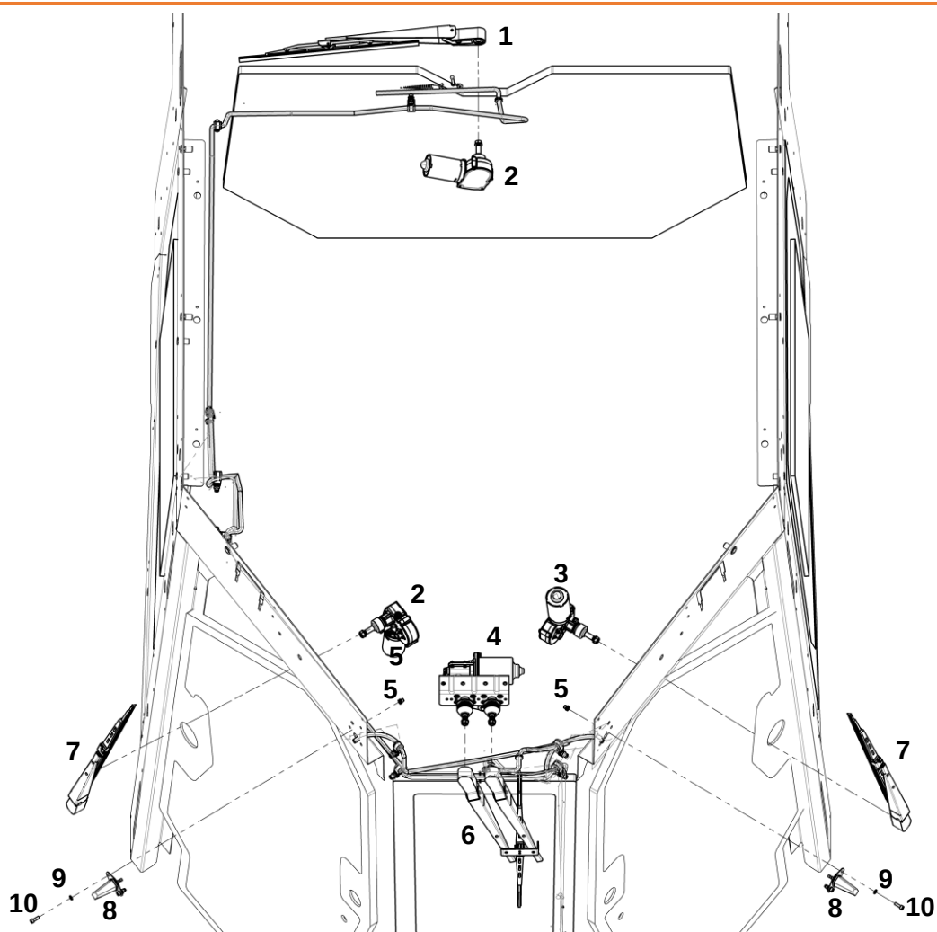
Стеклоочистители кабины
