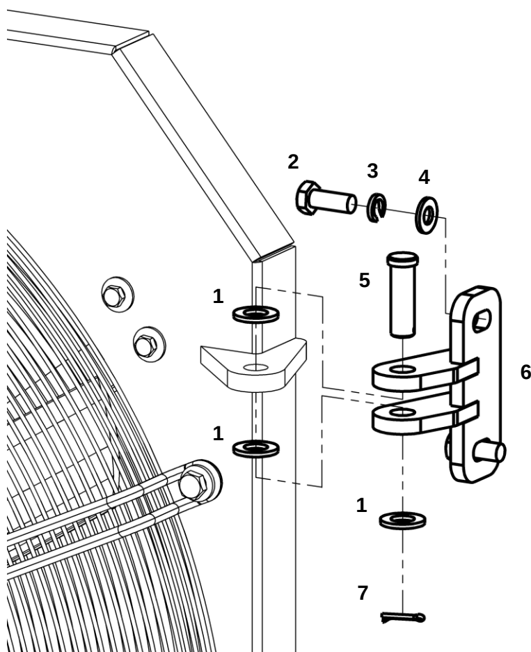
Установка петель
