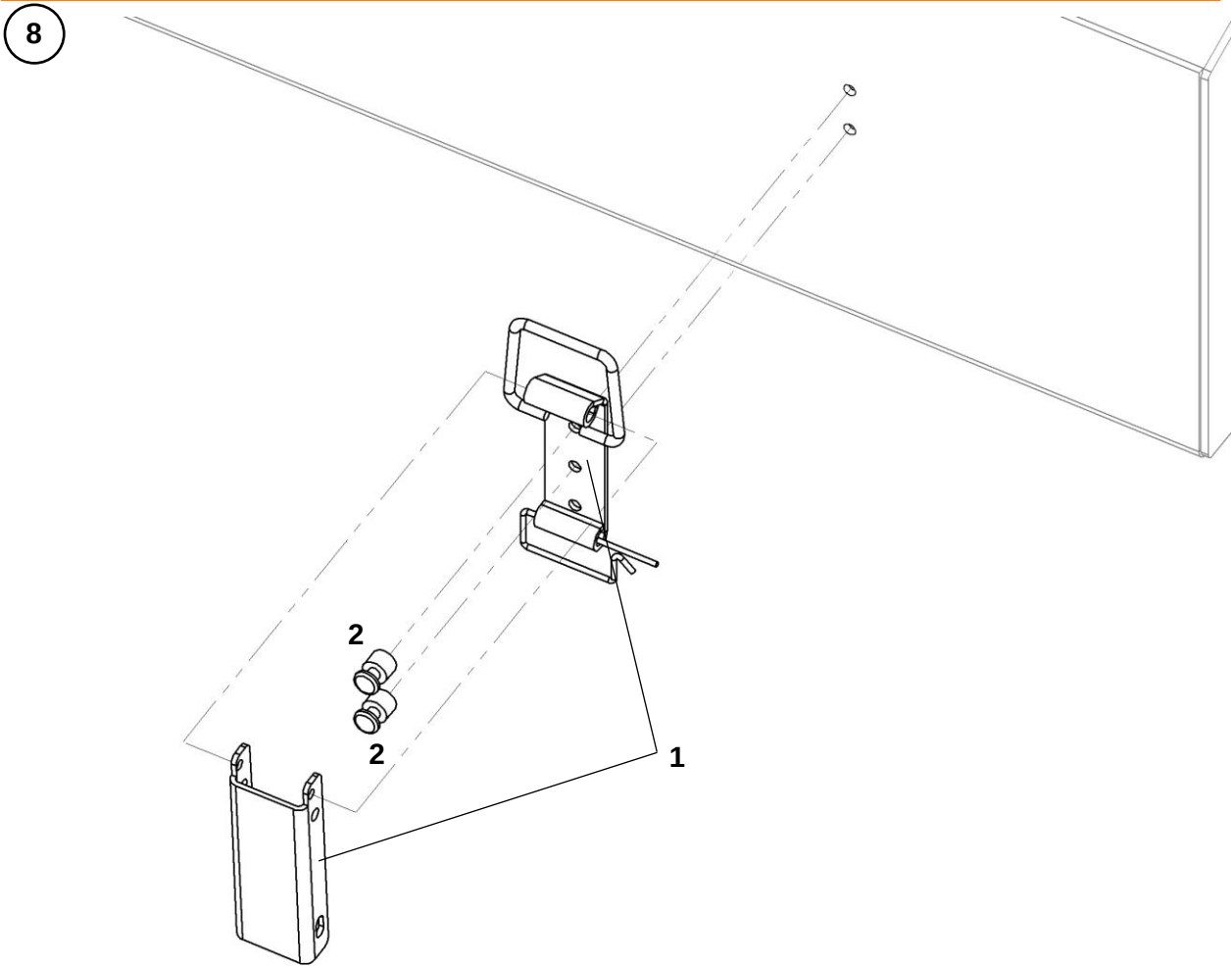
Крепление замка в сборе
