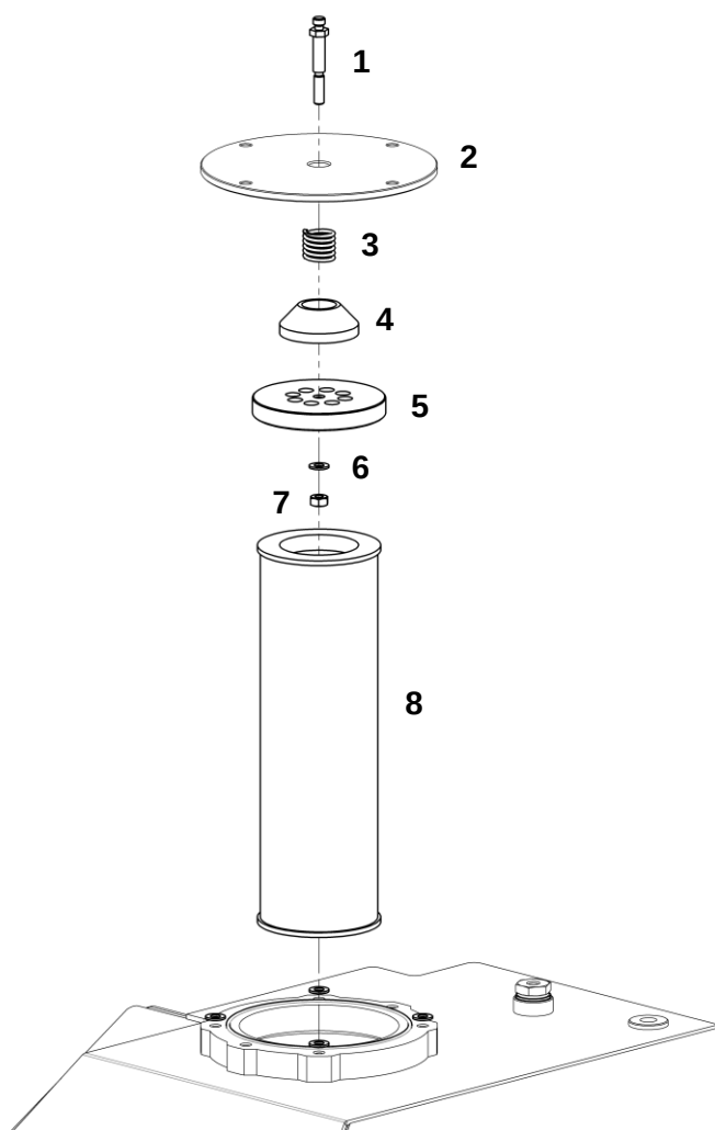
Крышка фильтра в сборе
