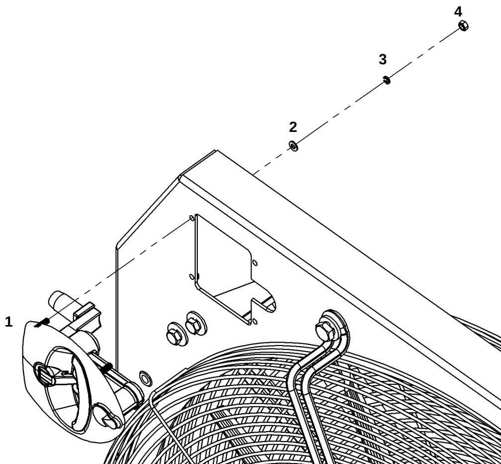
Крепление замка поворотного
