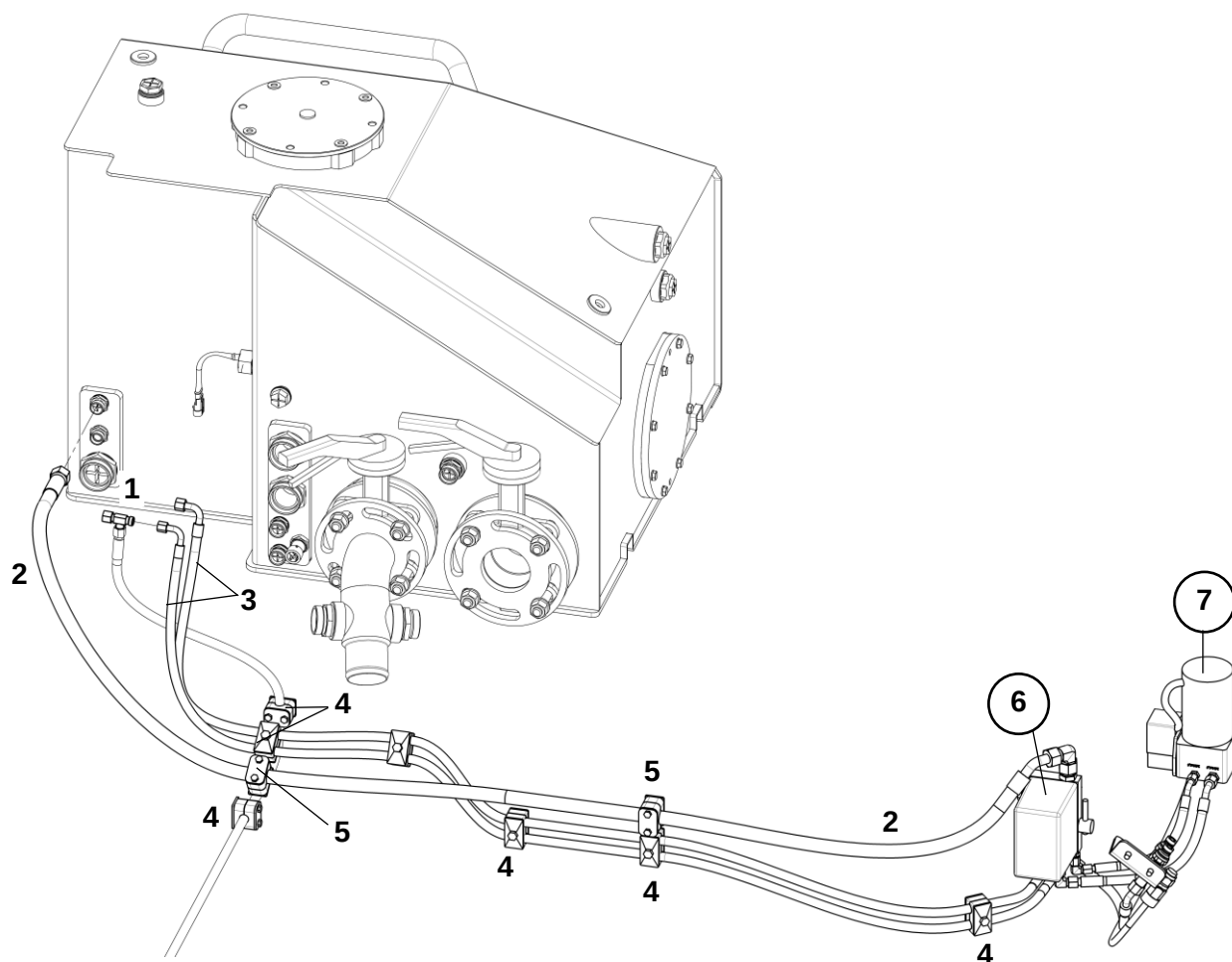
Трубопроводы гидросистемы подъема кабины
