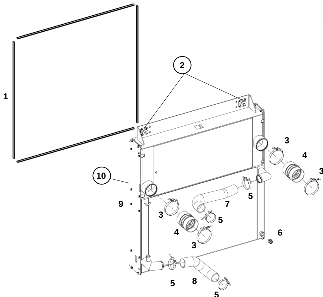
Блок радиатора в сборе
