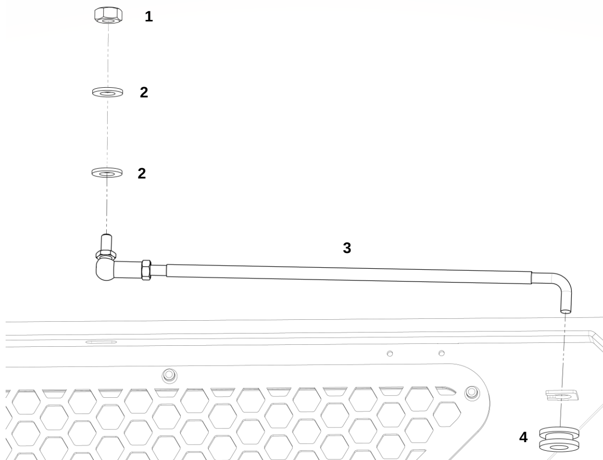
Створка в сборе
