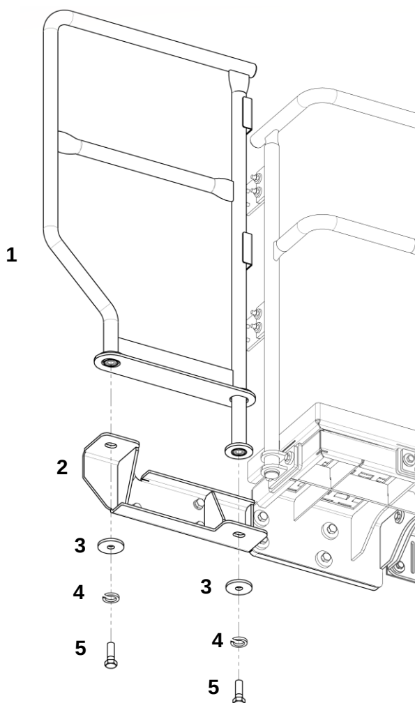
Боковые опоры в сборе
