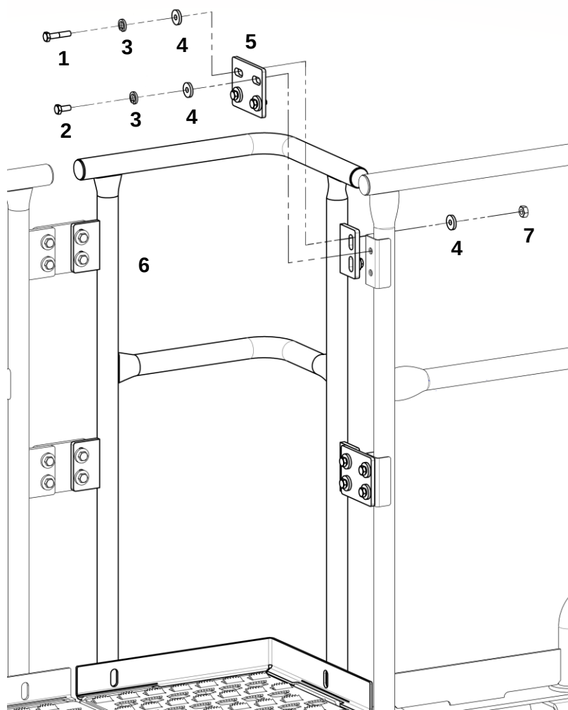
Боковые опоры в сборе
