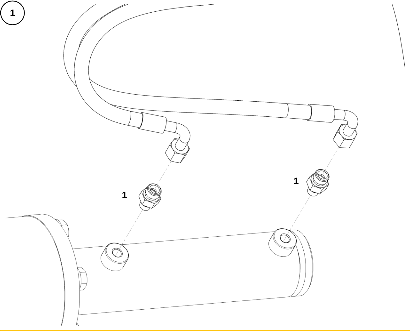
Крепление РВД к механизму смены высоты ножа
