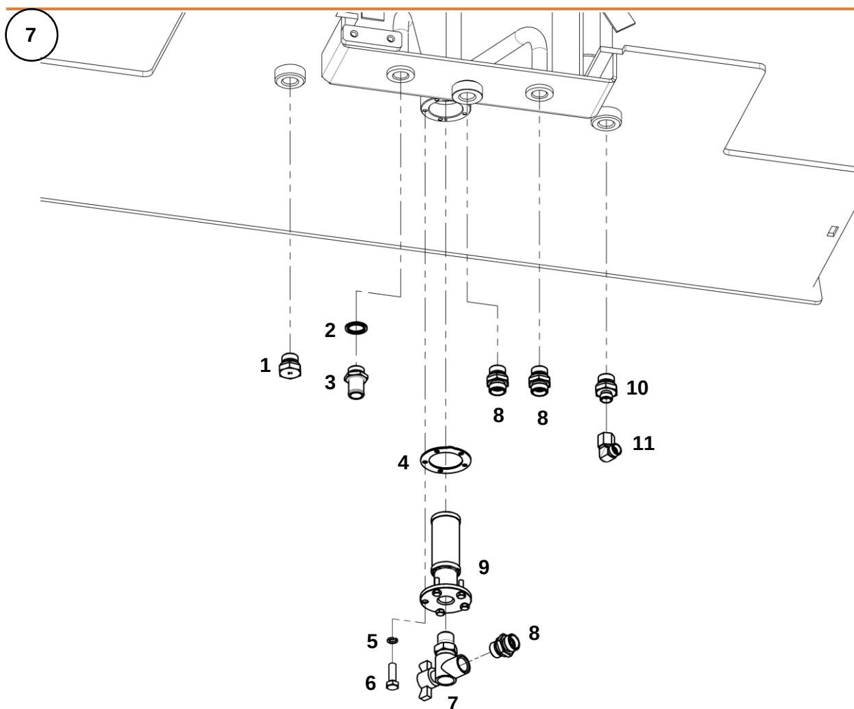
Установка кранов
