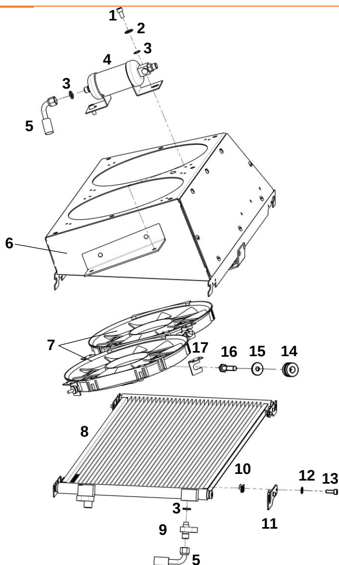
Блок конденсора
