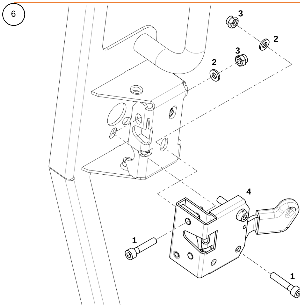
Замок двери
