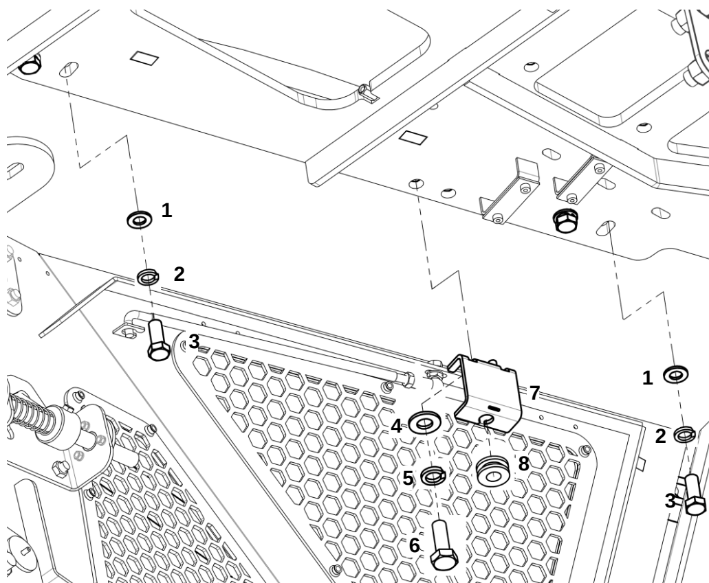
Крепление плиты боковое
