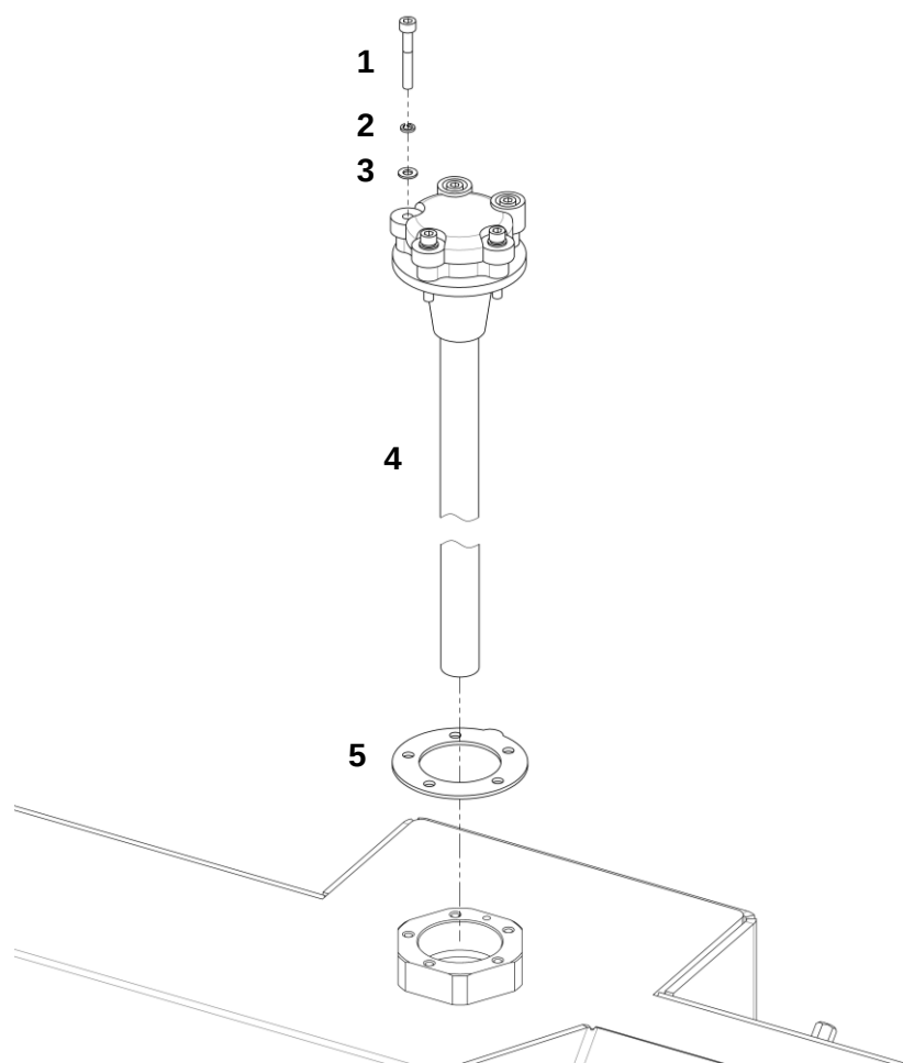
Датчик уровня топлива
