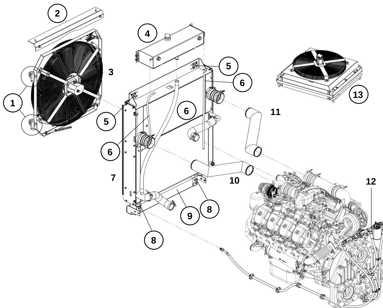
Система охлаждения
