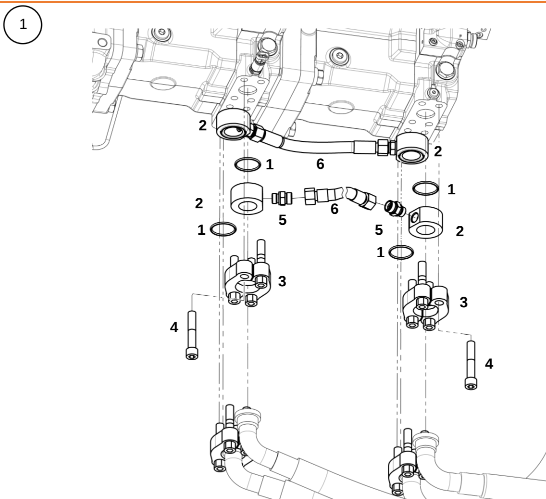
Крепление РВД к раздаточному редуктору
