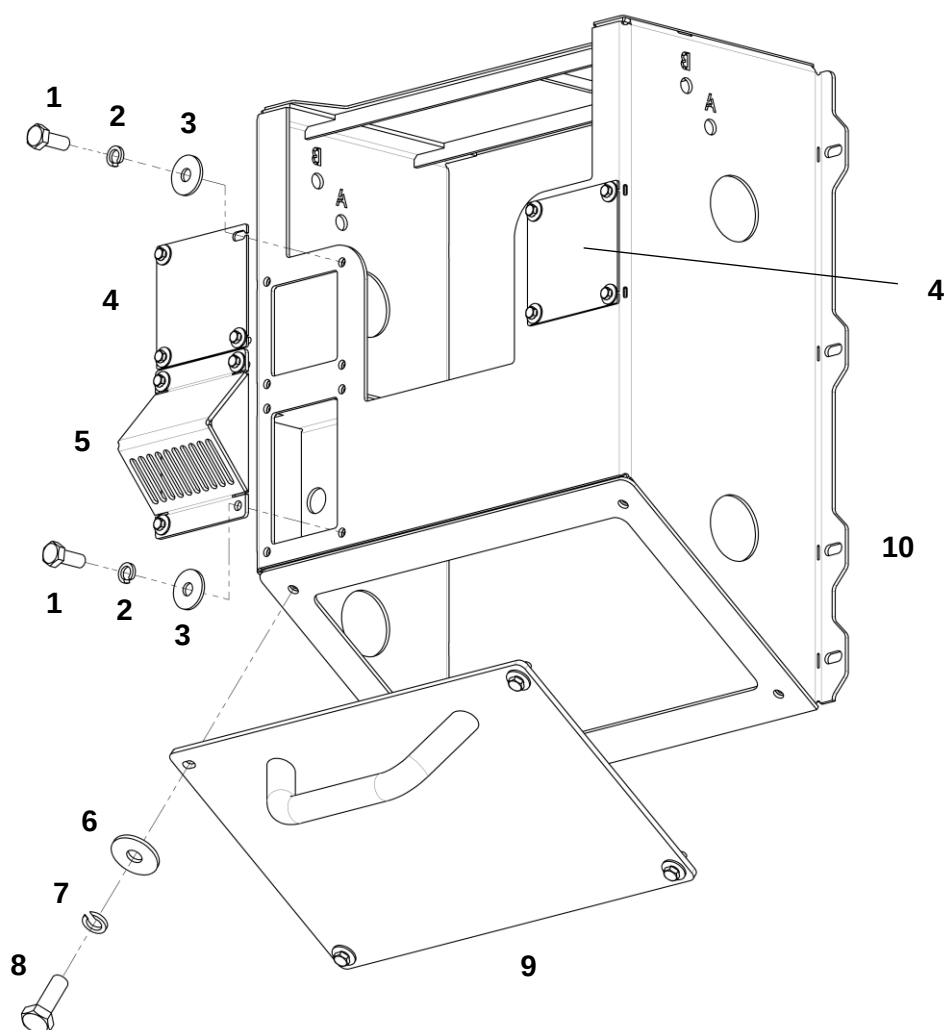
Кожух в сборе
