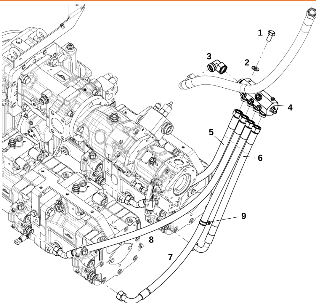
Плита подпитки
