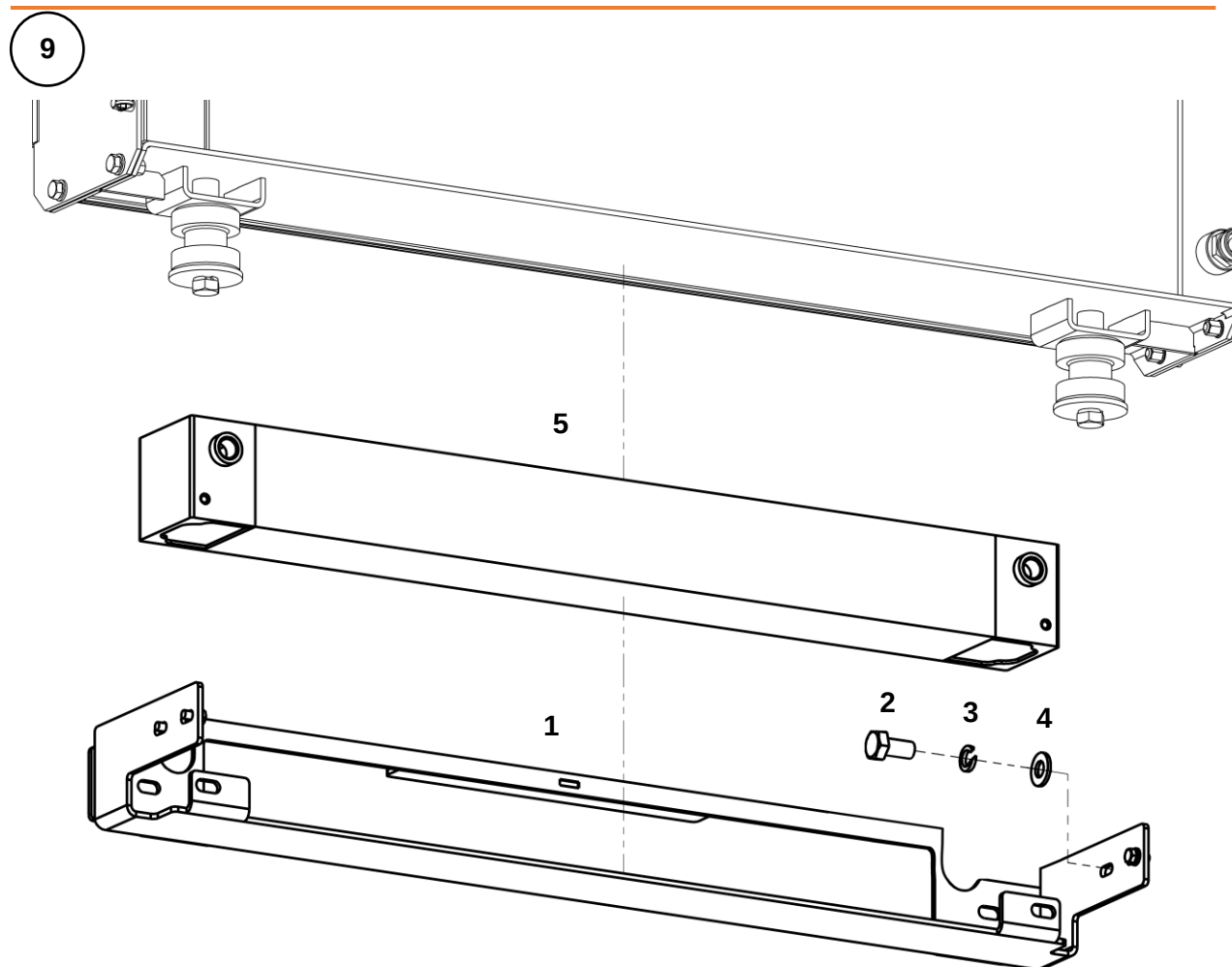
Крепление кронштейна радиатора в сборе
