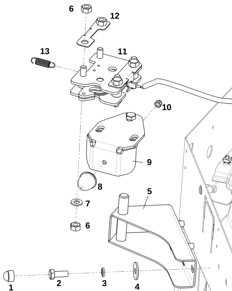
Фиксатор двери кабины
