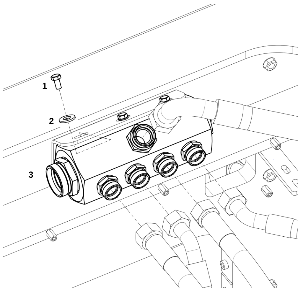
Соединение с коллектором
