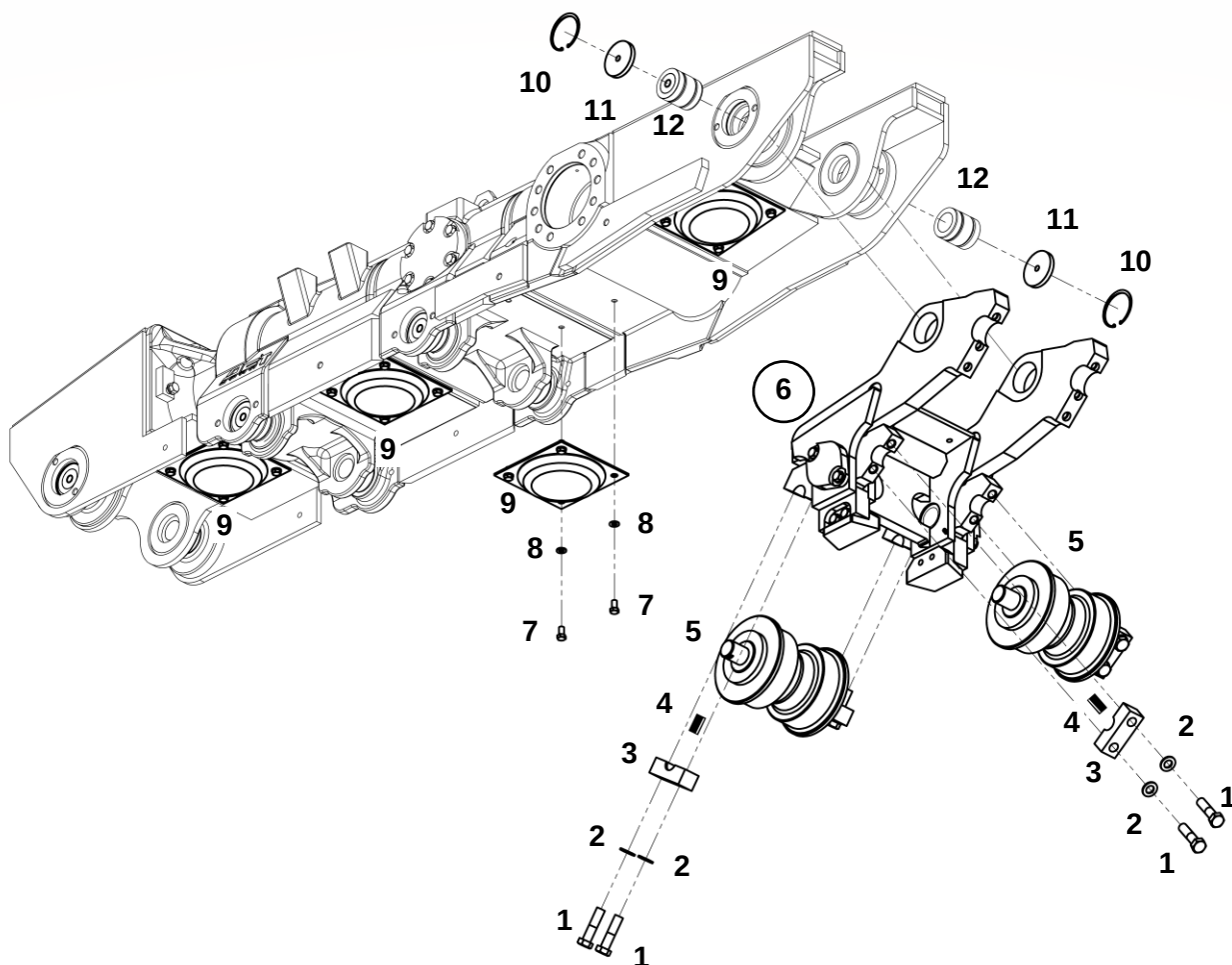
Каретка задняя в сборе
