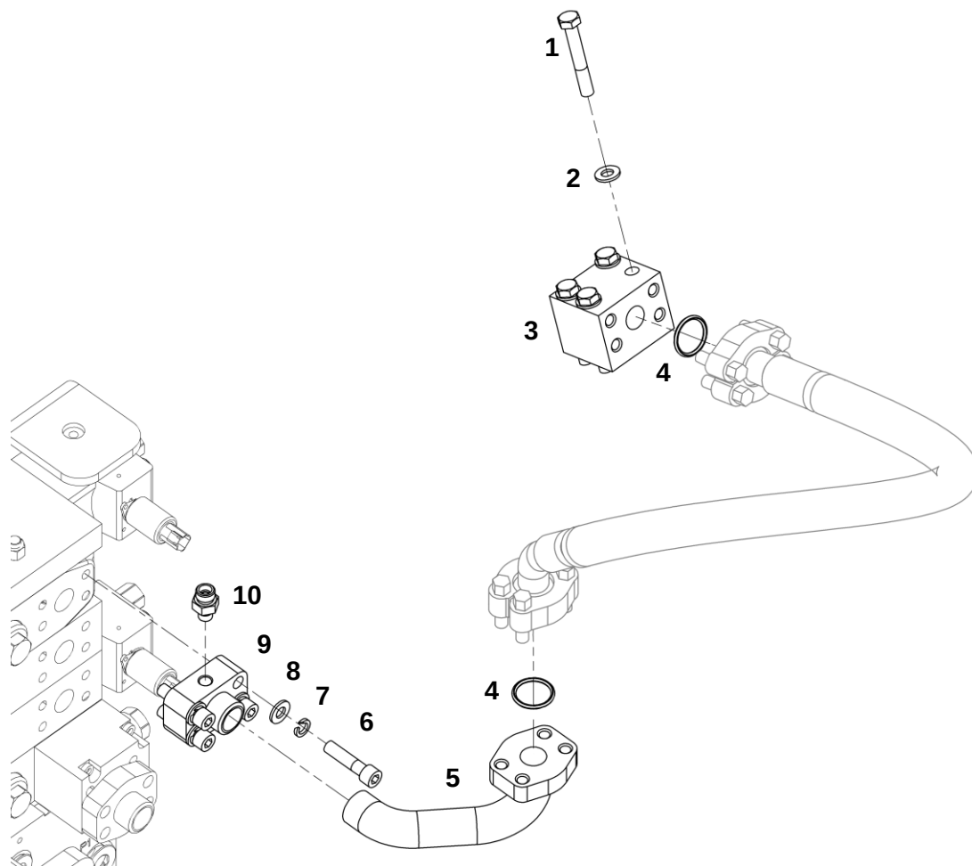
Крепление РВД к гидрораспределителю
