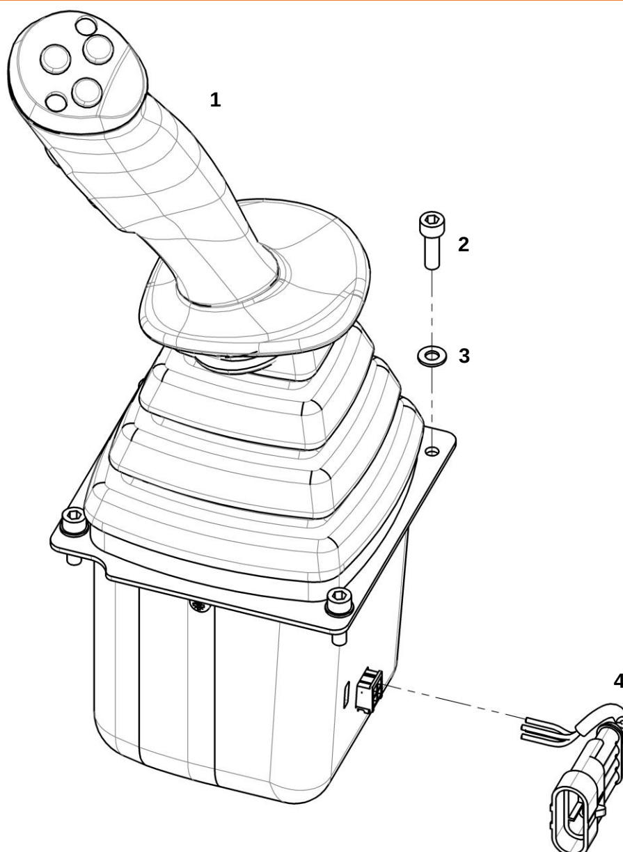
Джойстик правый
