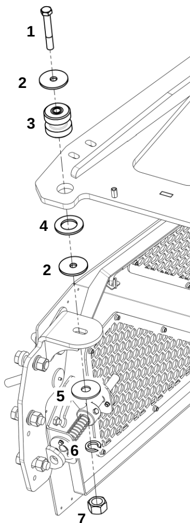
Крепление плиты спереди
