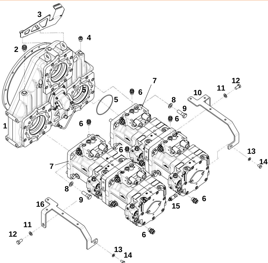
Редуктор раздаточный в сборе
