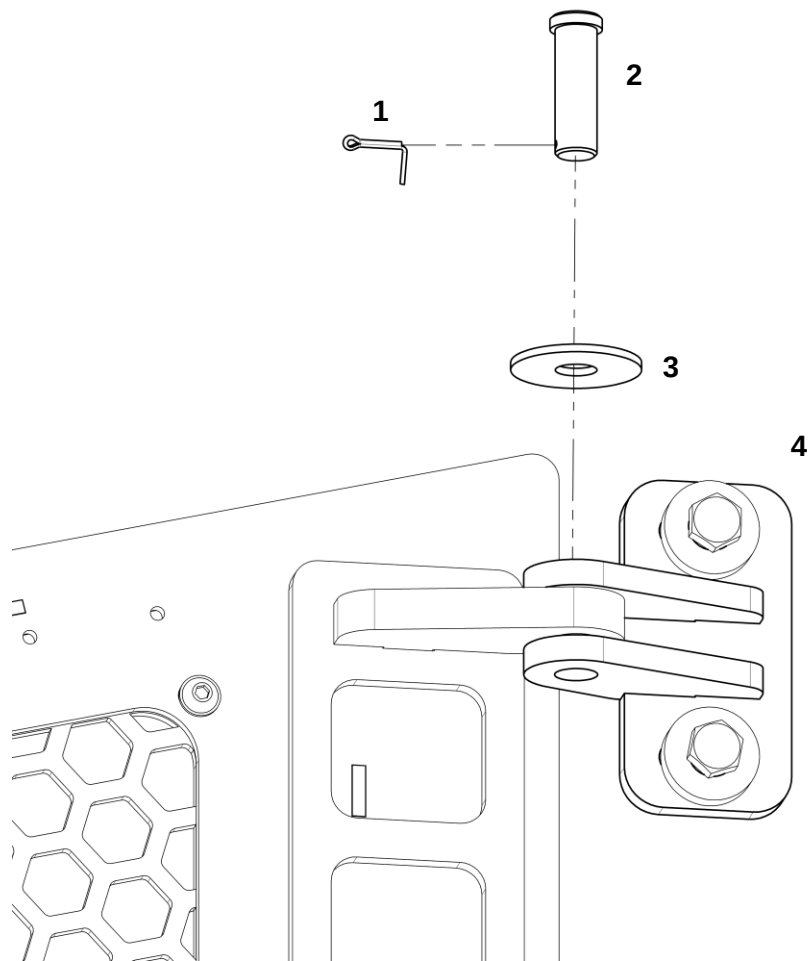
Крепление петли
