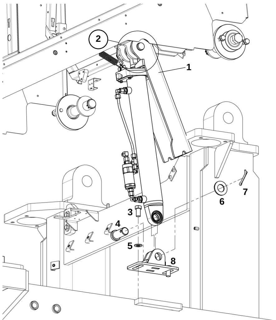
Установка механизма подъема кабины
