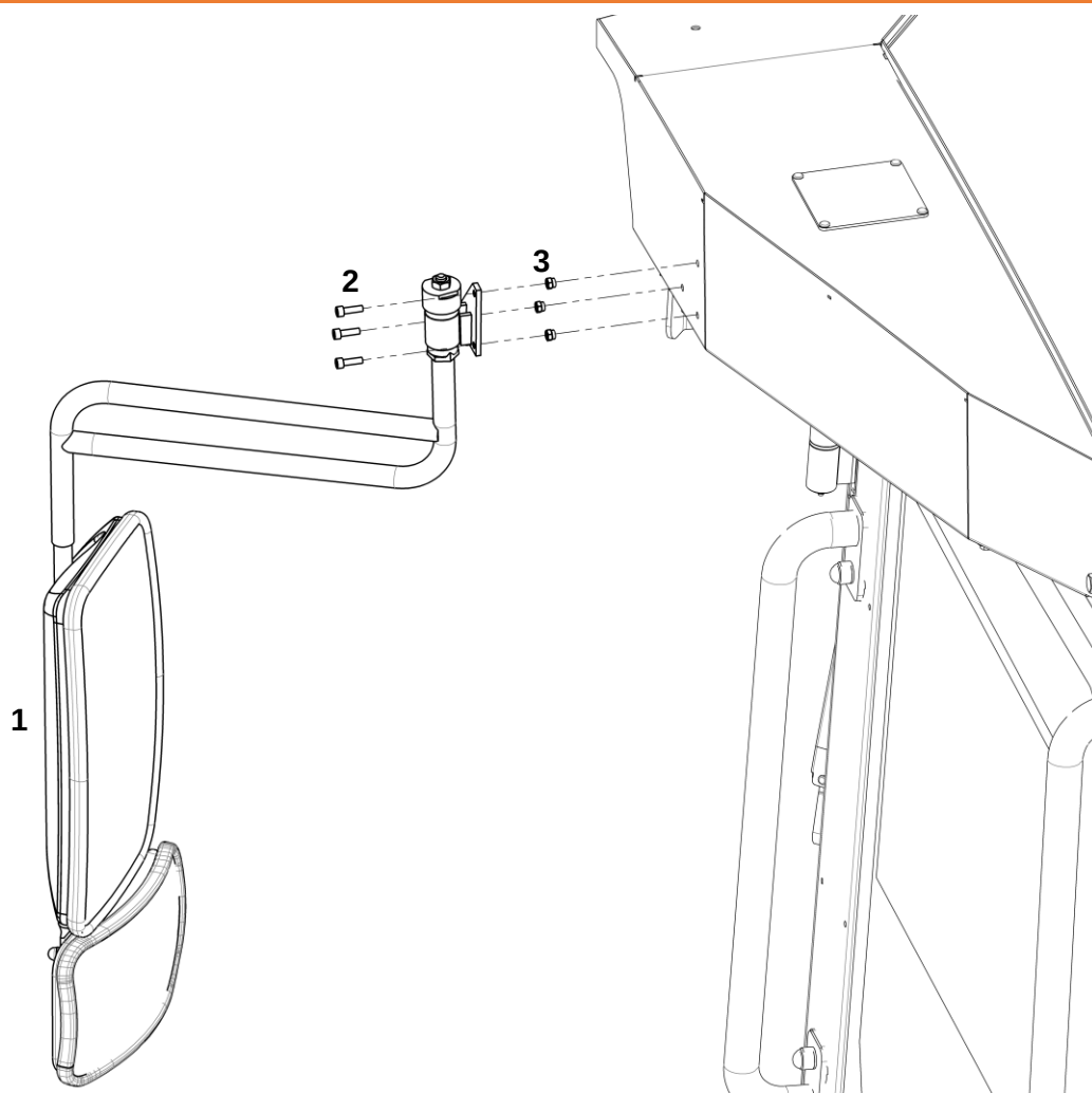
Зеркала кабины
