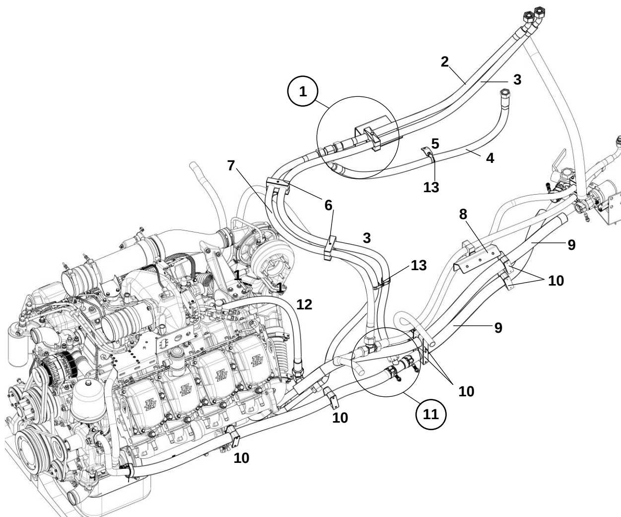
Система предпускового подогрева двигателя
