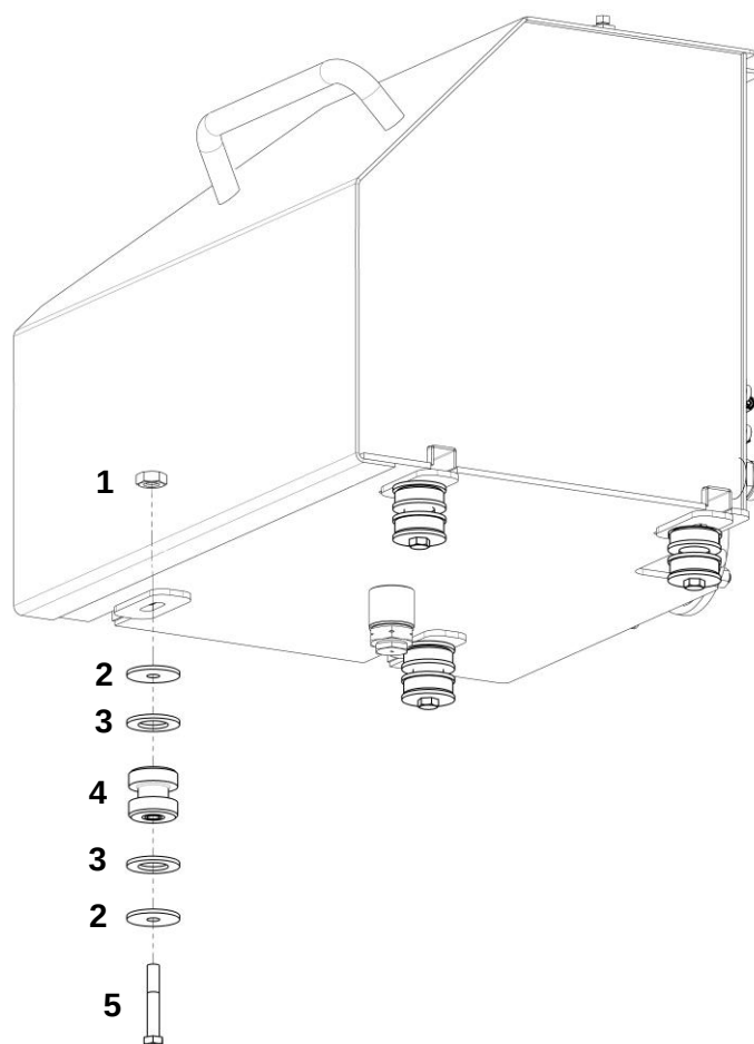
Крепеж бака гидравлического
