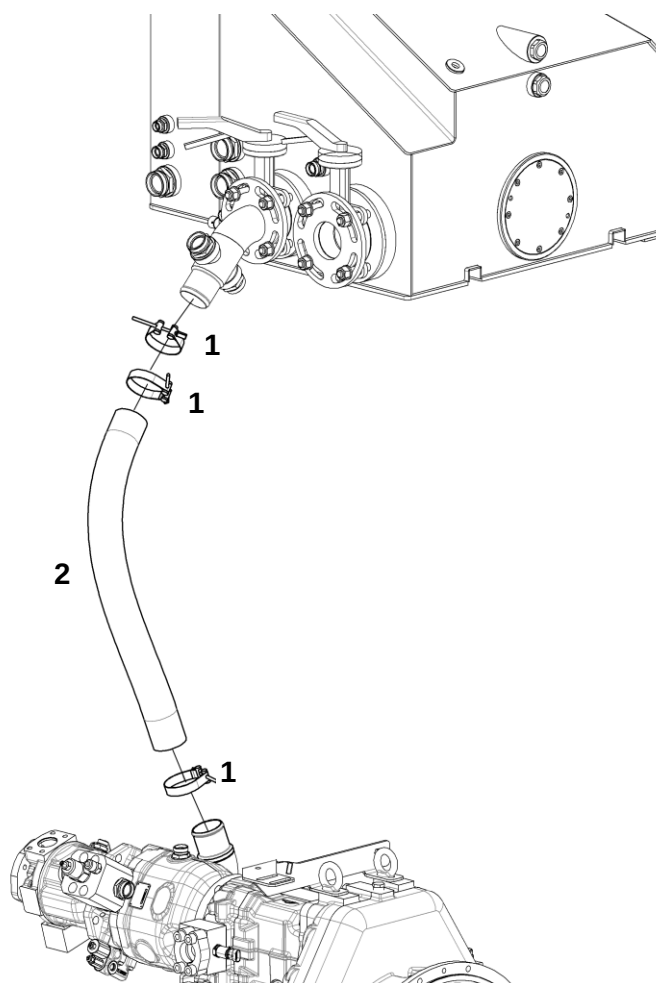
Трубопроводы гидросистемы трансмиссии
