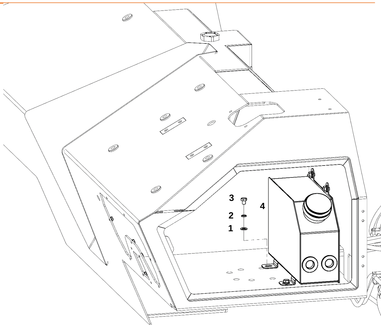
Крепление бака
