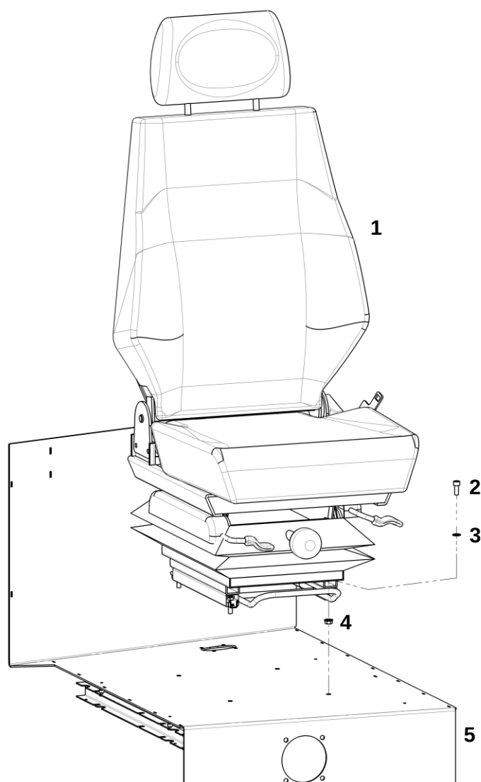
Установка сиденья оператора
