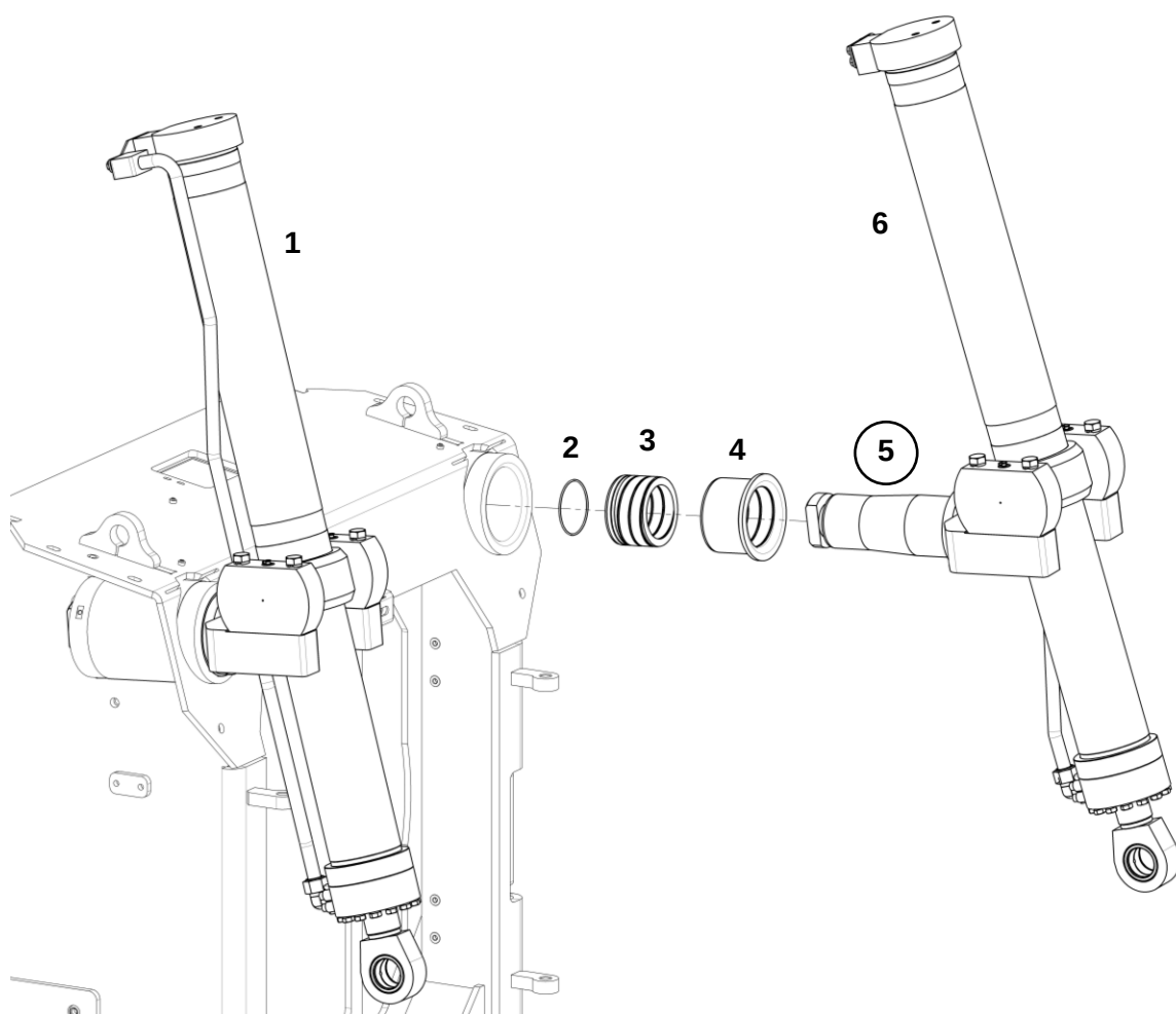
Гидроцилиндры переднего навесного оборудования
