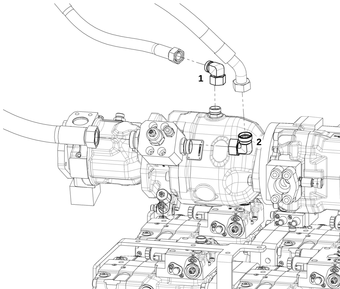
Предохранительный клапан
