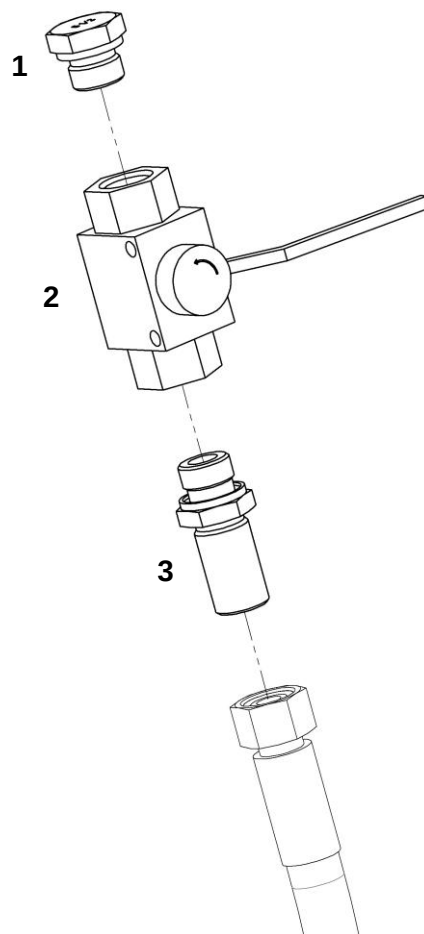
Кран шаровый
