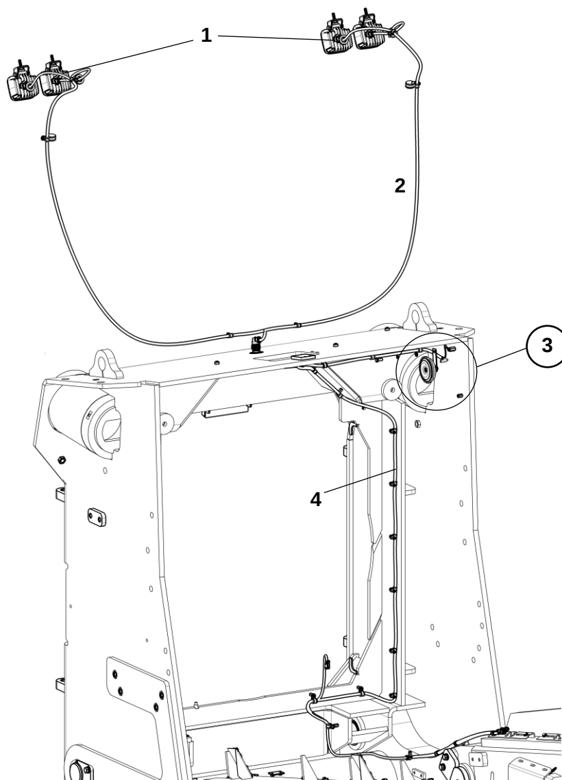
Жгут передних фар и сигнала
