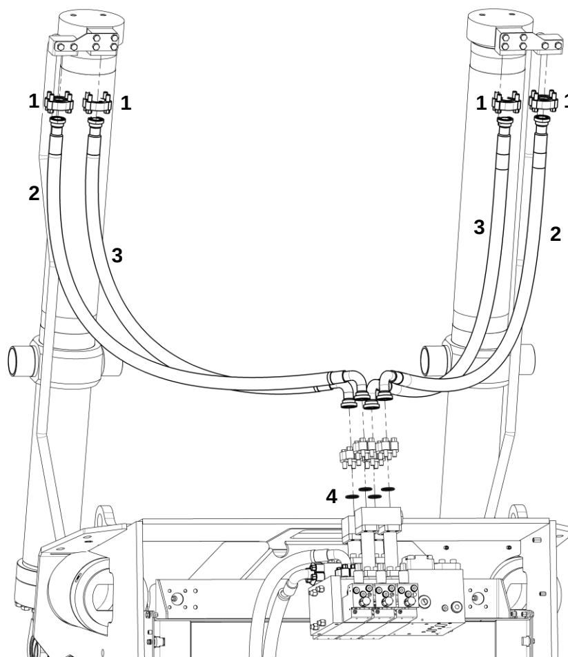
Внутренняя гидросистема переднего оборудования
