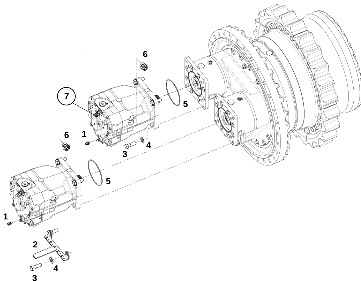
Мотор-редуктор
