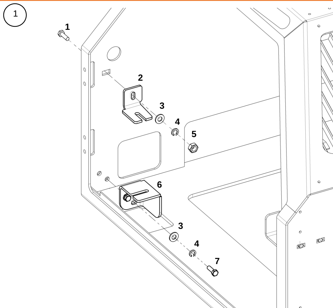
Корпус ящика в сборе
