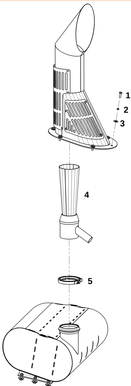
Труба выхлопная
