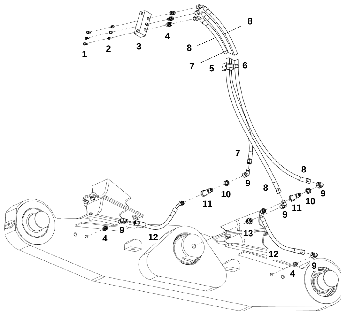
Система смазки балансирной балки
