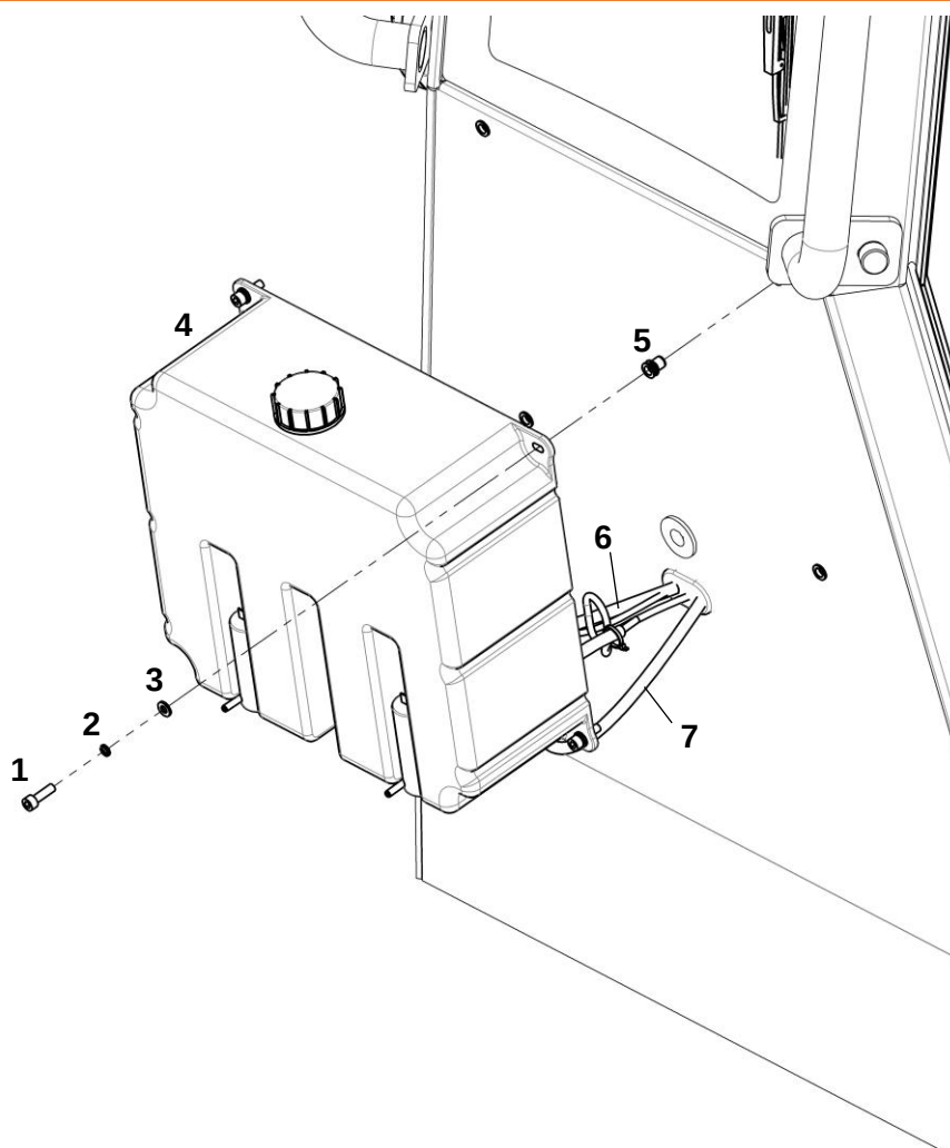
Бачок омывателя
