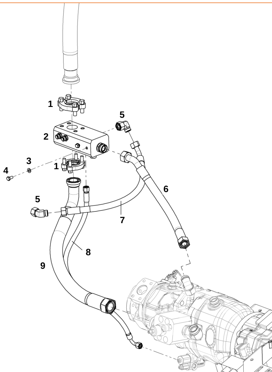
Коллектор сливной
