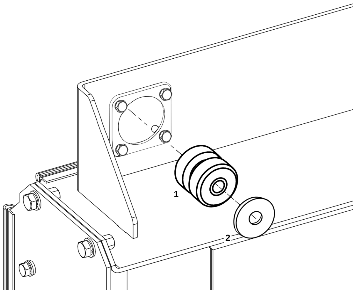
Виброизолятор в сборе
