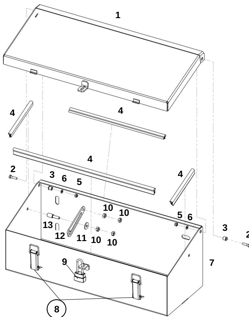
Ящик инструментальный
