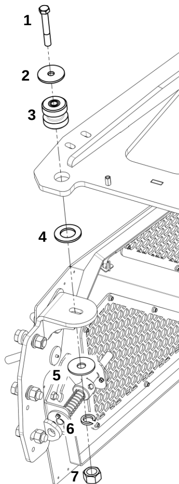
Крепление плиты сзади
