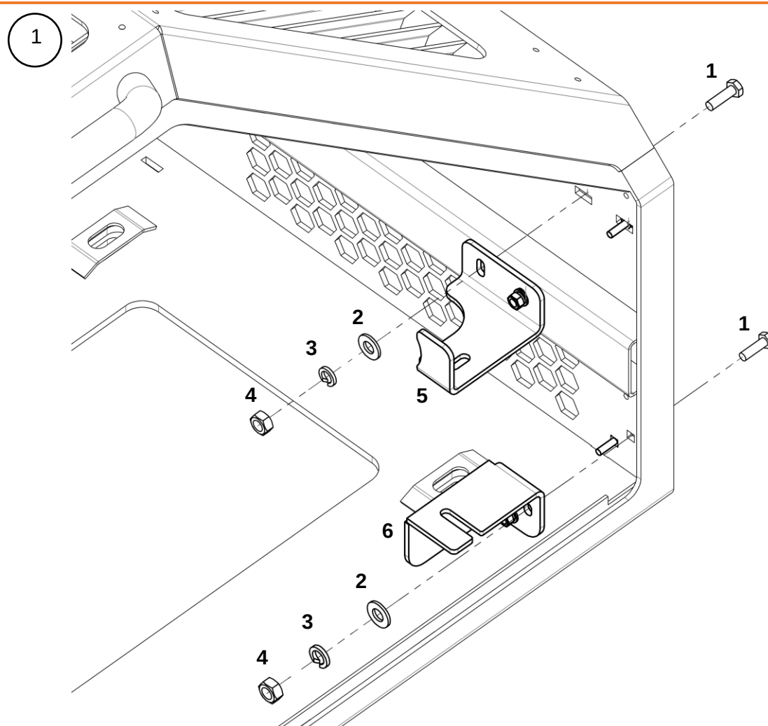
Корпус ящика в сборе
