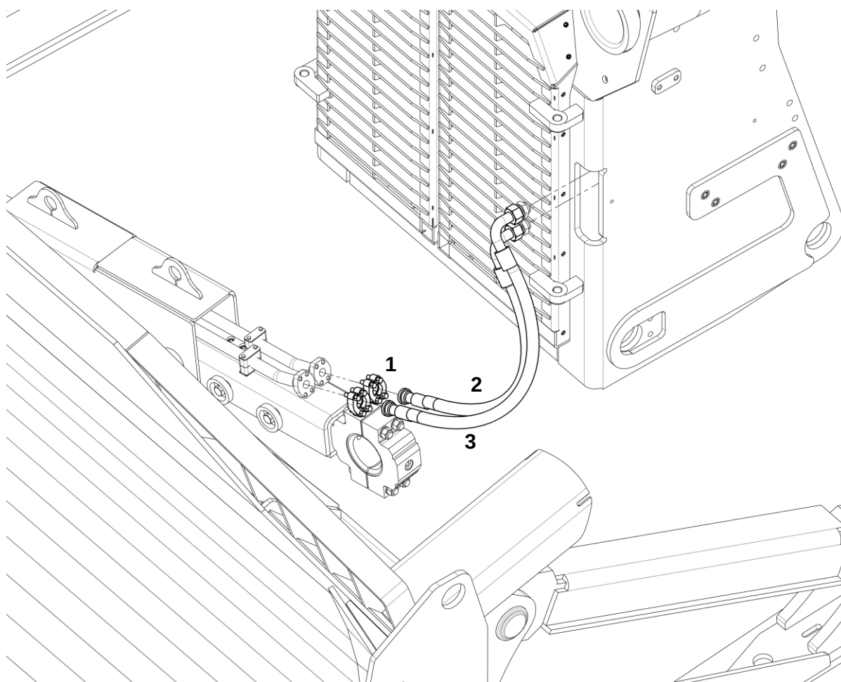
Трубопроводы переднего навесного оборудования
