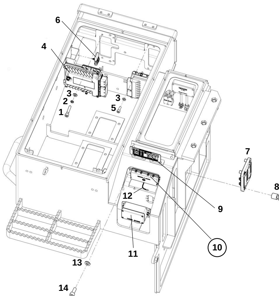
Контроллер трансмиссии
