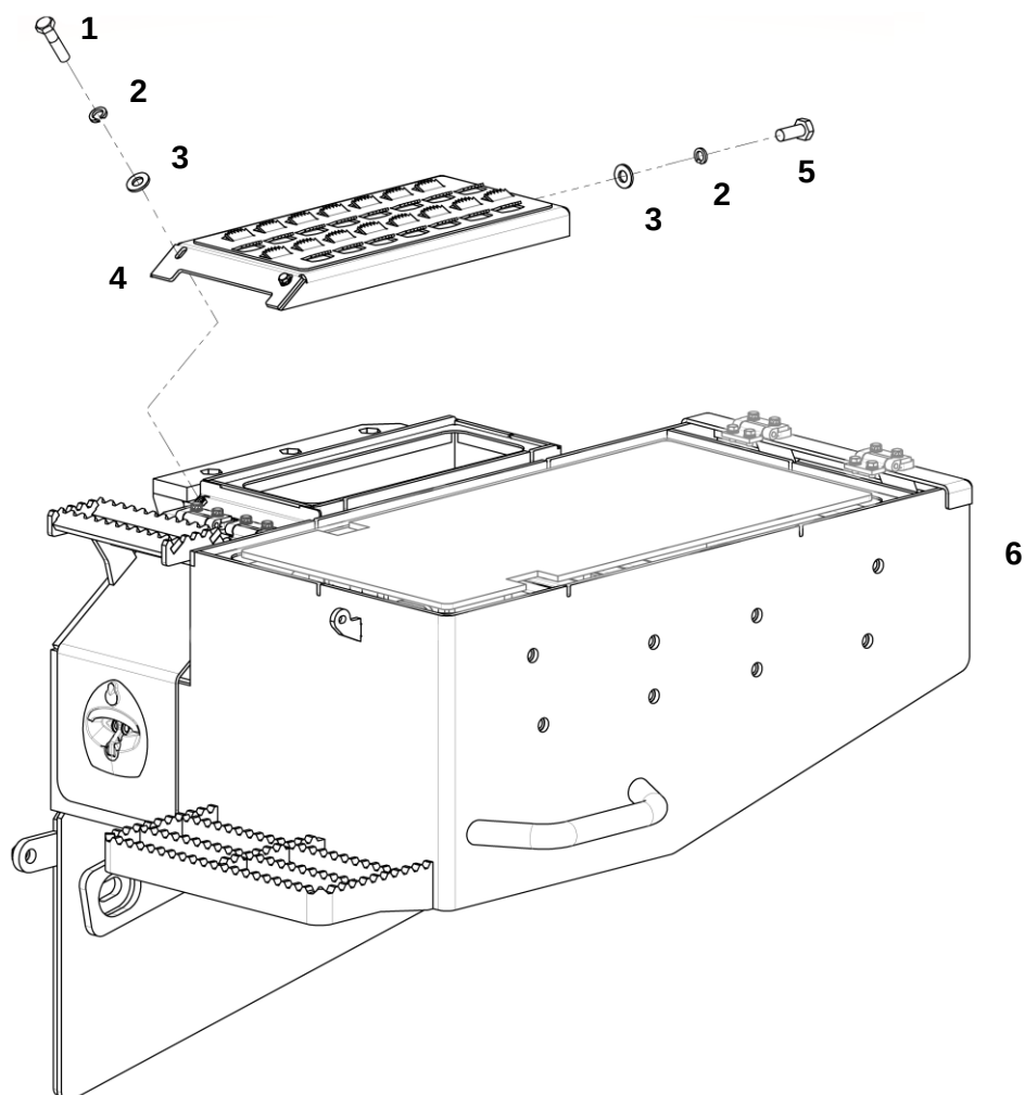
Подножка
