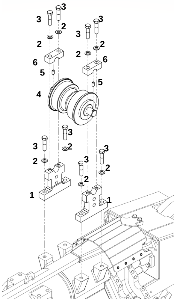
Крепление катка поддерживающего к тележке
