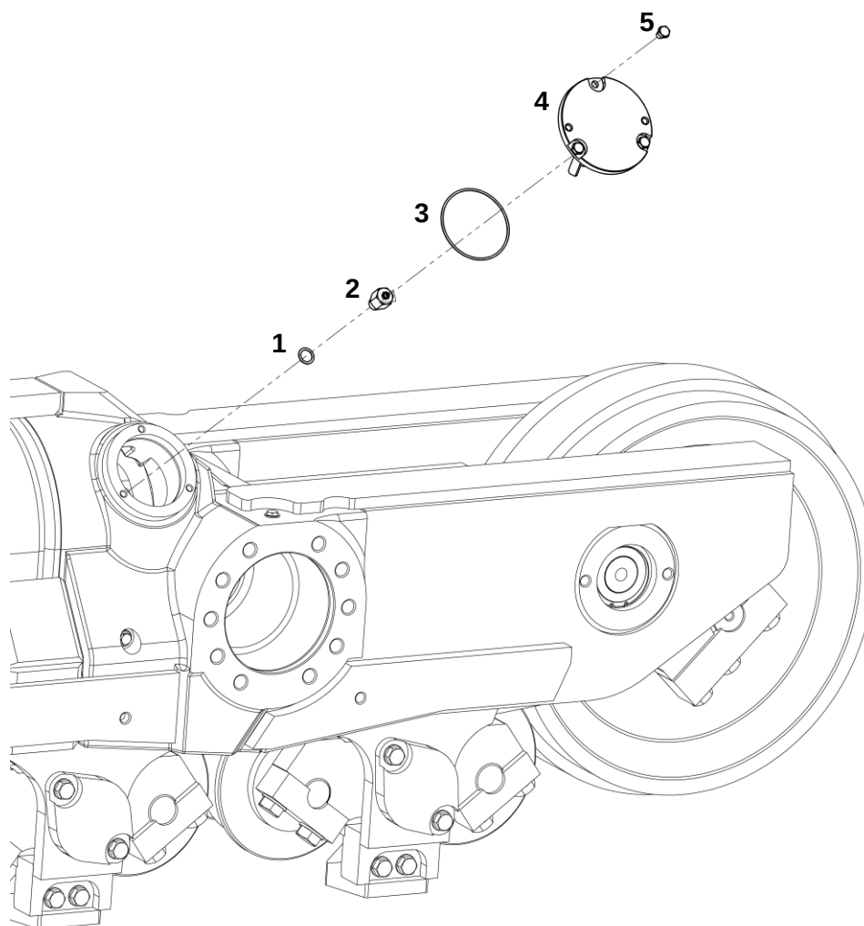
Установка клапана
