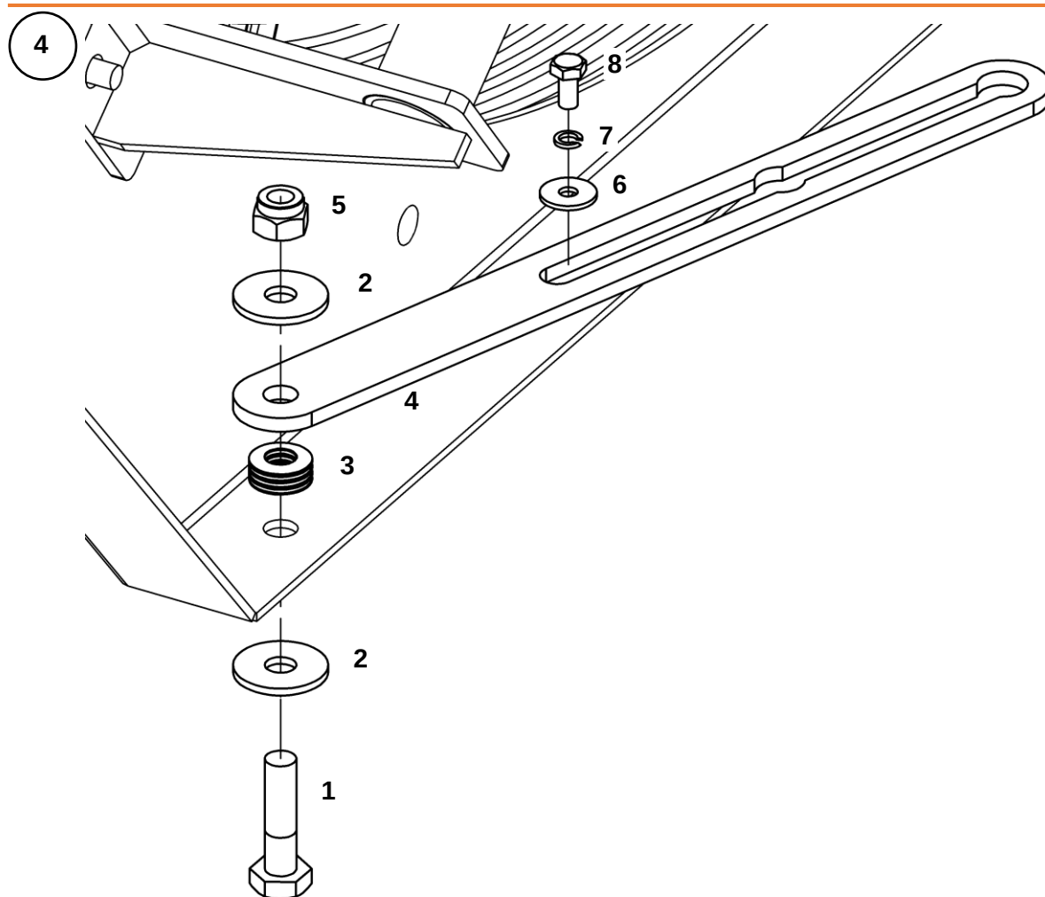
Установка стопора к раме вентилятора
