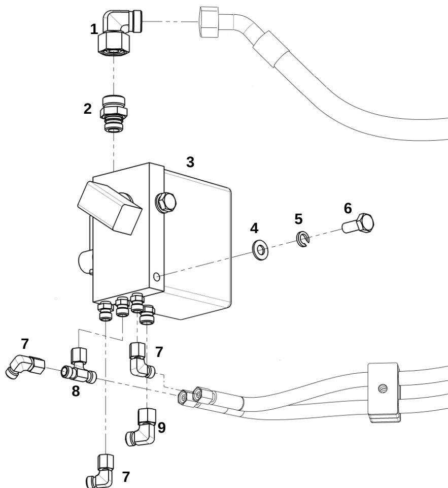
Насос ручной в сборе
