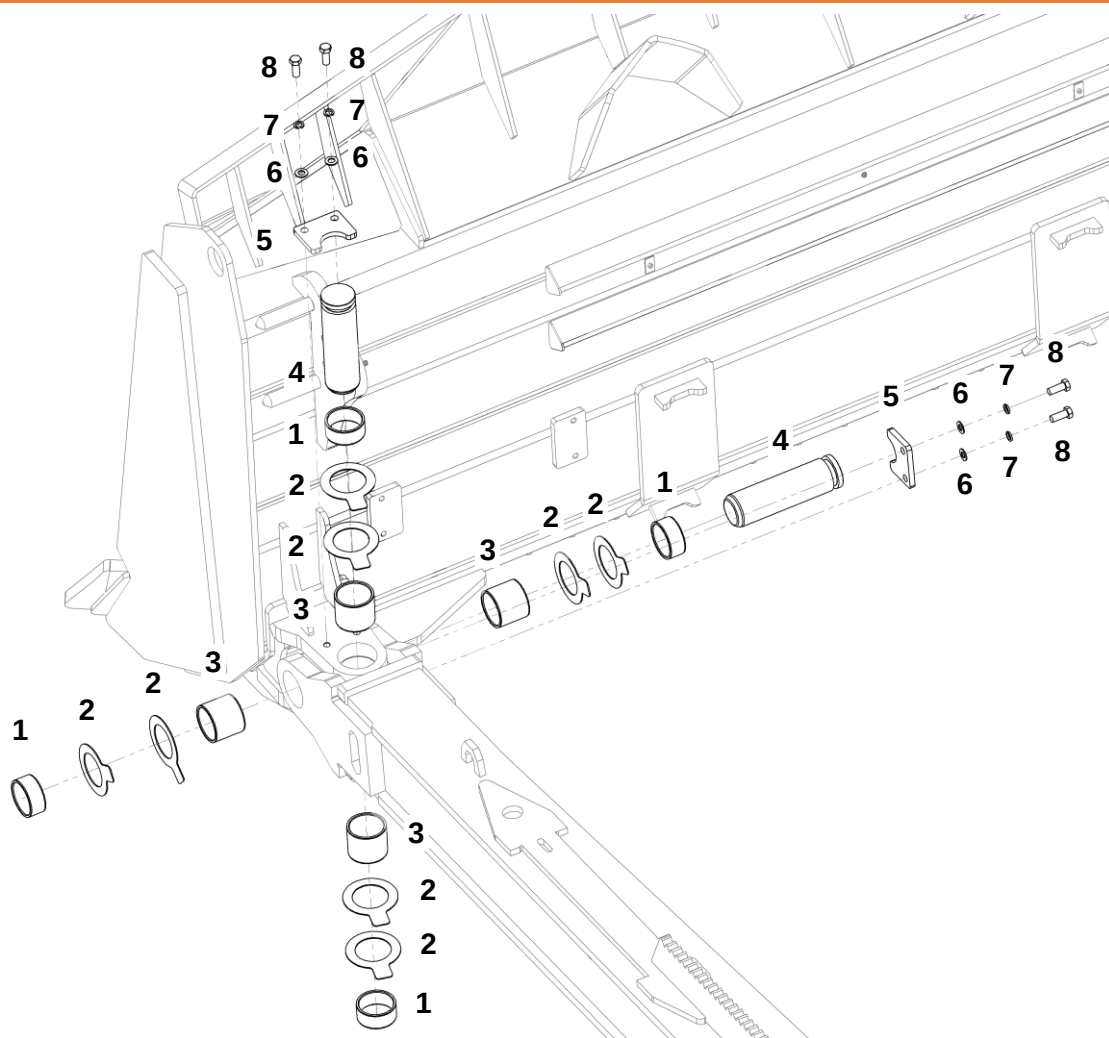
Крепление бруса
