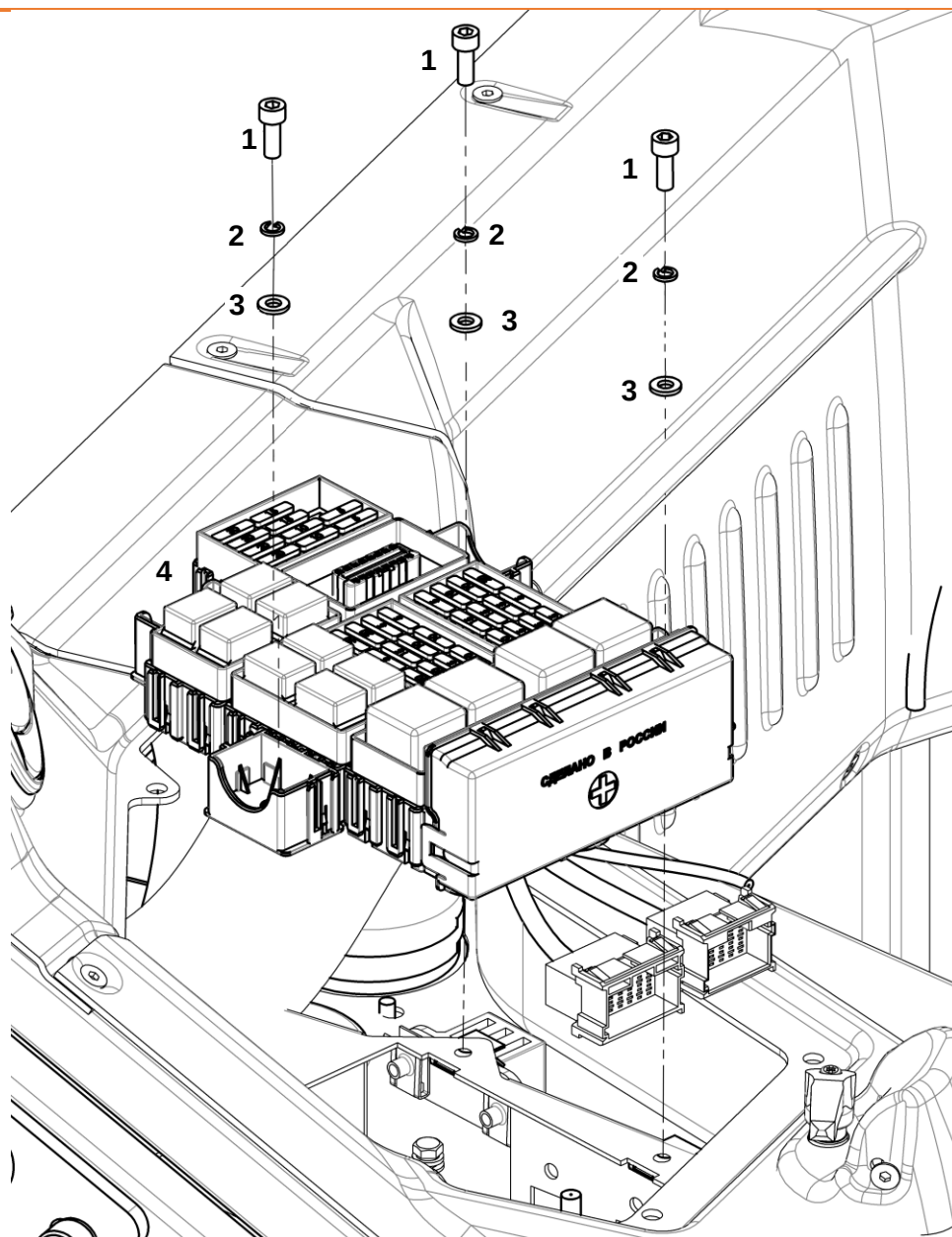
Блок предохранителей и реле
