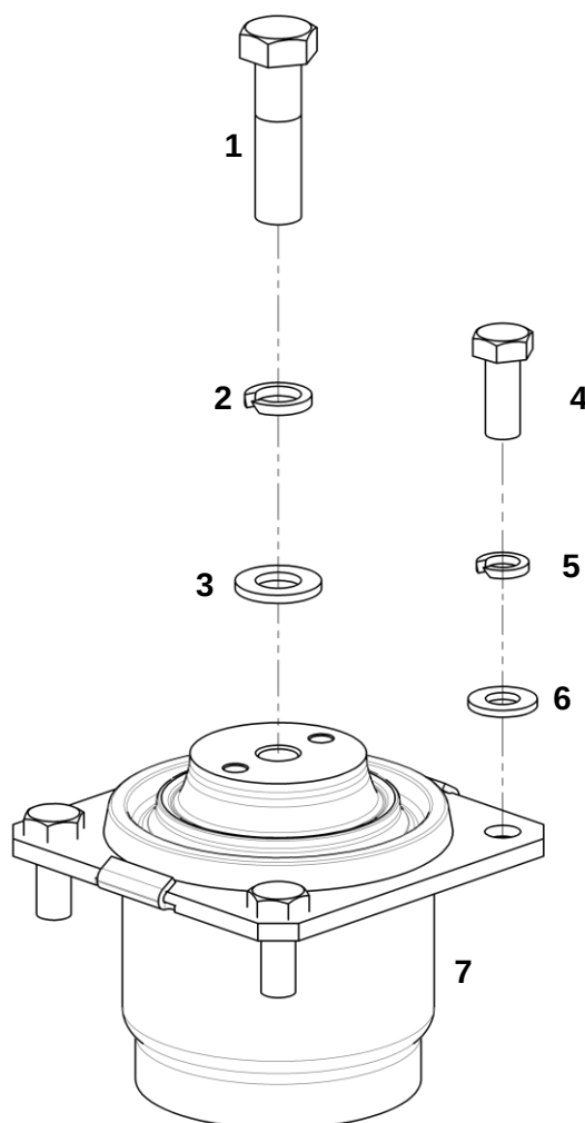
Система подрессоривания верхняя
