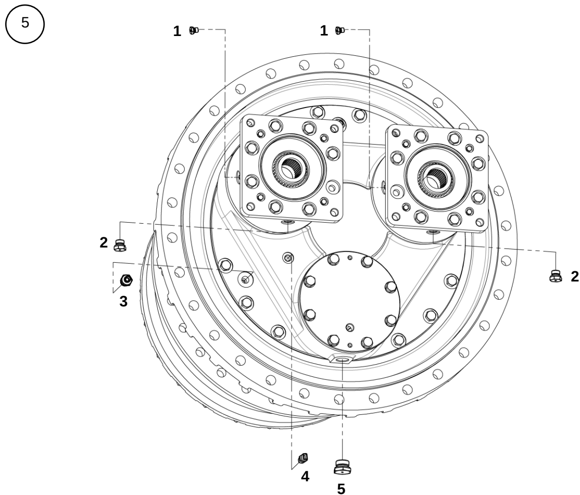
Редуктор хода
