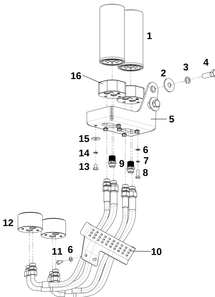
Комплект переноса масляных фильтров
