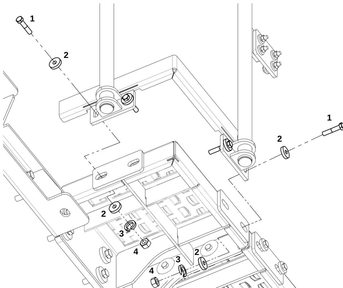
Боковые опоры в сборе
