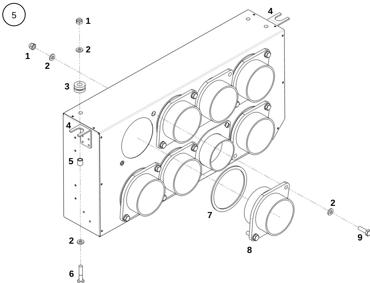
Блок распределения потоков
