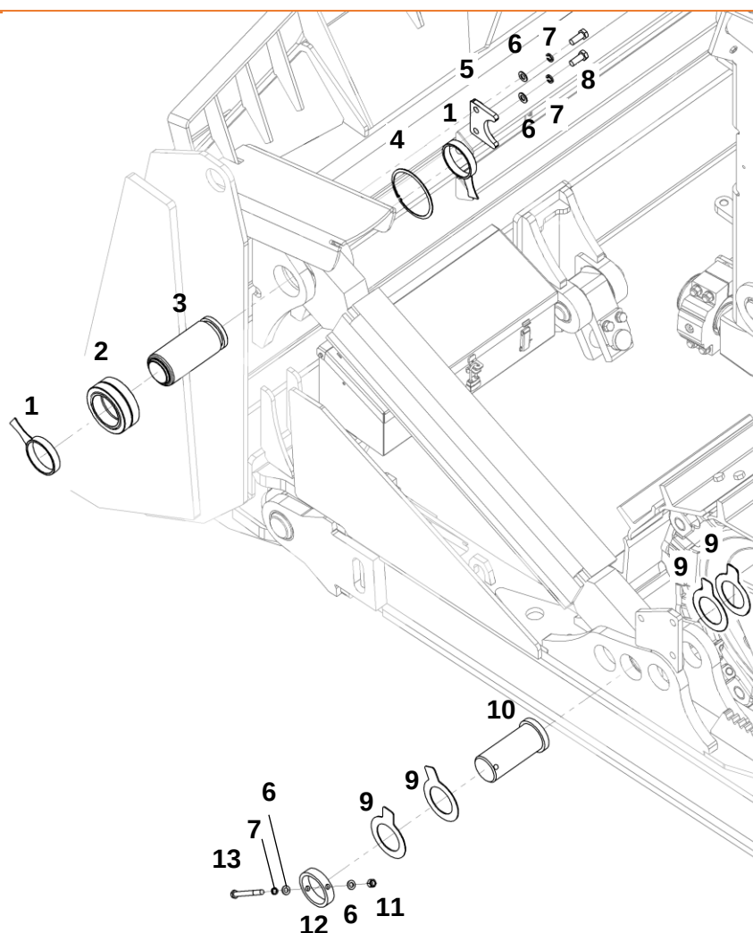
Крепление гидроцилиндра
