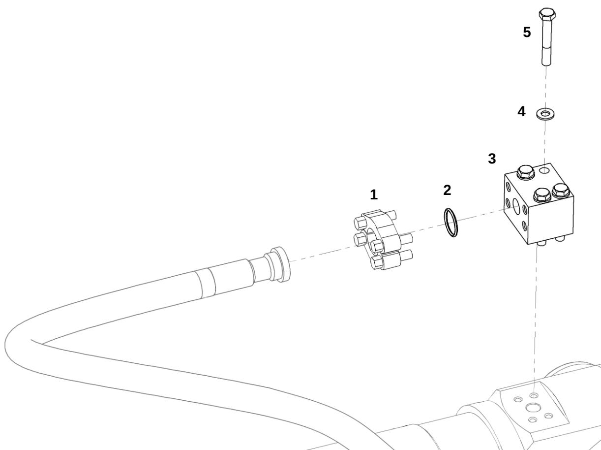
Крепление РВД к гидроцилиндру
