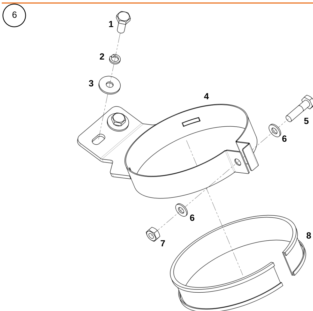
Хомут в сборе
