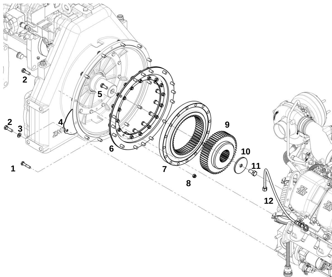
Силовой агрегат в сборе
