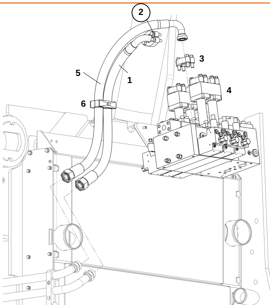
Гидрораспределитель в сборе
