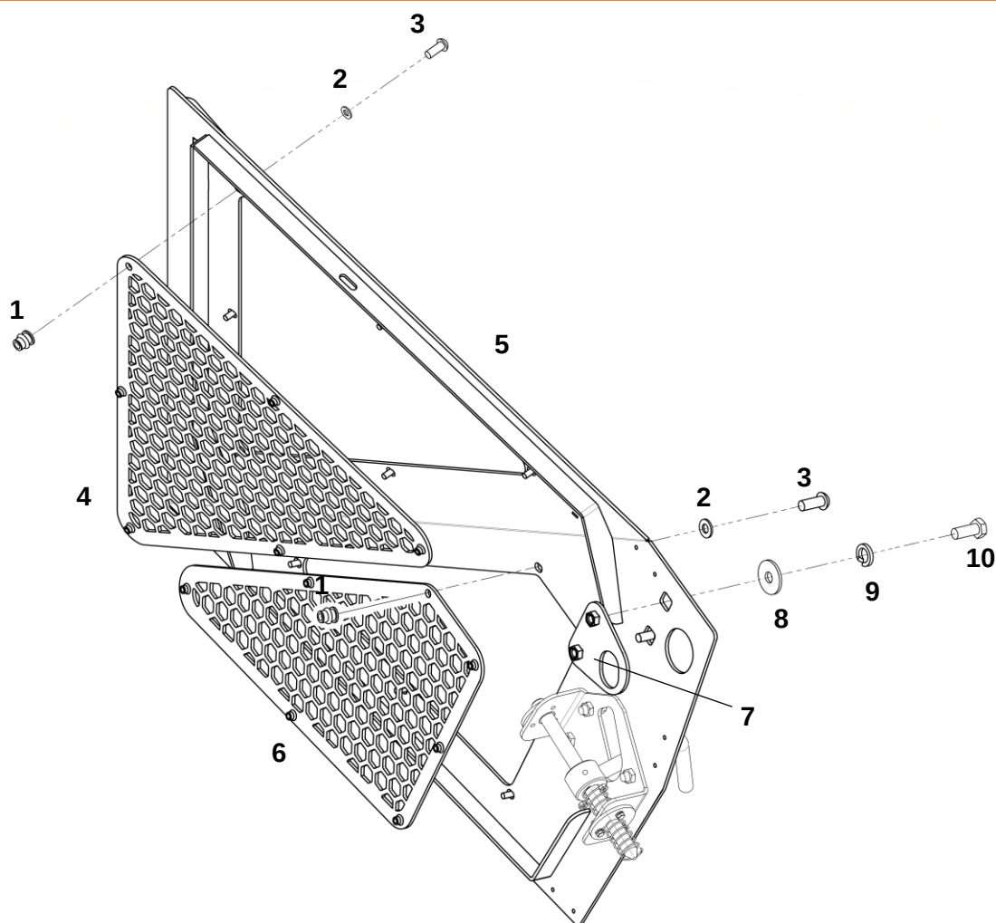
Створка в сборе
