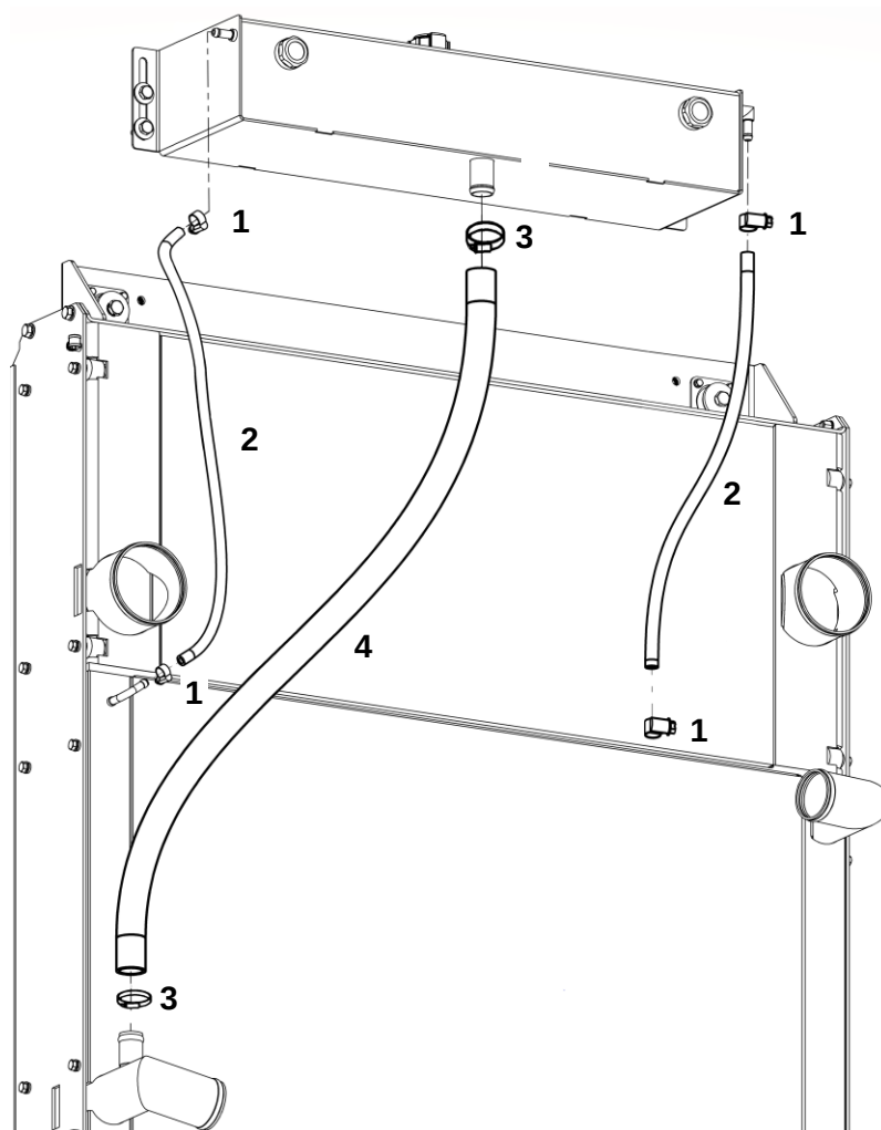
Установка рукавов к расширительному бачку
