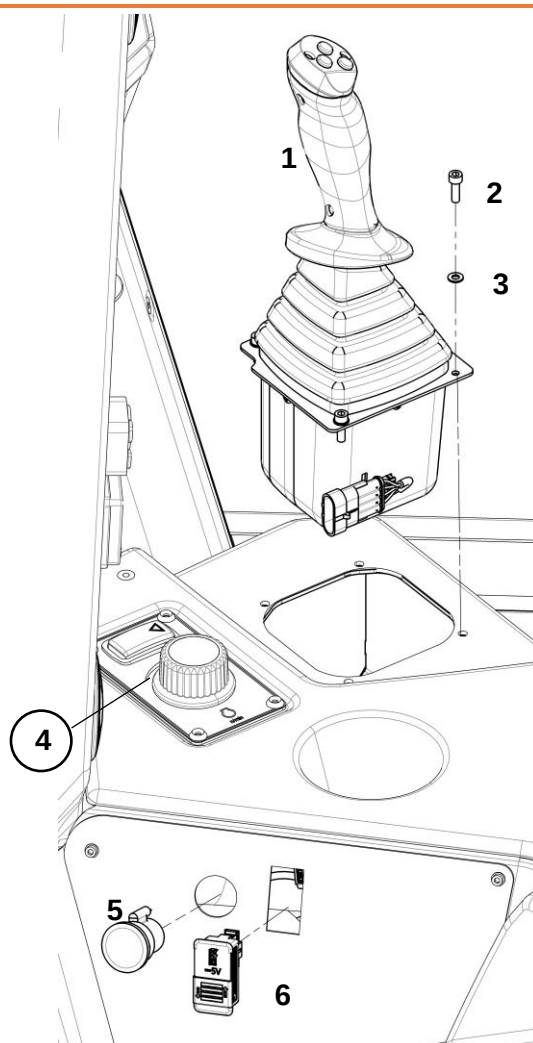
Пульт управления левый
