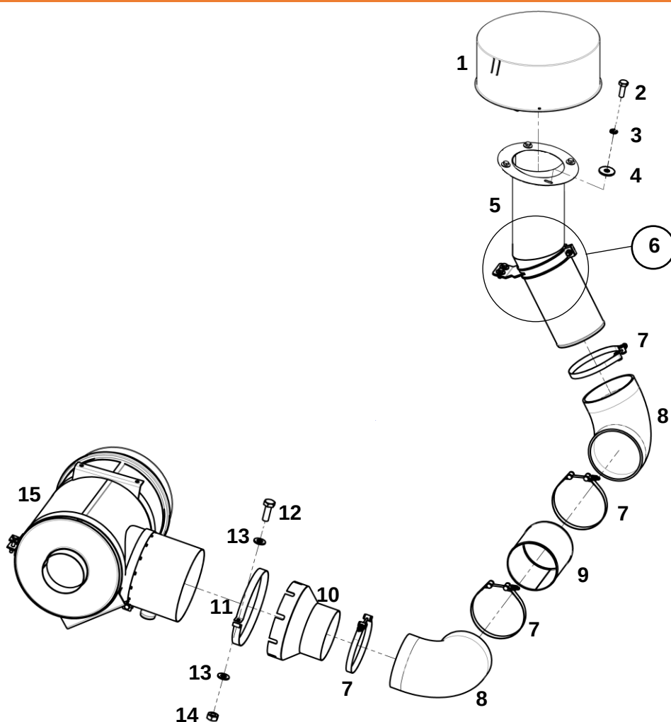
Фильтр предварительной очистки воздуха
