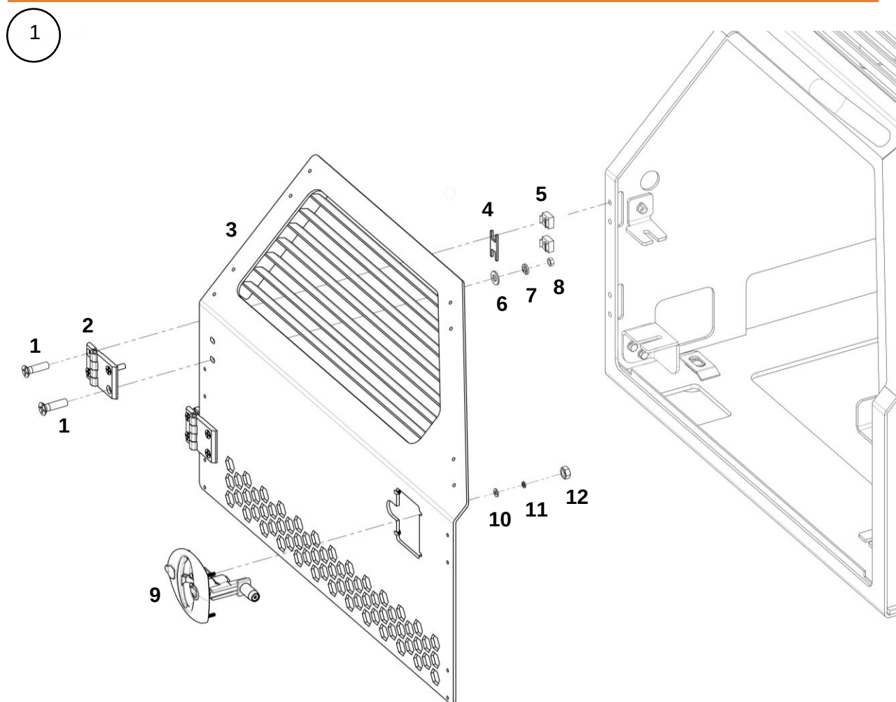
Корпус ящика в сборе
