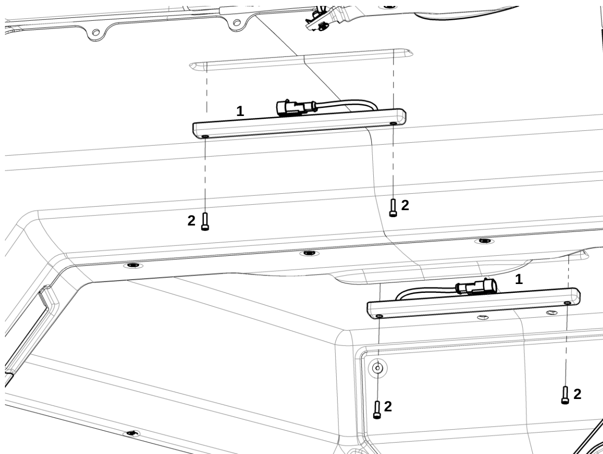
Элементы освещения кабины
