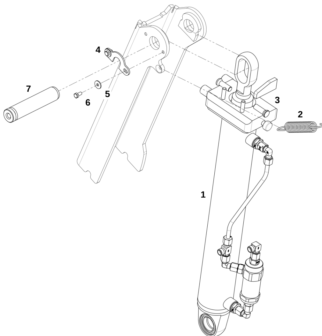
Соединение блокиратора и гидроцилиндра
