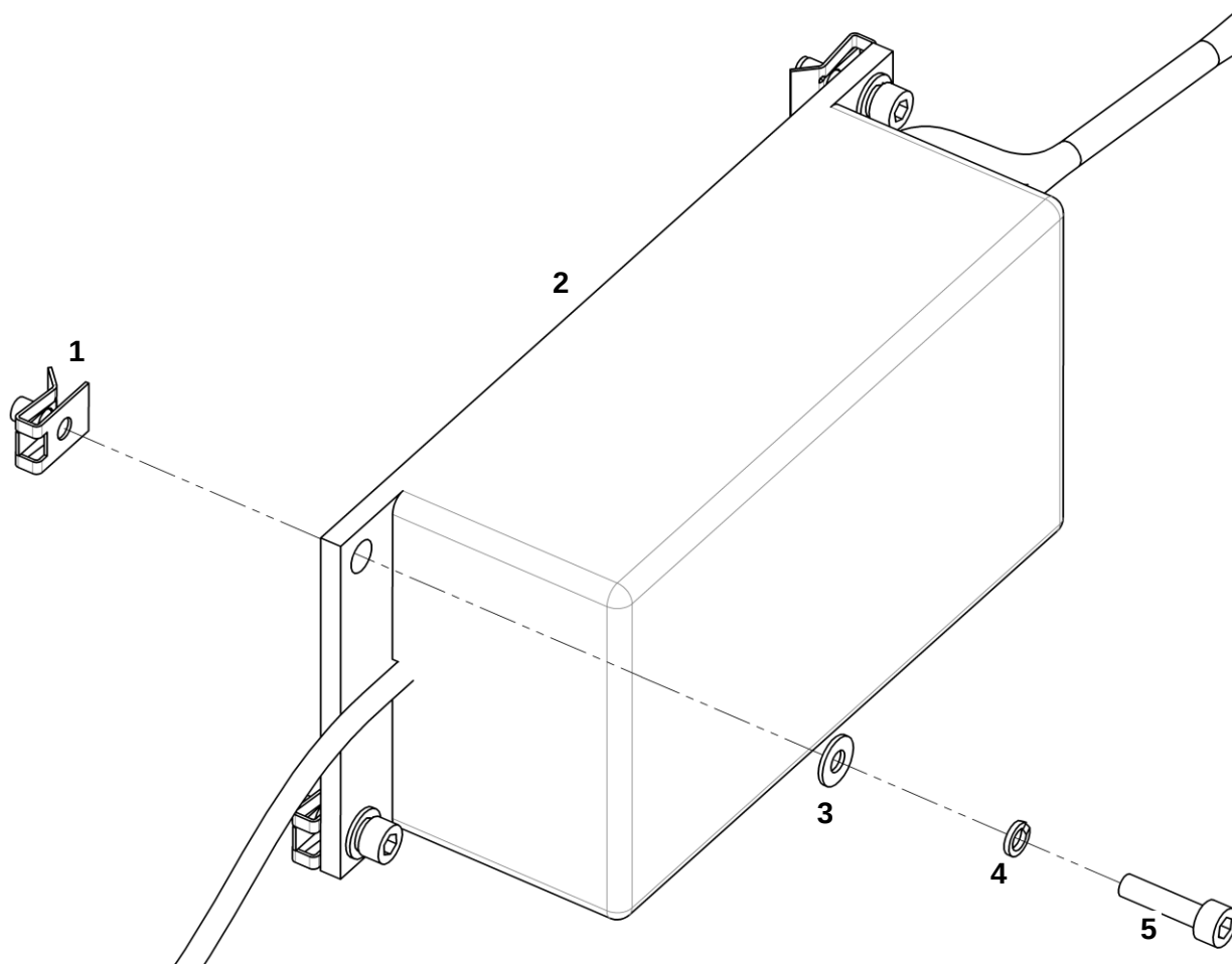
Преобразователь напряжения
