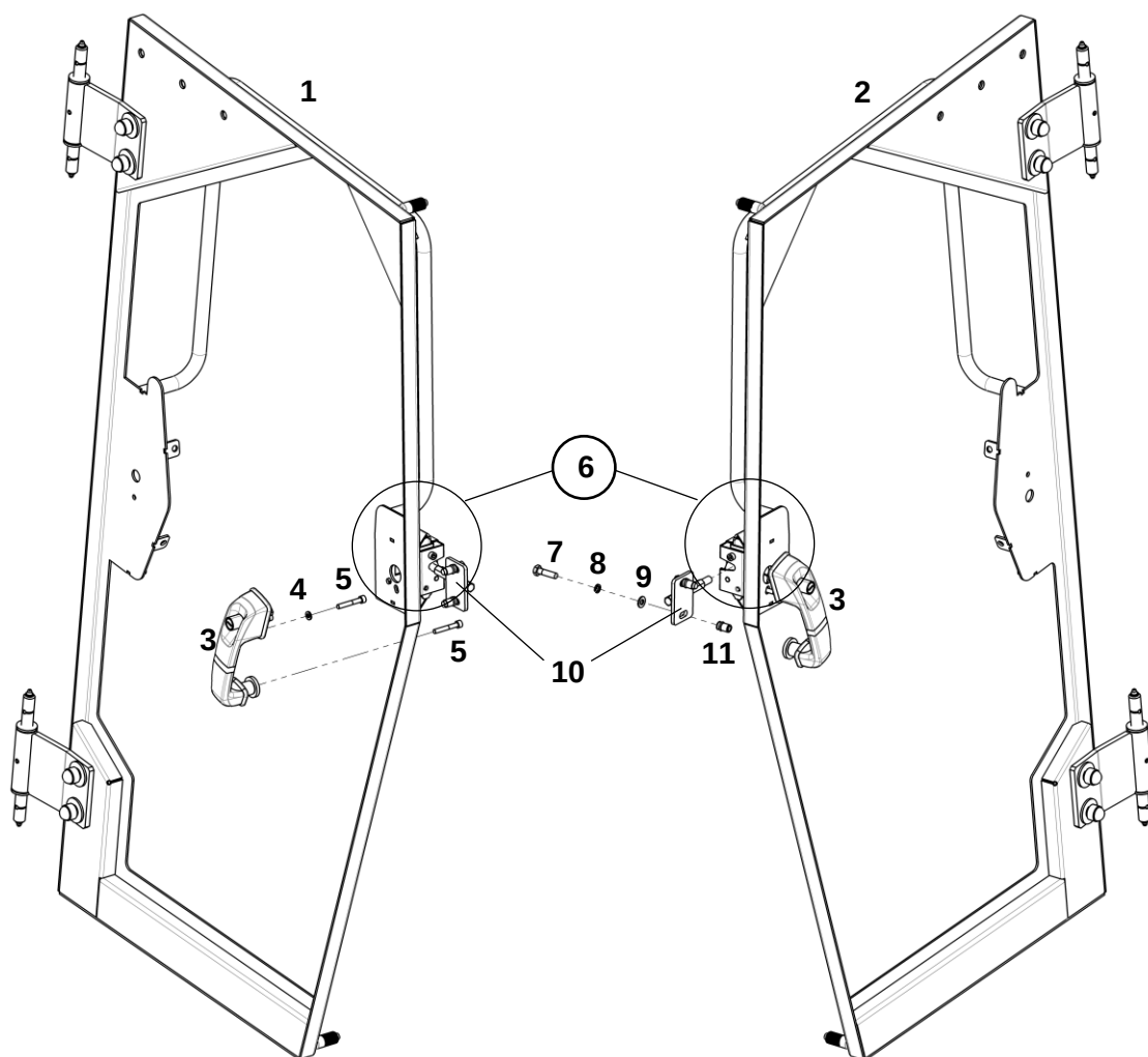
Дверь кабины
