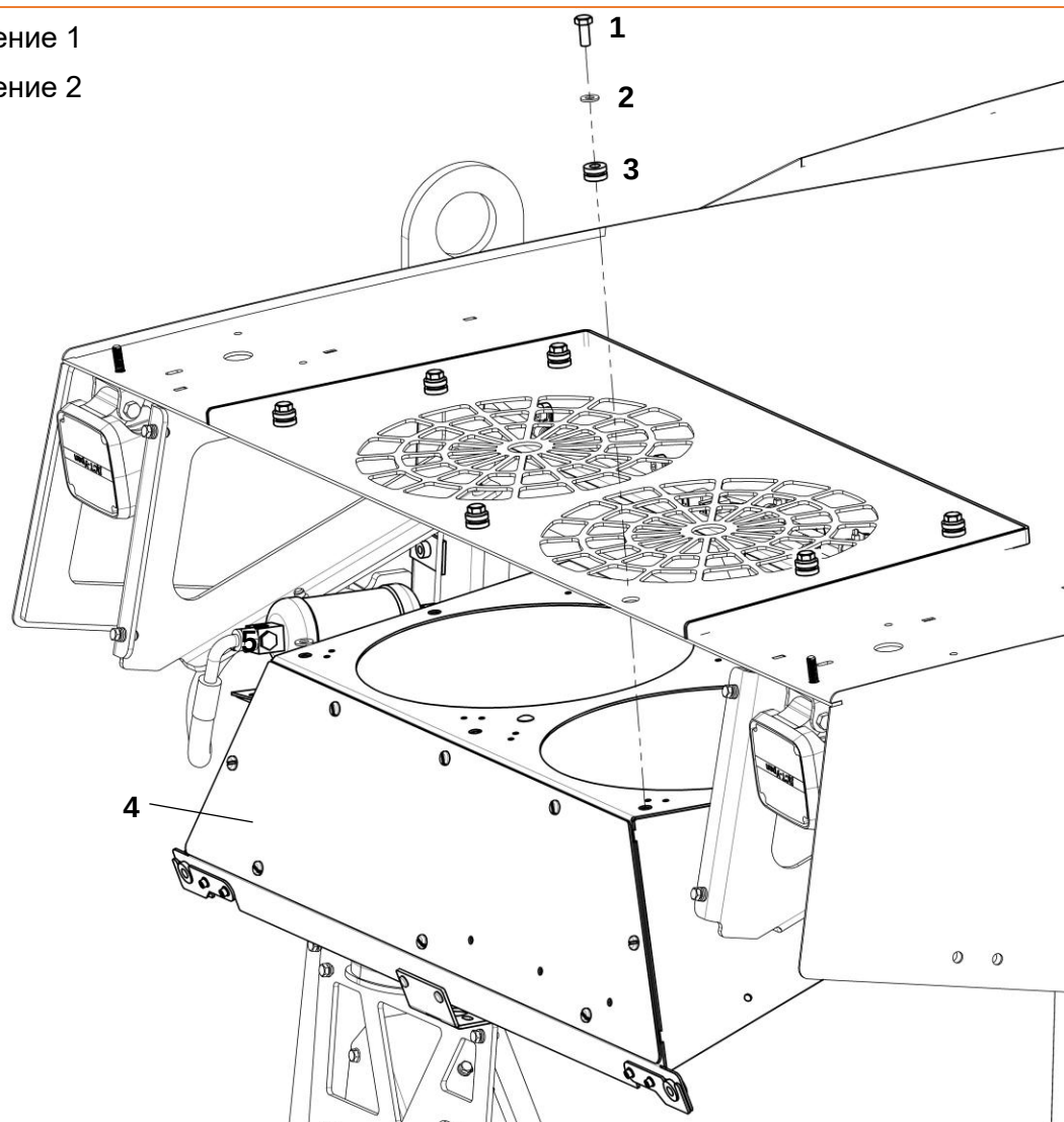
Установка блока конденсора
