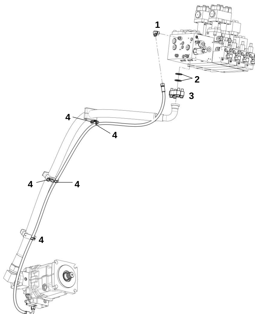
Подключение к распределителю отвала
