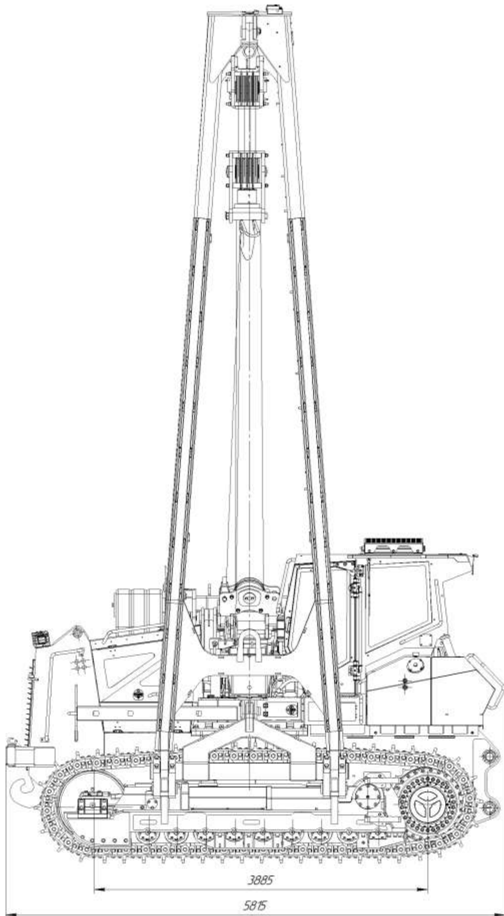
Рис. 1. Кран-трубоукладчик PL250 (вид со стороны стрелы).
