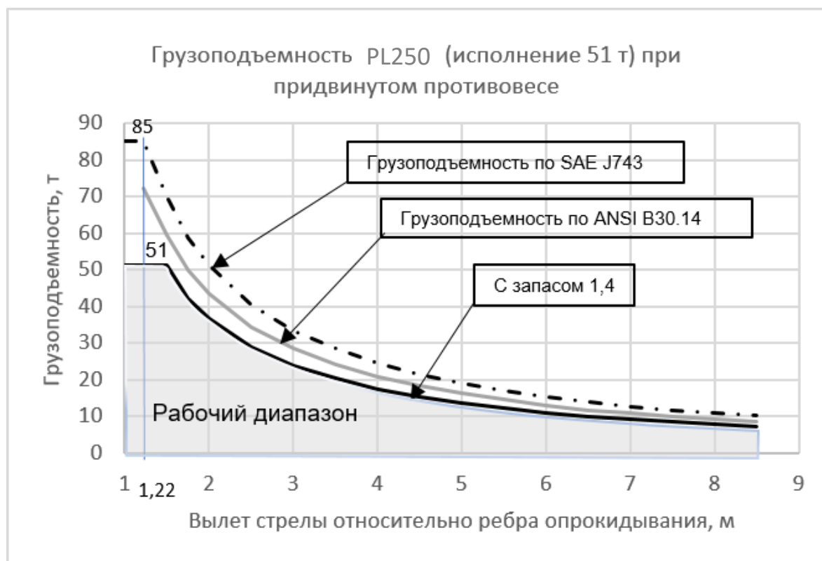
Рис. 4. Грузоподъемность PL250 при коэффициенте запаса грузовой устойчивости 1,4 и придвинутом противовесе
