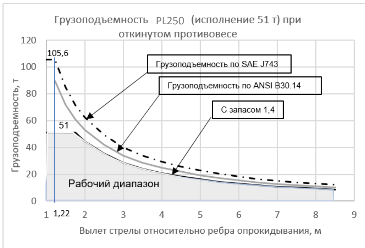
Рис. 3. Грузоподъемность PL250 при коэффициенте запаса грузовой устойчивости 1,4 и откинутах противовесе
