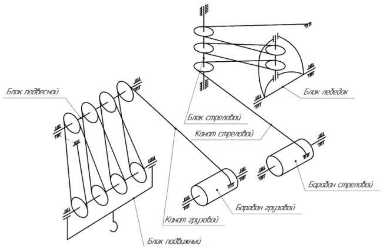
Схема запасовки канатов
