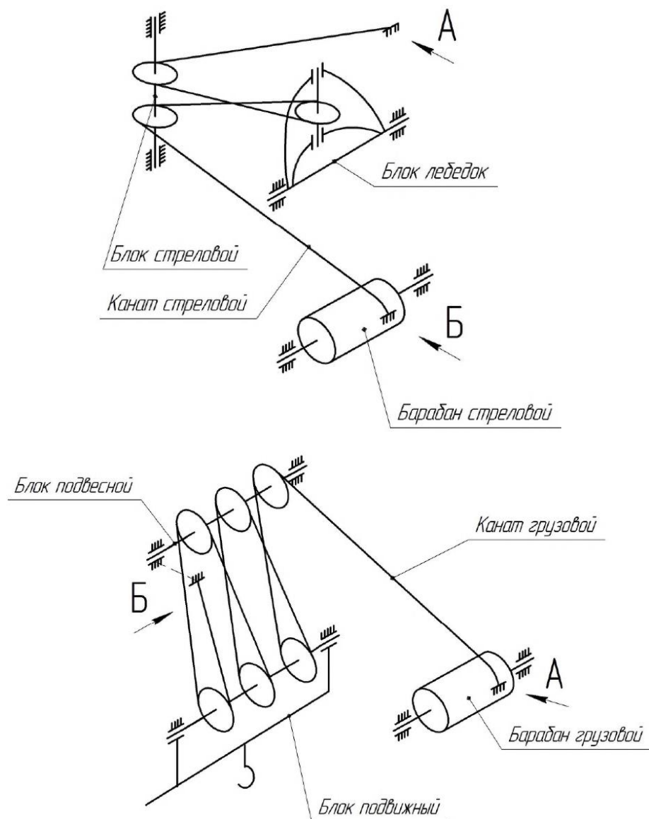
Схема запасовки канатов
