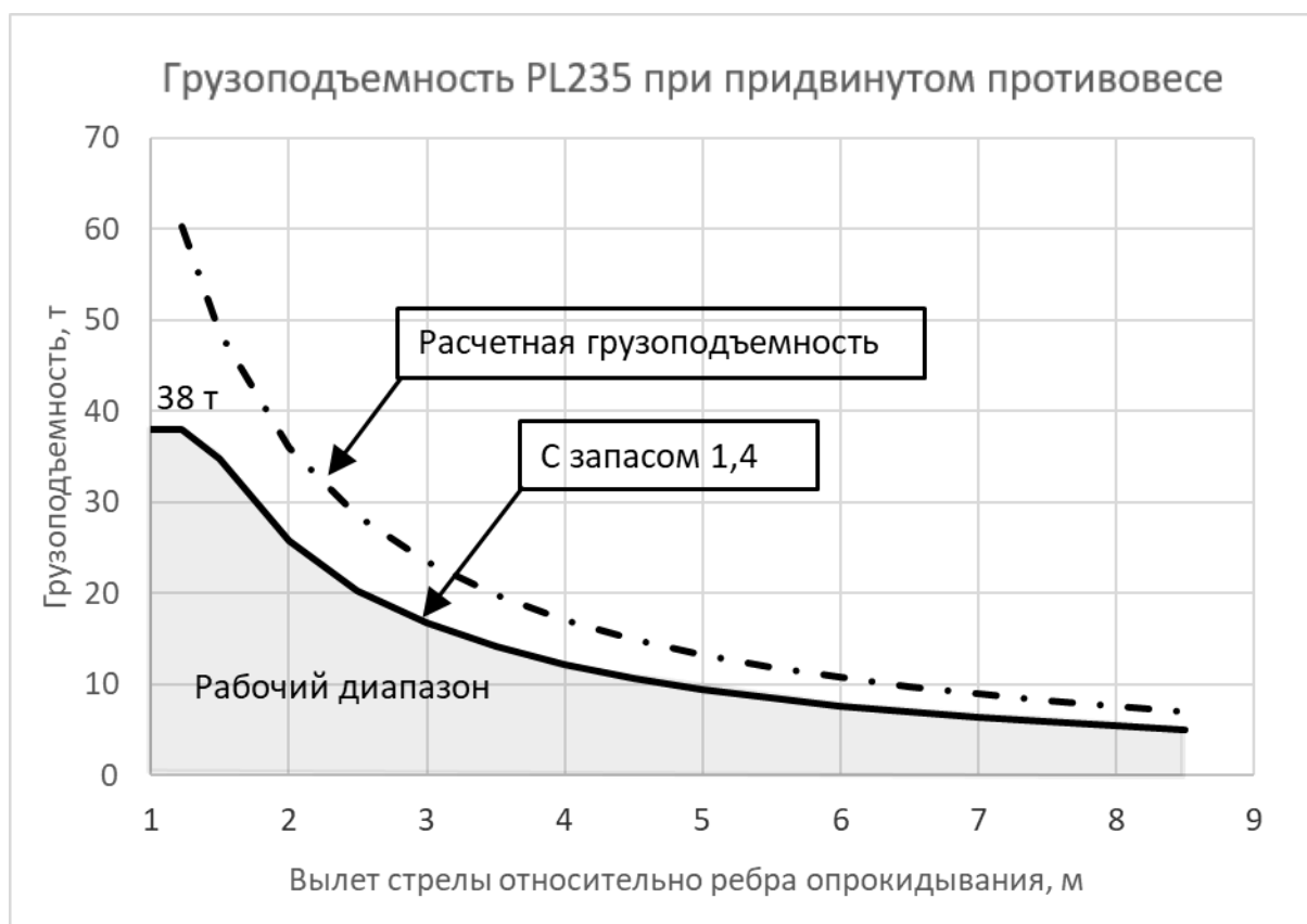
Рис. 4. Грузоподъемность PL235 при коэффициенте запаса грузовой устойчивости 1,4 и придвинутом противовесе
