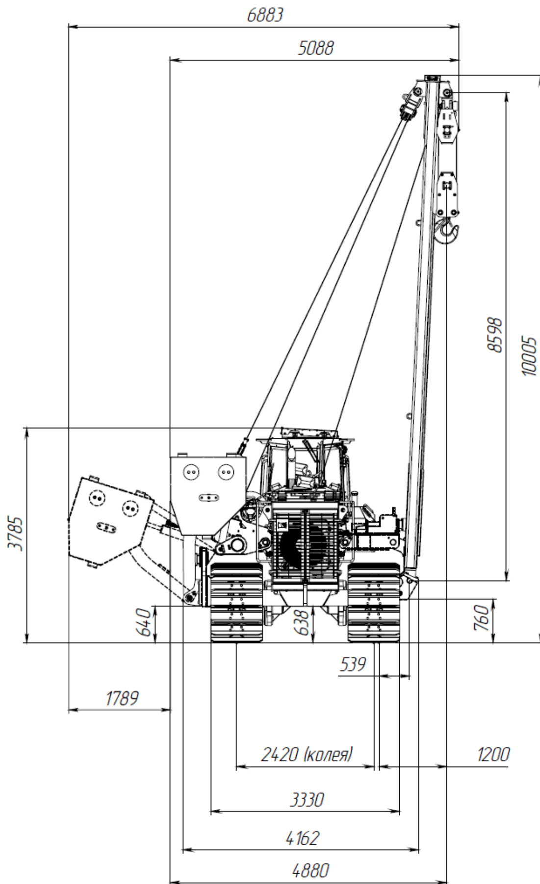
Рис. 2 (повернут). Кран-трубоукладчик PL235 (вид спереди)
