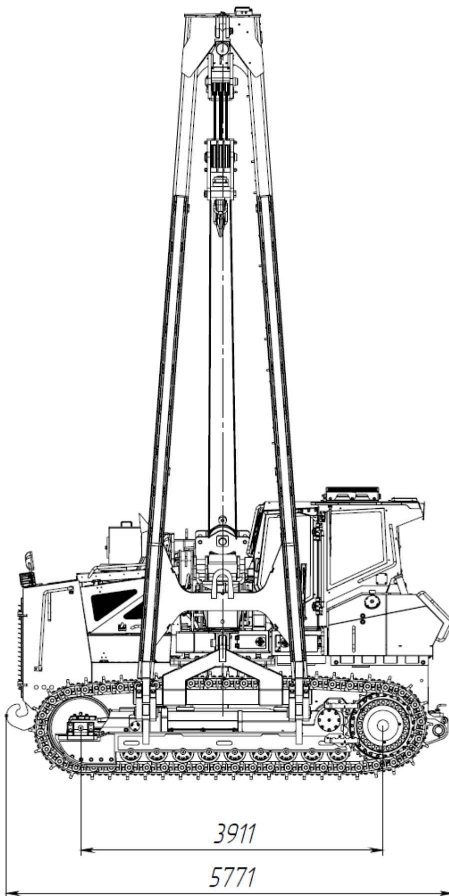
Рис. 1. Кран-трубоукладчик PL235 (вид со стороны стрелы).
