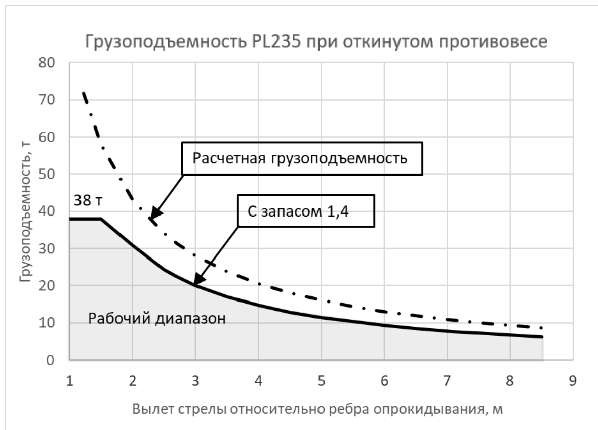
Рис. 3. Грузоподъемность PL235 при коэффициенте запаса грузовой устойчивости 1,4 и откинутах противовесе
