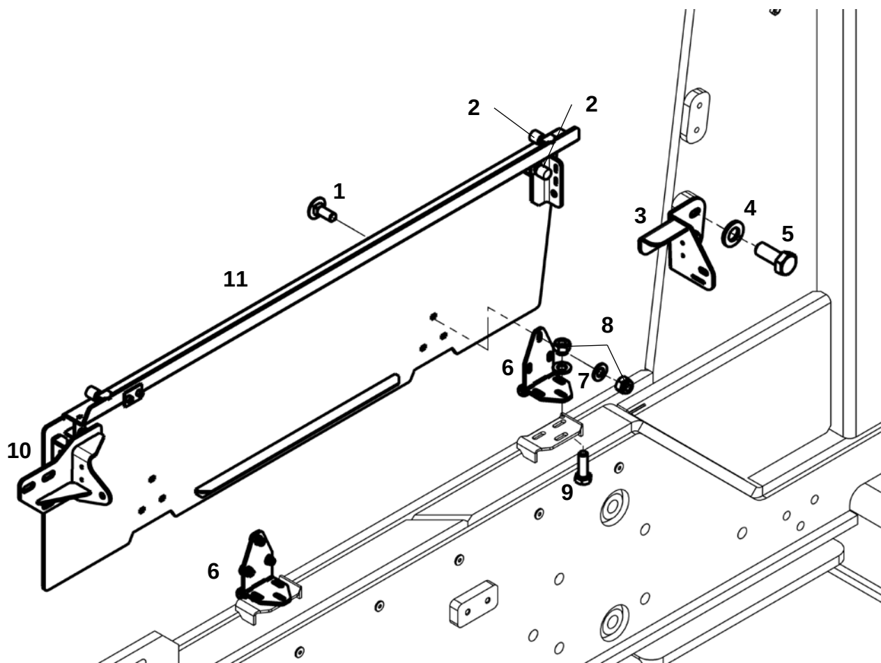
Крепление щита
