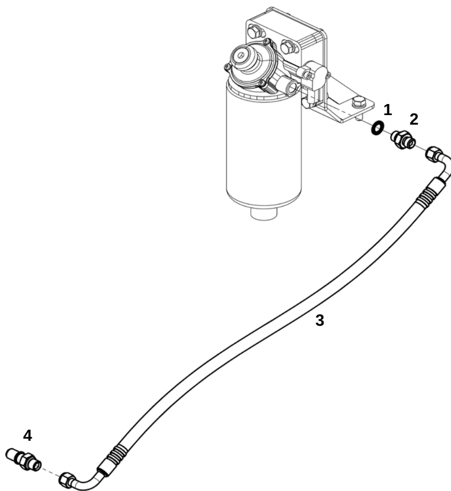
Топливопровод (ЯМЗ-536)
