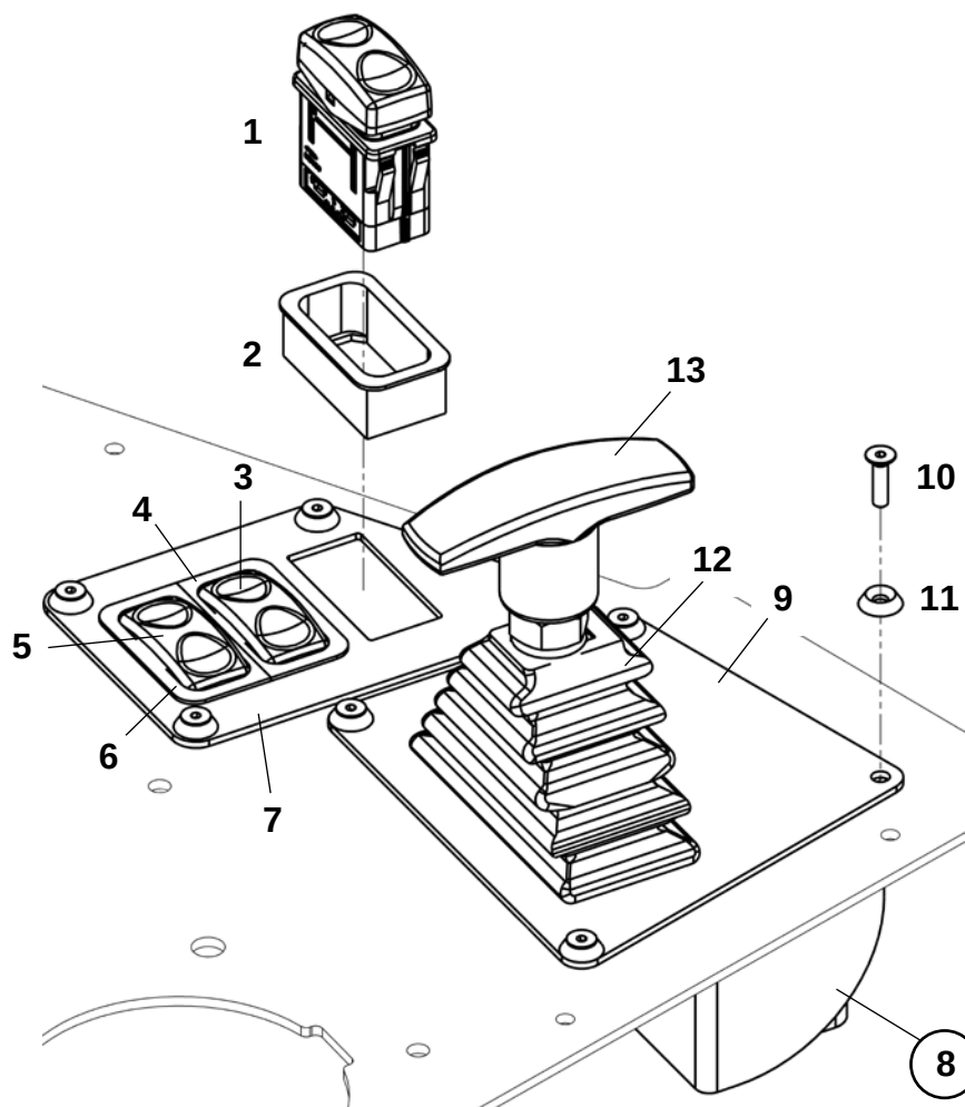
Обвязка левой тумбы
