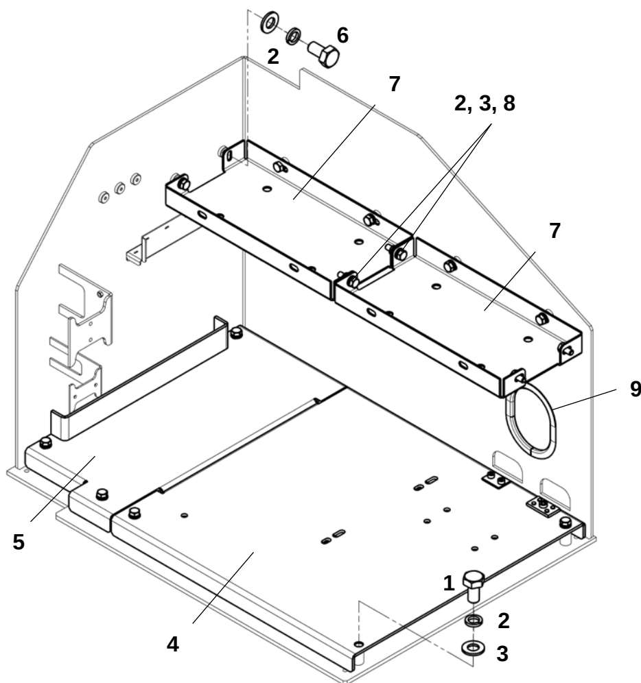
Ящик
