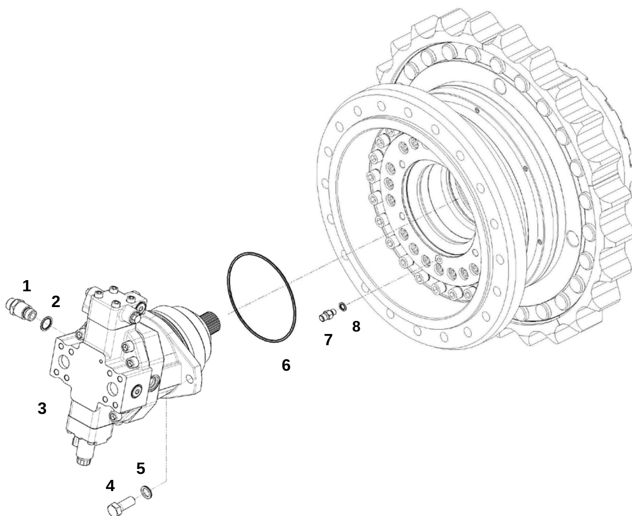
Комплект установки гидромотора
