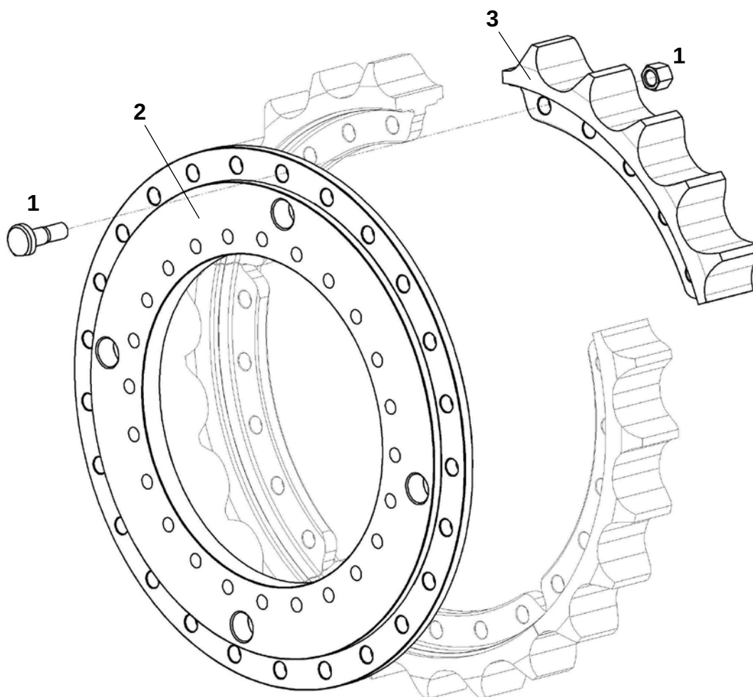
Комплект крепления сегментов
