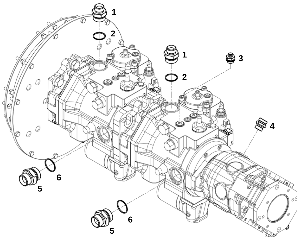
Комплект обвязки насосов гидравлических A4VG145, A10V0100
