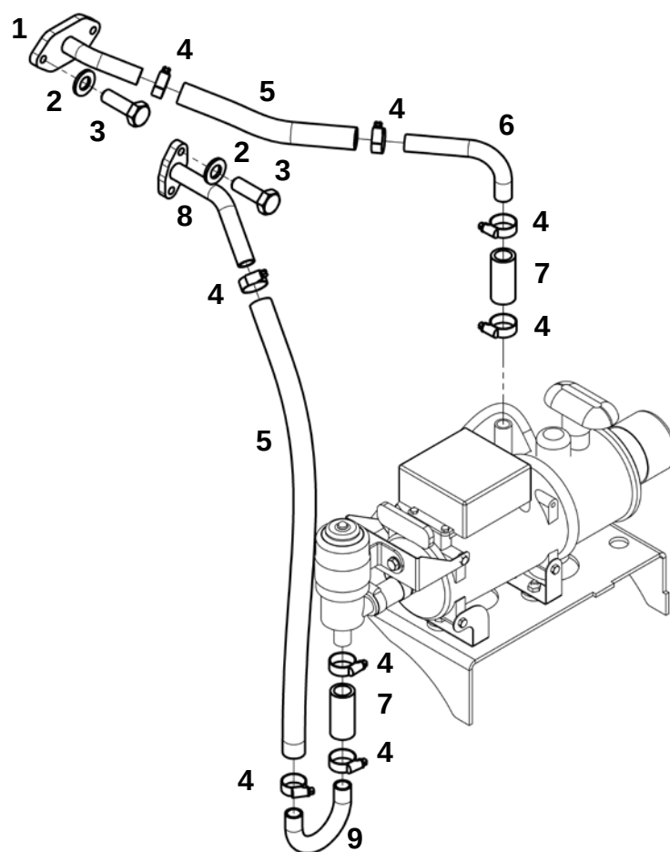
Установка ПЖД (ЯМЗ-536)
