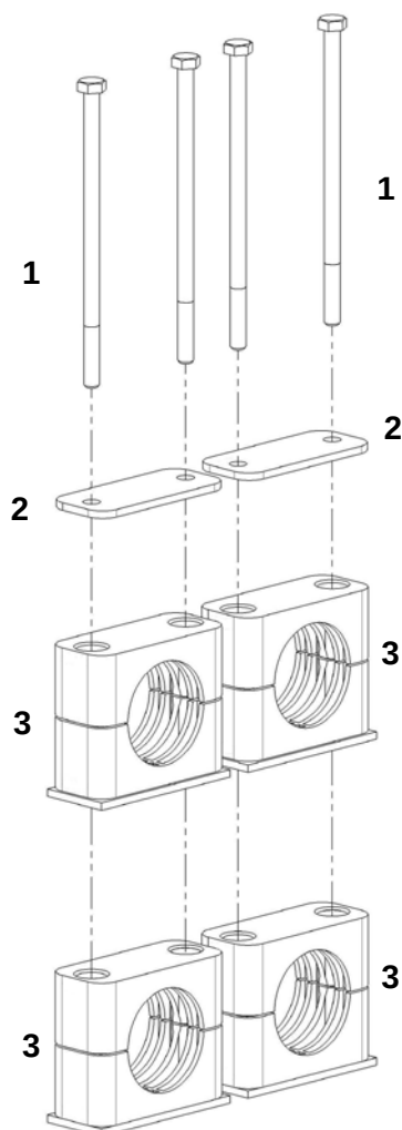
Зажим в сборе
