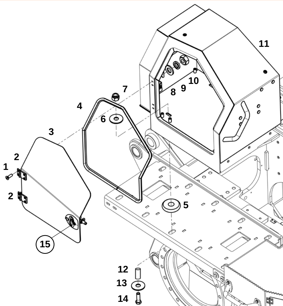
Установка ящика
