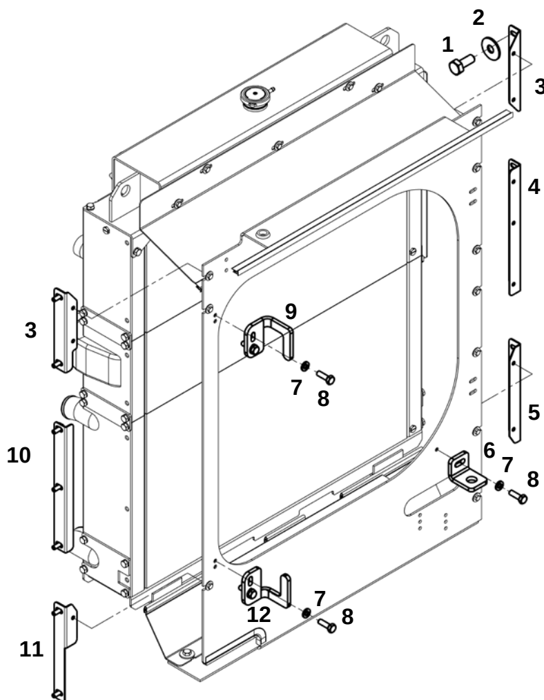
Комплект щитков капотирования
