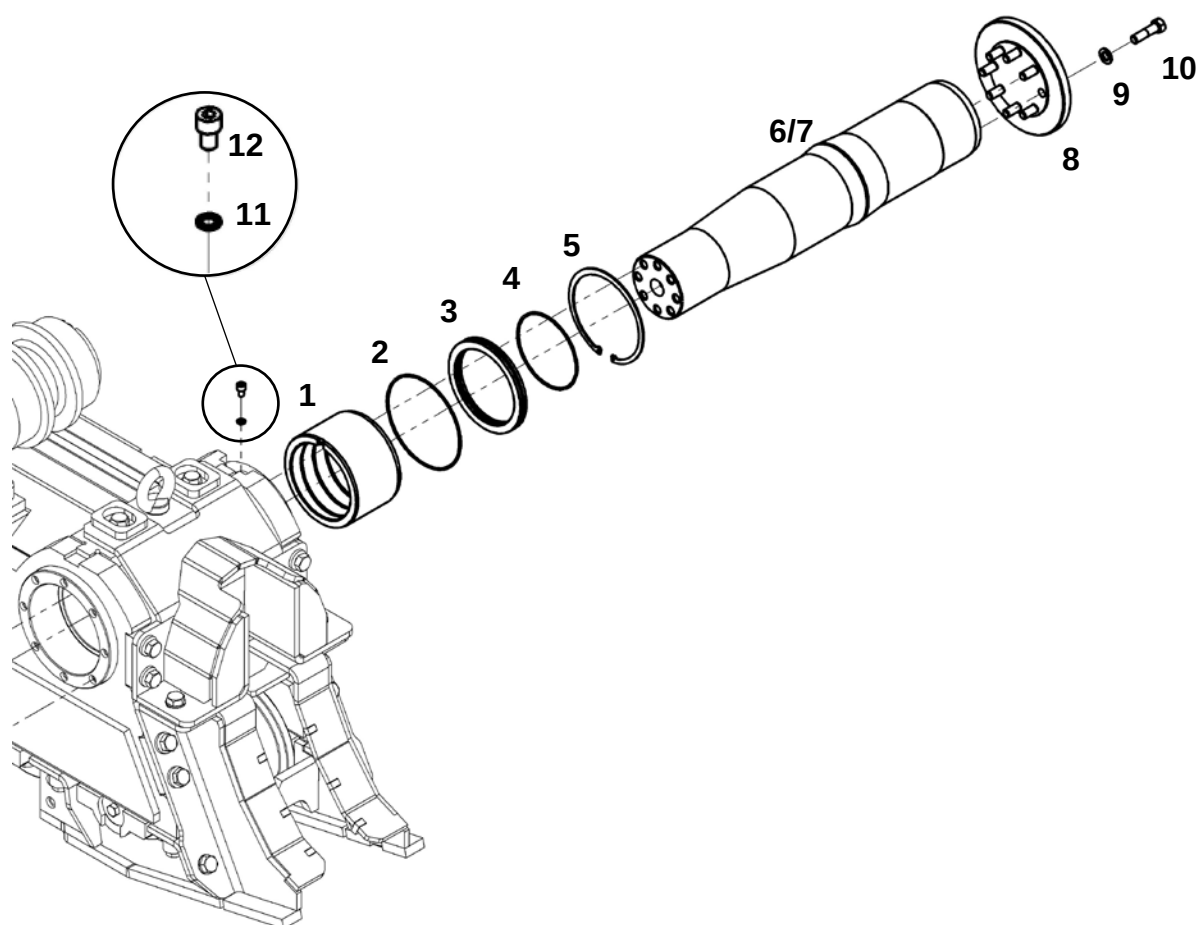
Полуось в сборе
