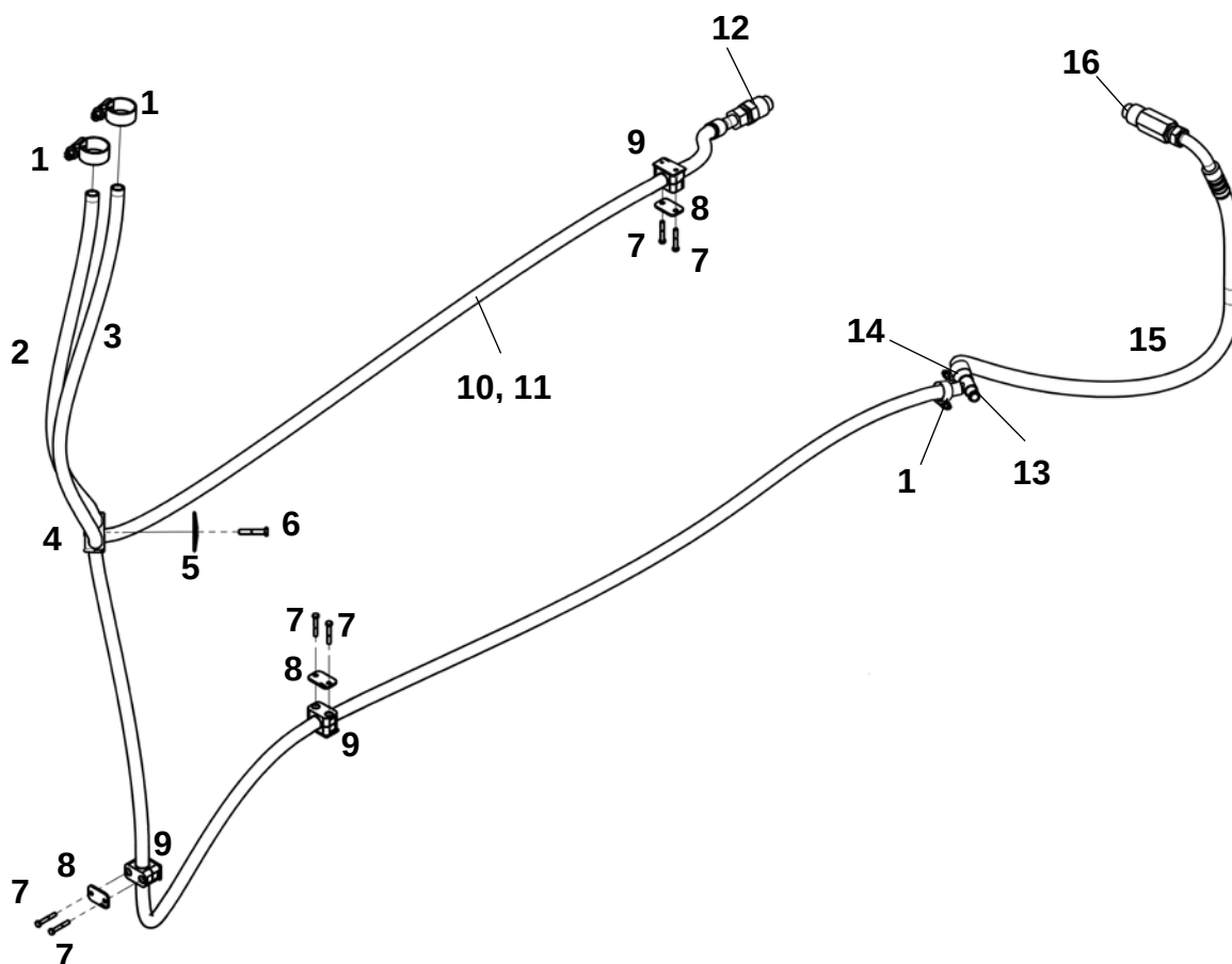
Рукава системы отопления кабины оператора (Cummins QSL 8.9)
