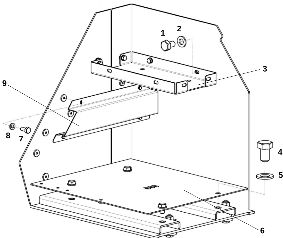
Ящик инструментальный (ЯМЗ-536; Cummins QSL 8.9)
