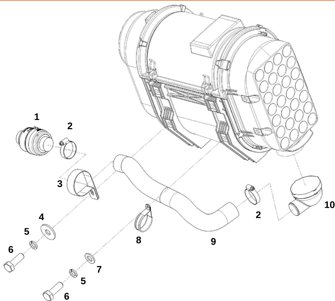
Комплект установки обратного клапана (ЯМЗ-536)
