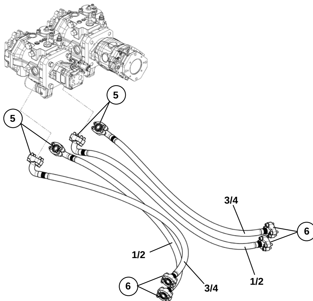
РВД трансмиссии (A4VG145)
