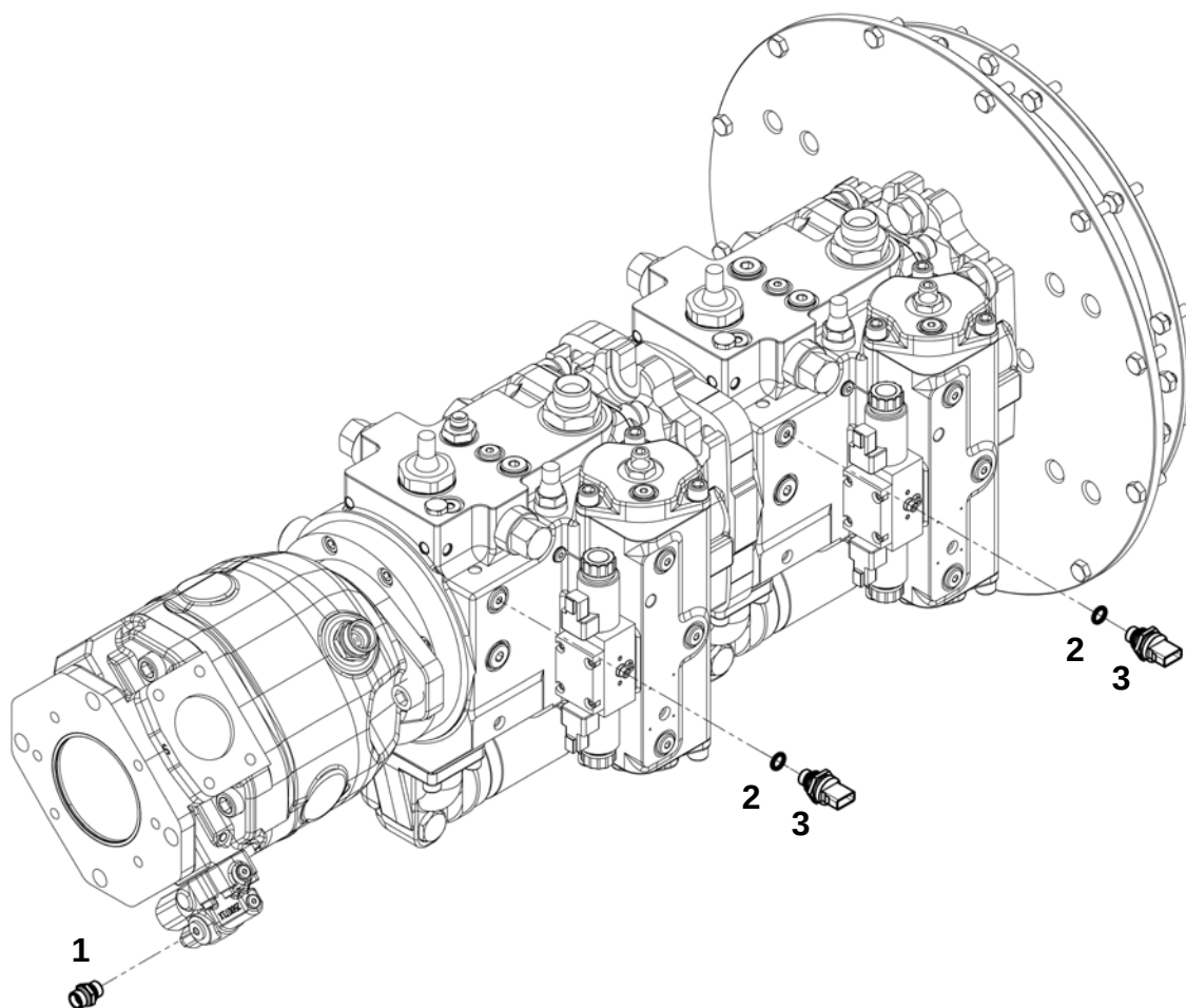
Комплект обвязки насосов гидравлических A4VG145, A10V0100
