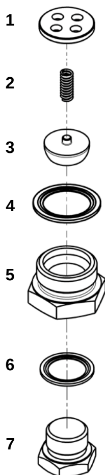
Пробка сливная
