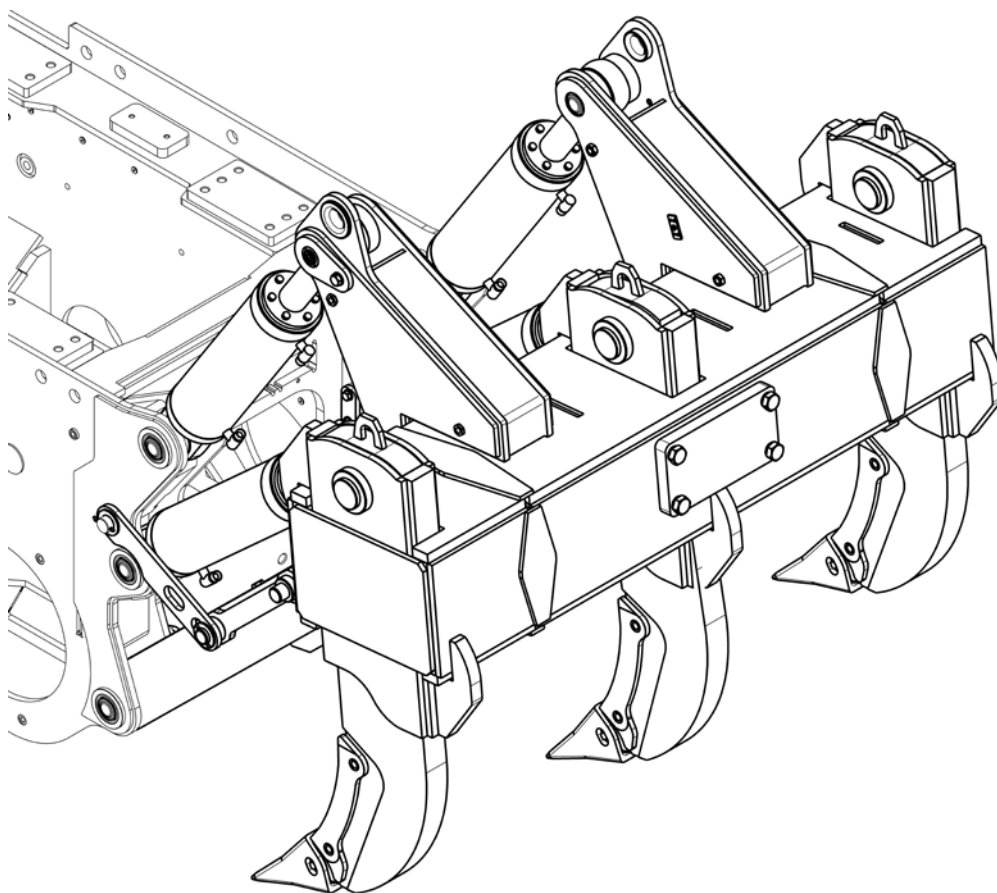
Рыхлитель трехзубый 2-х координатный
