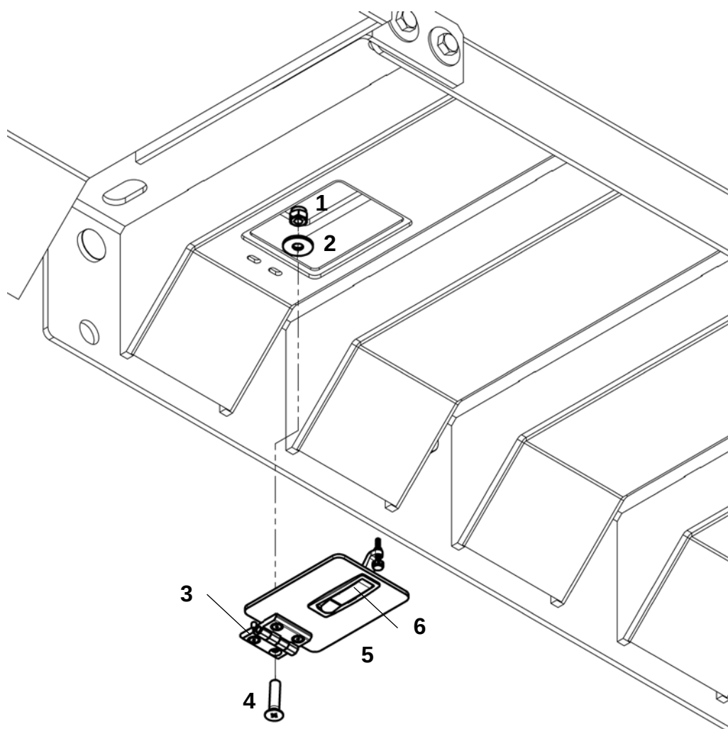
Установка замка
