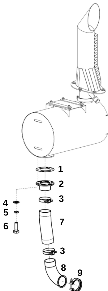
Выпускной тракт (Cummins QSL 8.9)
