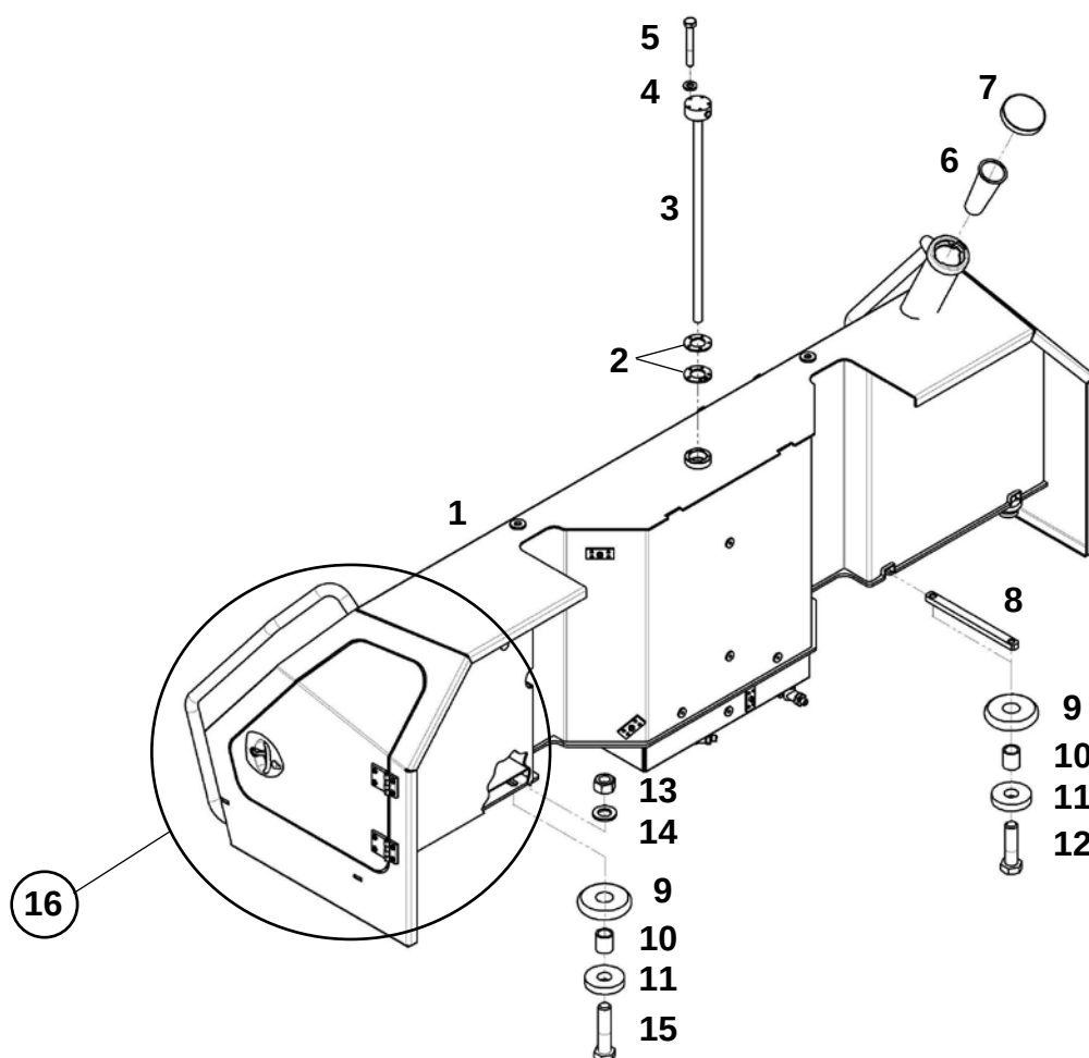
Топливный бак (ЯМЗ-536; Cummins QSL 8.9)
