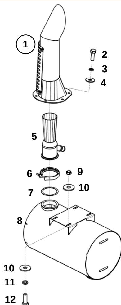
Труба выхлопная и глушитель (Cummins QSL 8.9)
