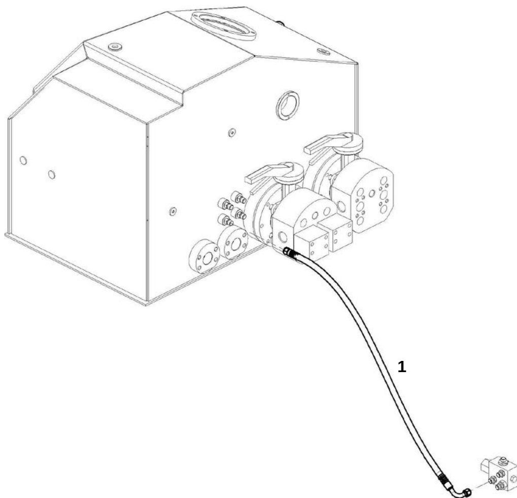
РВД слив с блока клапанов
