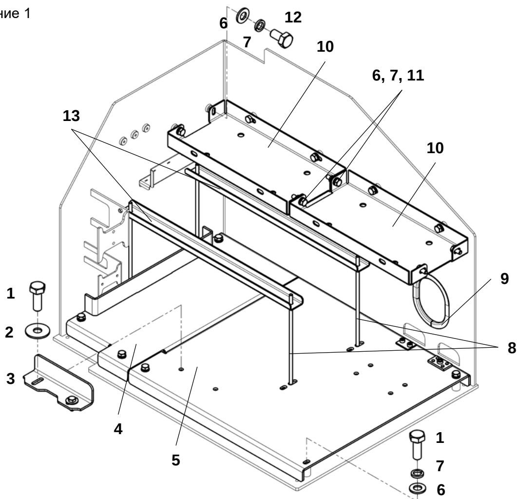
Ящик
