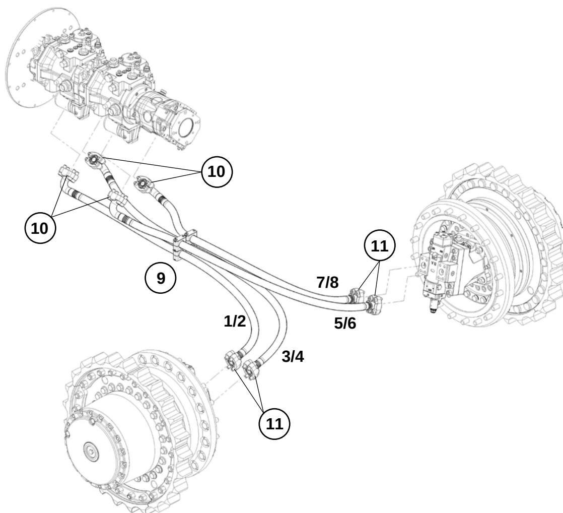
РВД трансмиссии (A4VG145, A4VG110)
