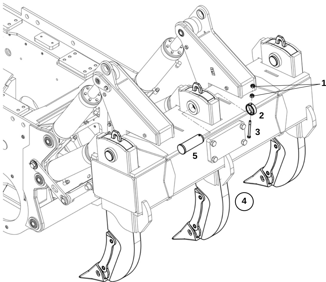
Крепление ножа трехзубого рыхлителя
