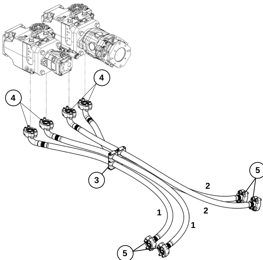
РВД трансмиссии (Н1-Р-147)
