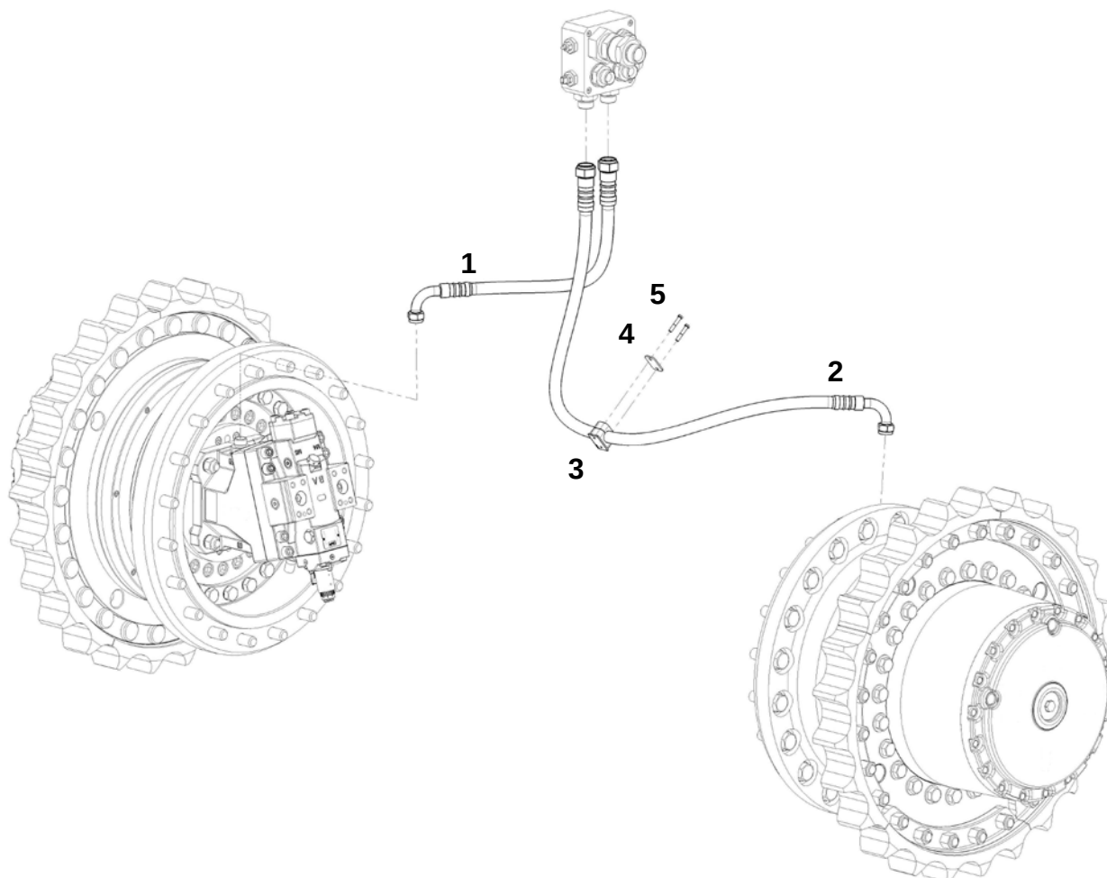
РВД дренажа гидромоторов (A6VE170; H1-B-210)
