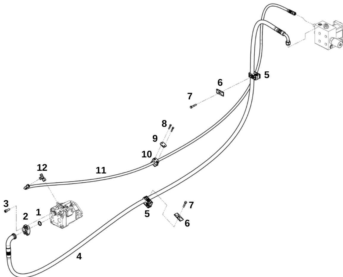
Система привода вентилятора Fan Drive (Cummins QSL 8.9; A10V028)
