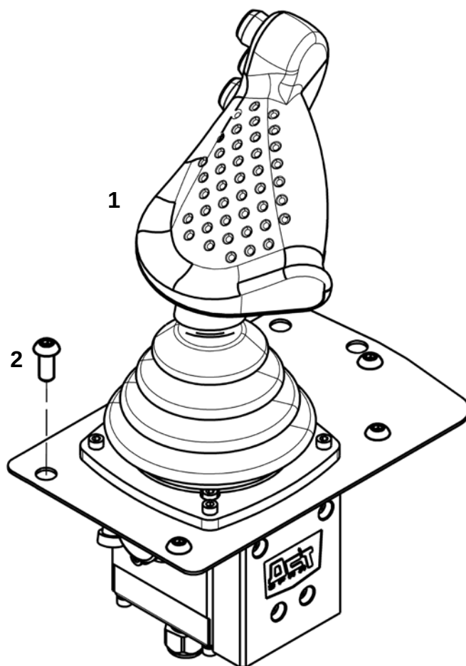
Установка джойстика навесного оборудования
