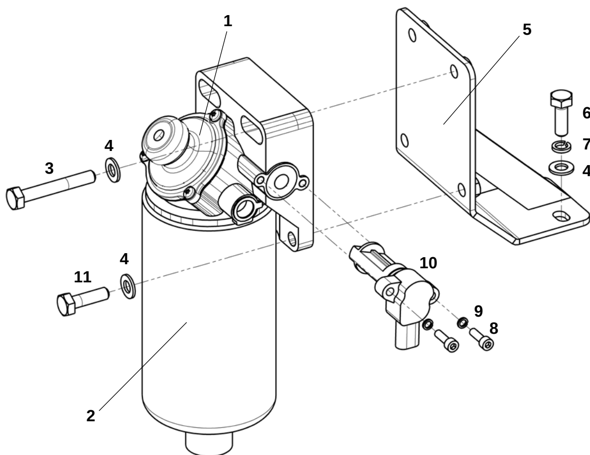
Корпус фильтра грубой очистки топлива в сборе (ЯМЗ-536)
