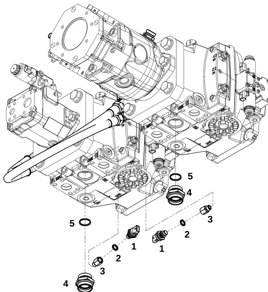
Комплект обвязки насосов гидравлических Н1-Р-147, А10V0100, А10V028
