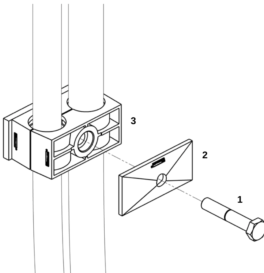
Зажим в сборе
