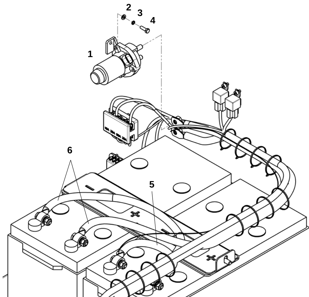
Подключение аккумуляторных батарей
