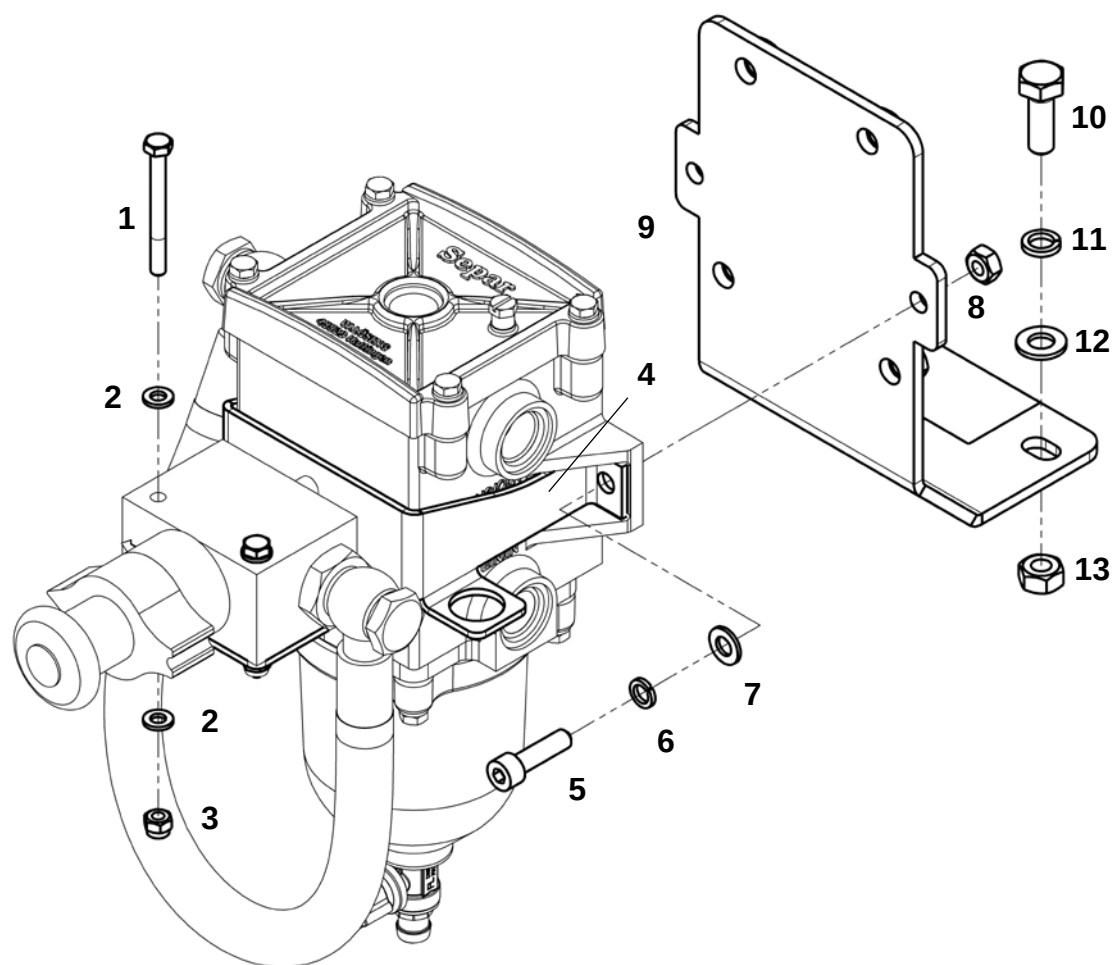
Корпус фильтра грубой очистки топлива в сборе (Cummins QSL 8.9)
