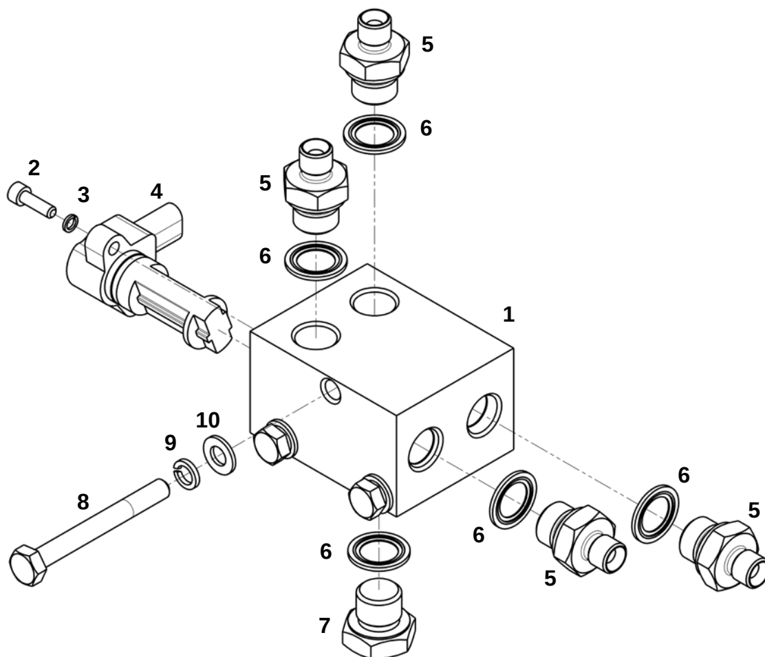
Плита в сборе (ЯМЗ-536)
