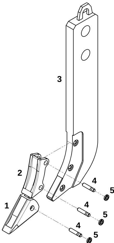
Нож в сборе
