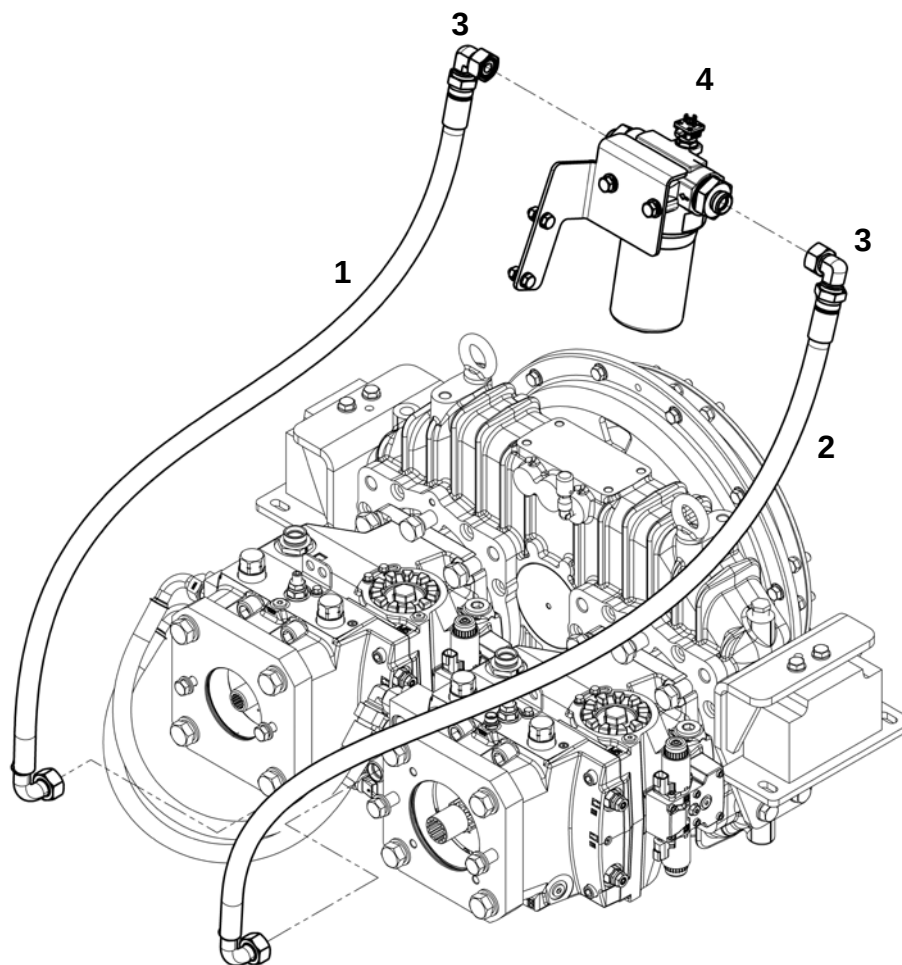
РВД от насоса к фильтру (Н1-В-147)
