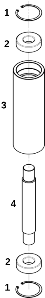
Ролик
