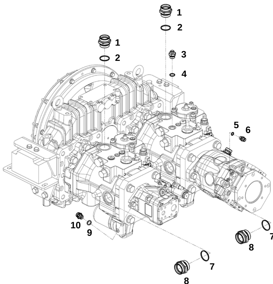
Комплект обвязки насосов гидравлических A4VG145, A10V0100, A10V028
