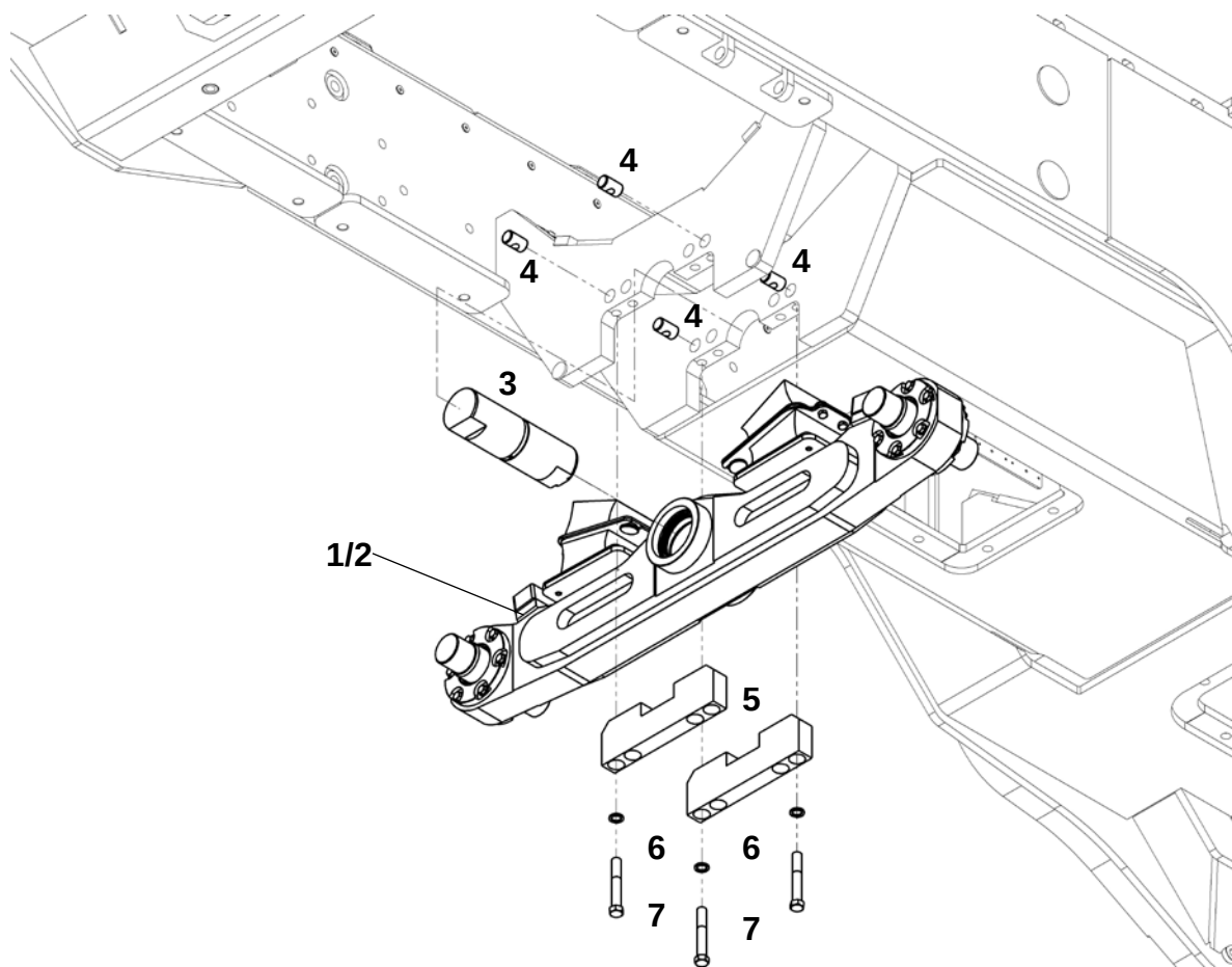
Балка балансирующая крепление к раме
