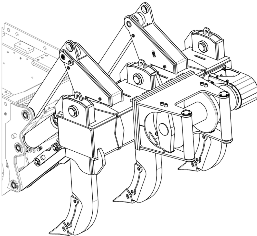
Рыхлитель трехзубый с лебедкой 30т
