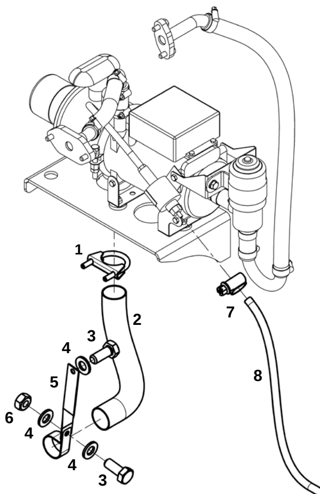
Комплект установки ПЖД (ЯМЗ-536)
