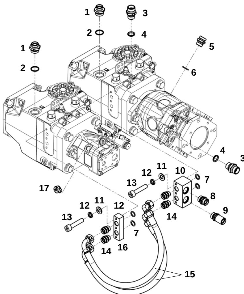
Комплект обвязки насосов гидравлических Н1-Р-147, А10V0100, А10V028
