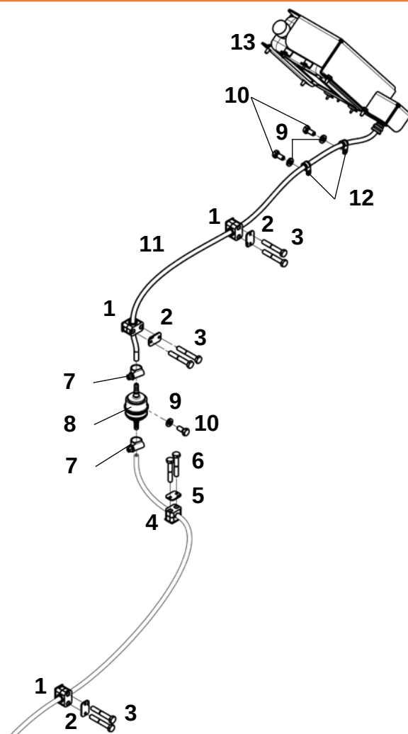
Комплект установки ПЖД (ЯМЗ-536; Cummins)
