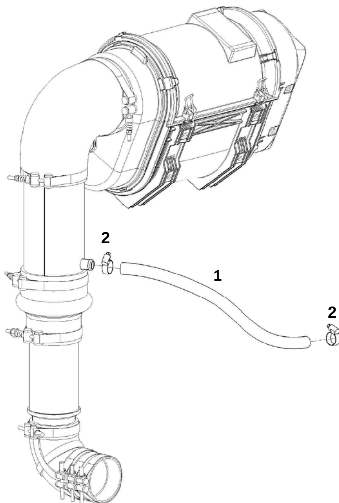
Рукав отбора вентиляции картерных газов (ЯМЗ-536)
