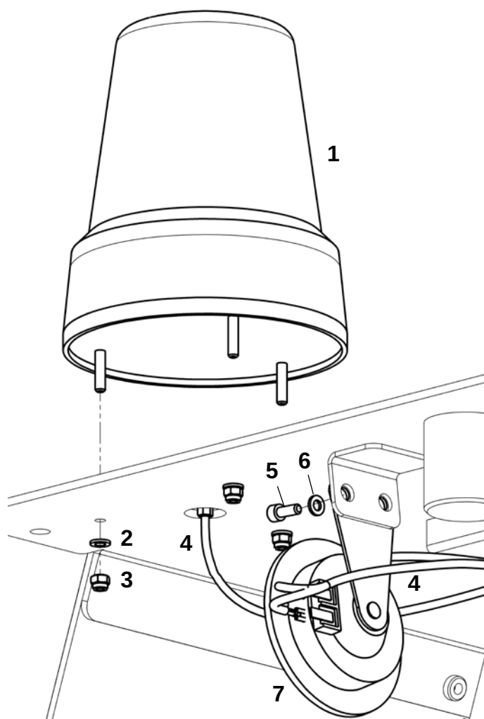
Маяк и звуковой сигнал
