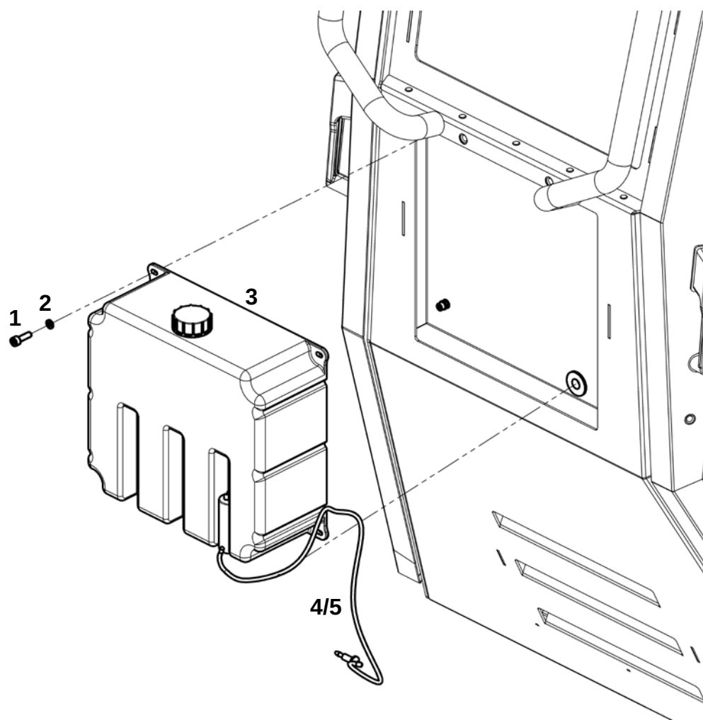
Бачок омывателя
