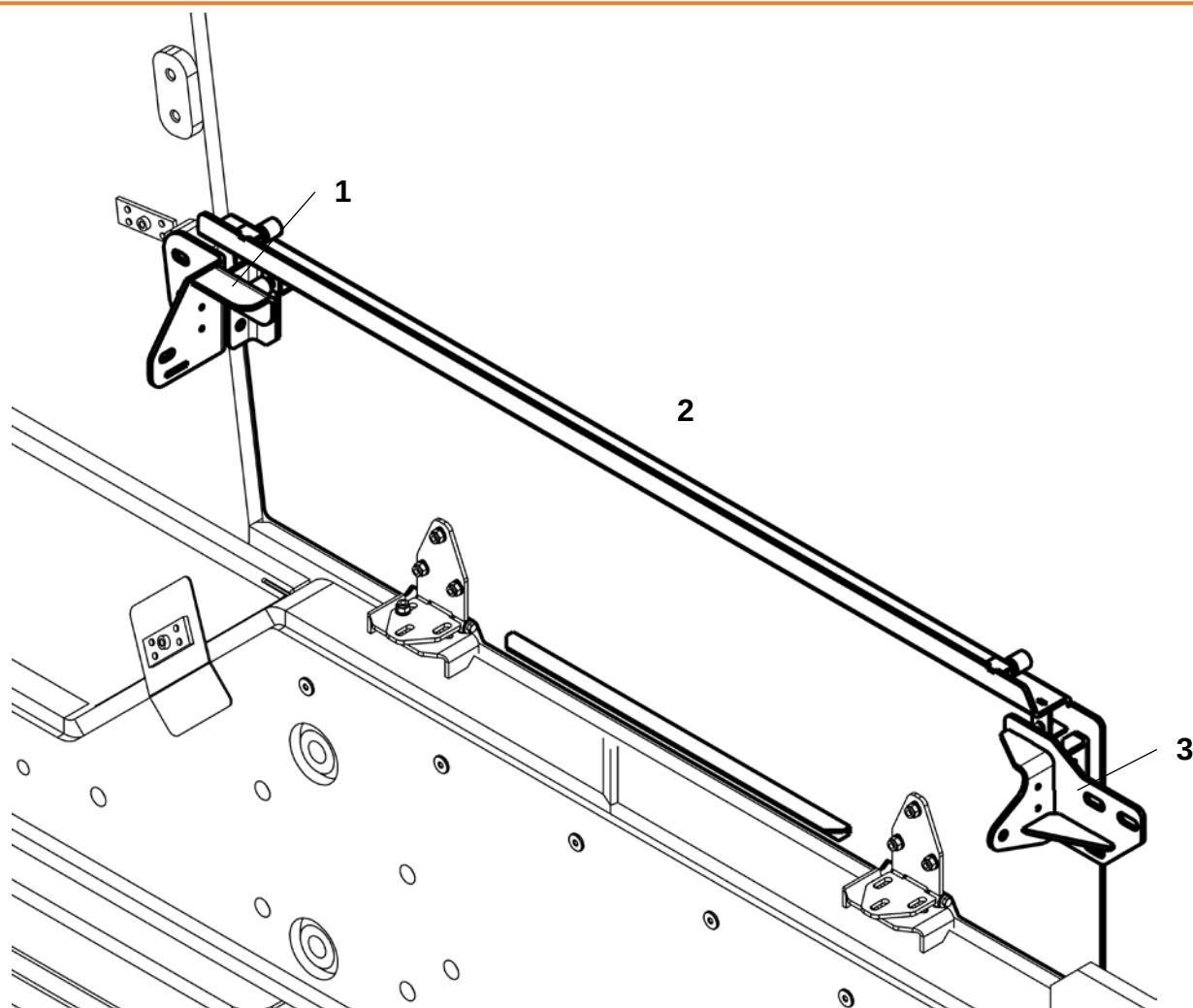
Крепление щита
