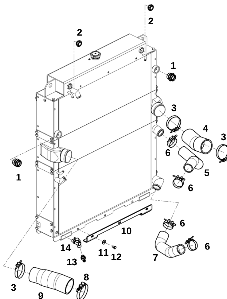
Блок радиатора в сборе (Cummins QSL 8.9)
