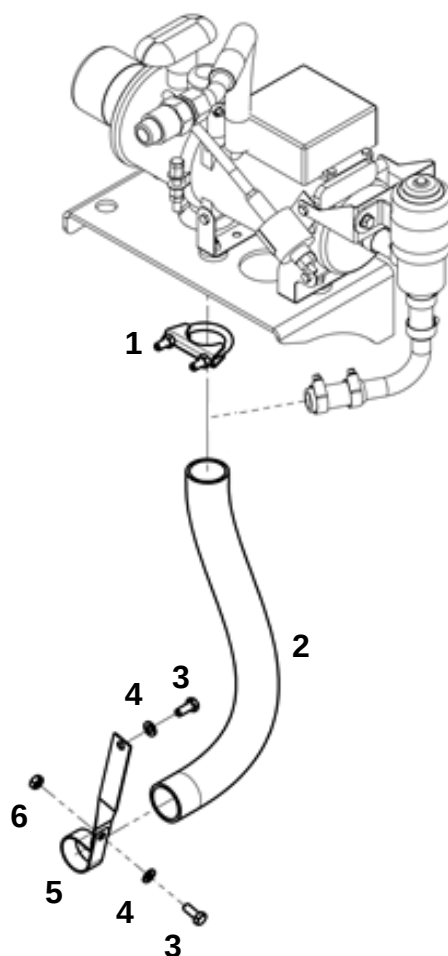
Предпусковой жидкостный подогреватель (Cummins QSL8,9)
