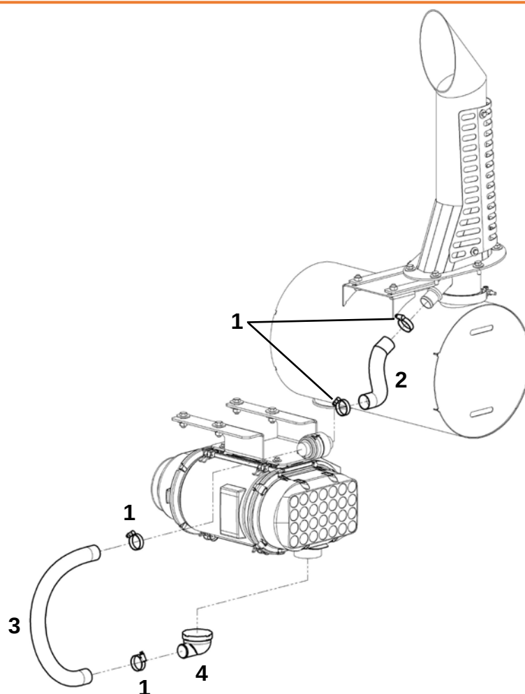
Система инжекционной очистки воздуха (Cummins QSL 8.9)
