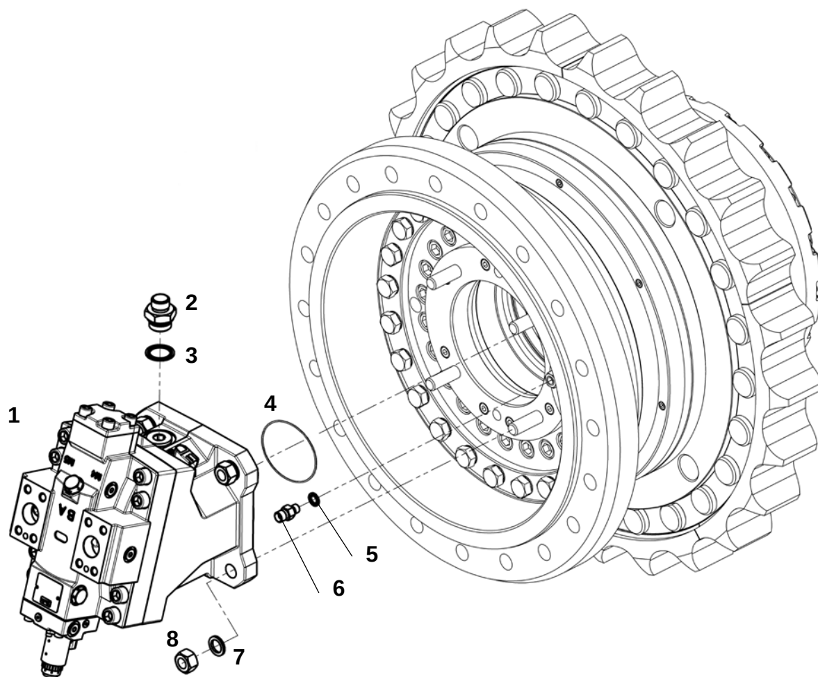
Комплект установки гидромотора
