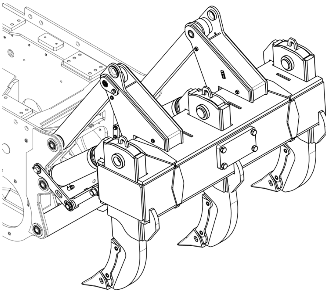
Рыхлитель трехзубый однокоординатный
