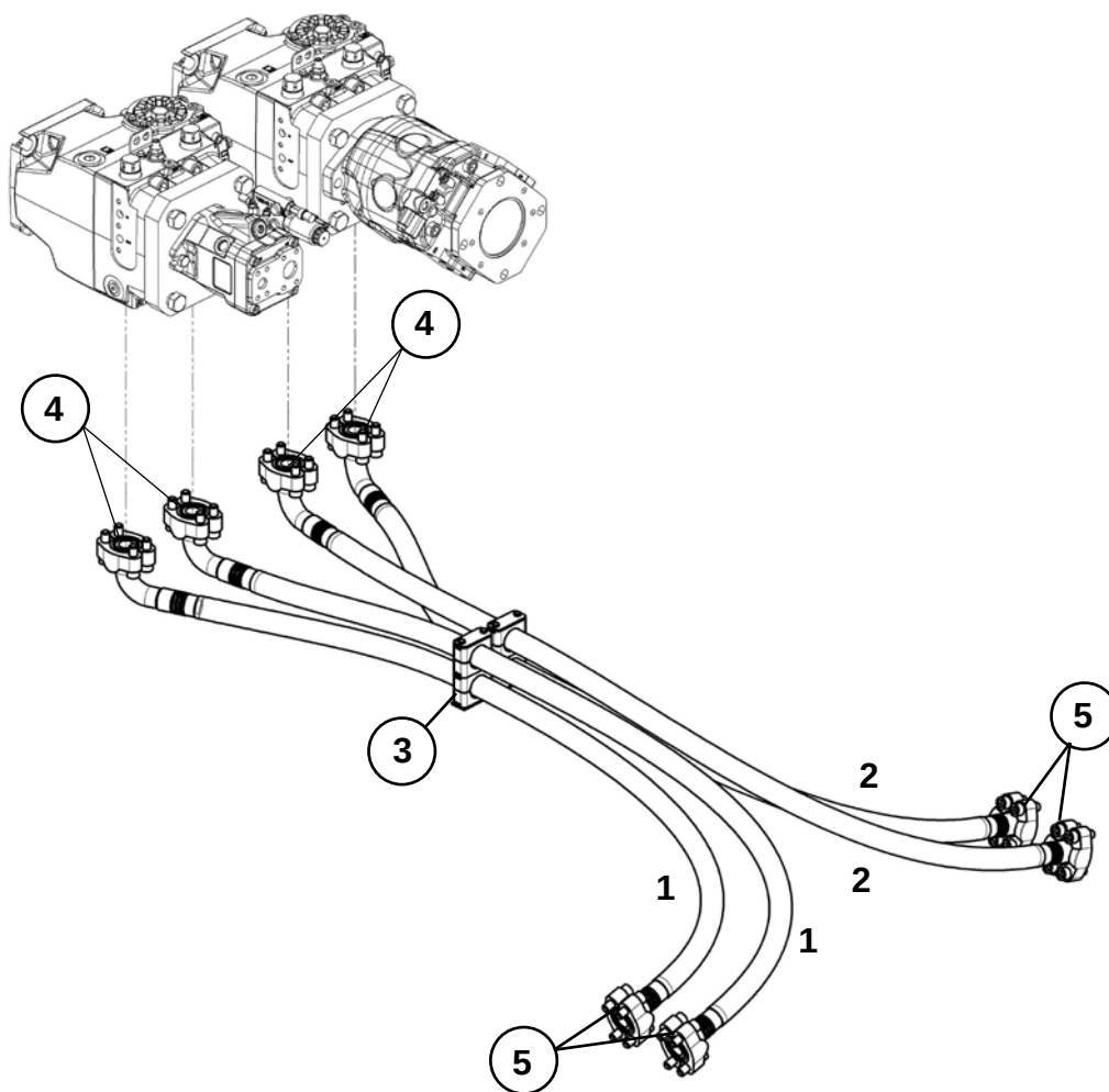
РВД трансмиссии (Н1-Р-147) (Болотное исполнение)
