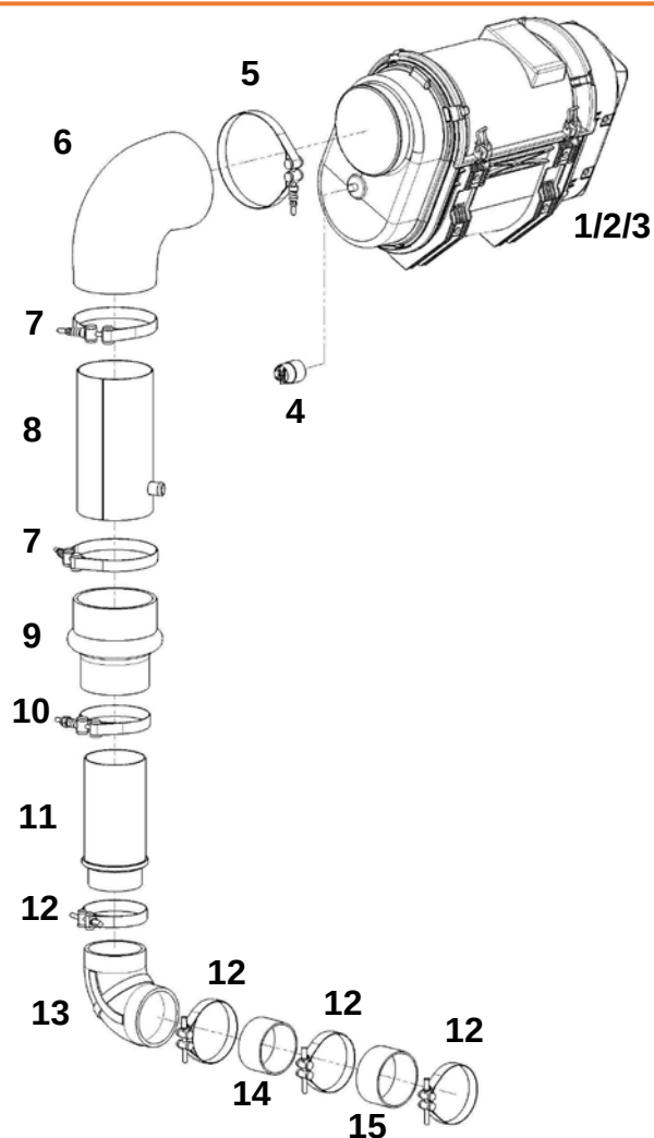
Впускной тракт (ЯМЗ-536)
