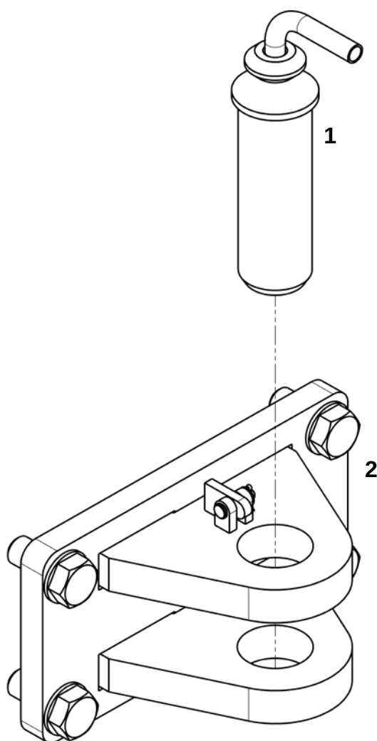
Установка жесткого прицепного устройства
