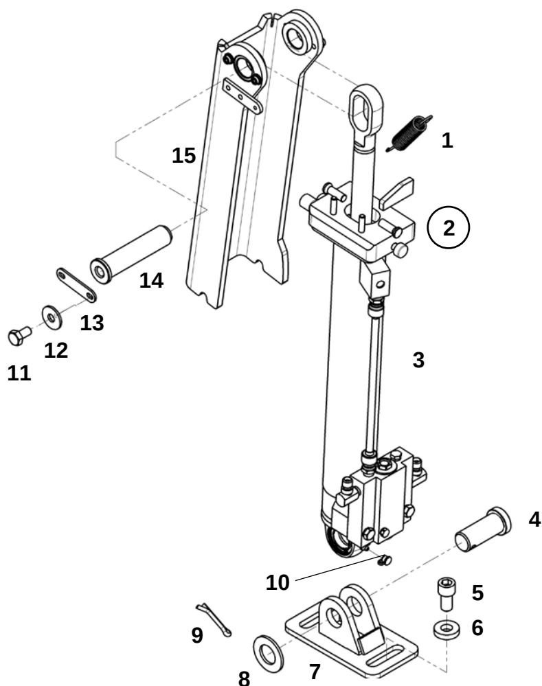
Гидроцилиндр с блокиратором
