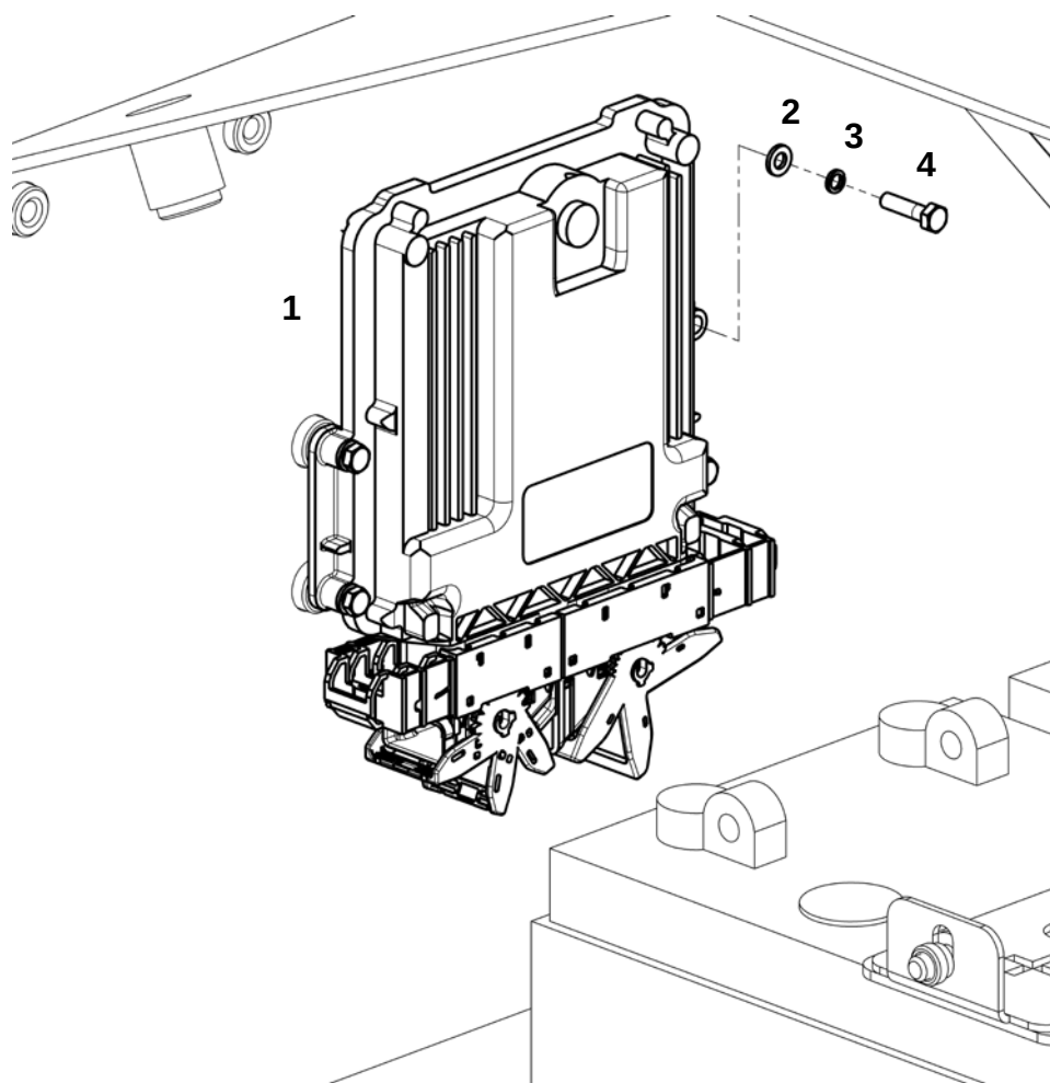
Установка контроллера ГСТ
