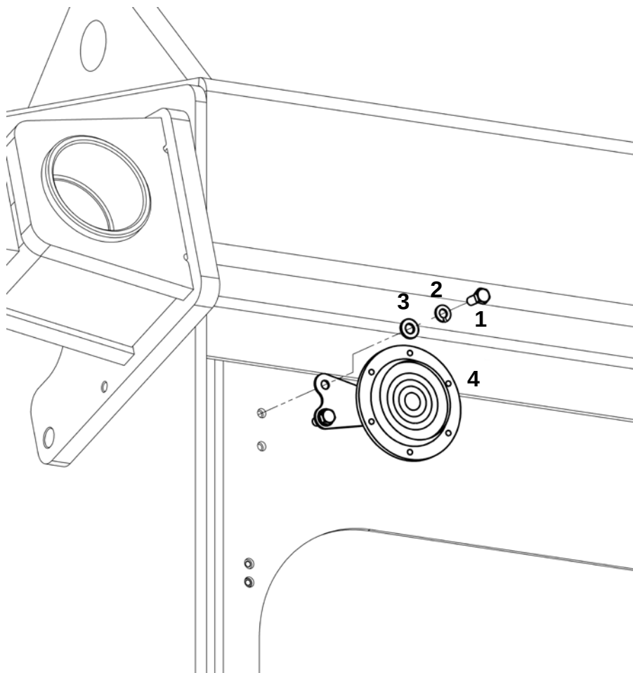
Установка звукового сигнала
