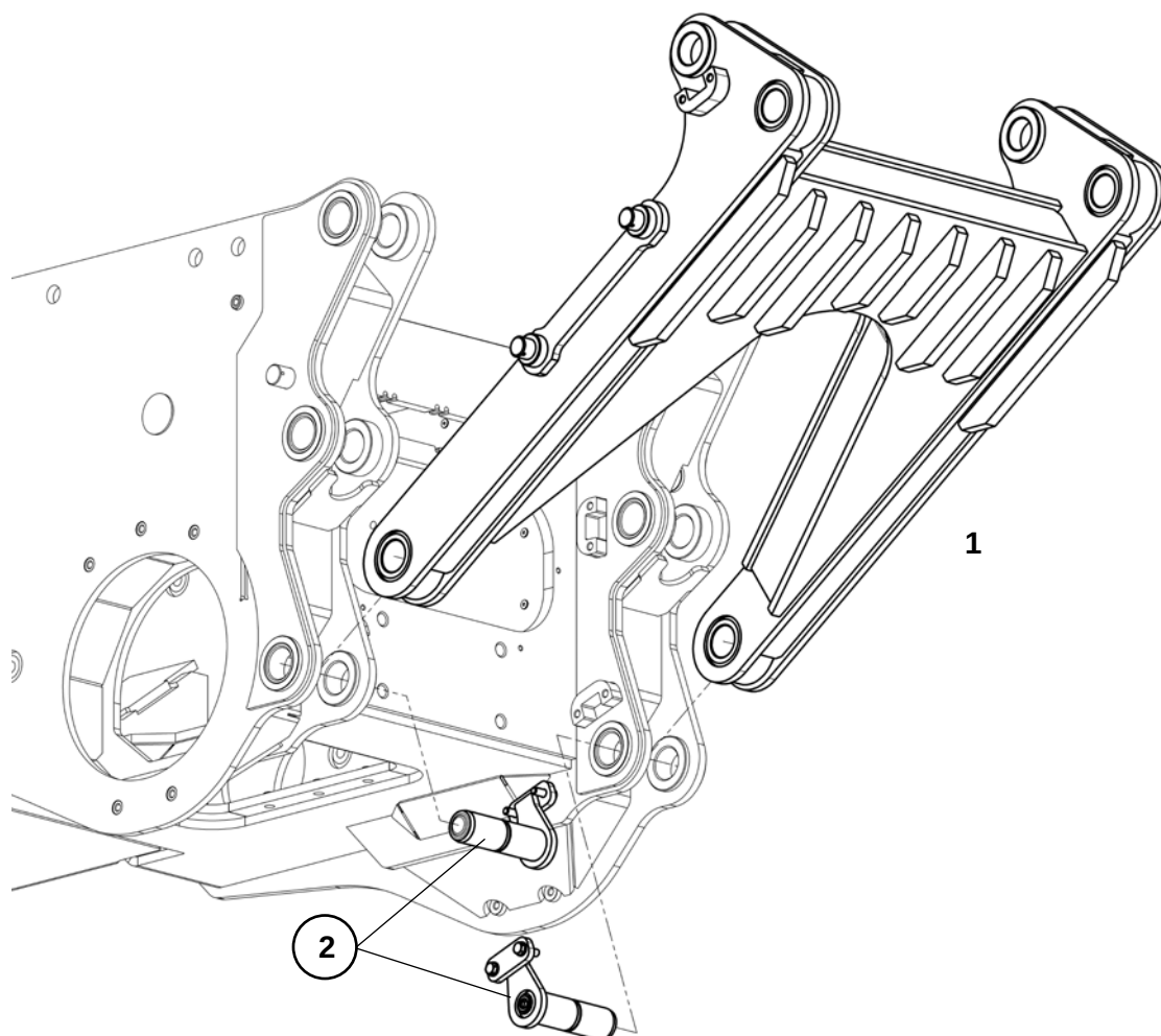
Крепление звена
