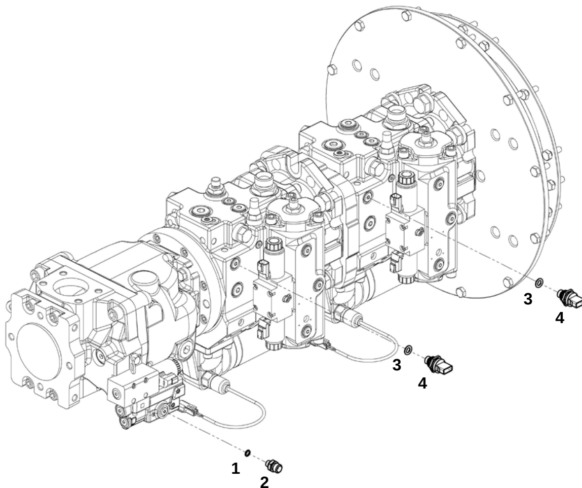
Комплект обвязки насосов гидравлических A4VG110, ERR100
