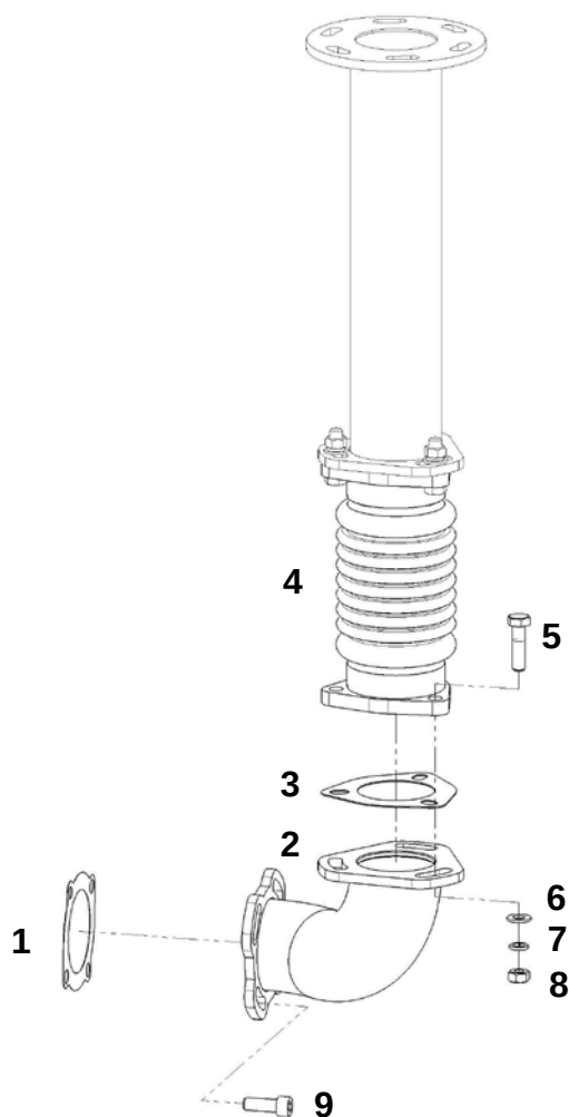
Воздухопровод выпускной (ЯМЗ-536)
