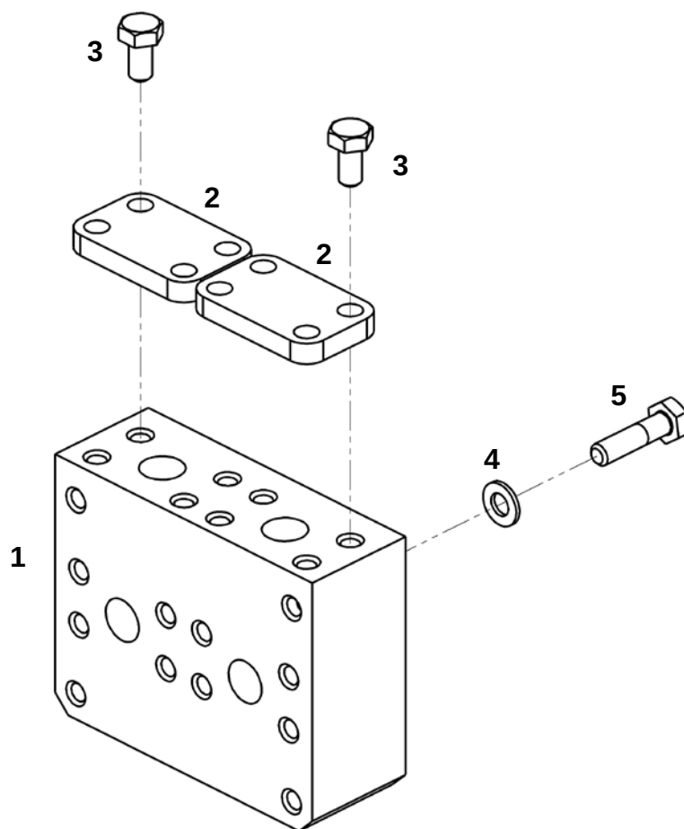
Плита переходная
