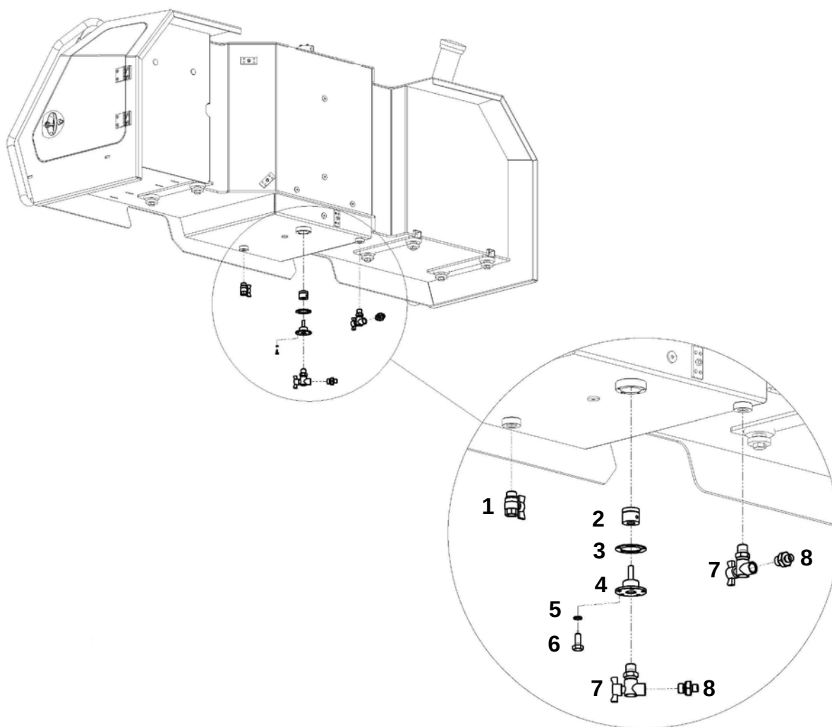
Топливный бак (ЯМЗ-536; Cummins QSL 8.9)
