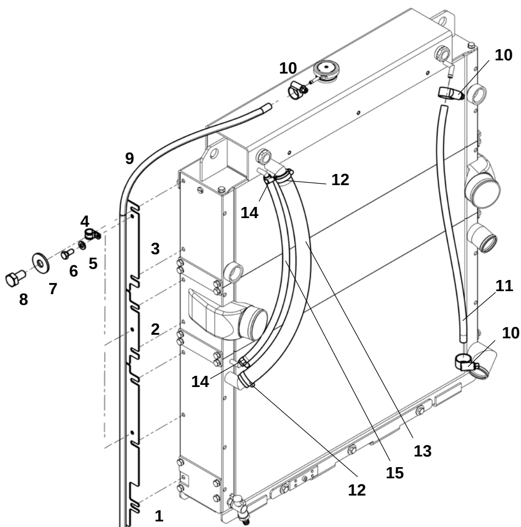
Рукава (Cummins QSL 8.9)
