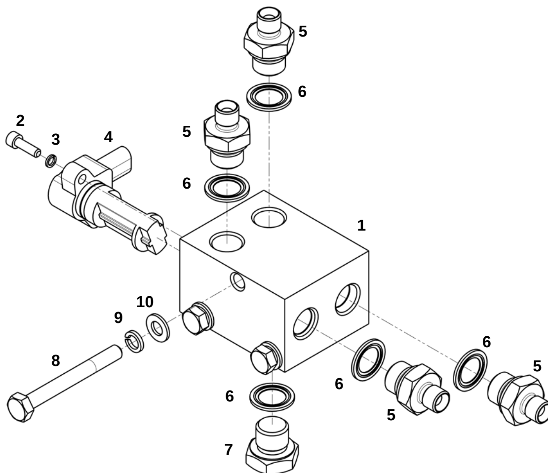
Плита в сборе (Cummins QSL 8.9)
