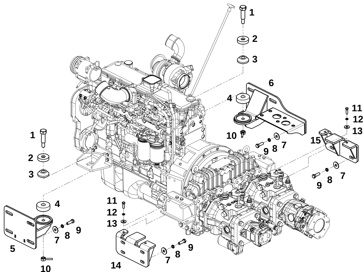
Силовой агрегат (Cummins QSL 8.9)
