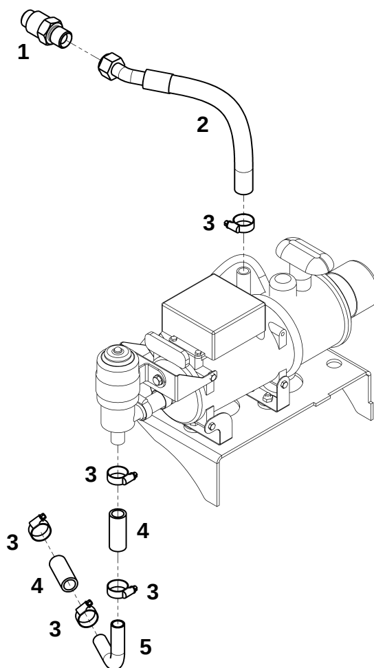
Предпусковой жидкостный подогреватель (Cummins QSL8,9)
