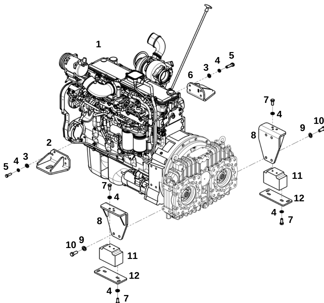
Двигатель с опорами
