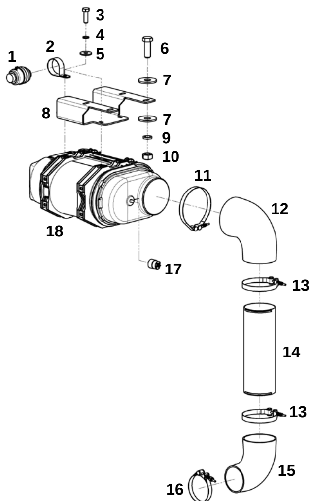
Впускной тракт (Cummins QSL 8.9)
