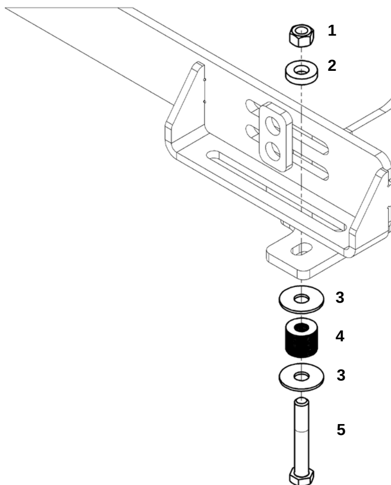
Крепление кронштейна (ЯМЗ-536)
