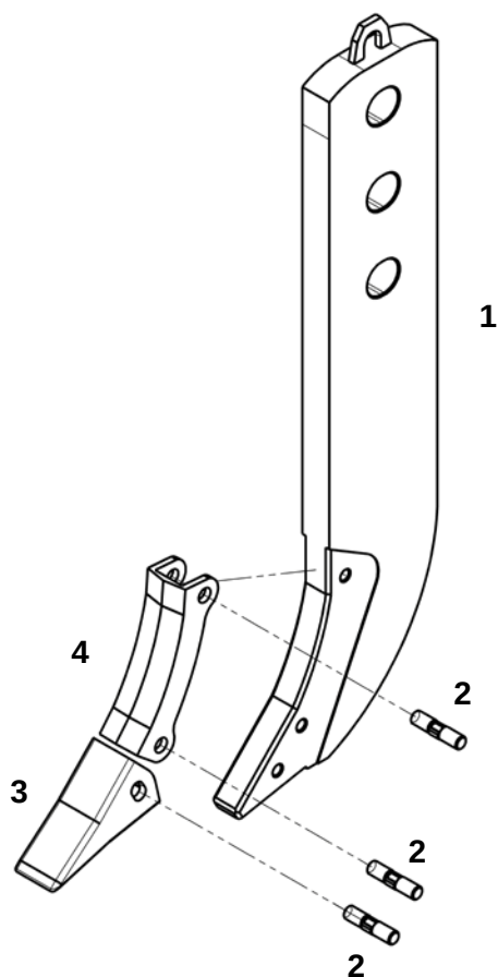
Нож в сборе
