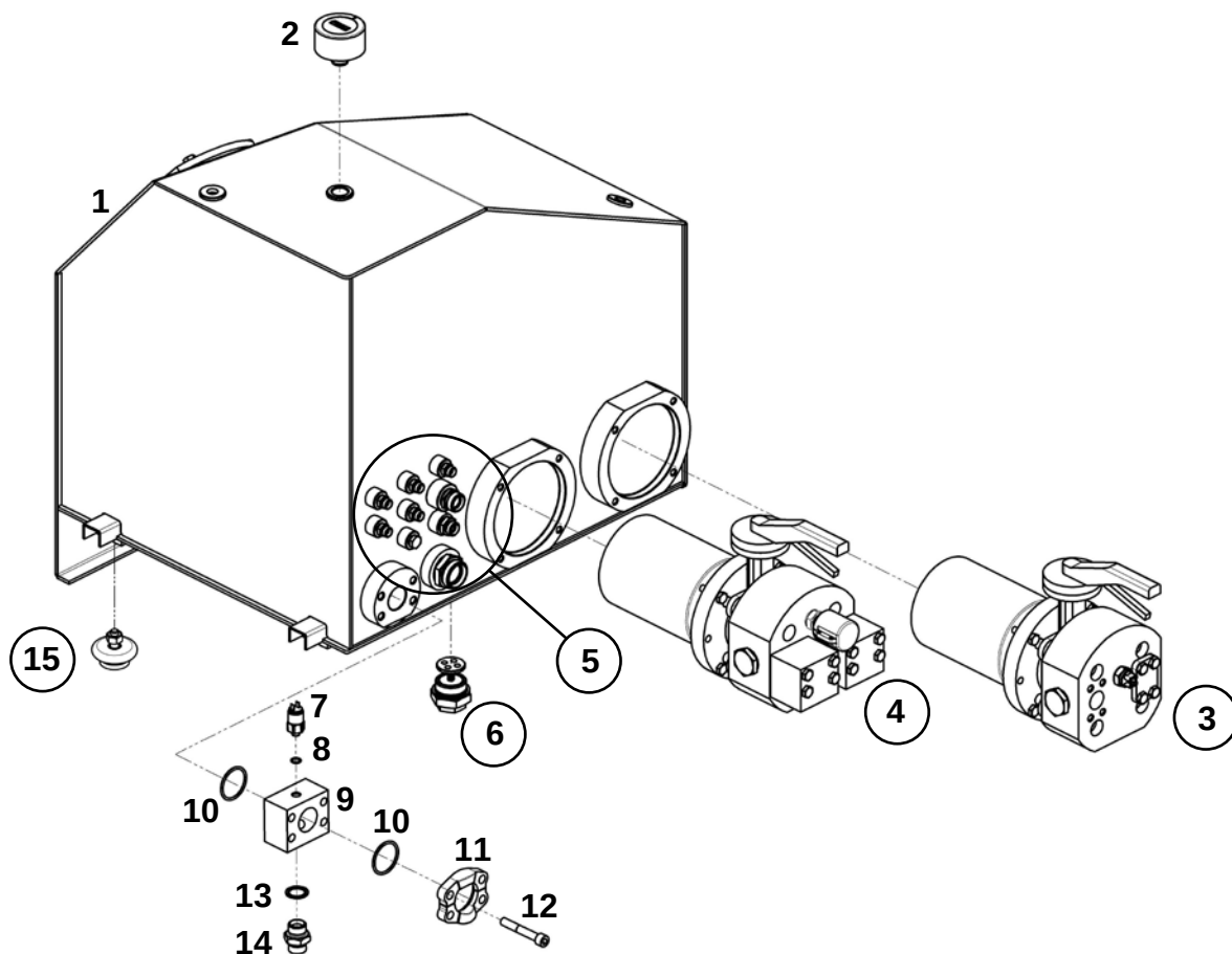
Бак гидравлический в сборе
