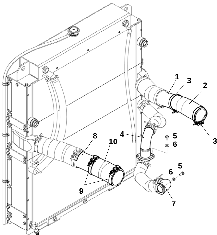
Рукава (Cummins QSL 8.9)
