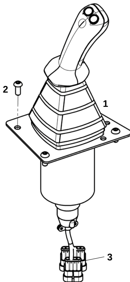
Установка джойстика движения
