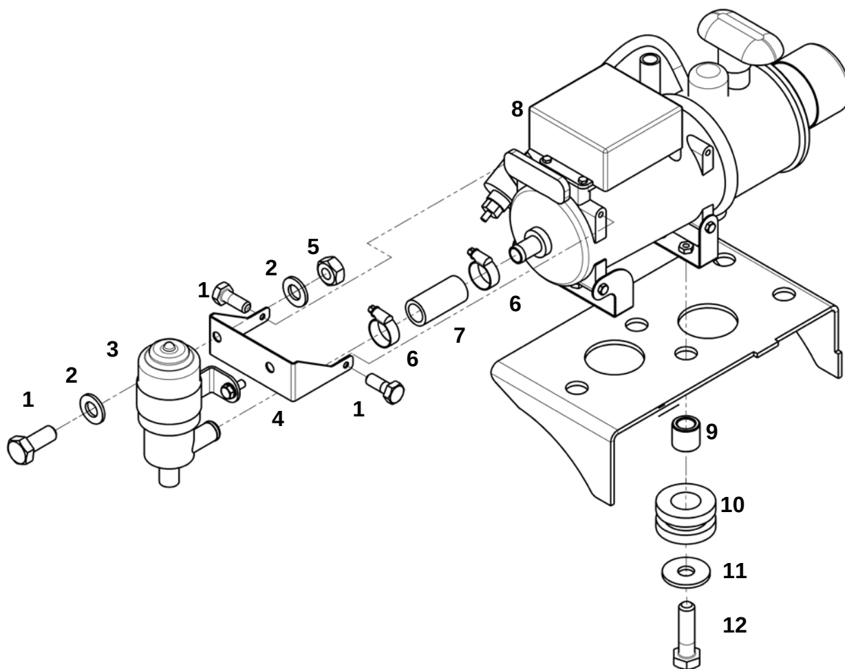
Предпусковой жидкостный подогреватель (ЯМЗ-536; Cummins QSL8,9)
