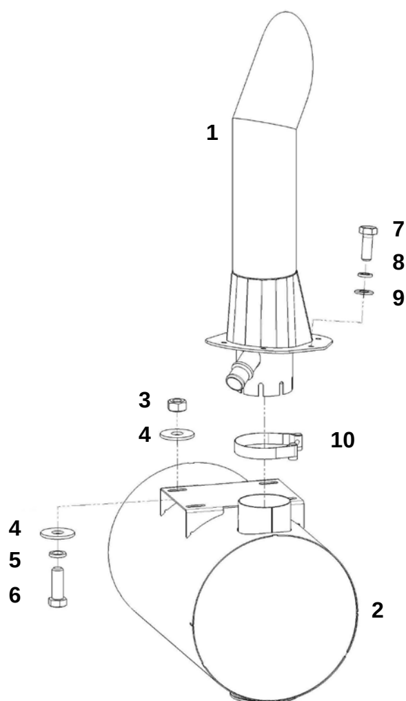
Труба выхлопная и глушитель (ЯМЗ-536)
