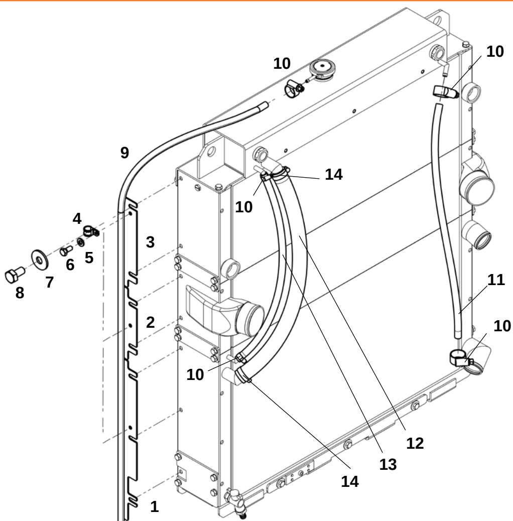
Рукава (ЯМЗ-536)
