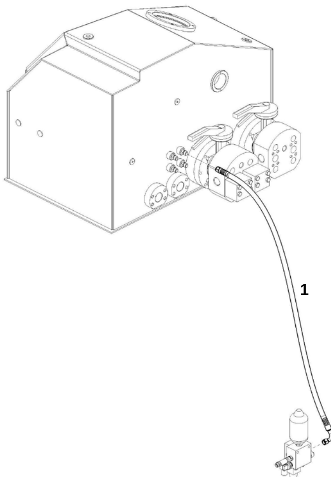
РВД слив с тормозной плиты в бак (A4VG145, A4VG110)
