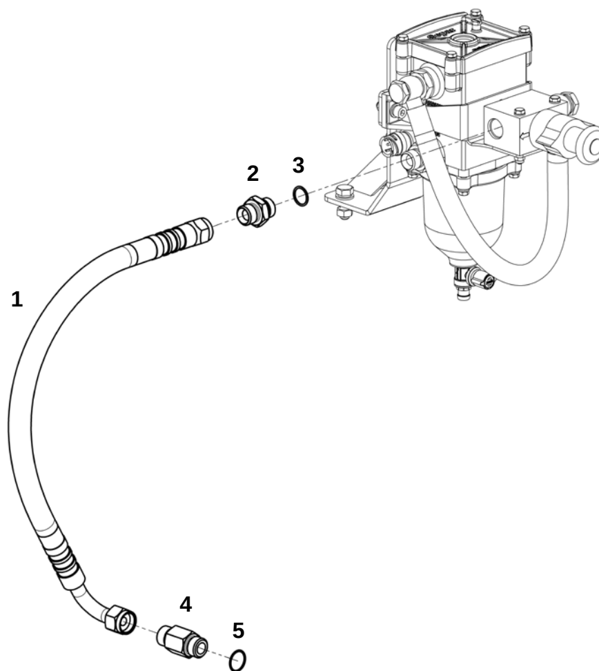
Топливопровод (Cummins QSL 8.9)
