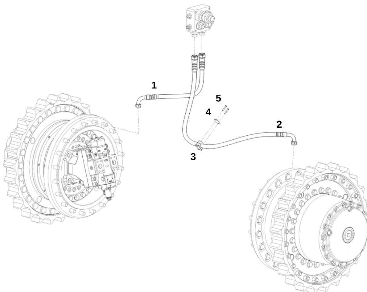
РВД дренажа гидромоторов (A6VE215)
