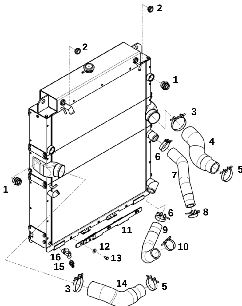
Блок радиаторов в сборе (ЯМЗ-536)
