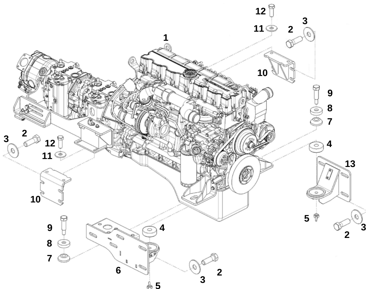
Силовой агрегат (ЯМЗ-536)
