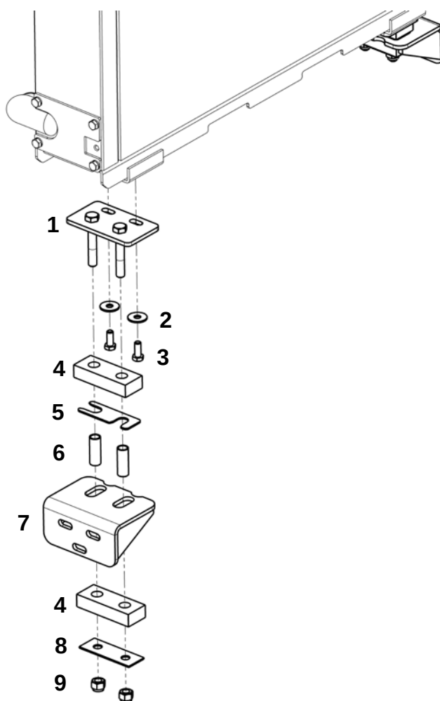
Комплект установки опор радиатора
