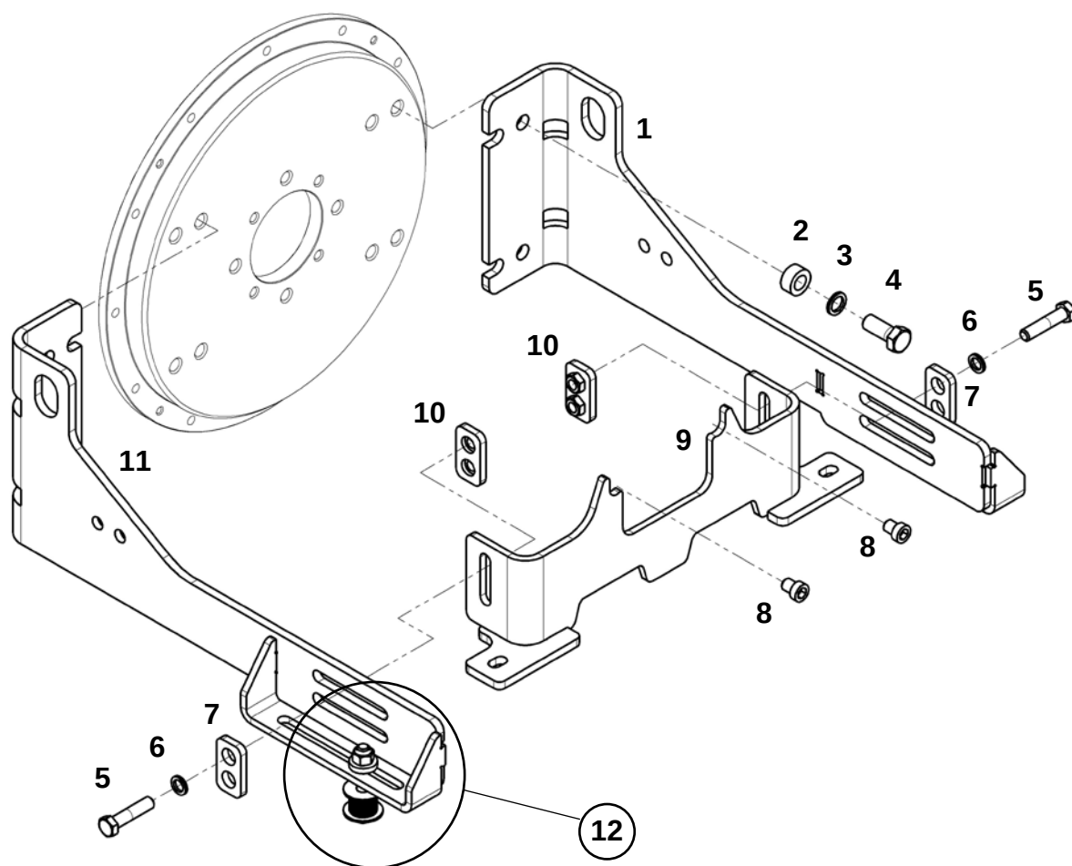
Подвес в сборе (ЯМЗ-536)
