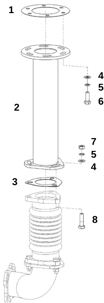
Воздухопровод выпускной (ЯМЗ-536)
