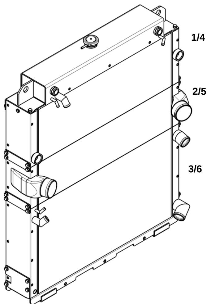
Сегменты блока радиаторов
