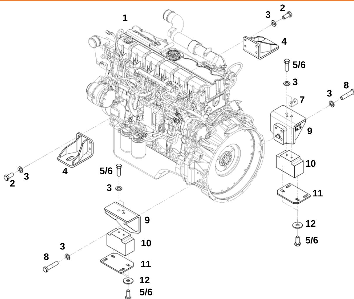
Двигатель с опорами
