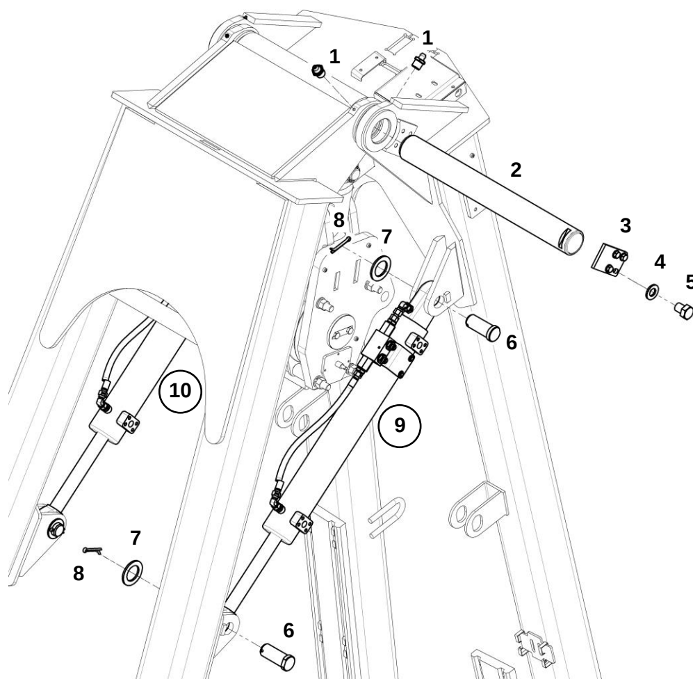
Стрела-опора в сборе
