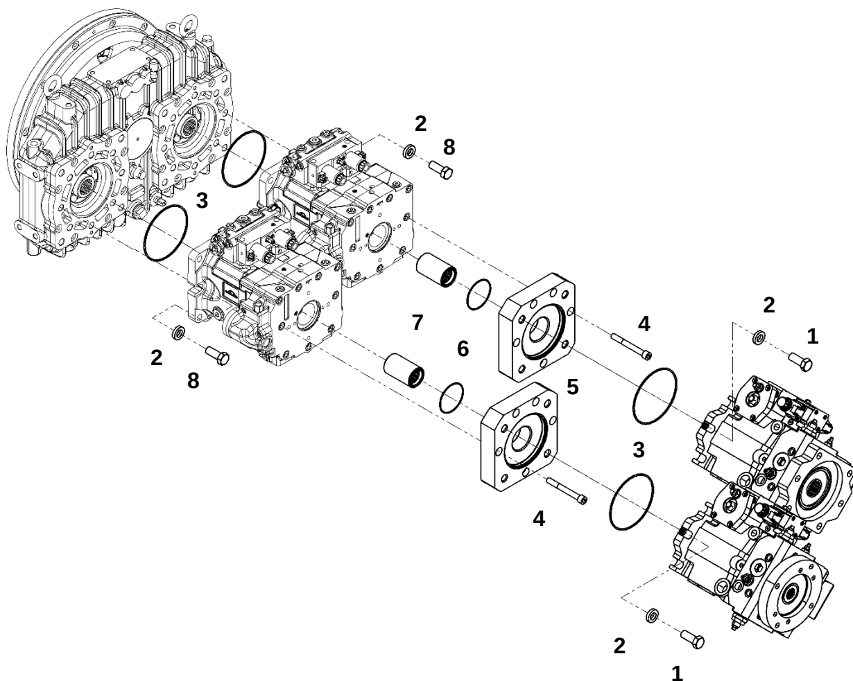
Силовой агрегат в сборе
