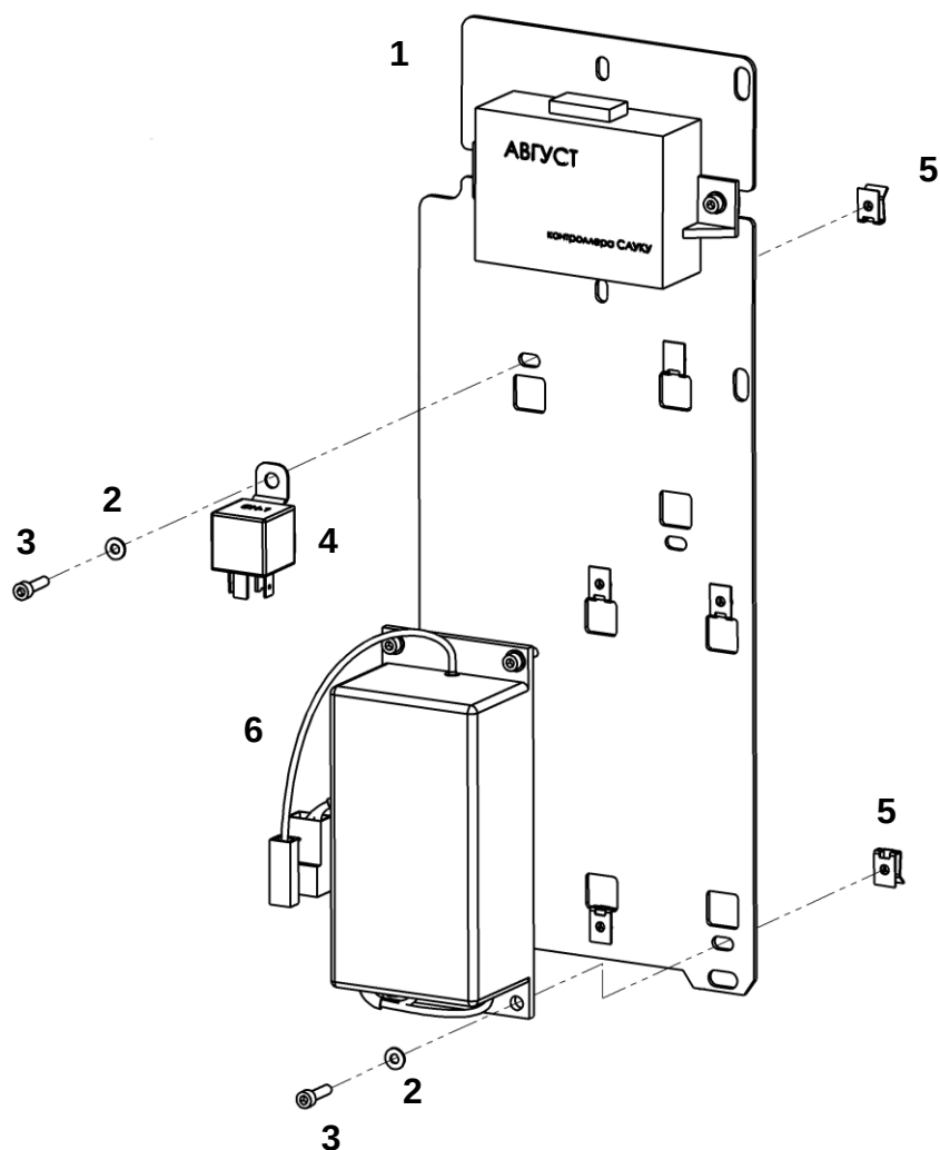
Панель в сборе
