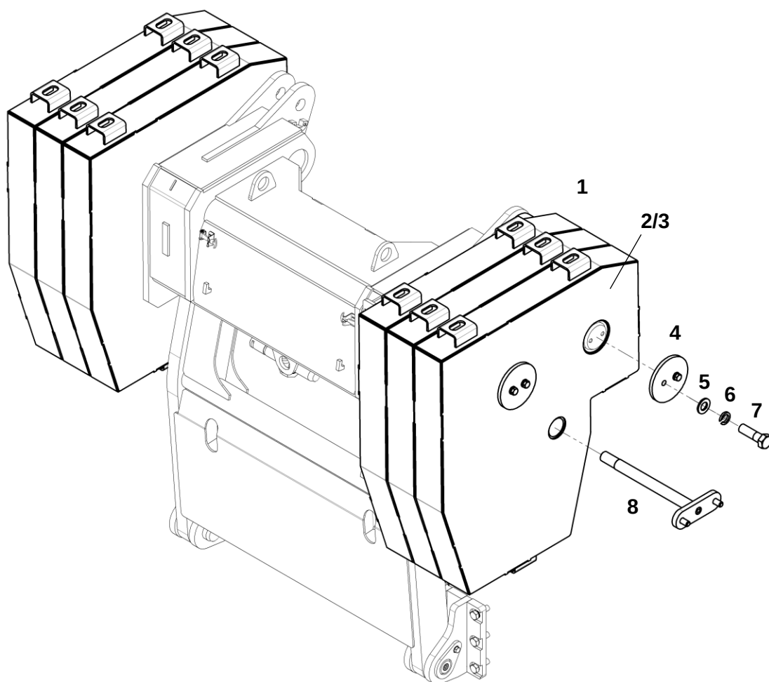
Контргруз в сборе
