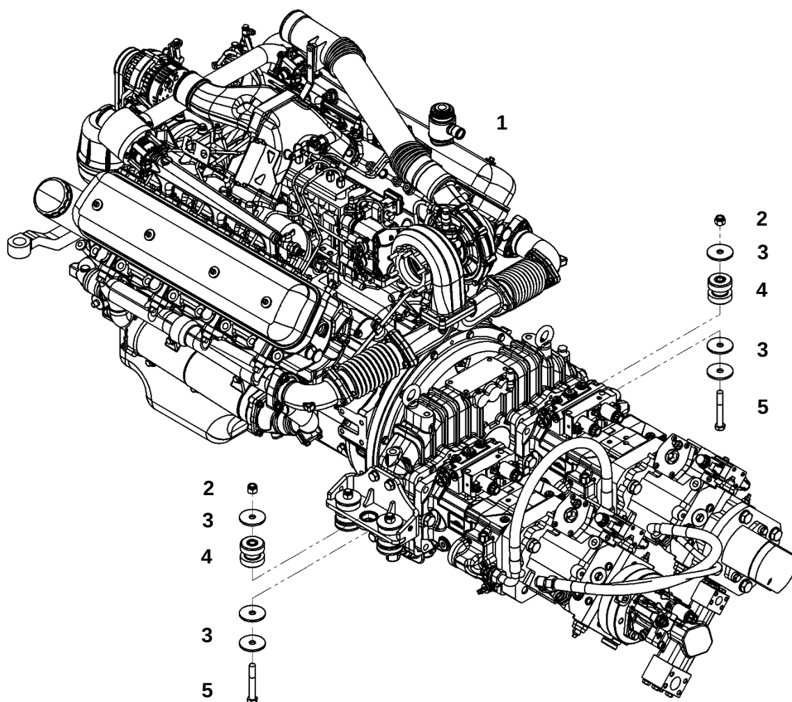
Установка силового агрегата
