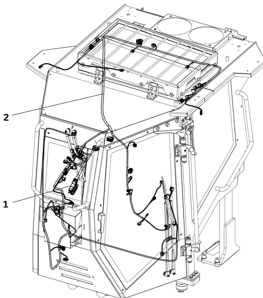
Электрооборудование кабины
