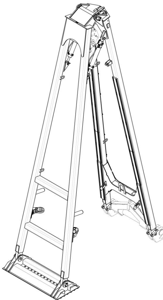
Стрела-опора в сборе
