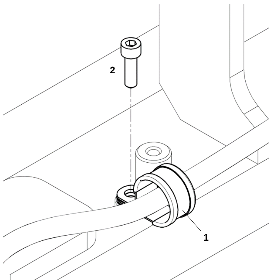
Крепление жгута
