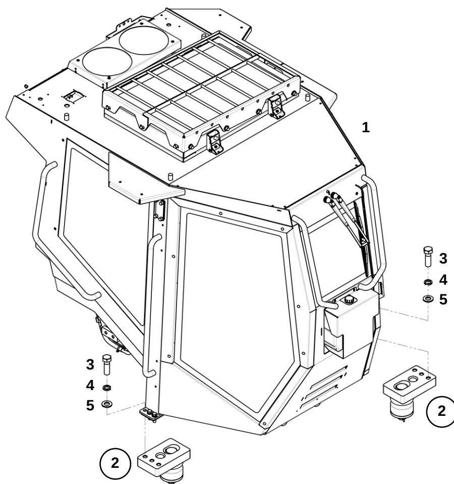
Кабина в сборе
