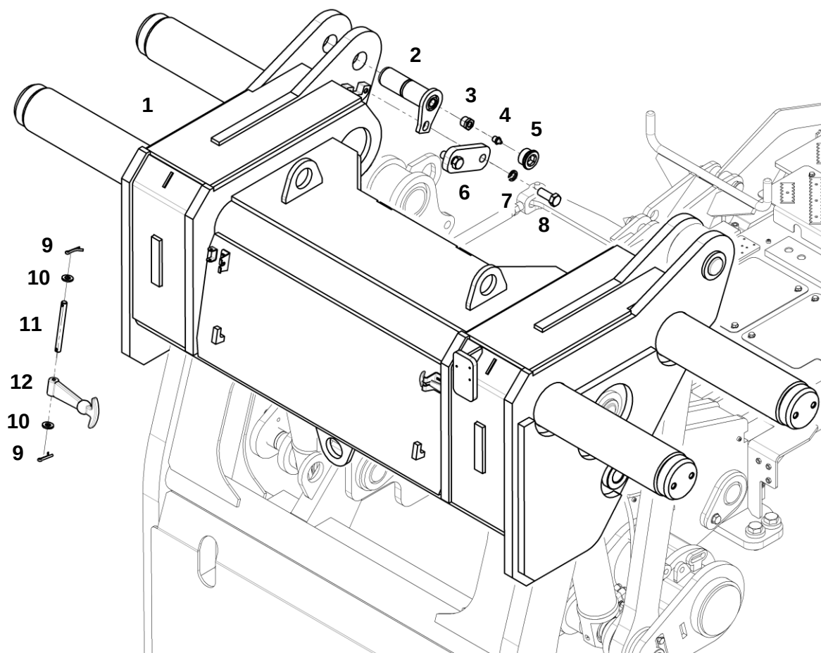
Контргруз в сборе
