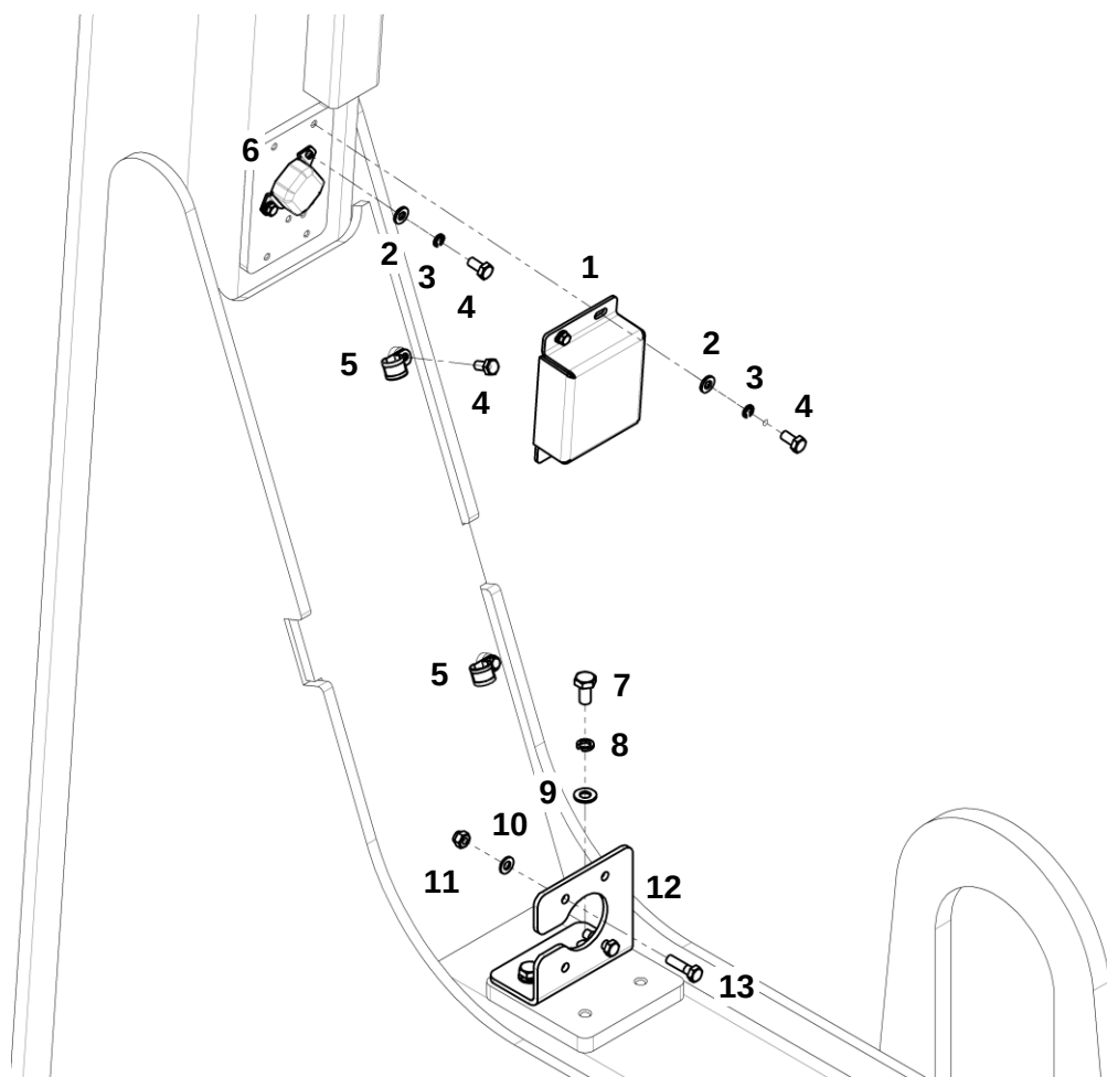
Датчики безопасности стрелы трубоукладчика
