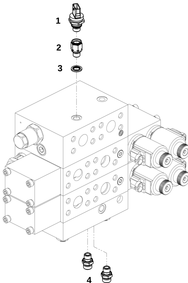
Гидрораспределитель в сборе
