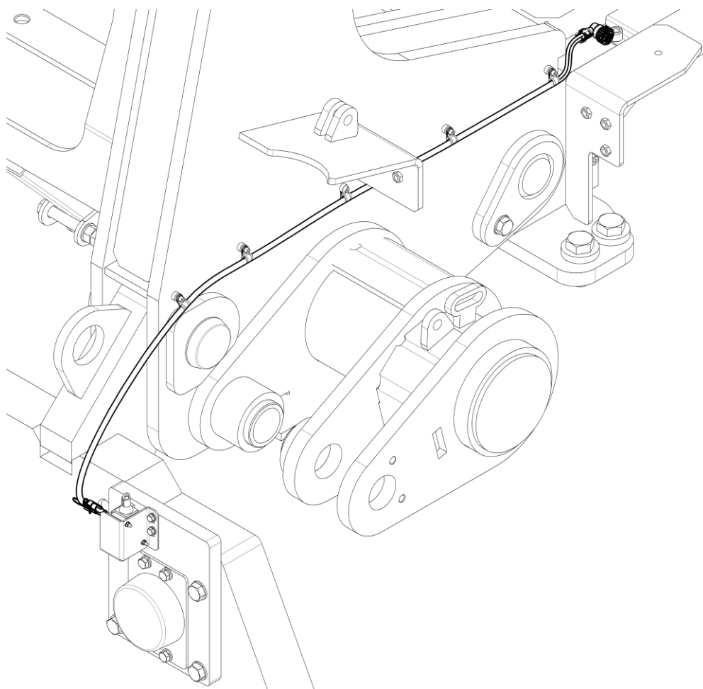
Система безопасности трубоукладчика
