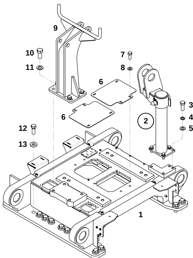
Элементы портала
