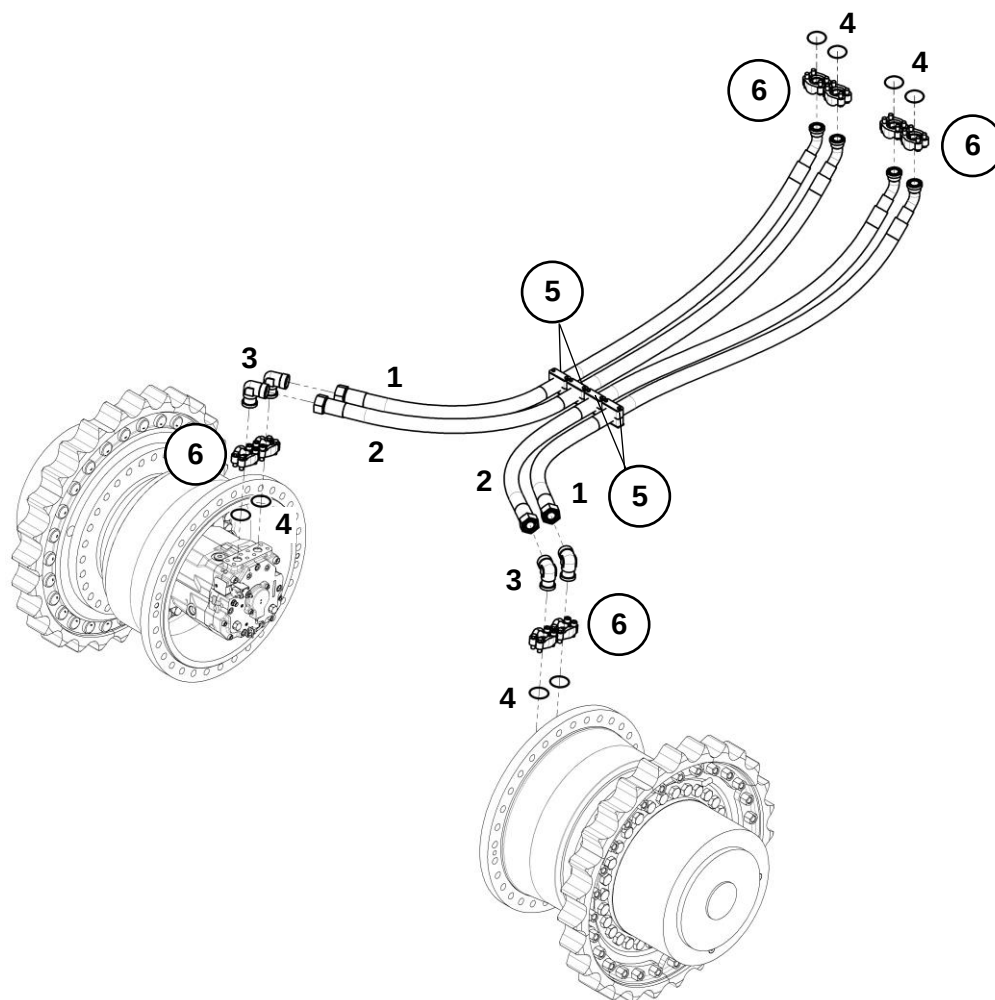
Трубопроводы гидросистемы трансмиссии
