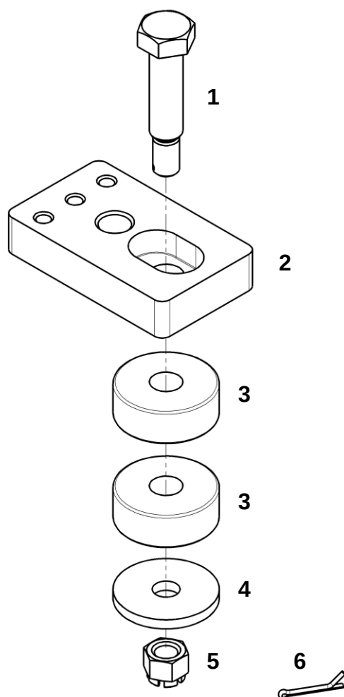
Опора кабины передняя
