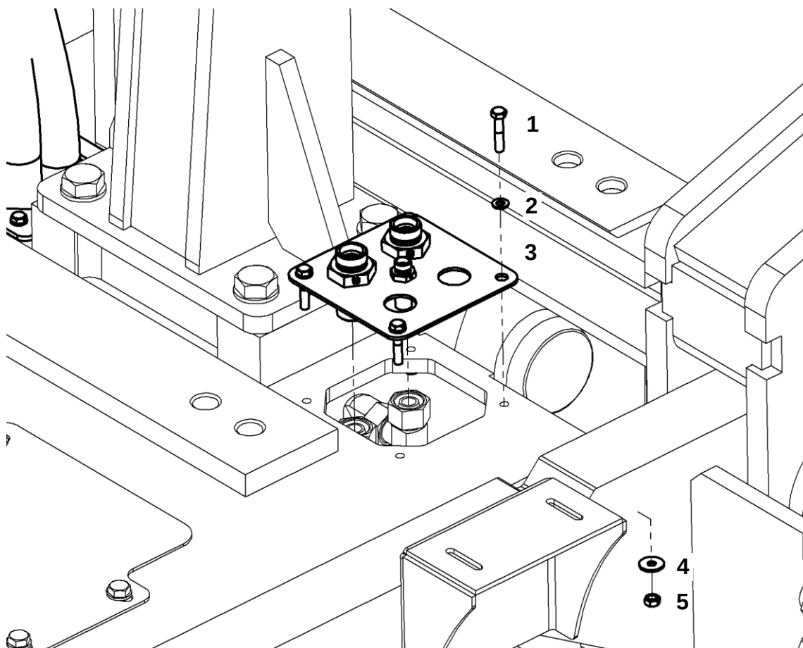
Трубопроводы гидросистемы навесного оборудования
