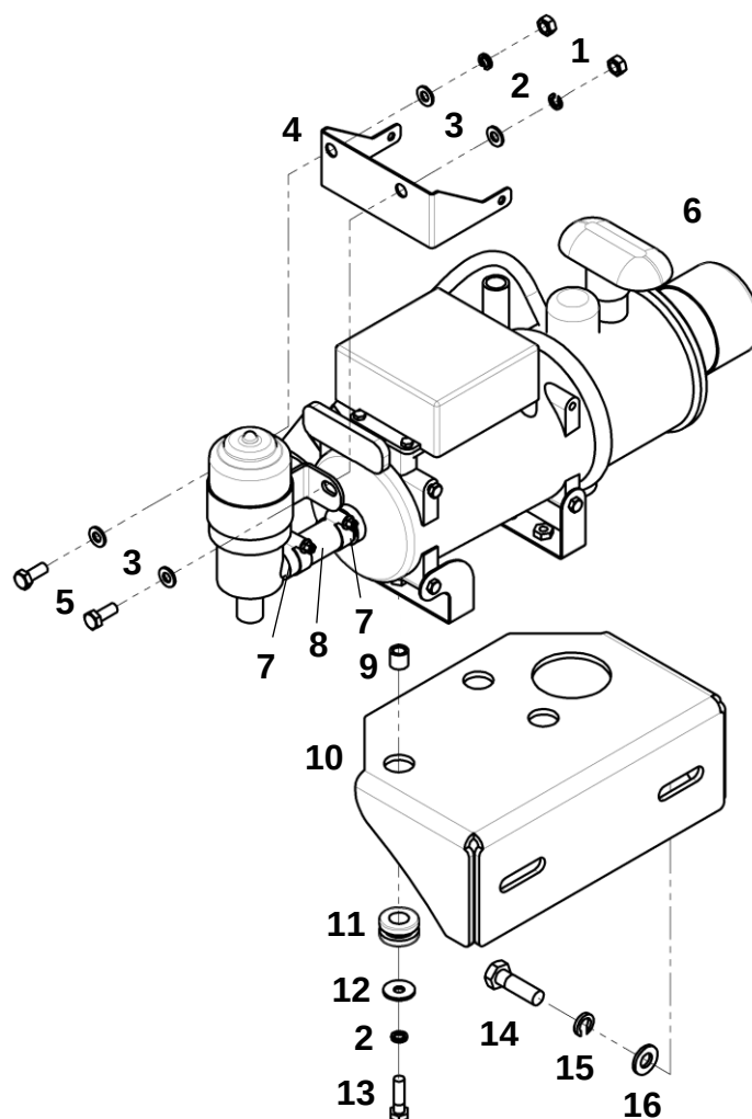
Система предпускового подогревателя
