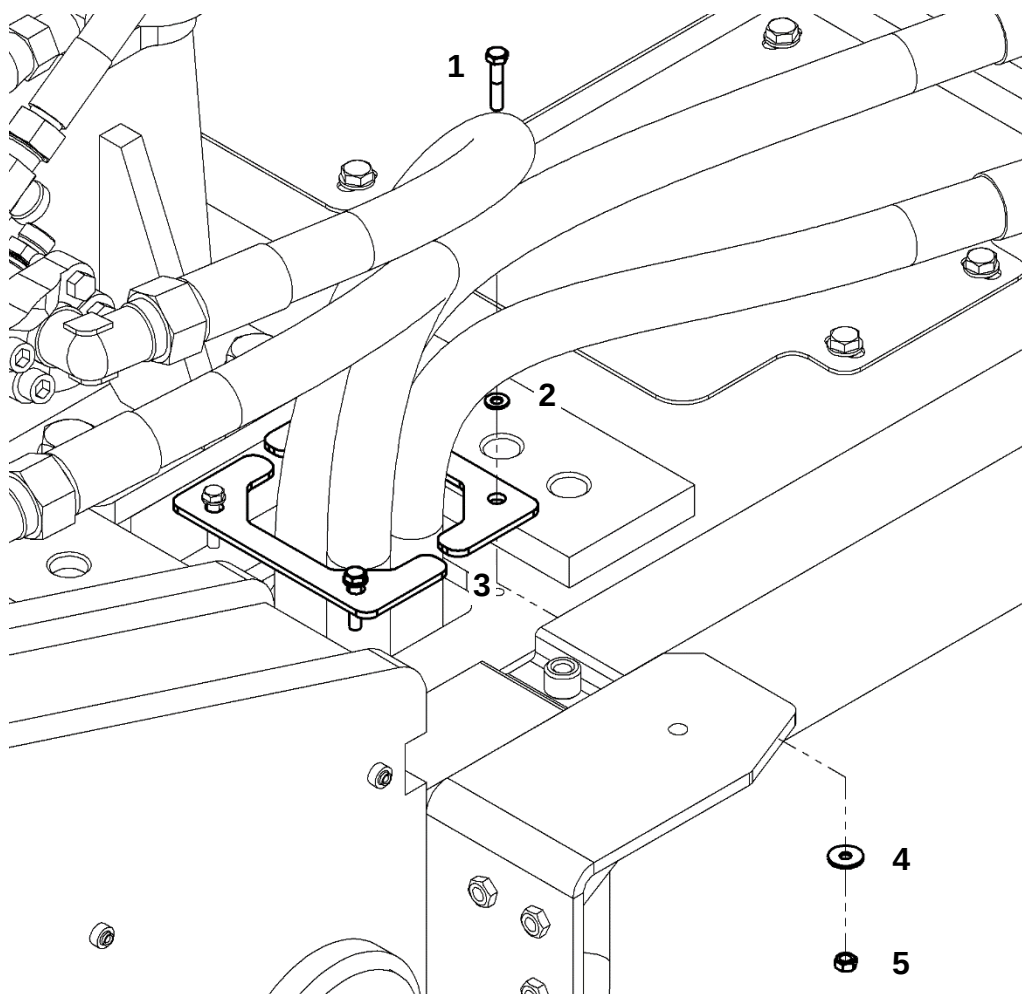
Трубопроводы гидросистемы навесного оборудования
