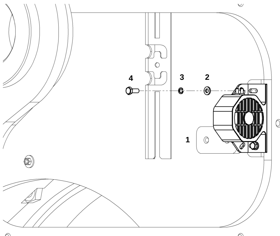
Сигнал движения задним ходом
