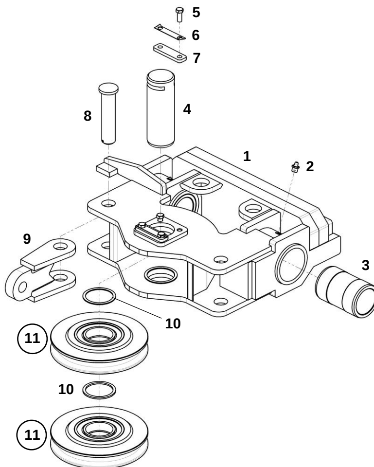
Блок лебедок
