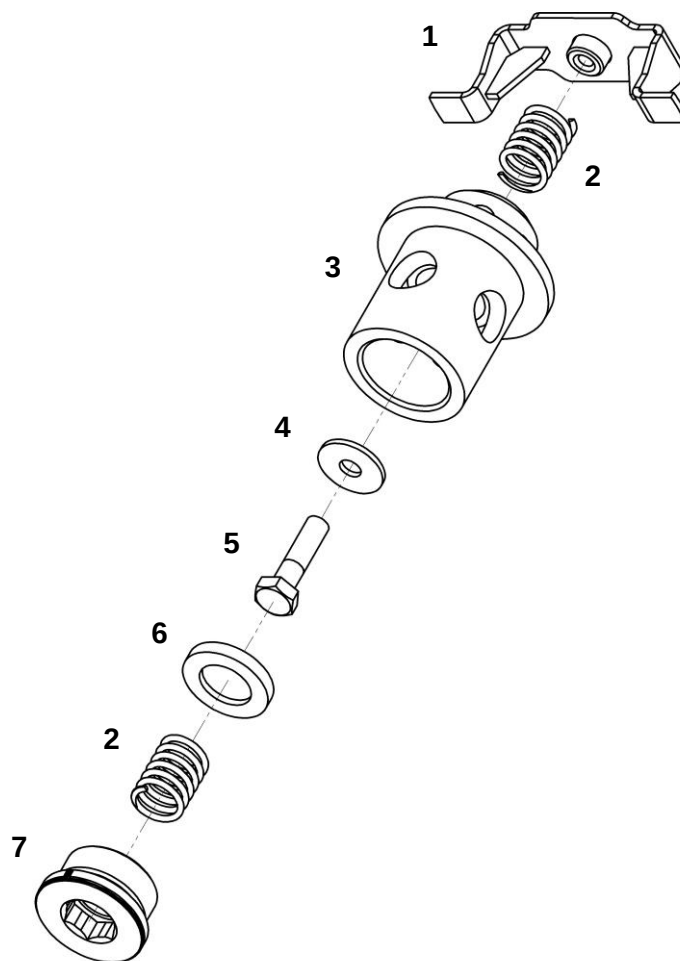
Клапан в сборе
