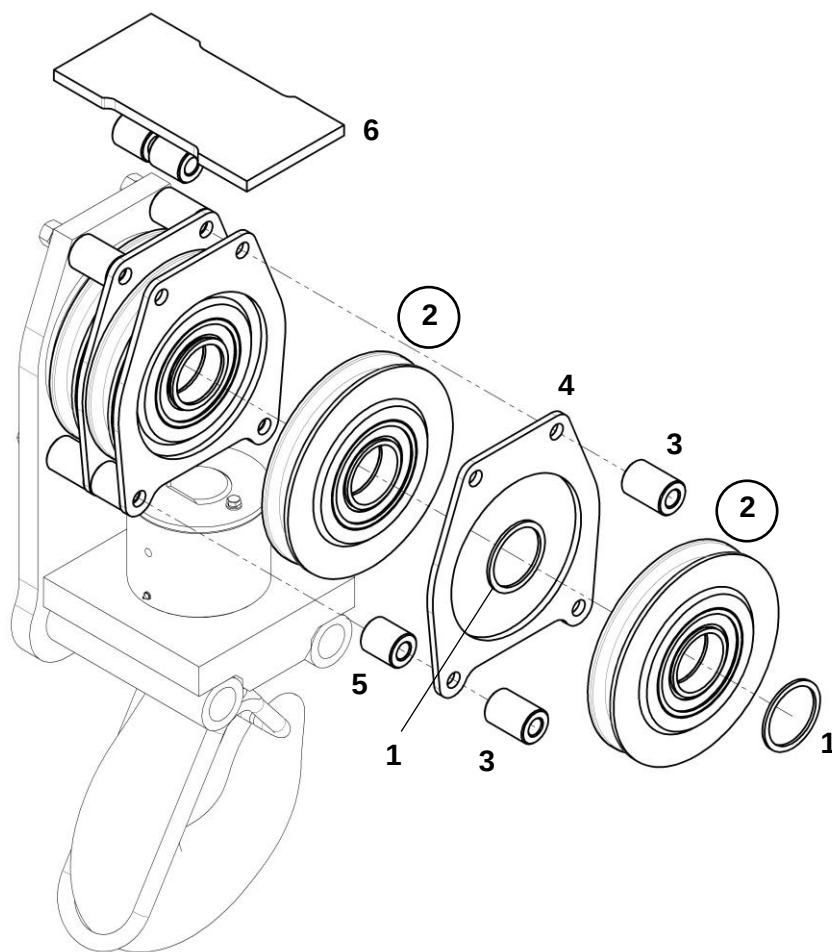
Блок подвижный
