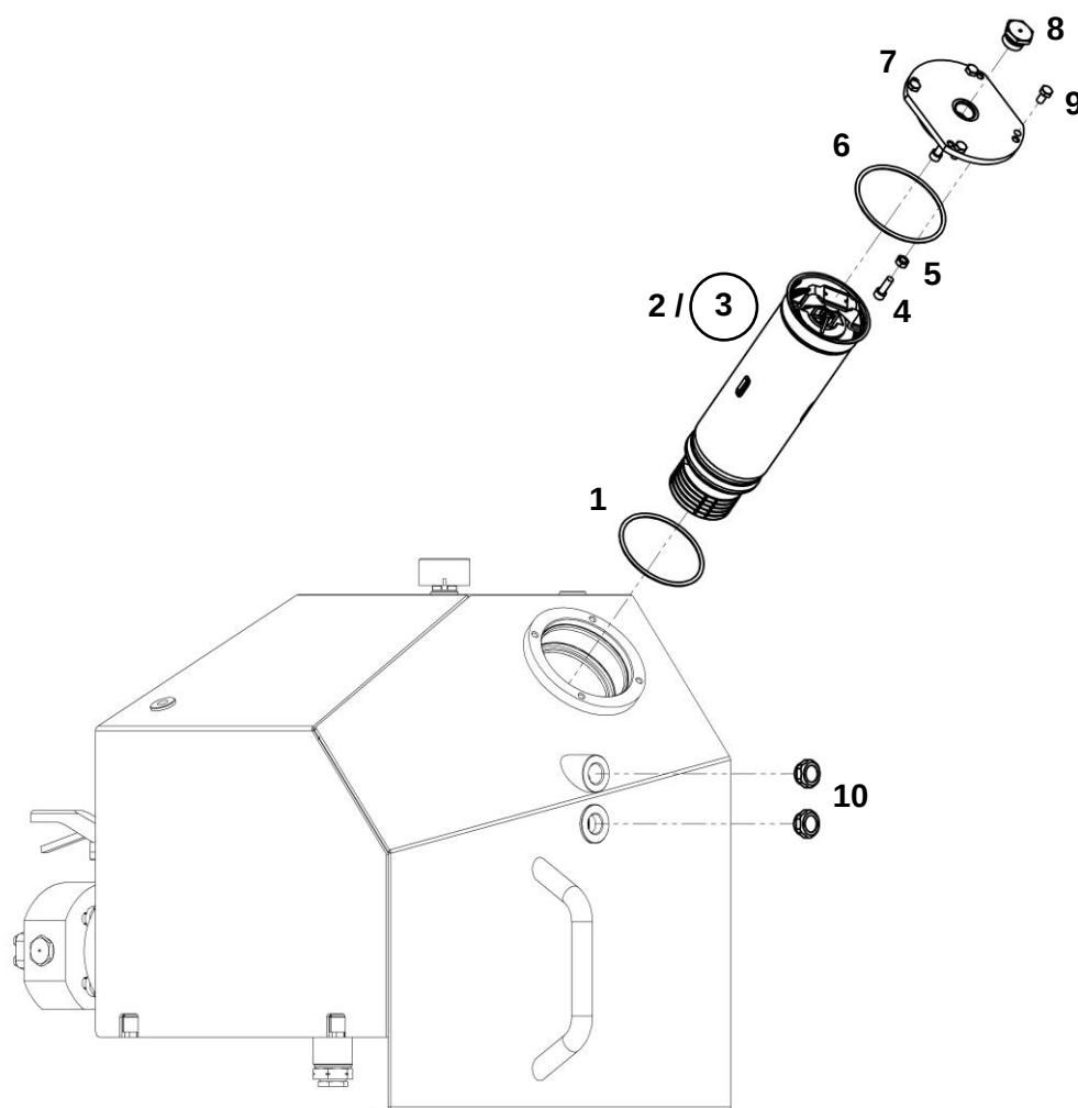
Бак гидравлический в сборе
