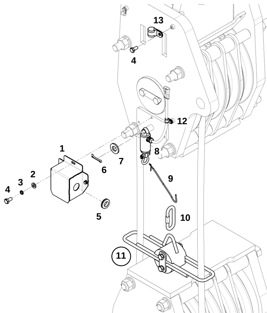
Датчик безопасности подвешенного блока
