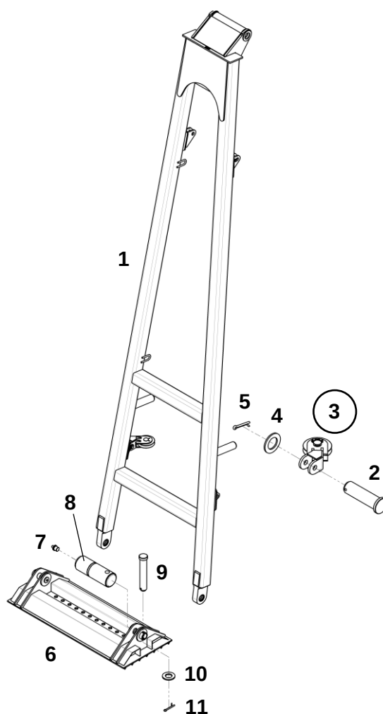
Стрела-опора в сборе
