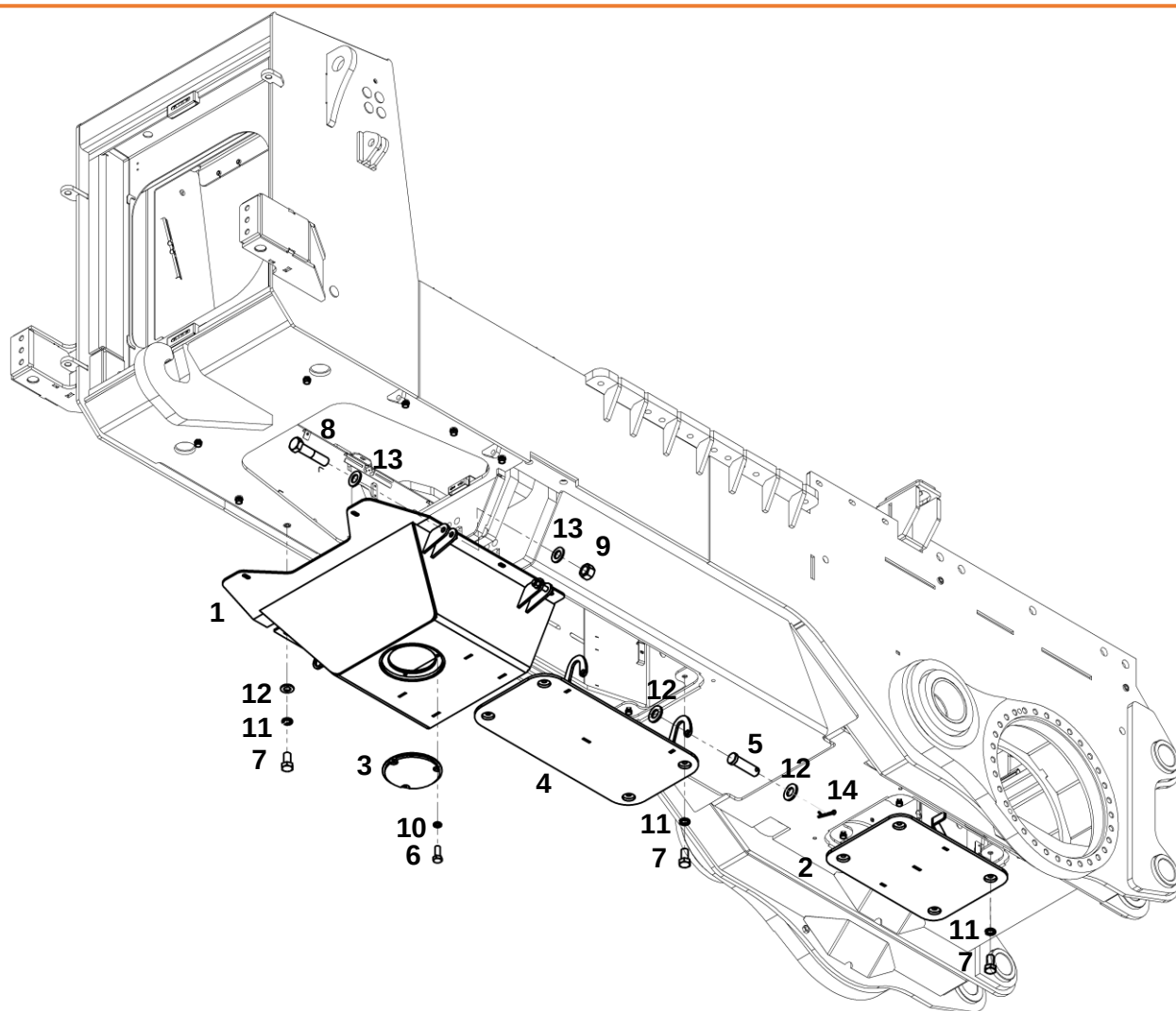
Броня в сборе
