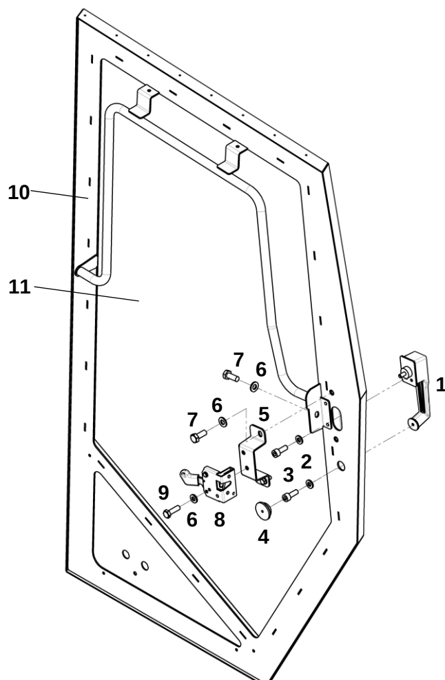
Дверь в сборе
