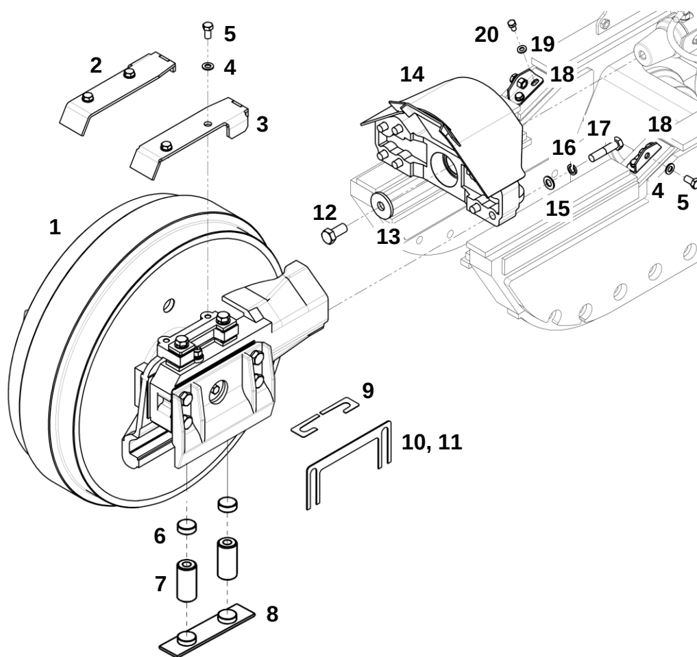
Тележка
