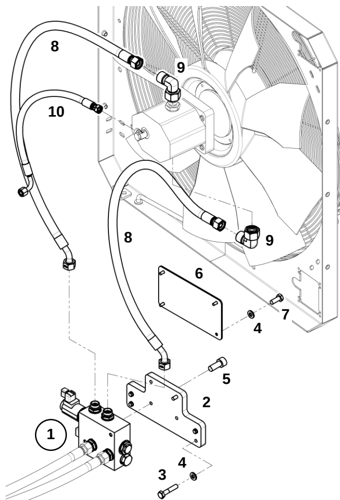
Гидропривод вентилятора
