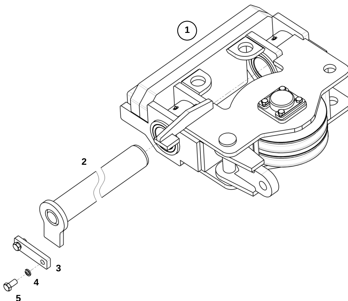
Блок лебедок
