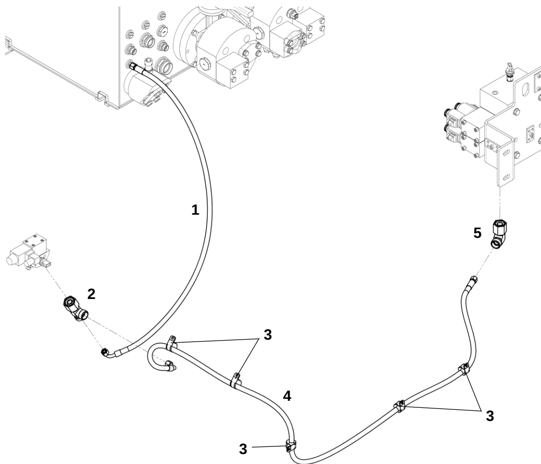
Трубопроводы гидросистемы трансмиссии
