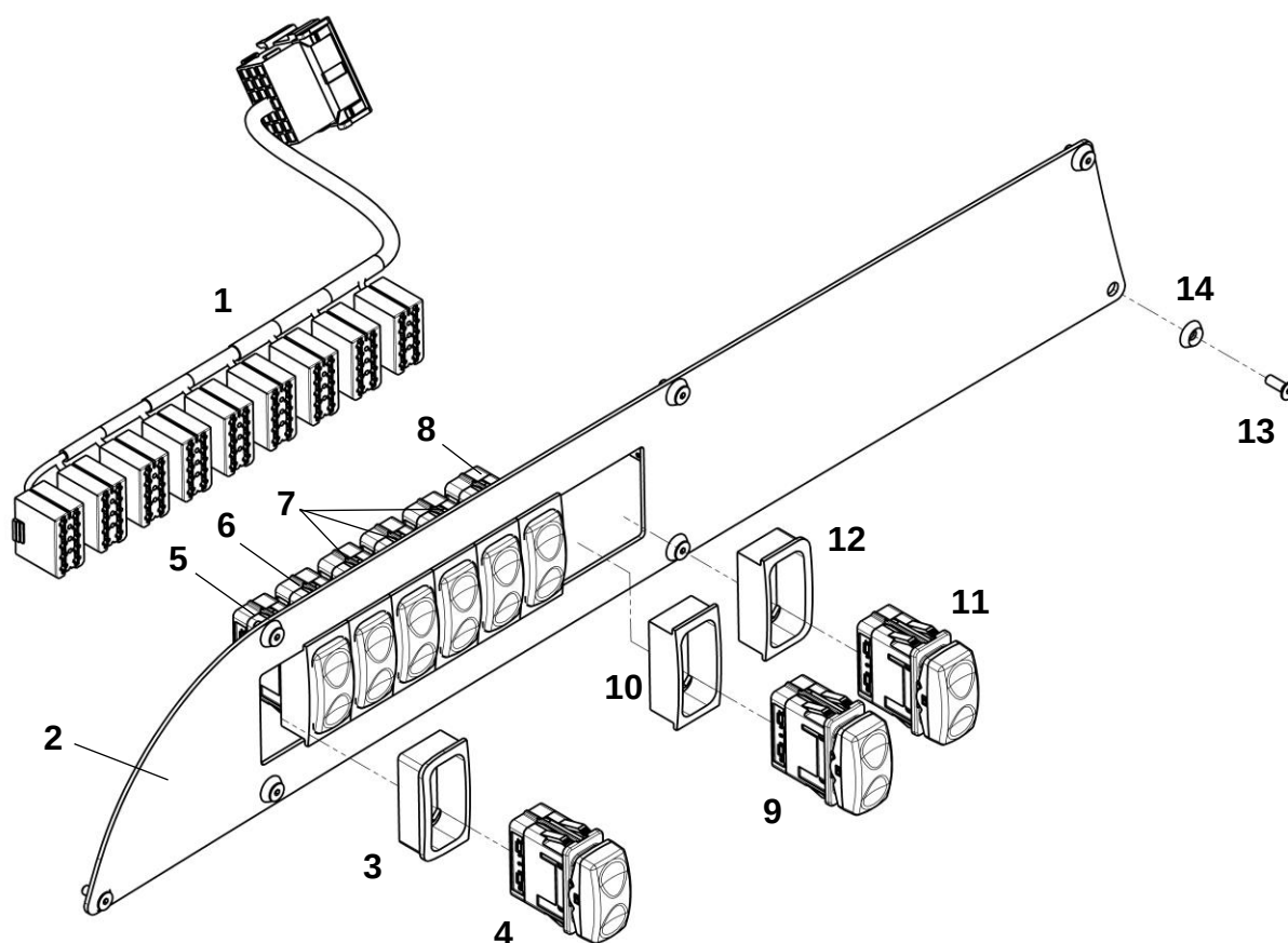
Пульт управления правый верхний
