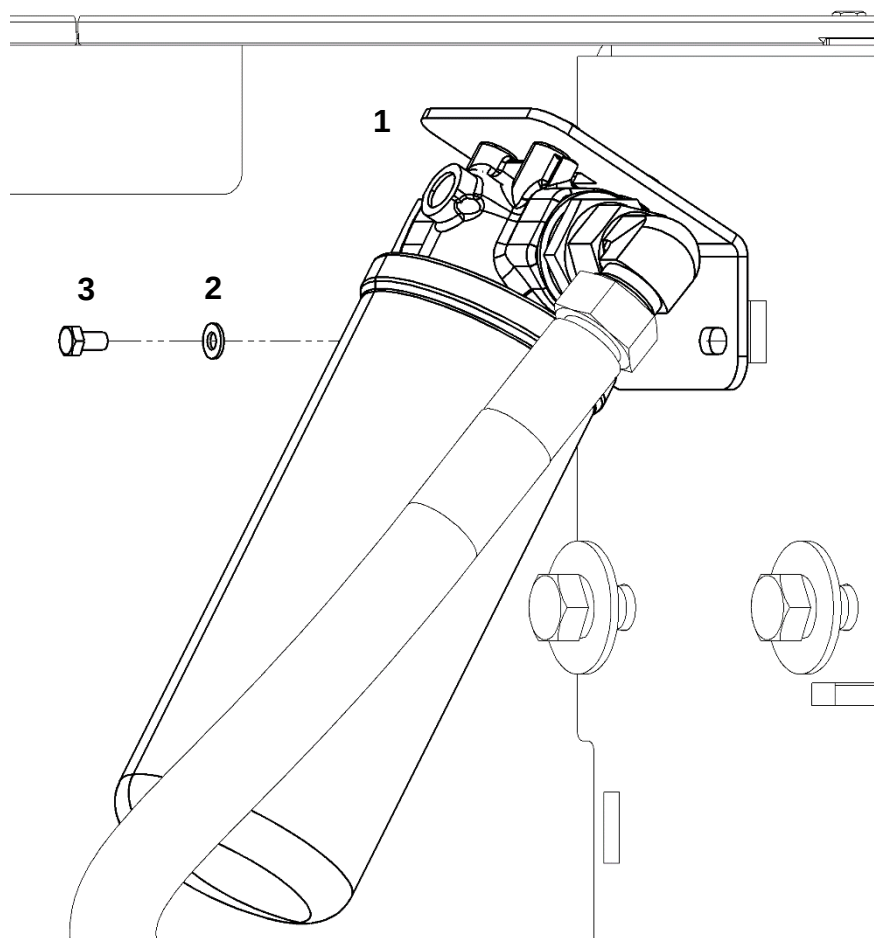
Трубопроводы гидросистемы навесного оборудования
