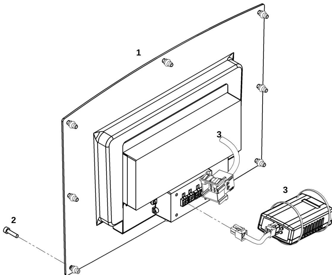
Приборный щиток в сборе
