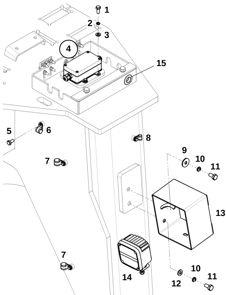
Датчики безопасности стрелы трубоукладчика
