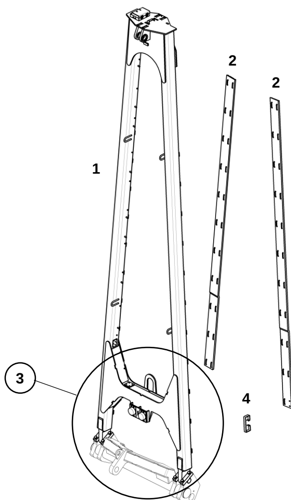
Стрела в сборе
