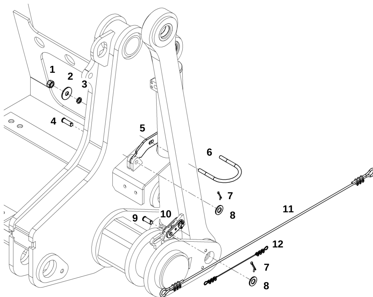
Установка крепежа гидроцилиндров
