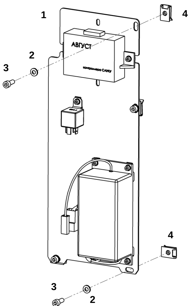
Электрооборудование кабины
