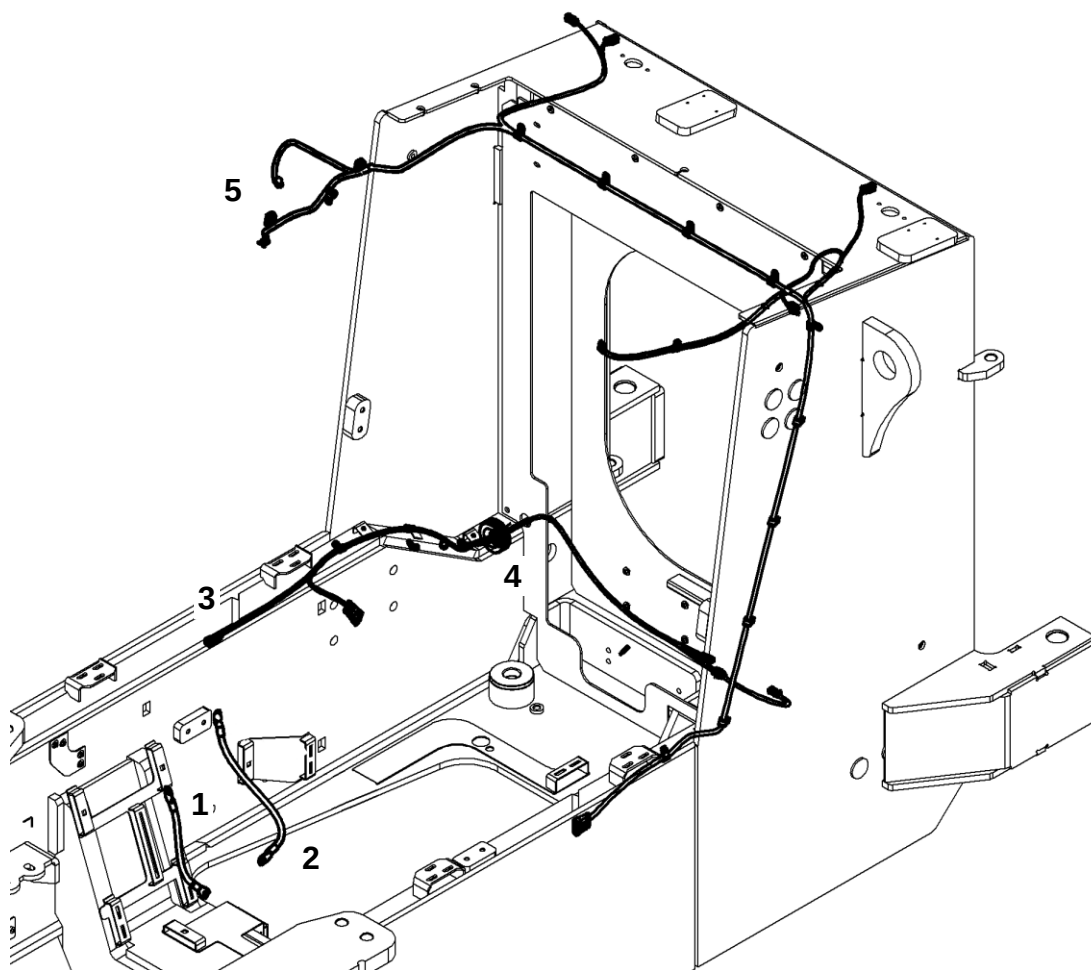
Электрооборудование (рамная часть)
