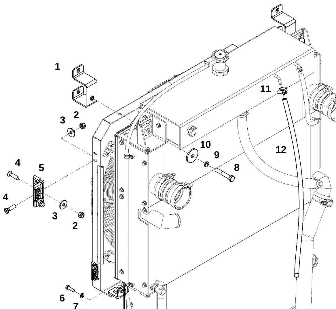
Система охлаждения
