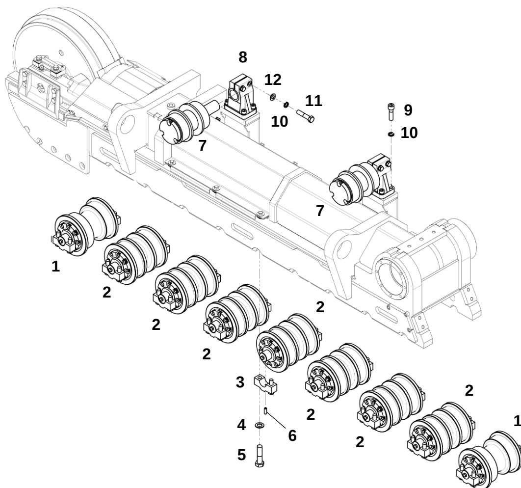
Тележка
