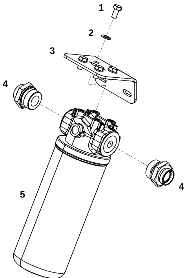
Фильтр напорный в сборе
