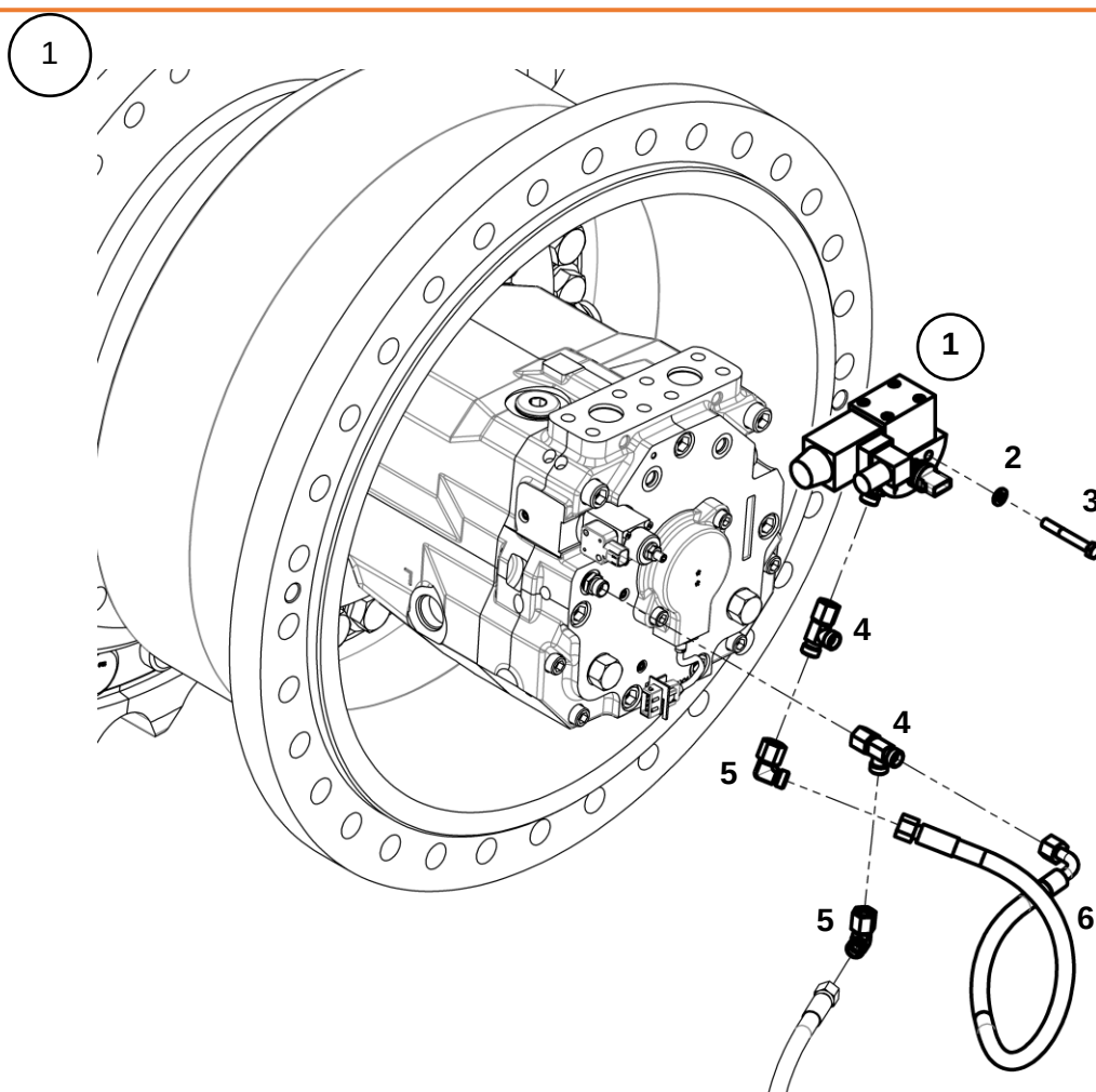
Подключение РВД к тормозной плите
