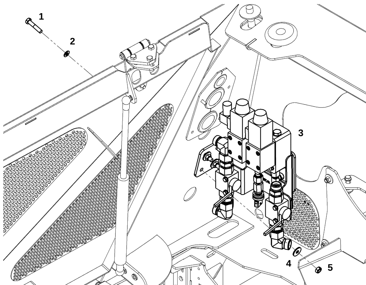
Трубопроводы гидросистемы навесного оборудования
