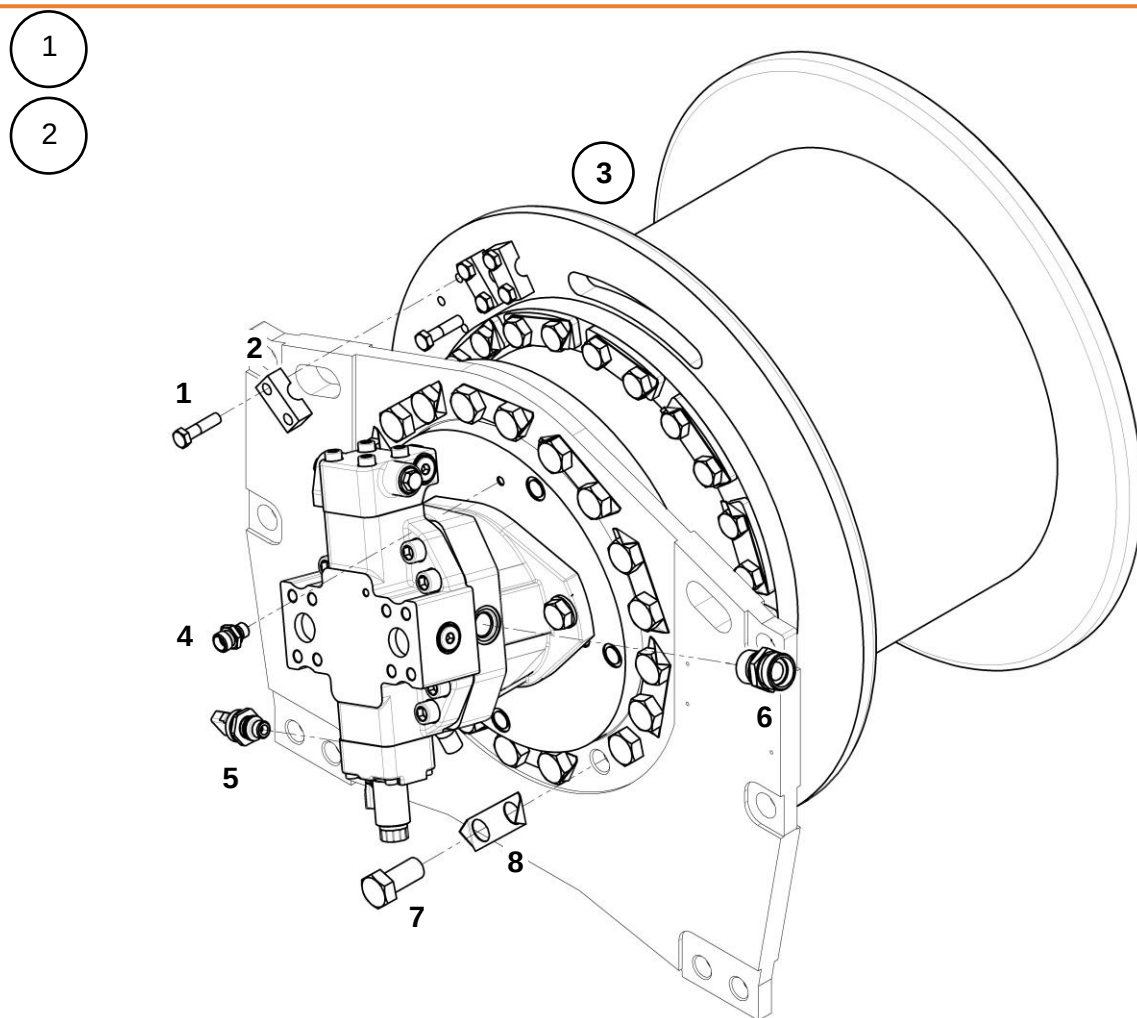
Лебедка гидравлическая
