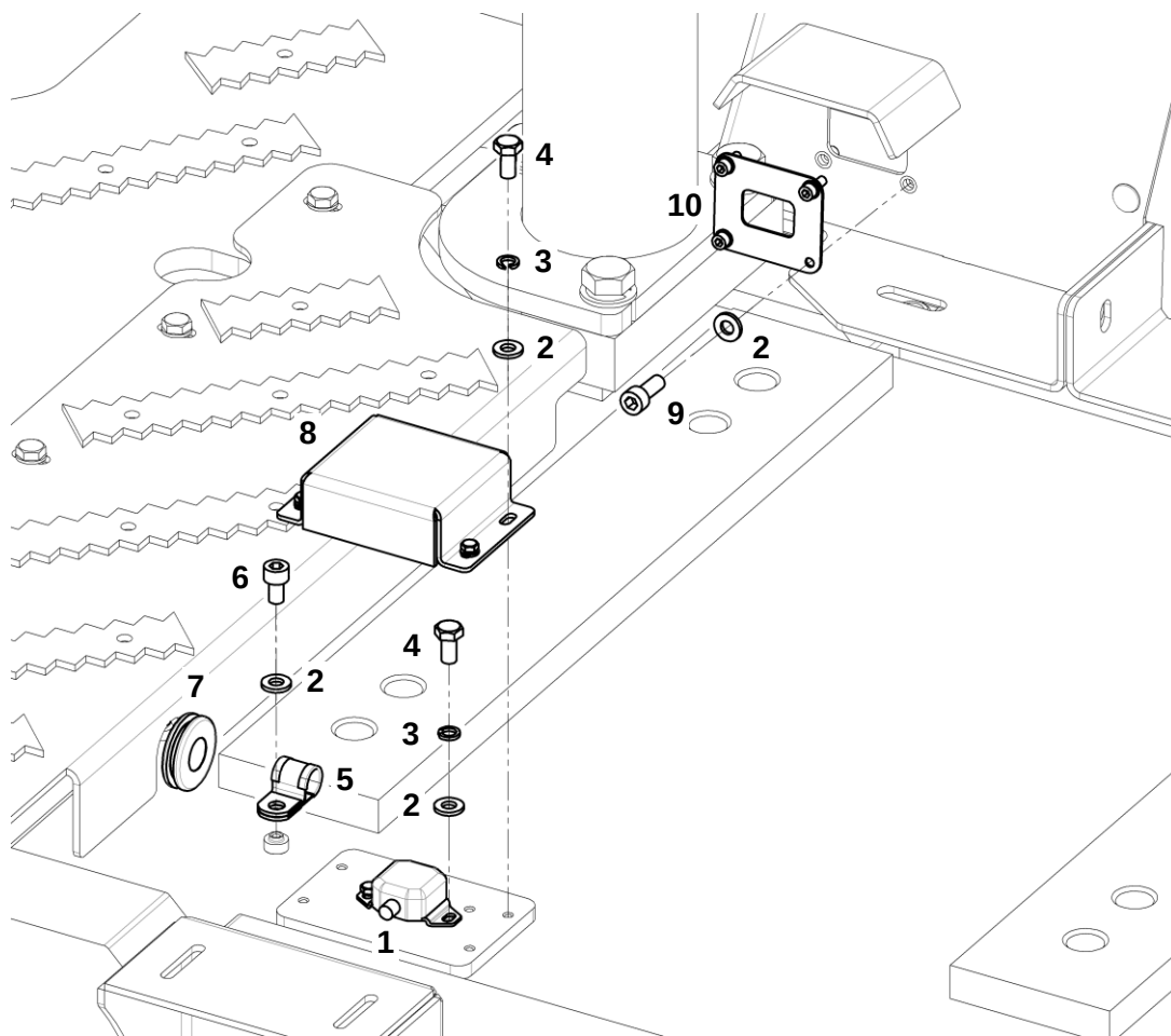
Датчики безопасности рамы портала
