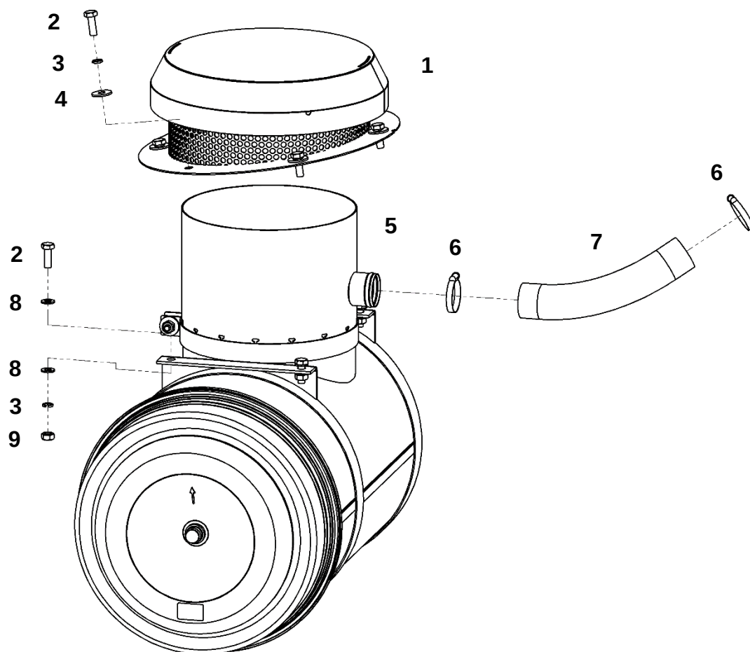
Система впуска-выпуска воздуха
