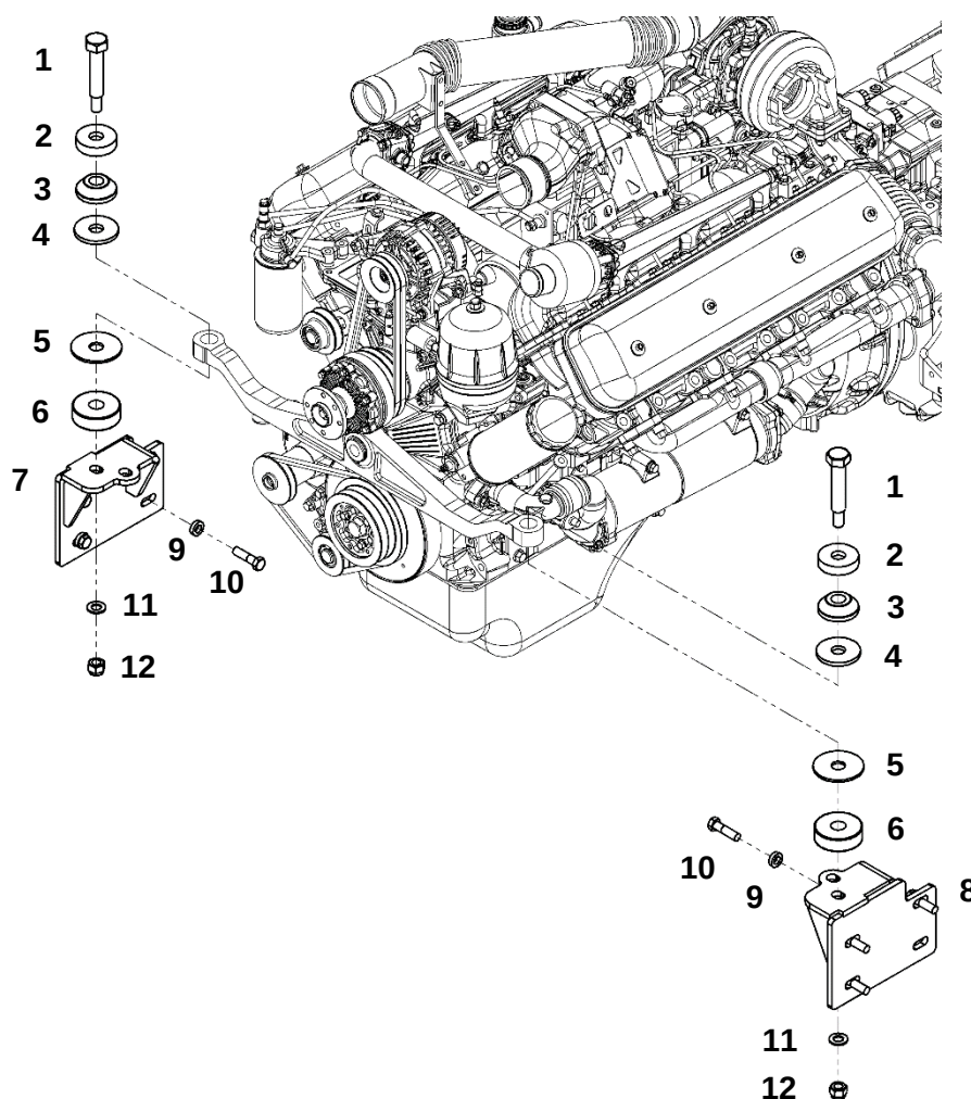
Установка силового агрегата
