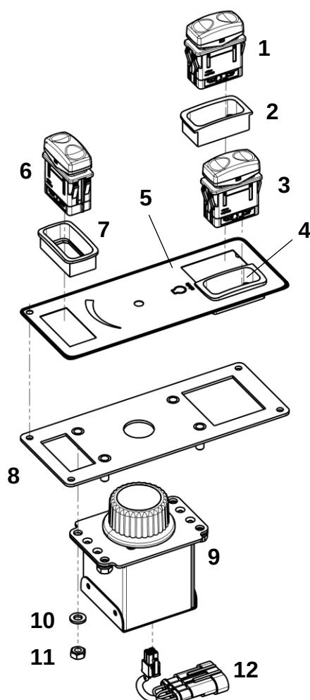
Панель управления
