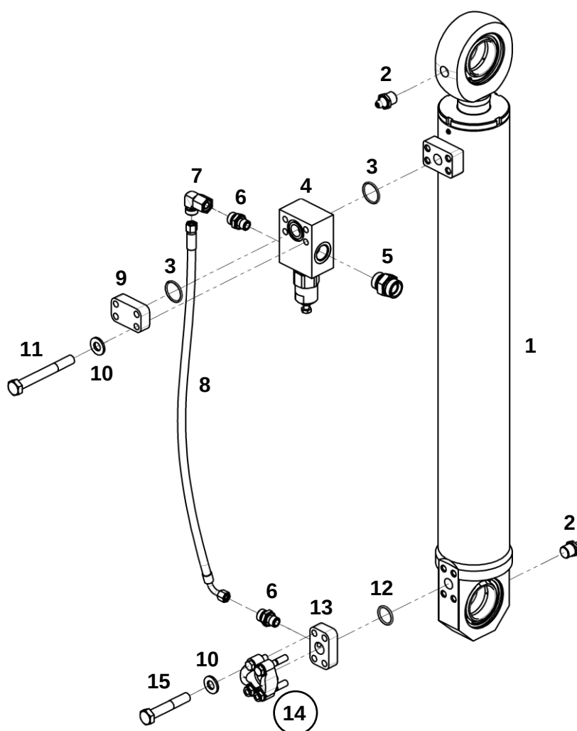
Гидроцилиндр в сборе
