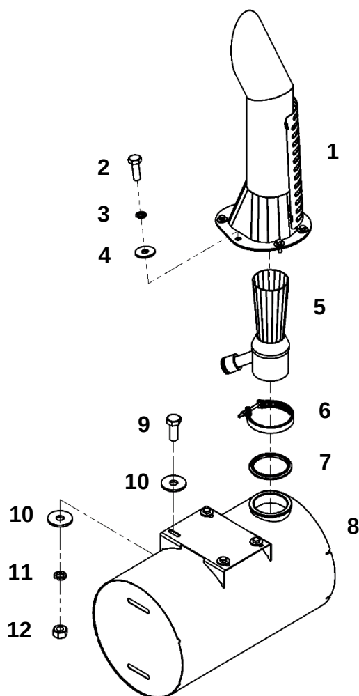
Система впуска-выпуска воздуха
