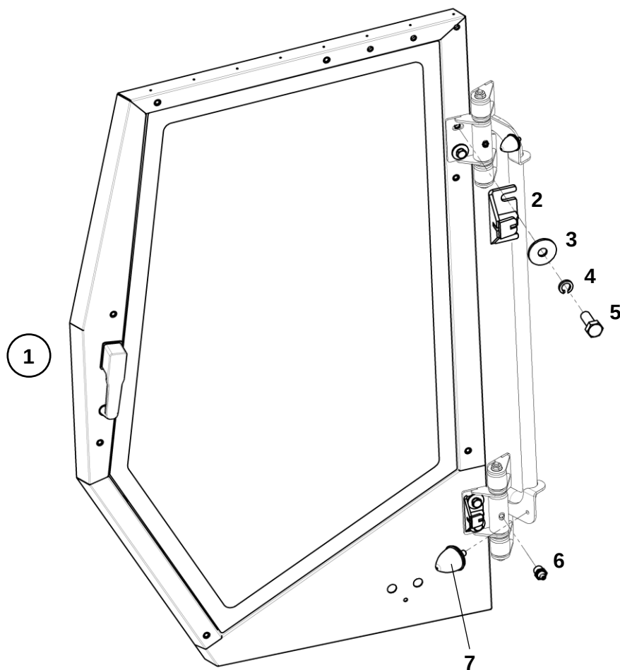
Дверь кабины
