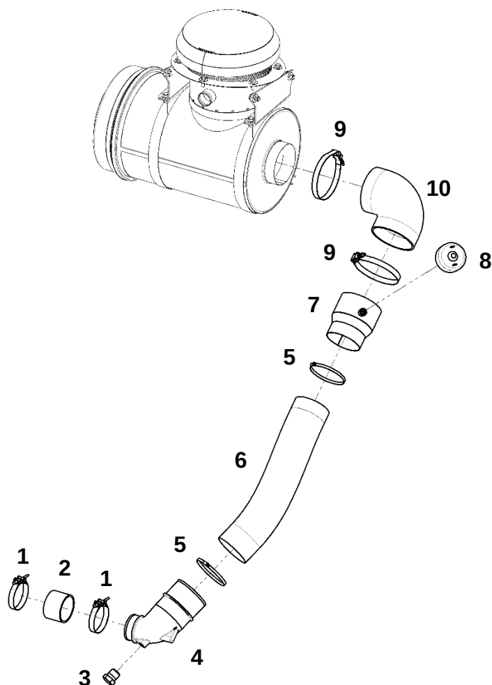
Система впуска-выпуска воздуха
