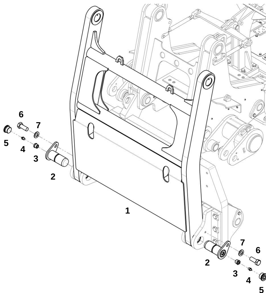
Контргруз в сборе
