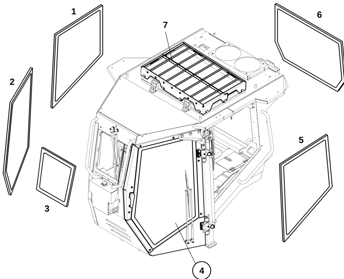
Кабина
