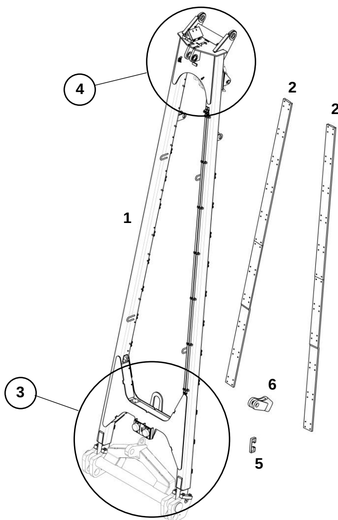
Стрела-опора в сборе
