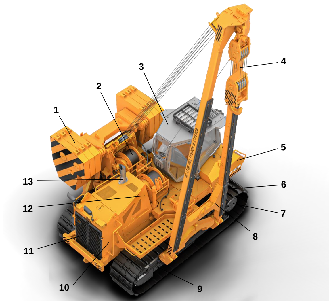
Кран-трубоукладчик ТГ35.80
