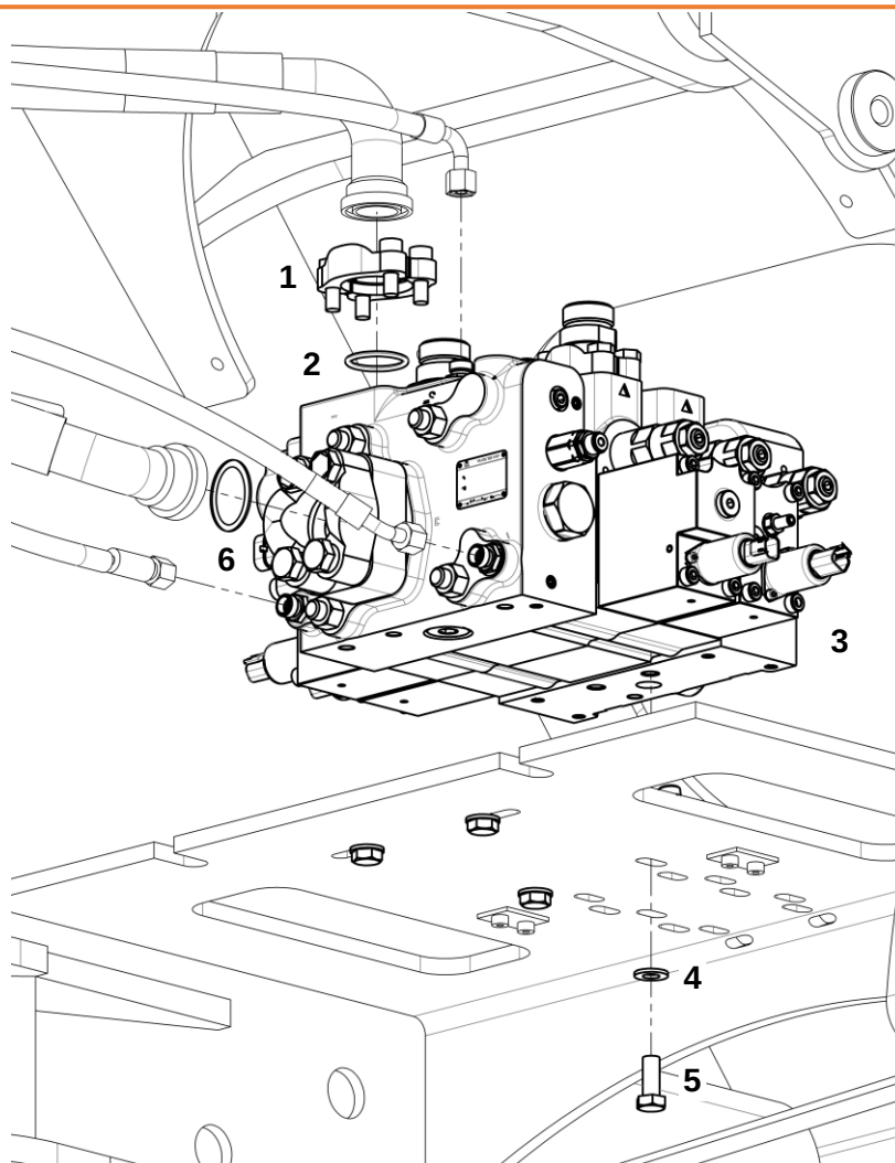
Подключение к гидрораспределителю
