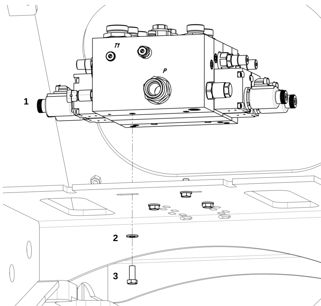
Крепление гидрораспределителя
