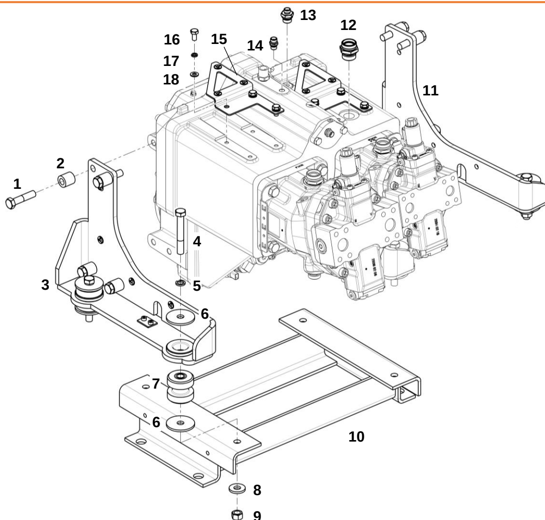
Коробка передач
