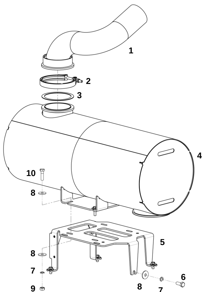
Система впуска воздуха и выпуска ОГ
