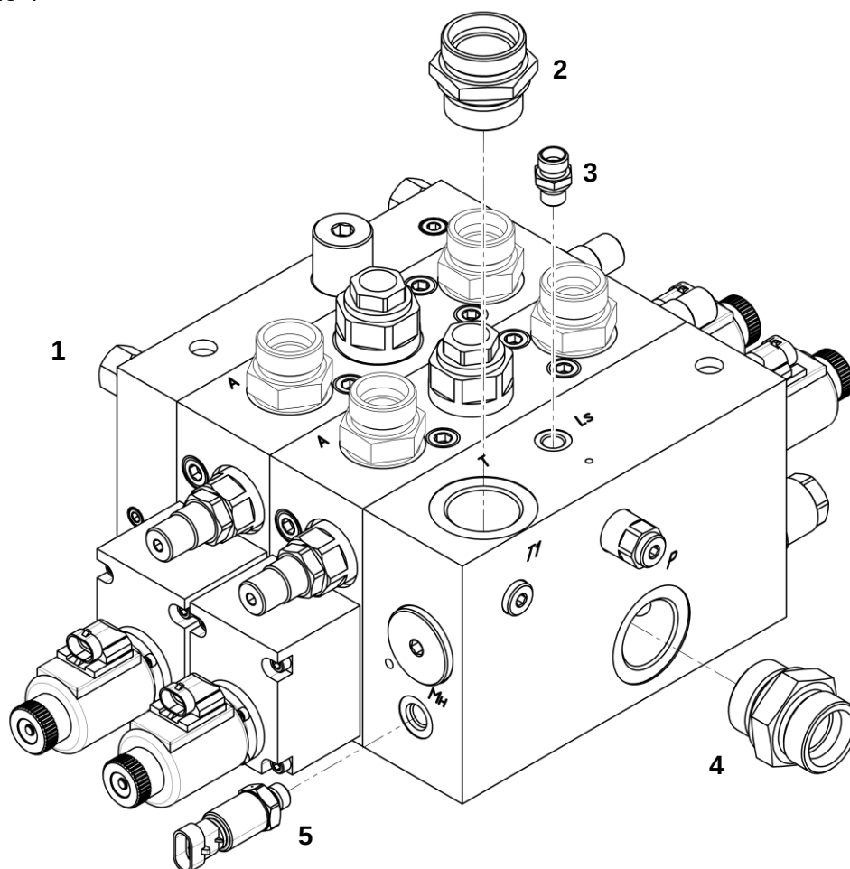
Гидрораспределитель в сборе
