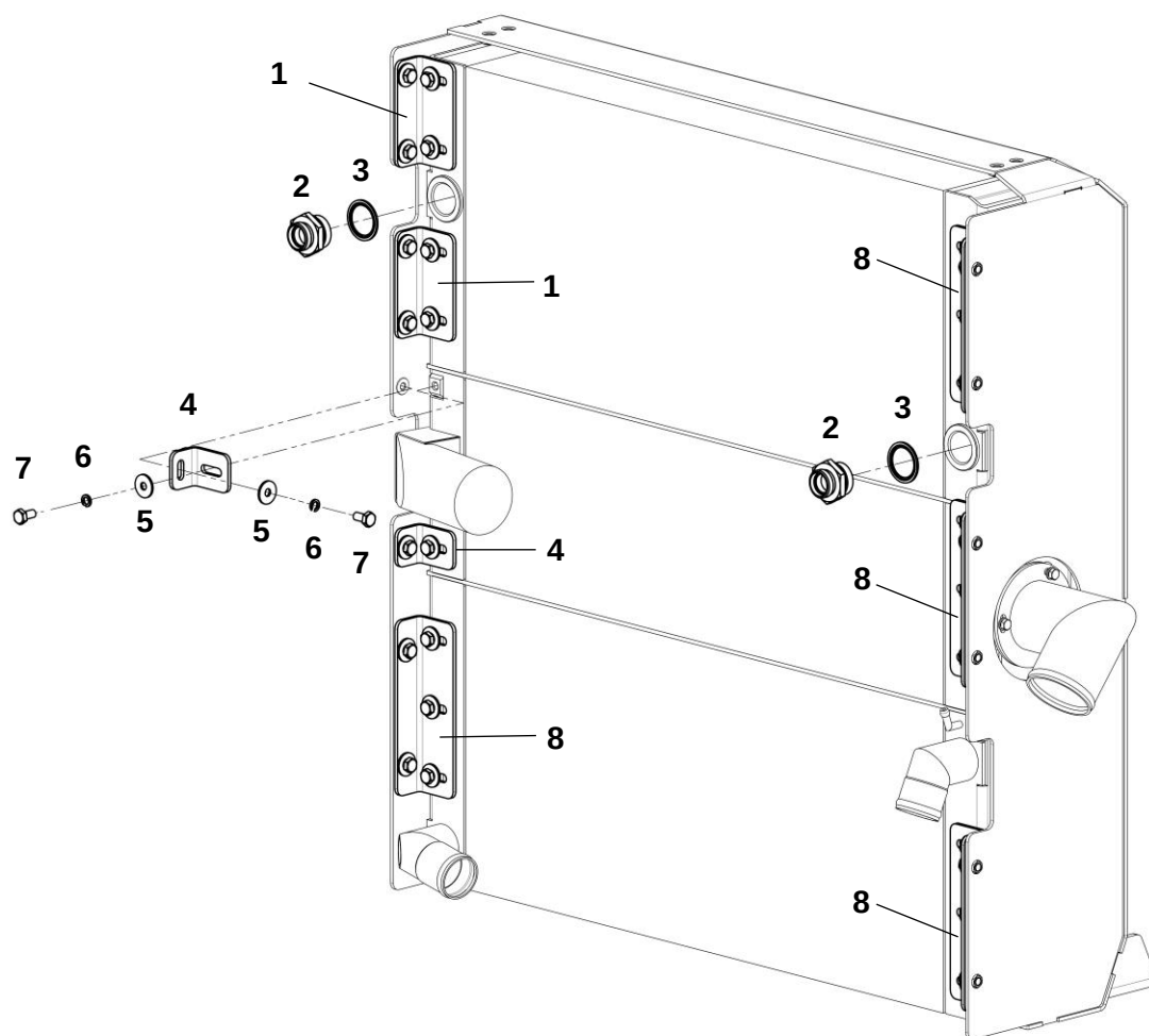
Блок радиаторов в сборе
