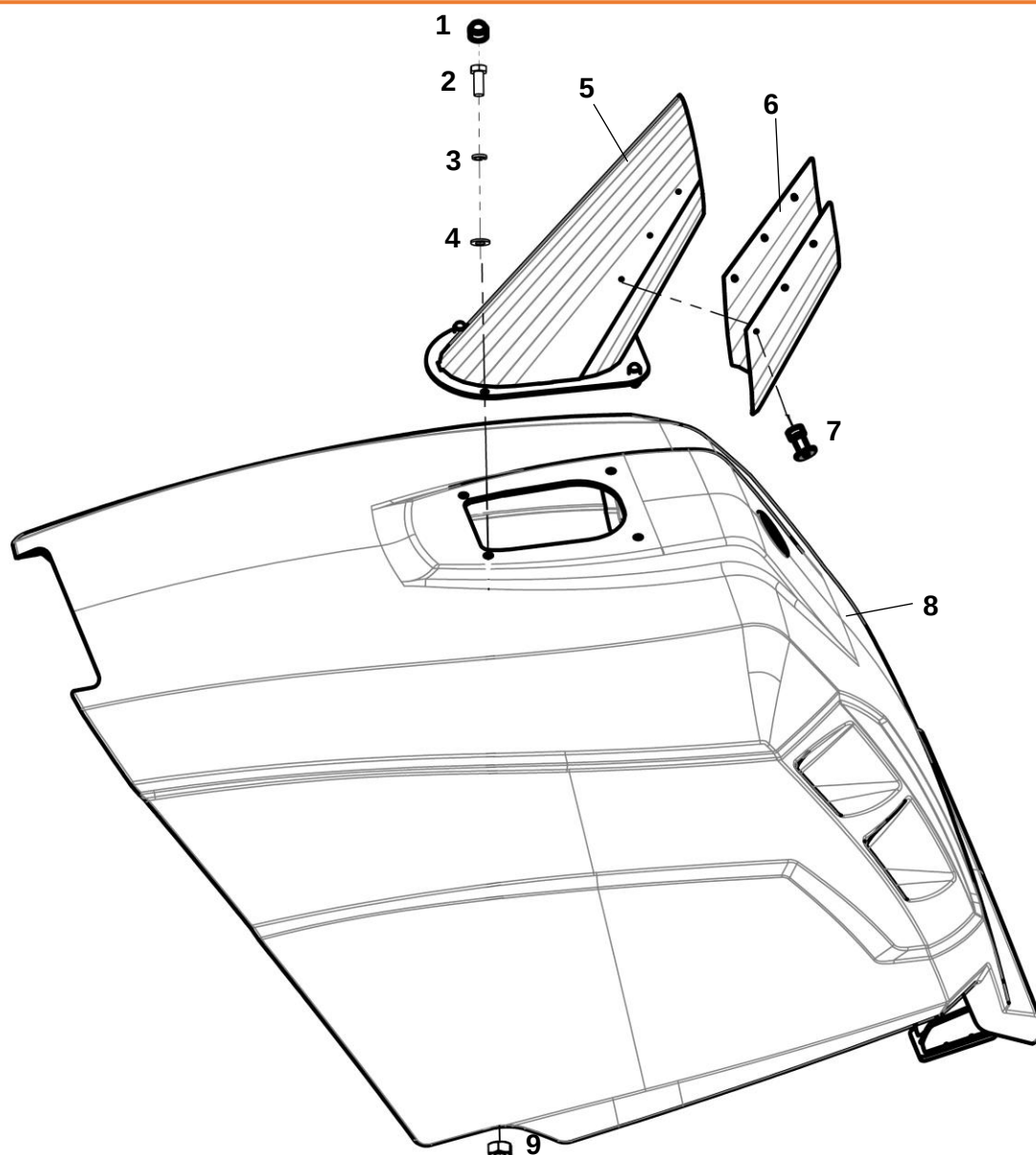
Установка капота
