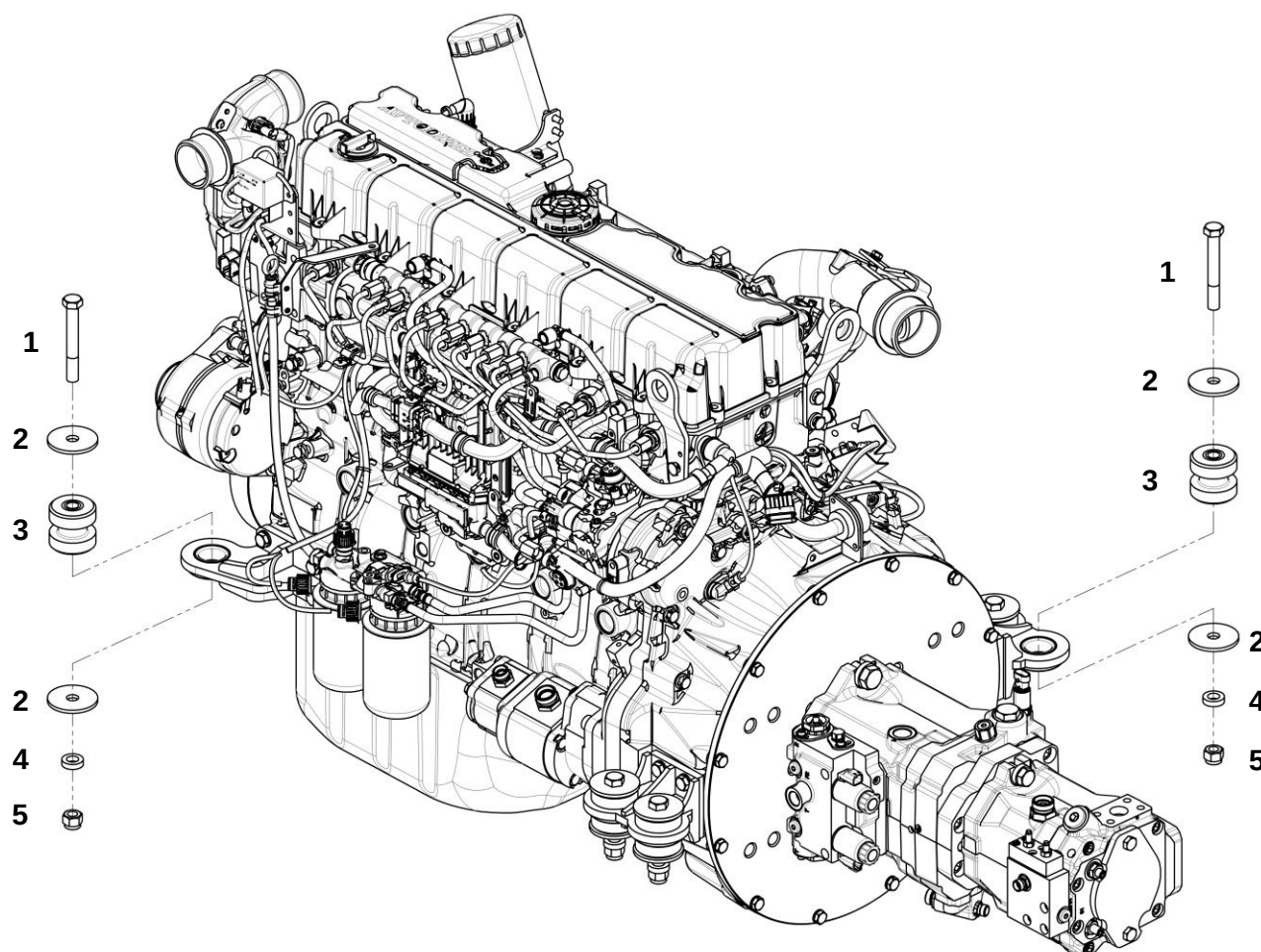
Силовой агрегат
