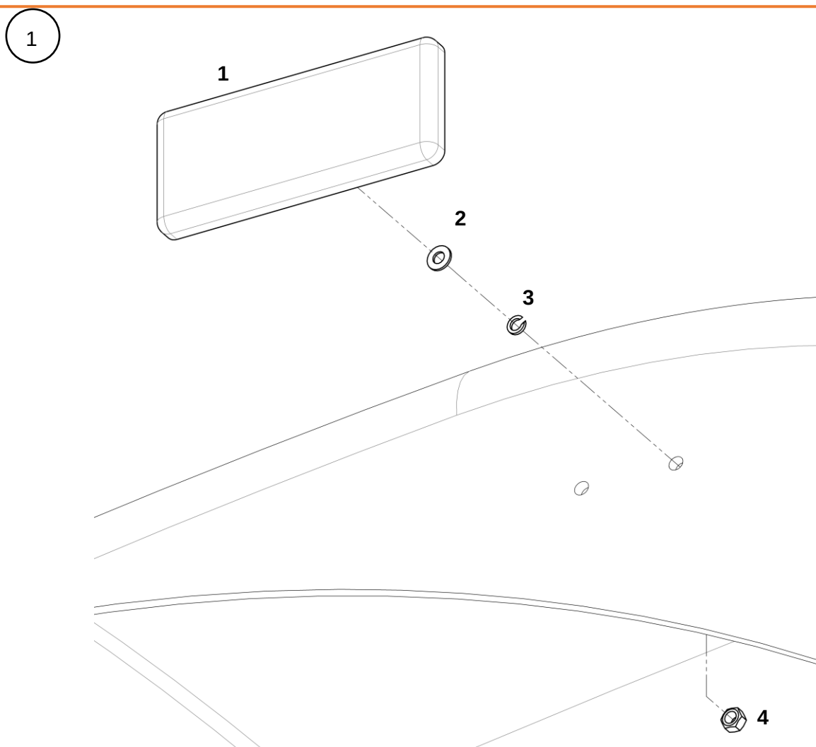
Установка световозвращателя
