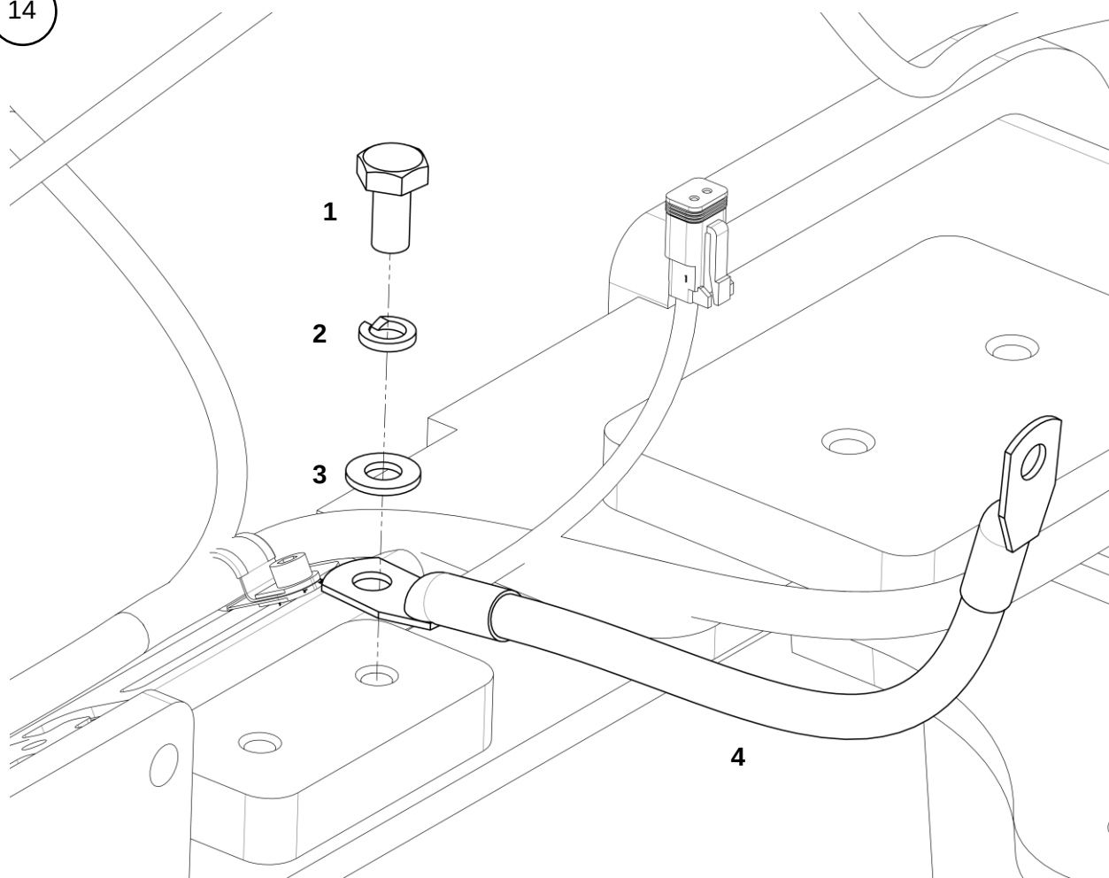
Крепление кабеля
