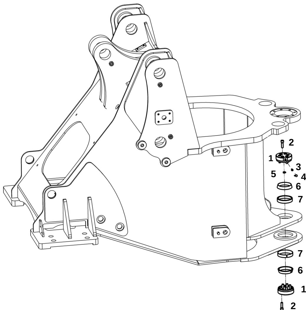
Рама
