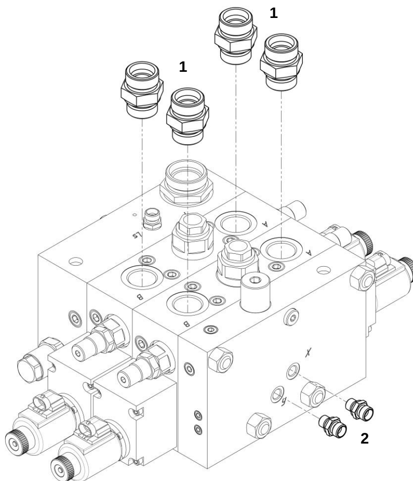
Гидрораспределитель в сборе
