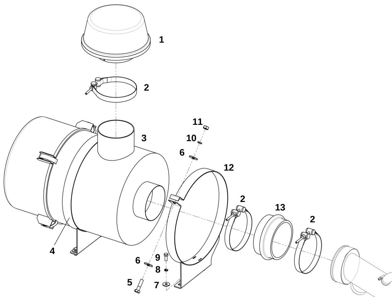
Система впуска воздуха и выпуска ОГ
