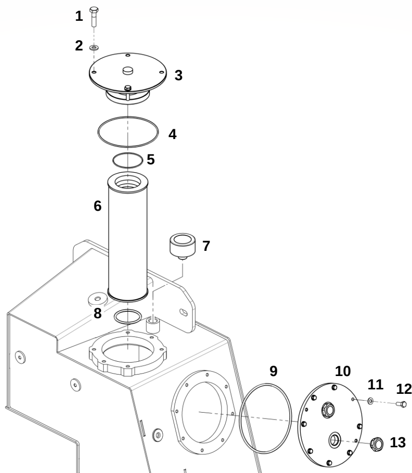
Бак гидравлический в сборе
