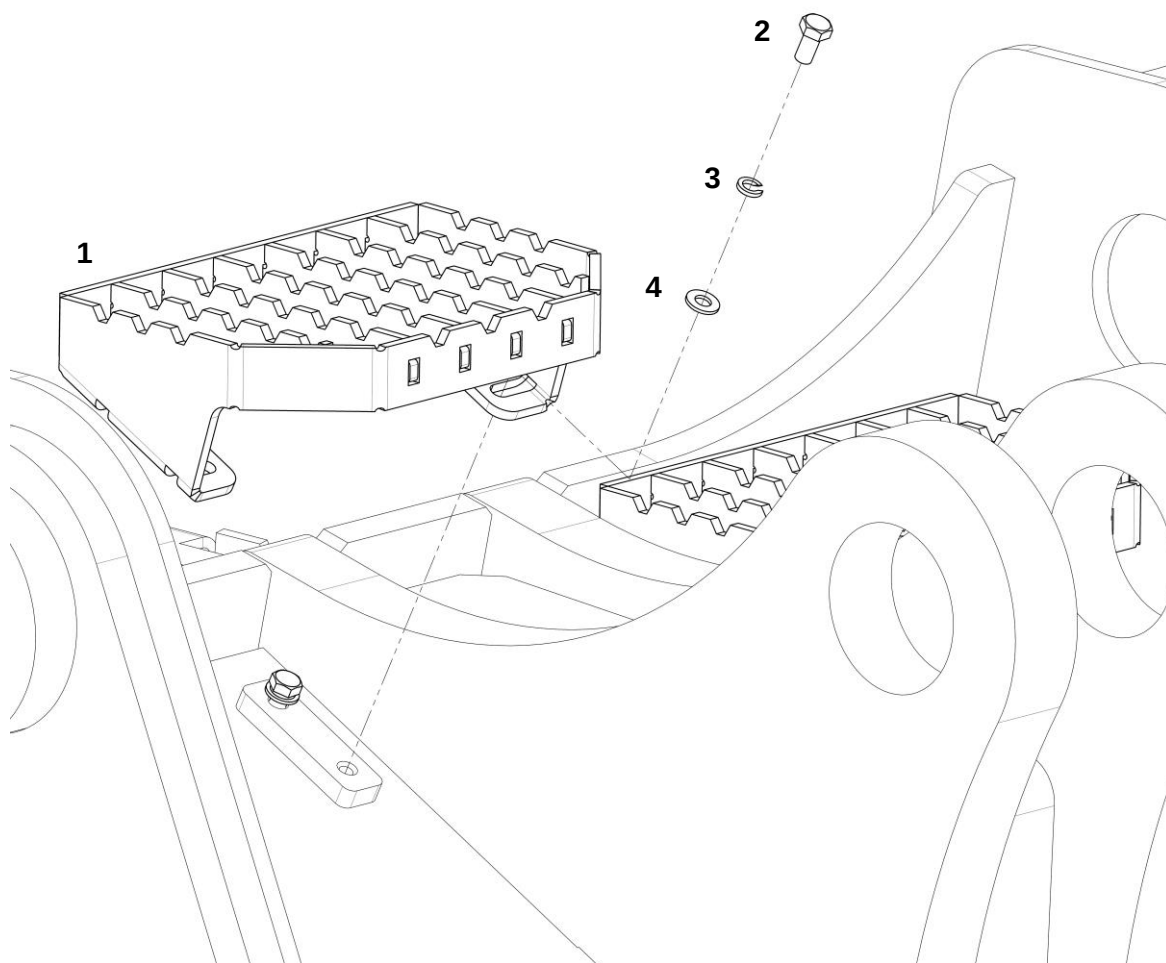
Облицовка
