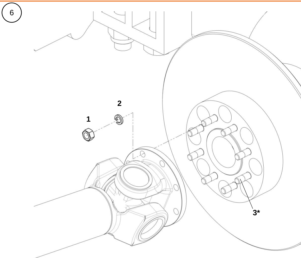
Крепление к переднему мосту
