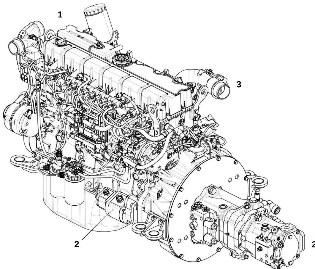
Силовой агрегат в сборе
