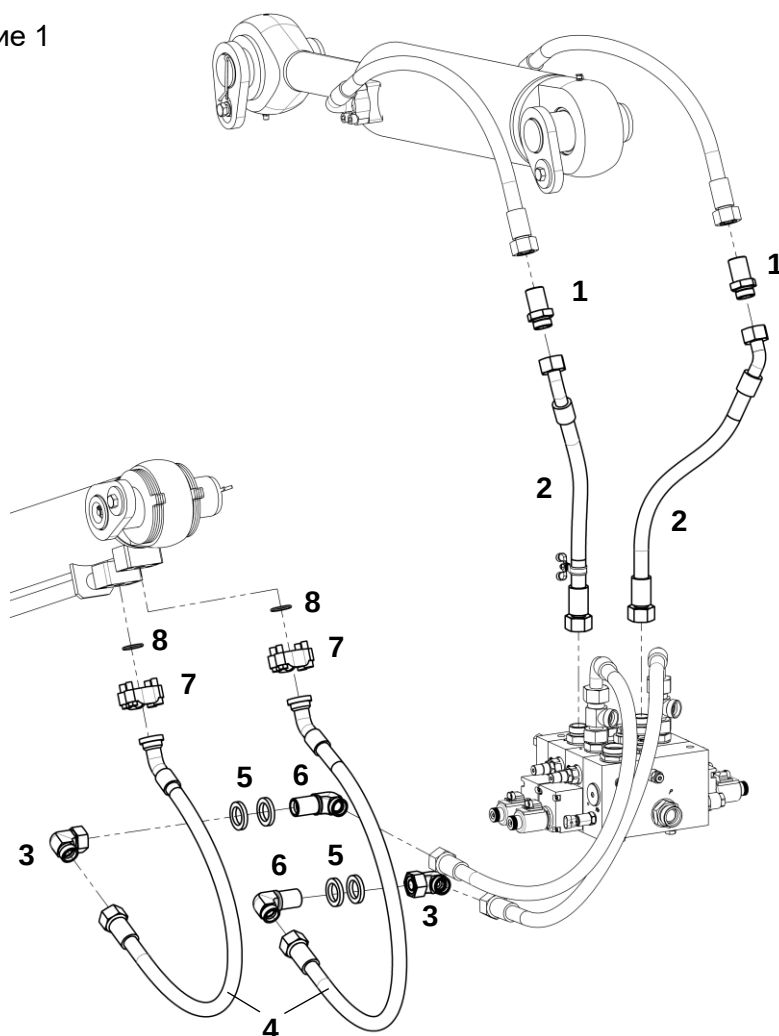
Подключение к гидрораспределителю
