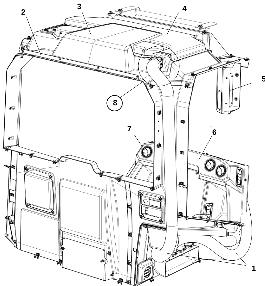
Облицовка кабины
