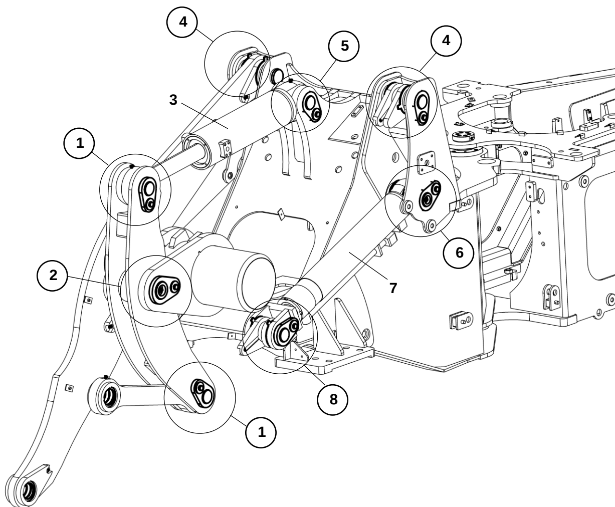
Рабочее оборудование
