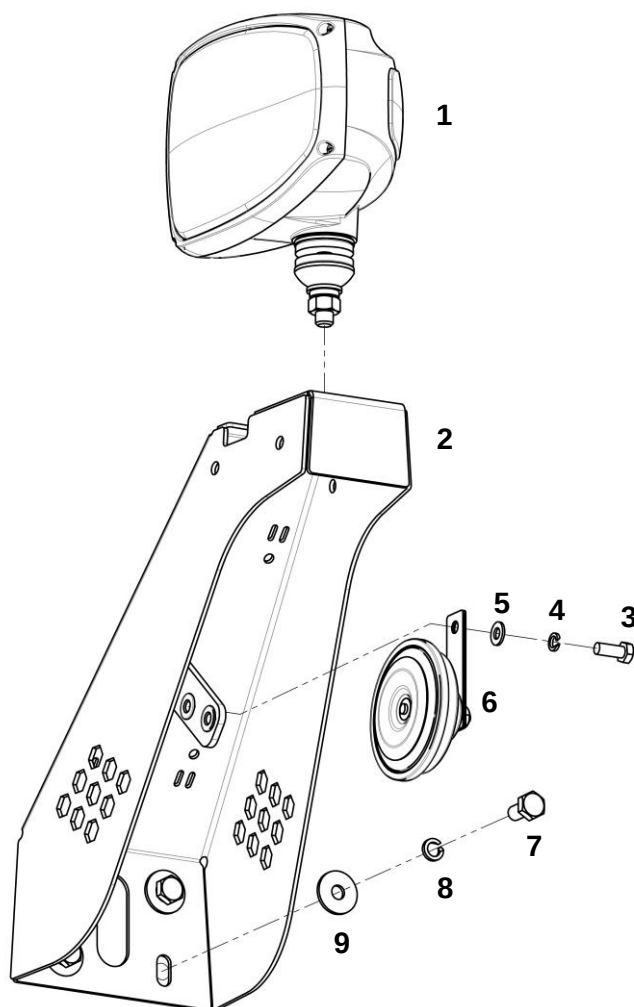
Передние фары и сигнал с элементами крепежа
