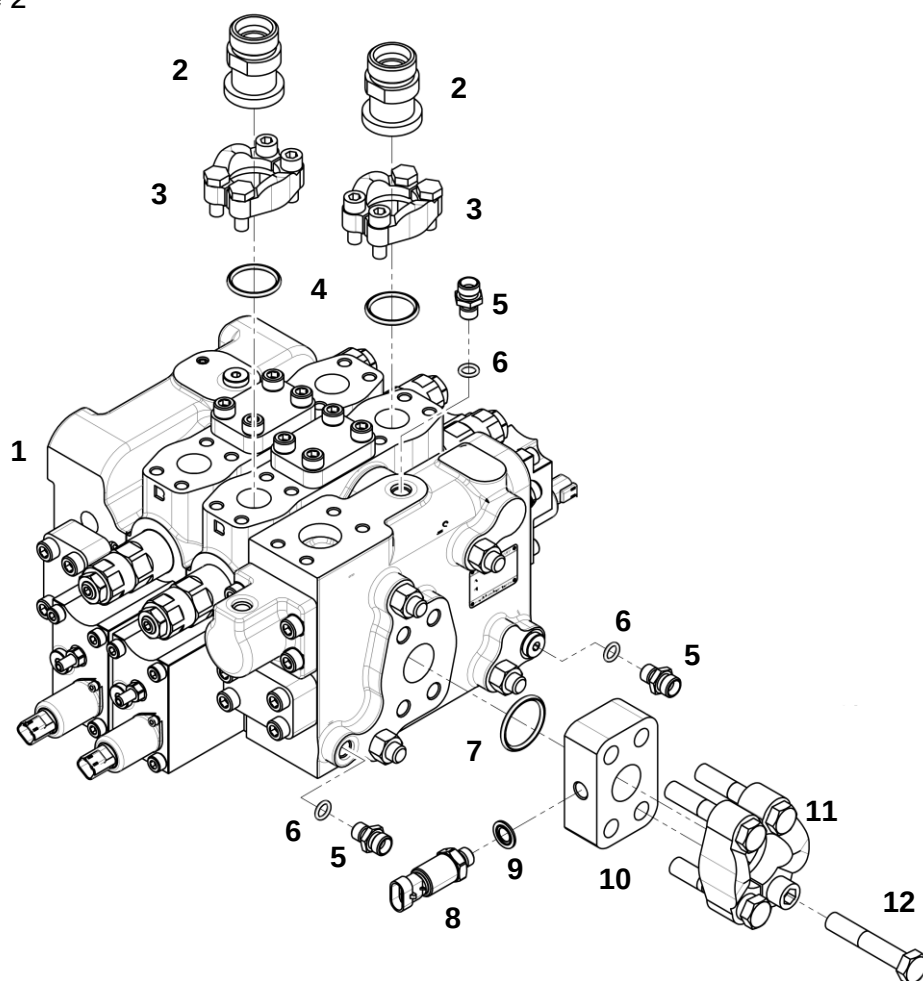
Гидрораспределитель в сборе
