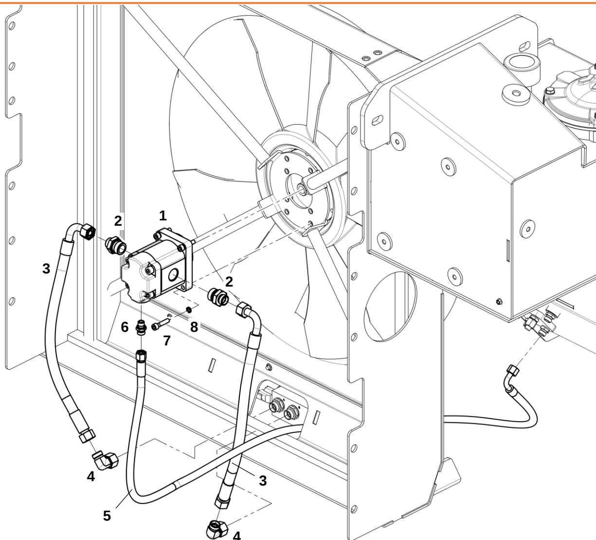
Гидропривод вентилятора
