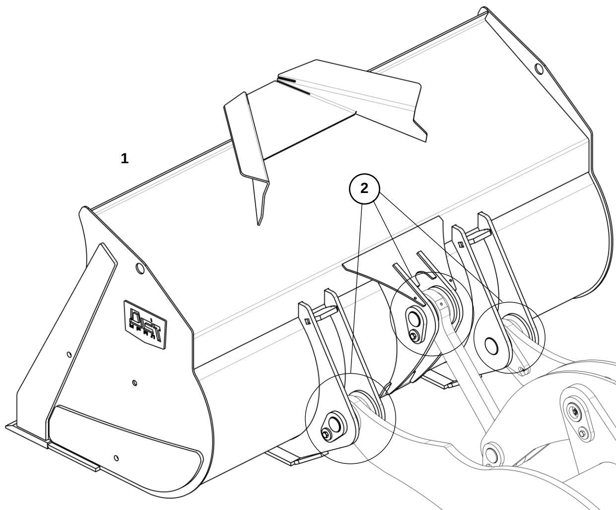
Оборудование навесное
