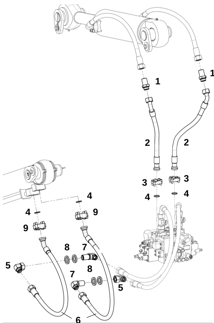
Подключение к гидрораспределителю
