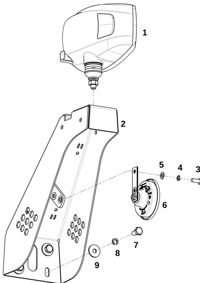
Передние фары и сигнал с элементами крепежа
