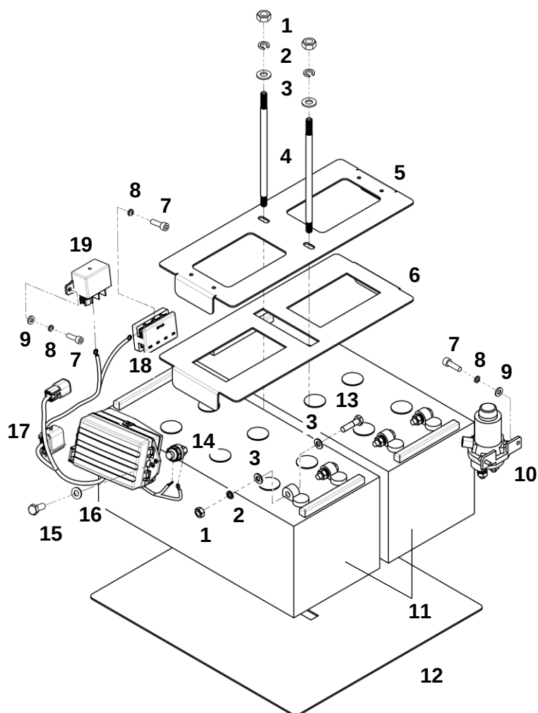
Аккумуляторные батареи с элементами крепежа
