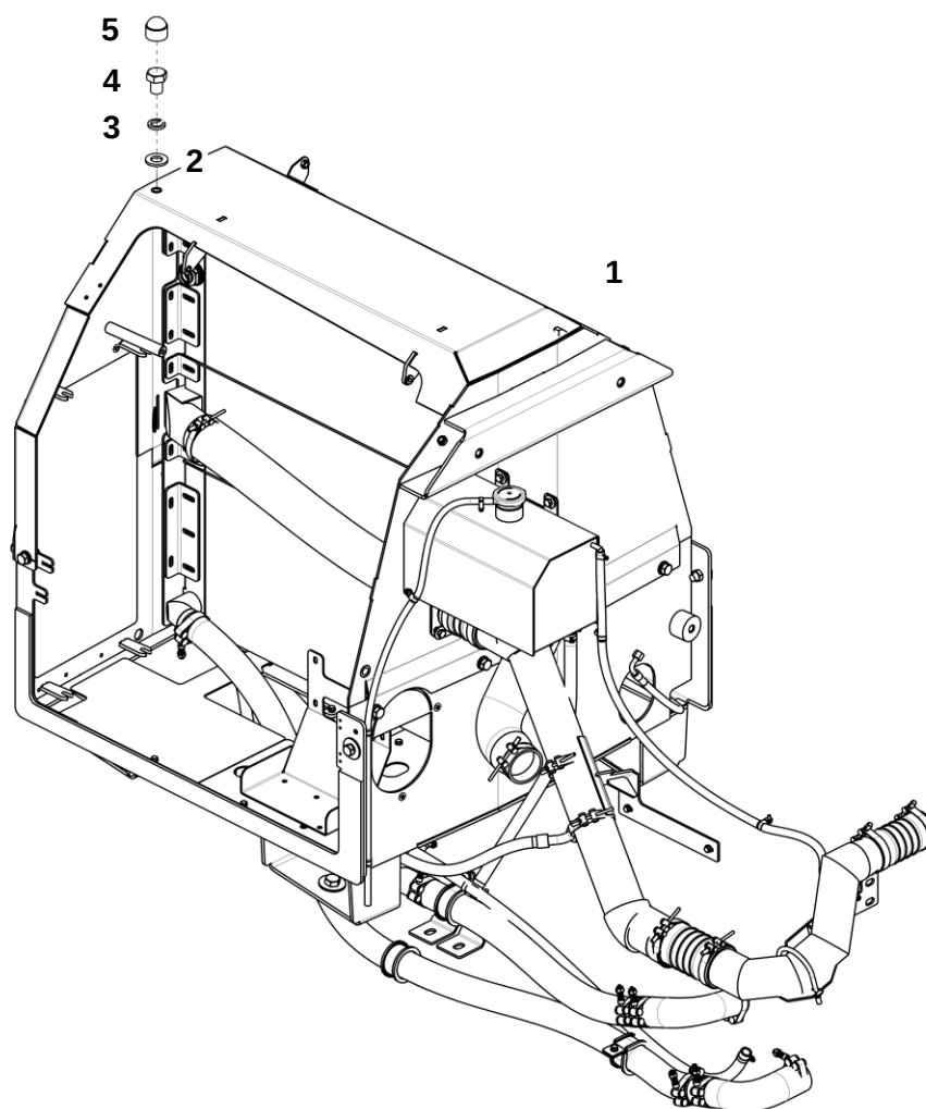
Система охлаждения
