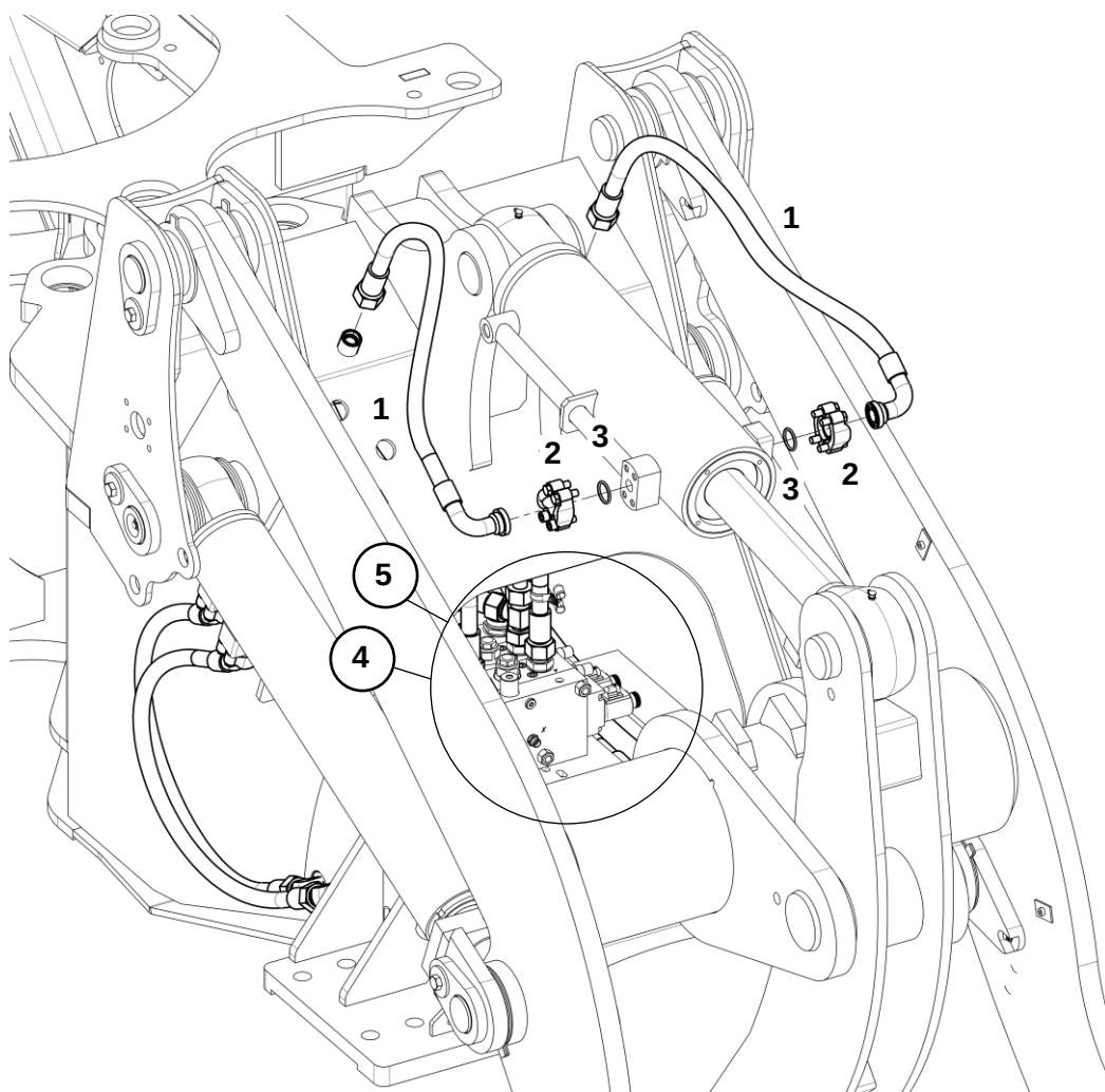
Гидравлика навесного оборудования
