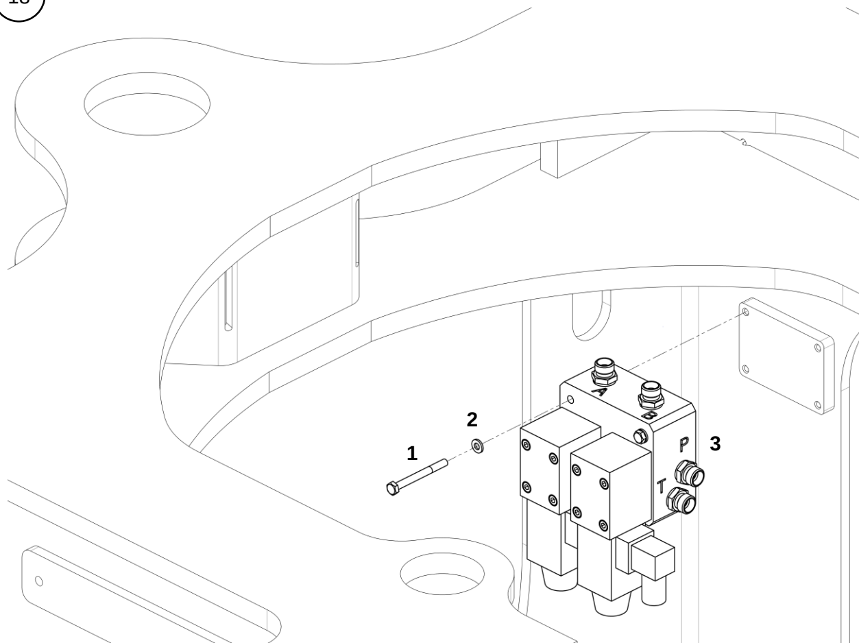
Плита с крепежом
