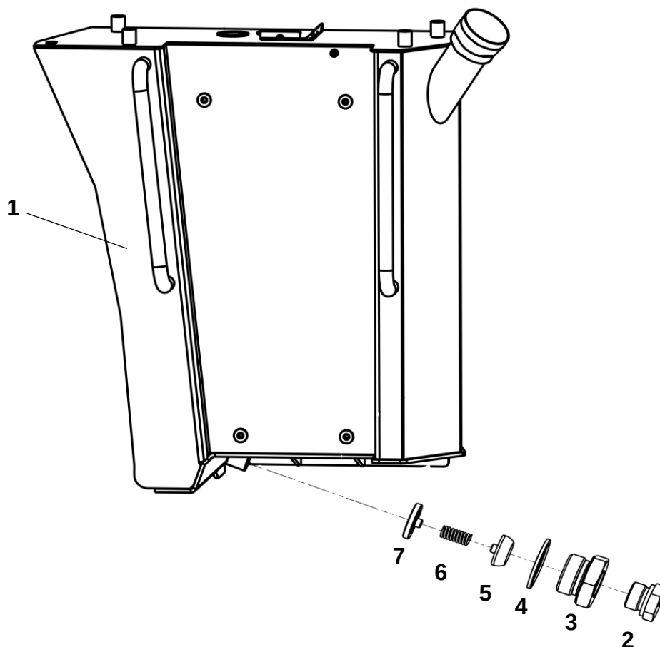
Топливный бак в сборе
