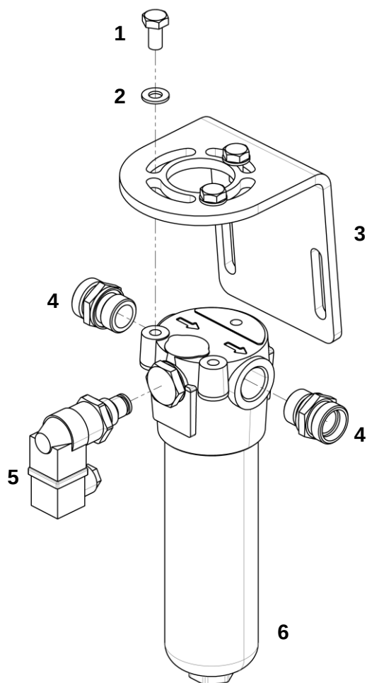
Фильтр напорный FMM в сборе
