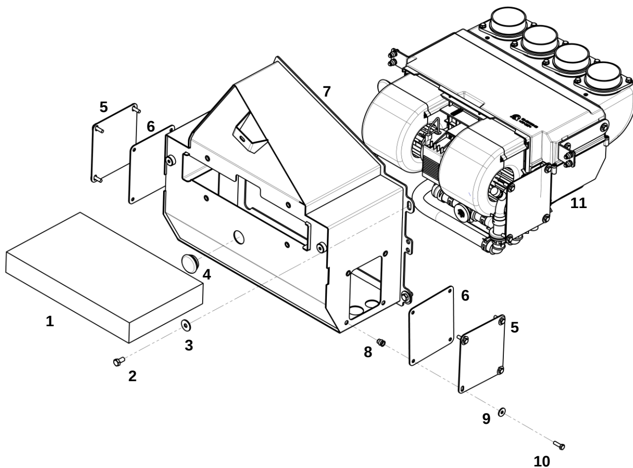
Блок испарительно-отопительный
