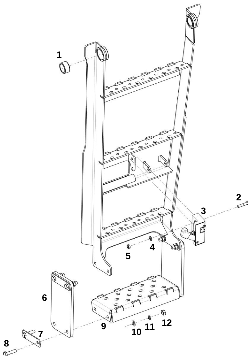
Установка лестницы (правой)
