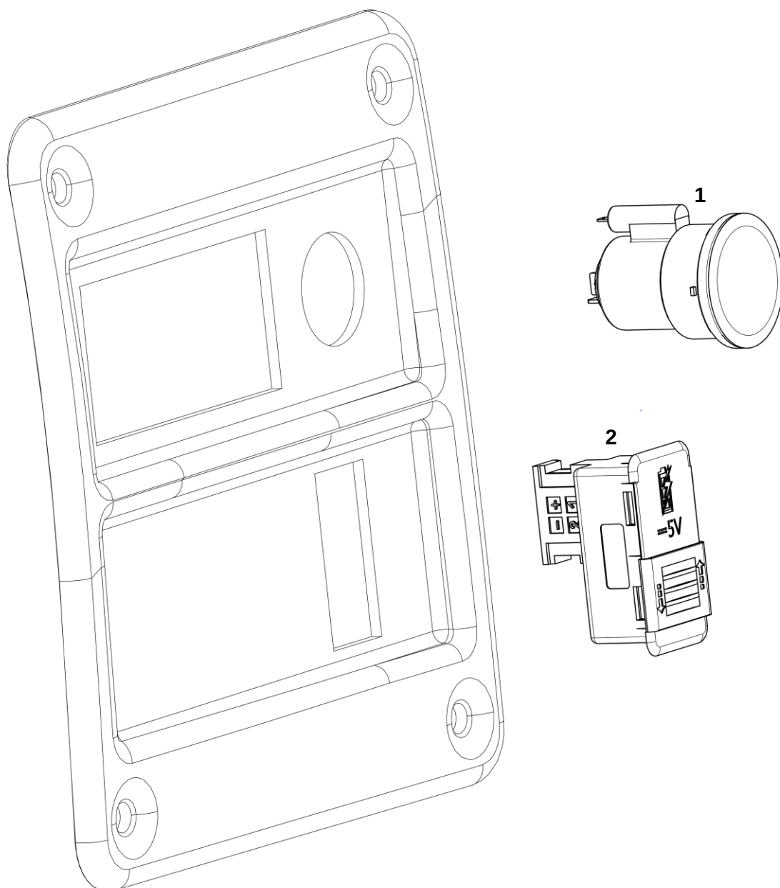
Панель управления задняя
