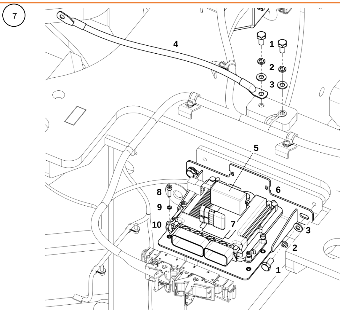
Контроллер в сборе
