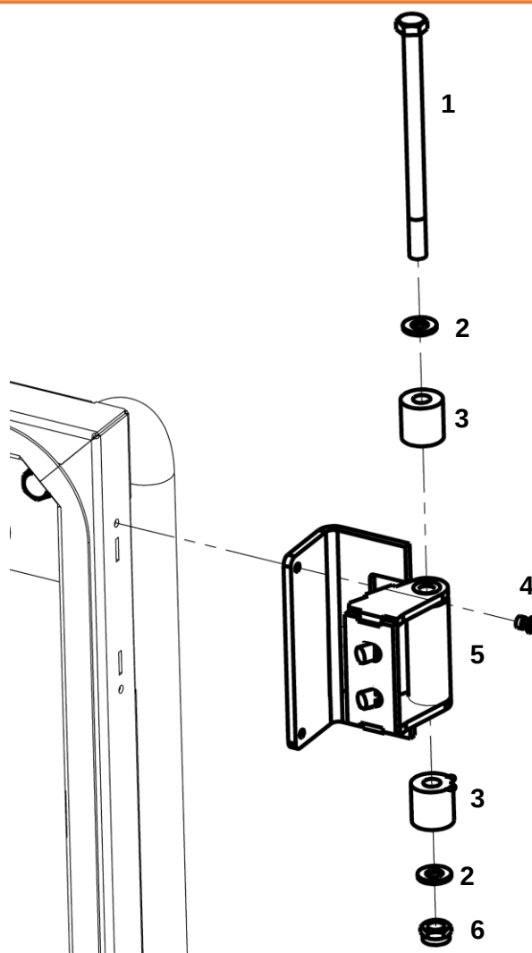
Петля двери
