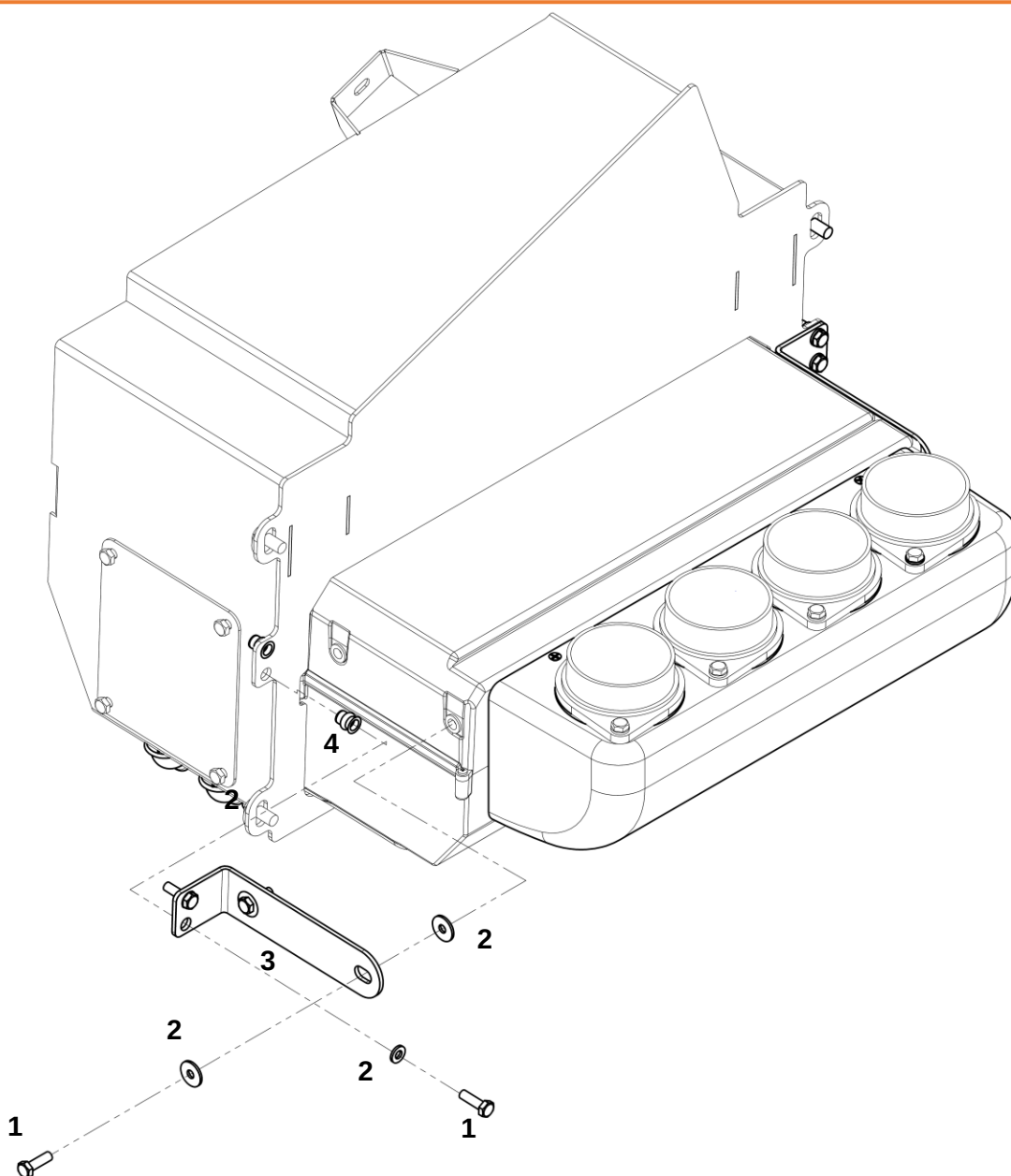
Блок испарительный
