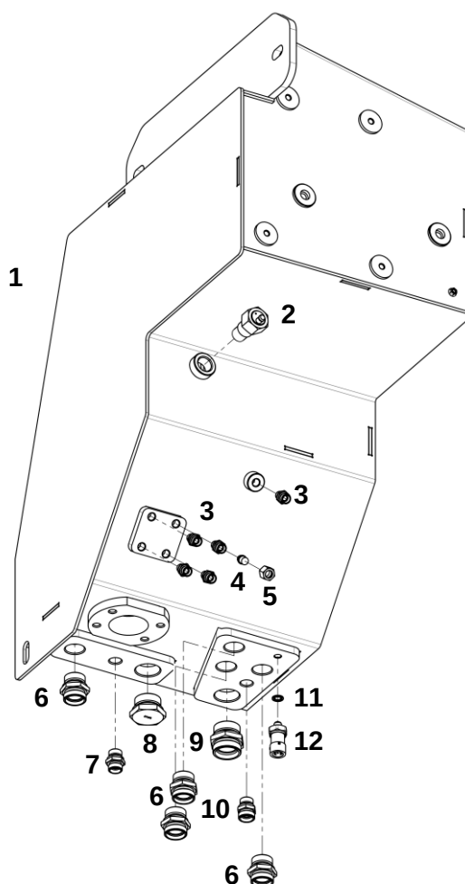
Бак гидравлический в сборе
