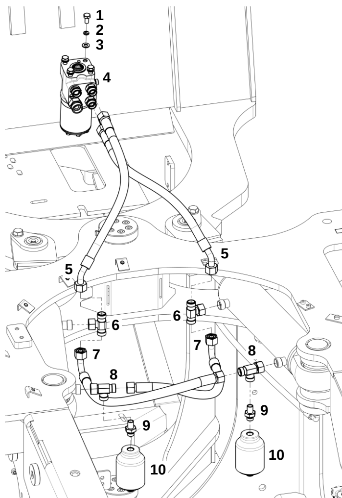
Гидравлика рулевого
