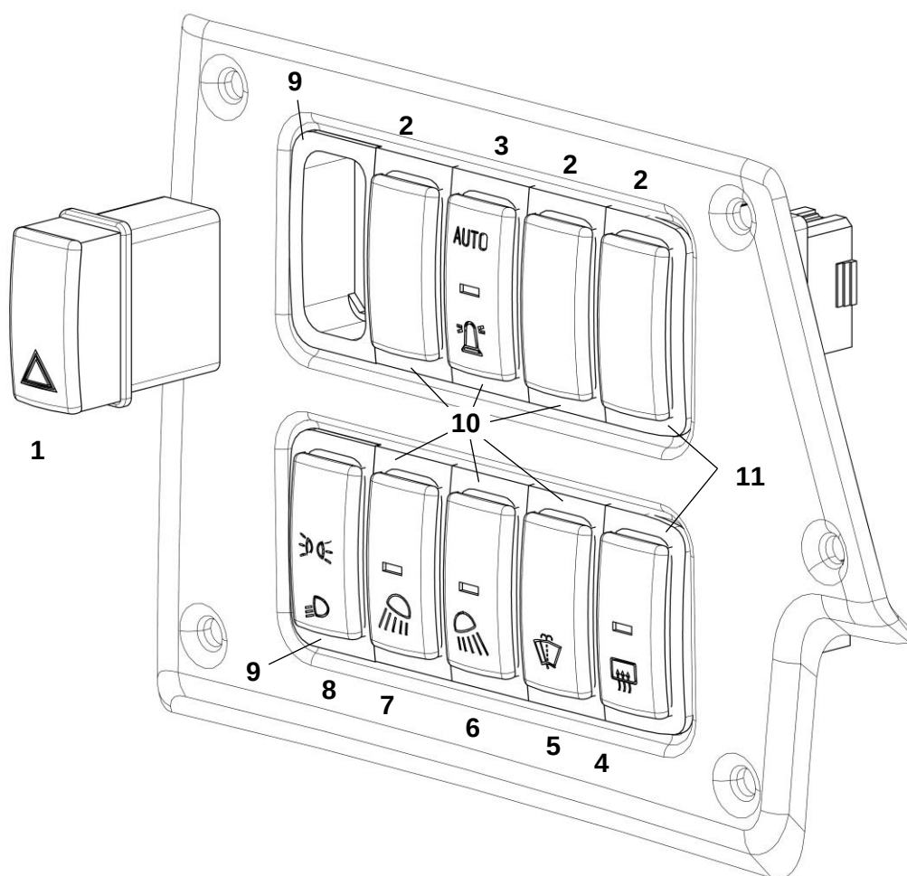
Панель выключателей
