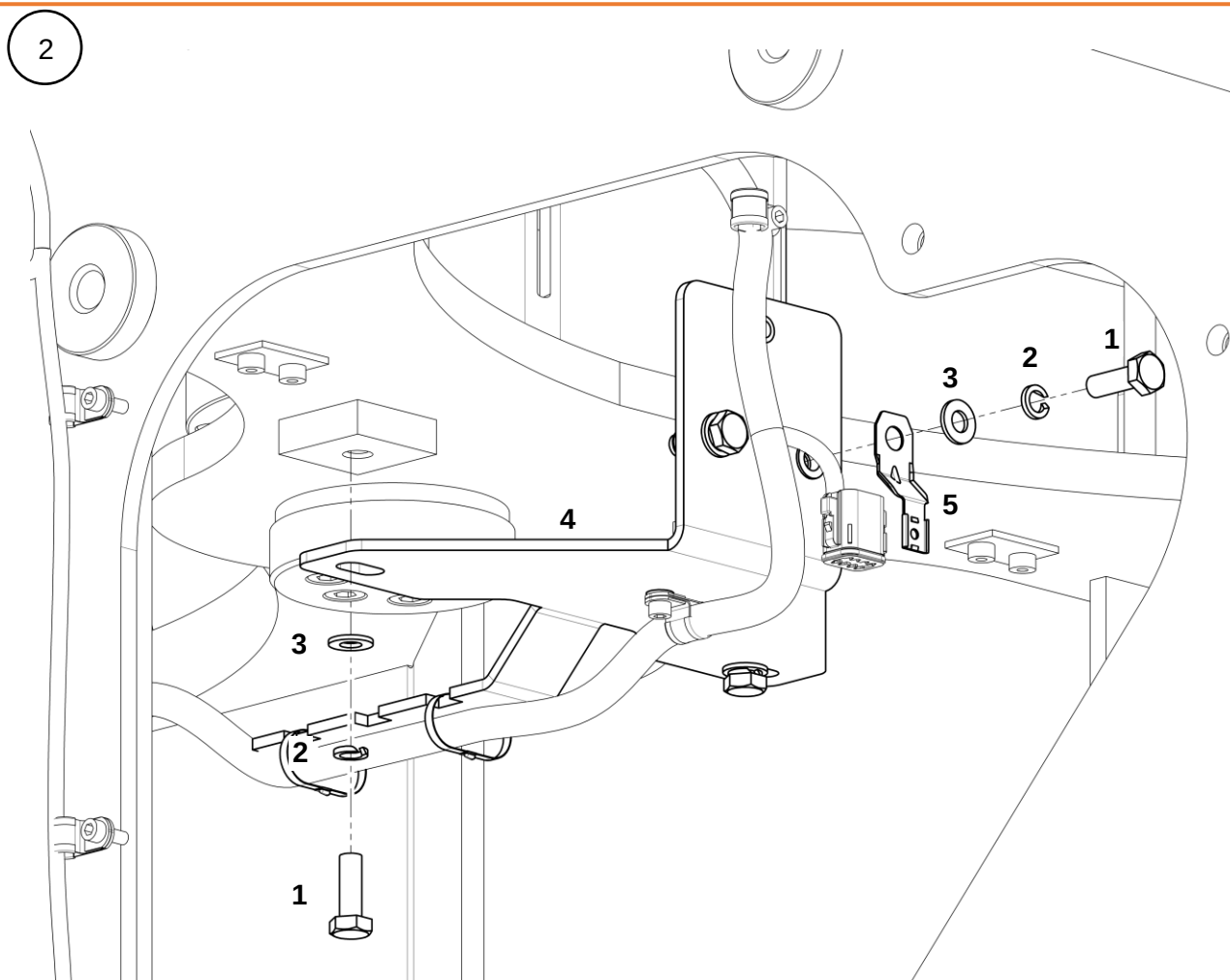
Кронштейн с крепежом
