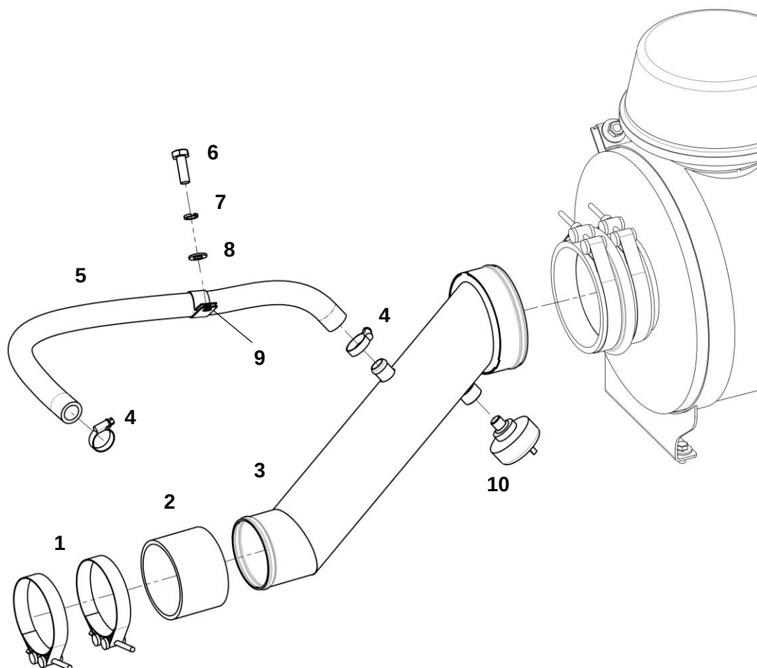
Система впуска воздуха и выпуска ОГ
