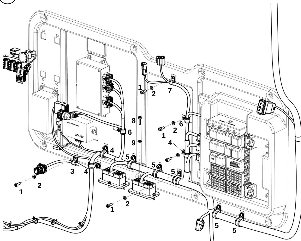
Соединение с панелью
