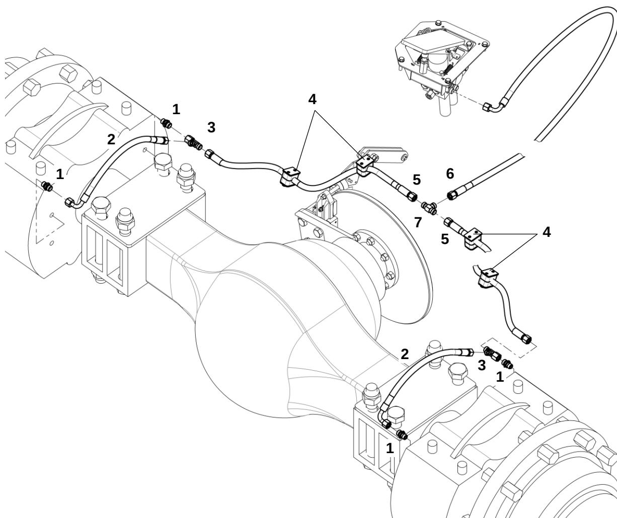
Гидравлика тормозной системы
