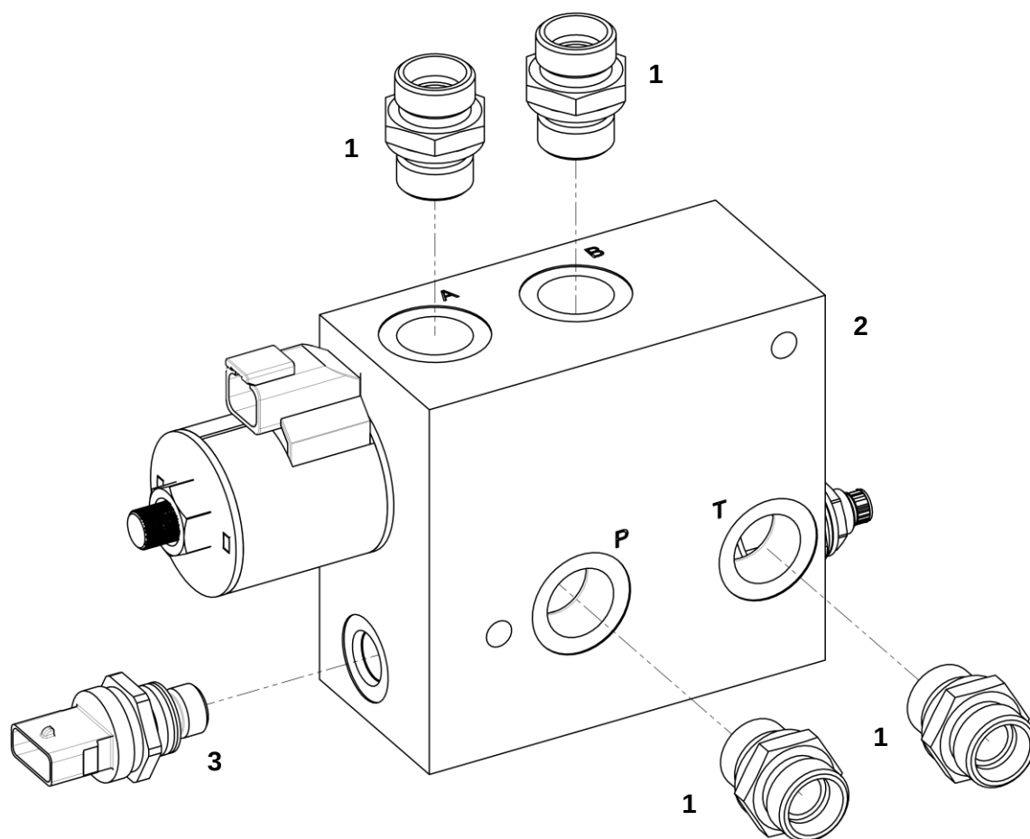
Клапанная коробка в сборе
