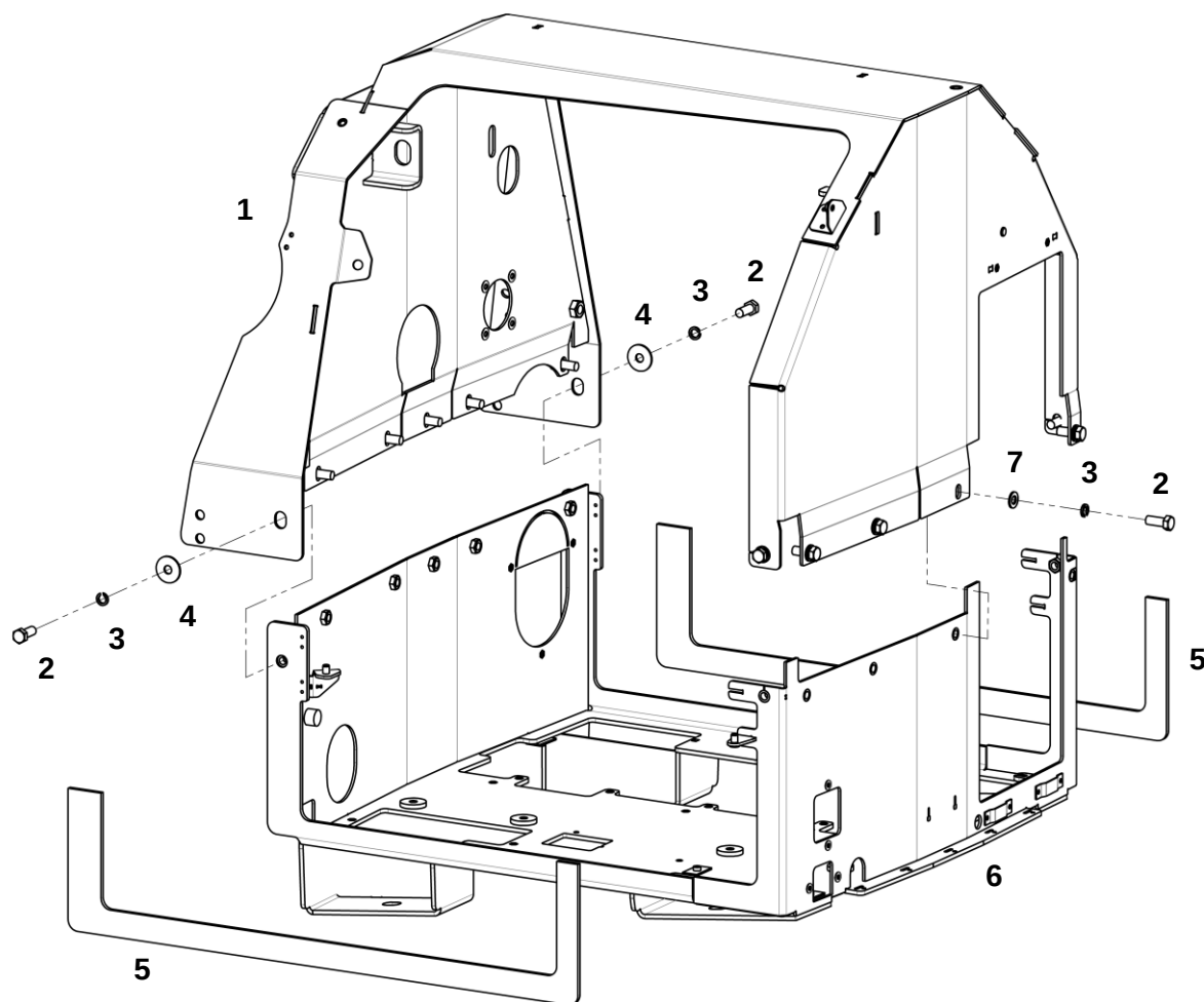
Каркас блока радиатора
