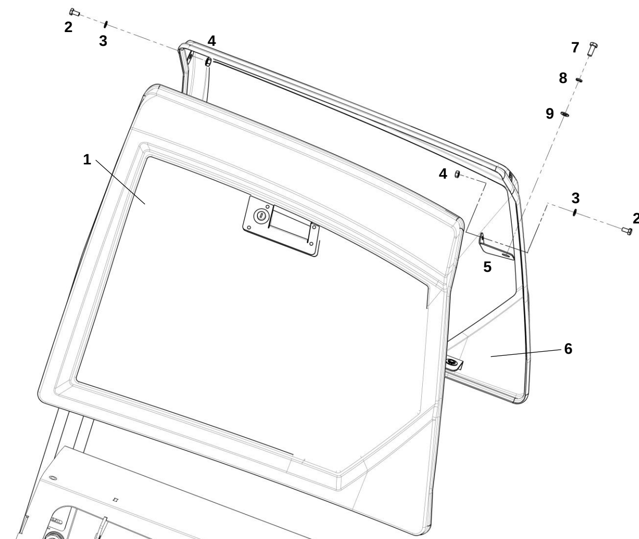
Створки блока радиатора
