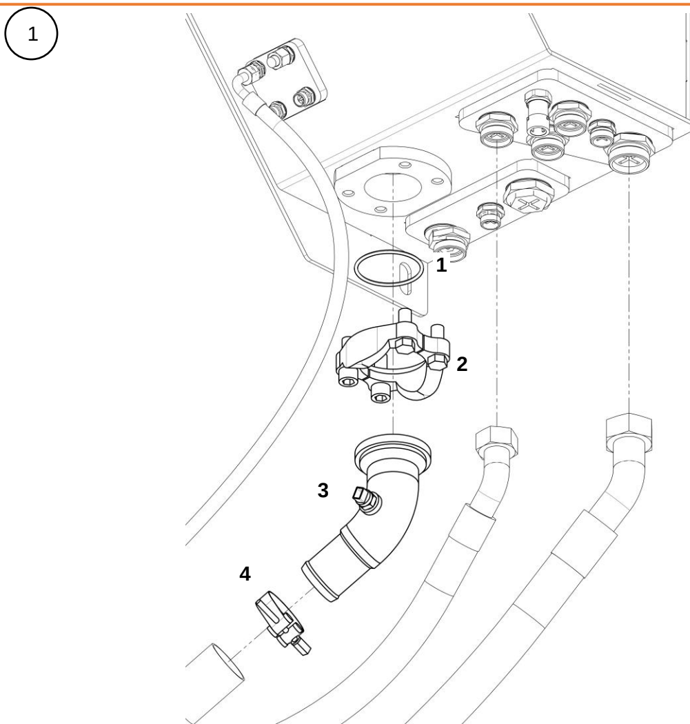
Соединение с гидравлическим баком
