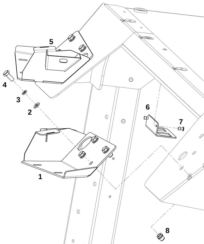
Установка панелей
