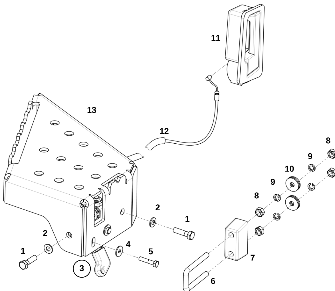
Механизм стопорения двери
