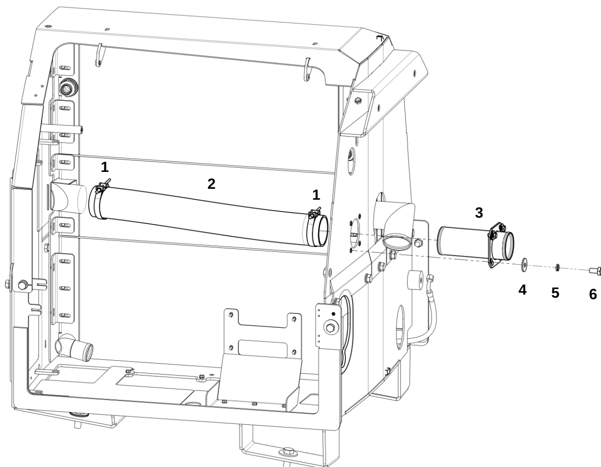
Корпус блока радиатора в сборе
