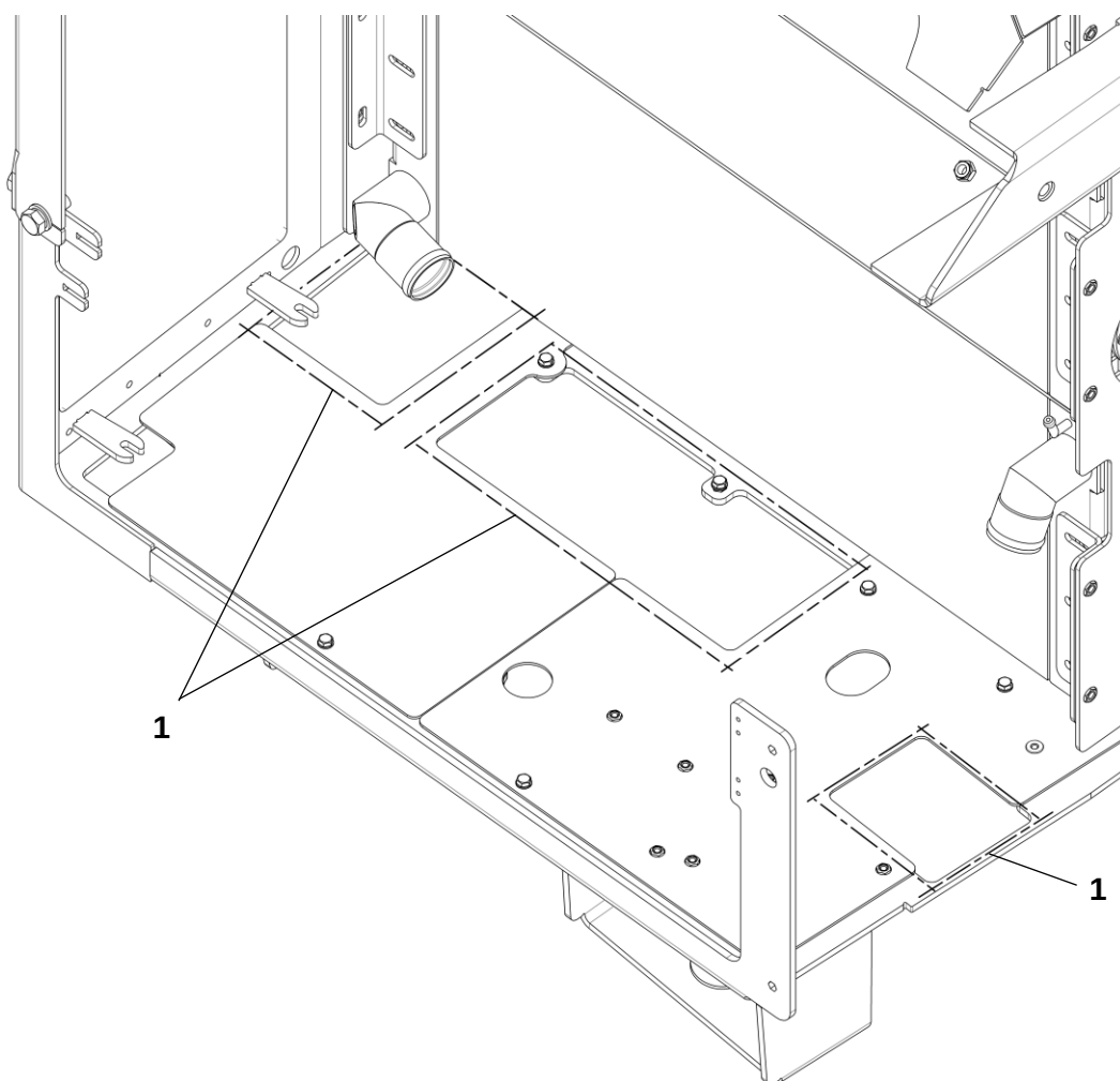
Корпус блока радиатора в сборе
