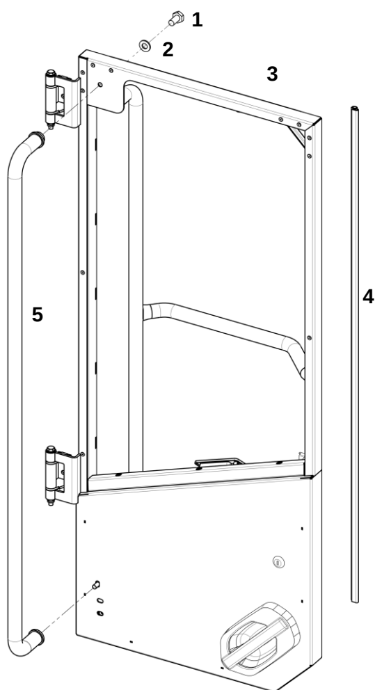
Дверь в сборе
