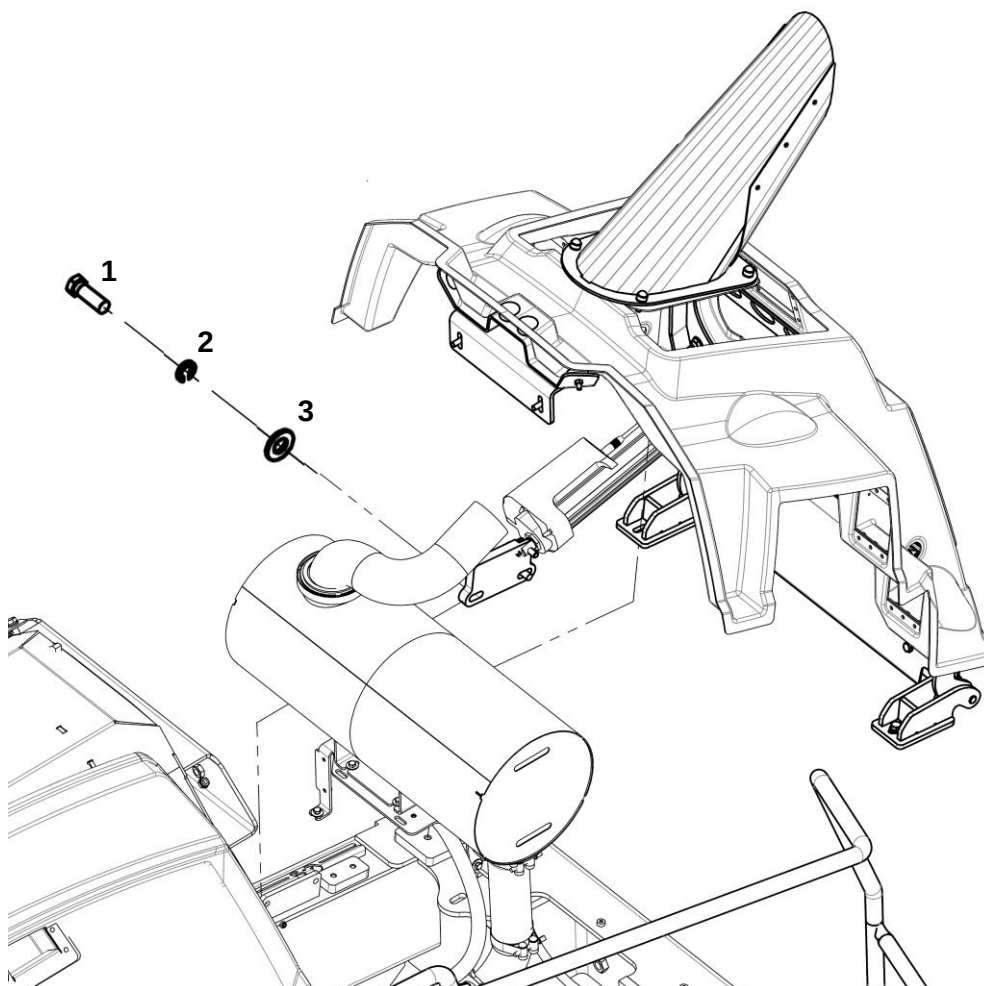
Установка капота
