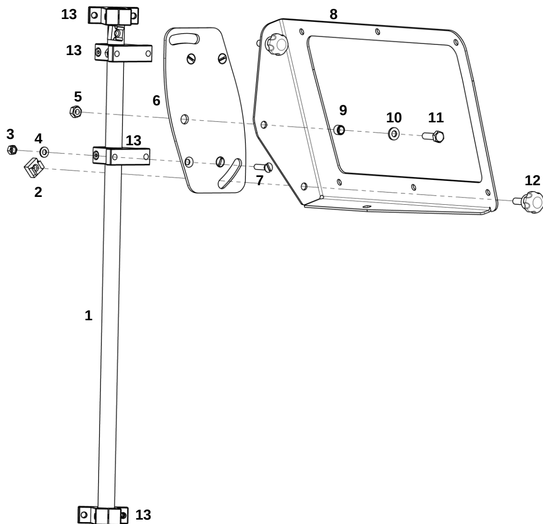
Кронштейн дисплея
