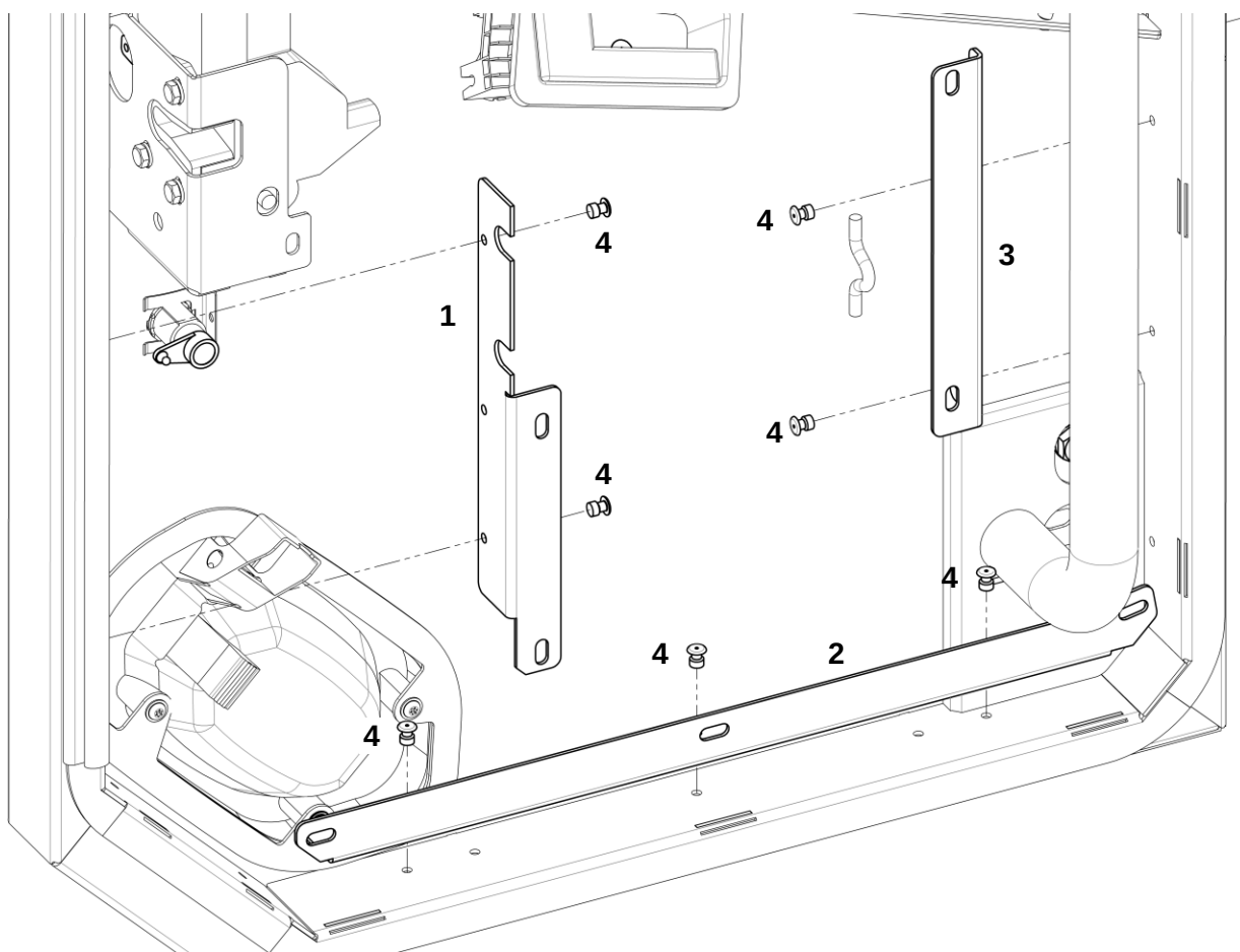
Дверь в сборе
