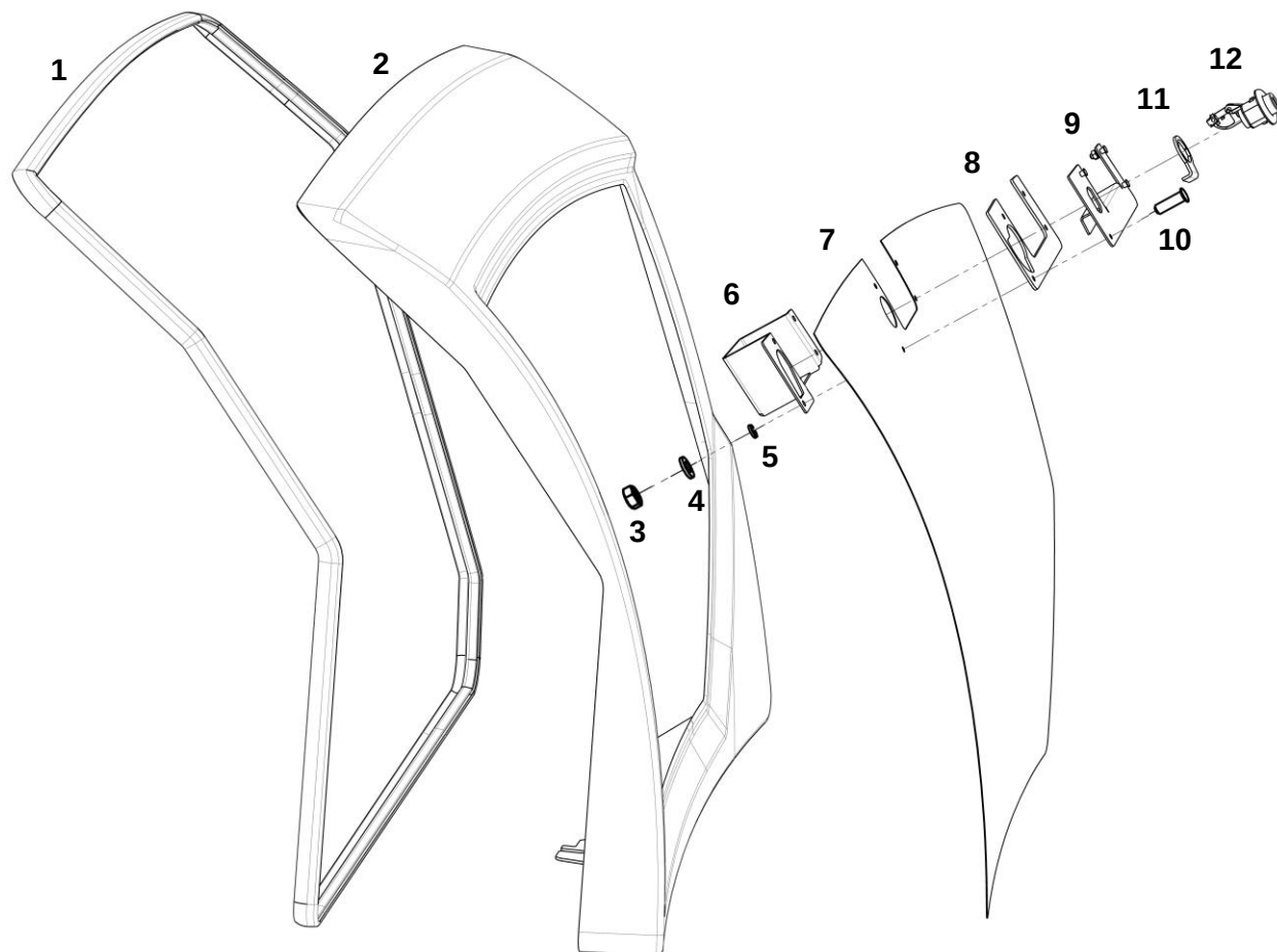
Створка в сборе
