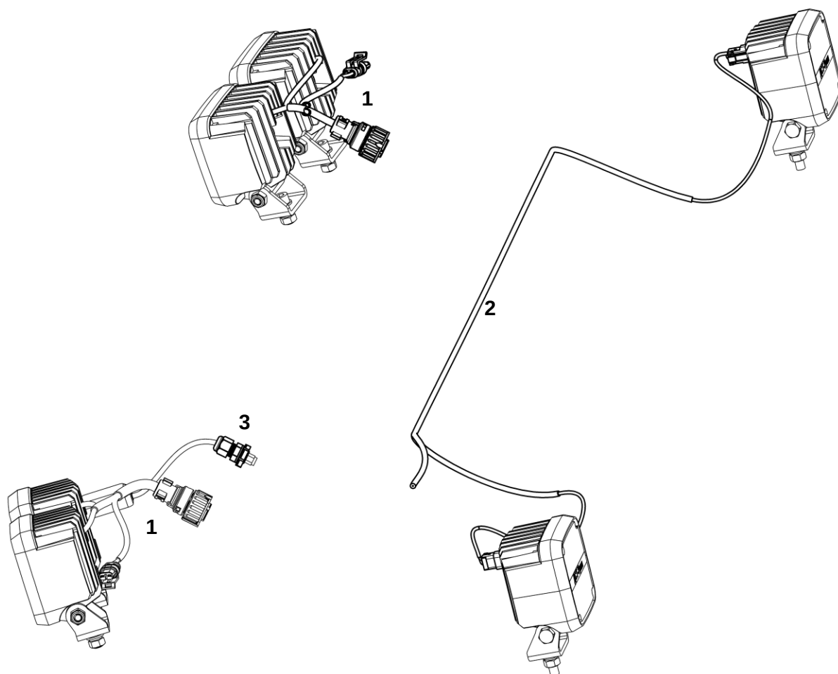
Элементы освещения кабины
