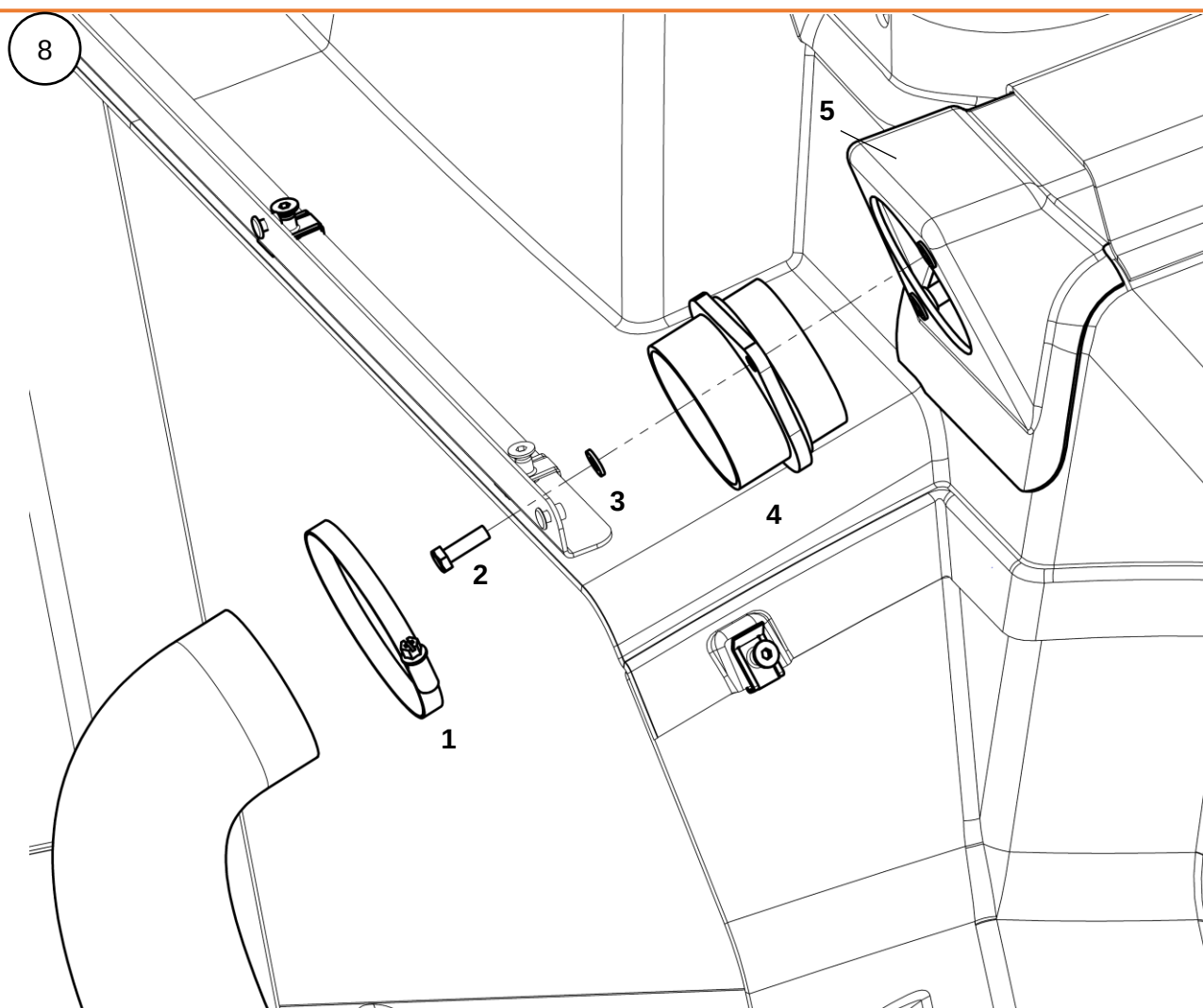
Крепление воздуховода
