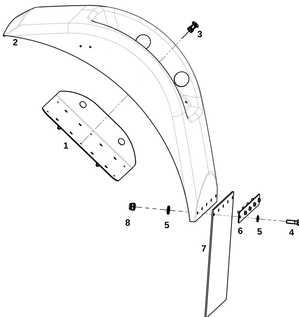
Крыло
