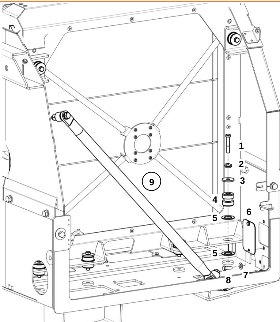
Корпус блока радиатора в сборе
