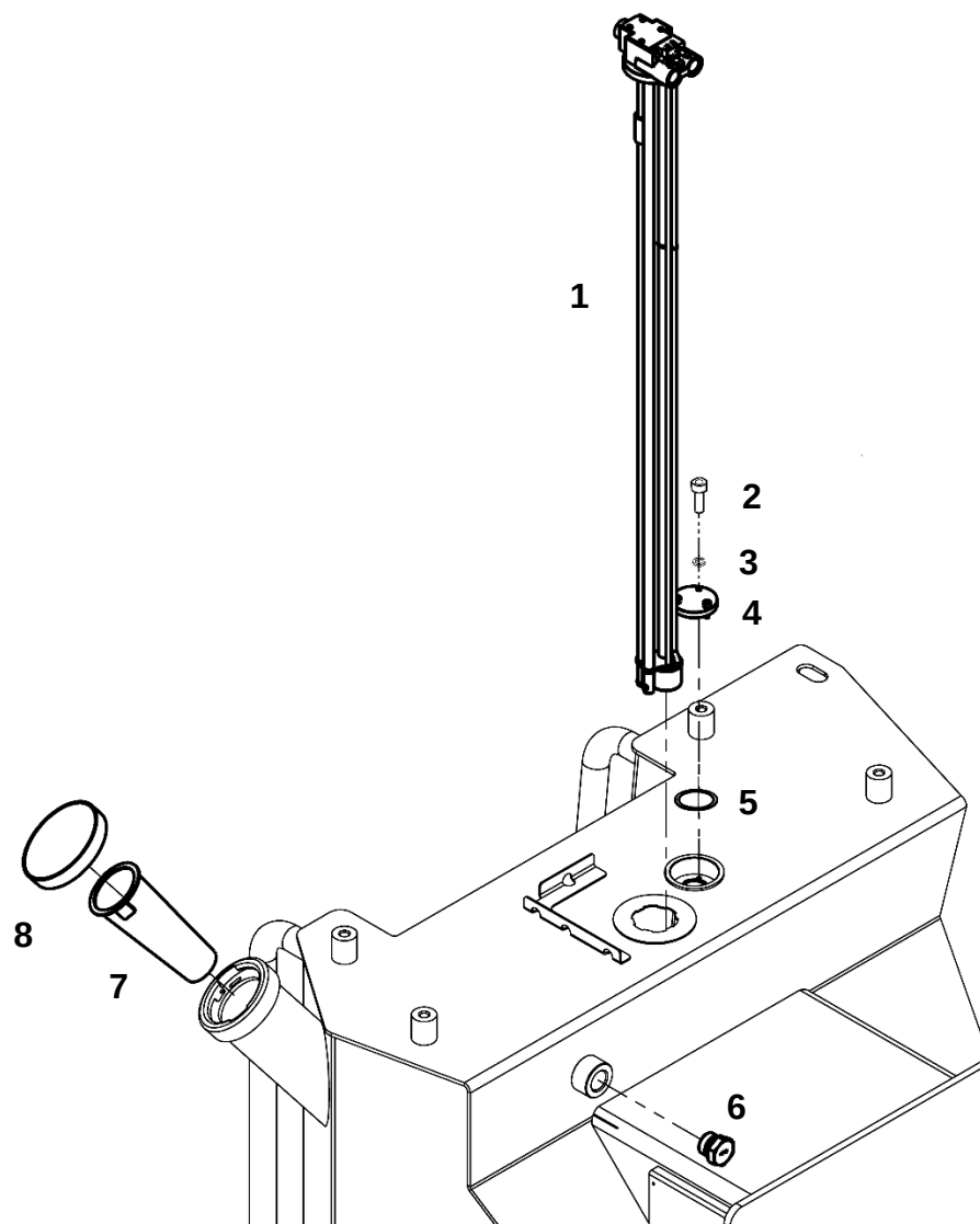
Топливный бак в сборе
