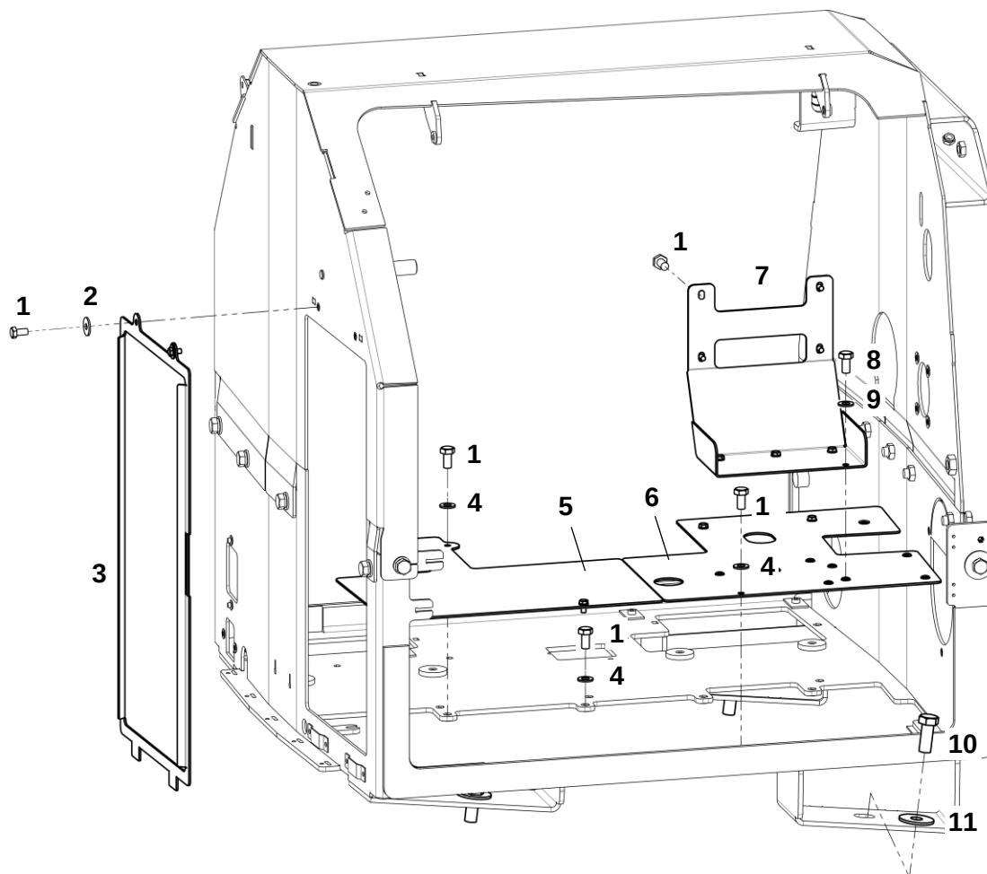
Корпус блока радиатора в сборе
