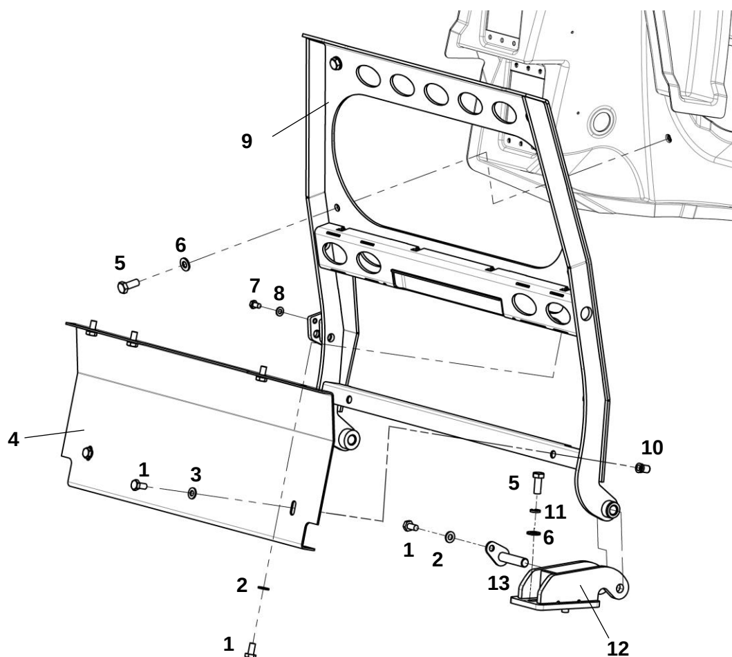
Установка капота
