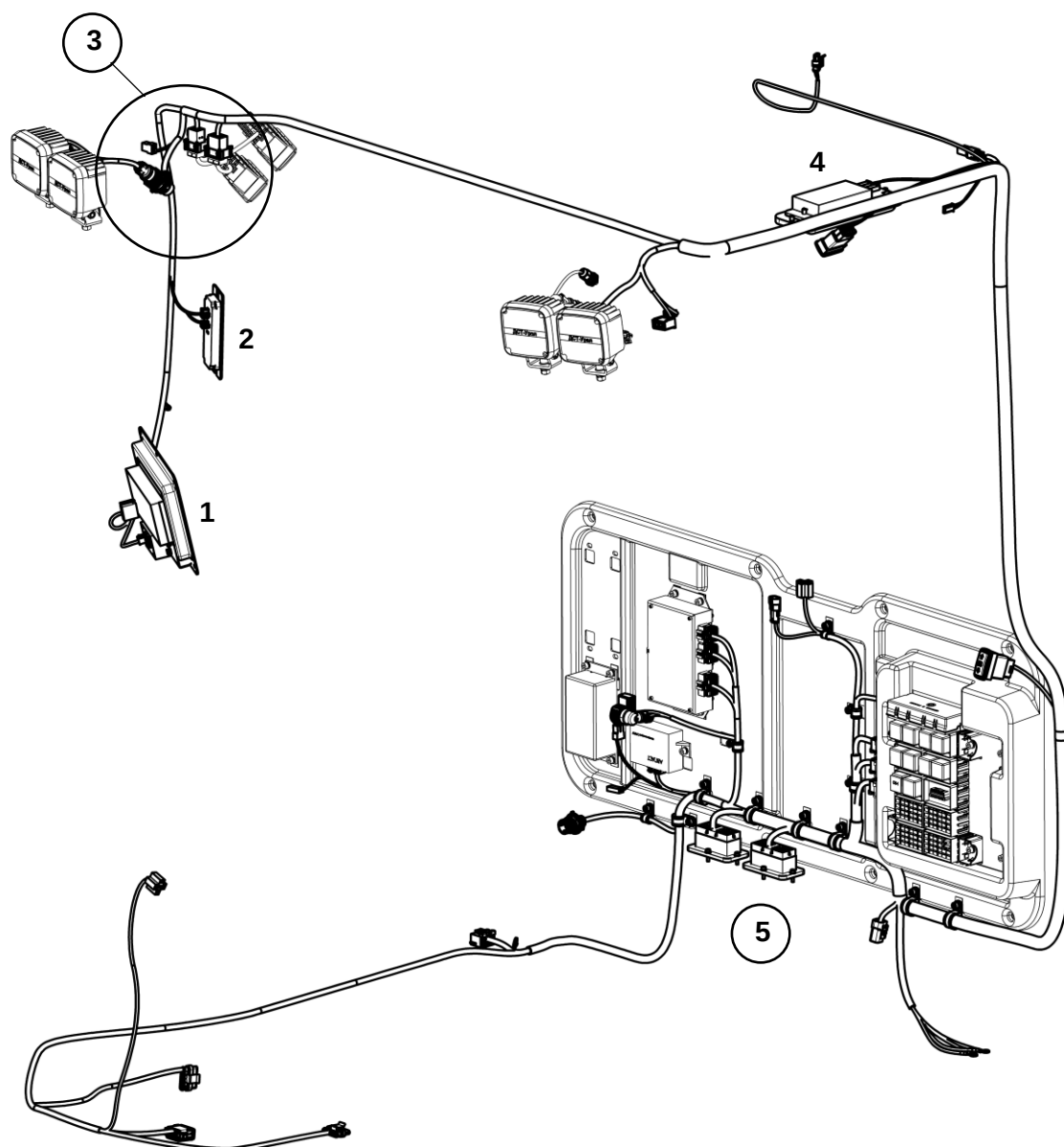
Электрооборудование кабины
