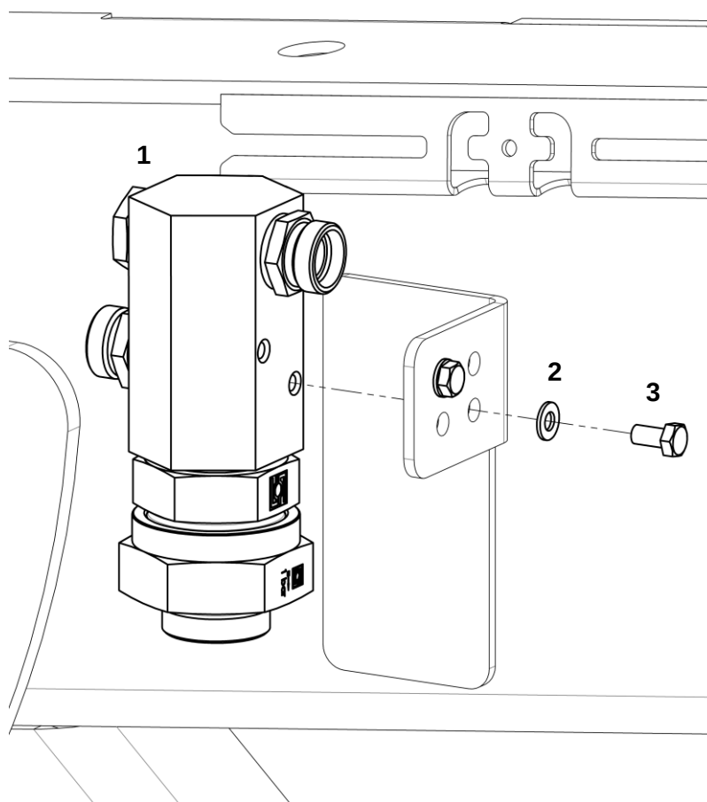
Коллектор с крепежом
