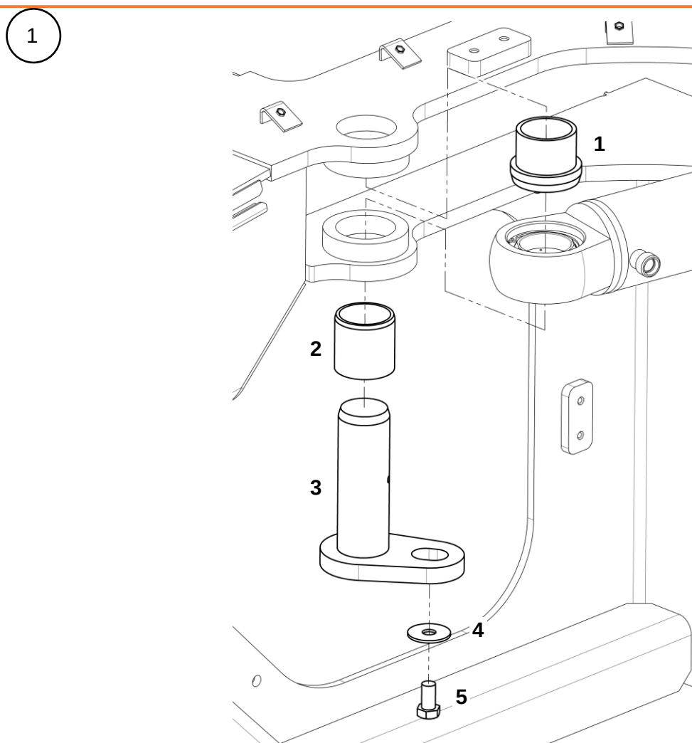
Крепление гидроцилиндров
