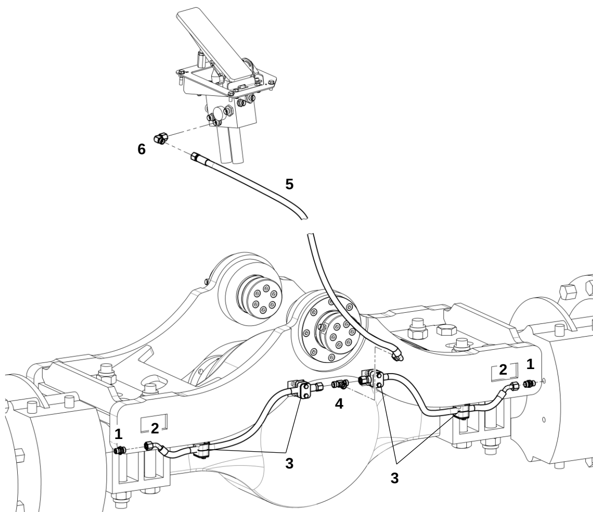
Гидравлика тормозной системы
