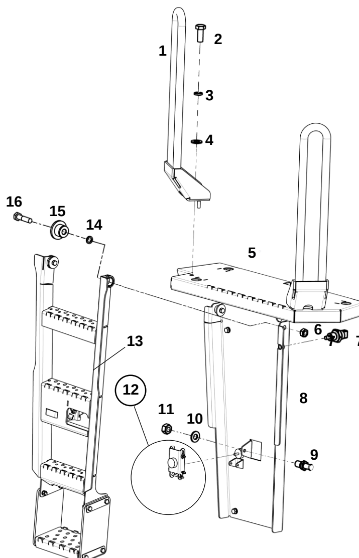
Установка лестницы
