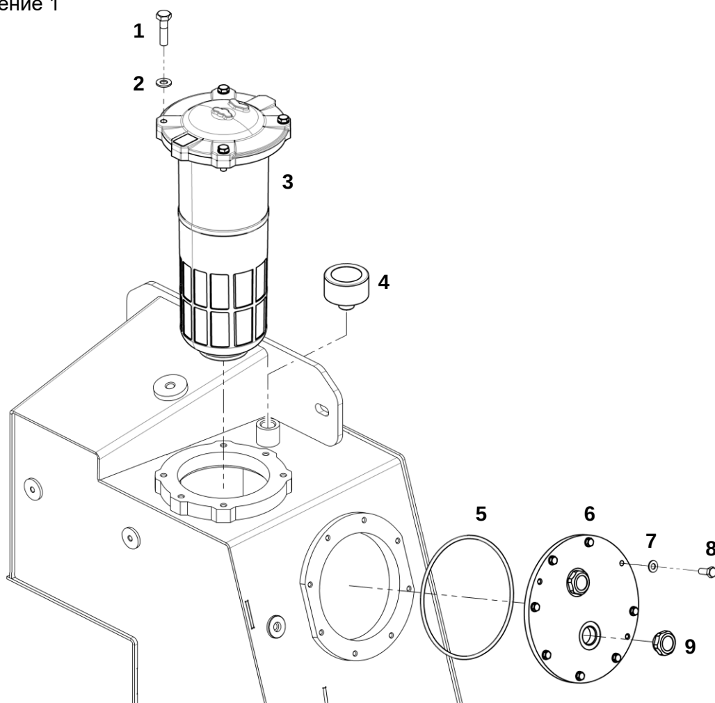
Бак гидравлический в сборе
