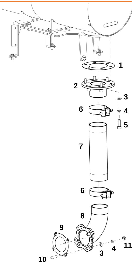
Система впуска воздуха и выпуска ОГ
