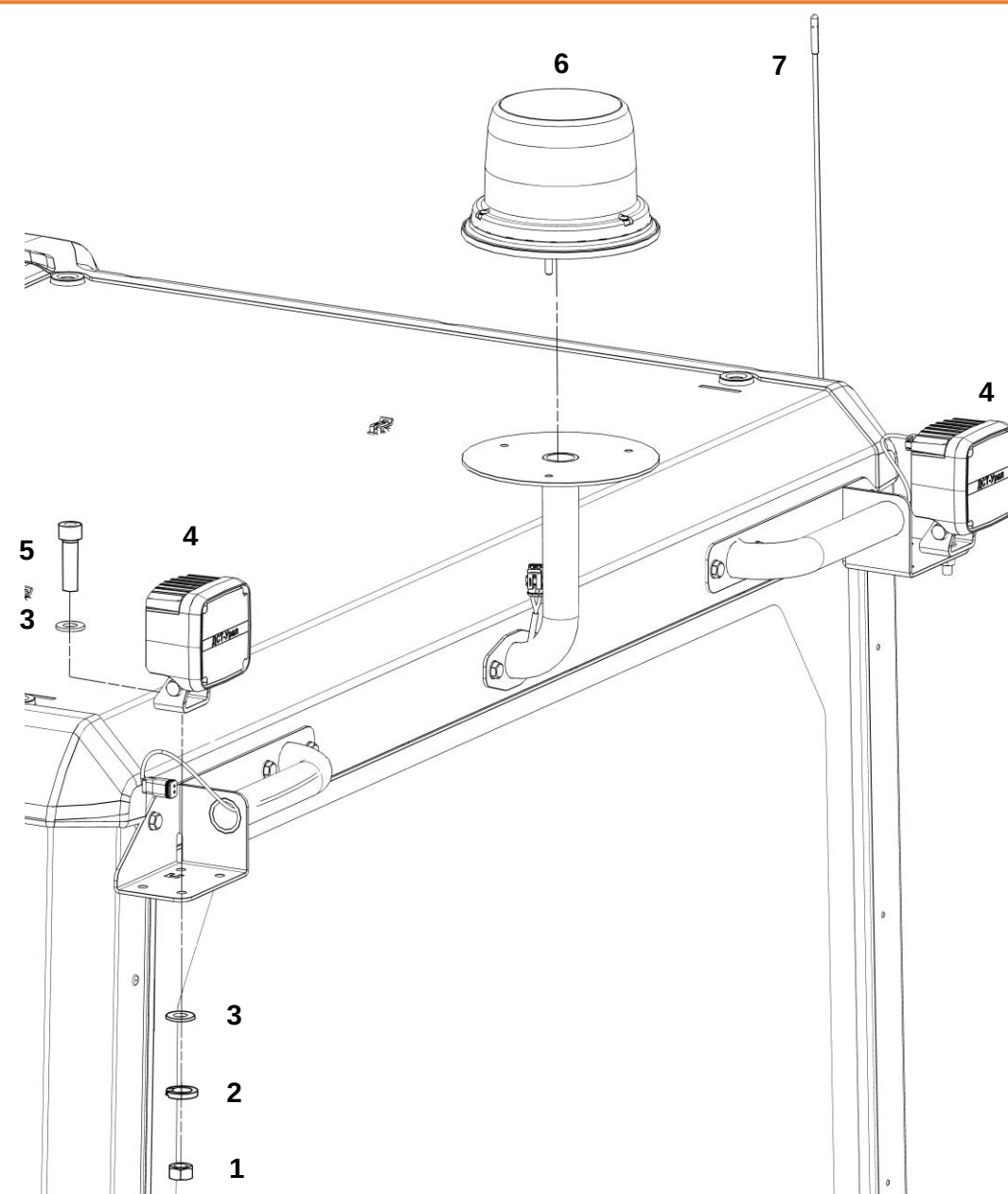
Кабина
