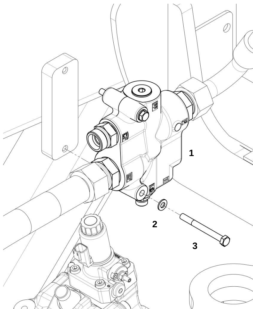
Клапан приоритета с креплением
