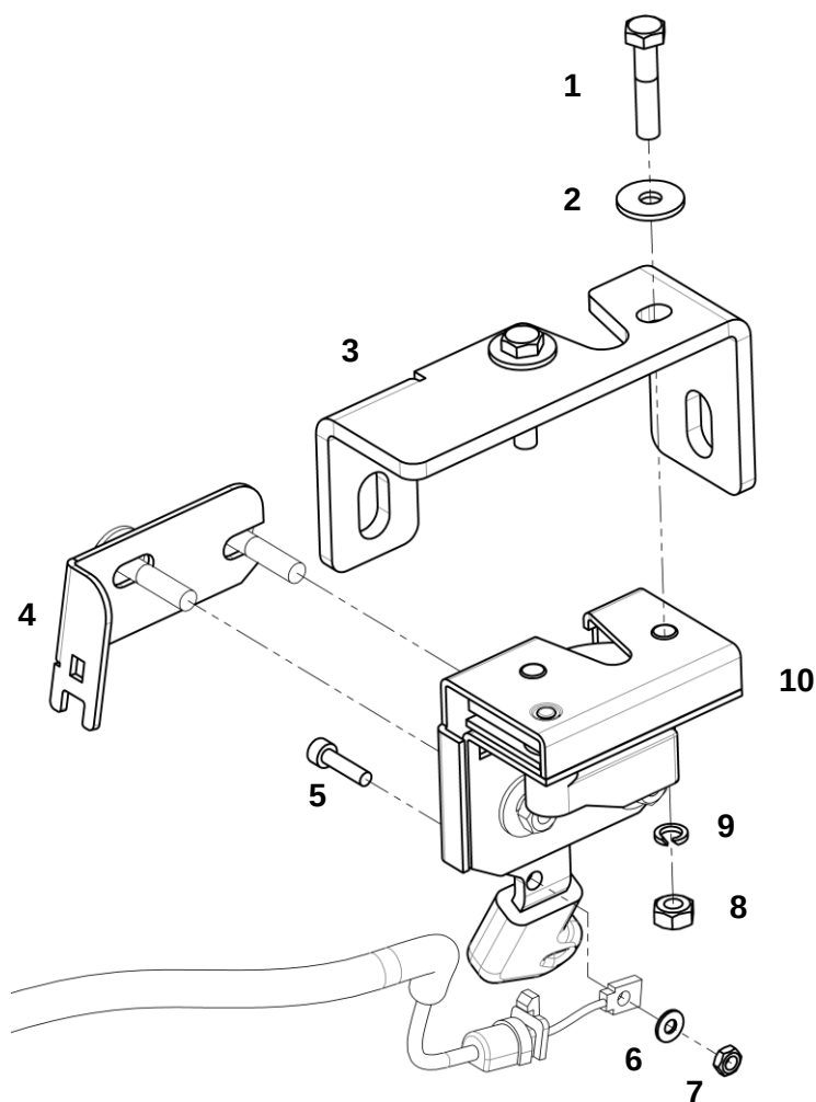
Механизм стопорения двери
