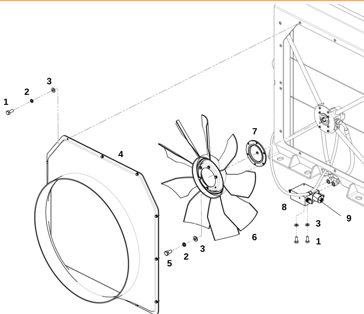
Гидропривод вентилятора
