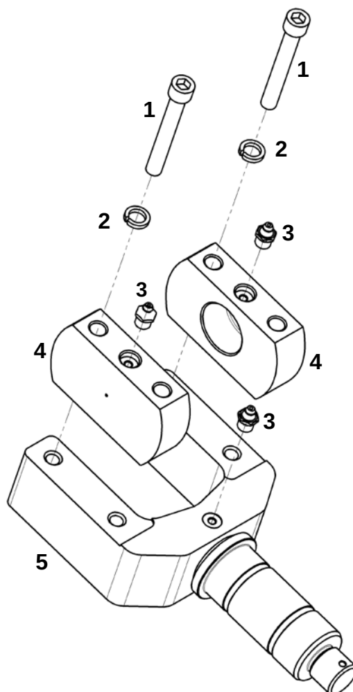
Вилка в сборке (ЯМЗ-536/238)
