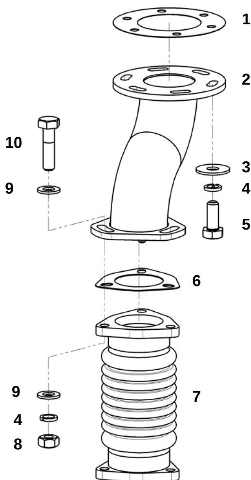
Отводы глушителя (ЯМЗ-536)
