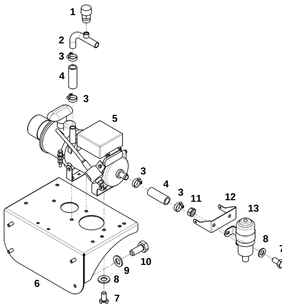
Установка ПЖД (ЯМЗ-238)
