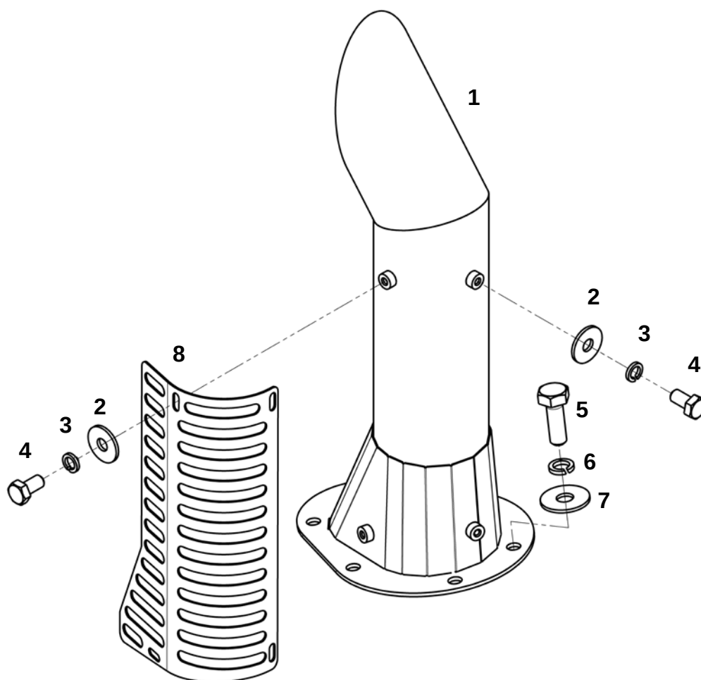
Труба выхлопная в сборе (ЯМЗ-238)
