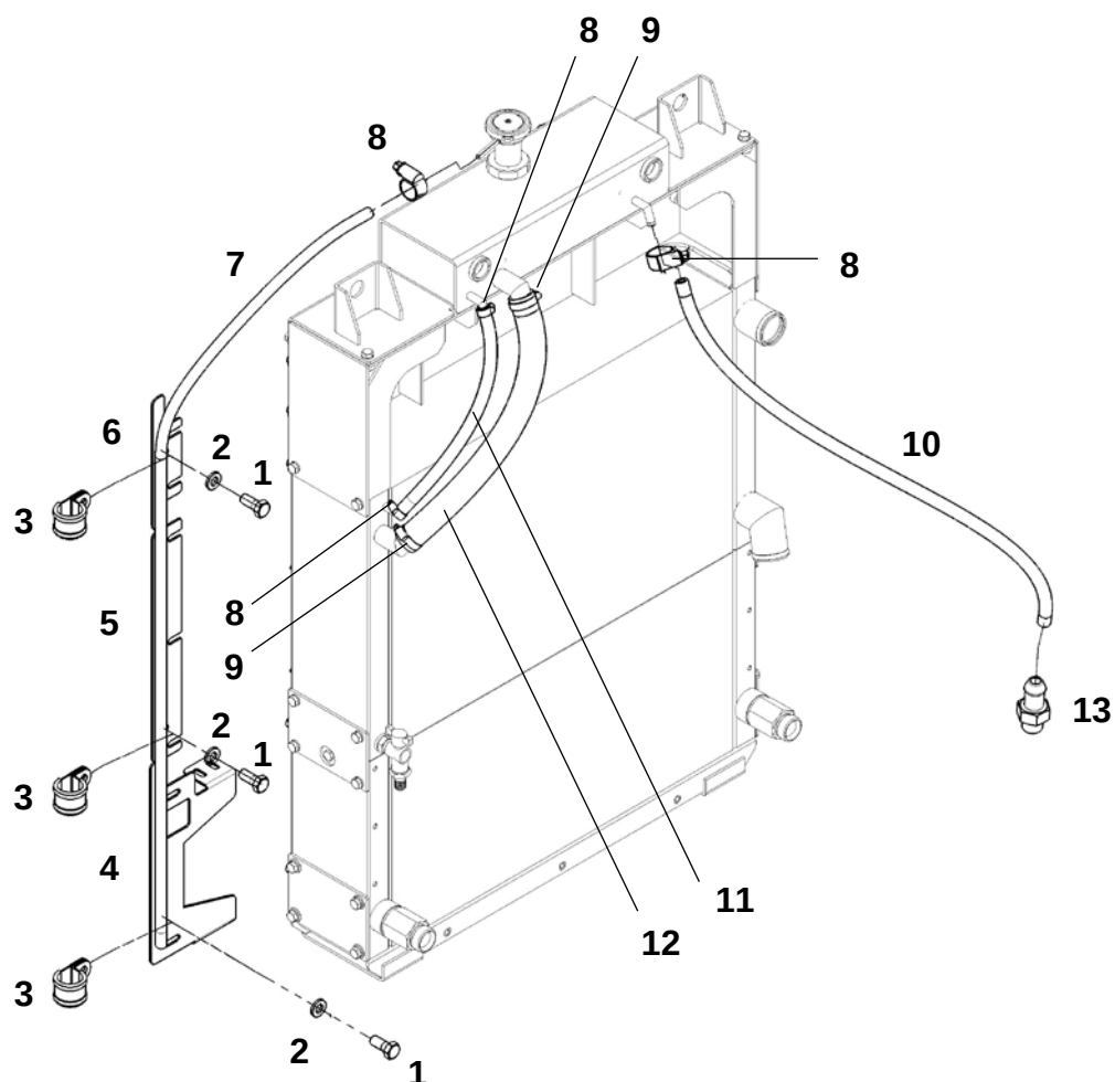
Рукава спуска воздуха (ЯМЗ-238)
