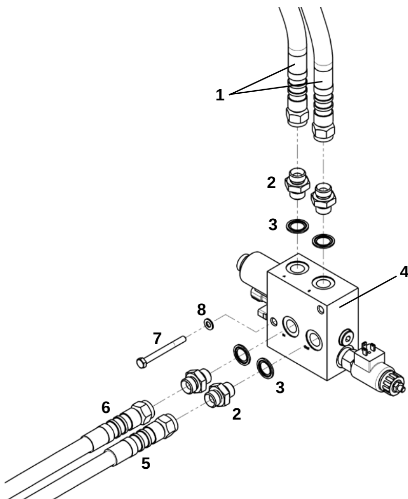
Клапанный блок в сборе (ЯМЗ-536/238)
