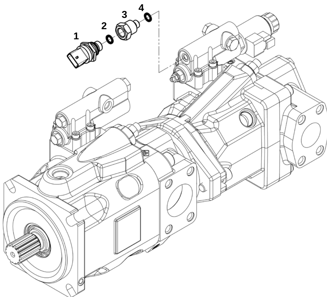
Комплект обвязки насосов гидравлических PVC85 и PVC28
