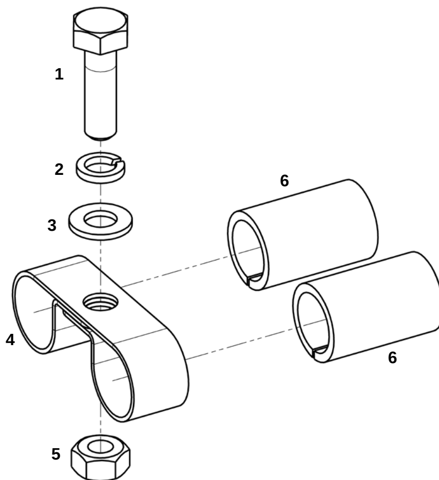
Хомут (ЯМЗ-238)
