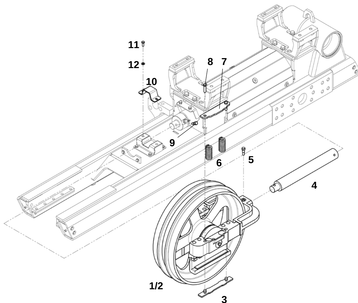
Натяжное колесо в сборе (ЯМЗ-536/238)
