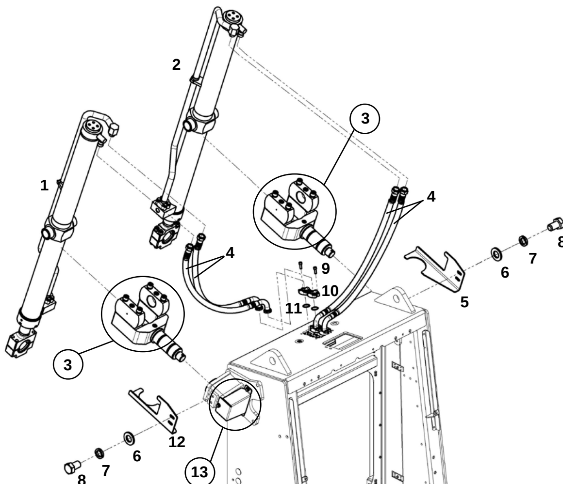
Установка гидроцилиндров (ЯМЗ-536/238)
