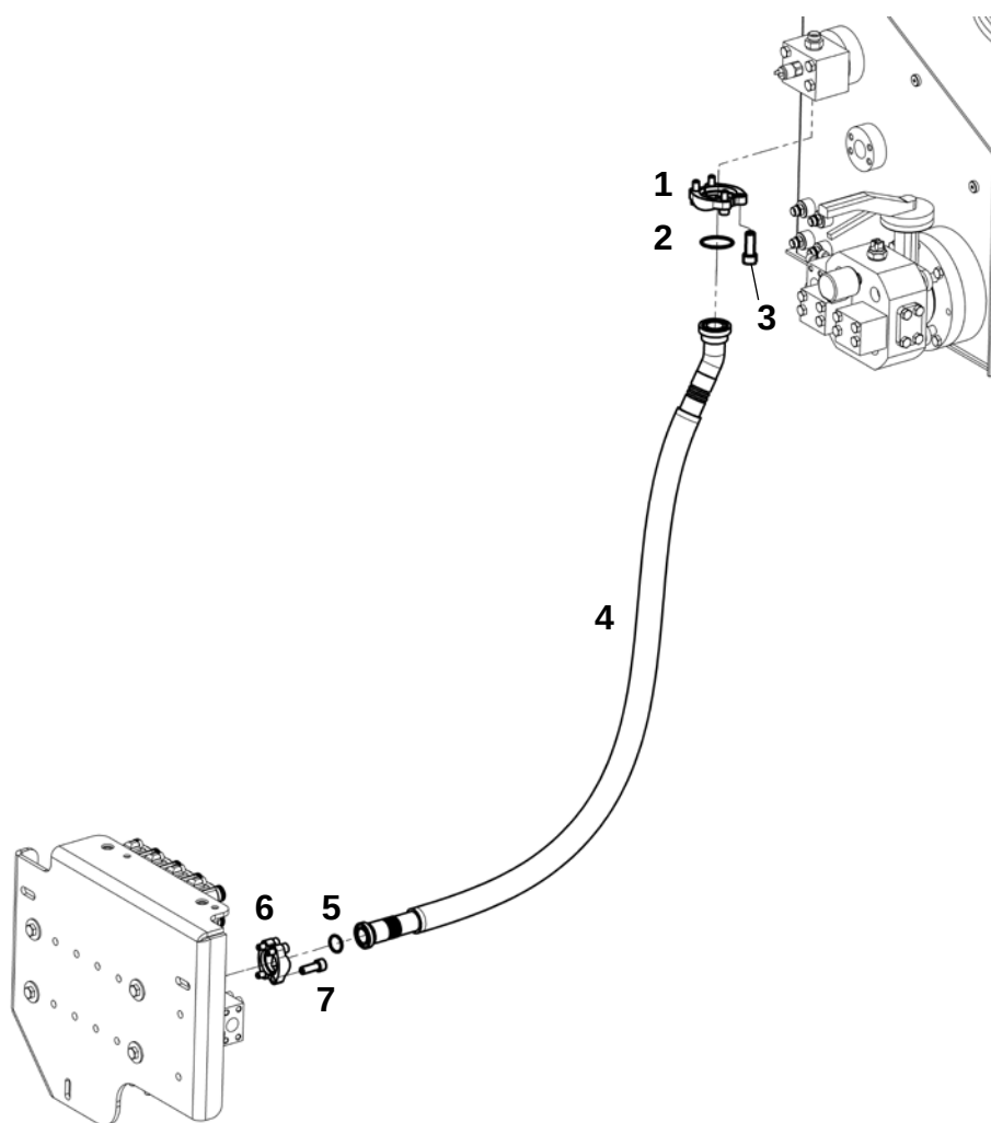
РВД (ЯМЗ-238)
