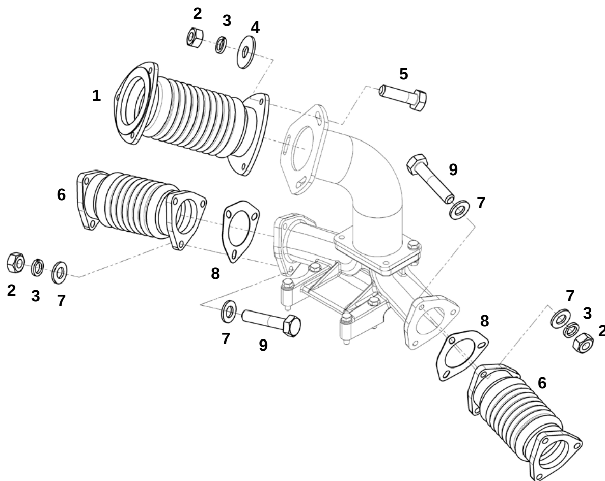
Отводы глушителя (ЯМЗ-238)
