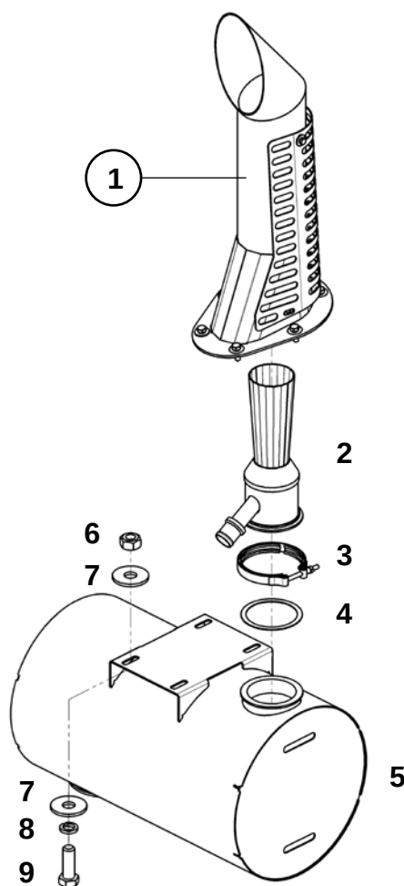
Труба выхлопная и глушитель (ЯМЗ-238)
