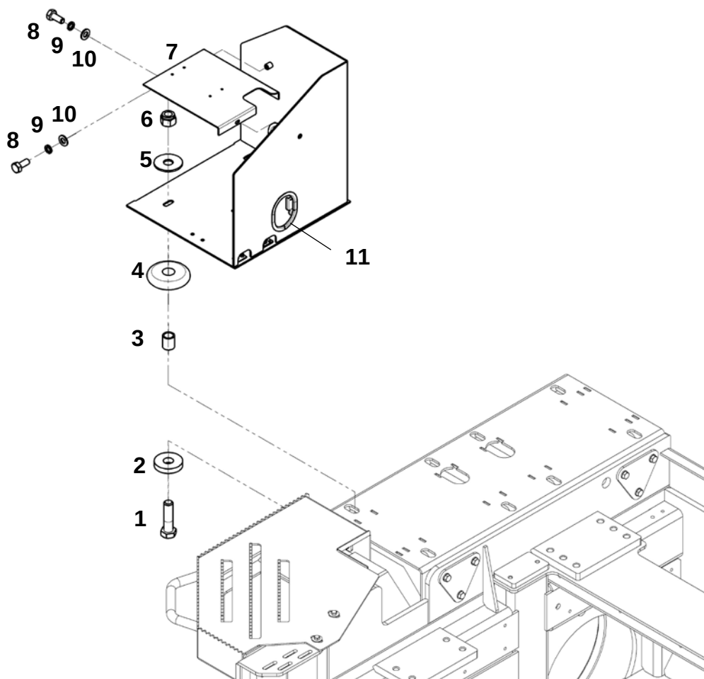
Ящик (ЯМЗ-536/238)
