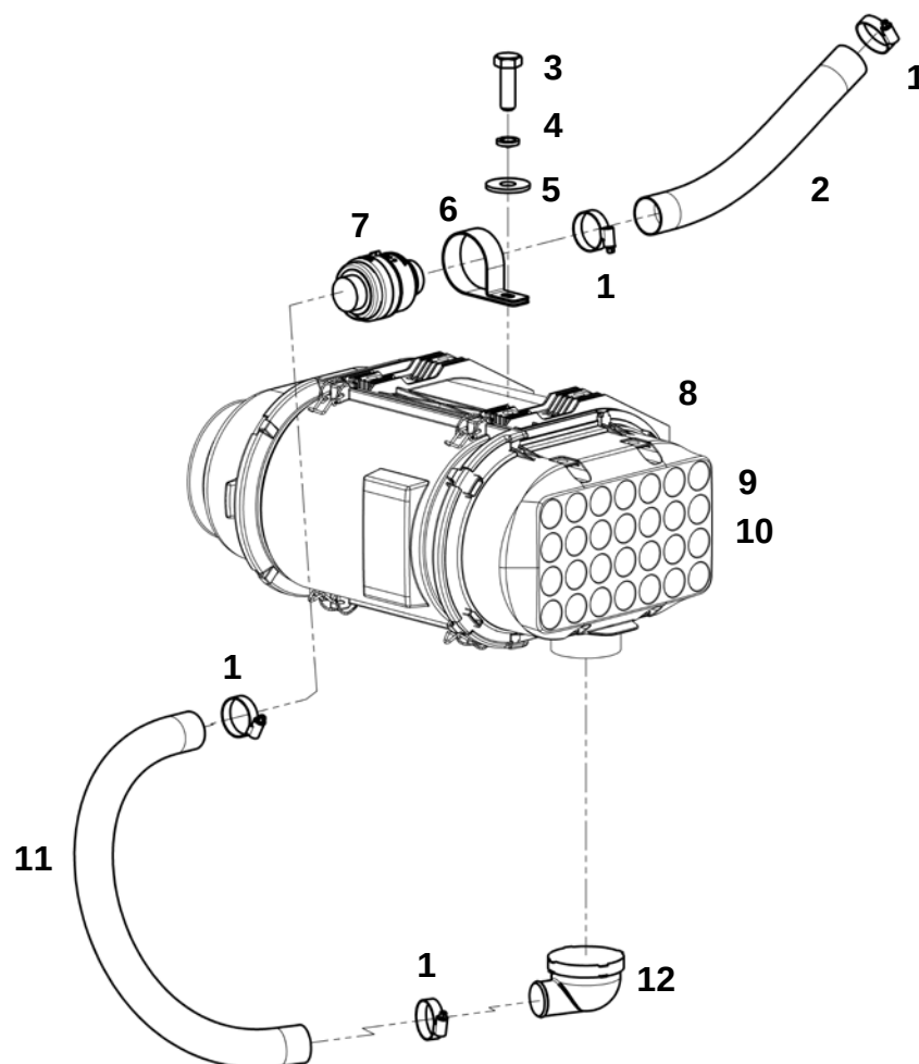
Воздушный фильтр (ЯМЗ-238)
