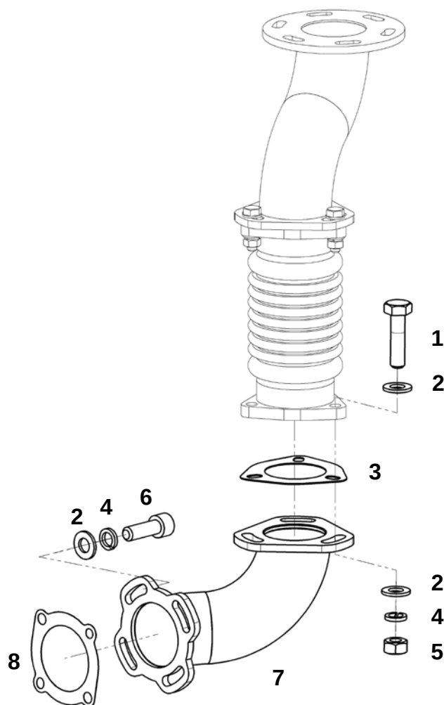
Отводы глушителя (ЯМЗ-536)
