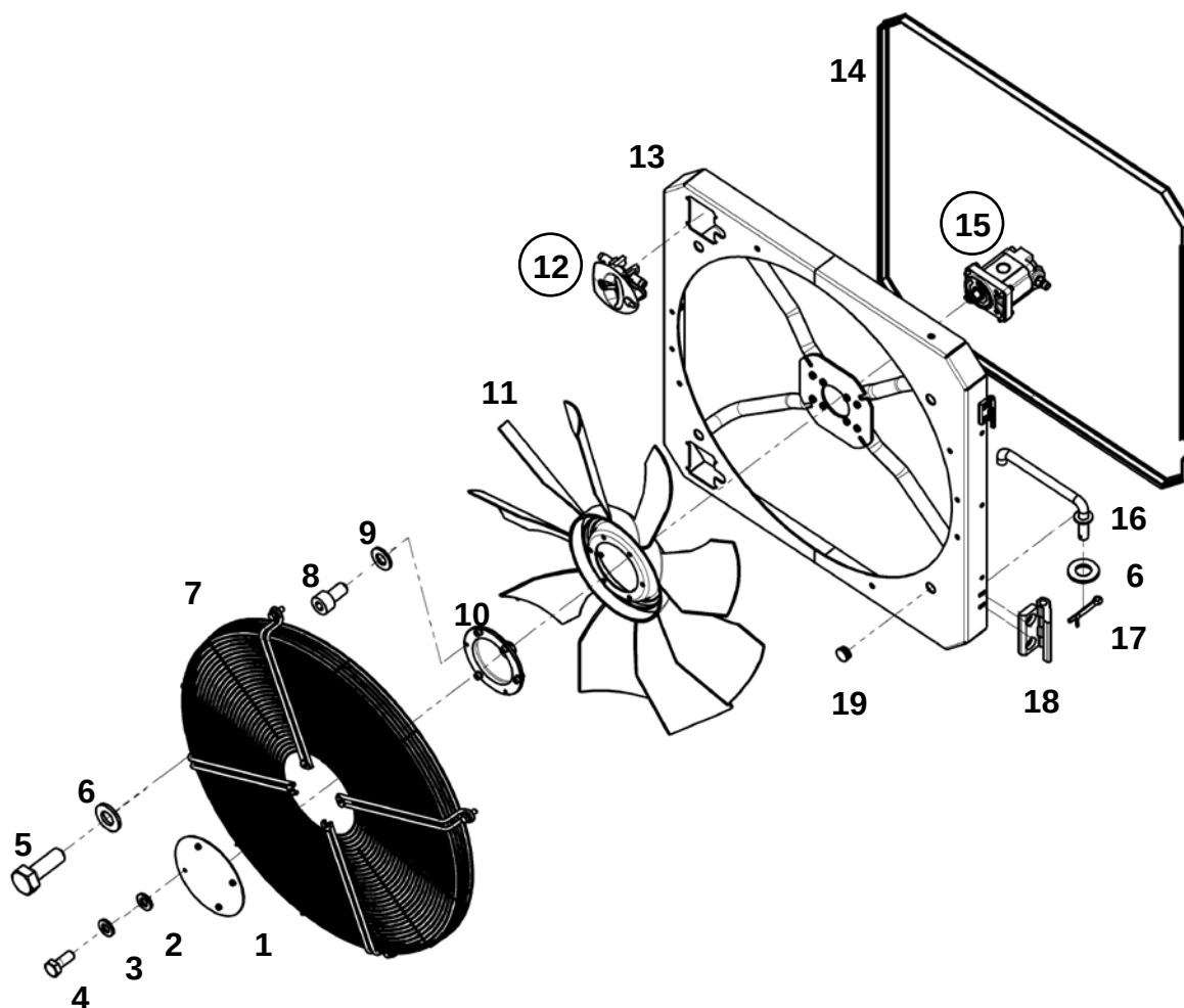
Рама с вентилятором (ЯМЗ-536/238)
