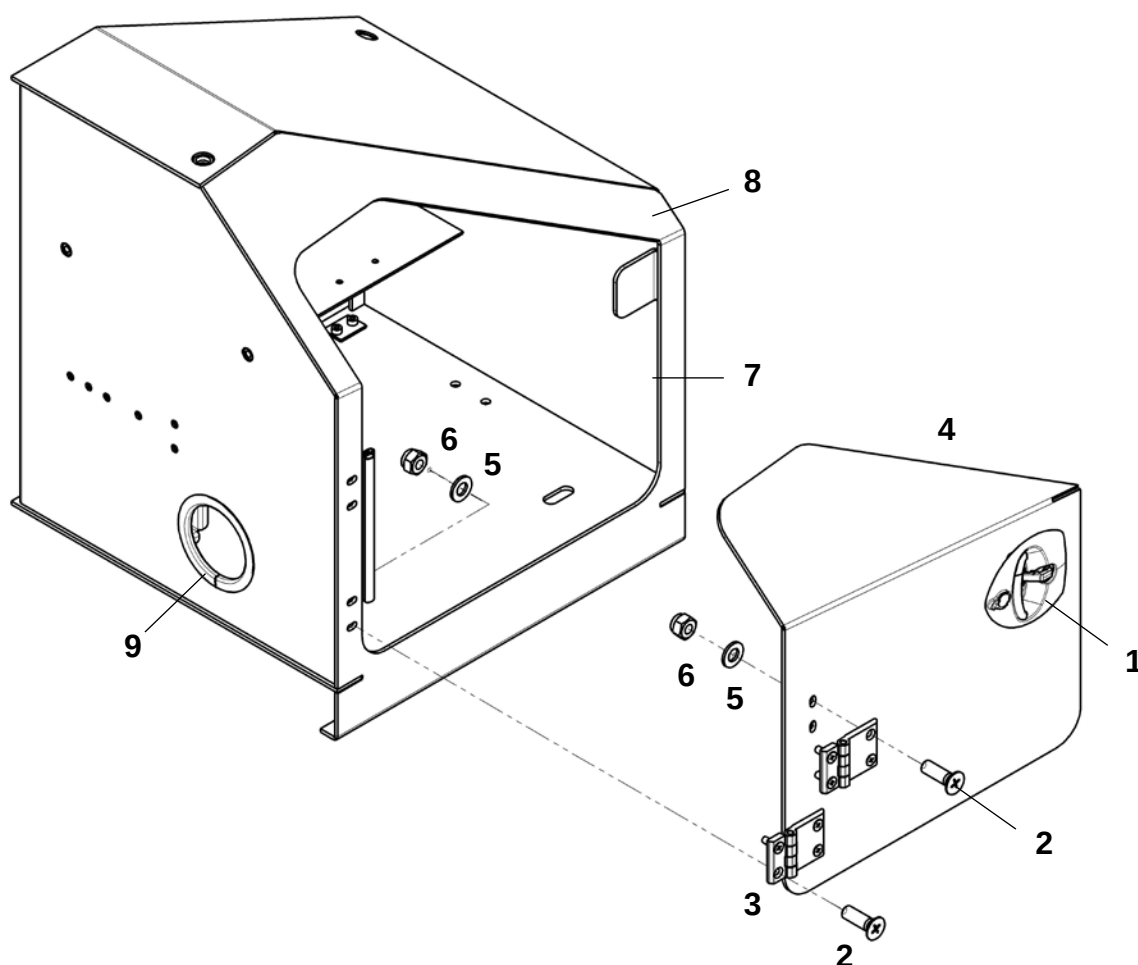
Ящик (ЯМЗ-536/238)
