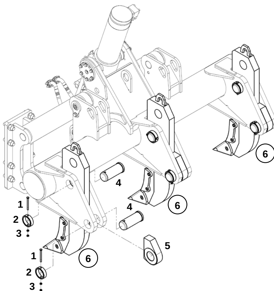
Крепление ножа трехзубого рыхлителя
