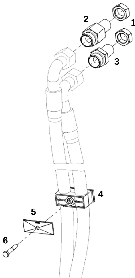
РВД (ЯМЗ-536/238)
