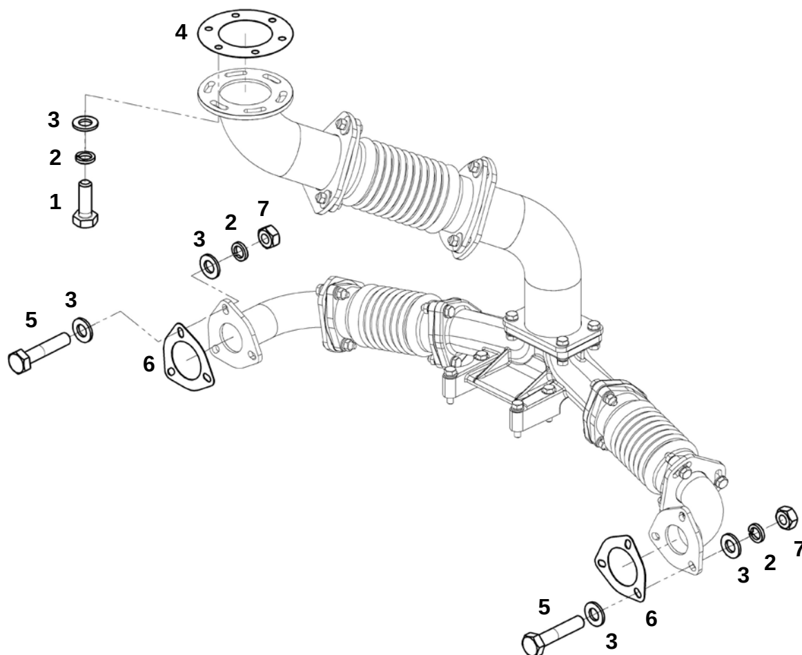
Отводы глушителя (ЯМЗ-238)
