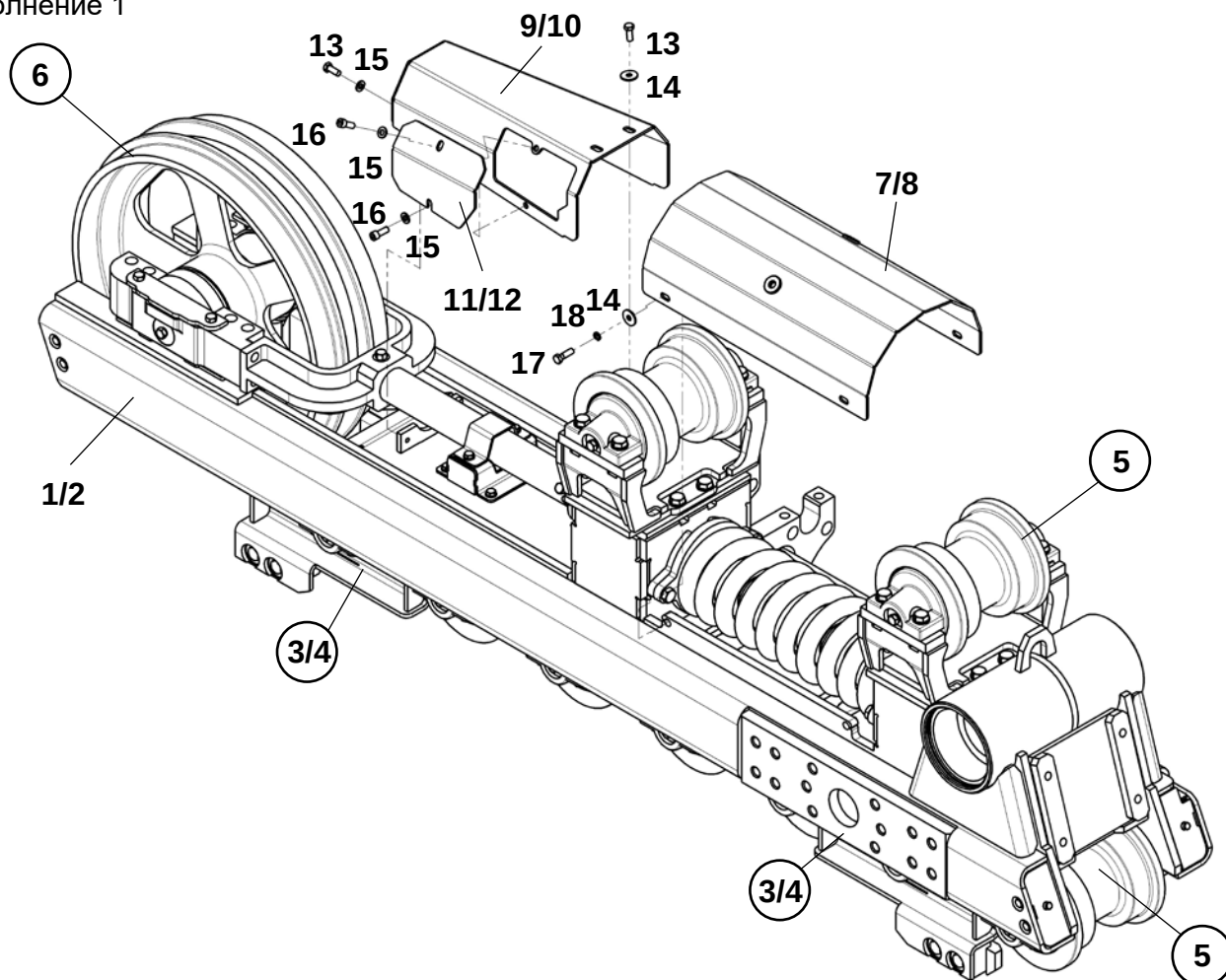
Тележка ходовая в сборе (ЯМЗ-536/238)
