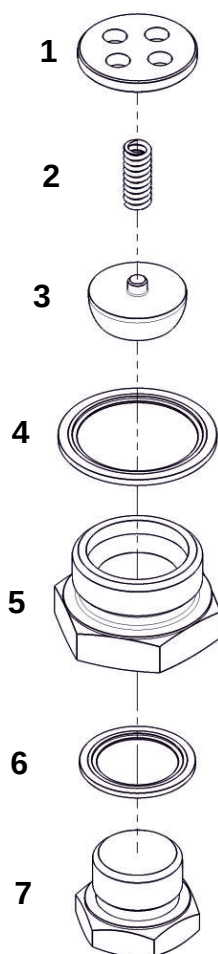
Пробка сливная (ЯМЗ-536/238)
