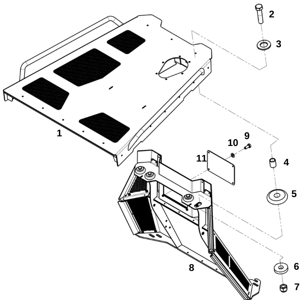
Перегородка, капот (ЯМЗ-238)
