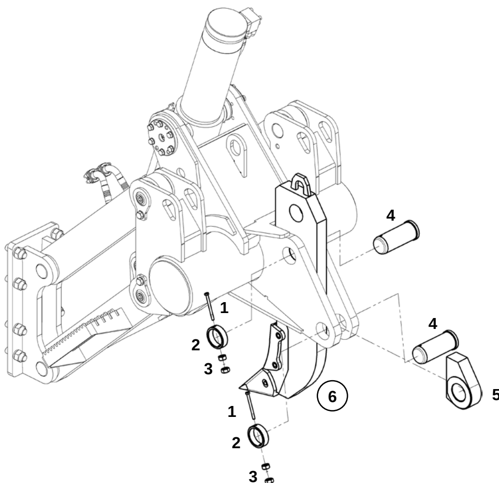
Крепление ножа однозубого рыхлителя
