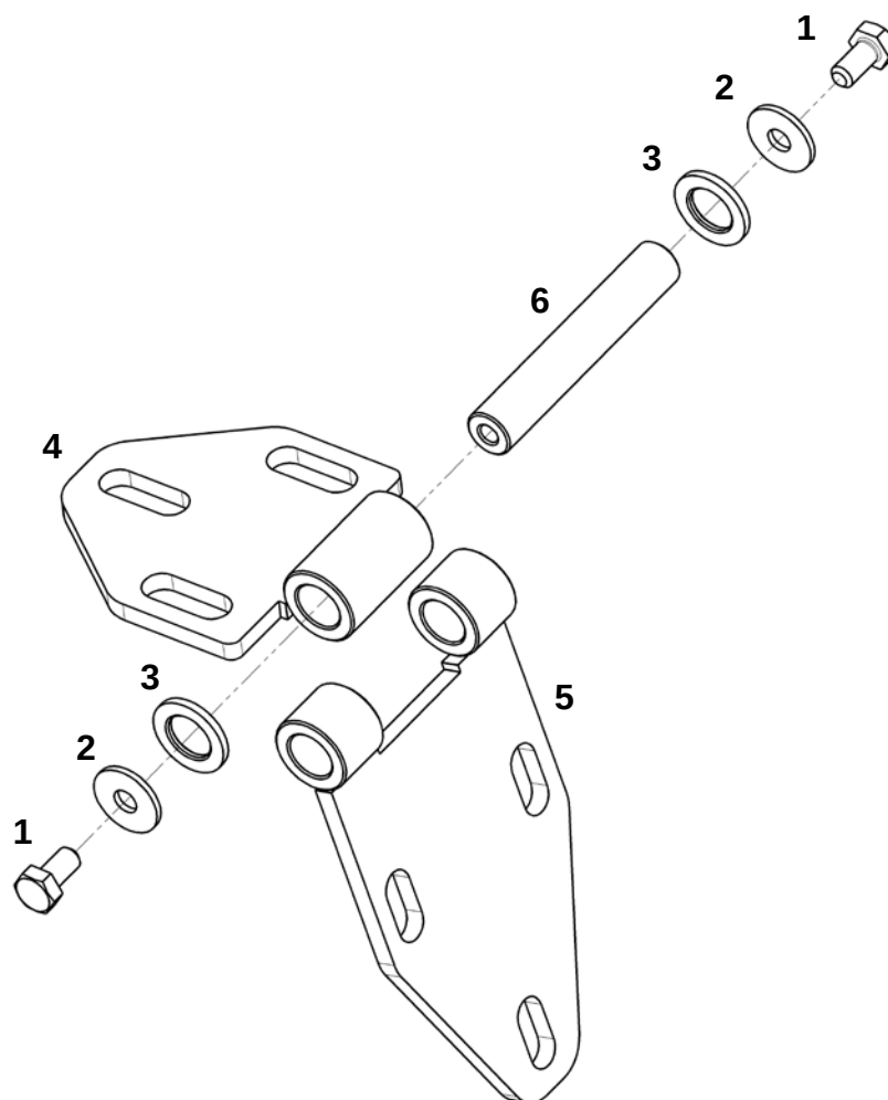
Петля в сборе (ЯМЗ-536/238)
