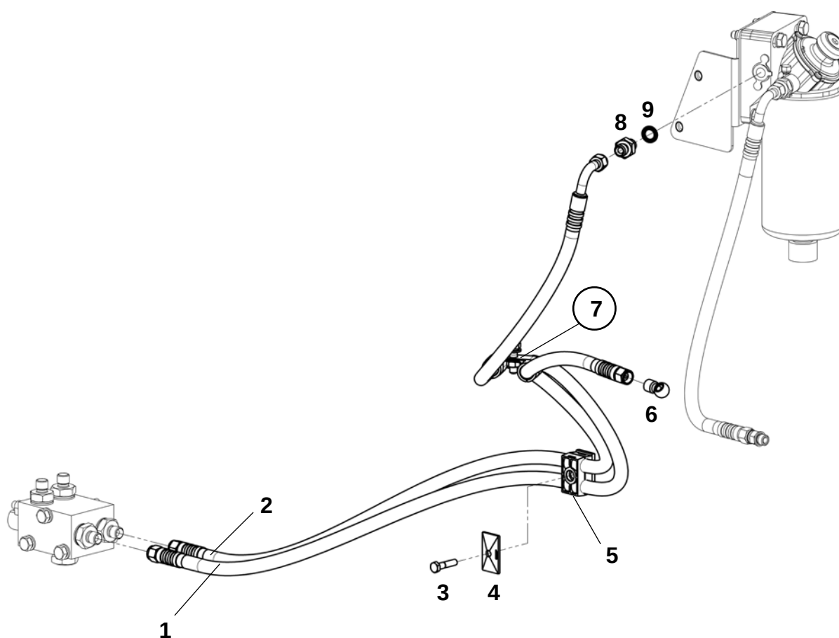
Топливопровод (ЯМЗ-238)
