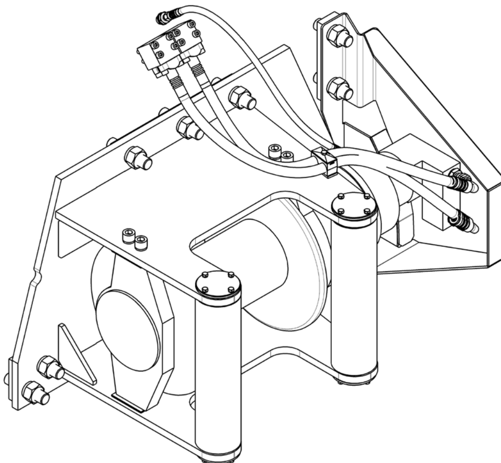
Лебедка 20т
