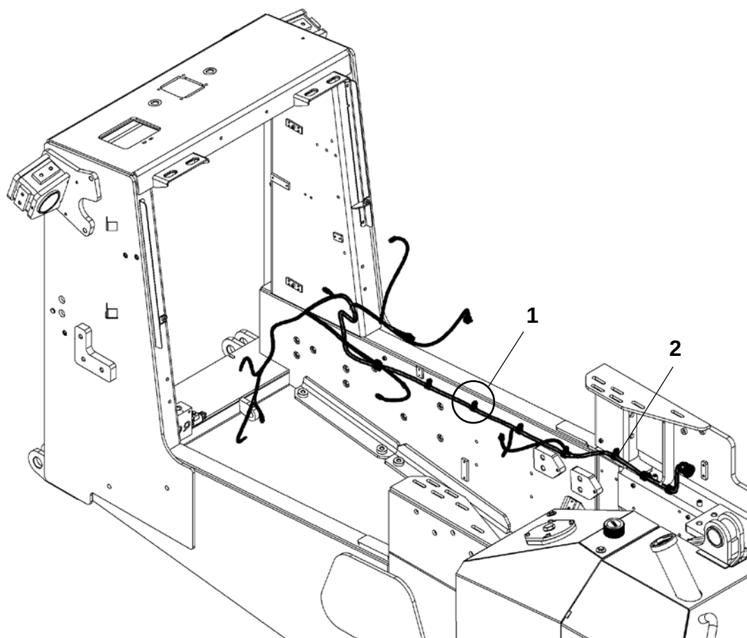
Жгут двигателя (ЯМЗ-238)
