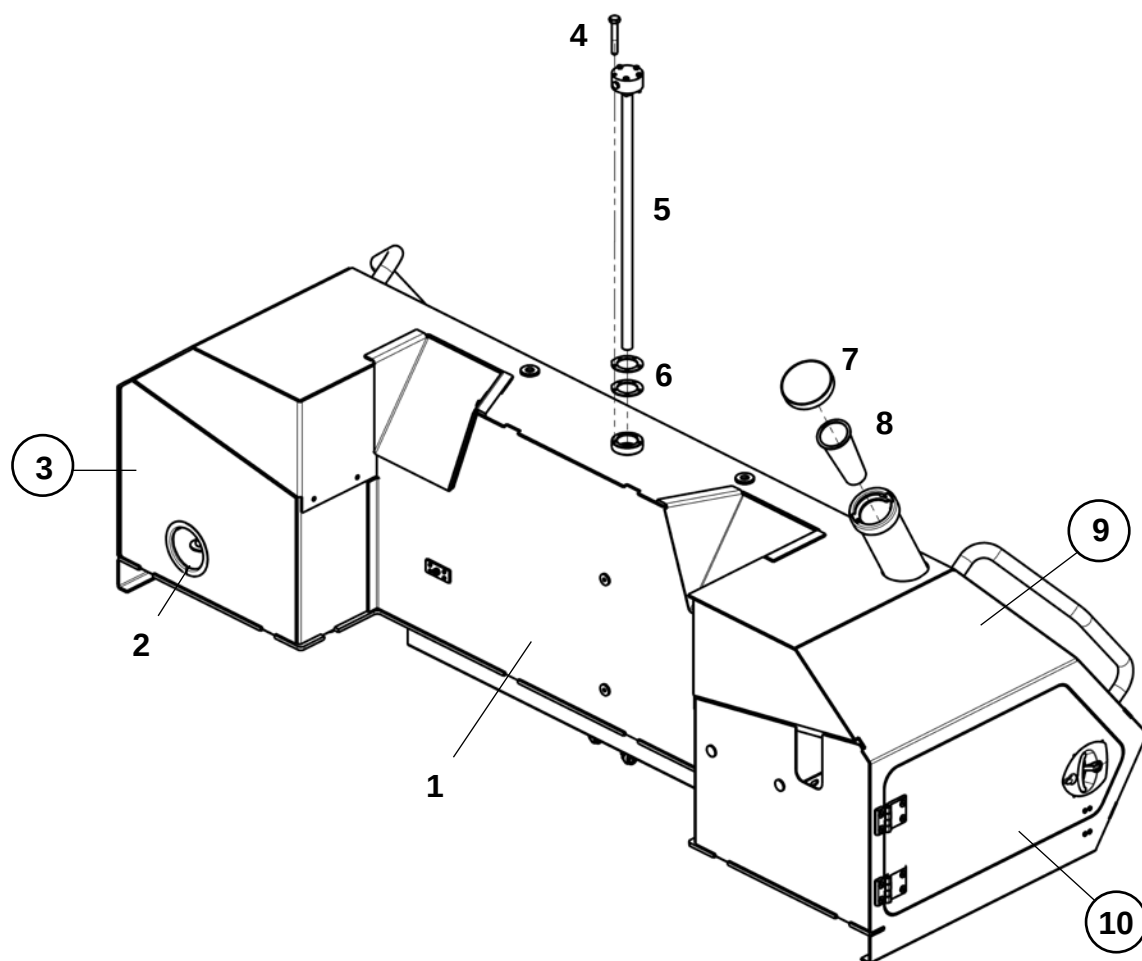
Топливный бак (ЯМЗ-536/238)
