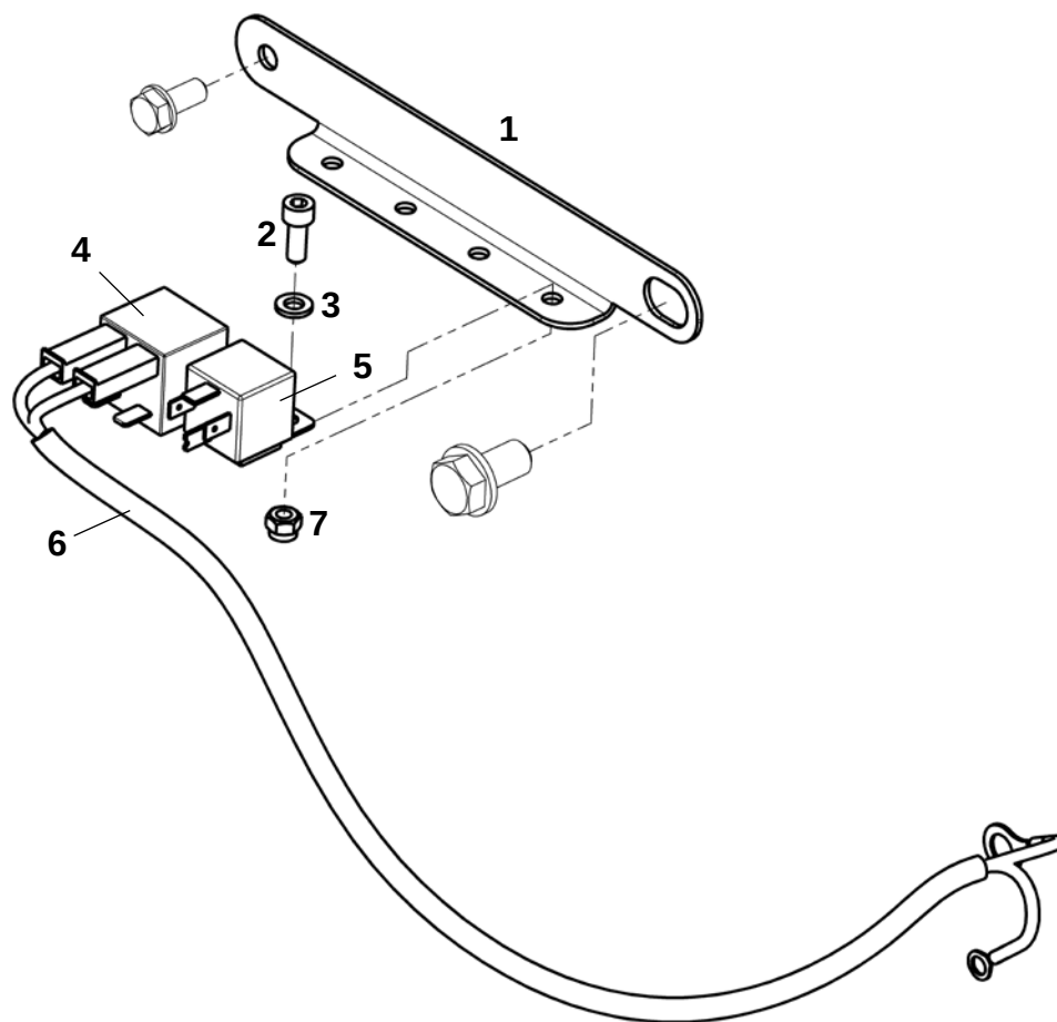
Установка реле стартера (ЯМЗ-536)
