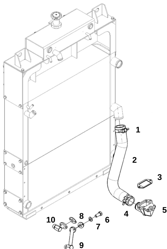
Комплект рукавов системы охлаждения (ЯМЗ-238)
