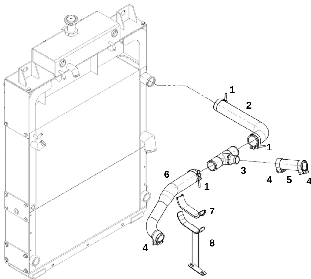
Комплект рукавов системы охлаждения (ЯМЗ-238)
