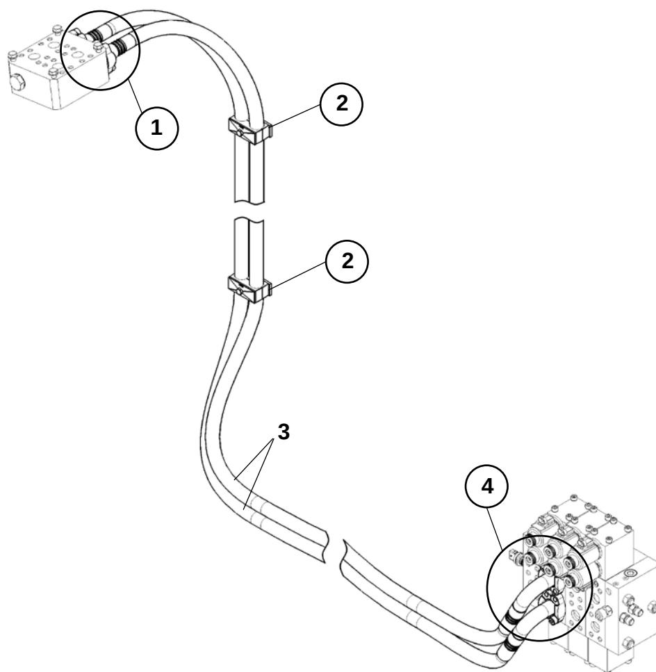
РВД (ЯМЗ-536/238)
