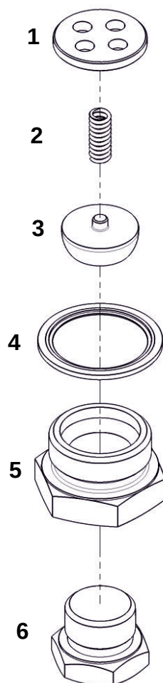
Пробка сливная (ЯМЗ-536/238)
