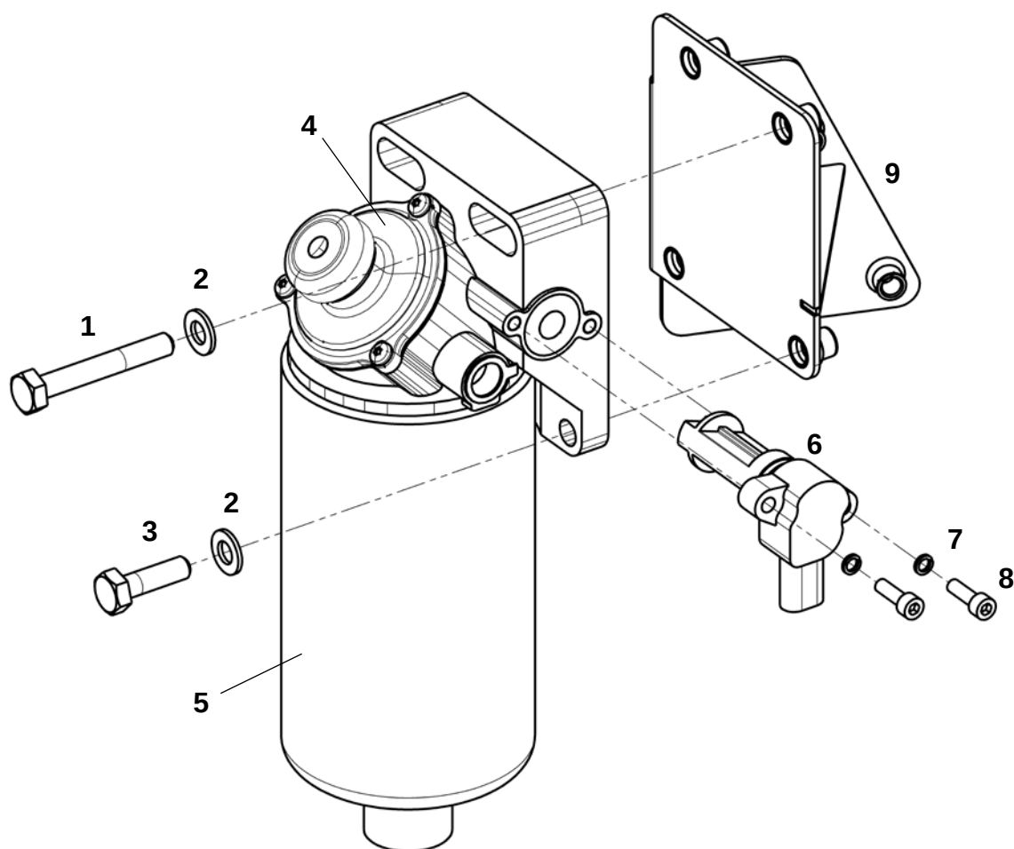
Корпус фильтра грубой очистки топлива в сборе (ЯМЗ-238)
