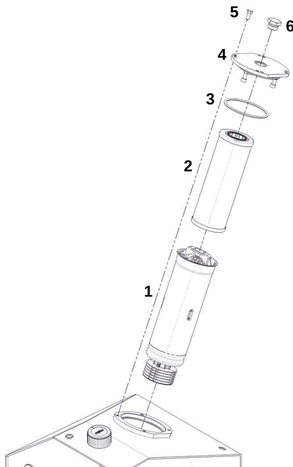
Фильтр в сливной линии (ЯМЗ-536/238)
