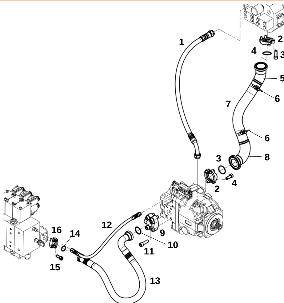
РВД (ЯМЗ-536)
