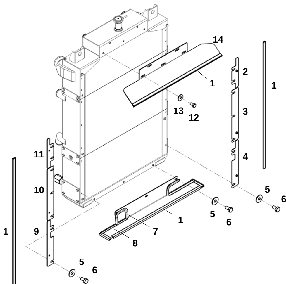
Комплект щитков капотирования (ЯМЗ-536)
