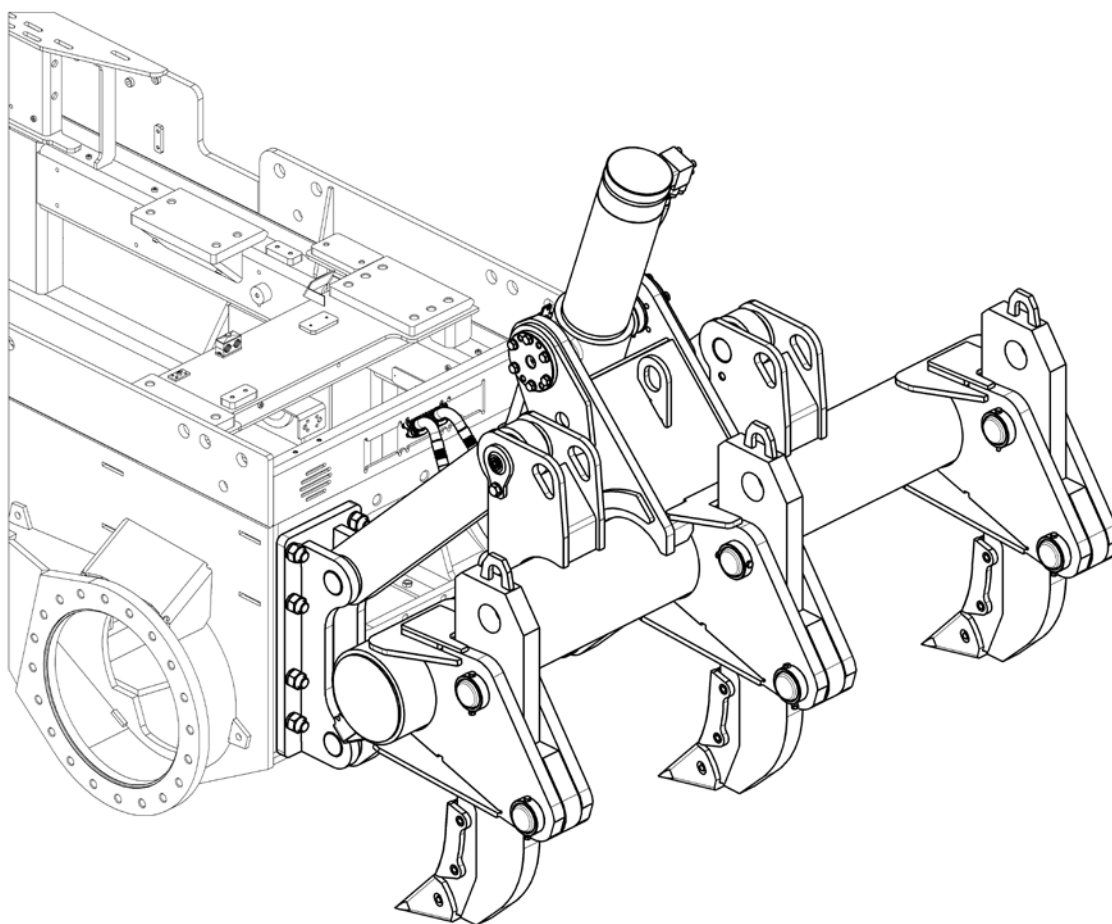
Рыхлитель трехзубый
