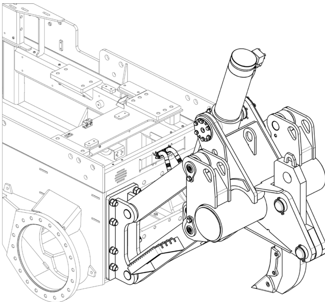
Рыхлитель однозубый
