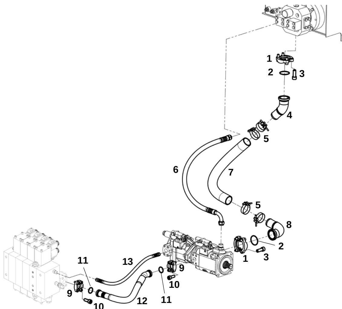
РВД (ЯМЗ-238)
