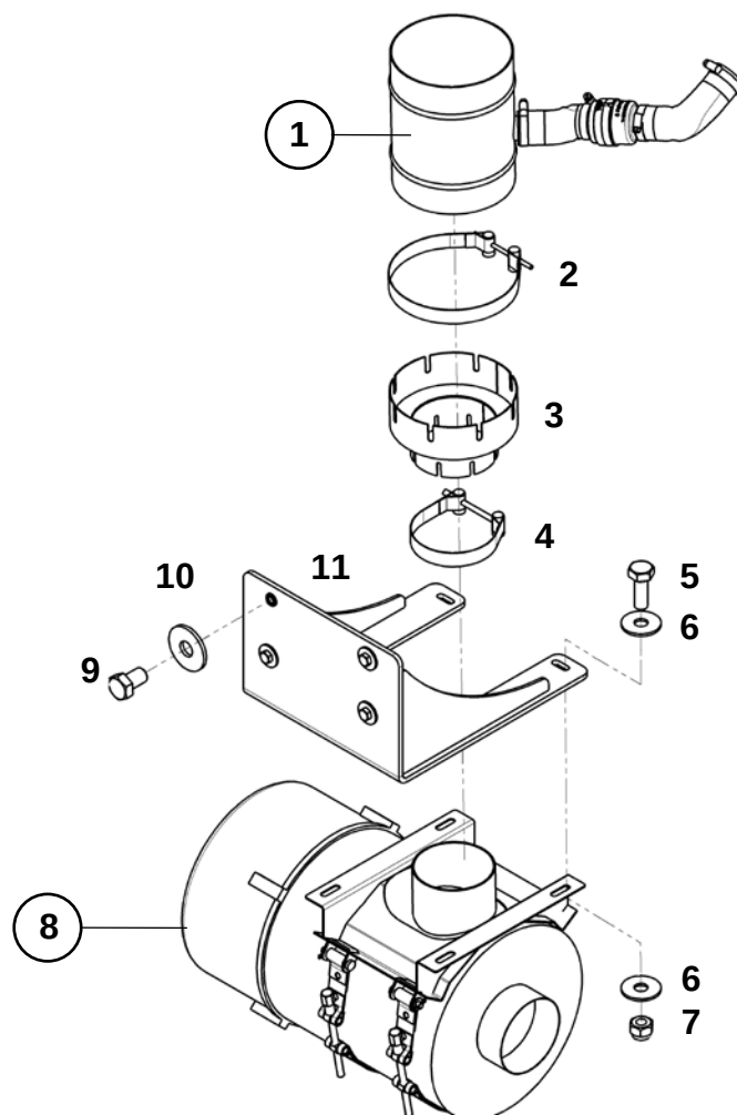
Мультициклон и фильтр воздушный (ЯМЗ-536)
