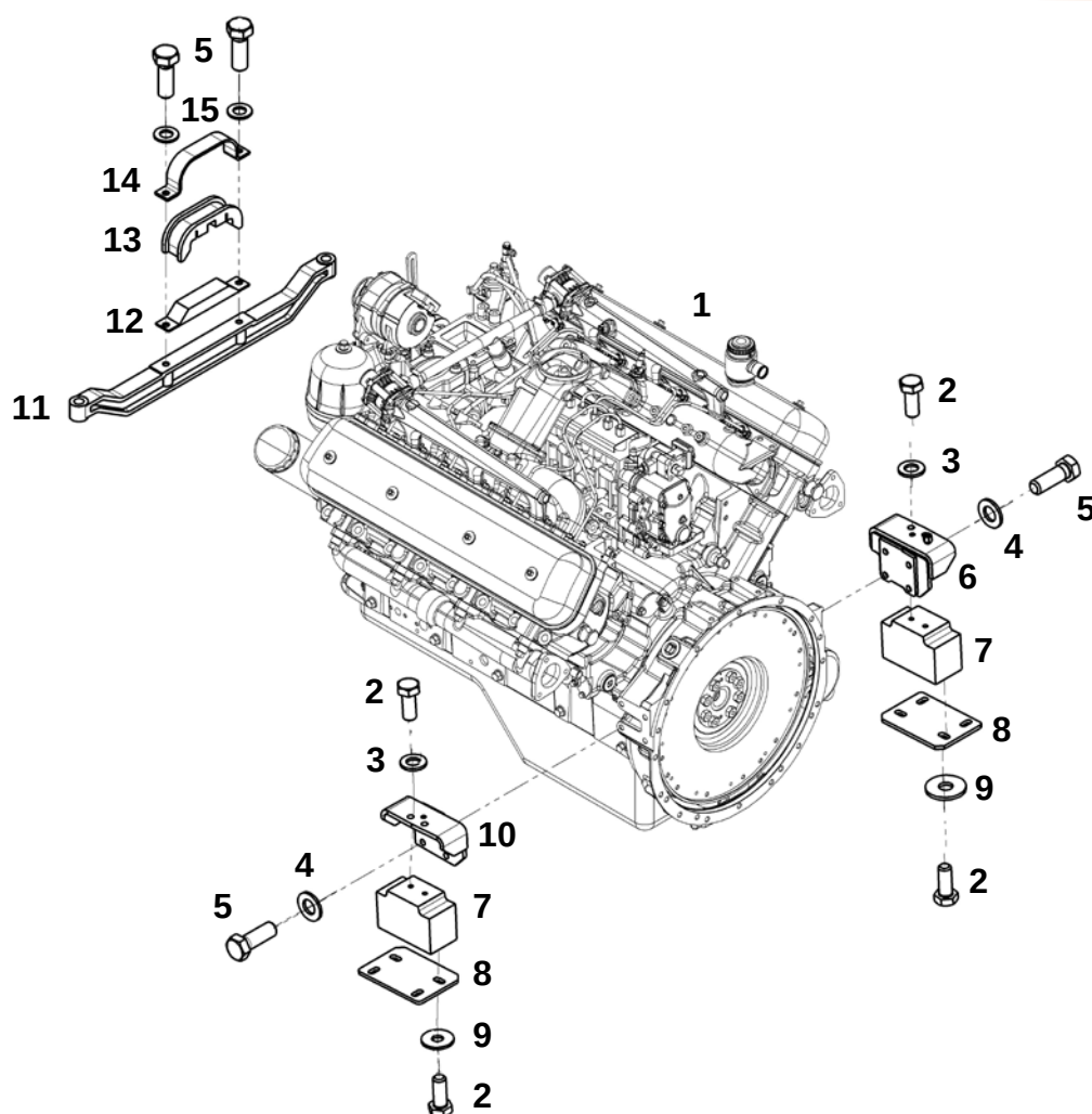
ЯМЗ-238
