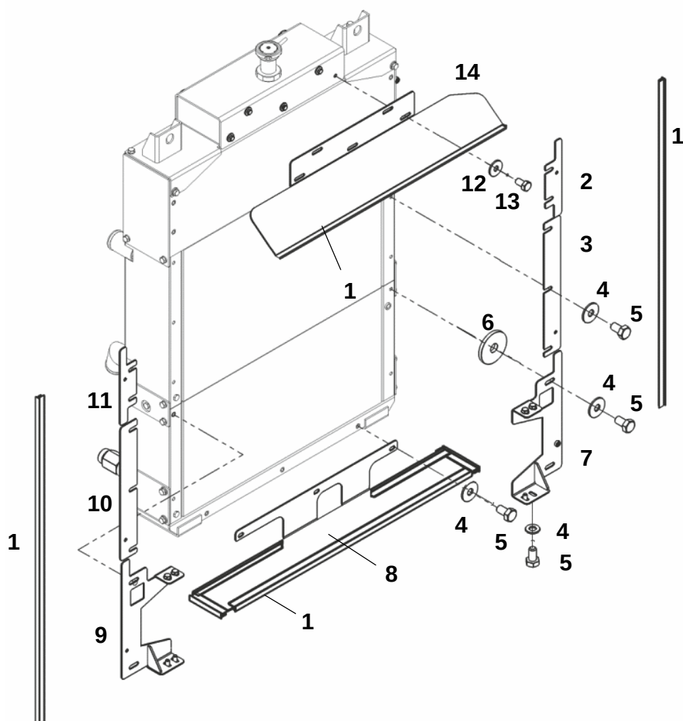
Комплект щитков капотирования (ЯМЗ-238)
