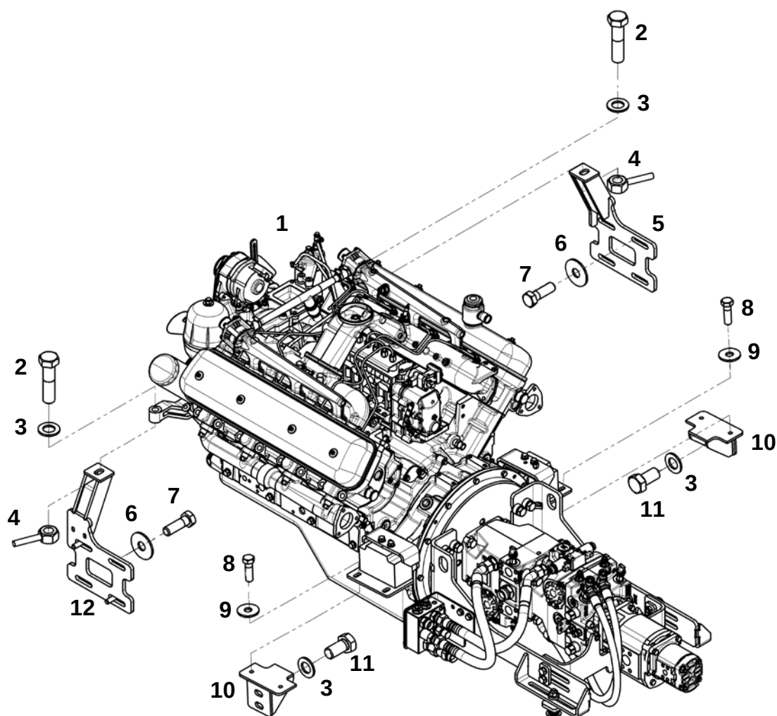
Силовой агрегат ЯМЗ-238
