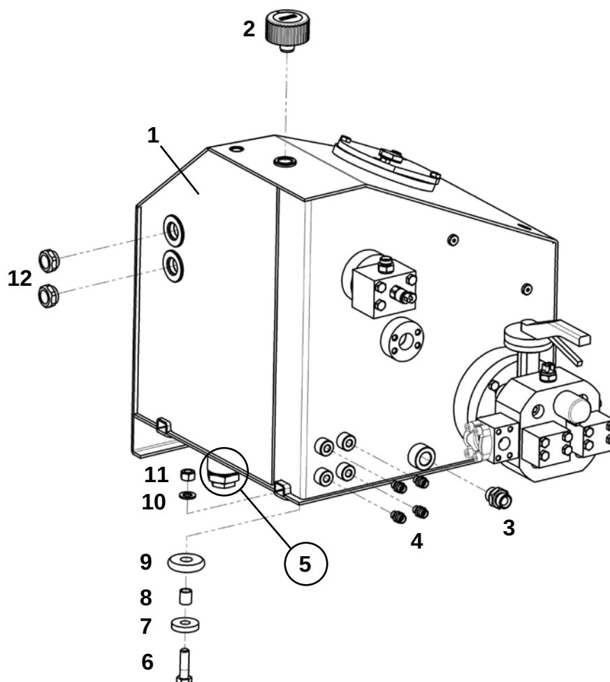
Бак гидравлический в сборе (ЯМЗ-536/238)
