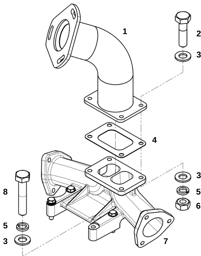
Отводы глушителя (ЯМЗ-238)
