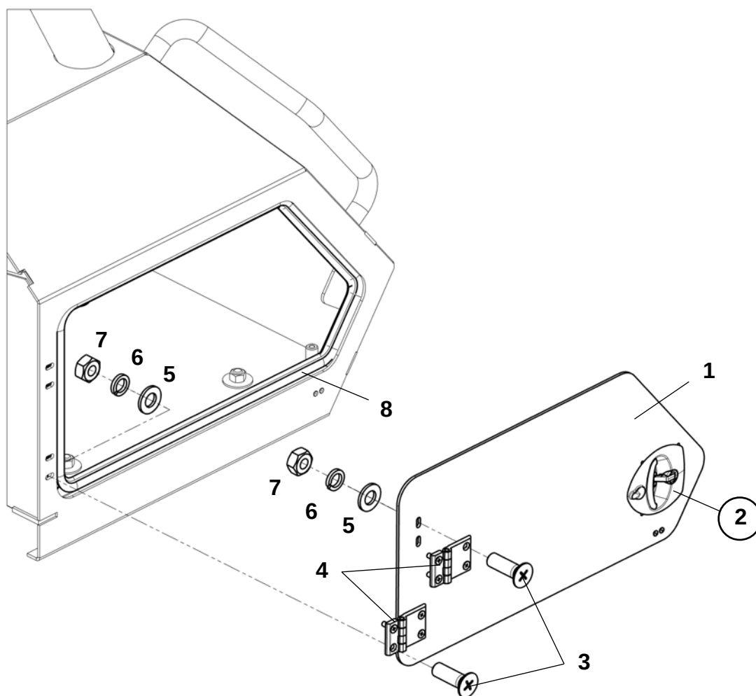
Створка (ЯМЗ-536/238)
