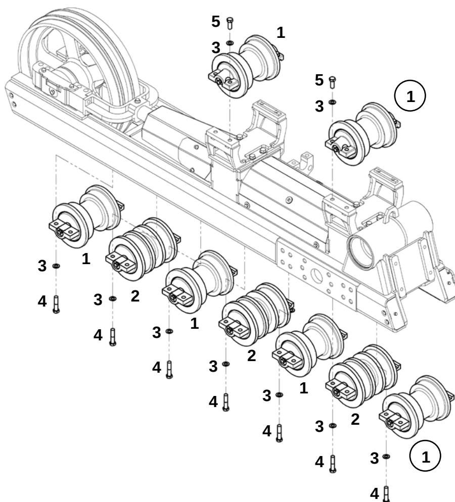
Каток опорный (ЯМЗ-536/238)
