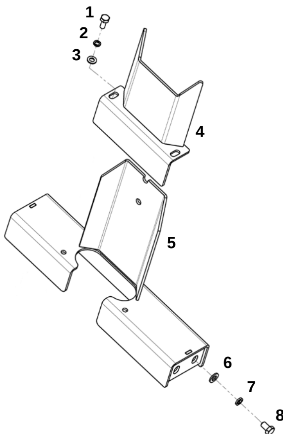
Кожух гидроцилиндра гидрперекося отвала
