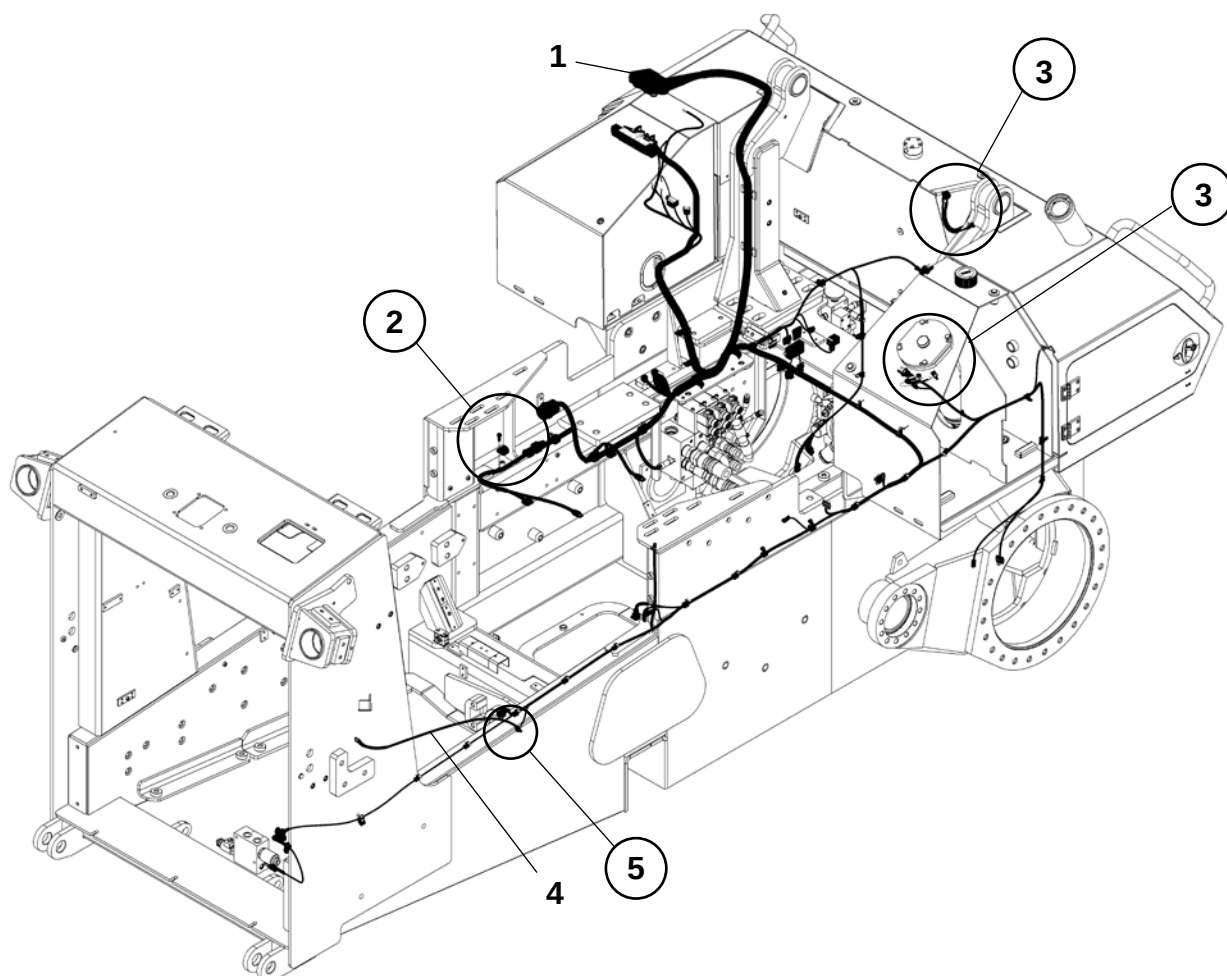
Жгут контроллера / кабель массы
