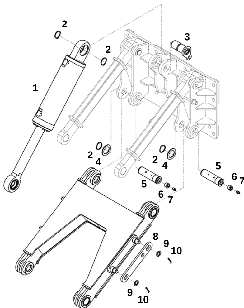
Крепление гидроцилиндра
