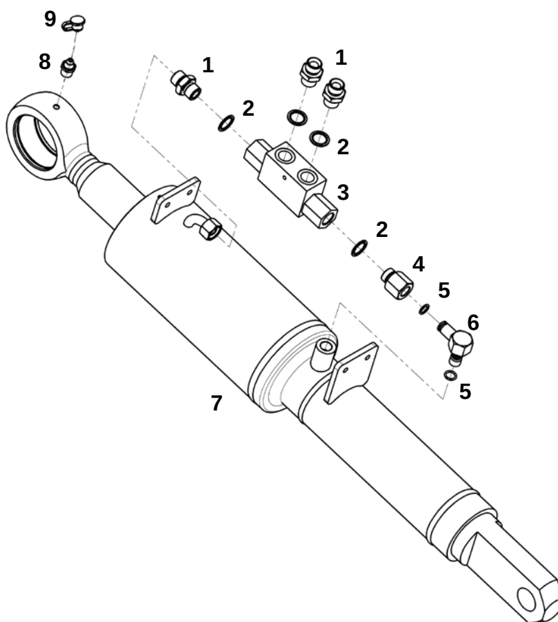
Гидроцилиндр перекоса отвала в сборе
