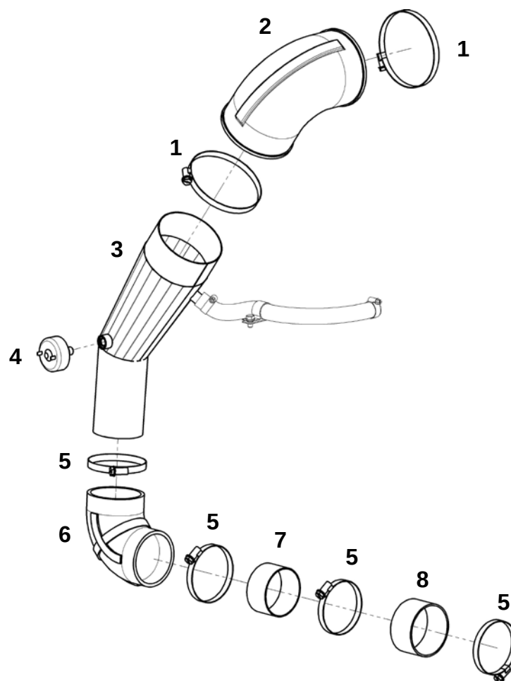
Впускной тракт (ЯМЗ-536)
