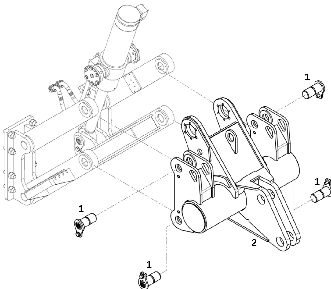
Крепление балки задней однозубого рыхлителя
