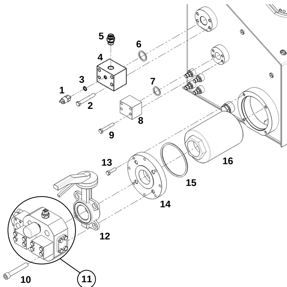
Компоненты гидравлического бака (ЯМЗ-536/238)
