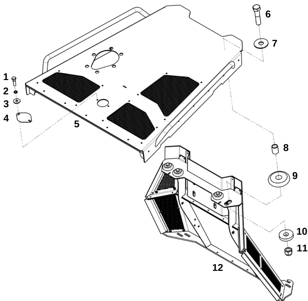
Перегородка, капот (ЯМЗ-536)
