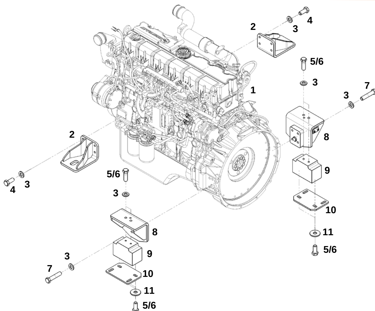
ЯМЗ-536
