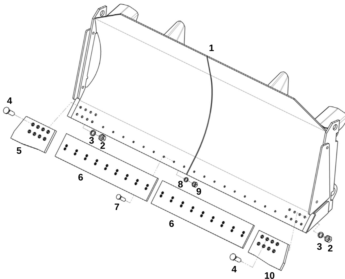
Отвал прямой – Тип В
