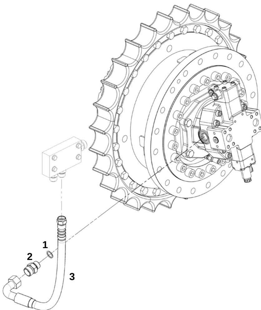
РВД дренажа левого гидромотора
