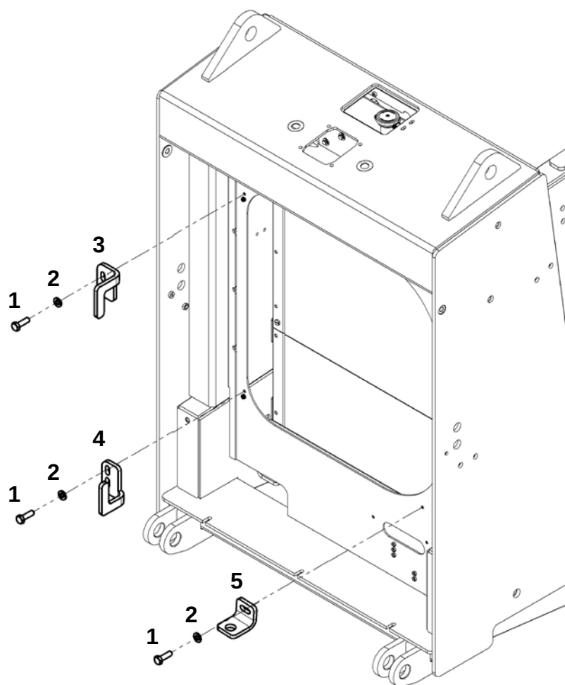
Комплект стопоров рамы вентиляторов (ЯМЗ-536/238)
