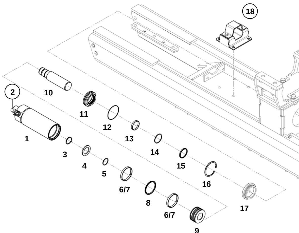
Механизм натяжения в сборе (ЯМЗ-536/238)
