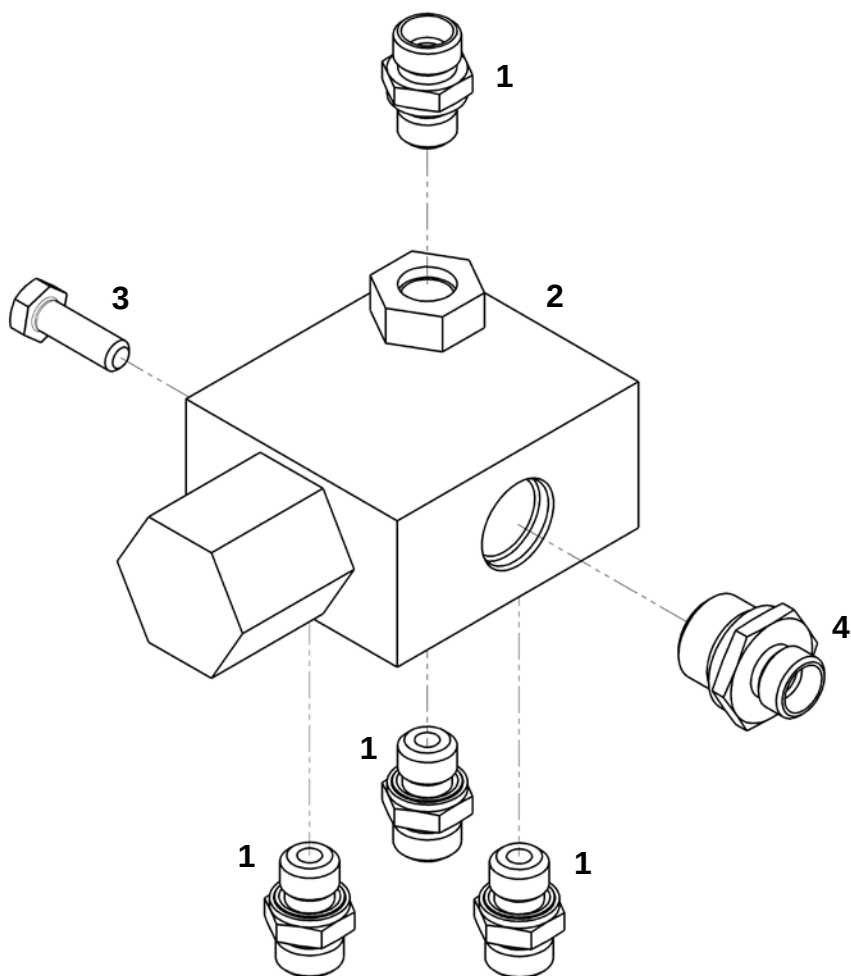
Блок клапанов в сборе (ЯМЗ-536/238)
