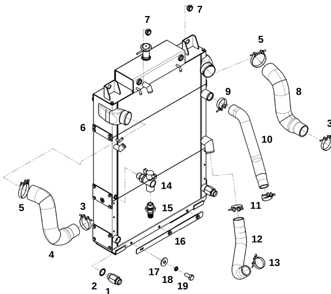
Блок радиаторов в сборе (ЯМЗ-536)
