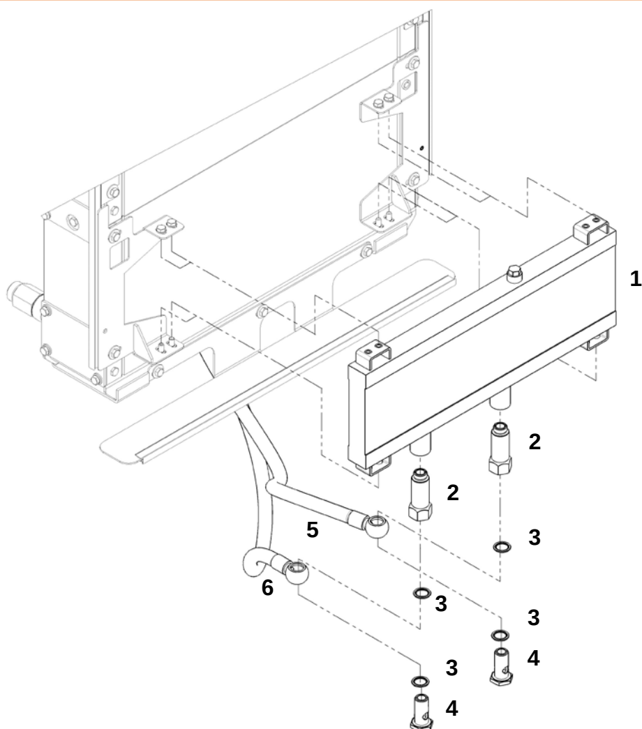
Комплект масляного радиатора ДВС (ЯМЗ-238)
