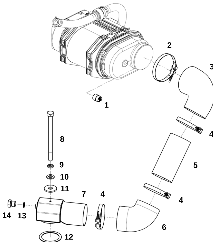
Впускной тракт (ЯМЗ-238)
