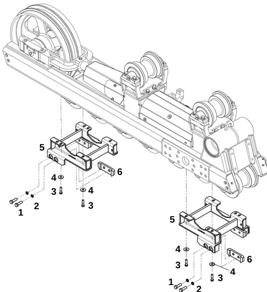
Элемент защиты от схода гусениц (ЯМЗ-536/238)
