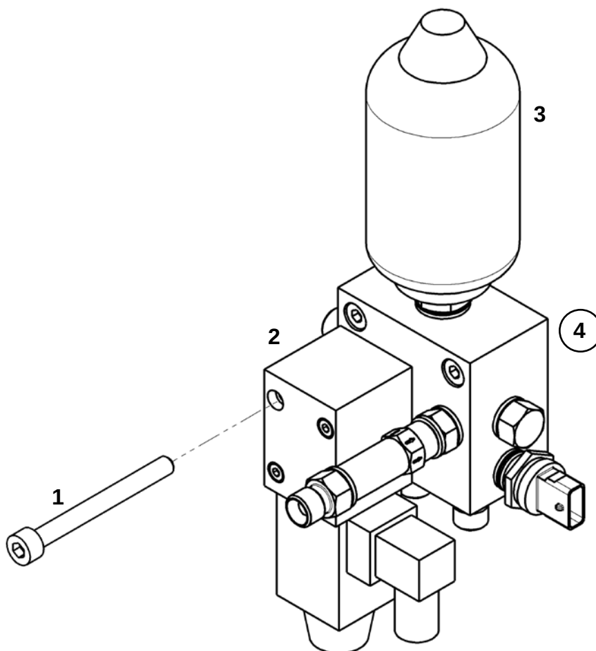
Плита тормозная в сборе (ЯМЗ-536/238)
