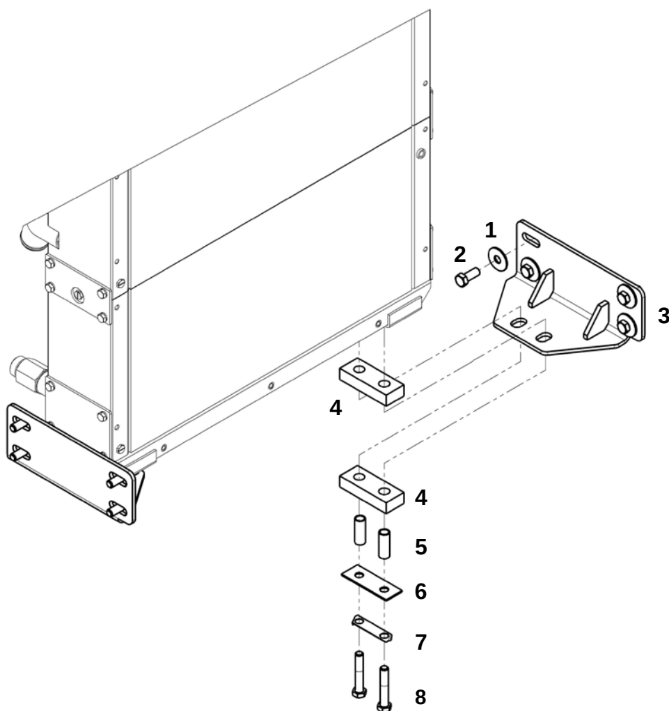
Комплект установки опор радиатора (ЯМЗ-536/238)
