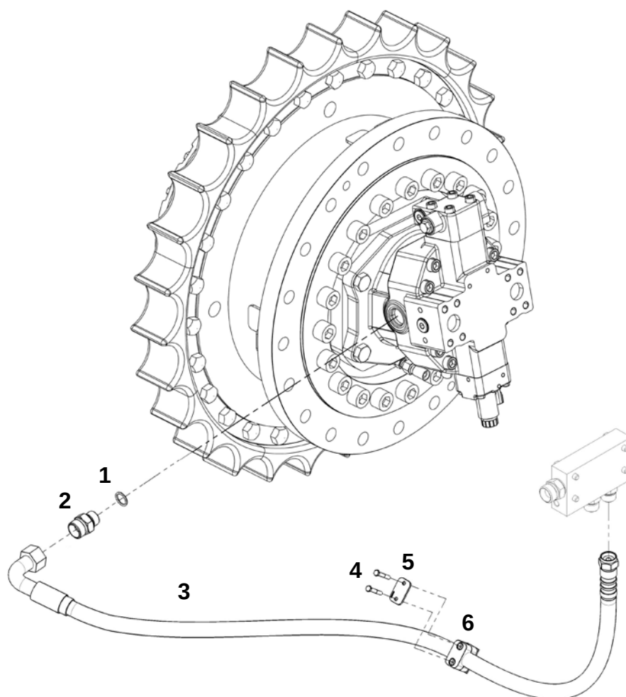
РВД дренажа правого гидромотора
