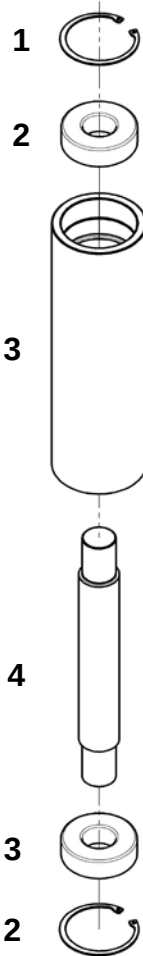
Ролик
