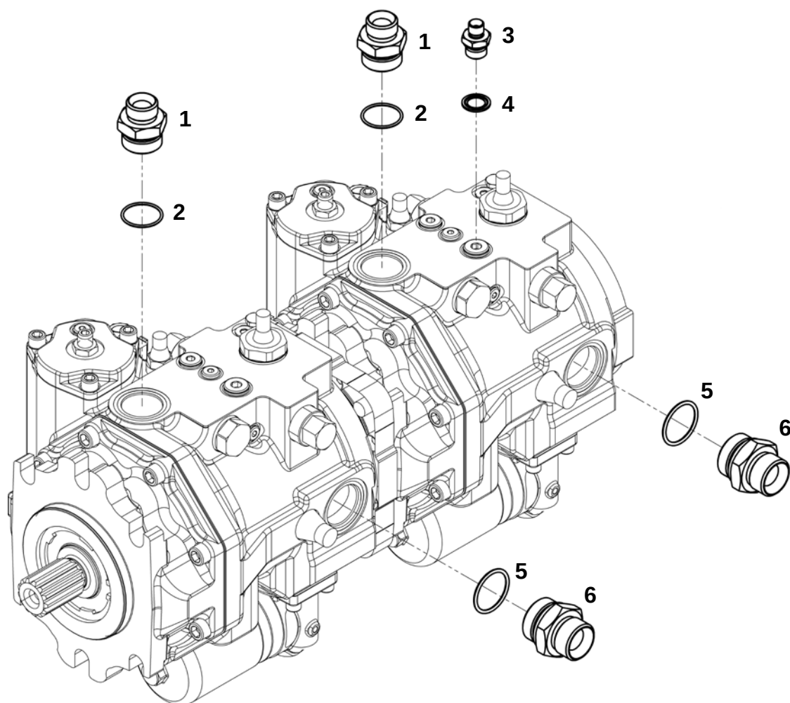
Комплект обвязки насосов гидравлических A4VG145
