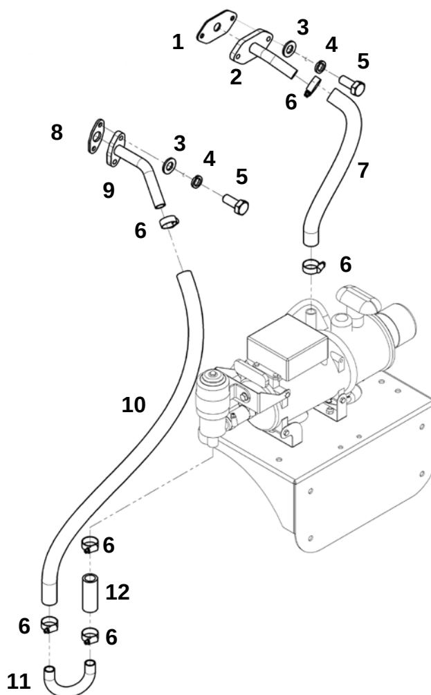
Установка ПЖД (ЯМЗ-536)
