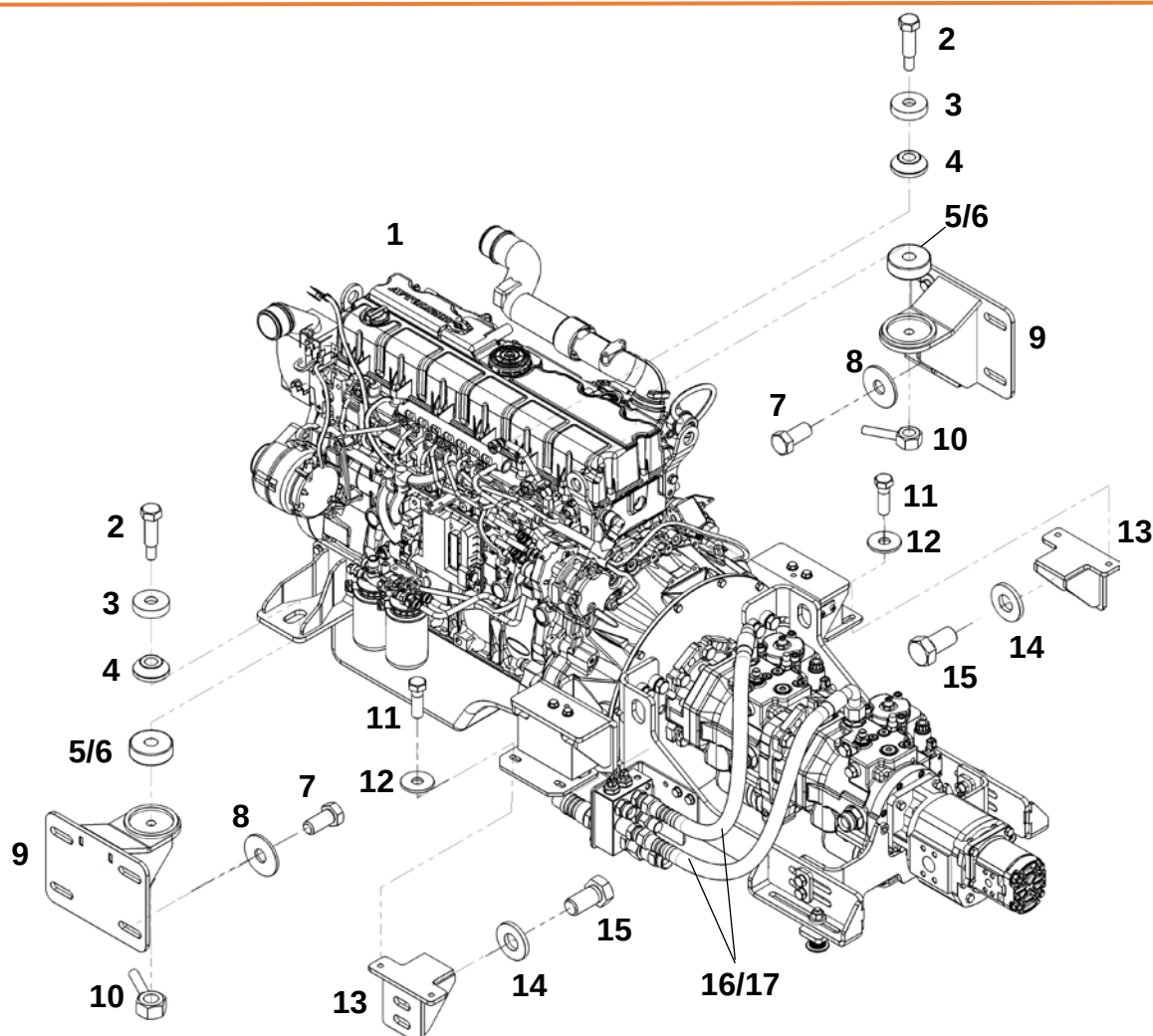
Силовой агрегат ЯМЗ-536
