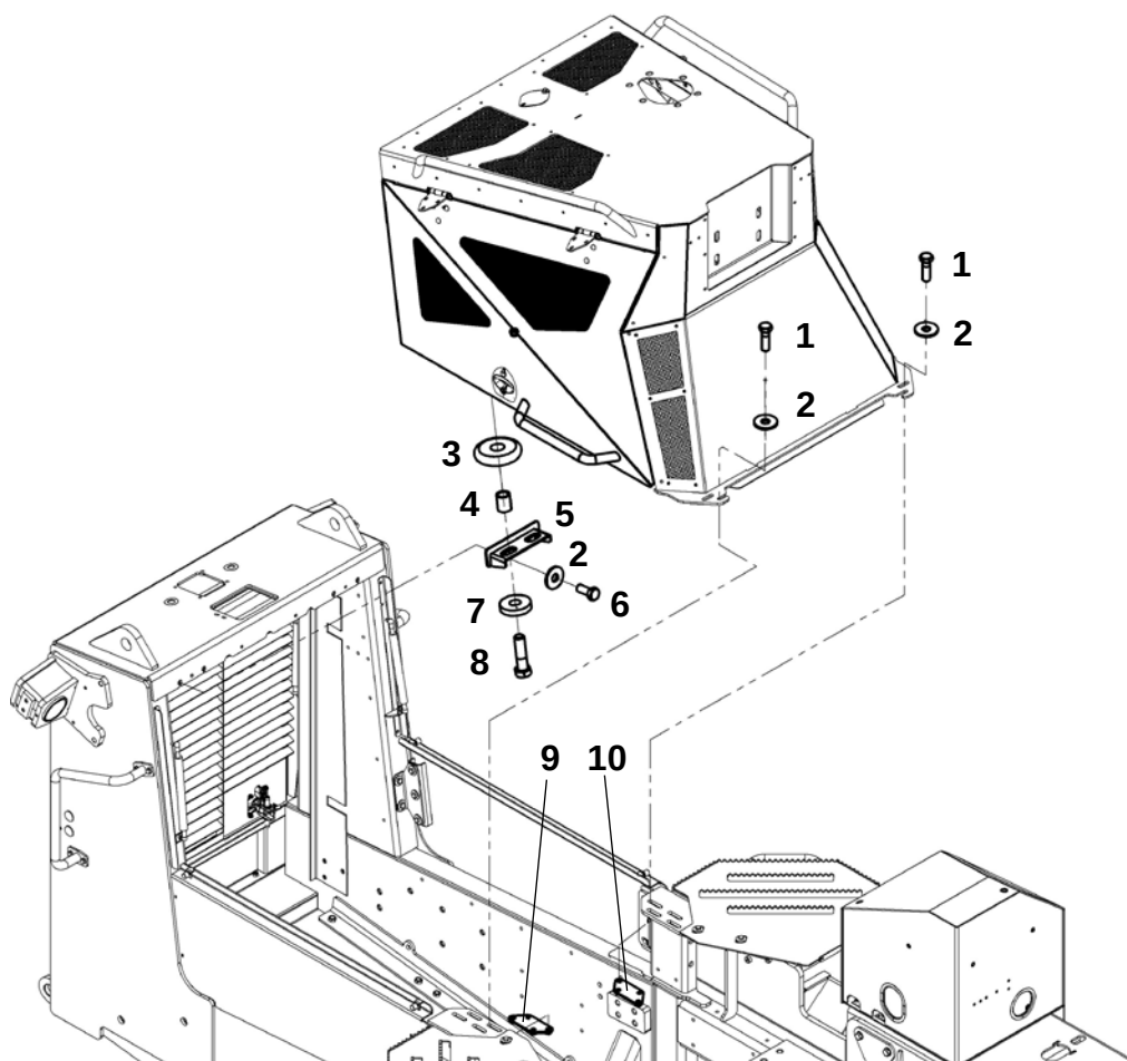
Крепление облицовки (ЯМЗ-536/238)
