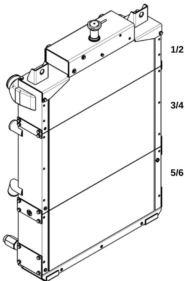
Сегменты блока радиаторов (ЯМЗ-536)
