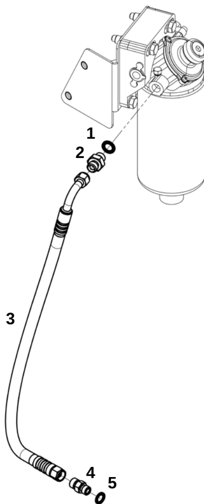
Топливопровод (ЯМЗ-238)
