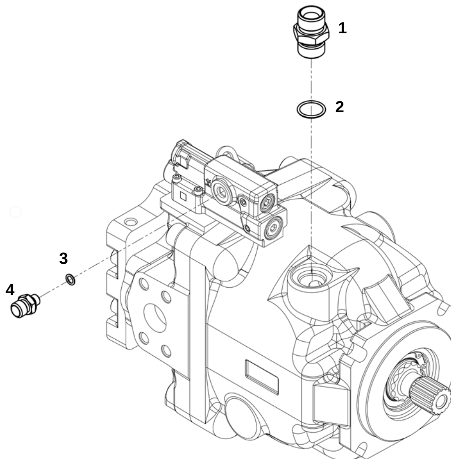
Комплект обвязки насосов гидравлических ER-R-100B
