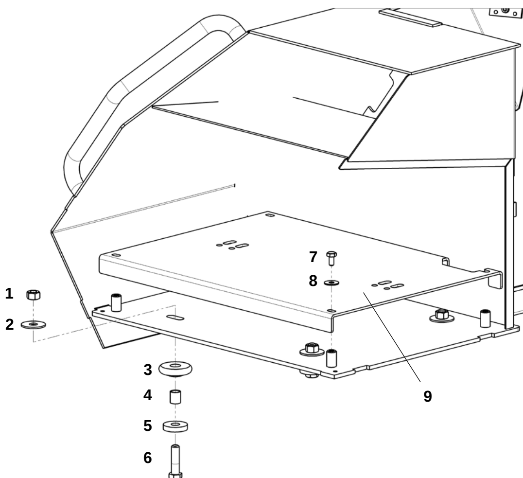
Ящик для аккумуляторных батарей (ЯМЗ-536/238)
