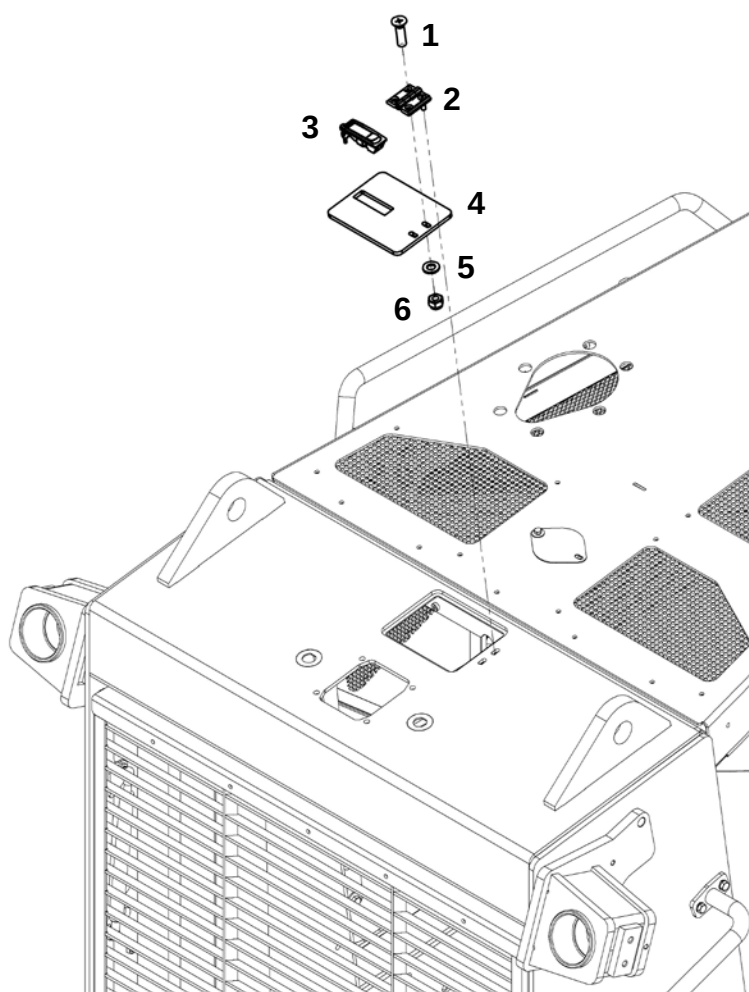
Крышка в сборе (ЯМЗ-536/238)
