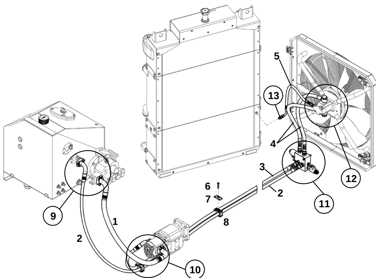
Система привода вентилятора Fan Drive (ЯМЗ-536/238)
