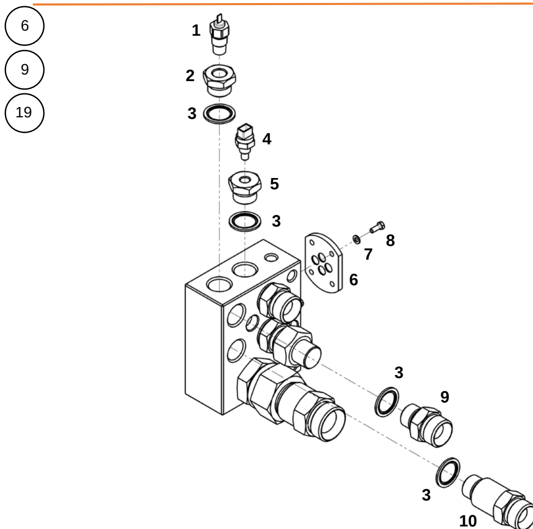
Крепление датчиков и штуцеров, установка заглушки
