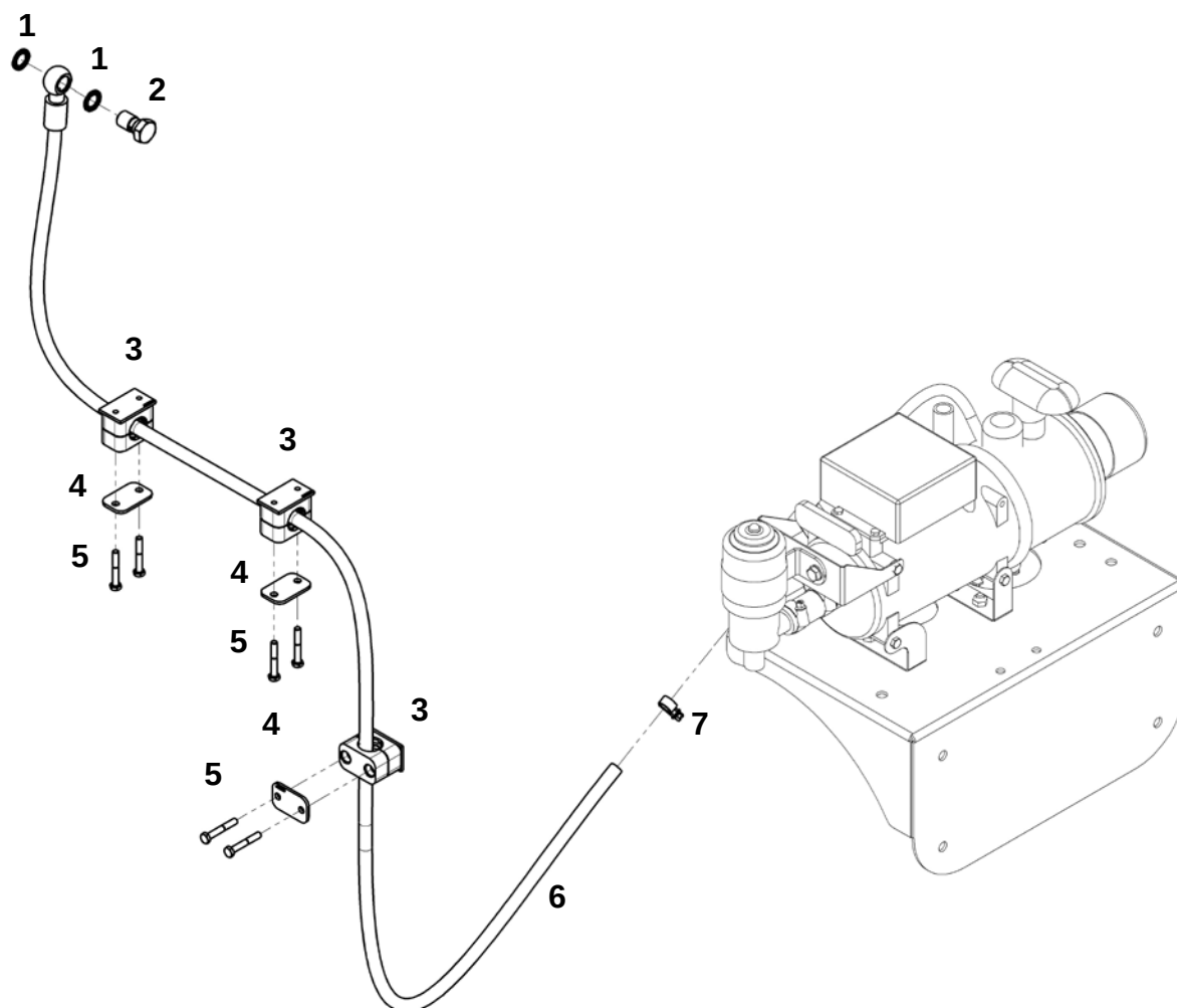
Установка ПЖД (ЯМЗ-536)
