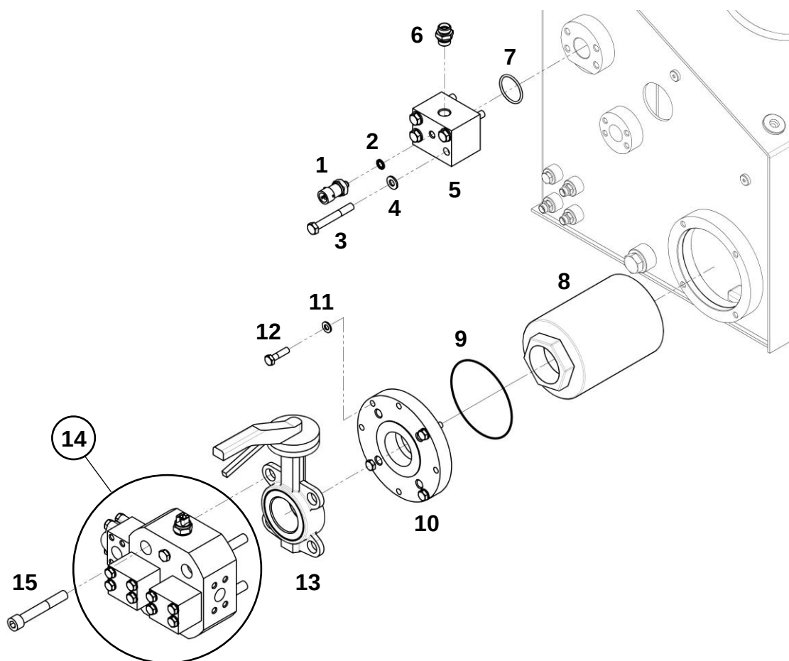
Компоненты гидравлического бака
