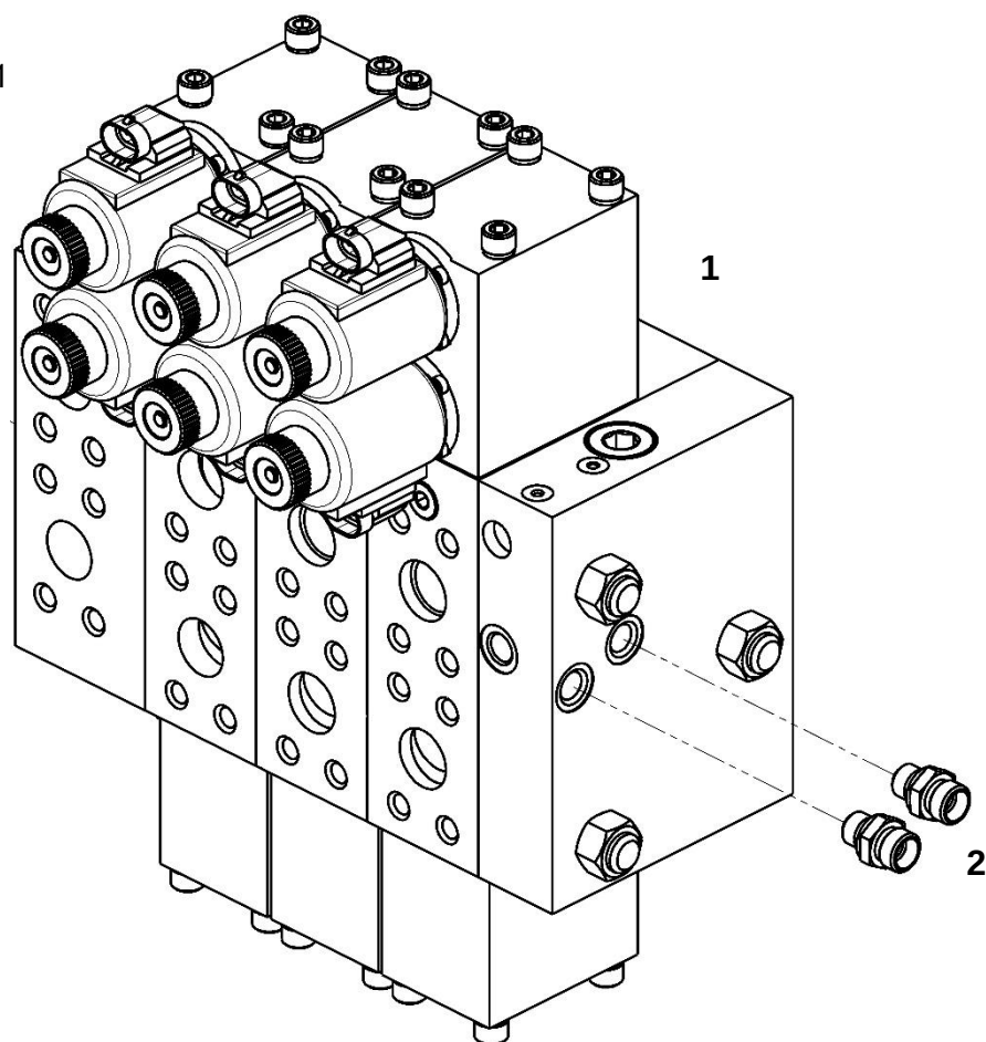
Гидрораспределитель в сборе
