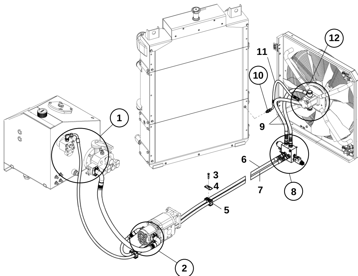
Система привода вентилятора Fan Drive
