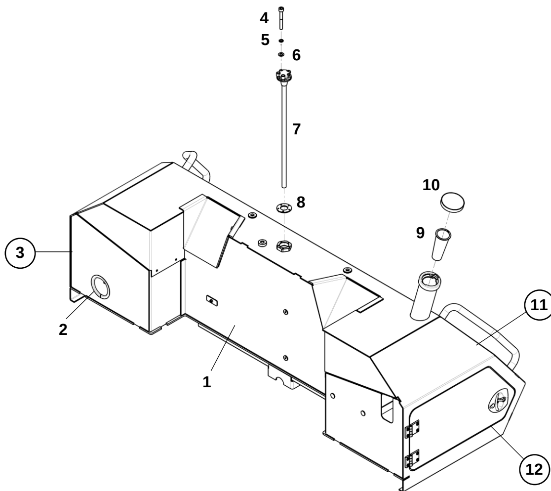
Топливный бак
