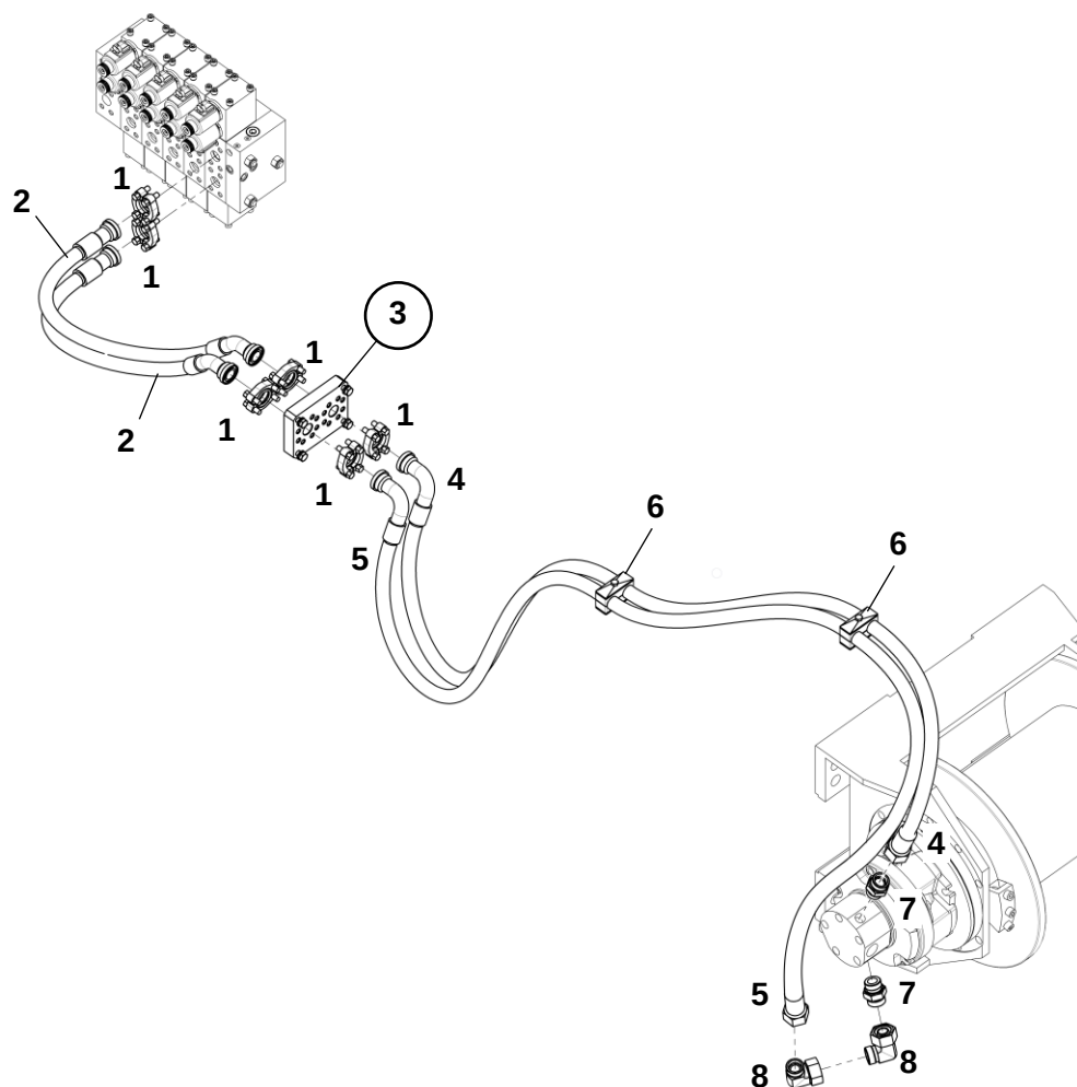
Трубопроводы заднего навесного оборудования
