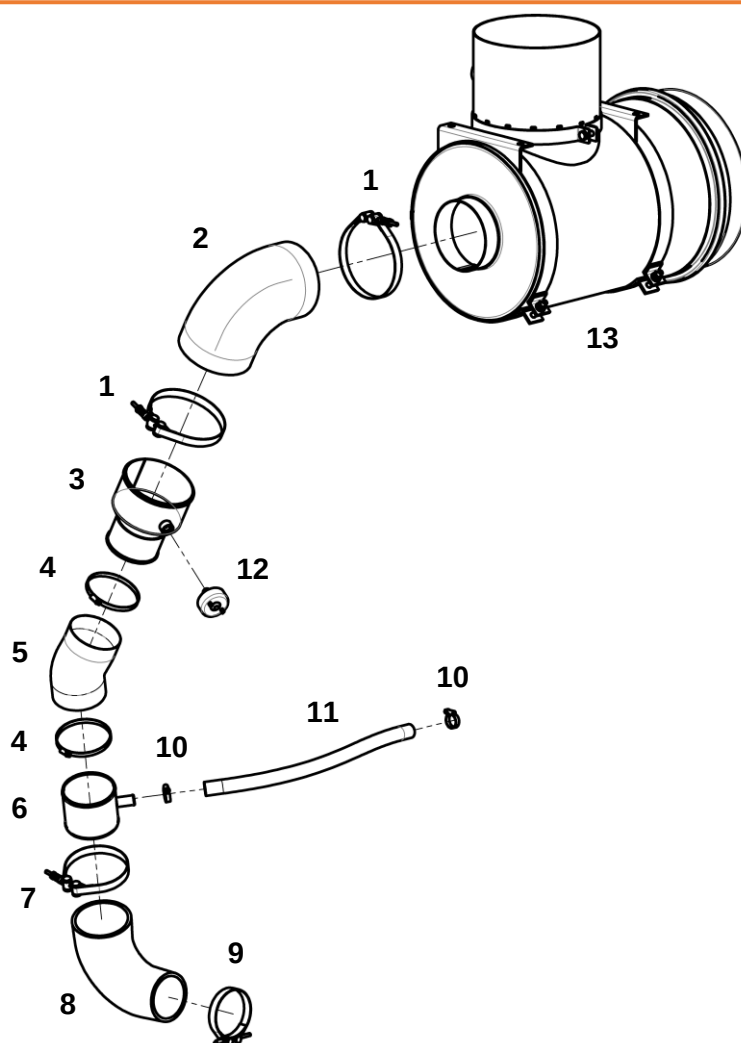
Впускной тракт
