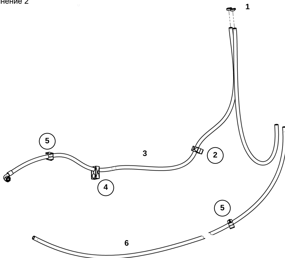
Рукава системы охлаждения
