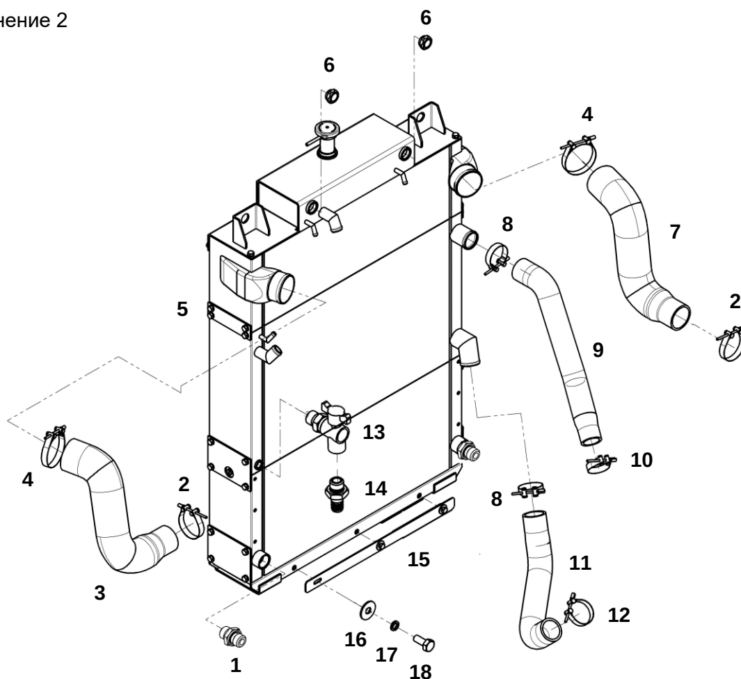
Блок радиаторов в сборе
