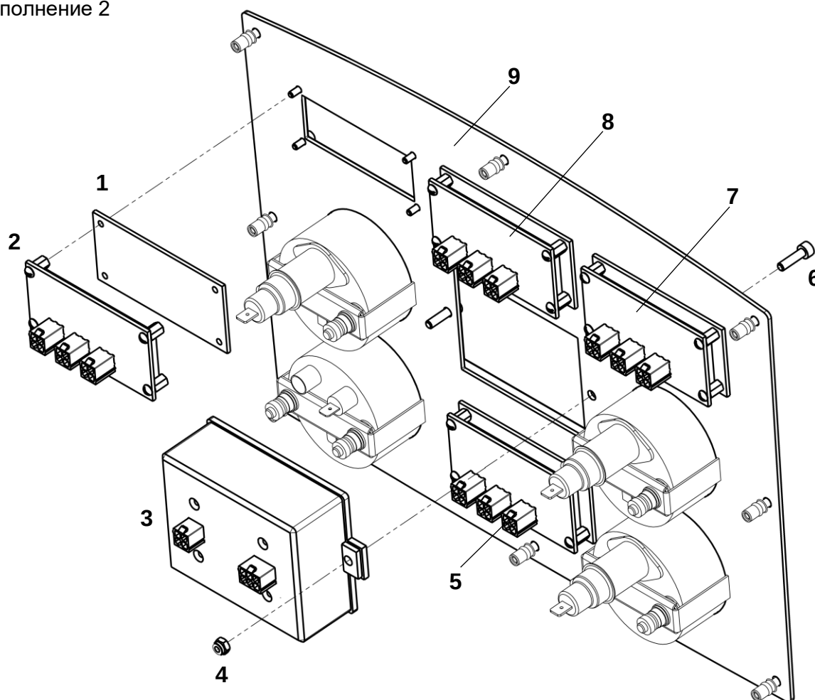
Передний щиток в сборе
