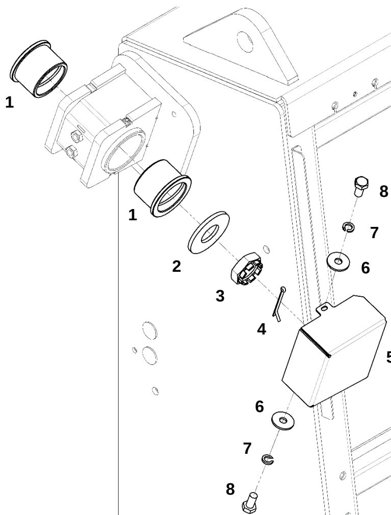
Втулки в сборе
