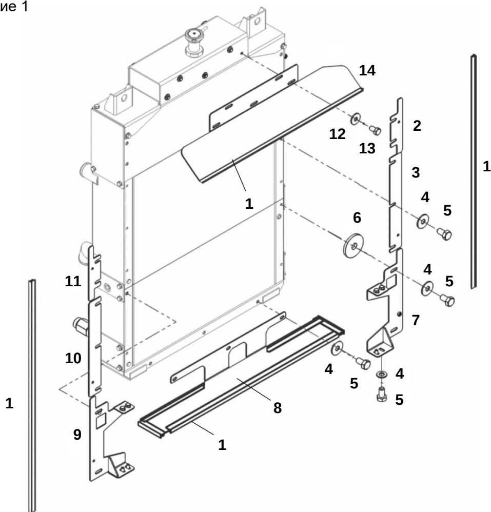
Комплект щитков капотирования
