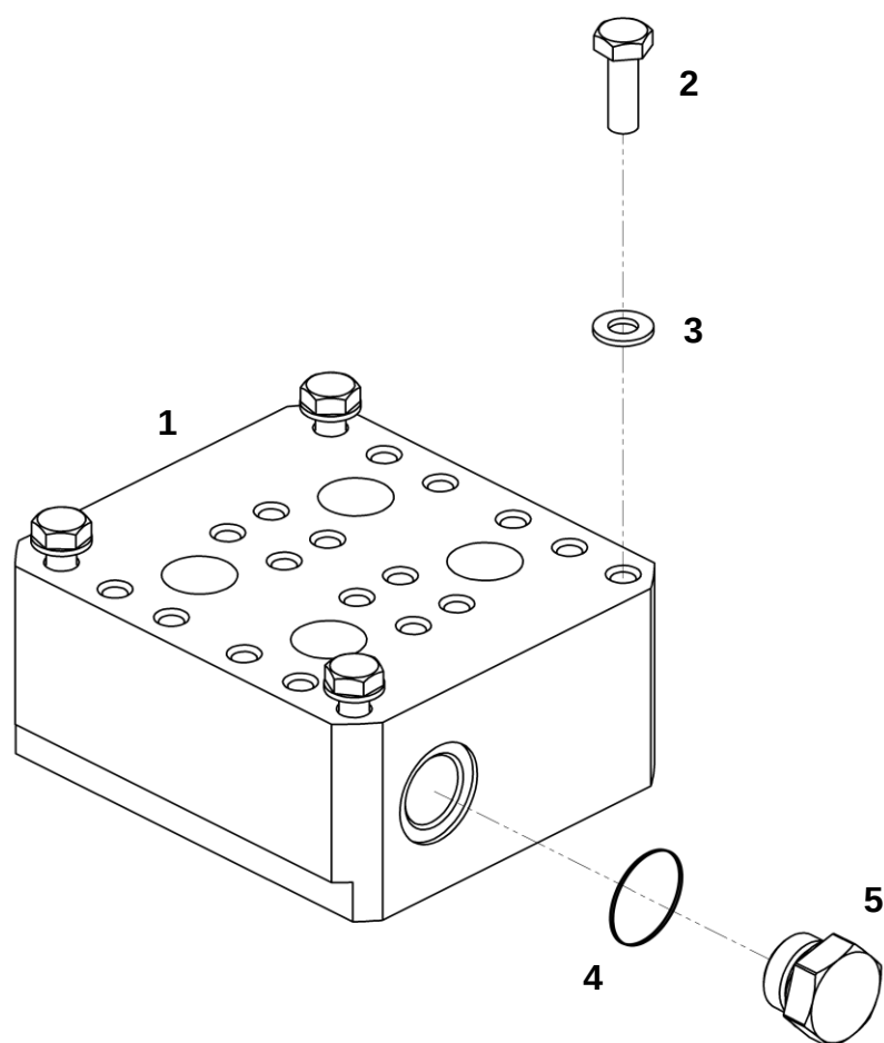
Плита в сборе
