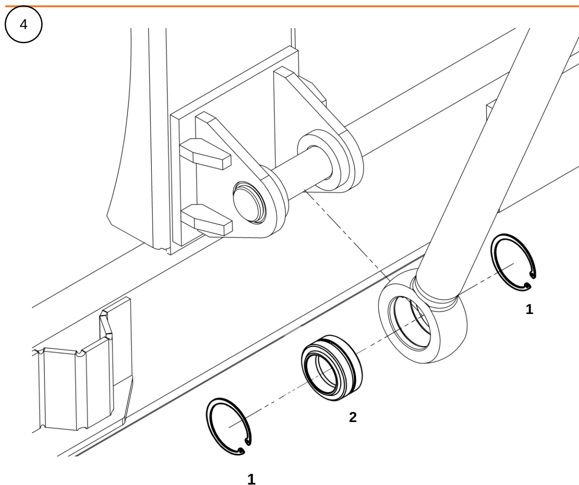
Крепление гидроцилиндра
