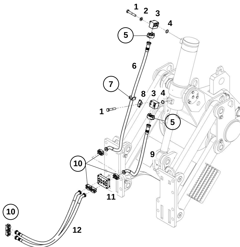
Гидроразводка рыхлительного оборудования
