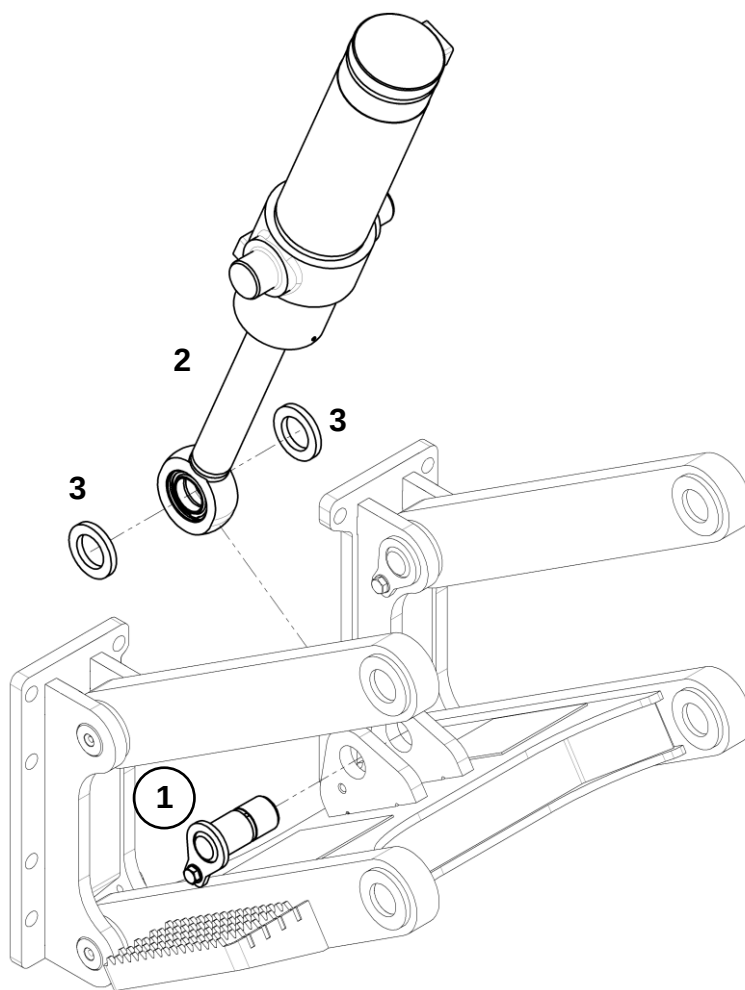
Крепление гидроцилиндра и балки задней
