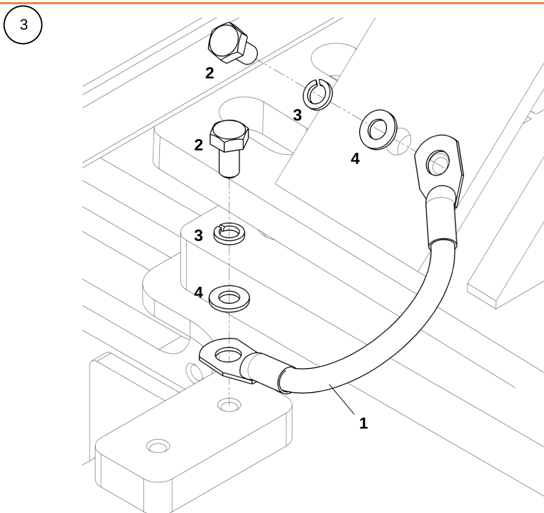
Крепление кабеля массы
