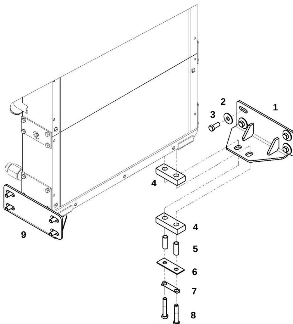
Комплект установки опор радиатора
