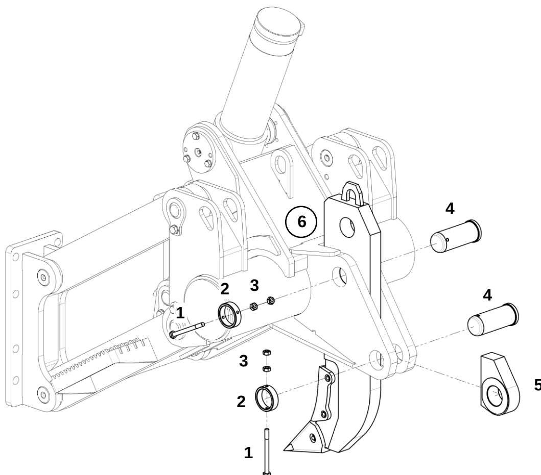
Крепление ножа однозубого рыхлителя
