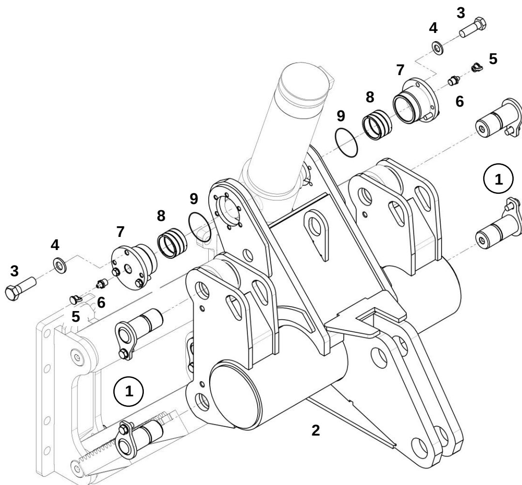
Крепление балки задней однозубого рыхлителя
