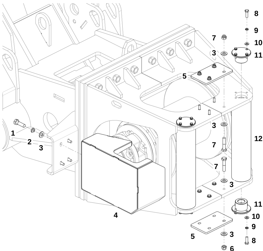
Балка с лебедкой
