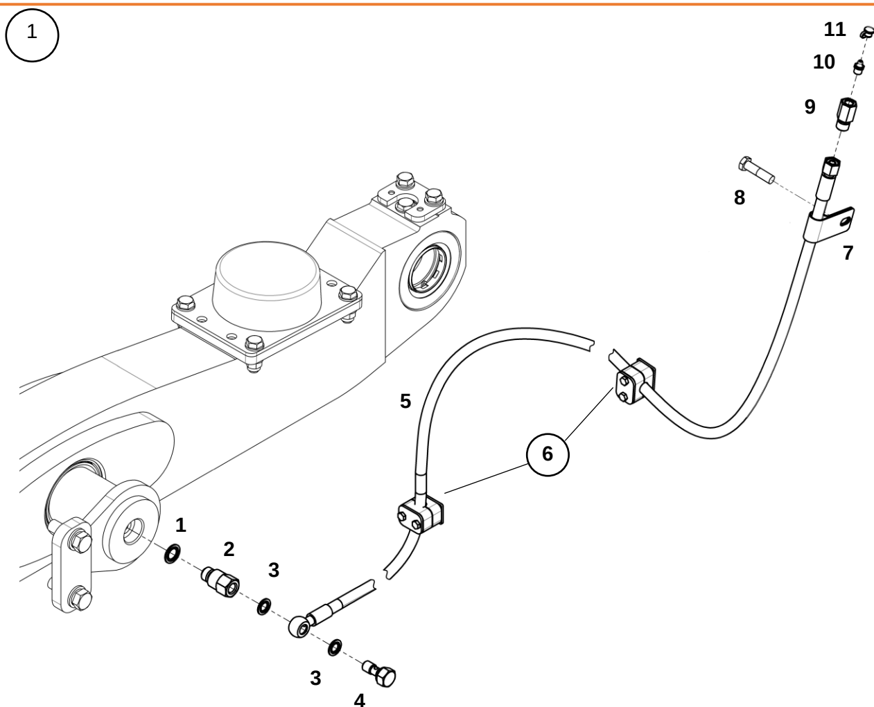
Смазка центральной оси балки
