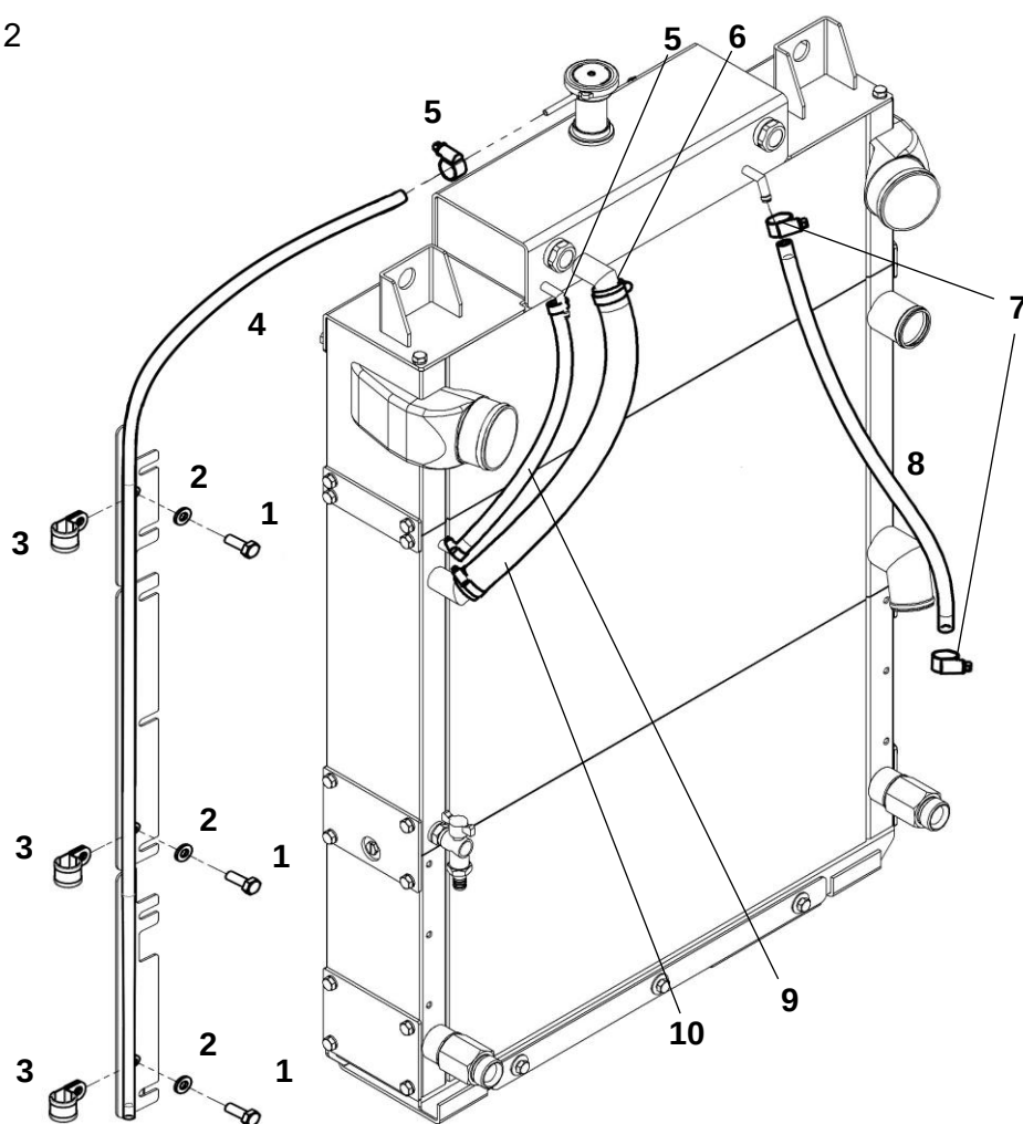
Рукава системы охлаждения
