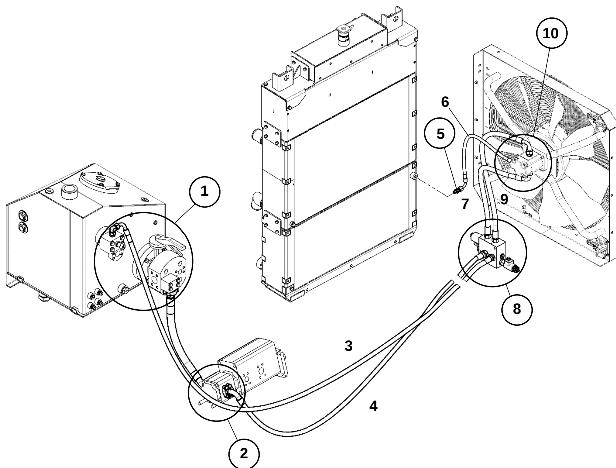
Система привода вентилятора Fan Drive
