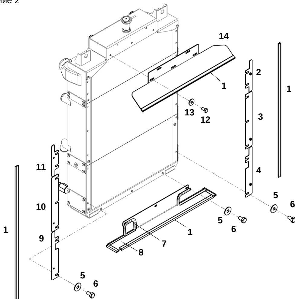
Комплект щитков капотирования
