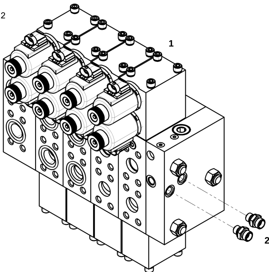
Гидрораспределитель в сборе
