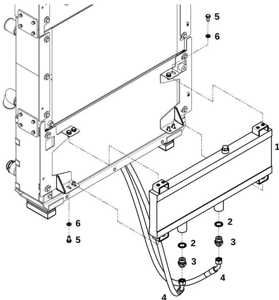
Масляный радиатор ДВС (крепление, подключение)
