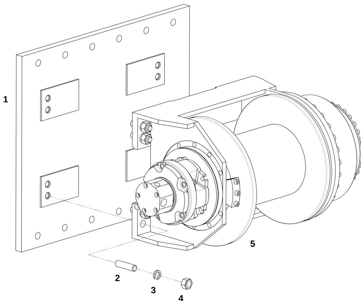
Лебедка в сборе
