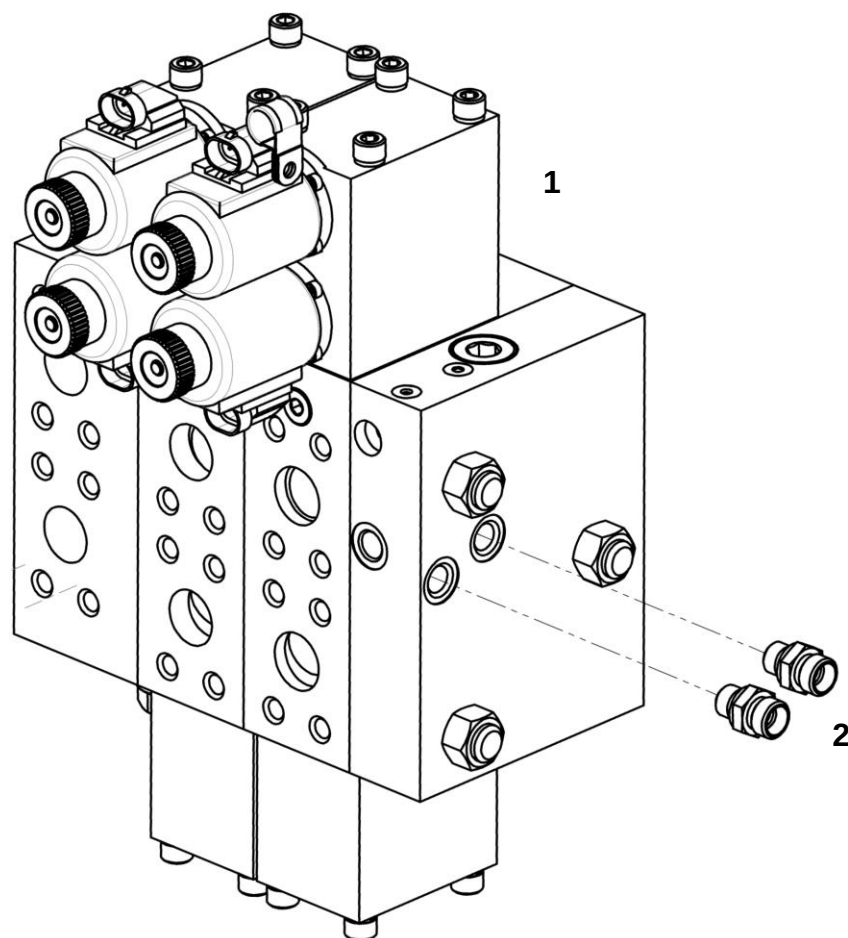
Гидрораспределитель в сборе
