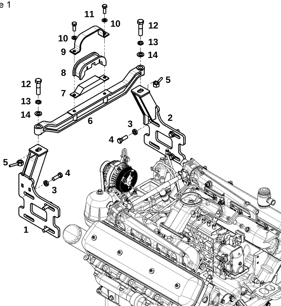
Передние опоры двигателя
