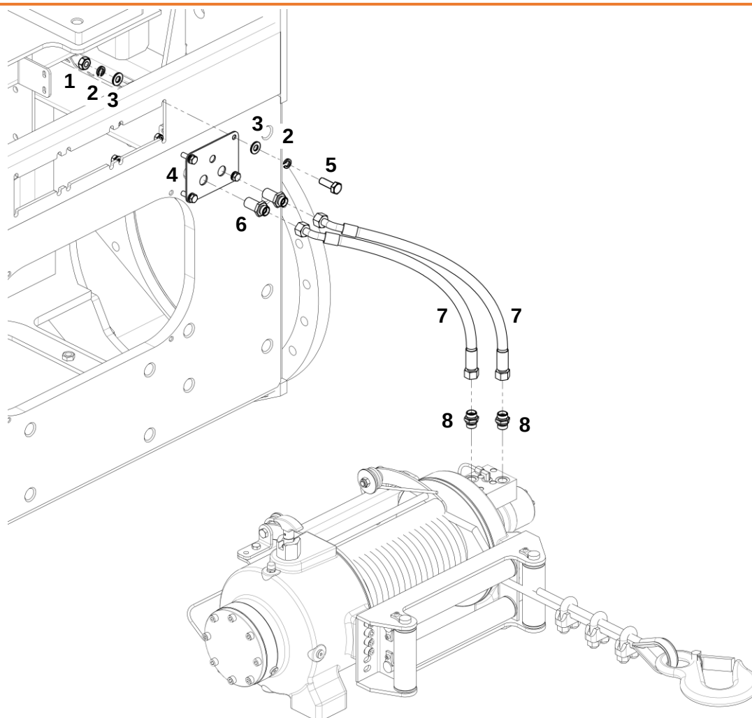
Трубопроводы лебедки
