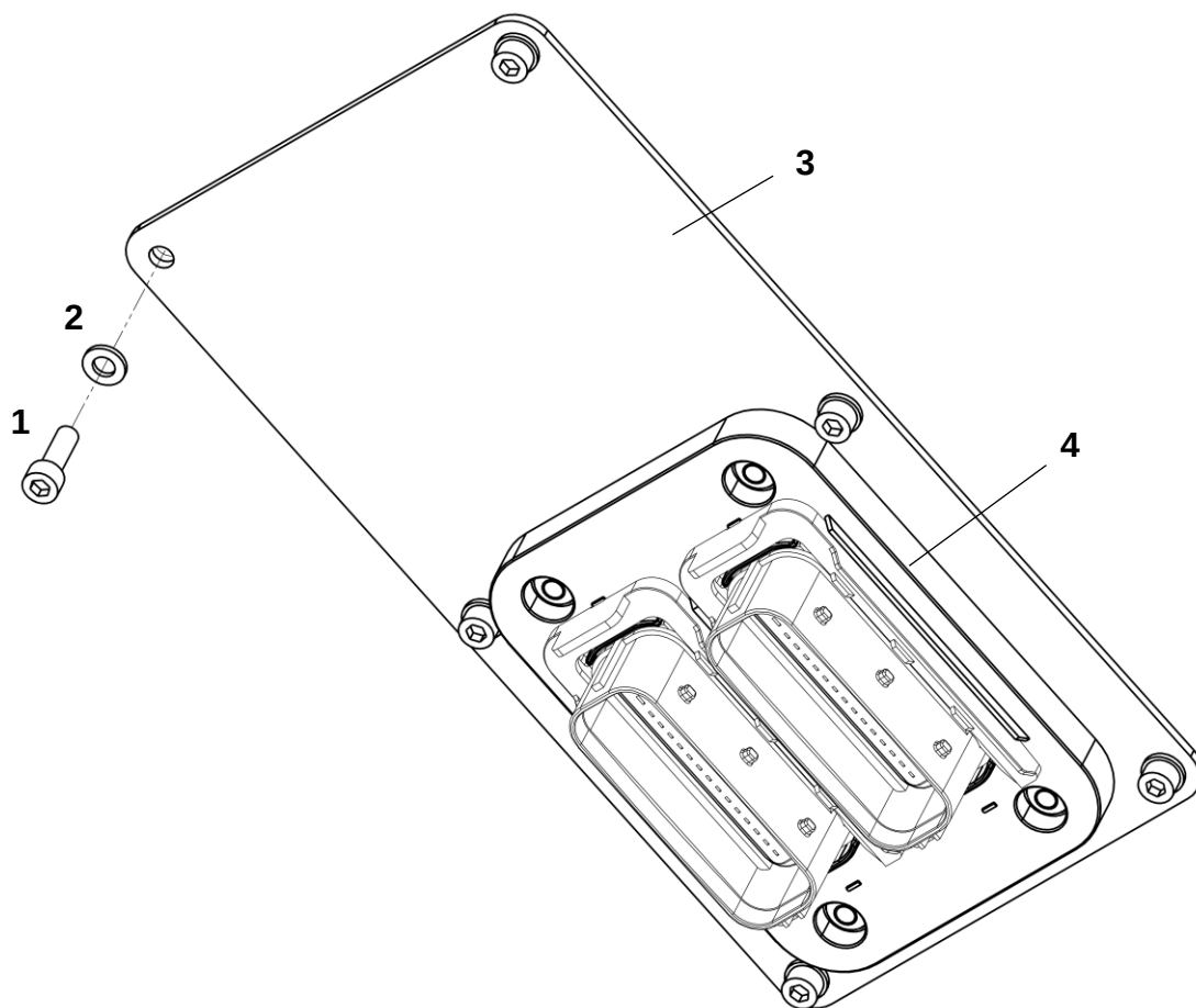
Панель переходная
