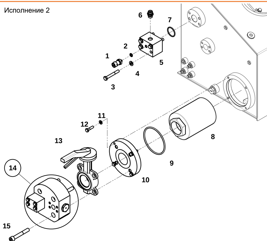
Компоненты гидравлического бака
