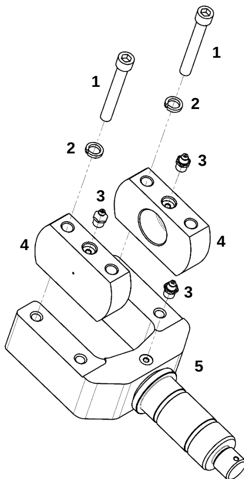
Вилка в сборе
