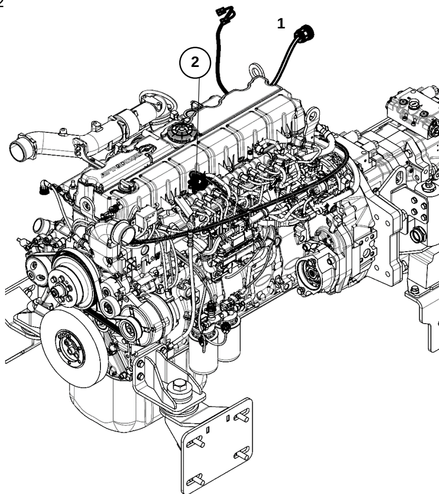
Жгут двигателя ЯМЗ 536
