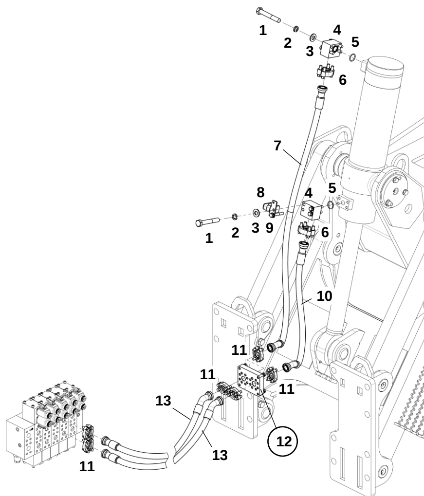
Трубопроводы заднего навесного оборудования
