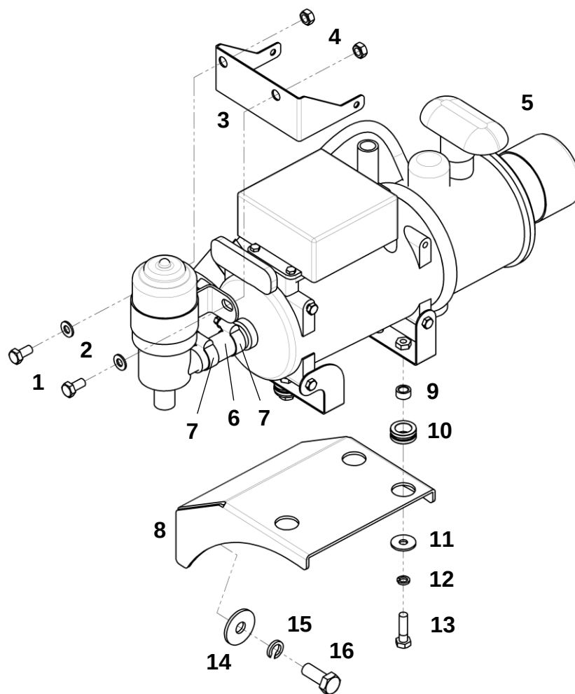
Предпусковой жидкостный подогреватель
