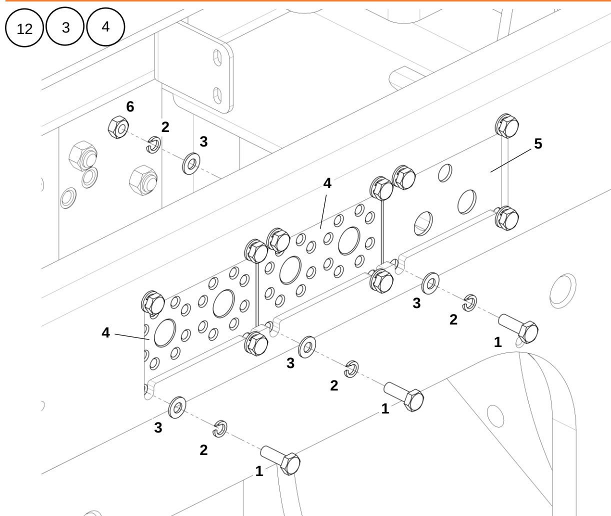
Установка переходных плит и щитка
