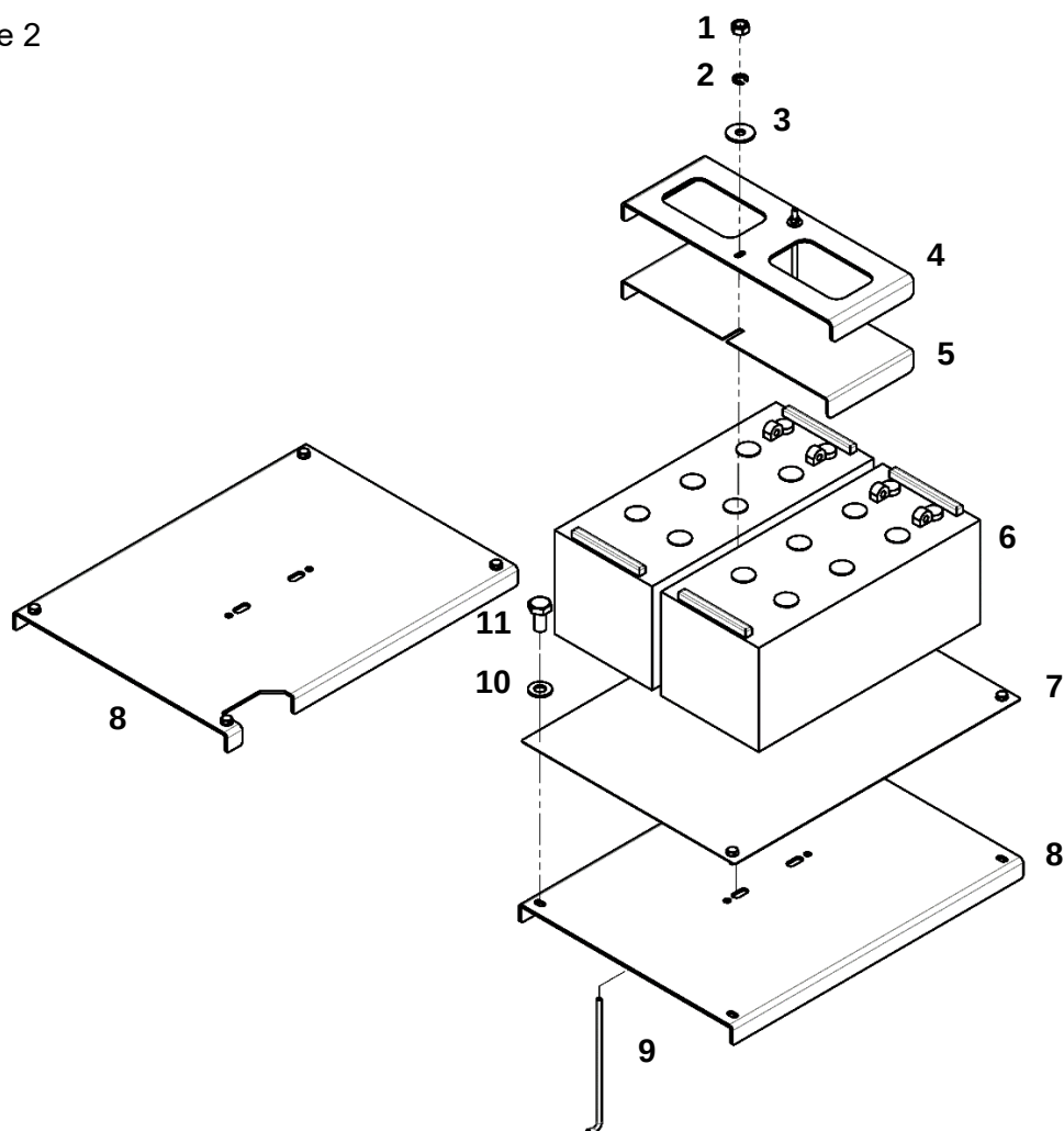
Батареи аккумуляторные с элементами крепежа
