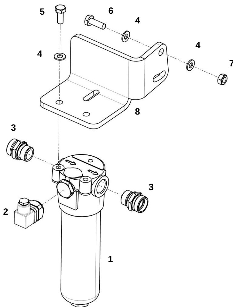
Фильтр в сборе
