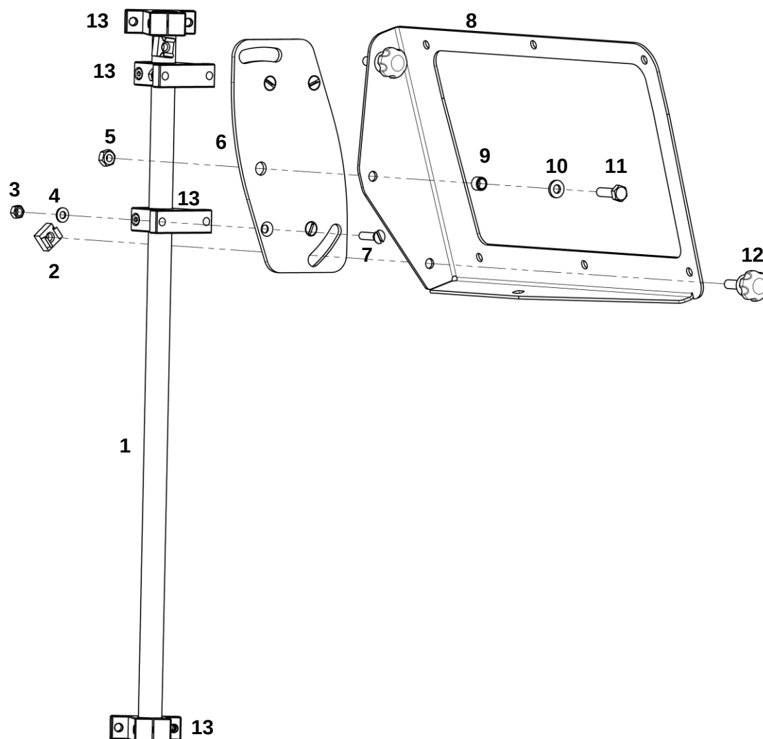
Кронштейн дисплея
