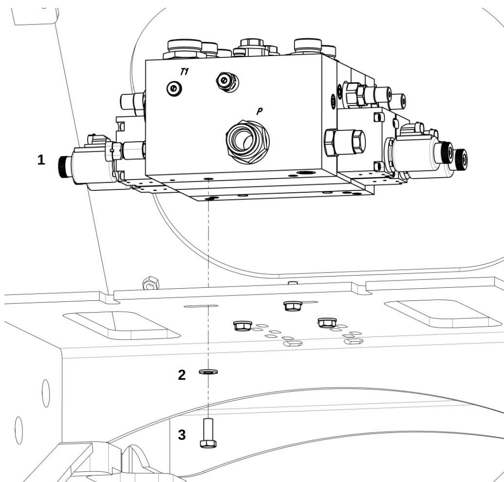
Крепление гидрораспределителя
