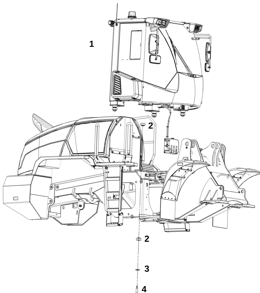
Кабина
