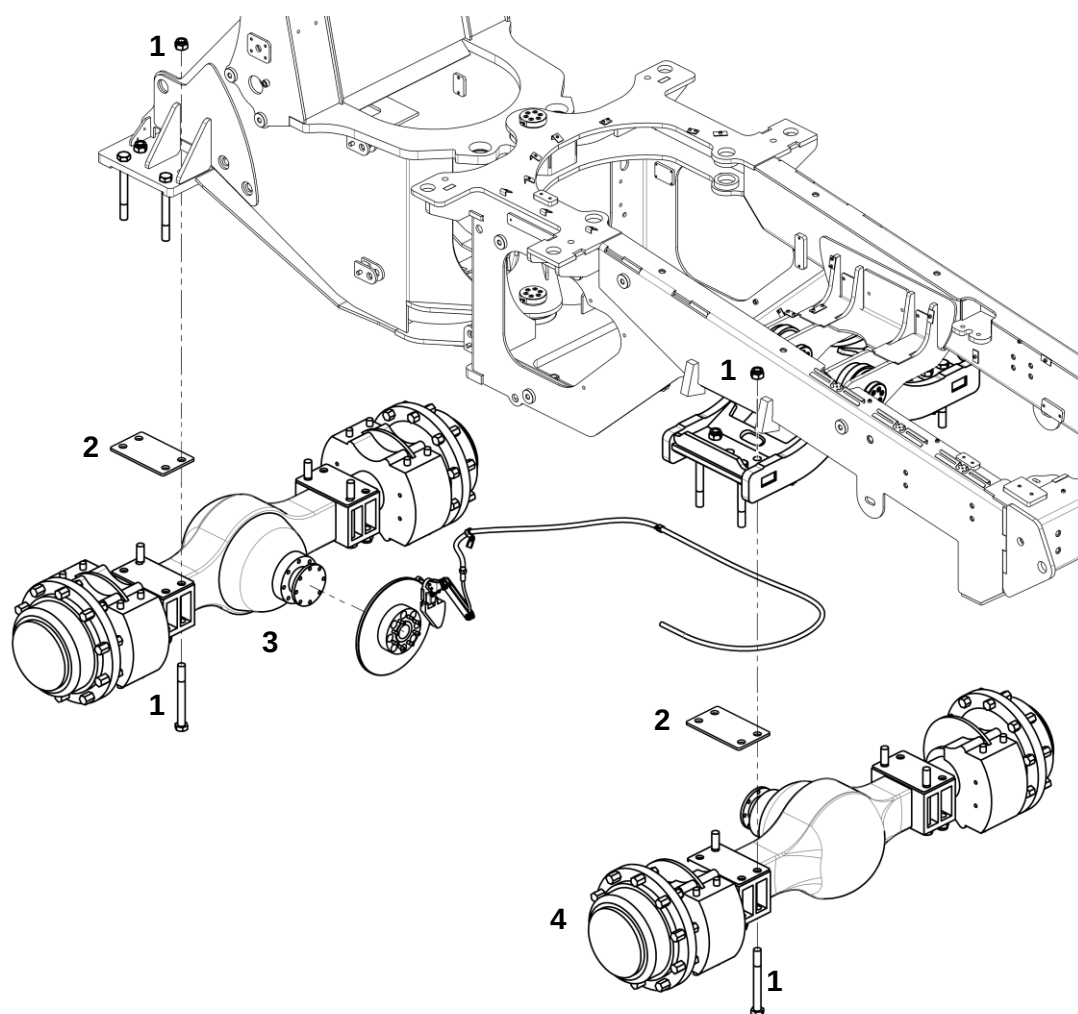
Ходовая система
