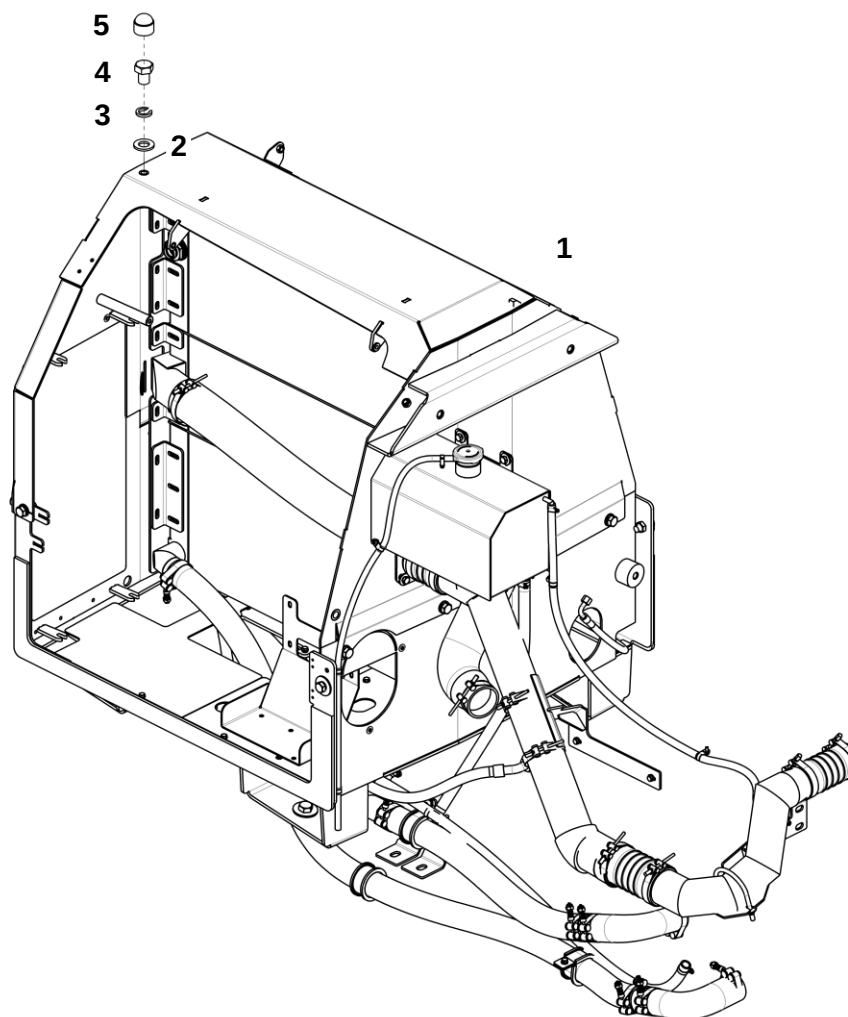
Система охлаждения
