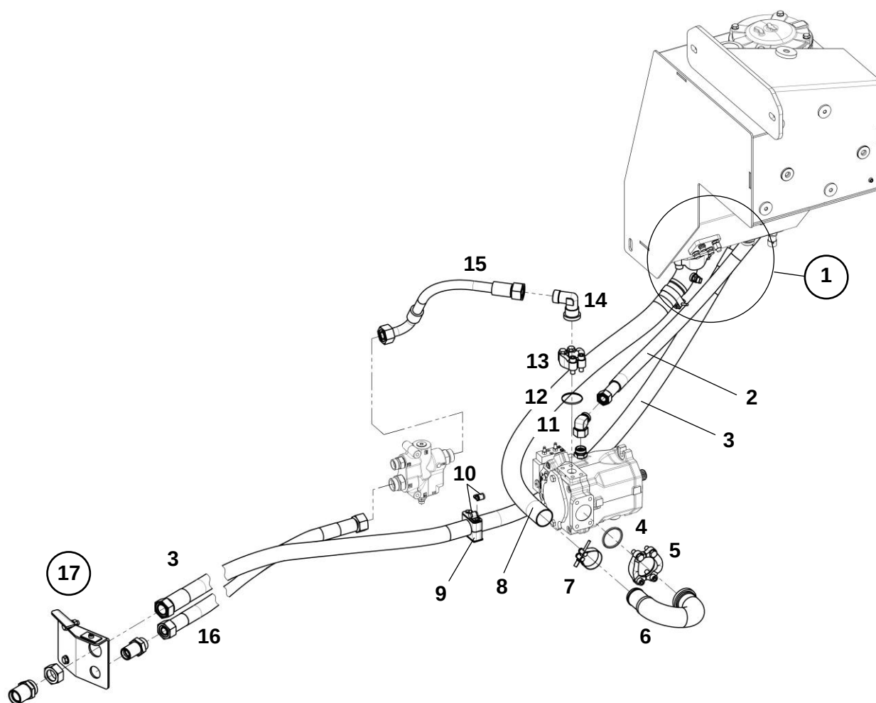
Гидравлика навесного оборудования
