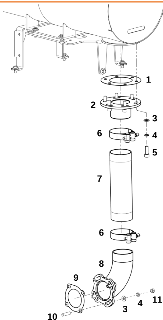
Система впуска воздуха и выпуска ОГ
