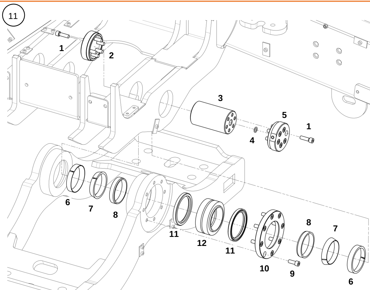
Крепление балки качения
