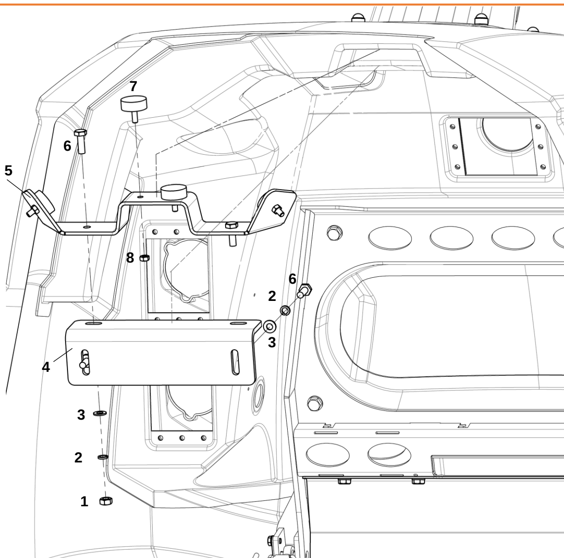
Установка капота
