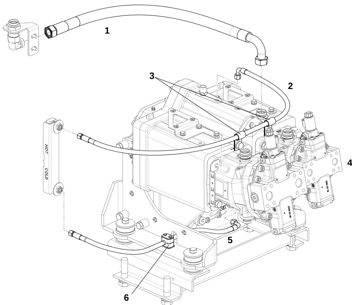
Коробка передач
