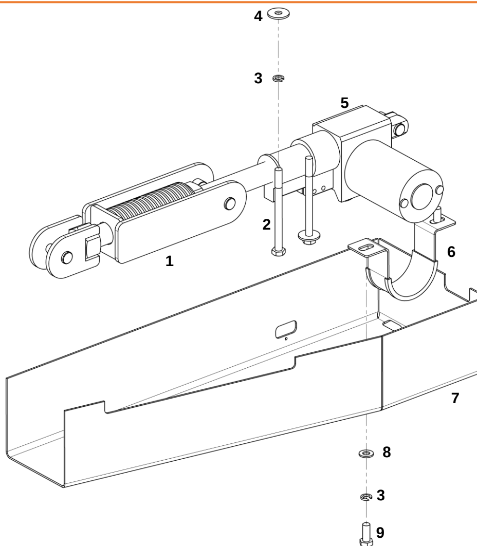
Корпус привода
