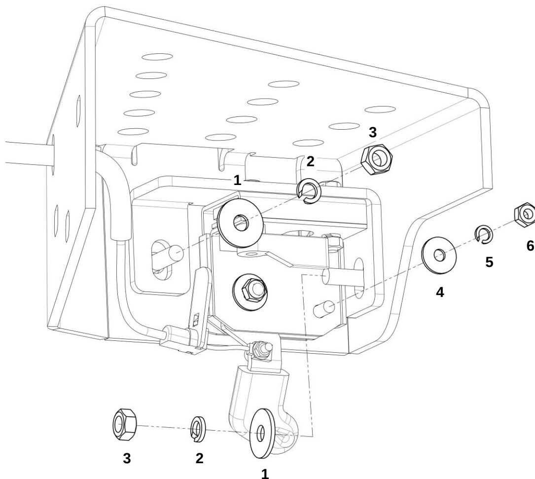
Крепление защелки кабины
