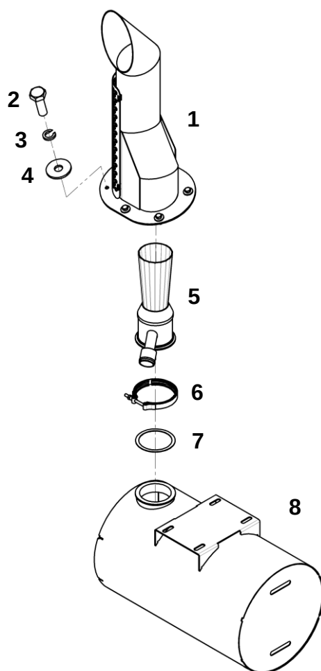
Труба выхлопная и глушитель
