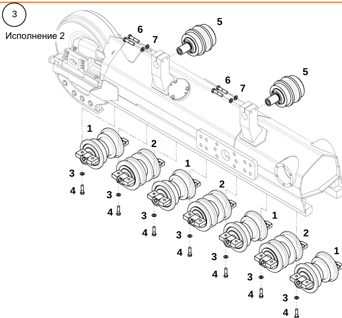
Катки опорные и поддерживающие
