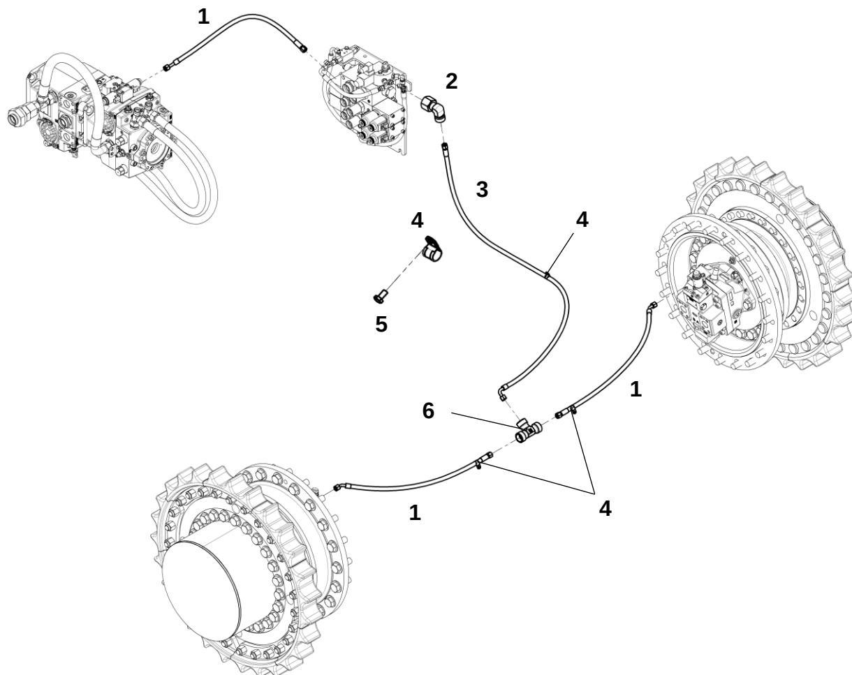
РВД растормаживания (Danfoss H1-P-130)
