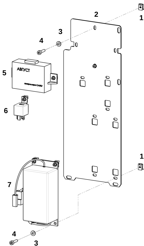
Панель в сборе
