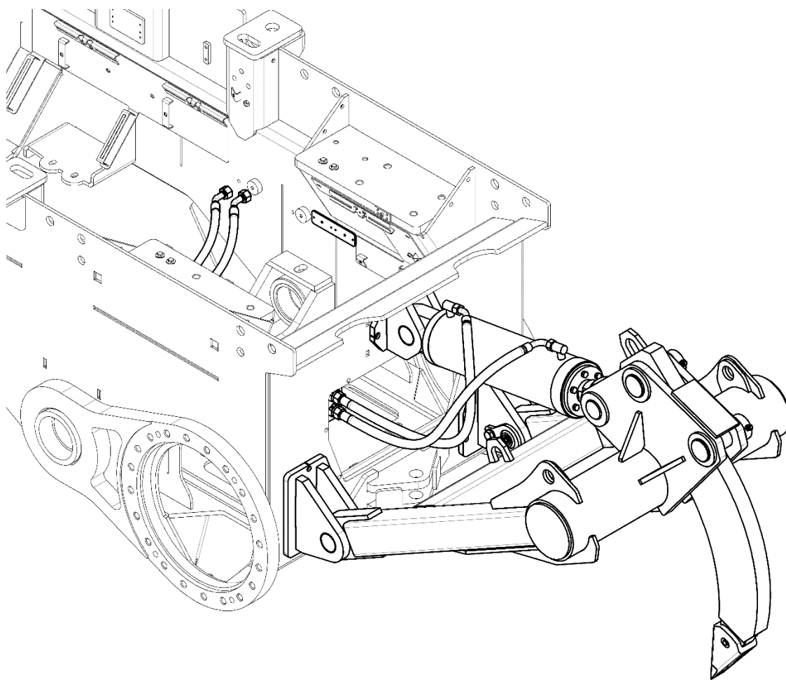
Рыхлитель однозубый в сборе
