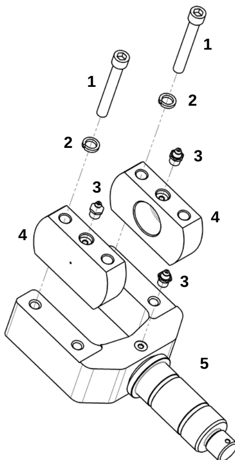
Вилка в сборе
