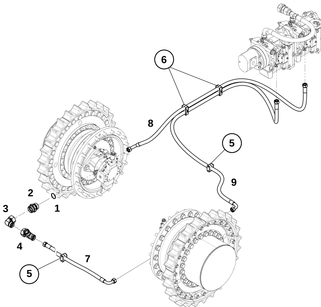
РВД дренажа гидромоторов (INI A4VG125) (Болотное исполнение)
