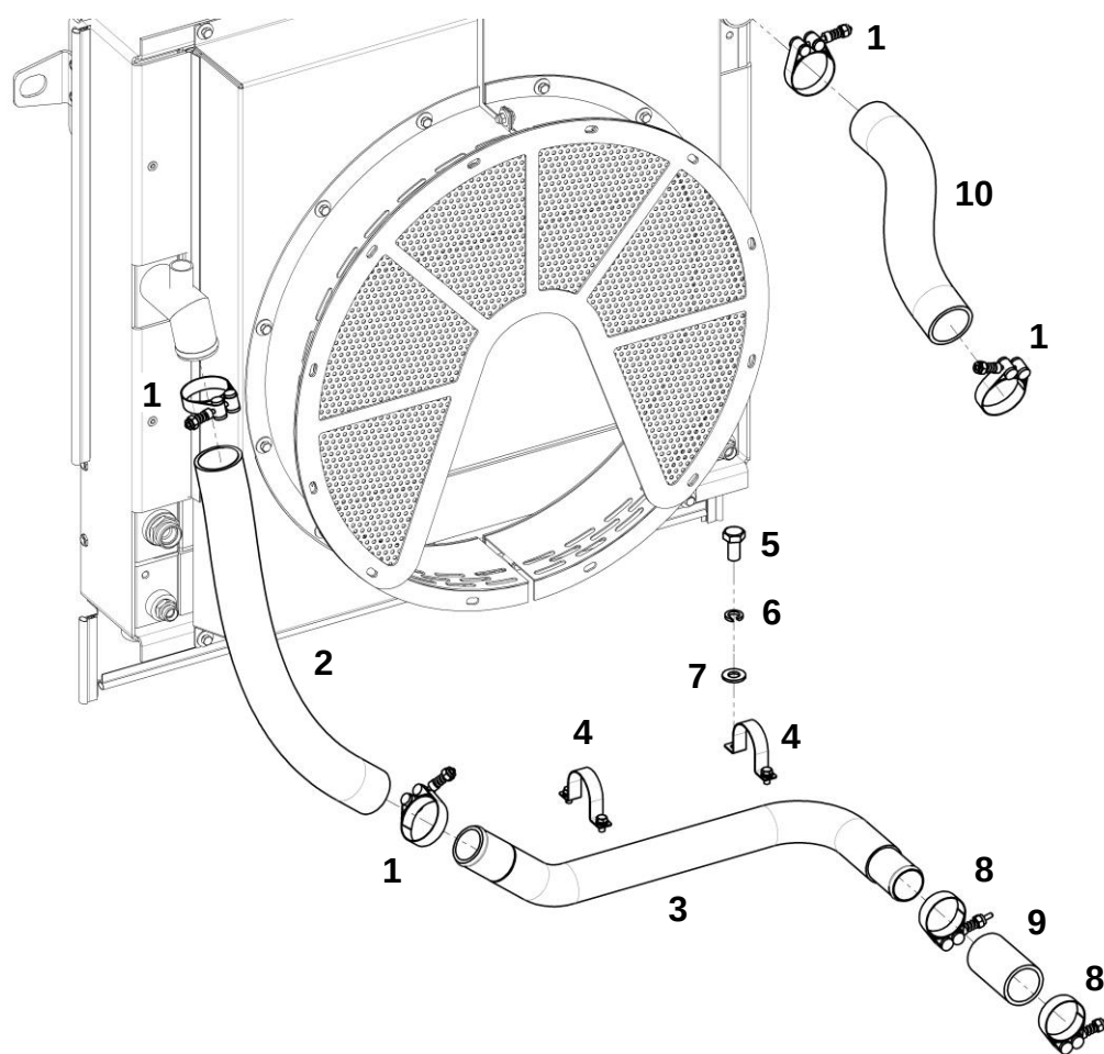
Комплект рукавов системы охлаждения
