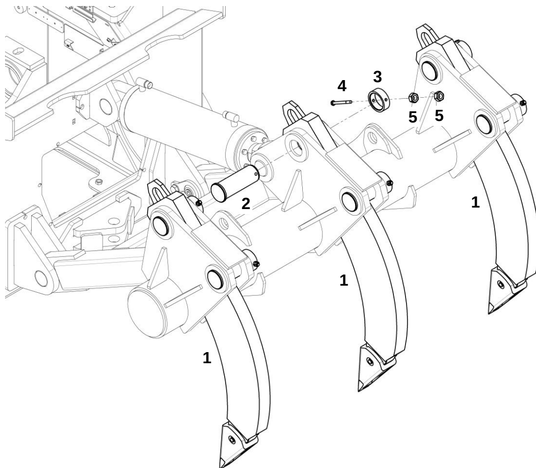
Установка ножей трехзубого рыхлителя
