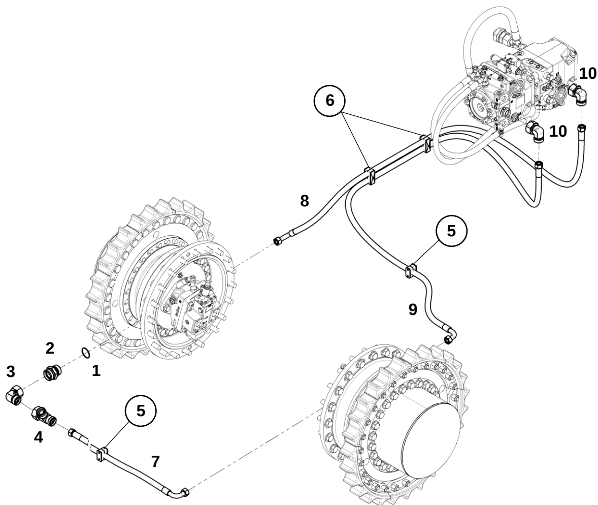
РВД дренажа гидромоторов (Danfoss H1-P-130) (Болотное исполнение)
