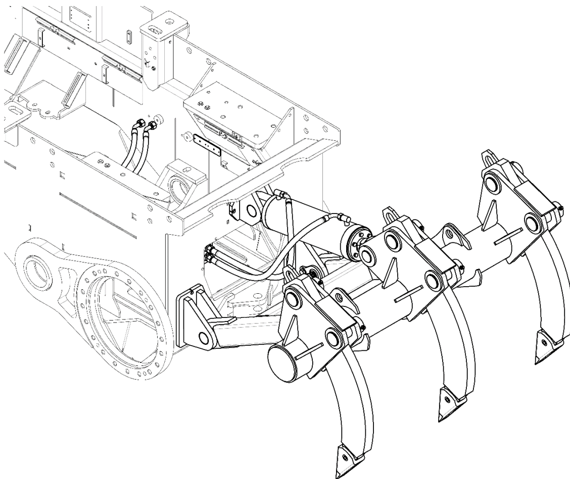
Рыхлитель трехзубый в сборе
