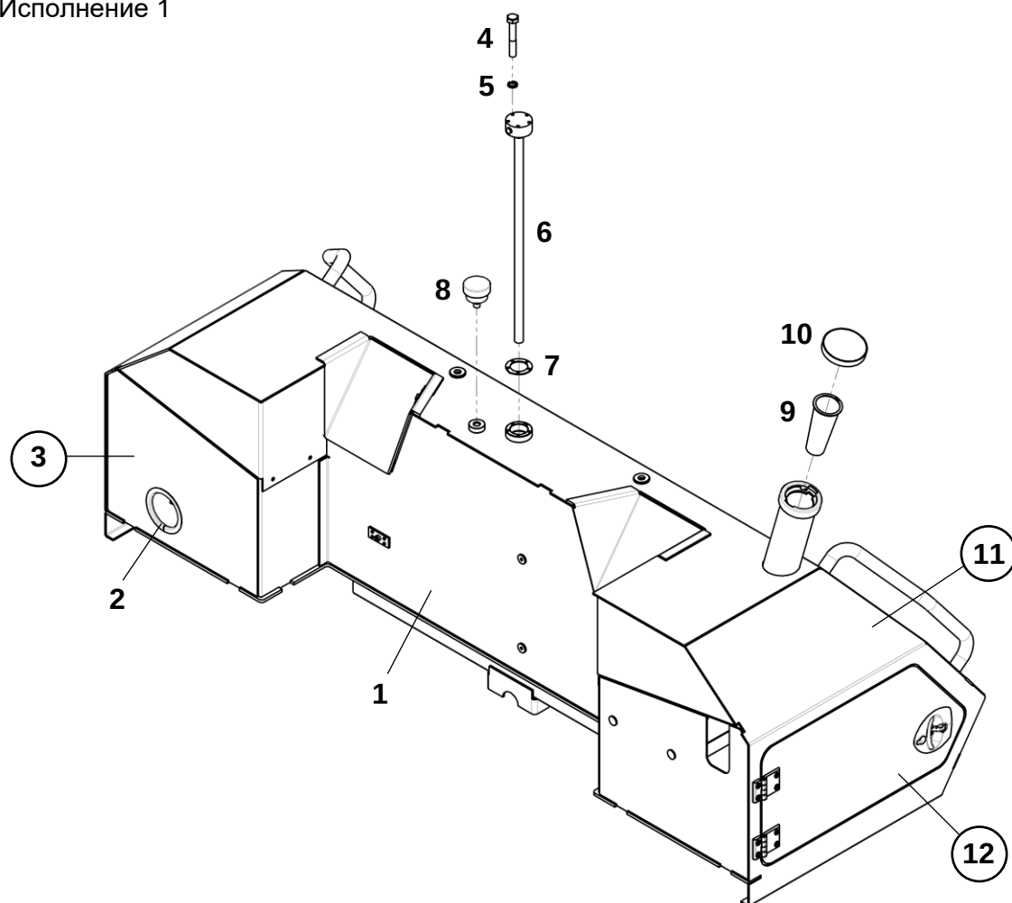
Топливный бак
