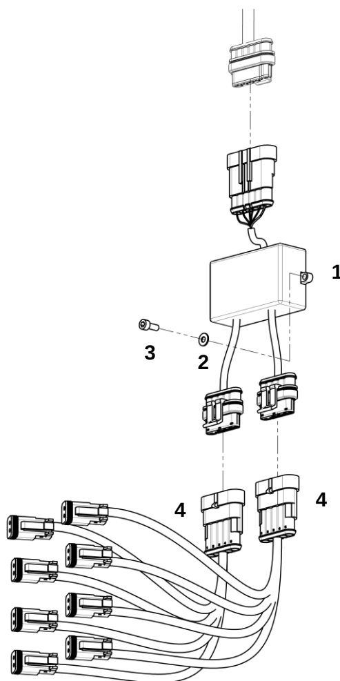
Жгуты навесного оборудования
