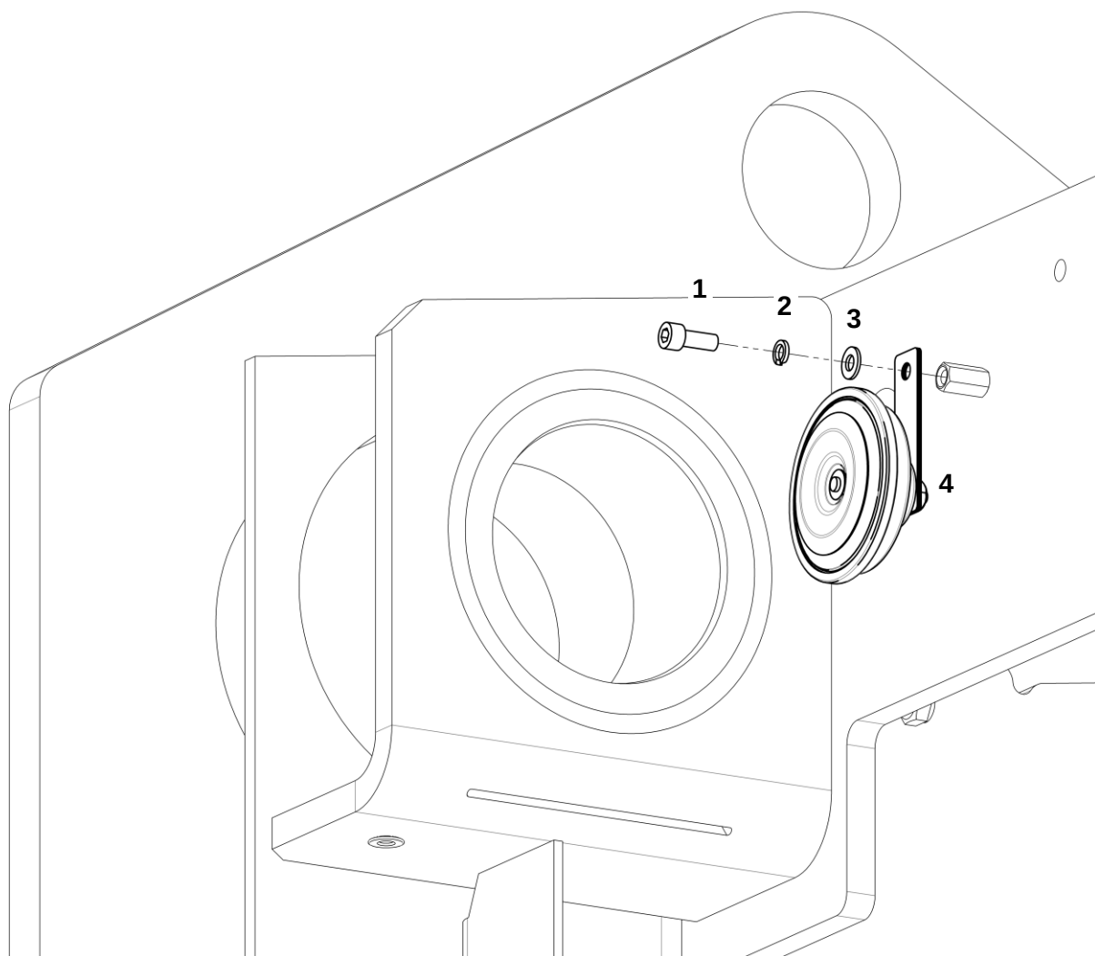
Сигналы звуковые с элементами крепежа
