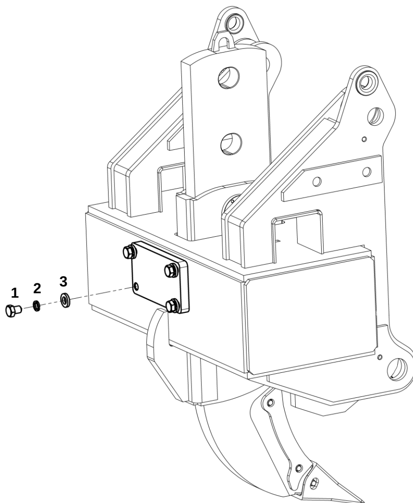
Рыхлитель 20 класса
