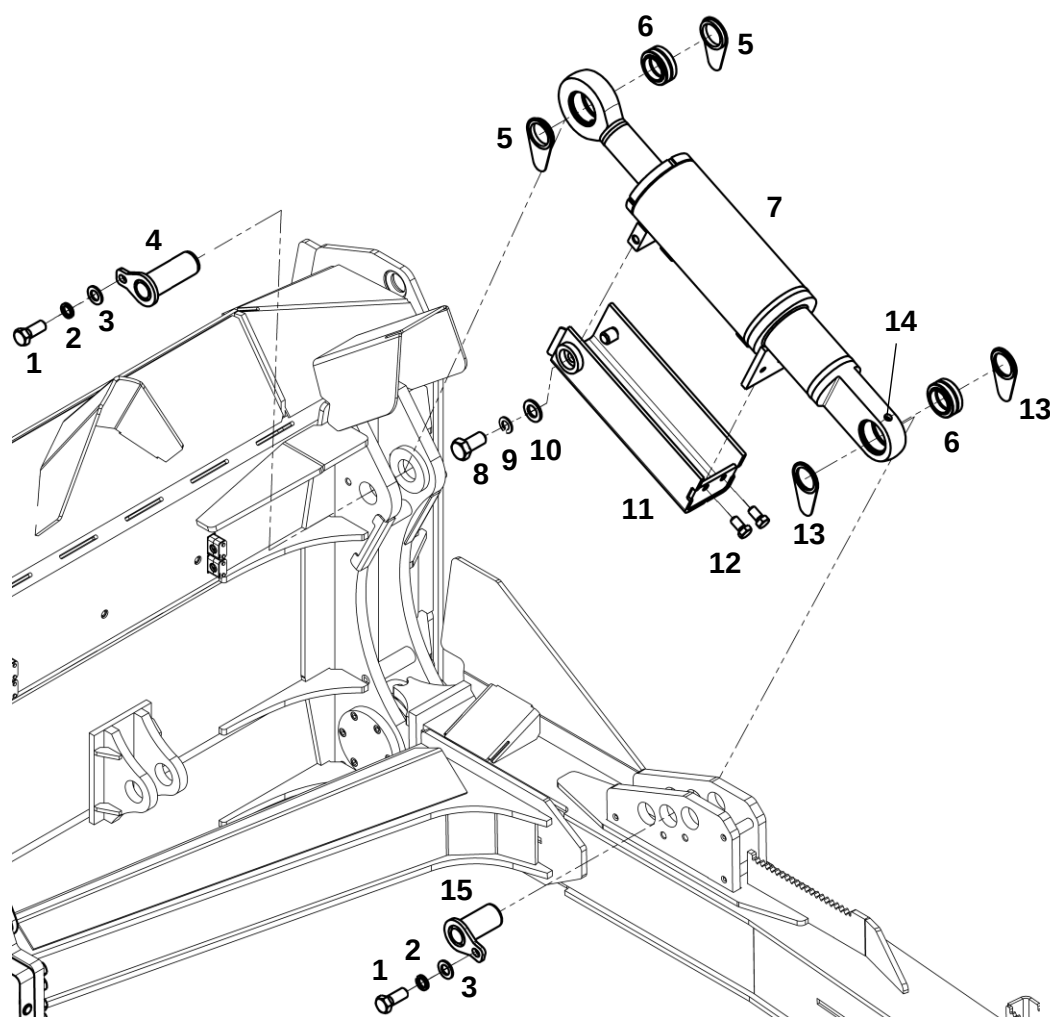
Установка ГЦ
