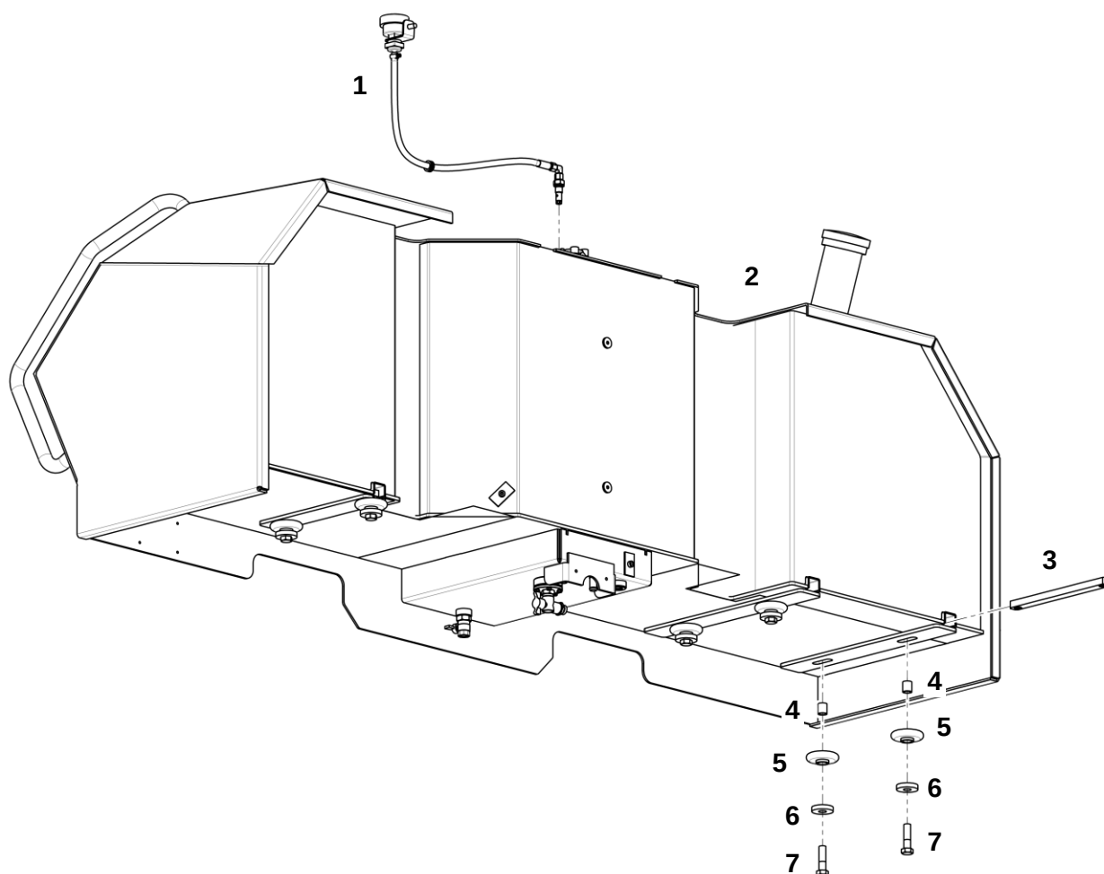
Топливная система
