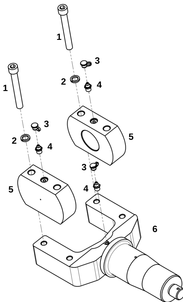
Вилка в сборе
