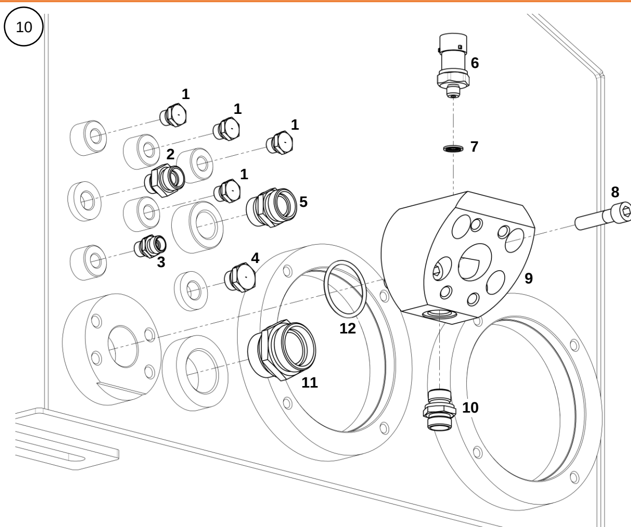
Штуцера с фланцем
