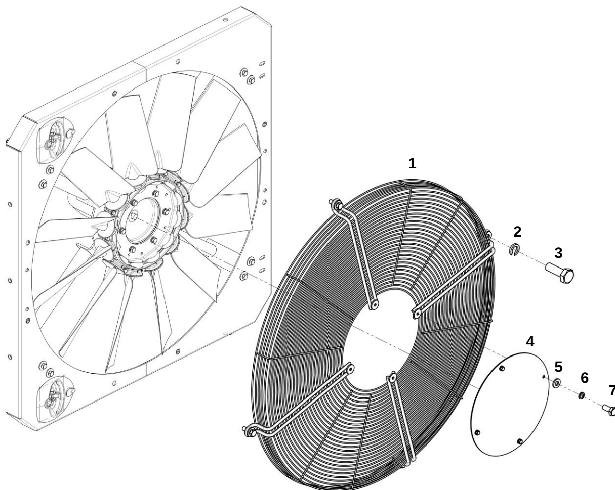
Рама с вентилятором
