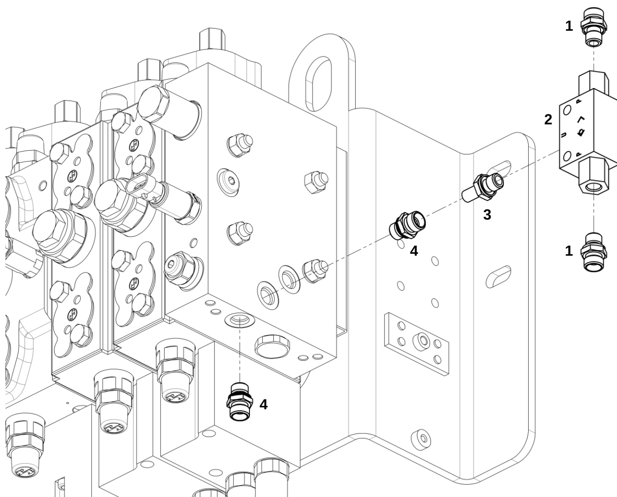
Гидрораспределитель в сборе
