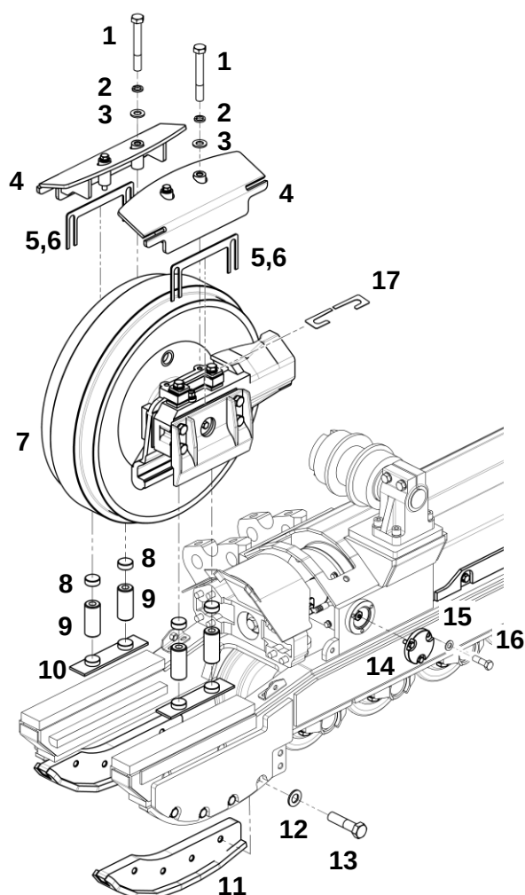
Установка колеса направляющего
