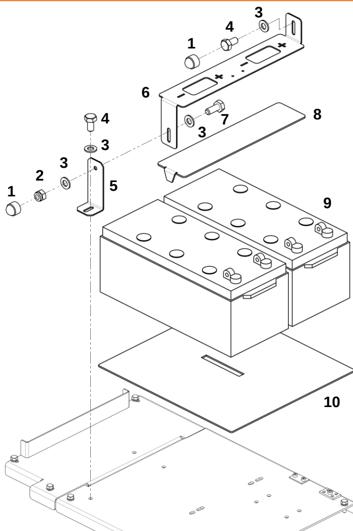
Аккумуляторные батареи с элементами крепления
