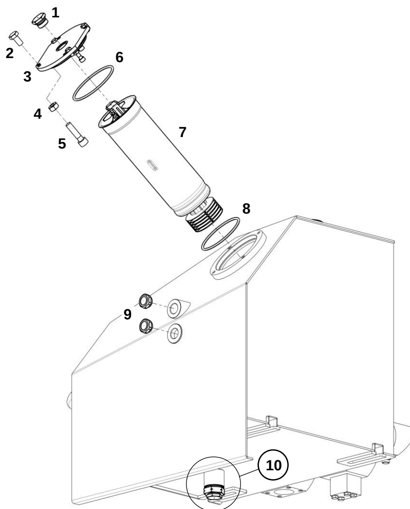
Бак гидравлический в сборе
