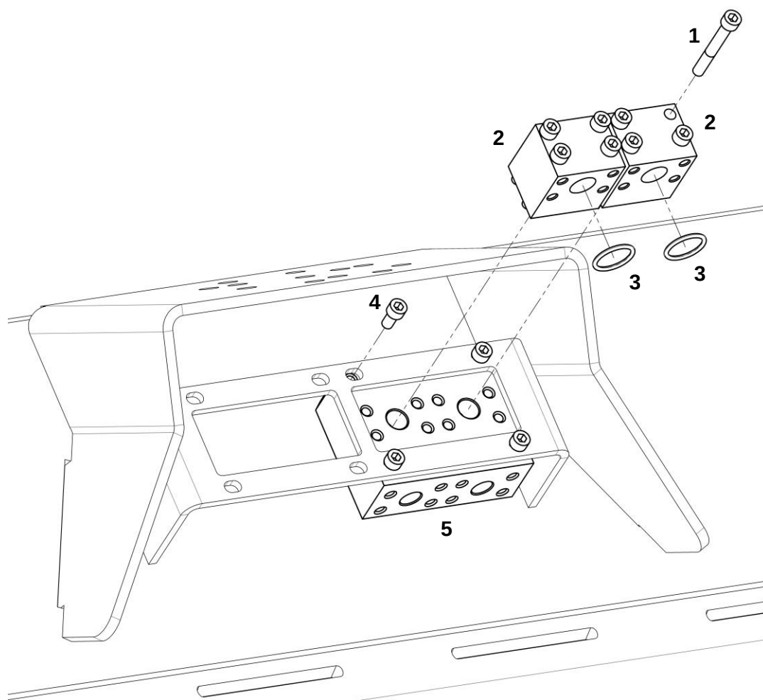
Плита переходная в сборе
