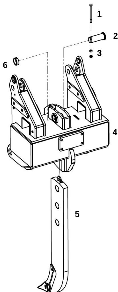
Рыхлитель 20 класса
