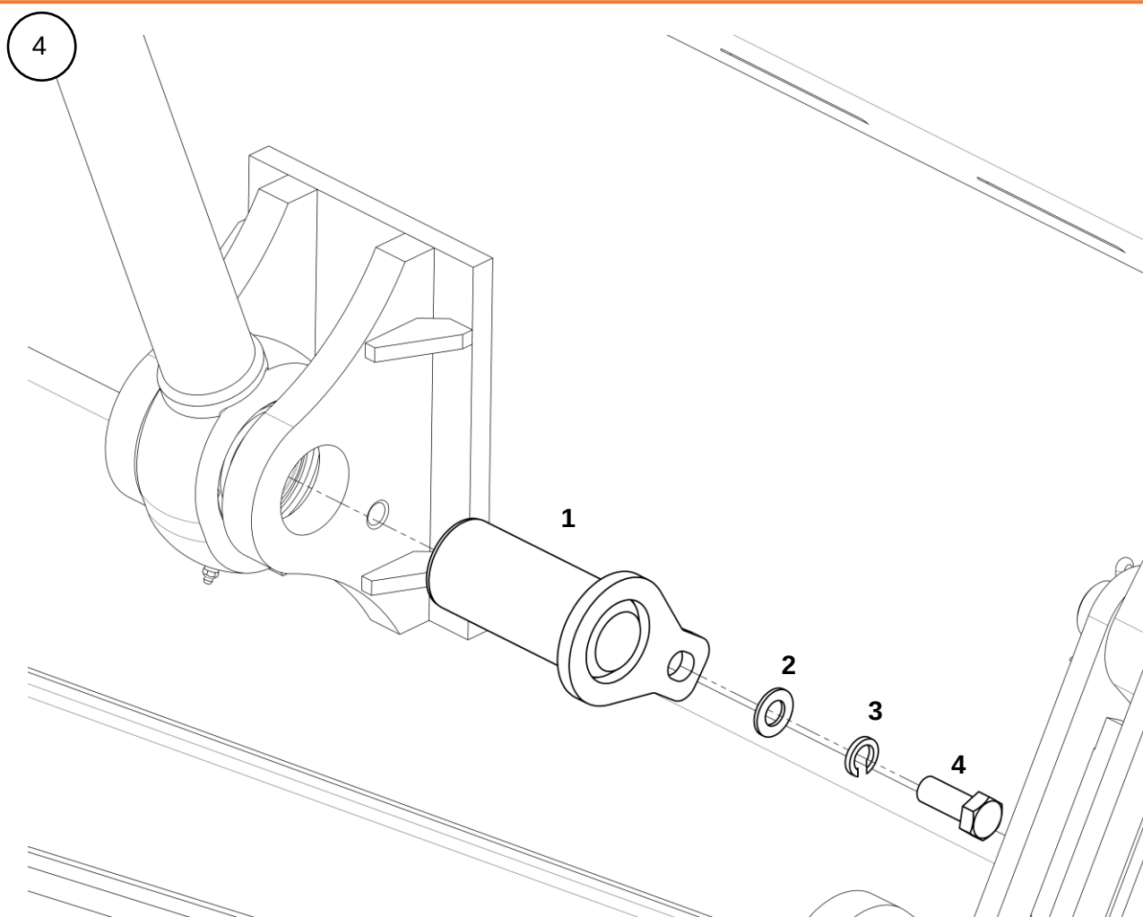
Крепление ГЦ навесного оборудования
