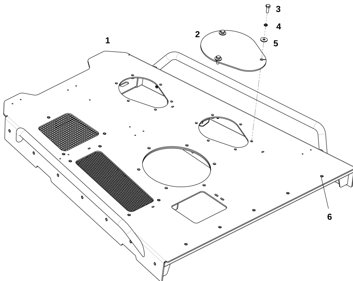
Капот
