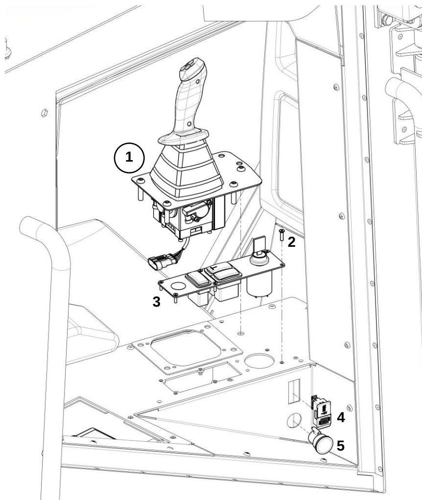
Панель управления
