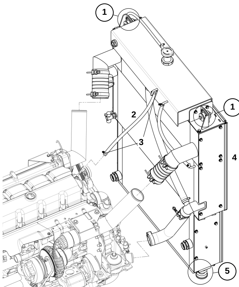
Система охлаждения
