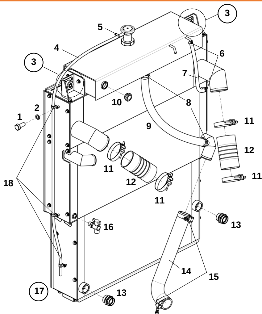
Блок радиаторов в сборе
