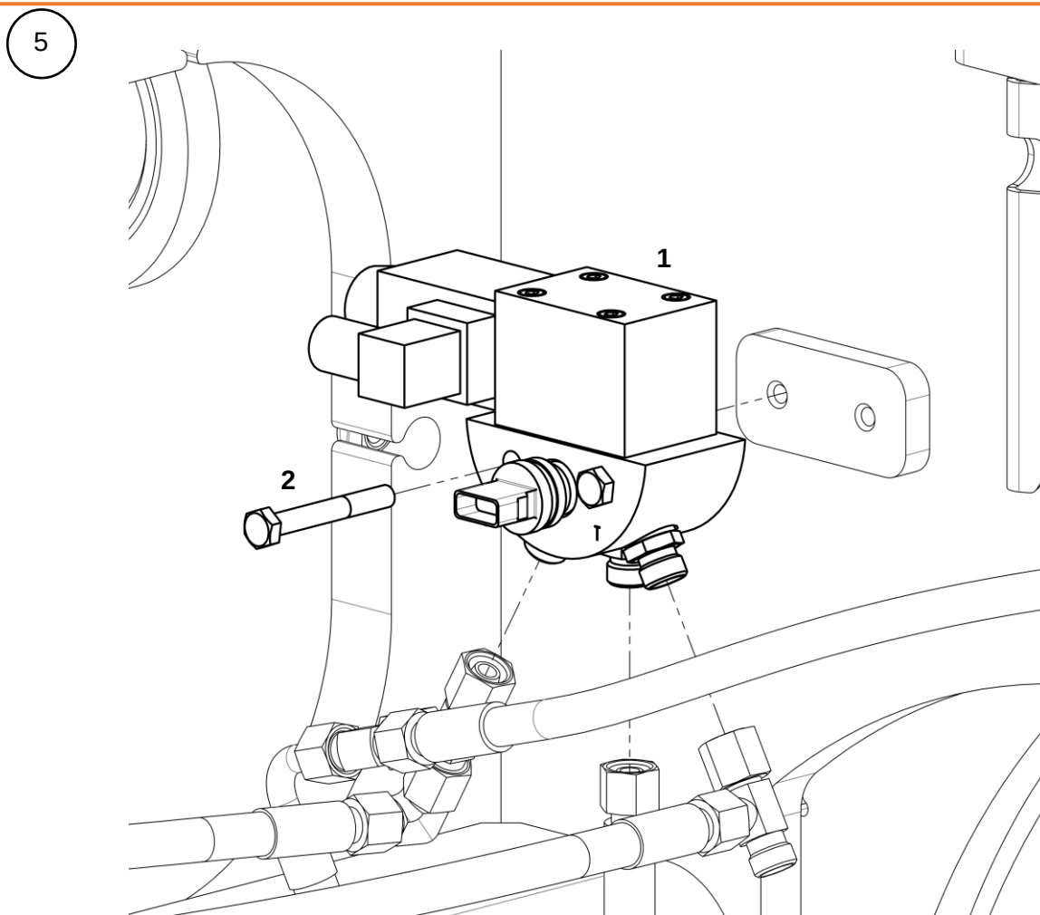
Крепление тормозной плиты
