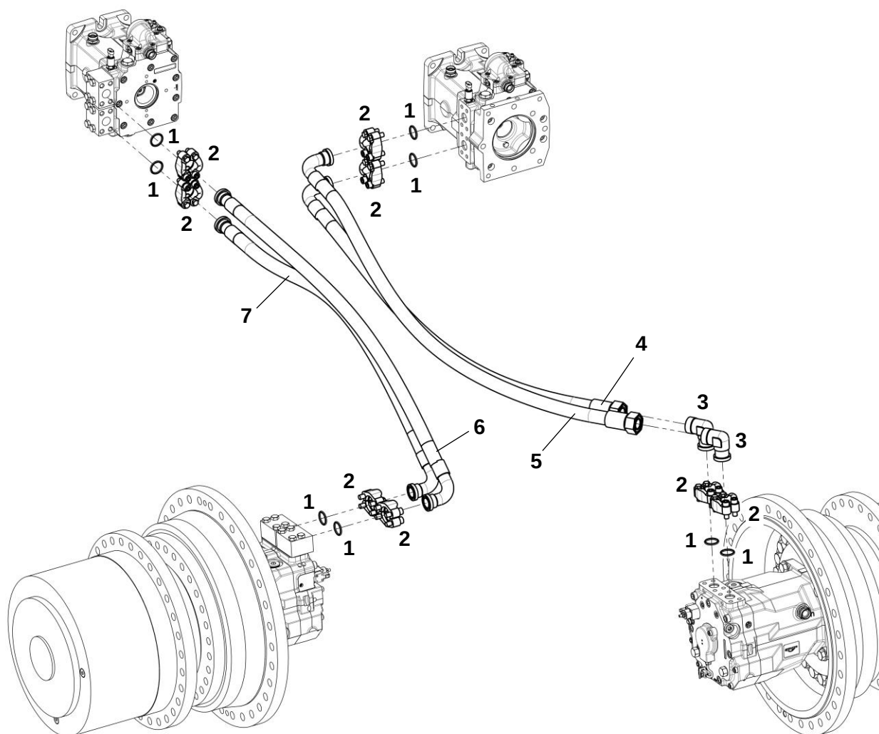
Трубопроводы гидросистемы трансмиссии
