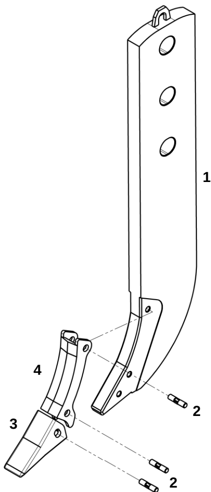
Нож
