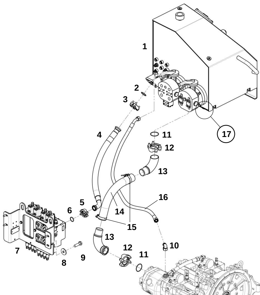
Трубопроводы гидросистемы навесного оборудования
