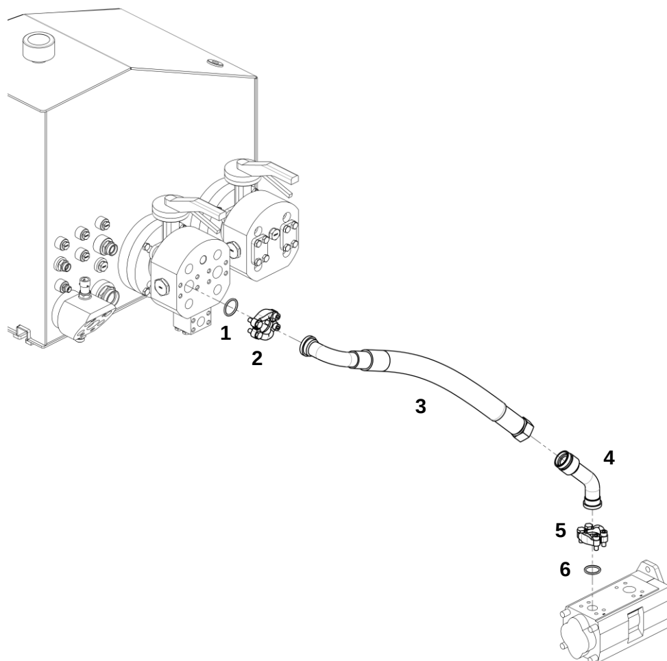
Трубопроводы гидропривода вентилятора
