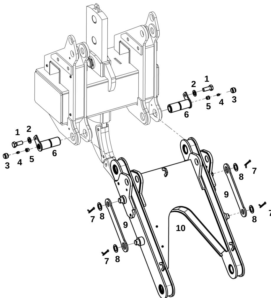
Рыхлитель 20 класса
