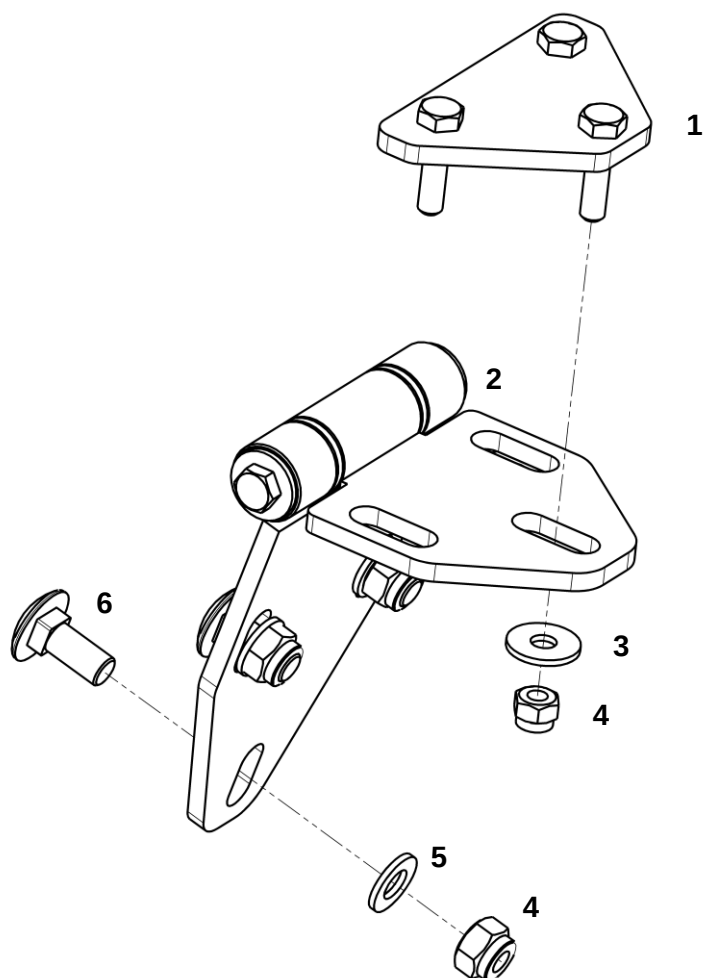
Петля в сборе
