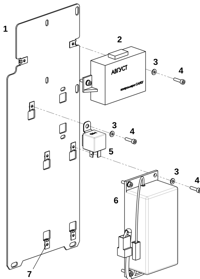
Панель в сборе
