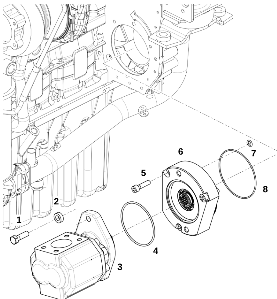
Установка насоса подпитки
