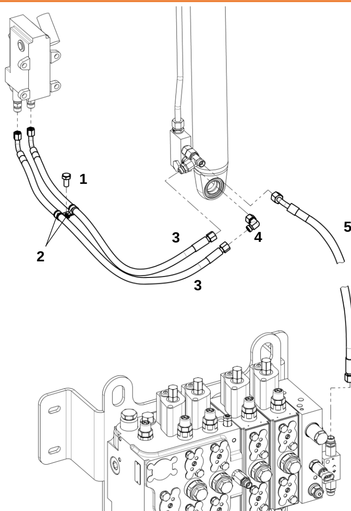
Трубопроводы гидросистемы подъема кабины
