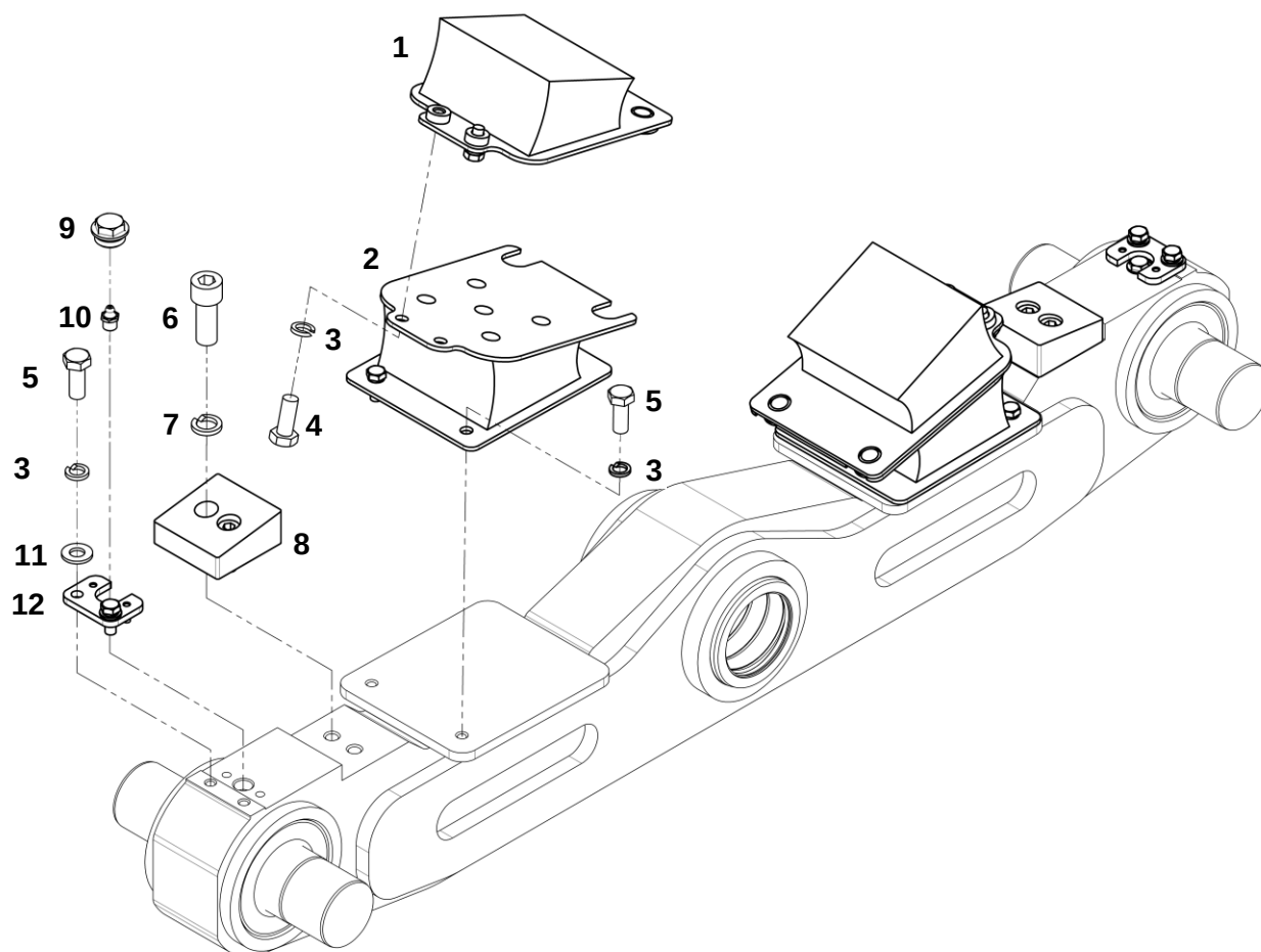
Балка балансирующая
