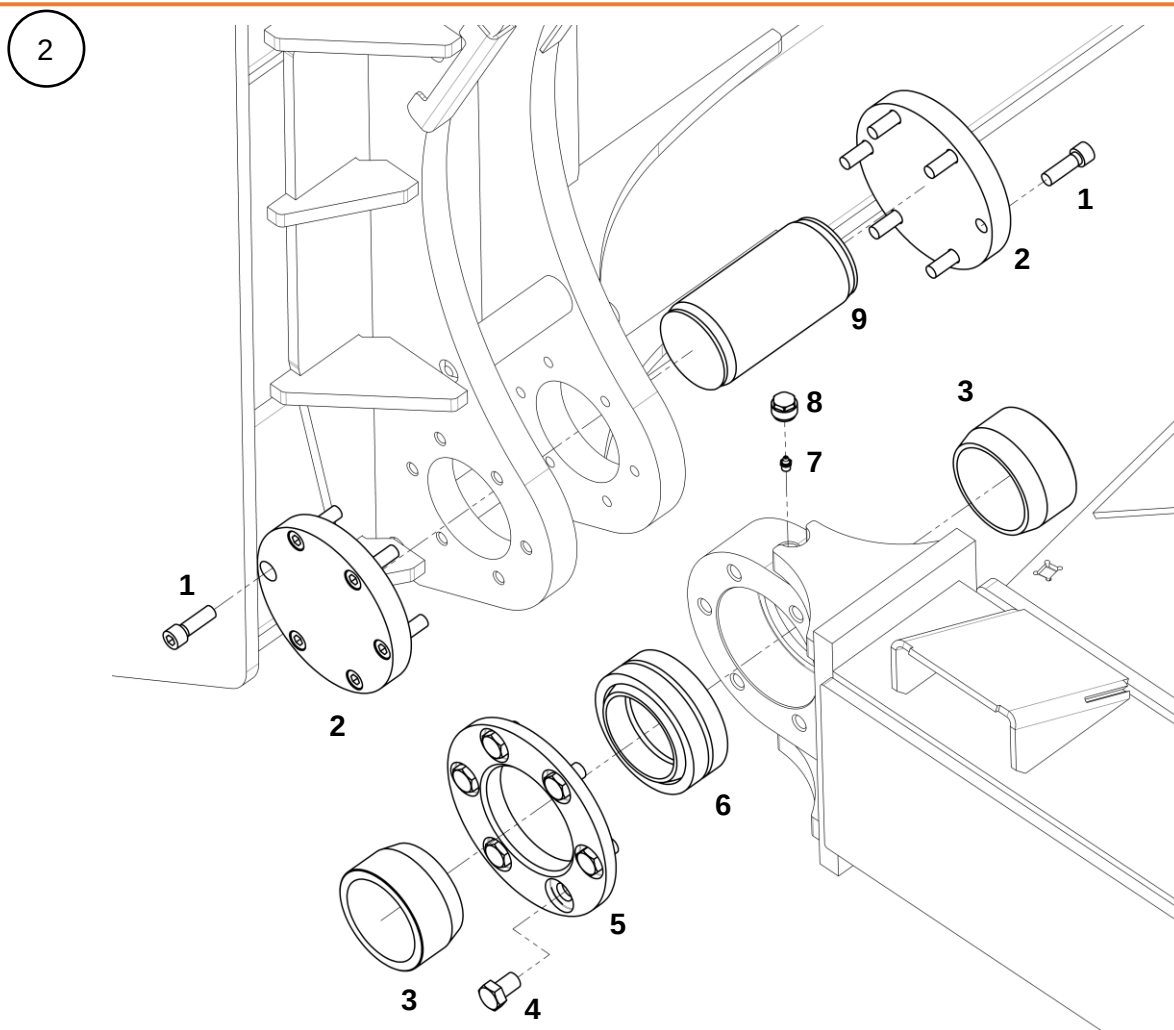
Крепление рамы к зеркалу
