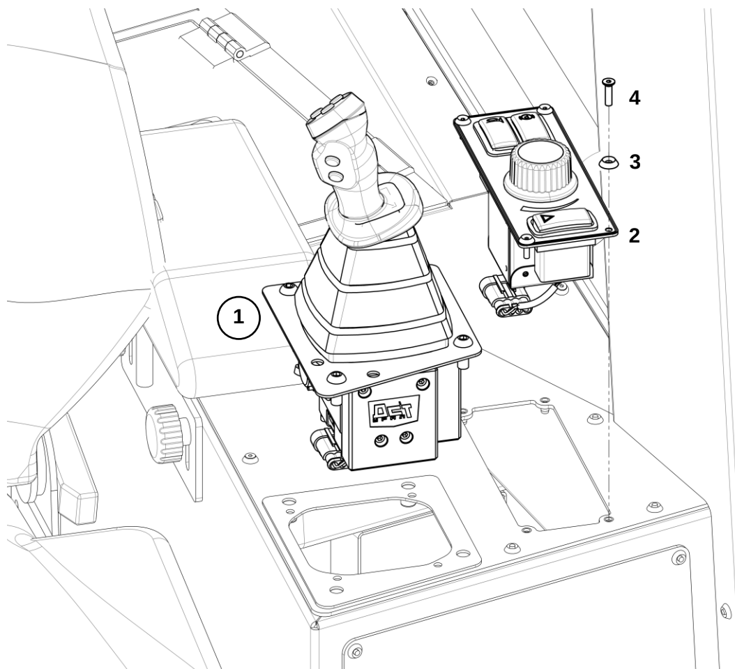
Пульт управления левый
