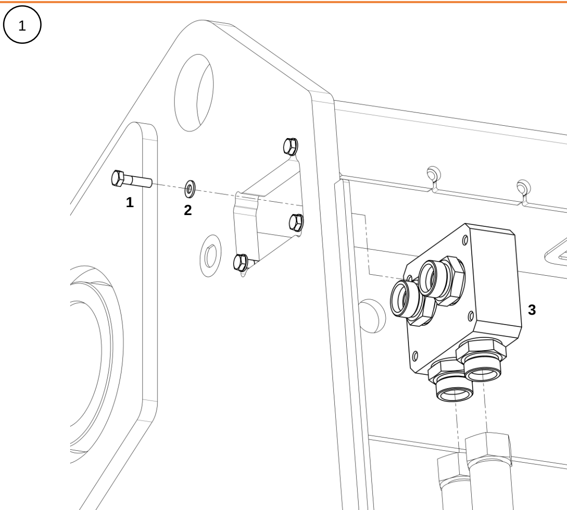
Плита переходная с креплением
