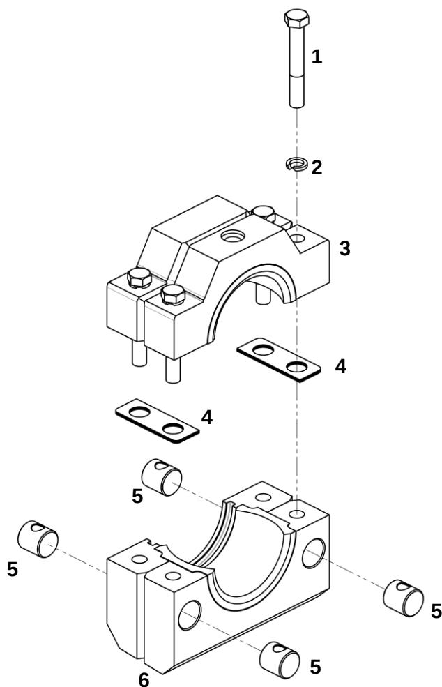
Бугель
