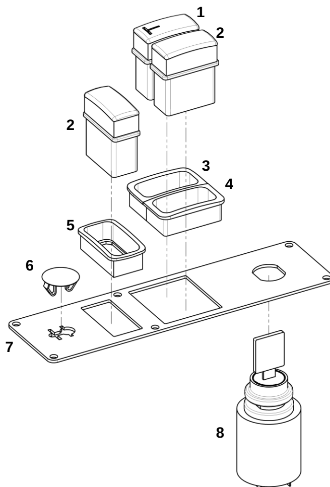
Панель управления
