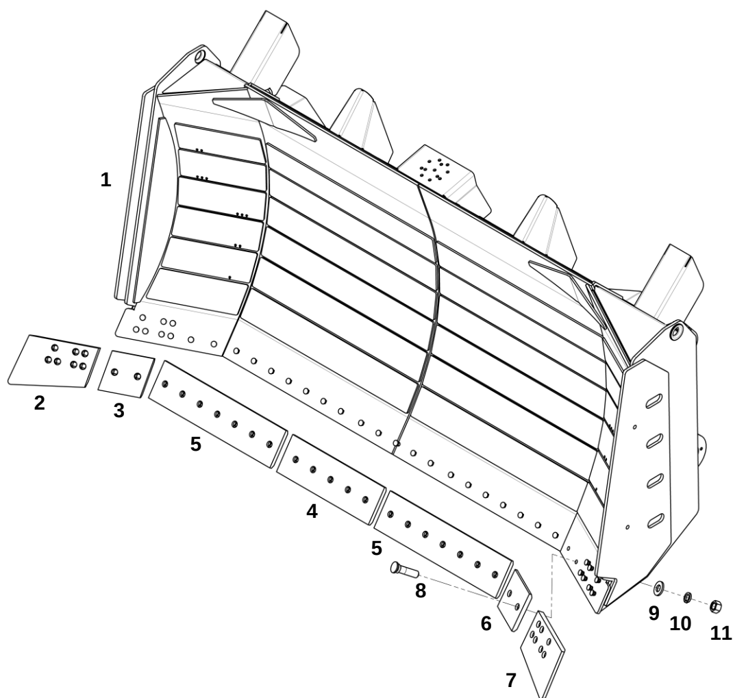
Зеркало в сборе
