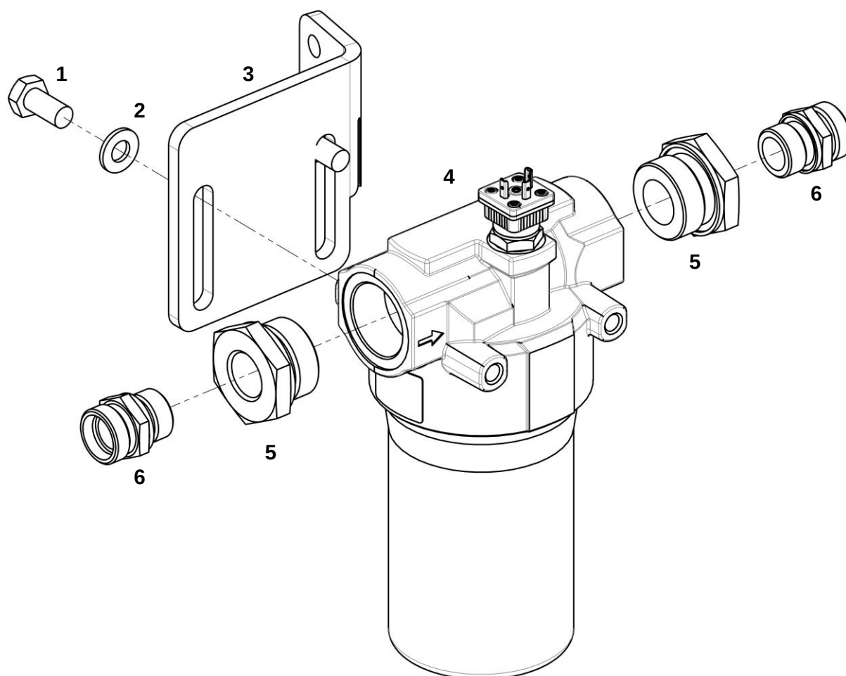
Фильтр в сборе
