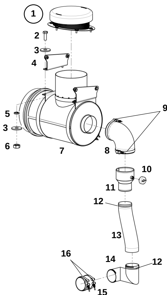
Система впуска воздуха и выпуска ОГ (впуск)
