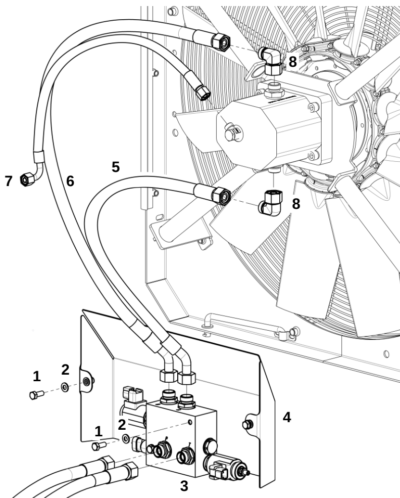
Подключение к гидромотору вентилятора
