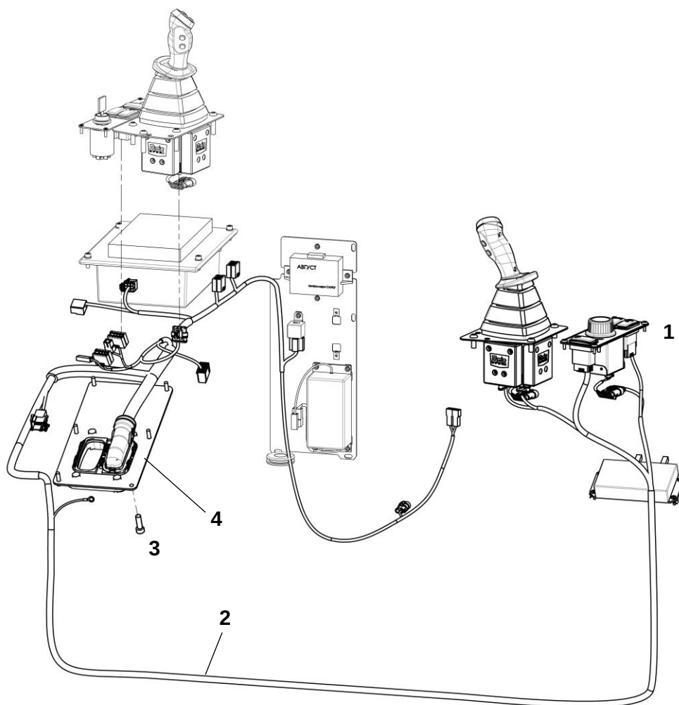
Электрооборудование кабины
