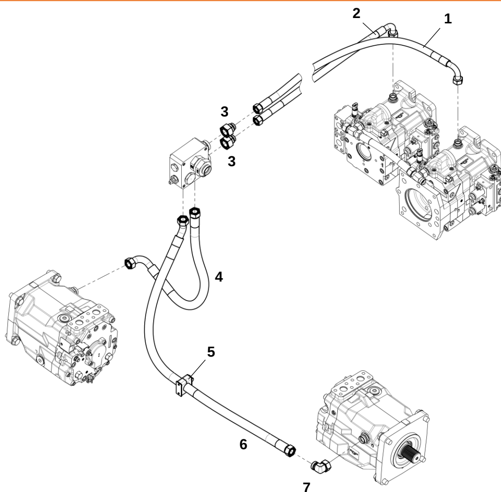
Трубопроводы гидросистемы трансмиссии
