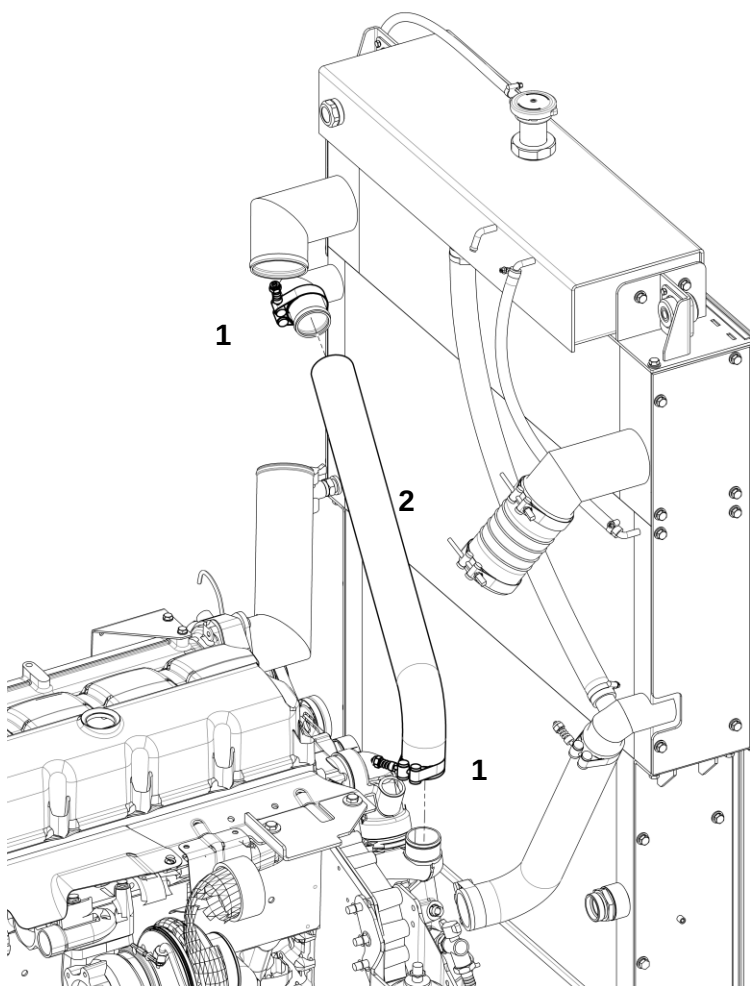
Система охлаждения
