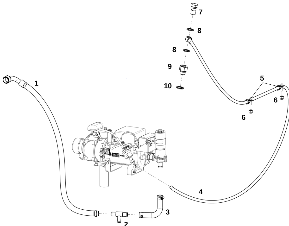
Система предпускового подогрева
