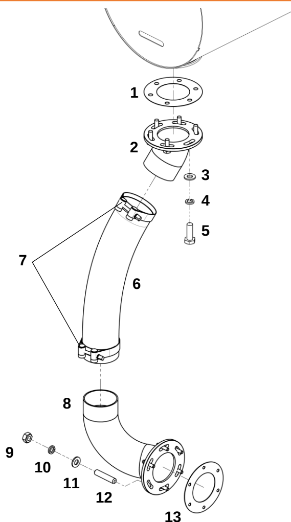
Система впуска воздуха и выпуска ОГ (выпуск)
