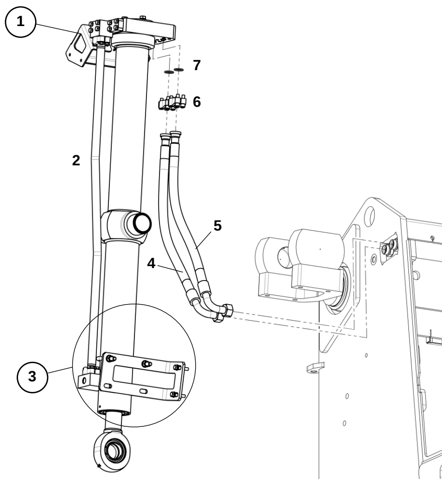
Гидроцилиндры переднего навесного оборудования
