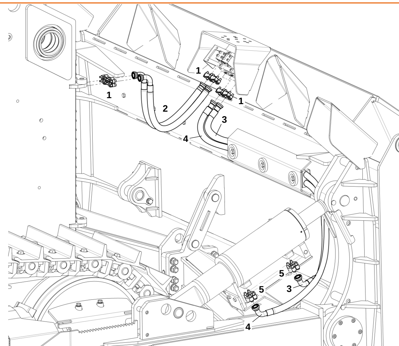
Установка бульдозерного оборудования
