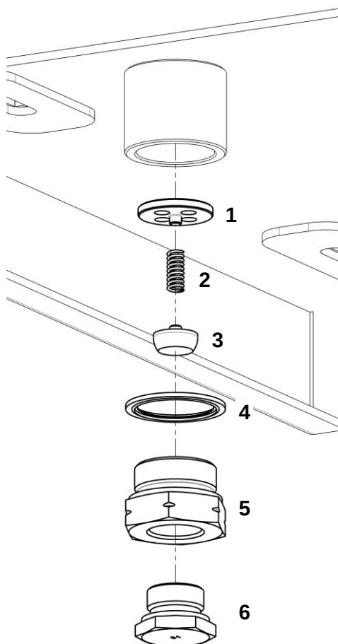
Пробка сливная в сборе
