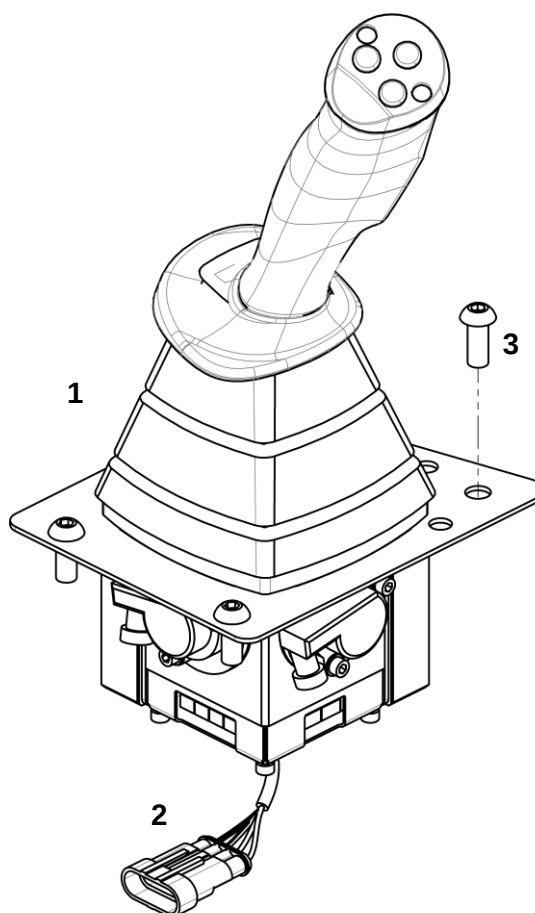
Джойстик в сборе
