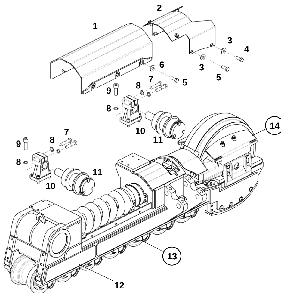
Тележка
