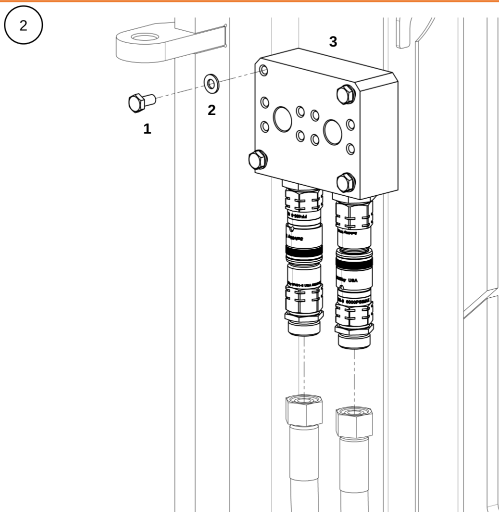
Плита с креплением
