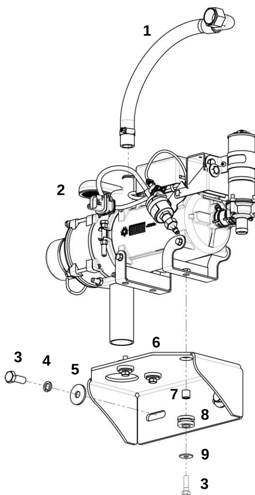
Система предпускового подогрева
