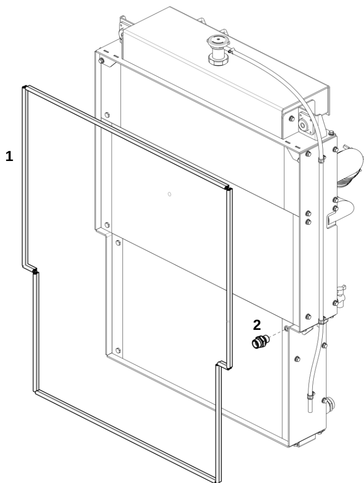
Блок радиаторов в сборе
