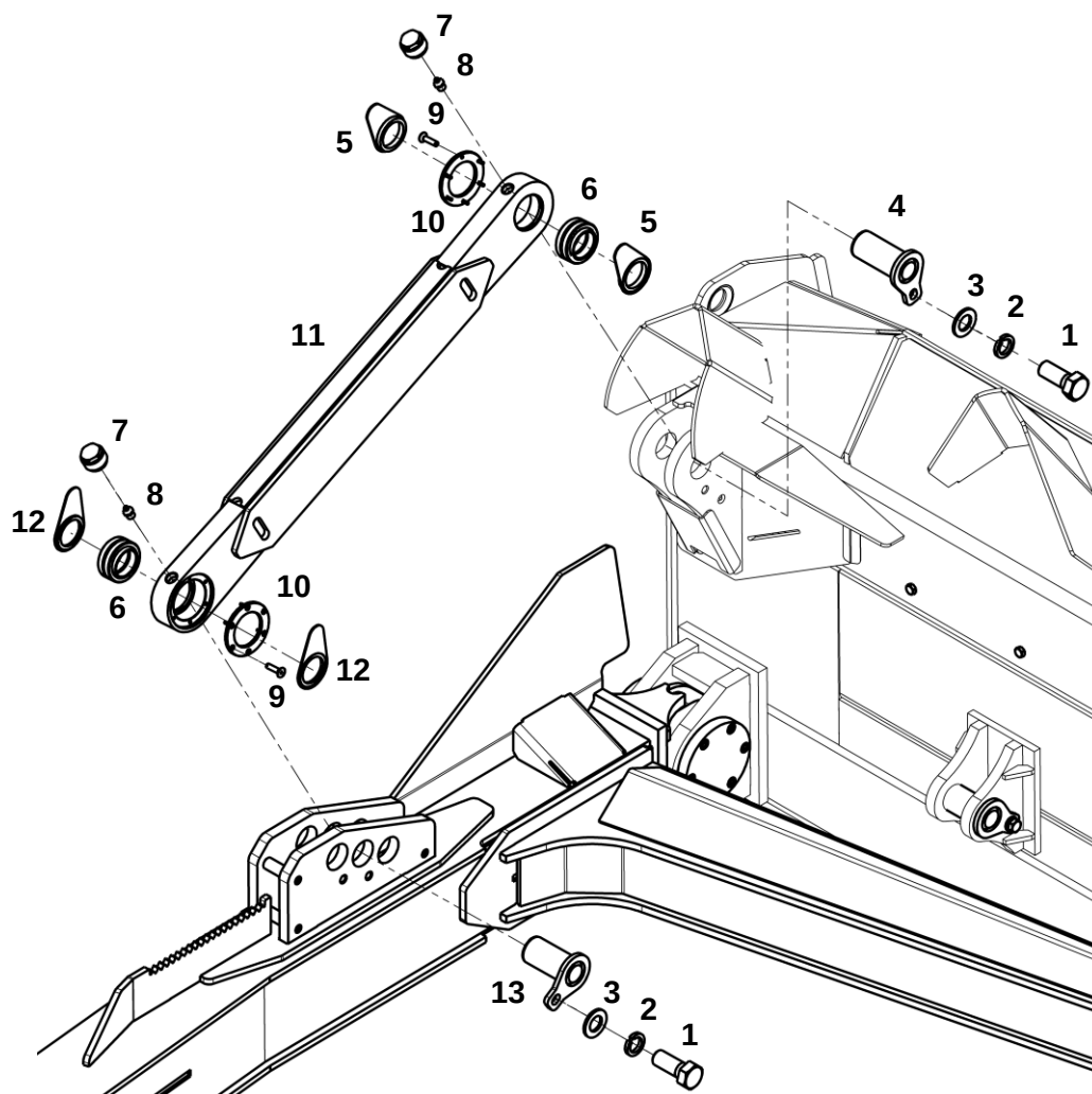
Установка тяги
