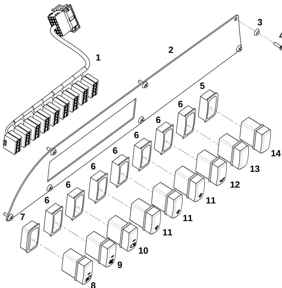
Пульт управления правый верхний
