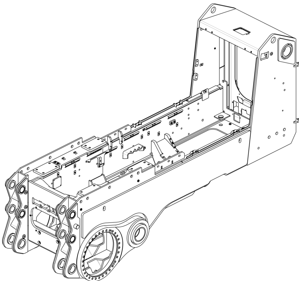
Рама
