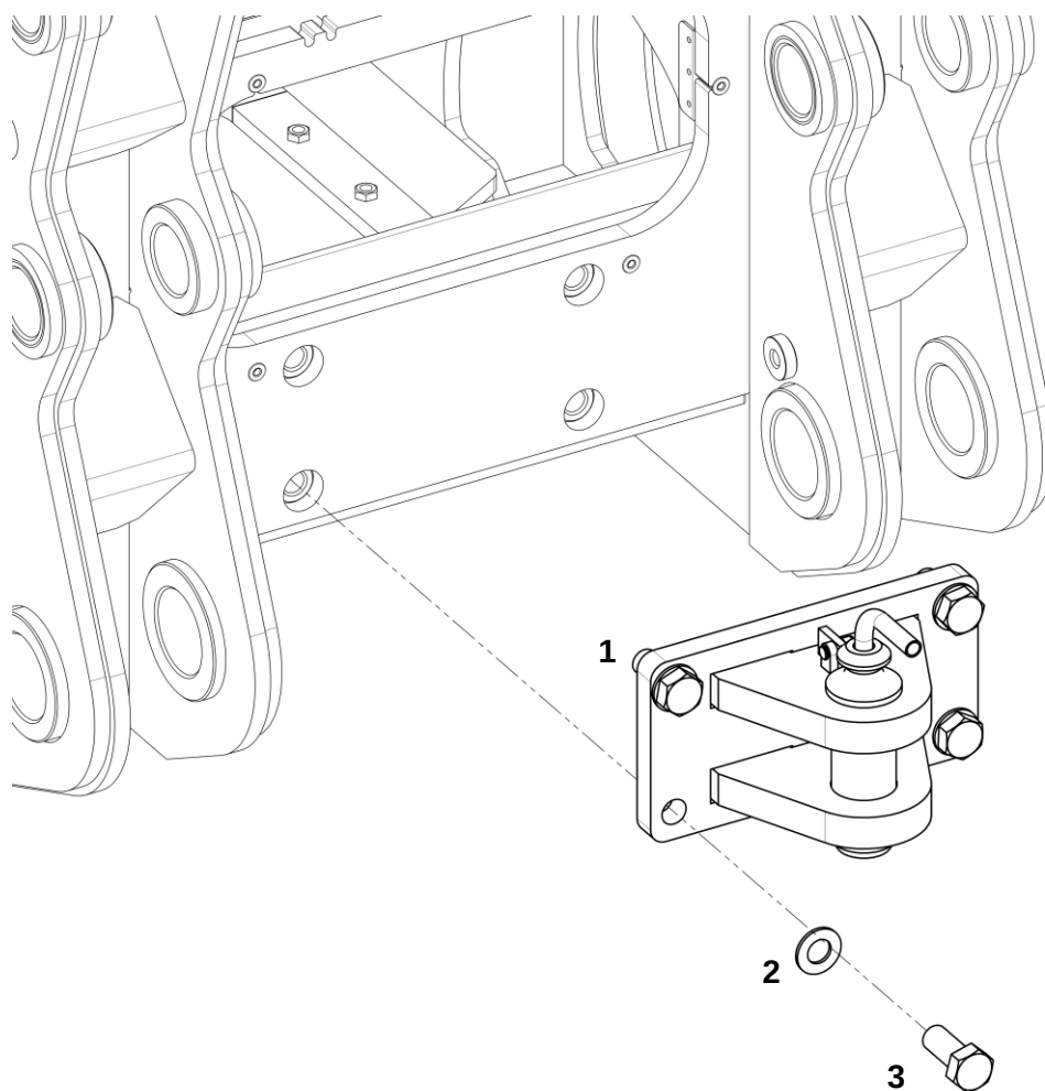
Установка ЖПУ
