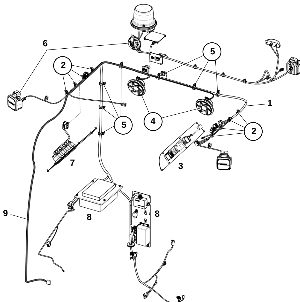
Электрооборудование кабины
