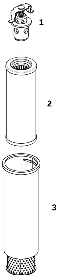
Фильтр в сборе
