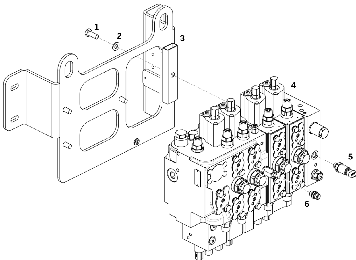
Гидрораспределитель в сборе
