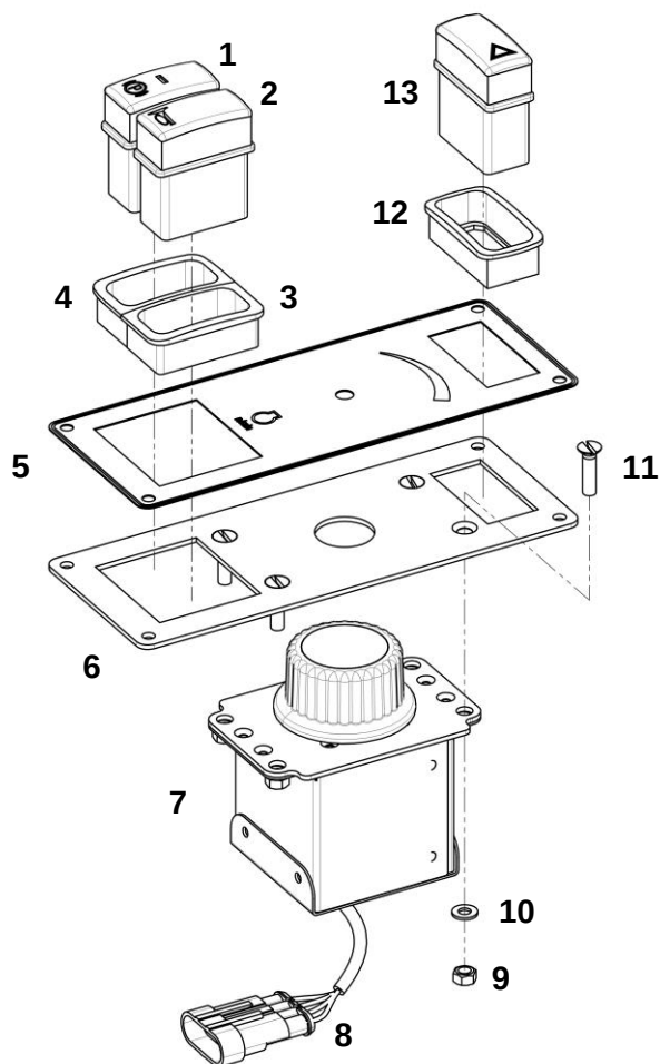
Панель управления
