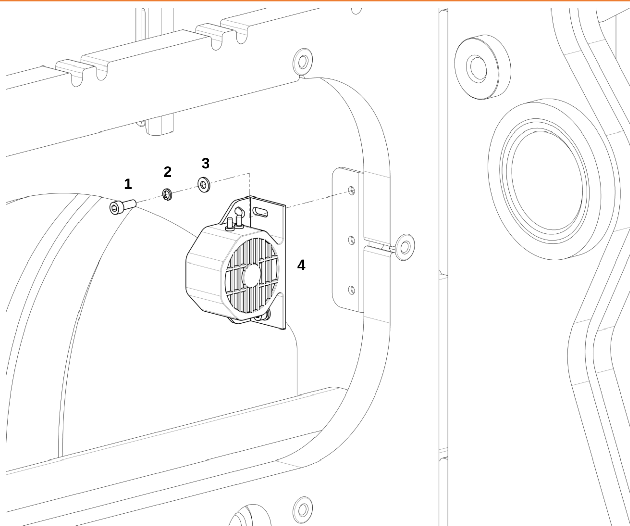
Сигналы звуковые с элементами крепежа
