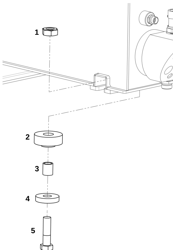
Крепление гидравлического бака
