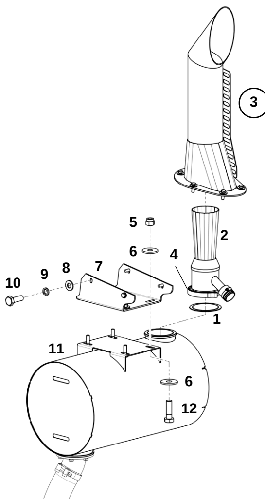
Система впуска воздуха и выпуска ОГ (выпуск)
