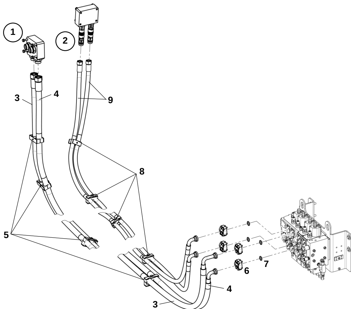
Трубопроводы гидросистемы навесного оборудования
