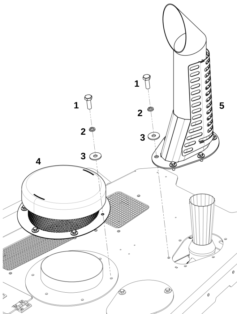
Установка воздухозаборника и выхлопной трубы
