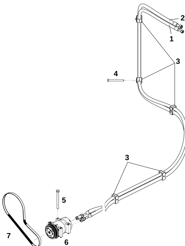
Установка компрессора кондиционера
