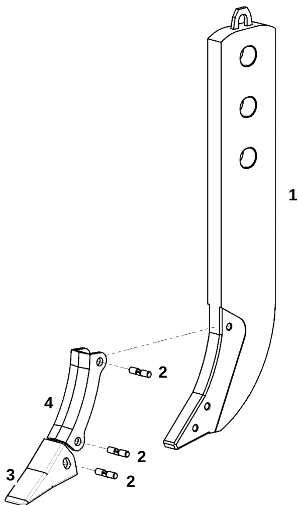
Нож в сборе
