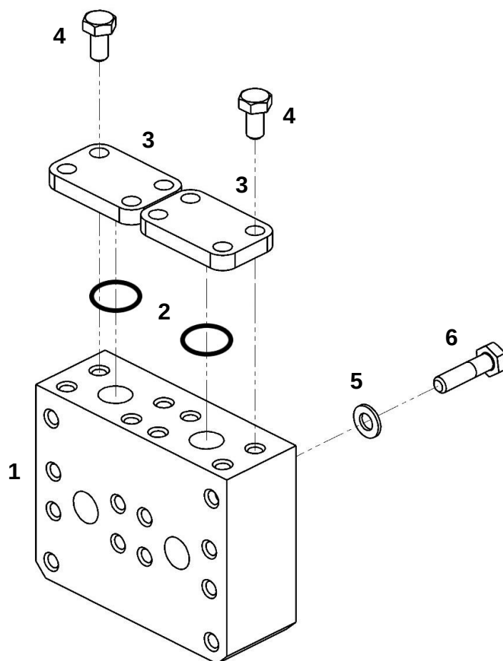
Плита переходная
