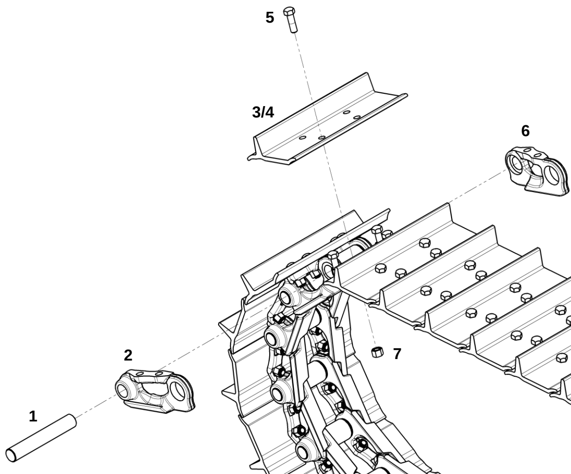
Комплект установки гусениц
