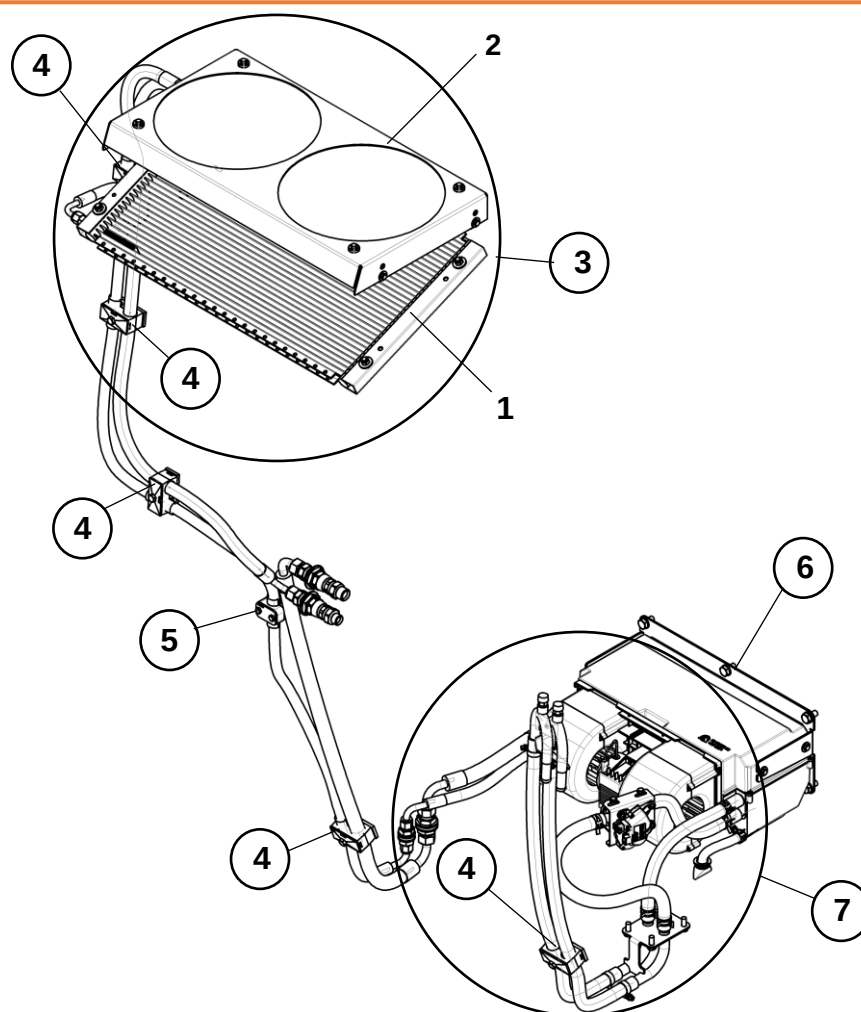
Система кондиционирования
