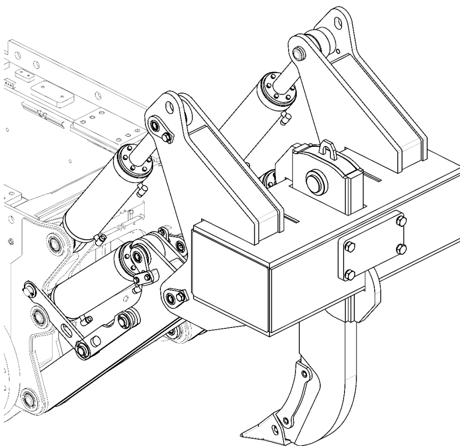
Рыхлитель однозубый 2-х координатный
