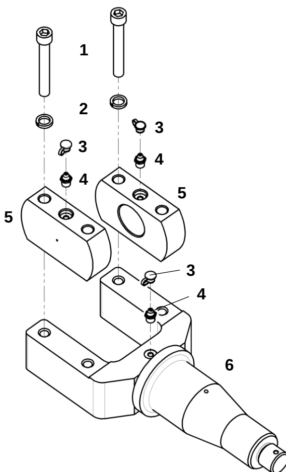
Вилка в сборе
