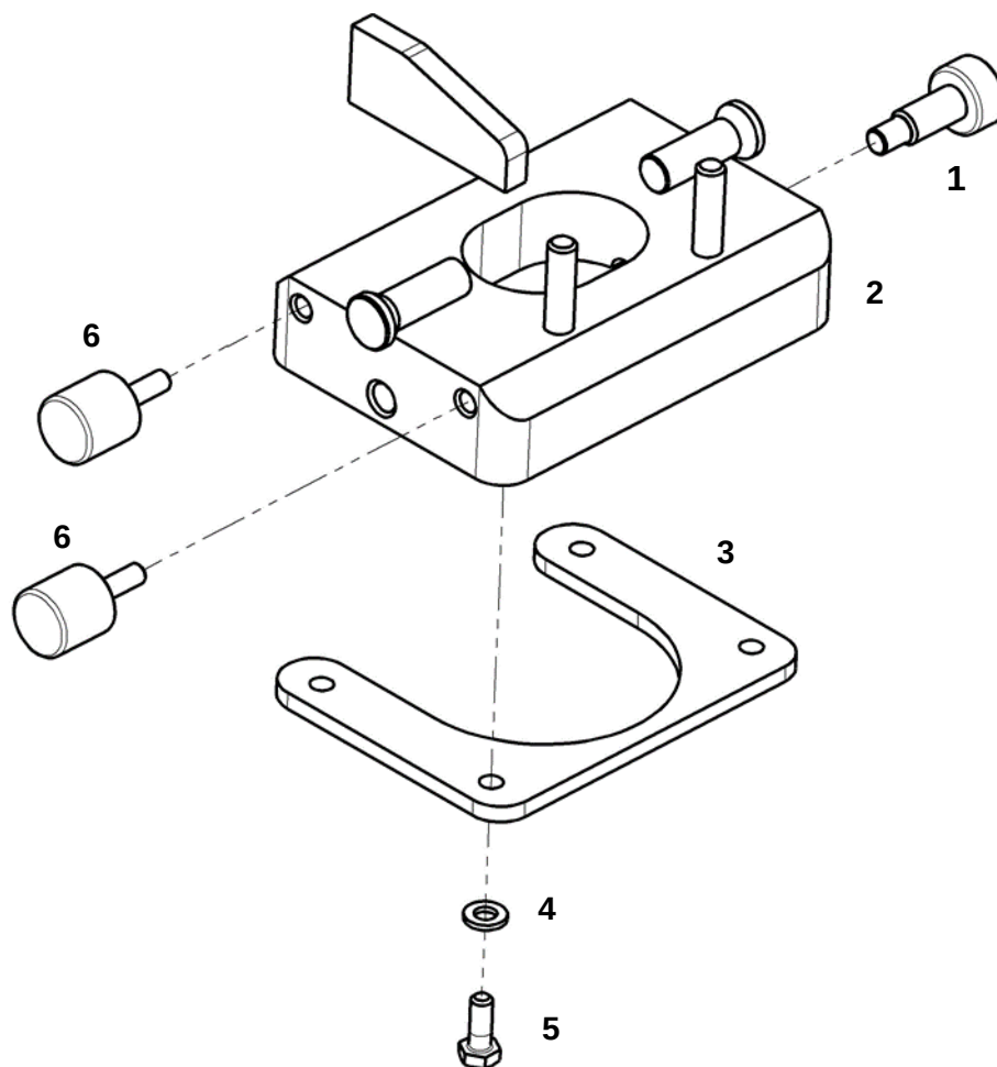
Опора в сборе
