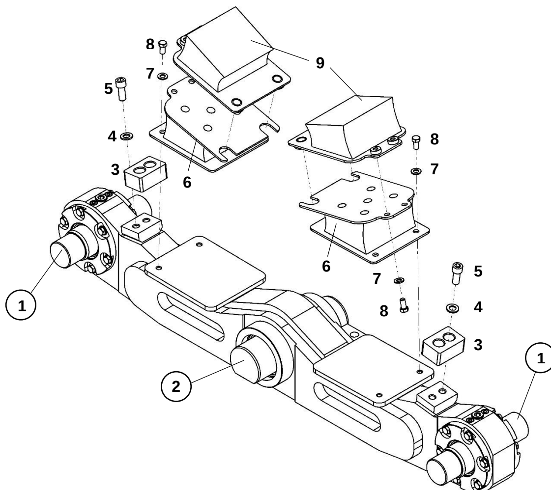
Балка балансирующая
