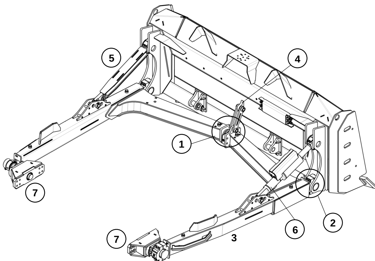
Толкающая рама
