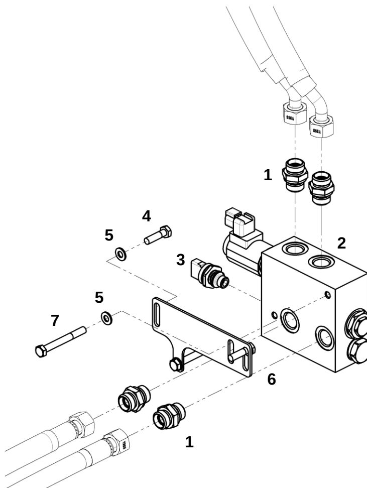
Клапанная коробка в сборе
