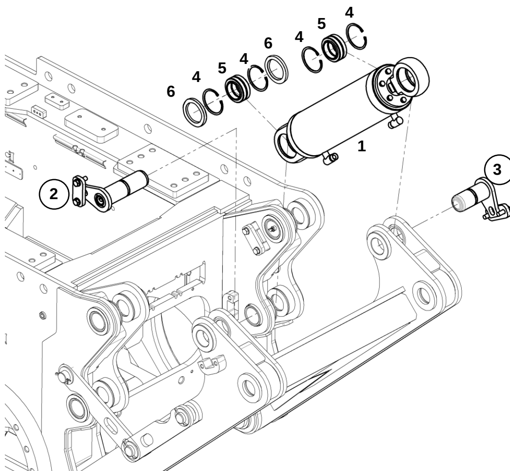
Крепление гидроцилиндра
