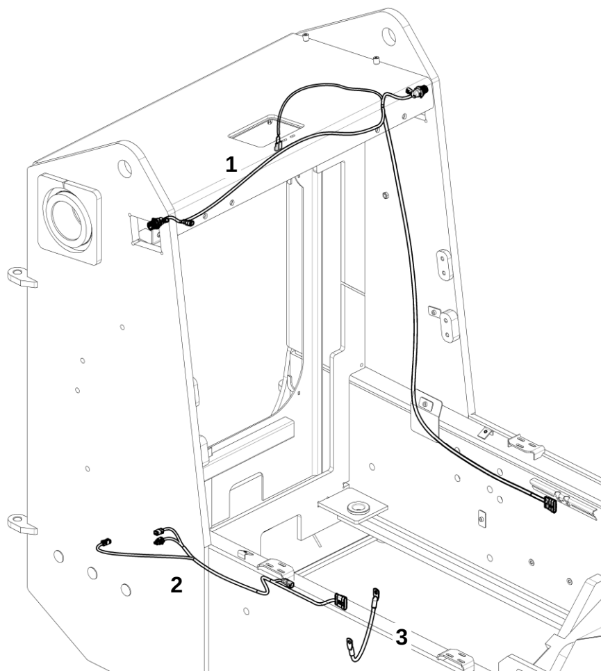
Жгут топливного бака
