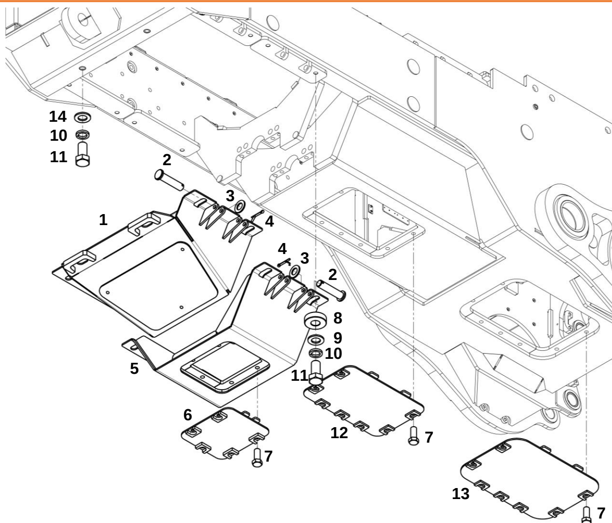
Установка защиты днища
