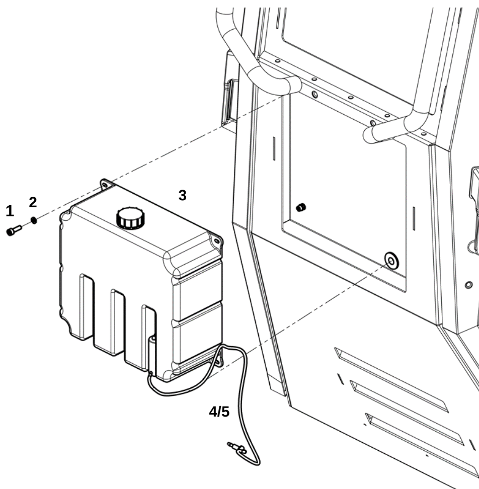
Бачок омывателя
