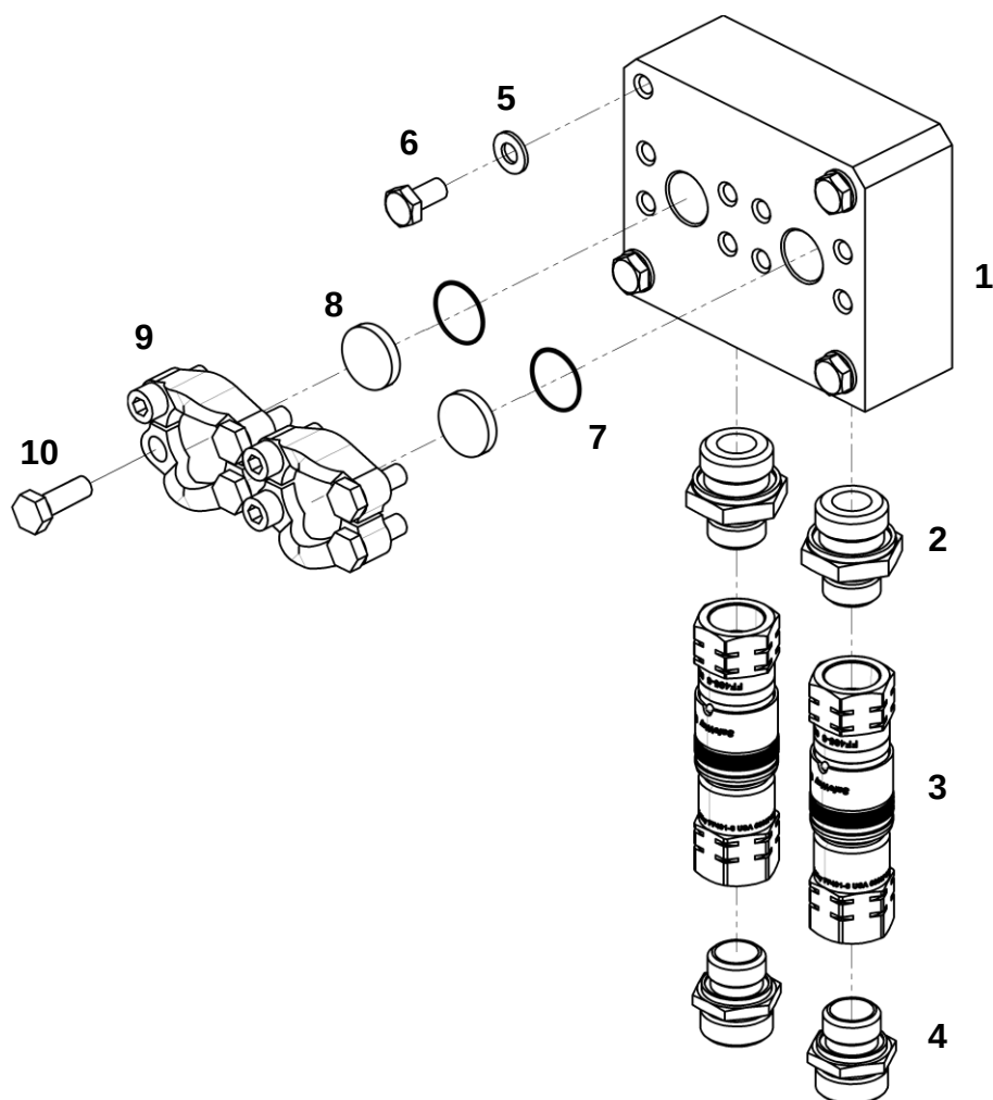
Плита в сборе
