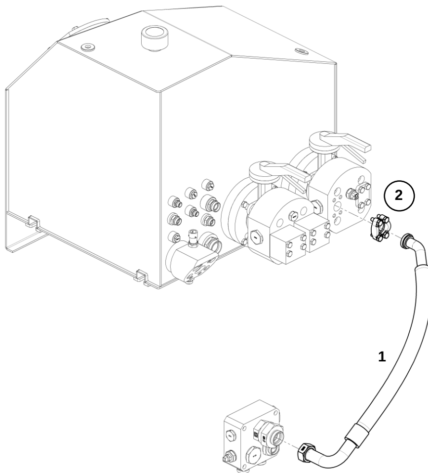
РВД слив с коллектора в бак
