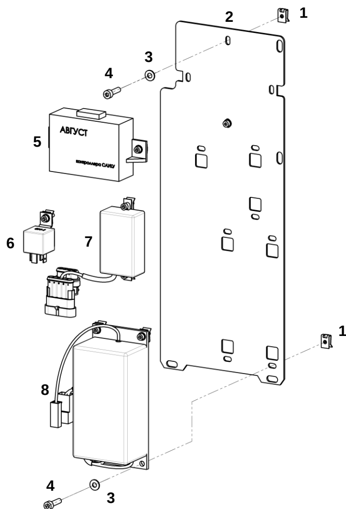
Панель в сборе
