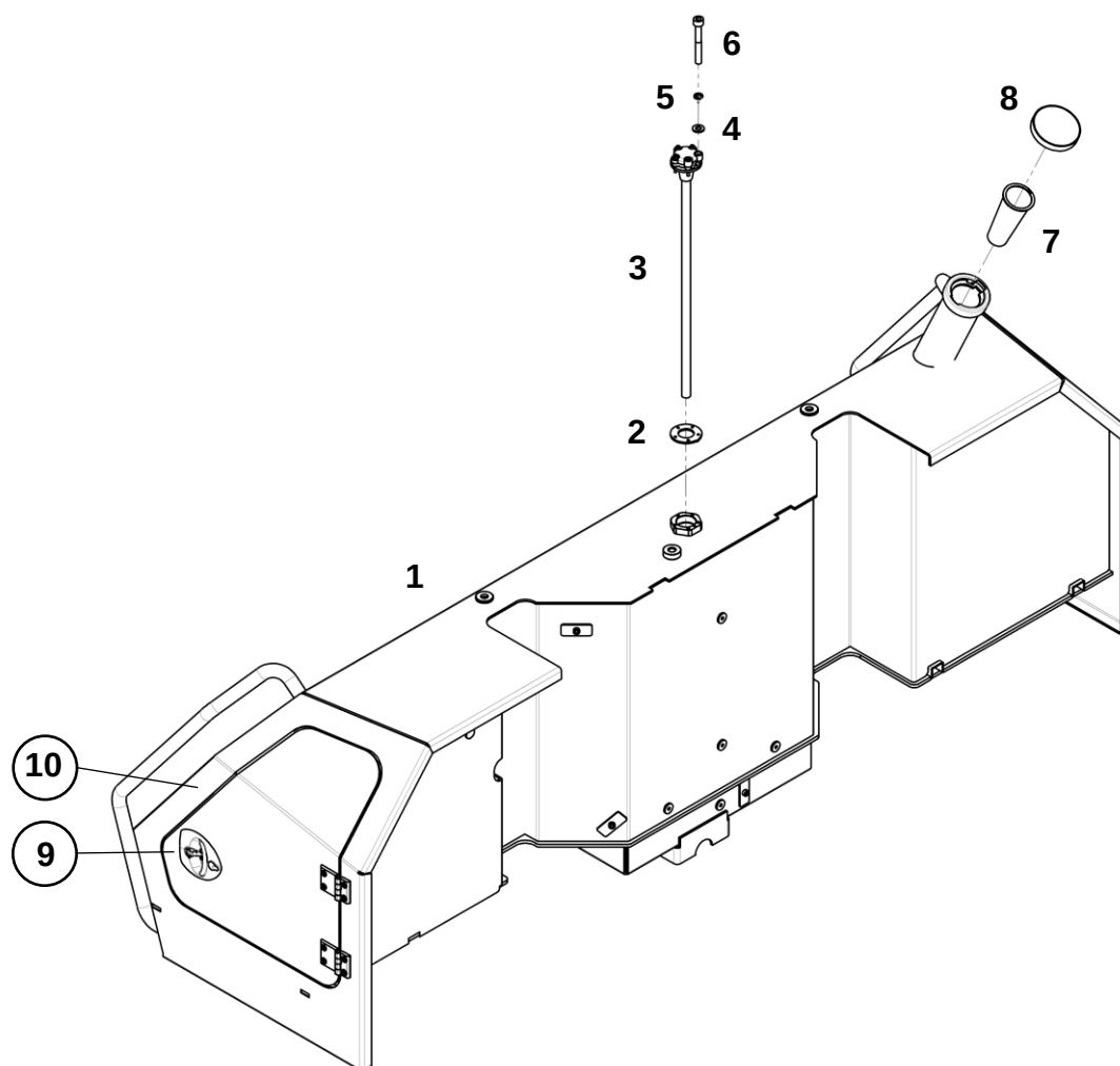
Топливный бак
