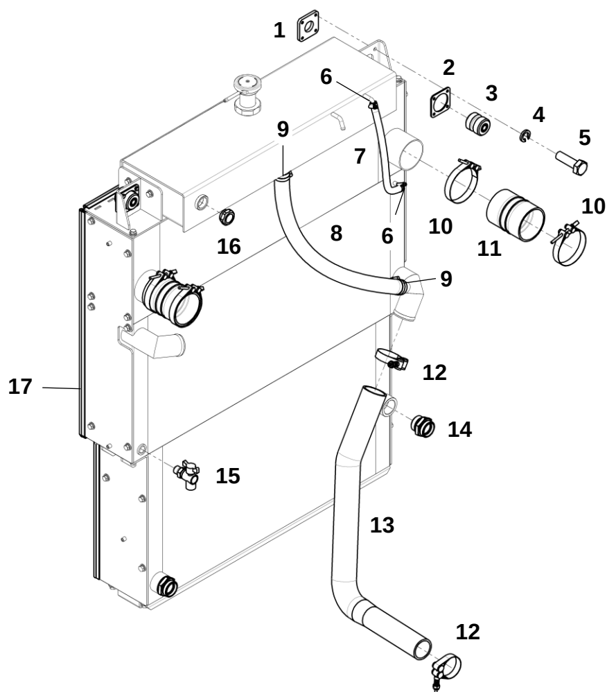
Блок радиатора в сборе
