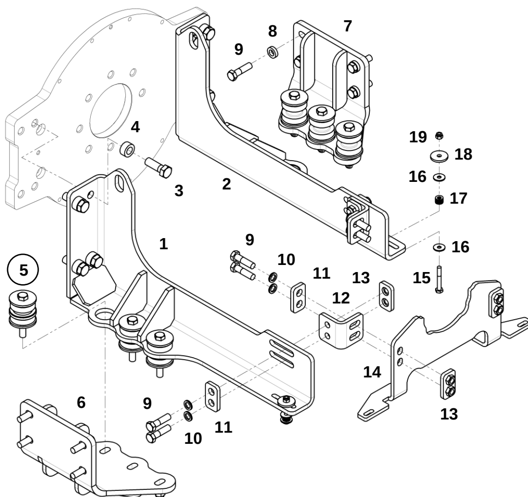
Подвес насосов гидравлических
