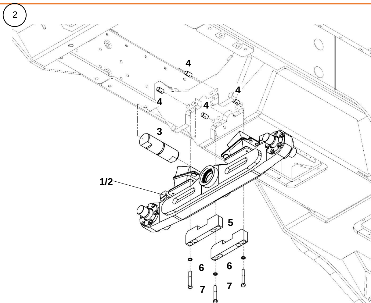
Балка балансирная крепление к раме
