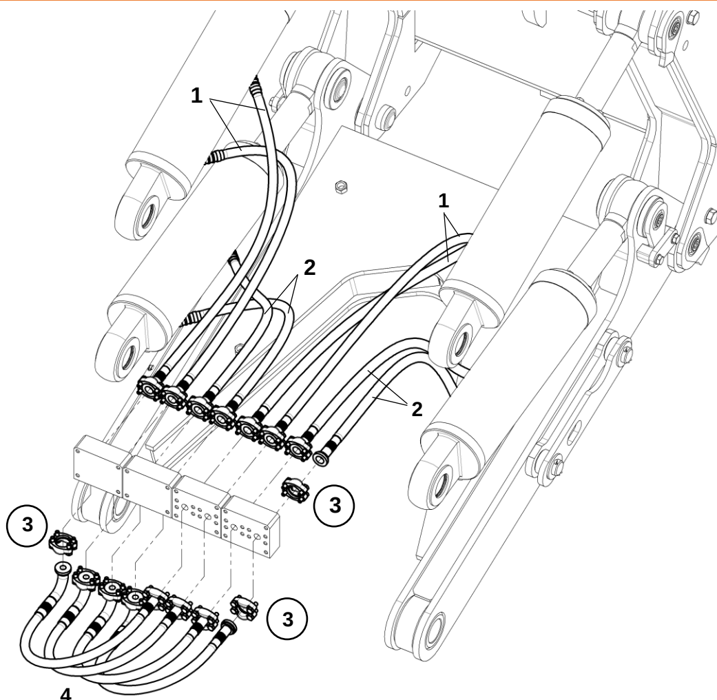
Гидроразводка рыхлительного оборудования
