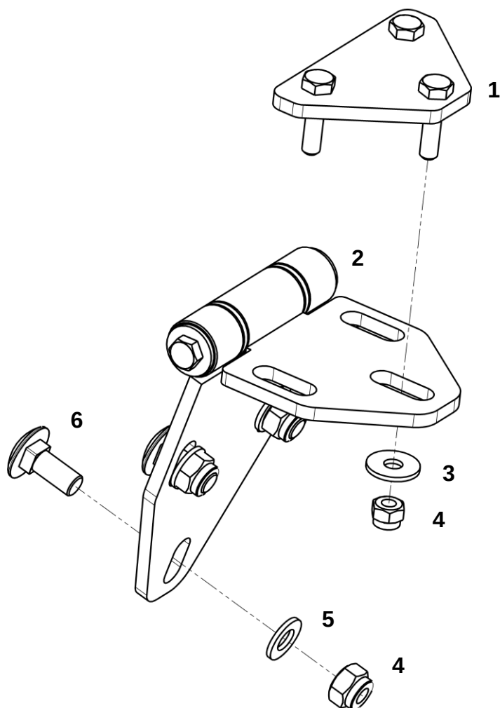
Крепление петли
