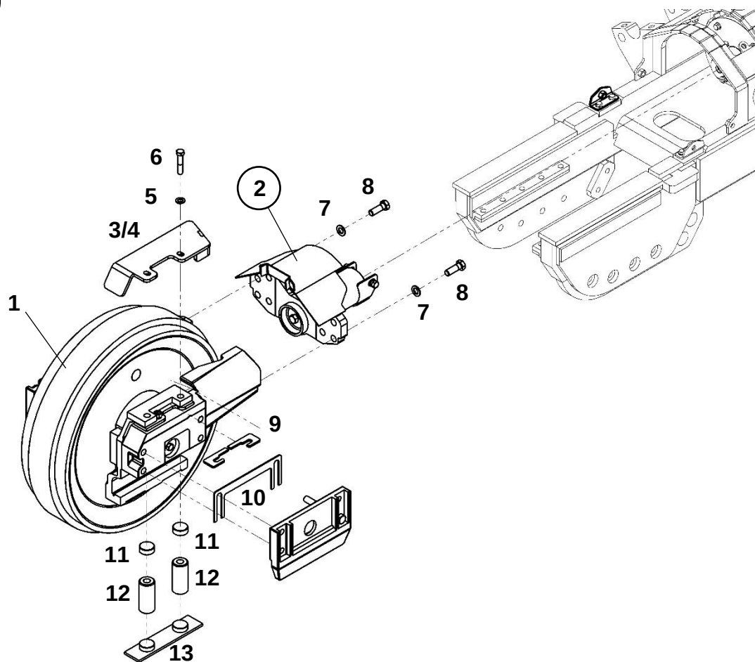
Колесо направляющее в сборе
