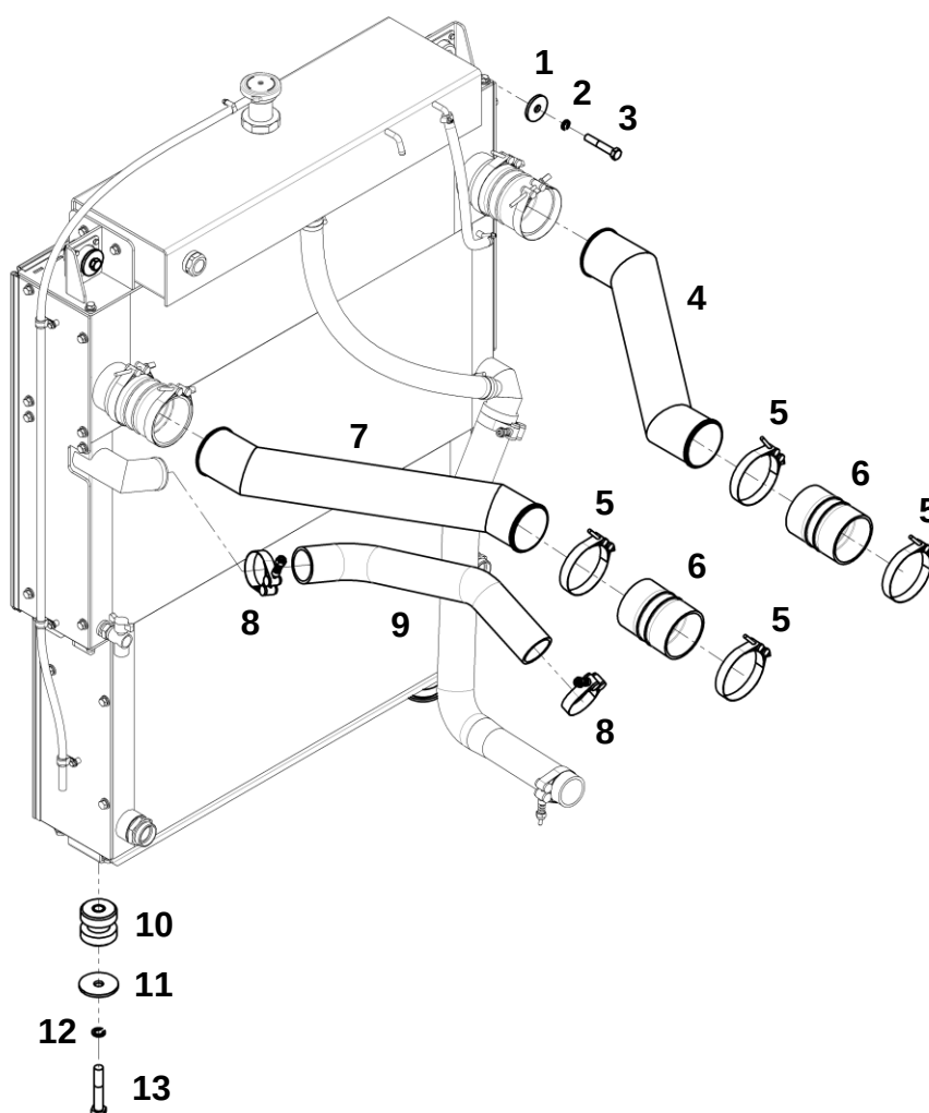
Блок радиатора в сборе
