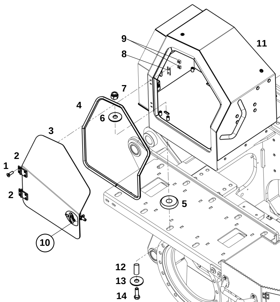
Установка ящика
