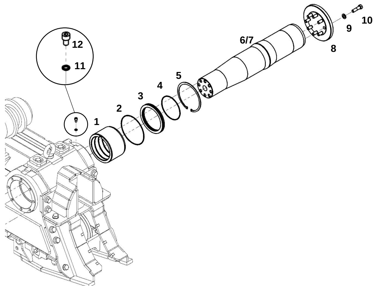
Полуось в сборе
