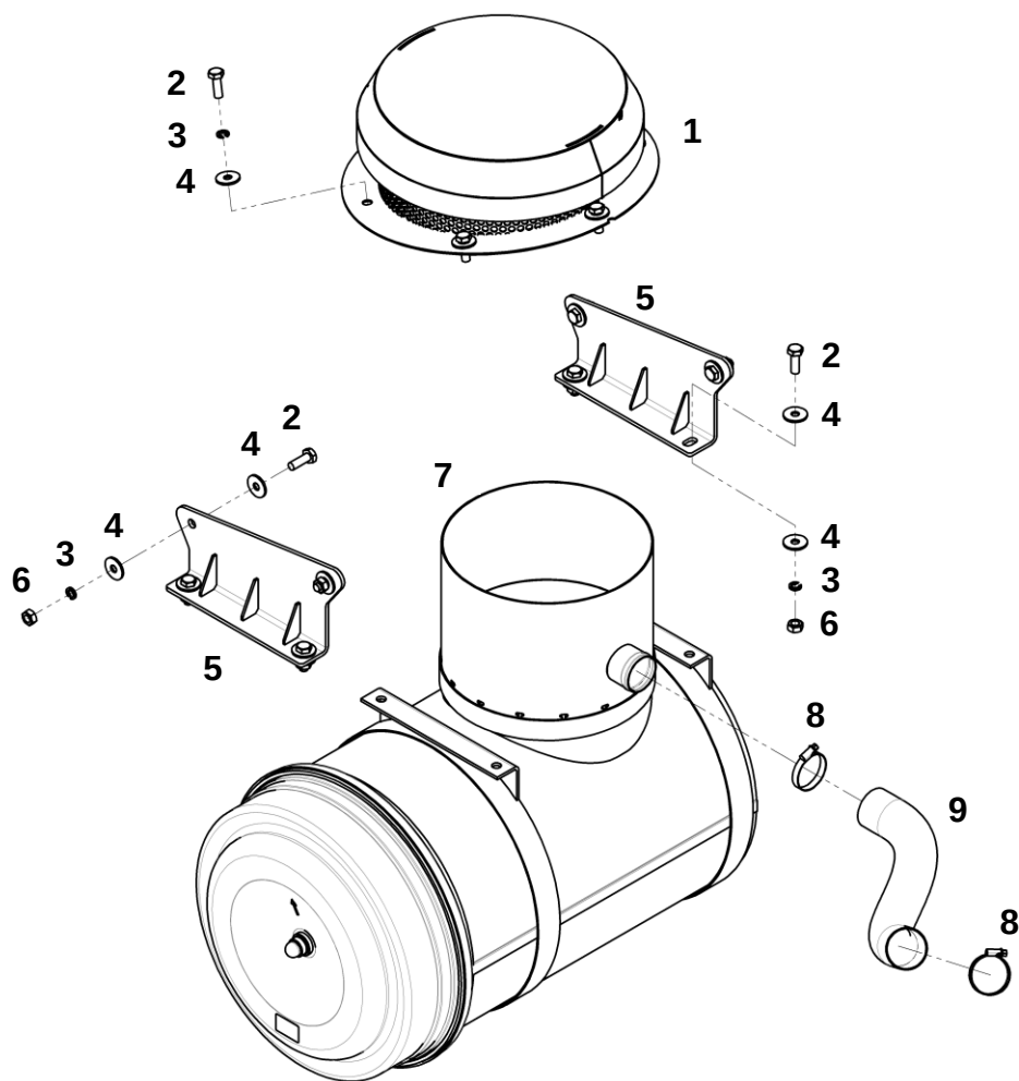
Воздушный фильтр
