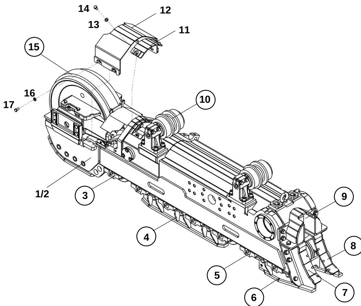
Тележка ходовая в сборе
