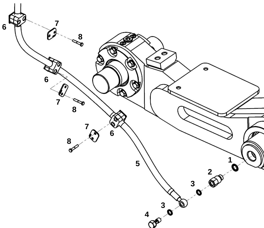
Смазка центральной оси балансирующей балки
