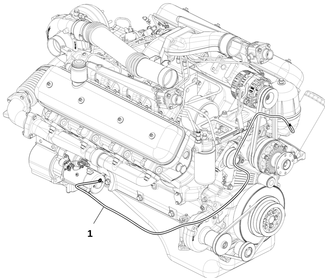
Перемычка стартер-генератор
