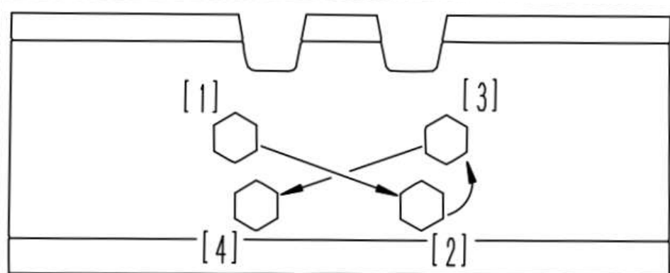
Рисунок 5.65. Схема затяжки крепежных болтов башмака гусеницы
