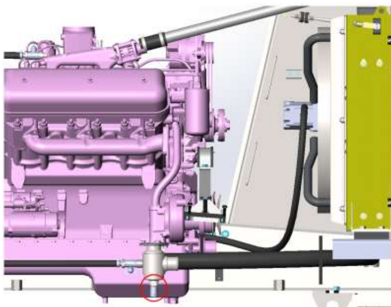
Рисунок 5.26. Кран для слива охлаждающей жидкости
