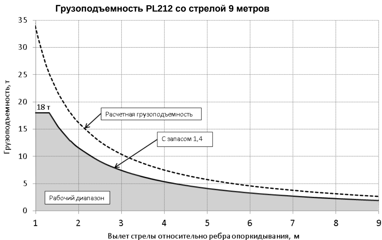
Рисунок 1.2. Грузовая характеристика крана-трубоукладчика PL212 со стрелой 9 метров
