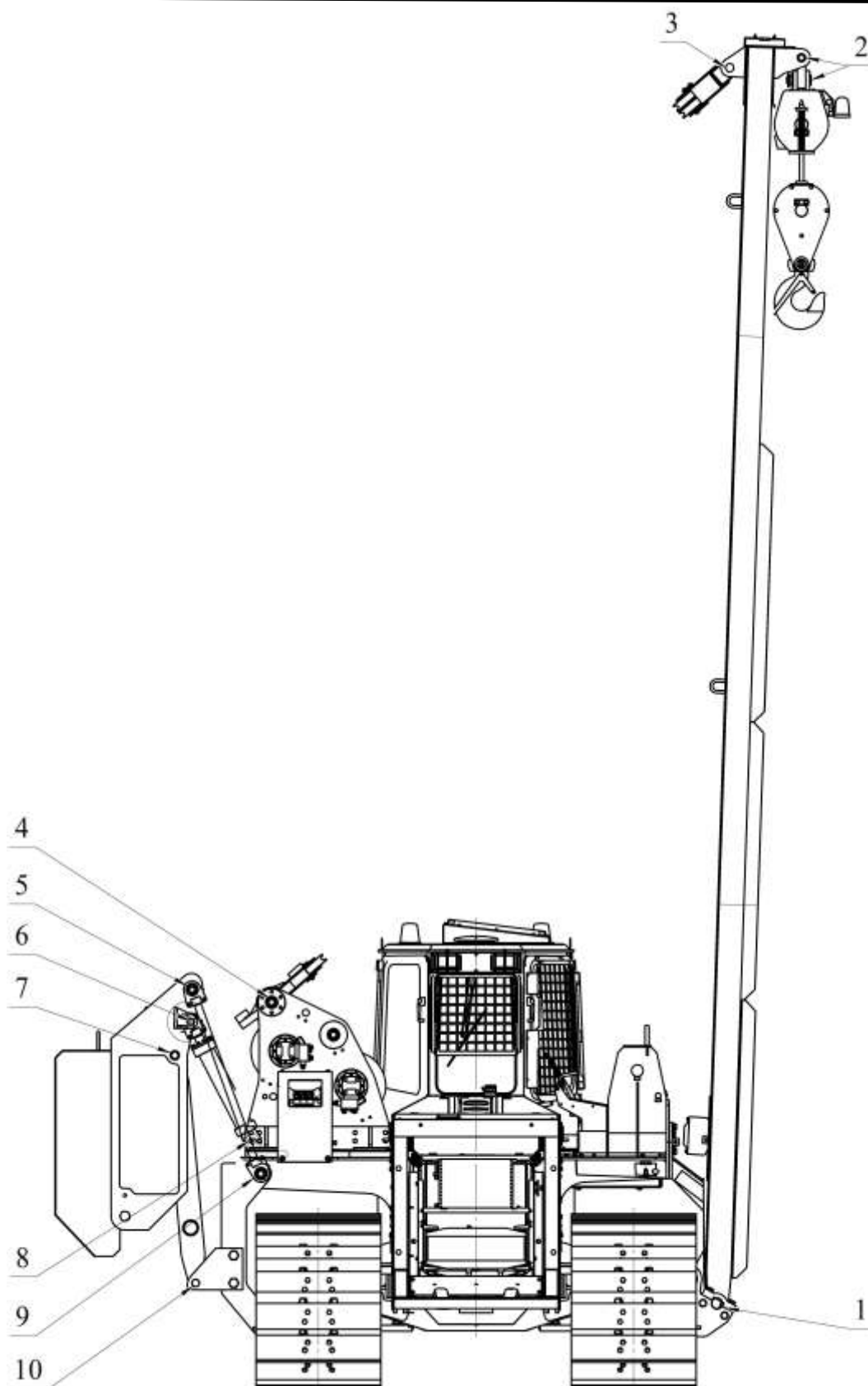
Рис. 3.36. Схема смазки грузоподъемного оборудования и контргруза (для PL212 грузоподъемностью 12 т смазка контргруза не требуется)
