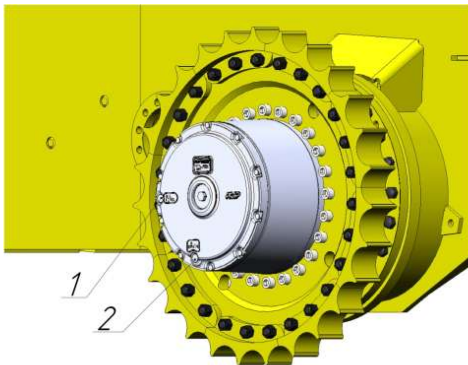
Рисунок 5.50. Редуктор механизма передвижения
