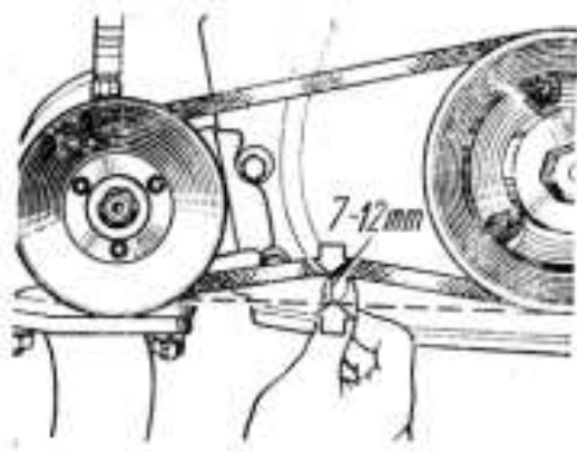
Рисунок 5.16. Проверка натяжения ремня привода водяного насоса
