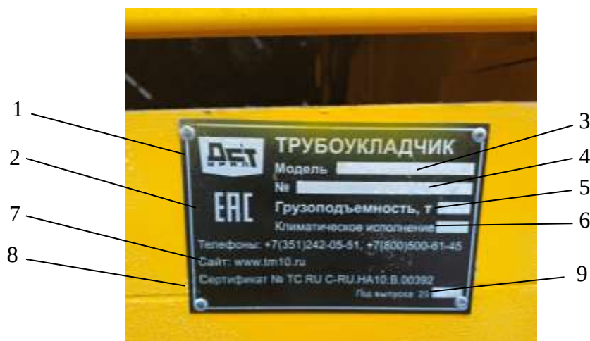
Рисунок 2.5. Табличка «Идентификационная табличка №1»
