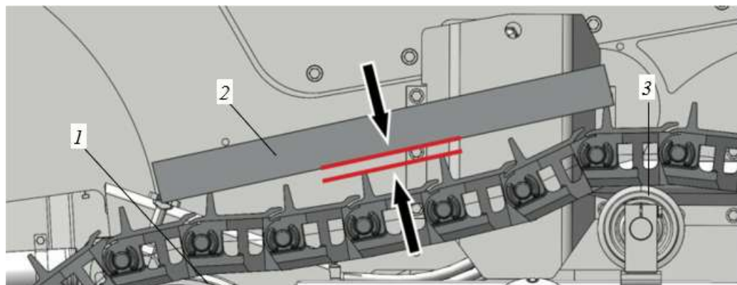
Рисунок 5.56. Проверка натяжения гусениц
