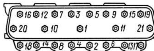
Рисунок 5.10. Последовательность протяжки головки блока цилиндров
