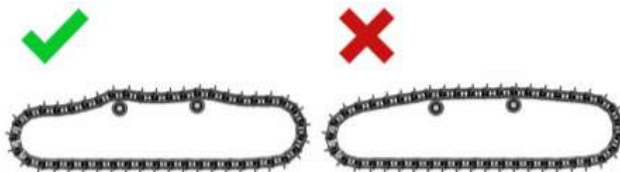
Рисунок 5.55. Натяжение гусеницы
