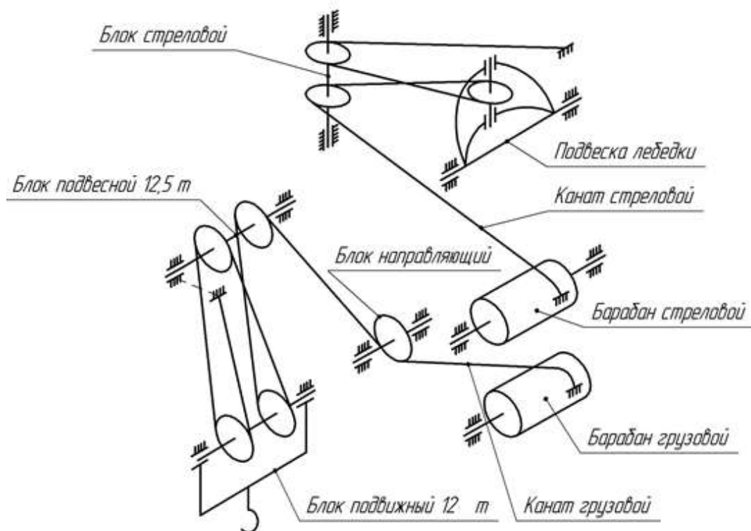
Рисунок 3.38. Схема запасовки канатов
