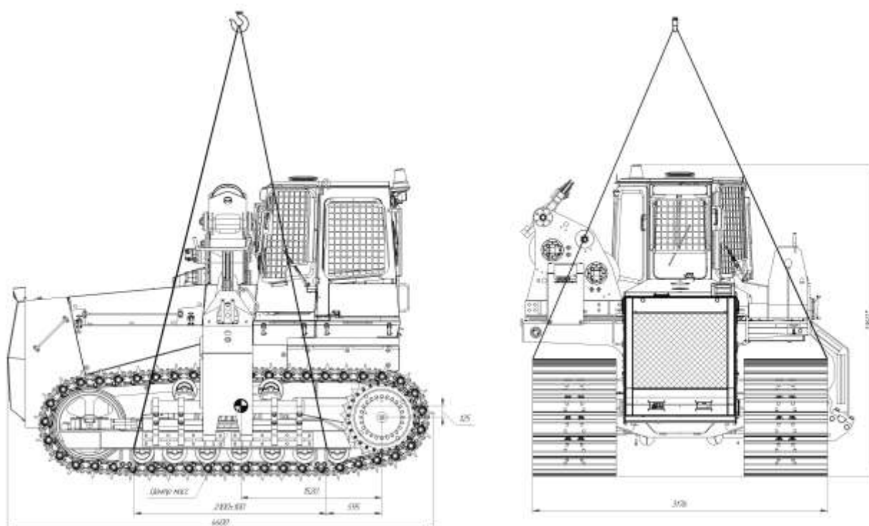
Рисунок 3.54. Места крепления грузоподъемных стропов
