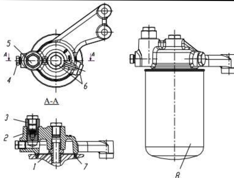
Рисунок 5.15. Фильтр тонкой очистки топлива со сменным фильтром
