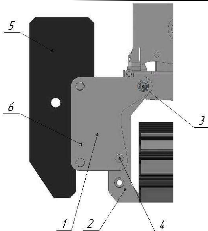
Рис. 3.39. Противовес PL212 для исполнения машины грузоподъемностью 12 т 1 – каретка контргрузов для исполнения машины грузоподъемностью 12 т; 2 – рама контргрузов; 3 – ось крепления рамы и каретки; 4 – болт; 5 – контргруз; 6 – штанга
