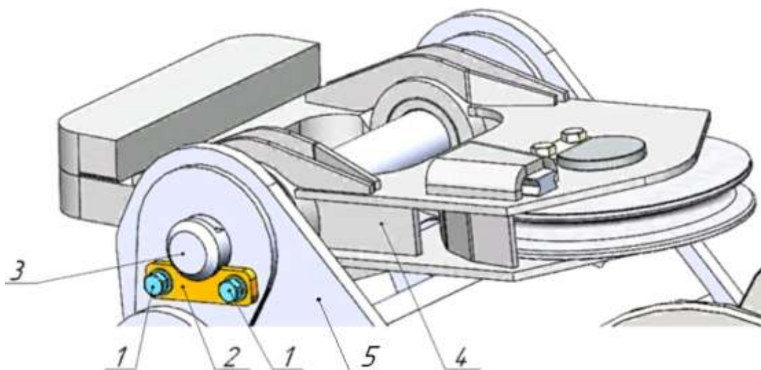
Рис. 3.37.1. Подвеска стреловая
