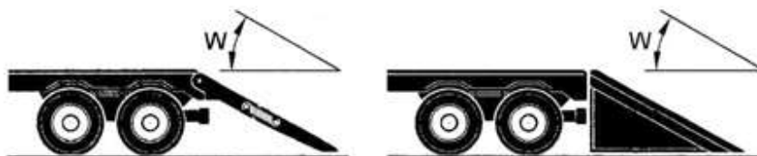
Рисунок 3.52. Наклон ramпы
