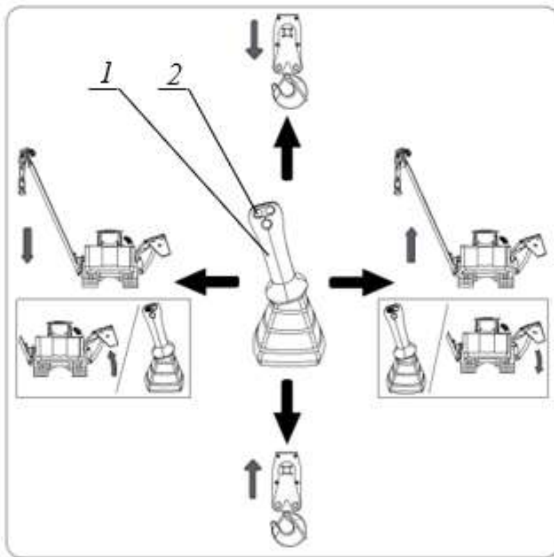
Рисунок 3.50. Схема управления грузоподъемным оборудованием
