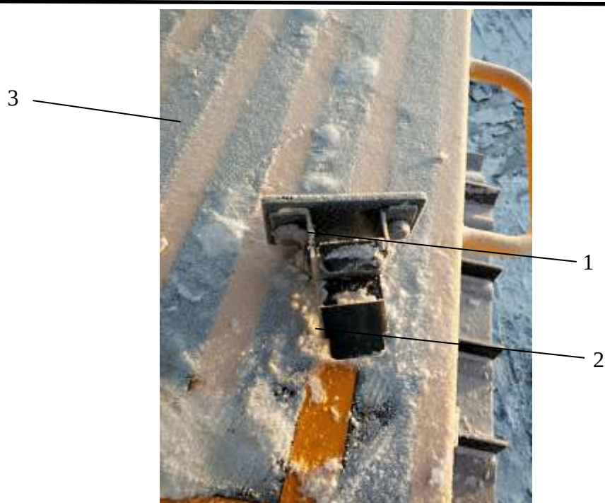
Рисунок 3.14. Блокиратор двери
