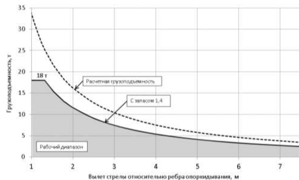
Рисунок 1.1. Грузовая характеристика крана-трубоукладчика PL212 со стрелой 7 метров
