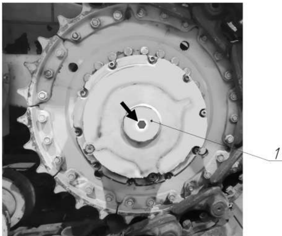
Рисунок 3.57. Крышка снятия вала для растормаживания редуктора
