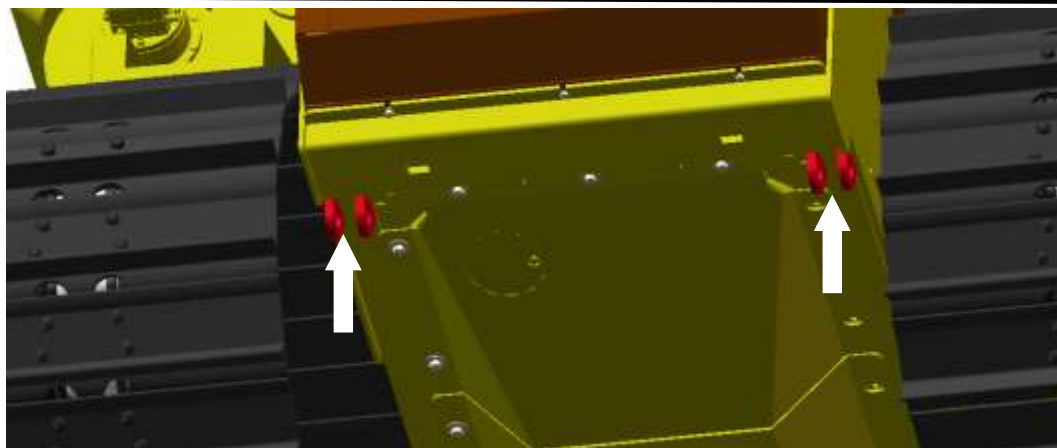
Рисунок 3.55. Буксировочные проушины
