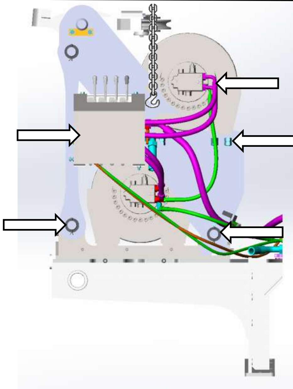
Рисунок 5.79. Демонтаж грузовой лебедки
