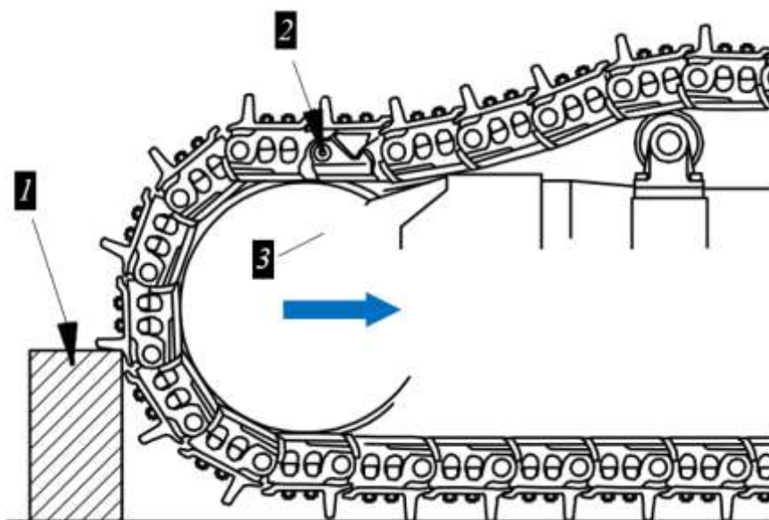
Рисунок 5.61. Процедура снятия натяжения с гусеничной цепи
