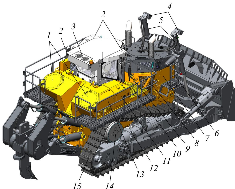
Рисунок 1.2. Общий вид бульдозера сзади
