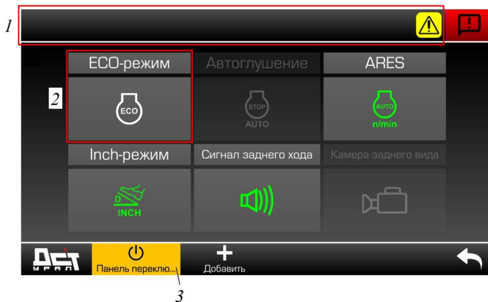
Рисунок 3.72. Панель переключателей
