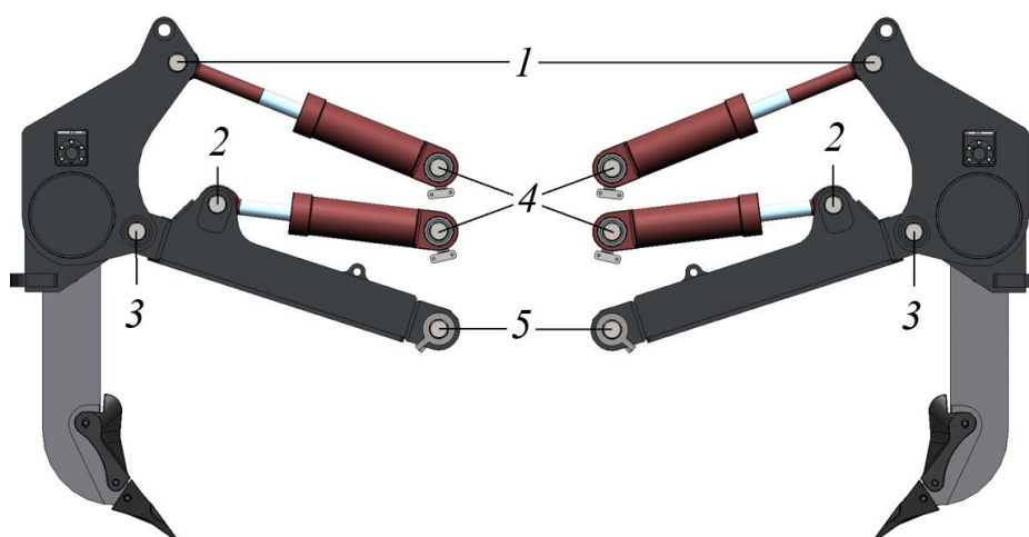
Рисунок 5.167. Схема смазка рыхлительного оборудования
