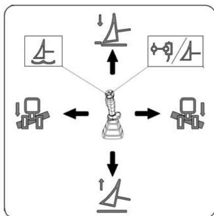
Рисунок 3.91. Схема управления бульдозерным оборудованием
