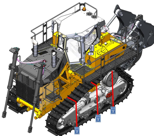
Рисунок 3.152. Крепление машины на грузовой платформе сбоку
