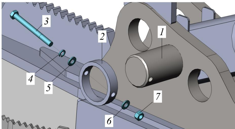
Рисунок 3.103. Демонтаж пальца гидроцилиндра перекоса отвала
