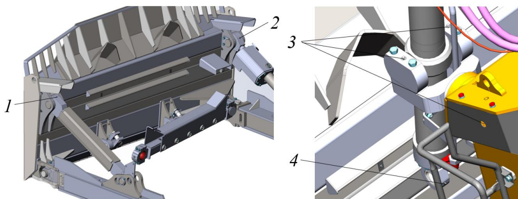
Рисунок 5.166. Схема смазки бульдозерного оборудования
