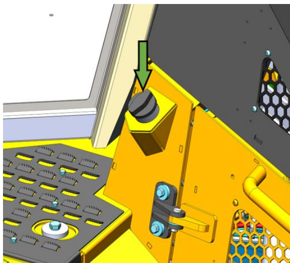
Рисунок 5.108. Место расположения маслоналивной горловины раздаточной коробки
