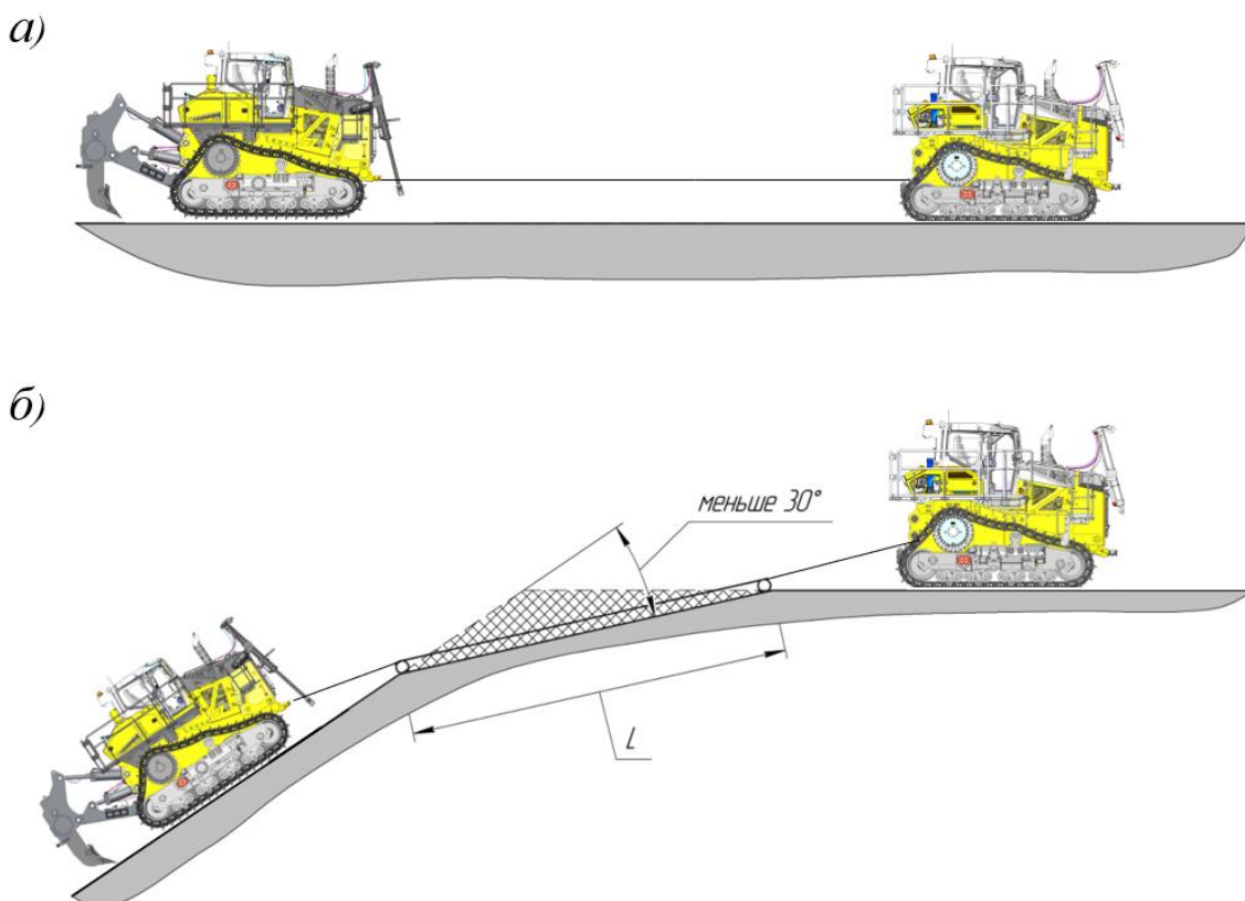
Рисунок 3.158. Вытаскивание трактора
