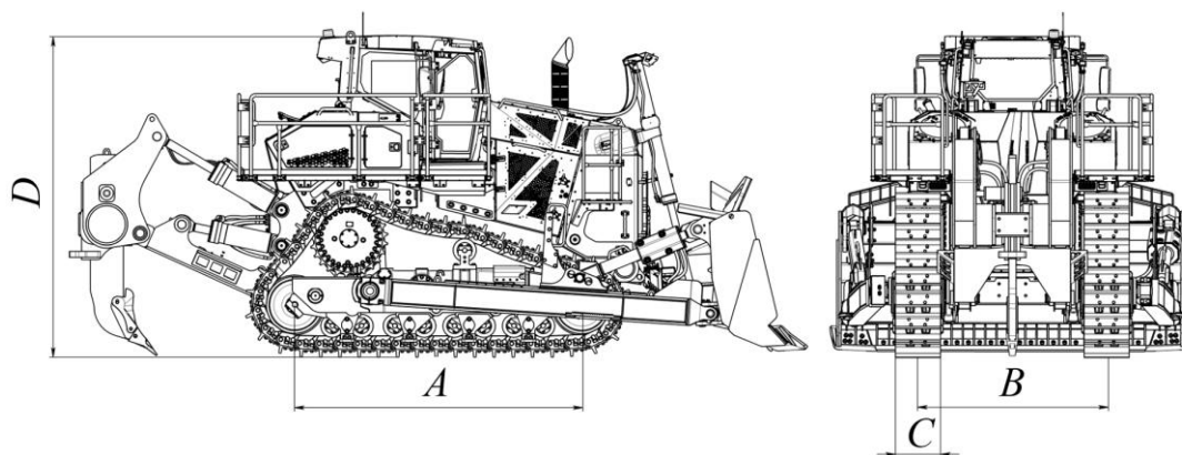
Рисунок 1.3. Габаритные размеры машины
