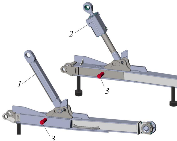
Рисунок 3.122. Фиксация тяги и гидроцилиндра в поднятом положении
