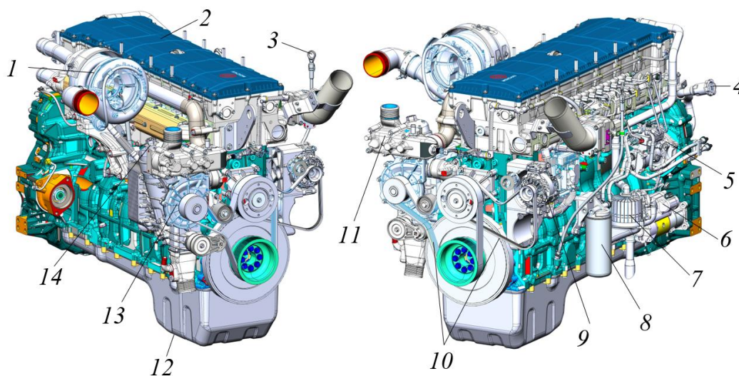
Рисунок 5.40. Точки контроля и обслуживания на двигателе Weichai WP17T
