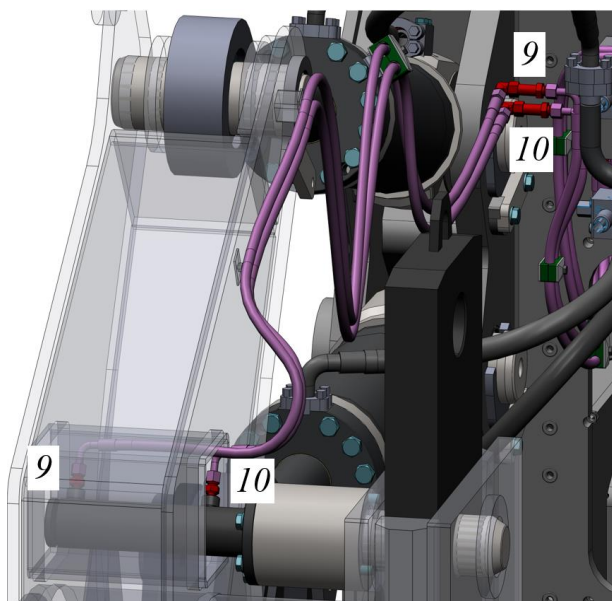
Рисунок 3.146. Подключение РВД к гидроцилиндру регулировки высоты ножа
