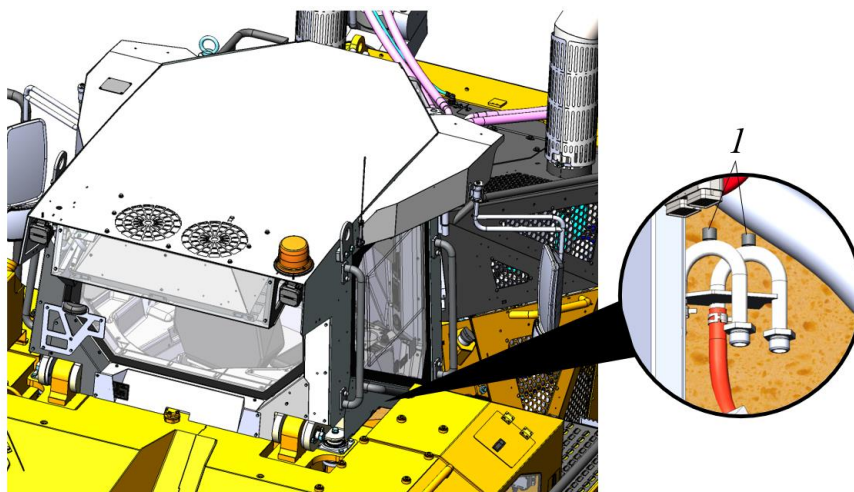
Рисунок 5.79. Процедура удаления воздуха из патрубков системы охлаждения ДВС
