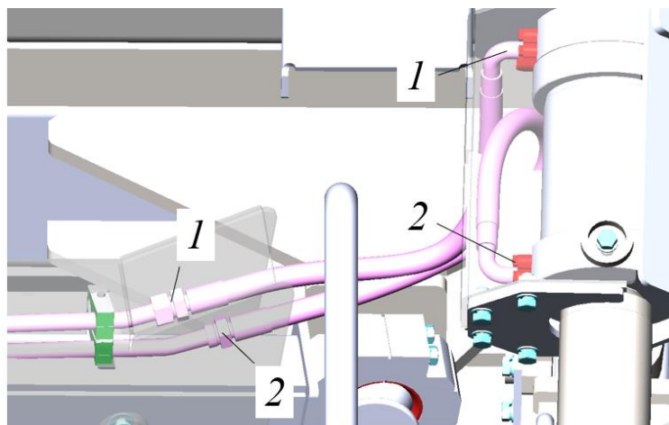
Рисунок 3.134. Монтаж РВД подключение к гидроцилиндру перекоса отвала
