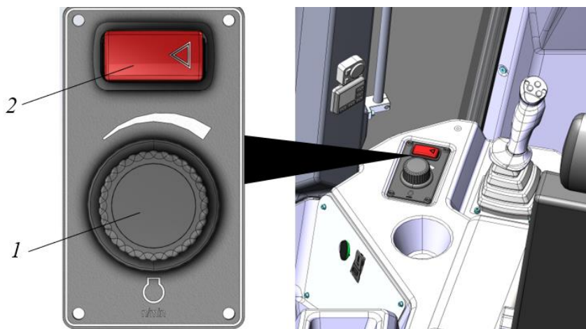
Рисунок 3.15. Панель управления
