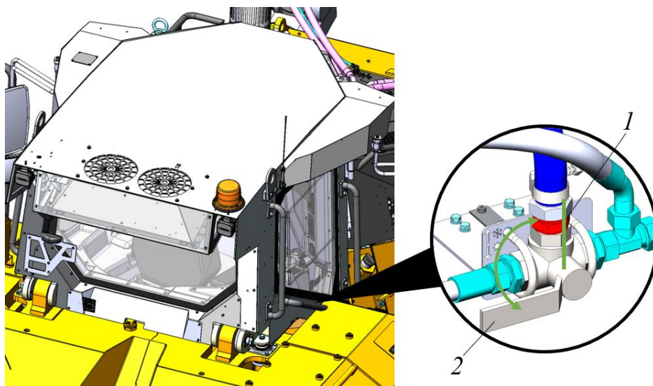
Рисунок 5.86. Кран ПЖД
