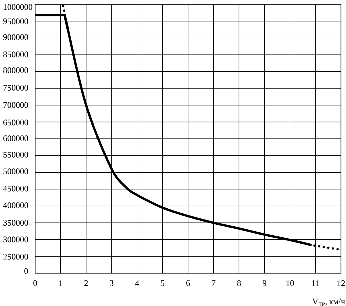
Рисунок 1.4. График тягово-скоростной характеристики ГСТ40
