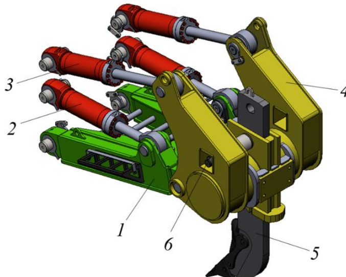
Рисунок 3.137. Рыхлитель однозубый
