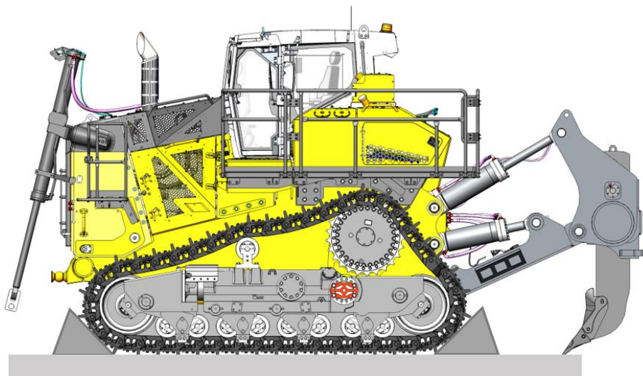
Рисунок 3.154. Установка противооткатных упоров под гусеницы
