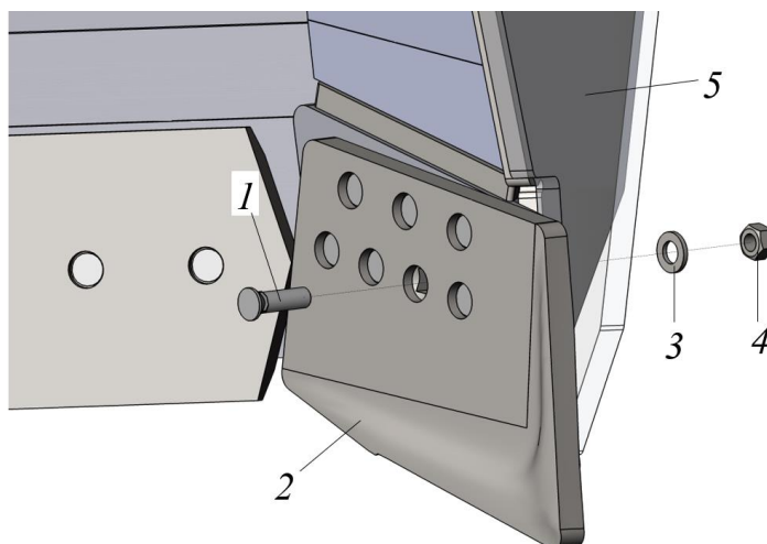
Рисунок 3.135. Нож боковой
