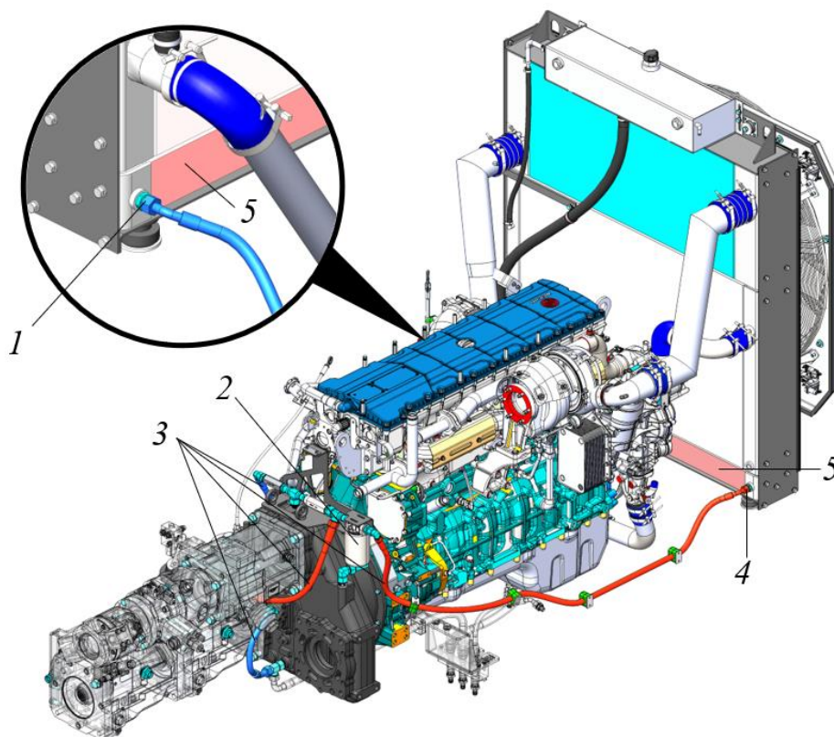
Рисунок 5.105. Система охлаждения раздаточной коробки
