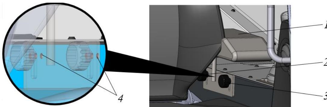
Рисунок 3.32. Регулировка подлокотника
