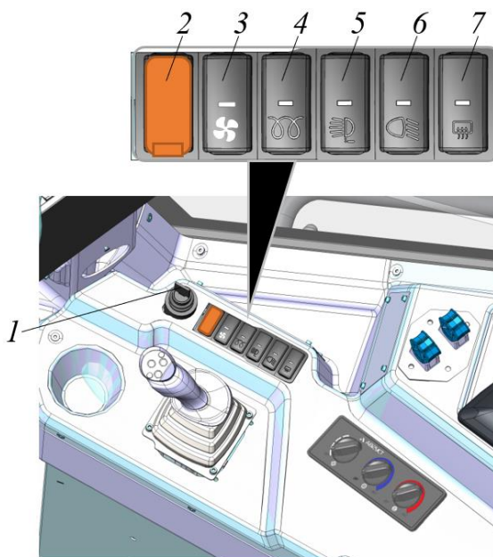
Рисунок 3.17. Органы управления правой тумбы
