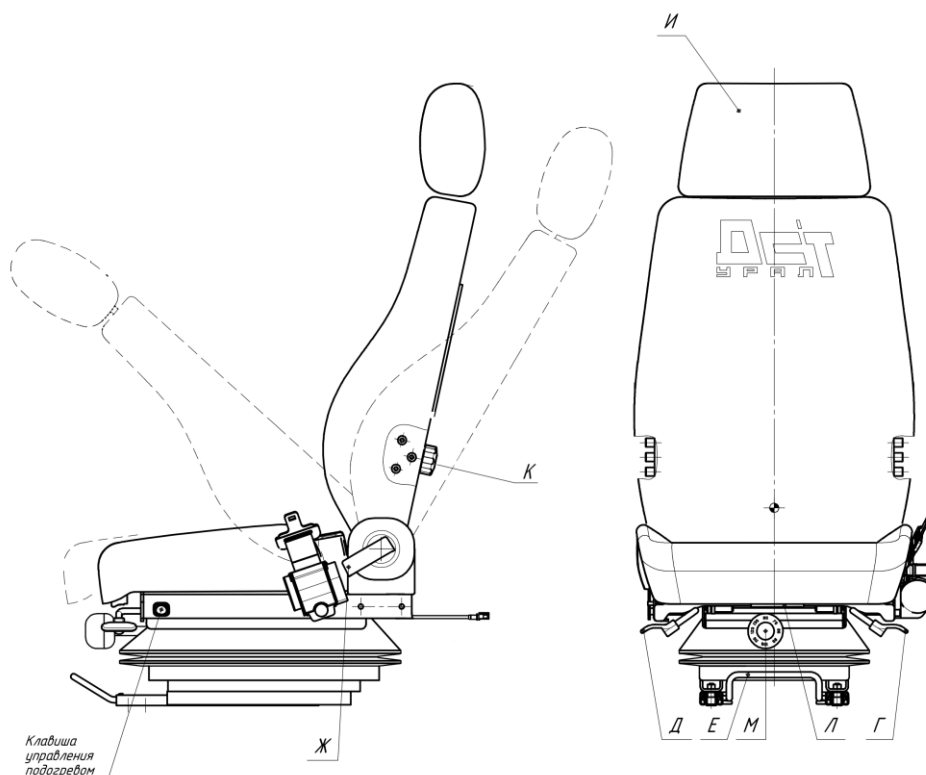
Рисунок 3.30. Сиденье оператора
