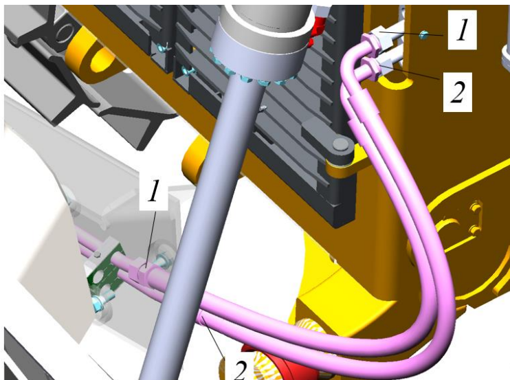
Рисунок 3.133. Монтаж РВД подключение к трактору
