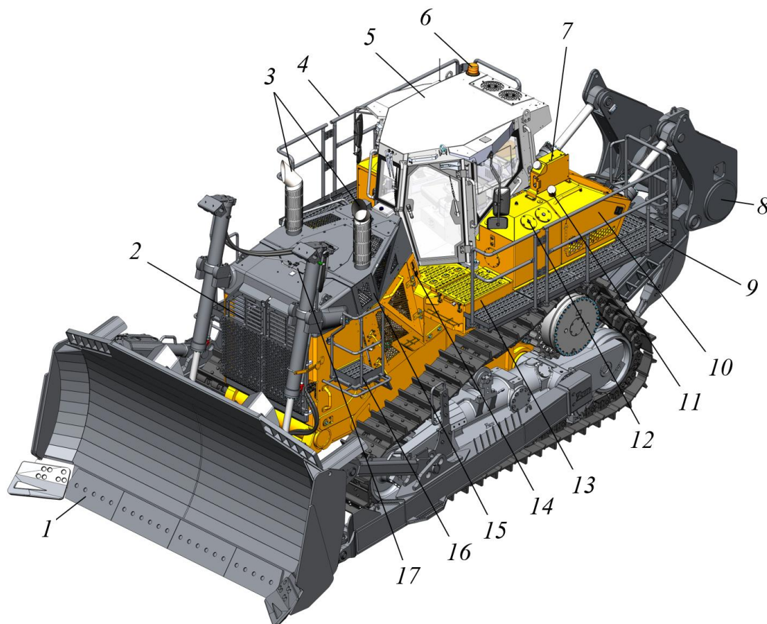
Рисунок 1.1. Общий вид бульдозера спереди
