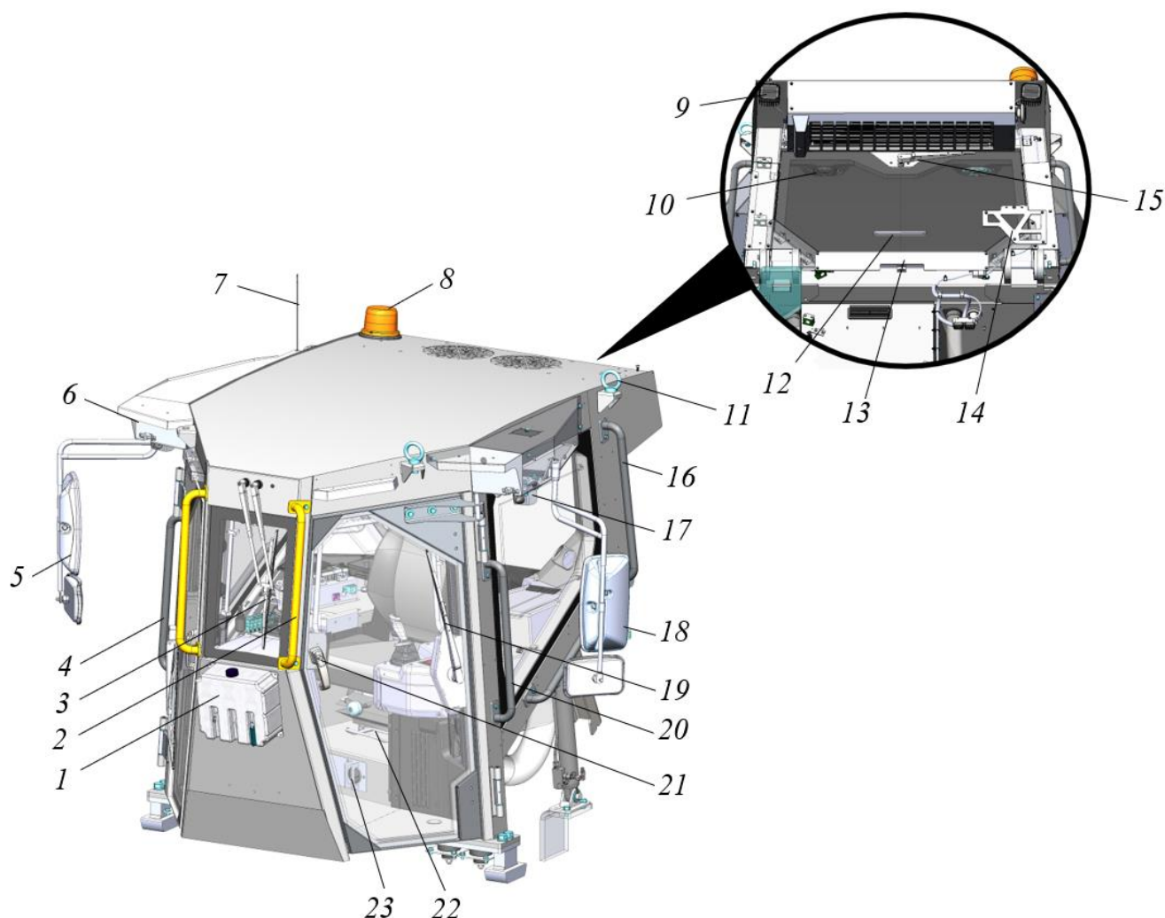
Рисунок 3.1. Кабина оператора
