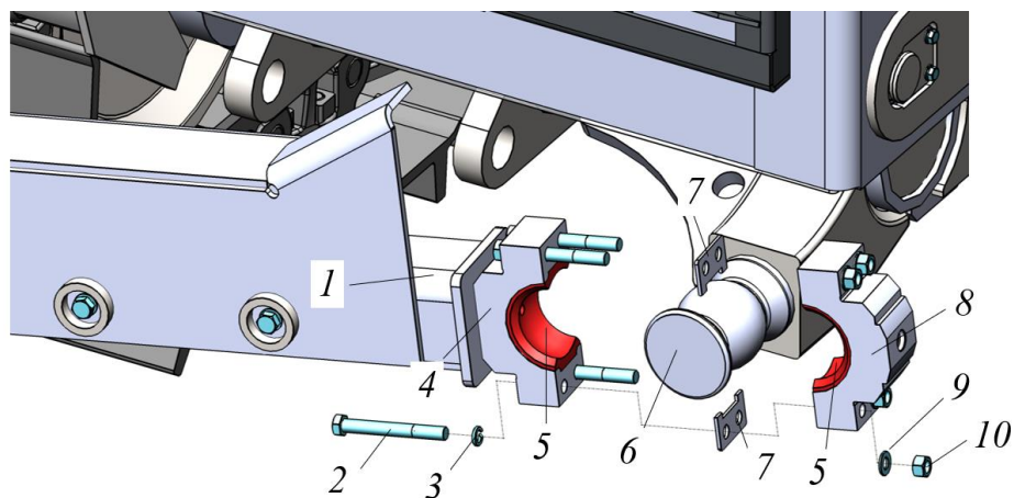
Рисунок 3.130. Установка тяги центральной на трактор
