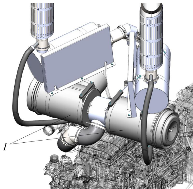
Рисунок 5.57. Воздушные фильтры
