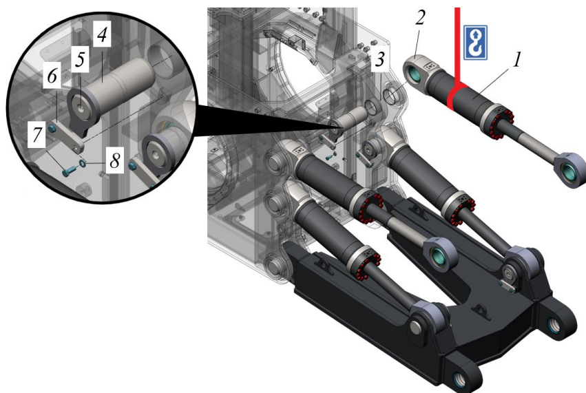
Рисунок 3.140. Установка верхних гидроцилиндров
