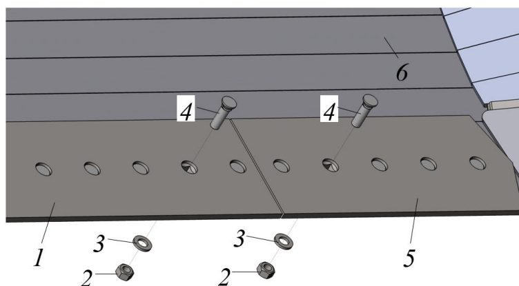
Рисунок 3.136. Нож средний
