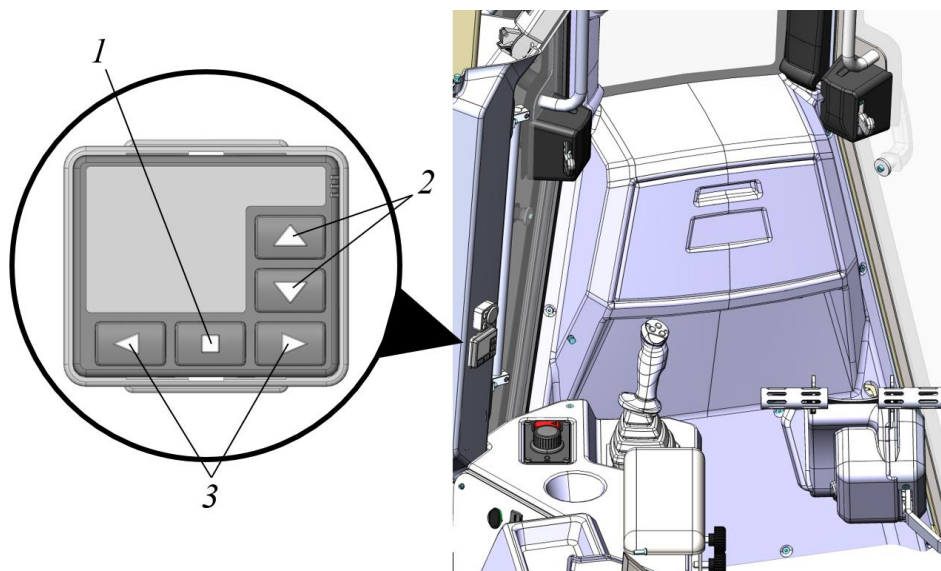
Рисунок 5.82. Расположение пульта управления ПЖД
