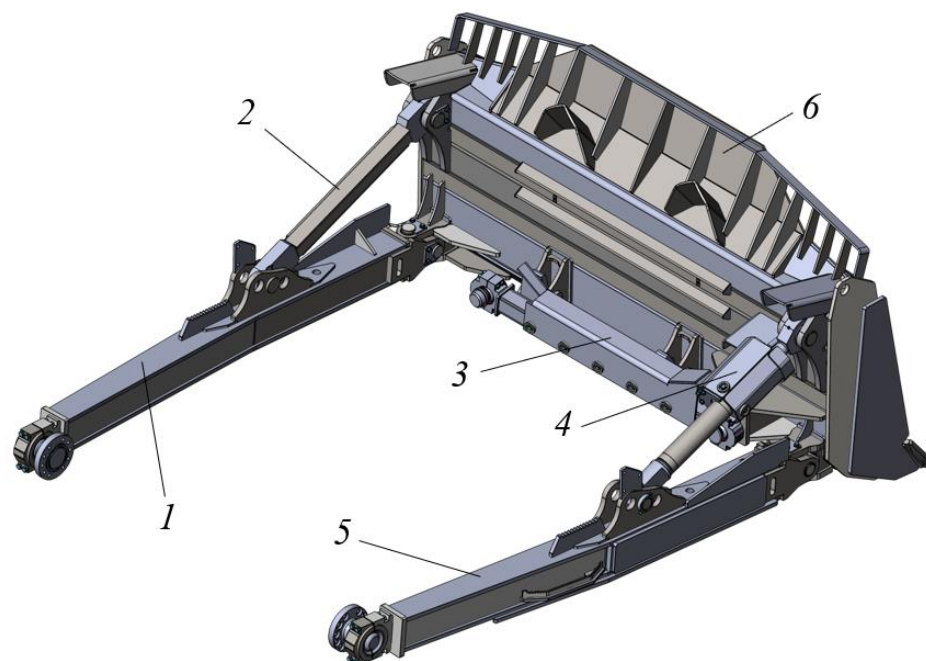
Рисунок 3.117. Бульдозерное оборудование
