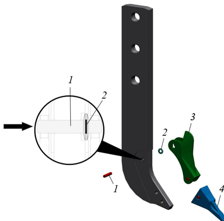
Рисунок 5.165 Процедура замены протектора и наконечника
