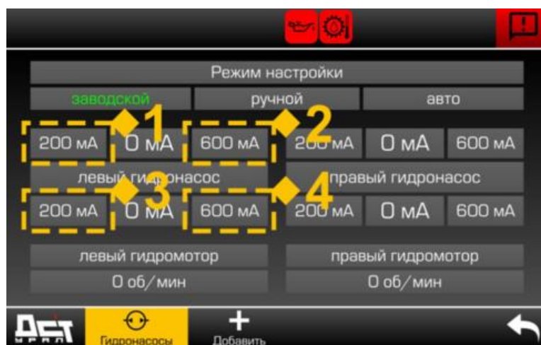
Рисунок 5.133. Минимальные и максимальные значения токов
