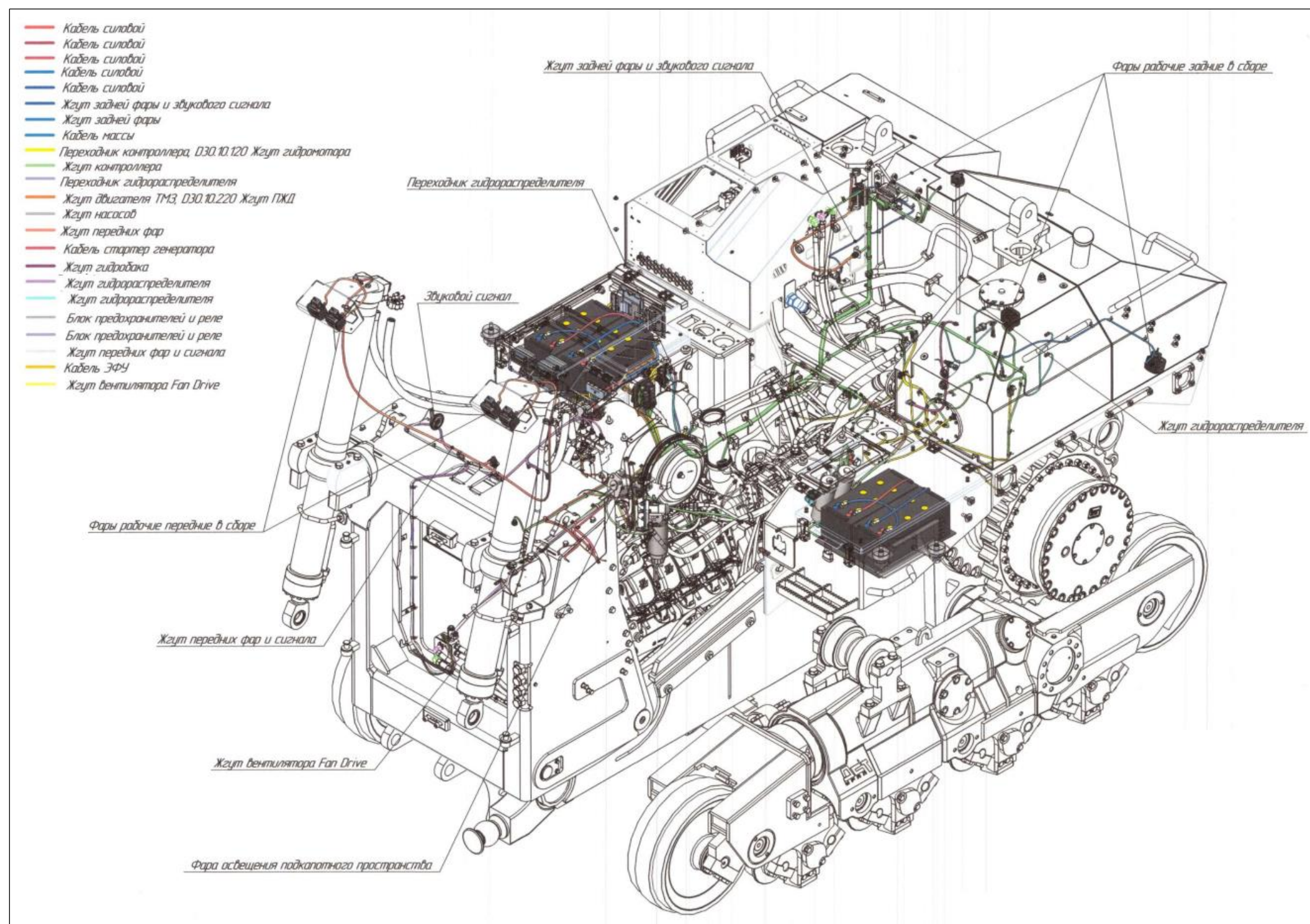
Рисунок 5.117. Разъемы и точки крепления массы GND
