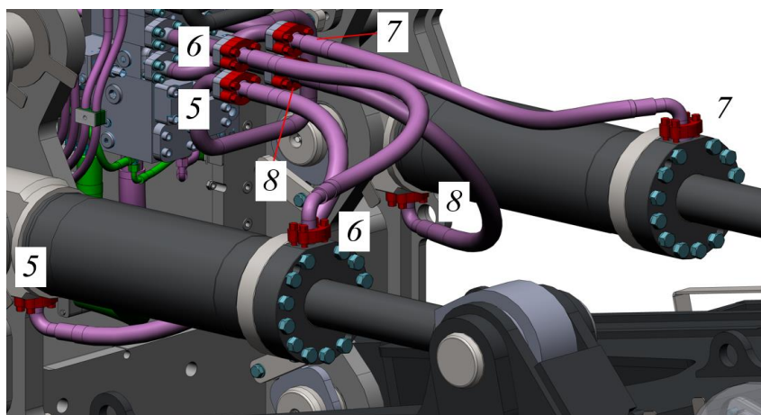
Рисунок 3.145. Подключение РВД к нижним гидроцилиндрам
