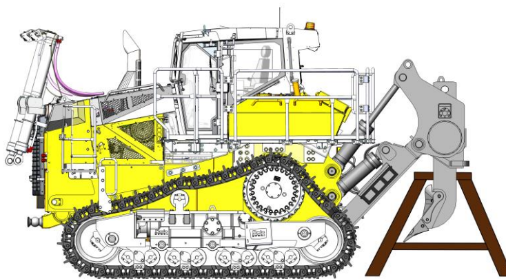
Рисунок 5.163 Подпорка под рыхлитель
