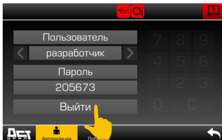
Рисунок 3.7. Деавторизация
