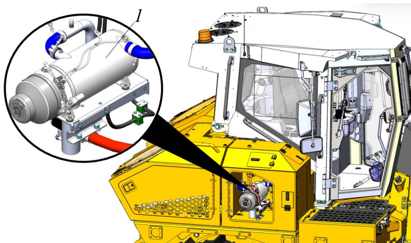
Рисунок 5.80. Расположение ПЖД
