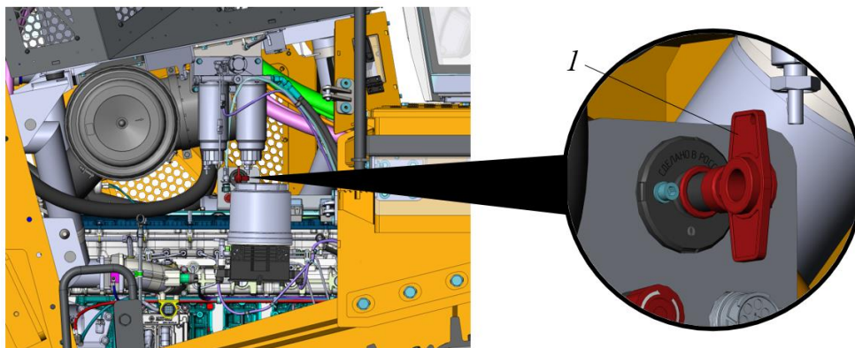
Рисунок 3.47. Главный выключатель АКБ
