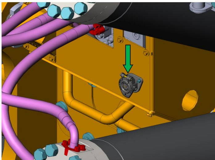
Рисунок 3.46. Розетка для подключения датчика положения рыхлителя
