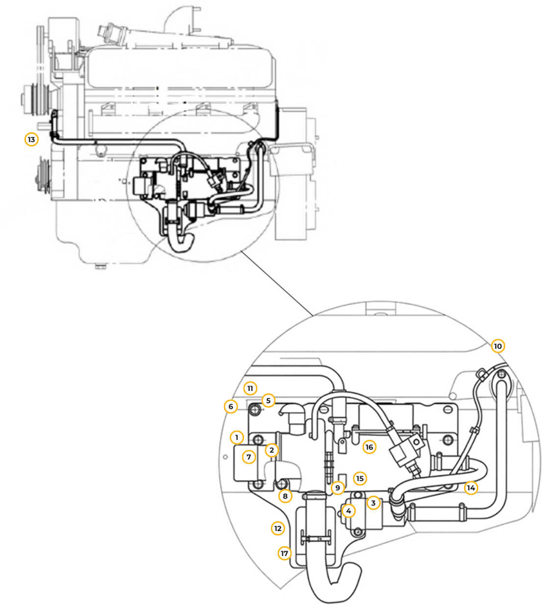
Рис. 23. Установка ПЖД
