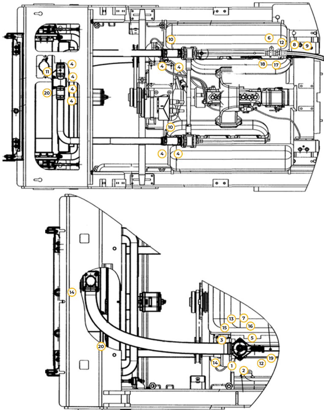
Рис. 12. Система охлаждения
