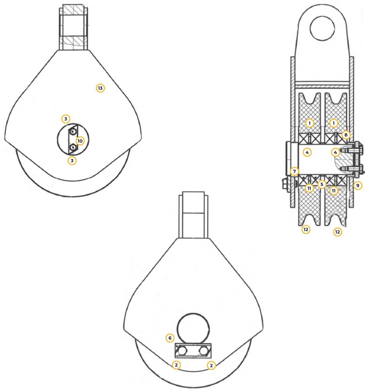
Рис. 123. Блок стреловой
