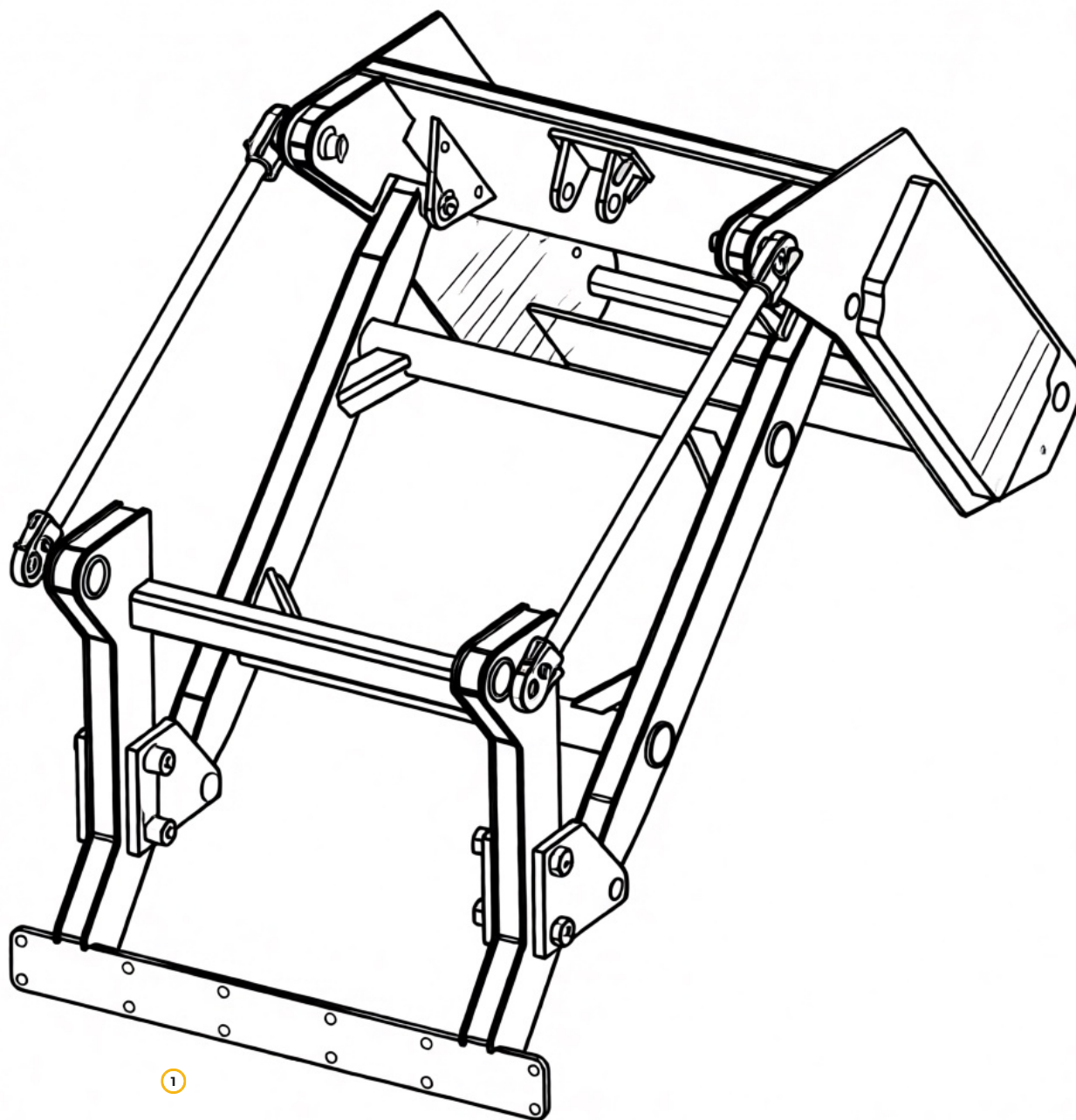
Рис. 113. Рама контргруза в сборе
