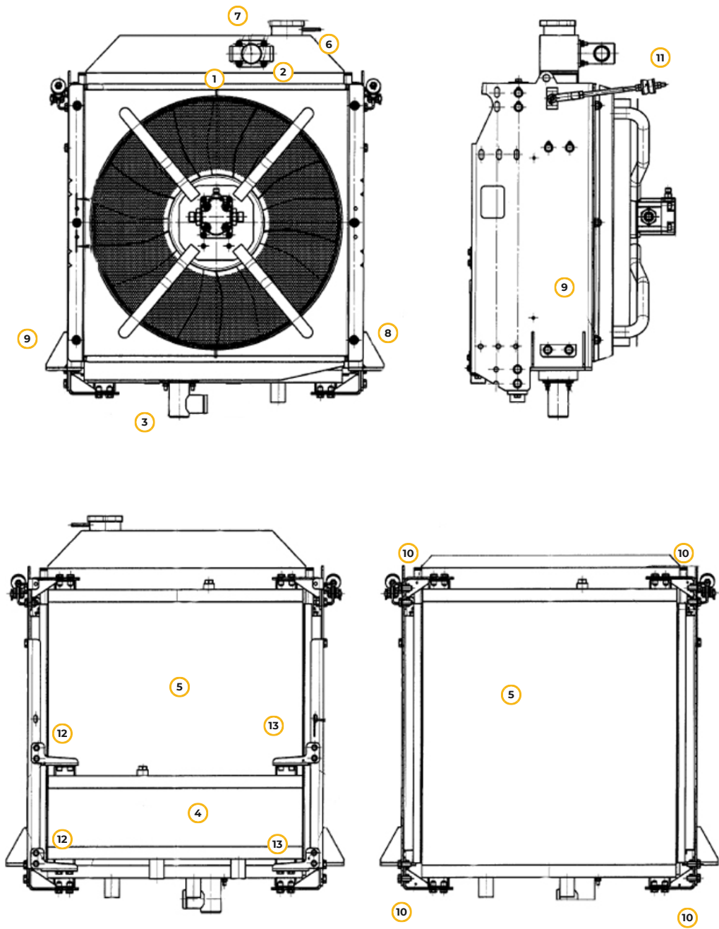
Рис. 14. Блок радиаторов в сборе
