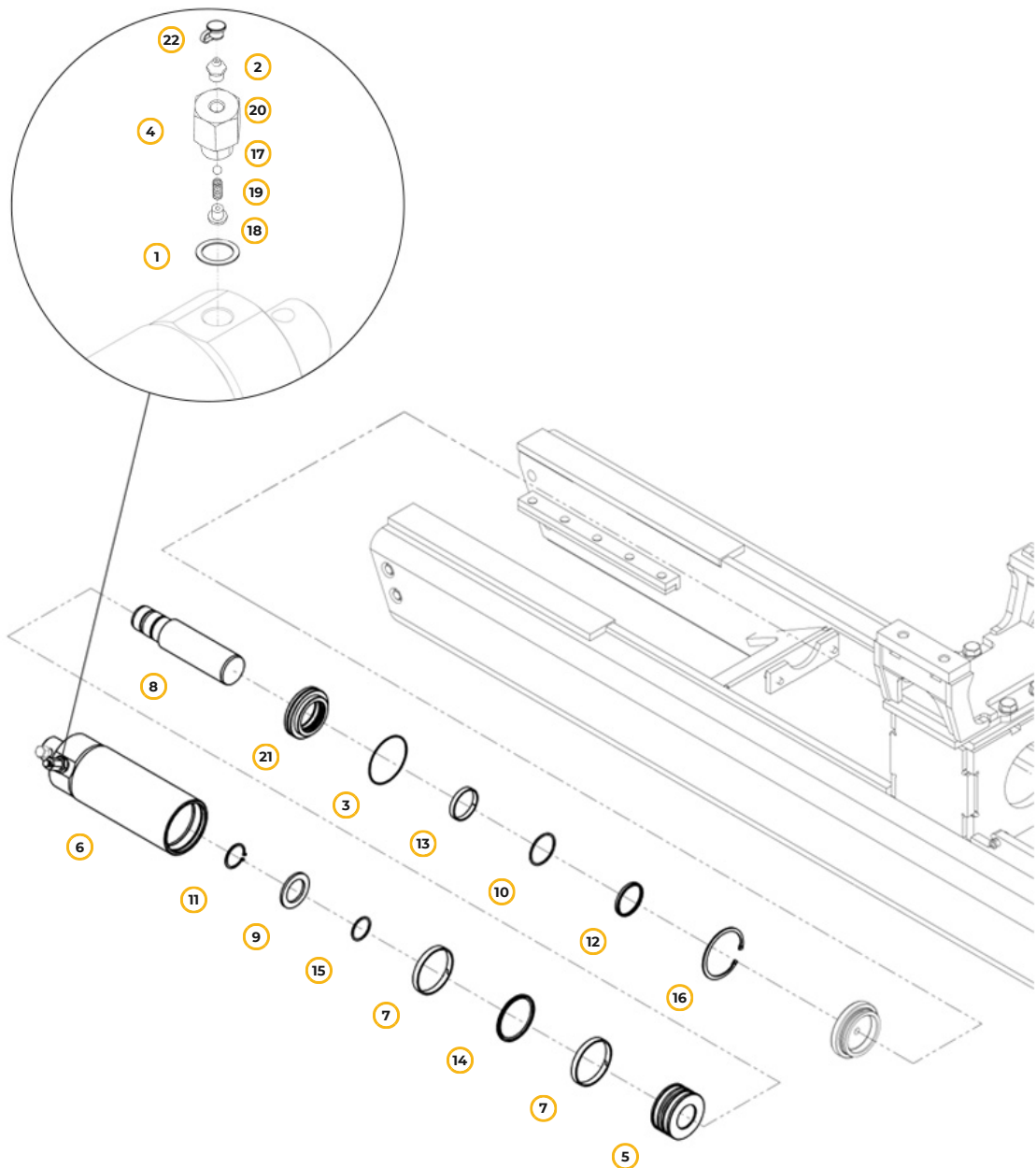
Рис. 44. Механизм натяжения
