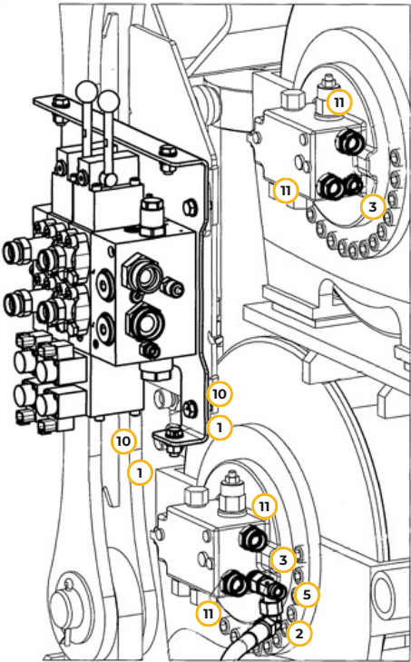
Рис. 50. РВД гидросистемы навесного оборудования
