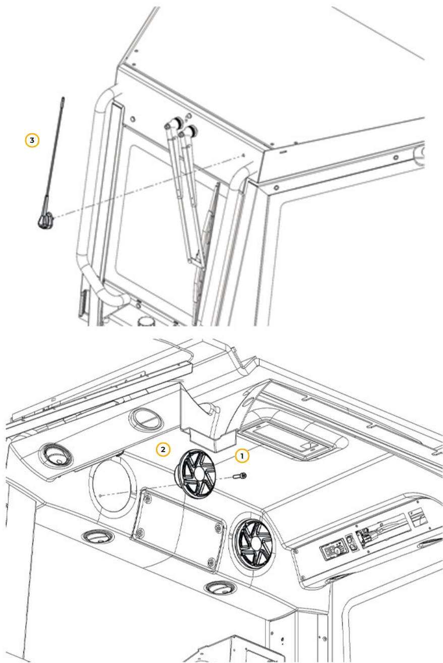
Рис. 68. Антенна и Колонки
