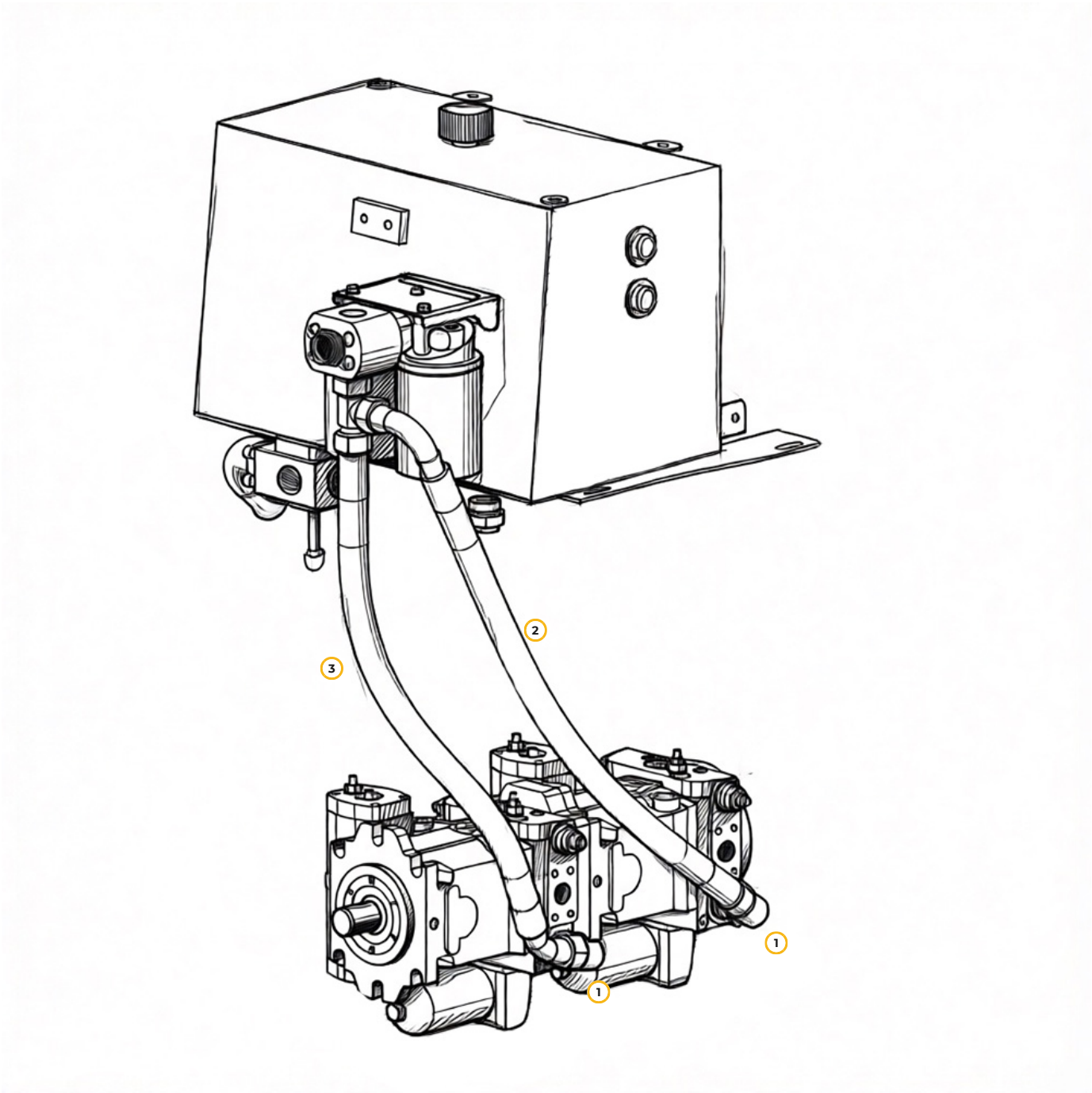
Рис. 61. Трубопроводы гидросистемы трансмиссии
