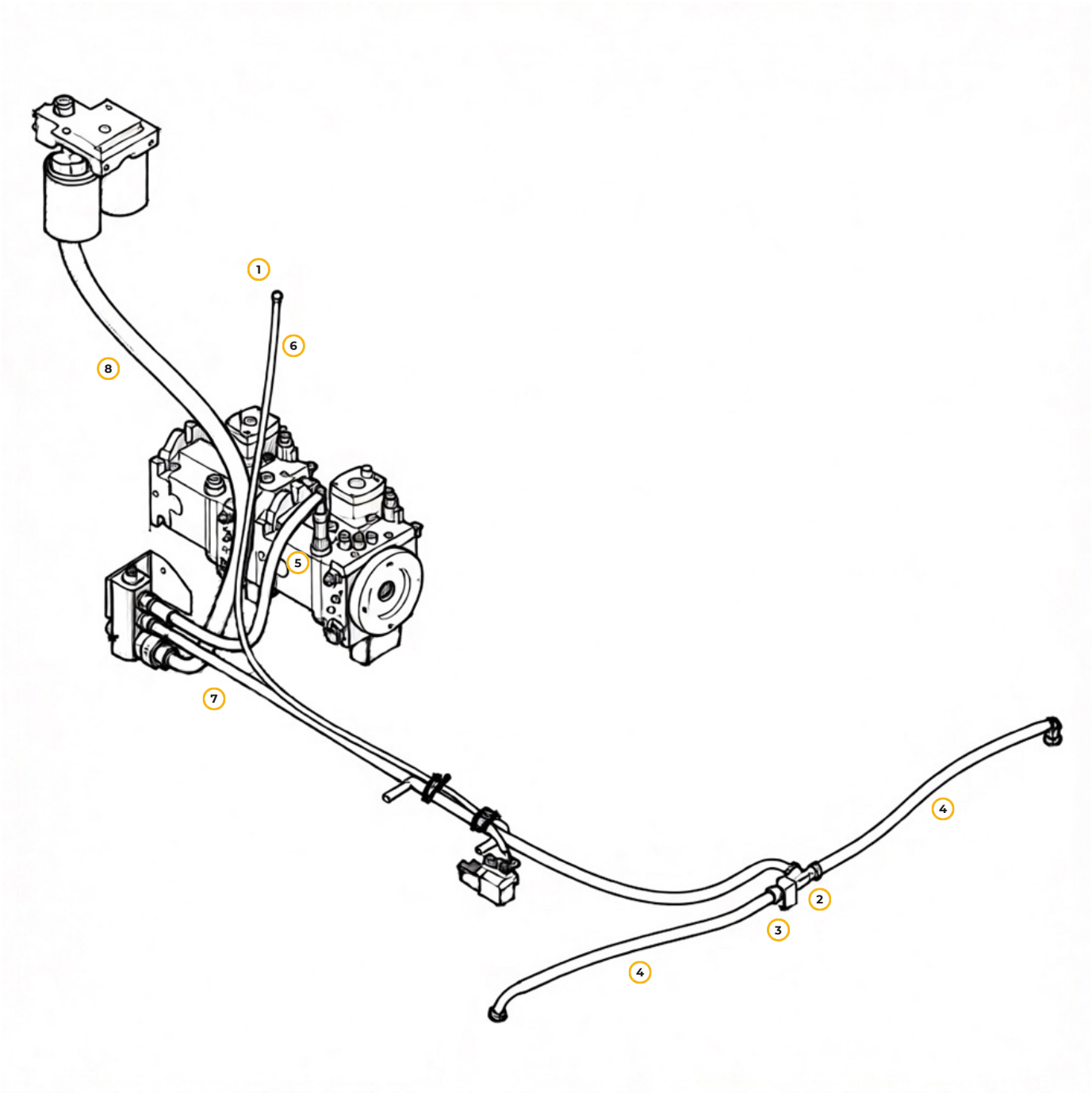
Рис. 62. Трубопроводы гидросистемы трансмиссии
