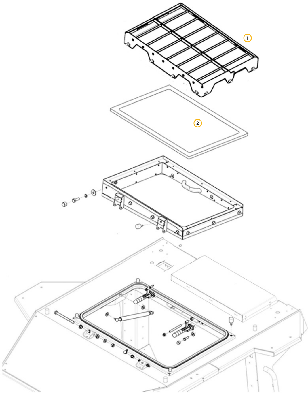
Рис. 109. Установка люка
