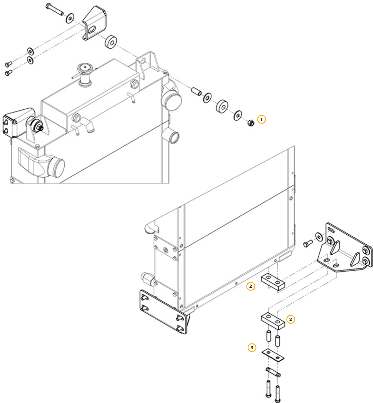
Рис. 13. Крепление радиатора
