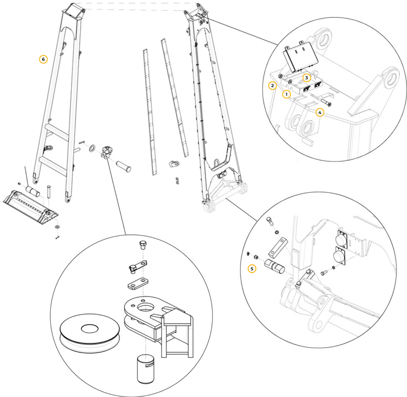
Рис. 119. Стрела в сборе
