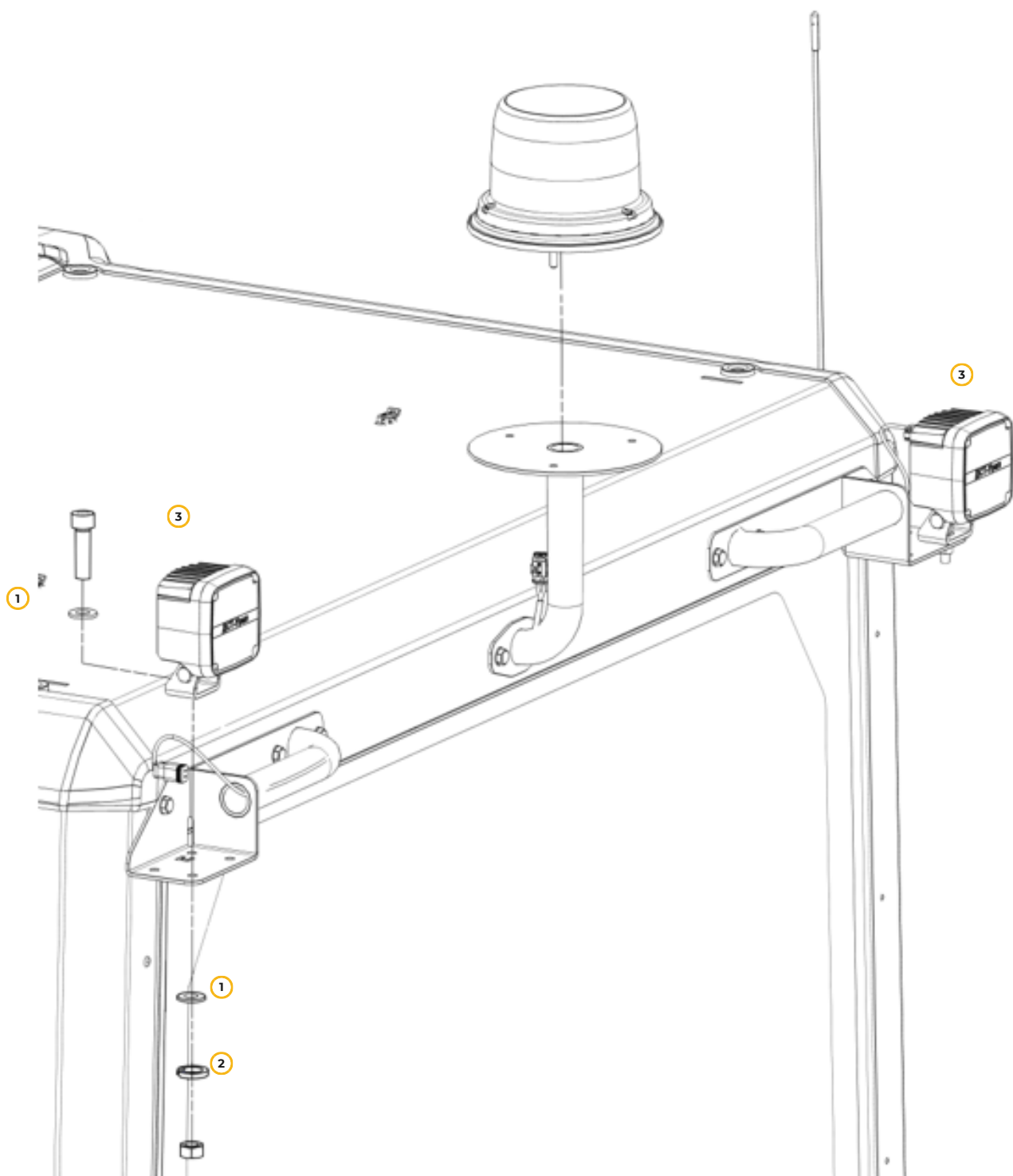
Рис. 71. Элементы освещения и звуковой сигнализации кабины
