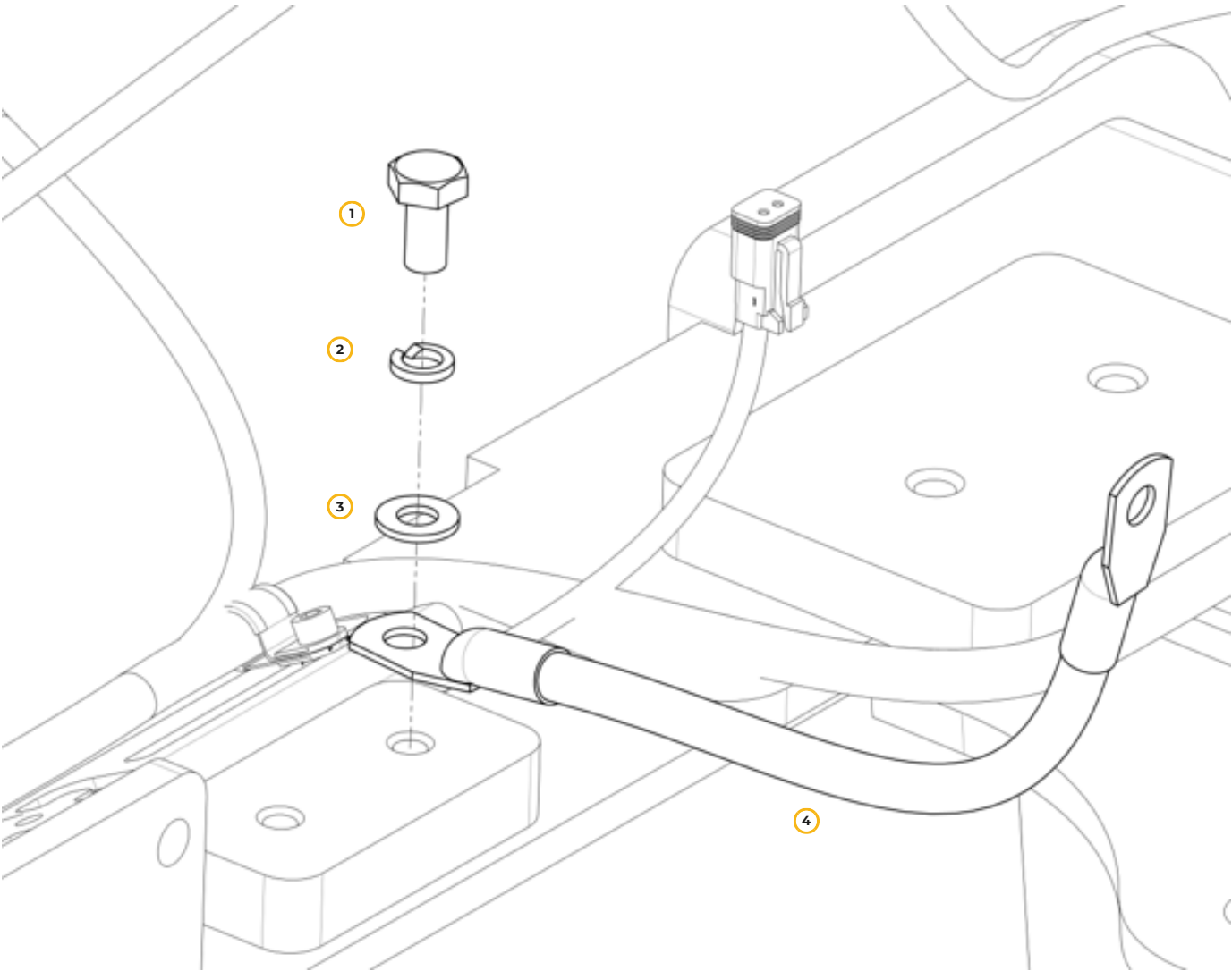
Рис. 85. Электрооборудование рамы
