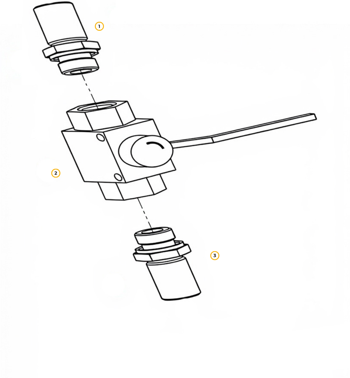
Рис. 50. Краны гидросистемы трансмиссии
