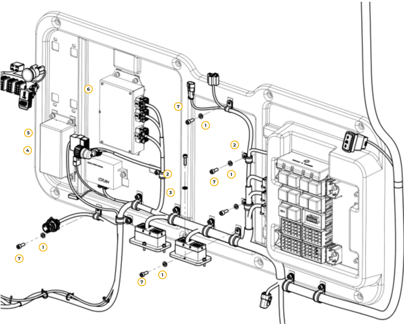
Рис. 59. Задняя панель в сборе
