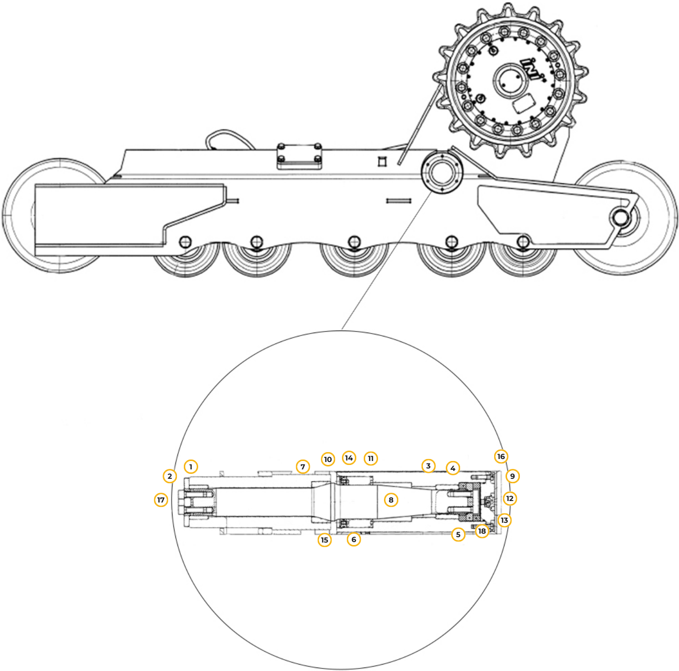
Рис. 21. Система ходовая
