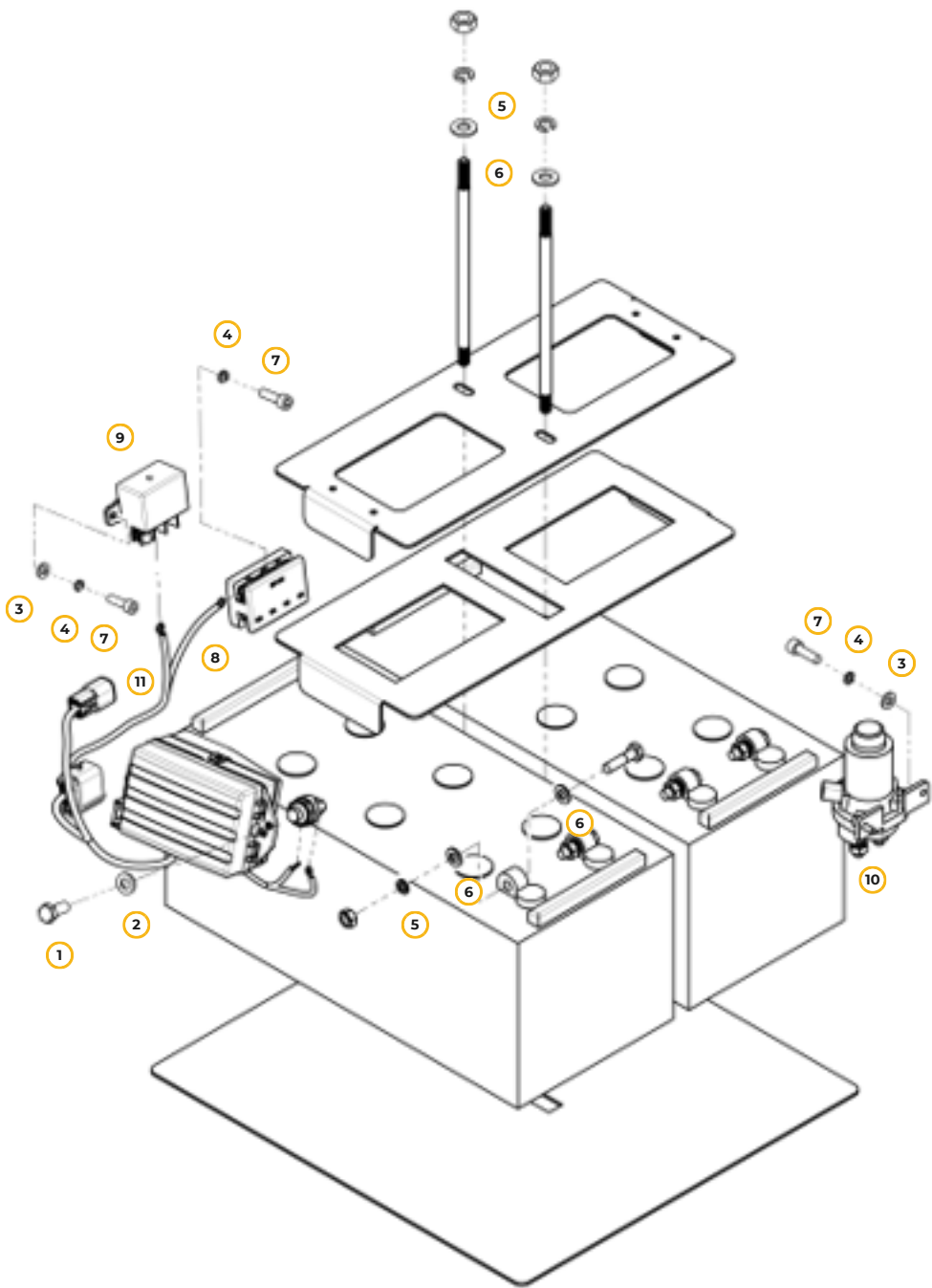
Рис. 76. Аккумуляторные батареи с элементами крепления
