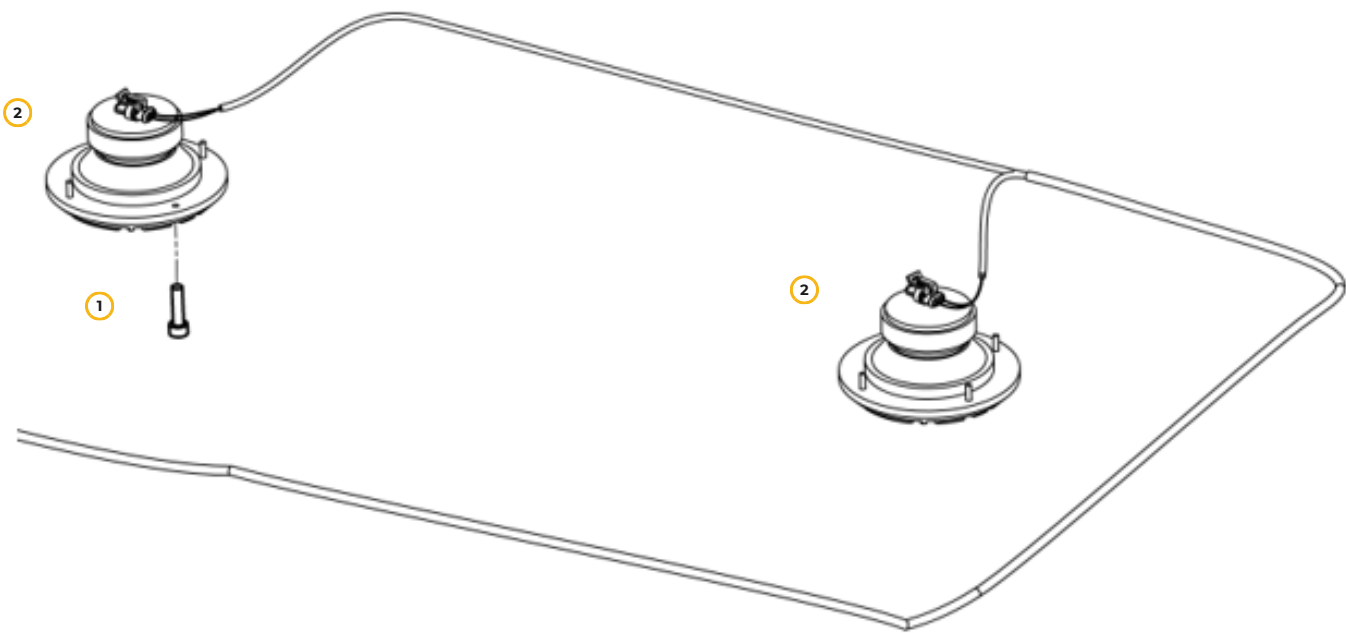
Рис. 60. Электрооборудование кабины
