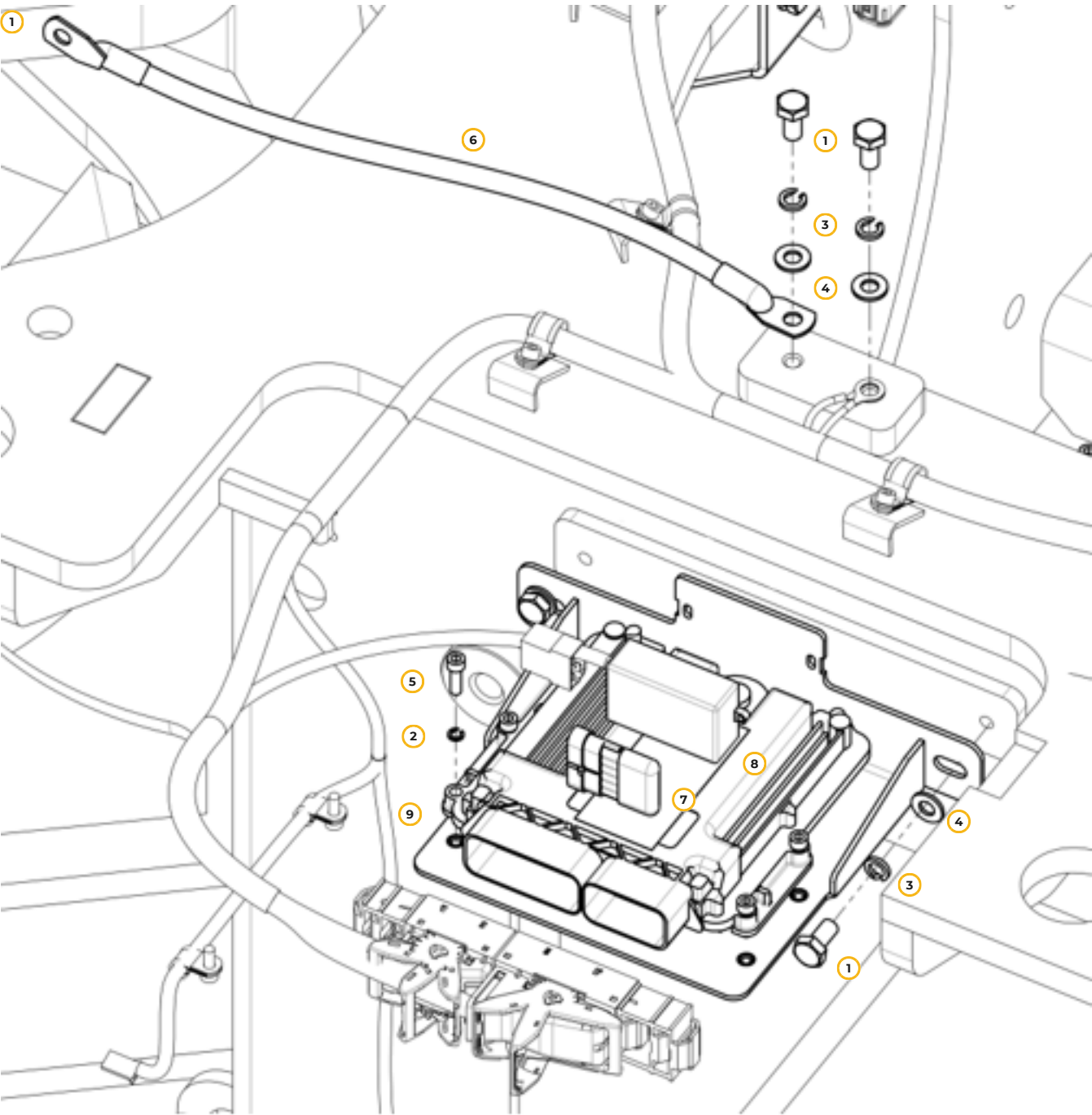
Рис. 84. Контроллер трансмиссии
