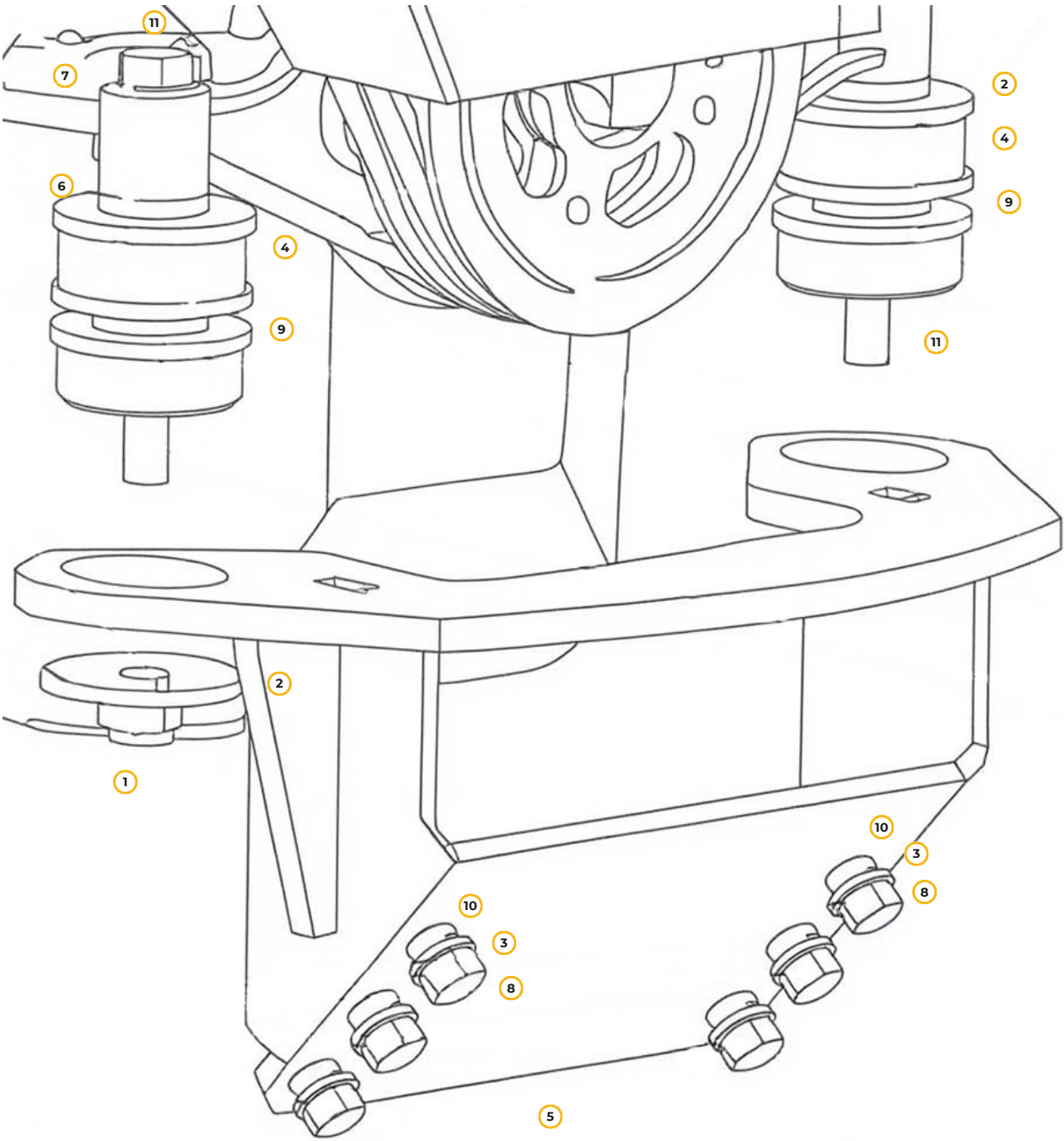
Рис. 1. Установка силового агрегата
