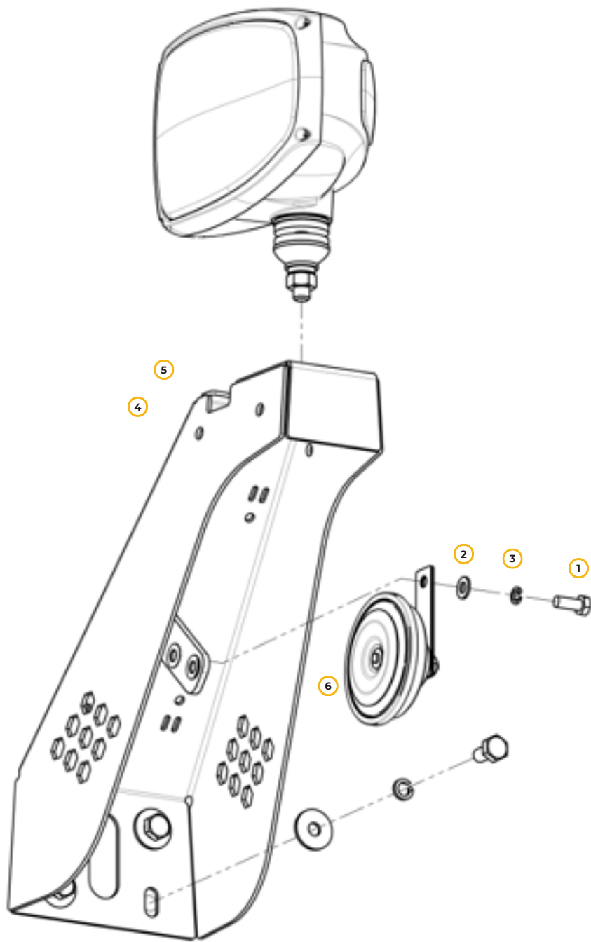
Рис. 70. Элементы освещения и звуковой сигнализации кабины
