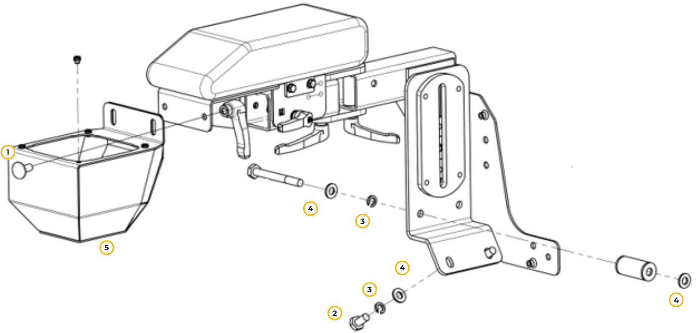
Рис. 94. Установка панелей
