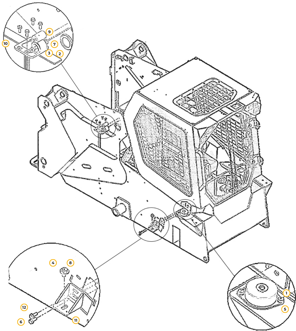
Рис. 90. Опоры кабины
