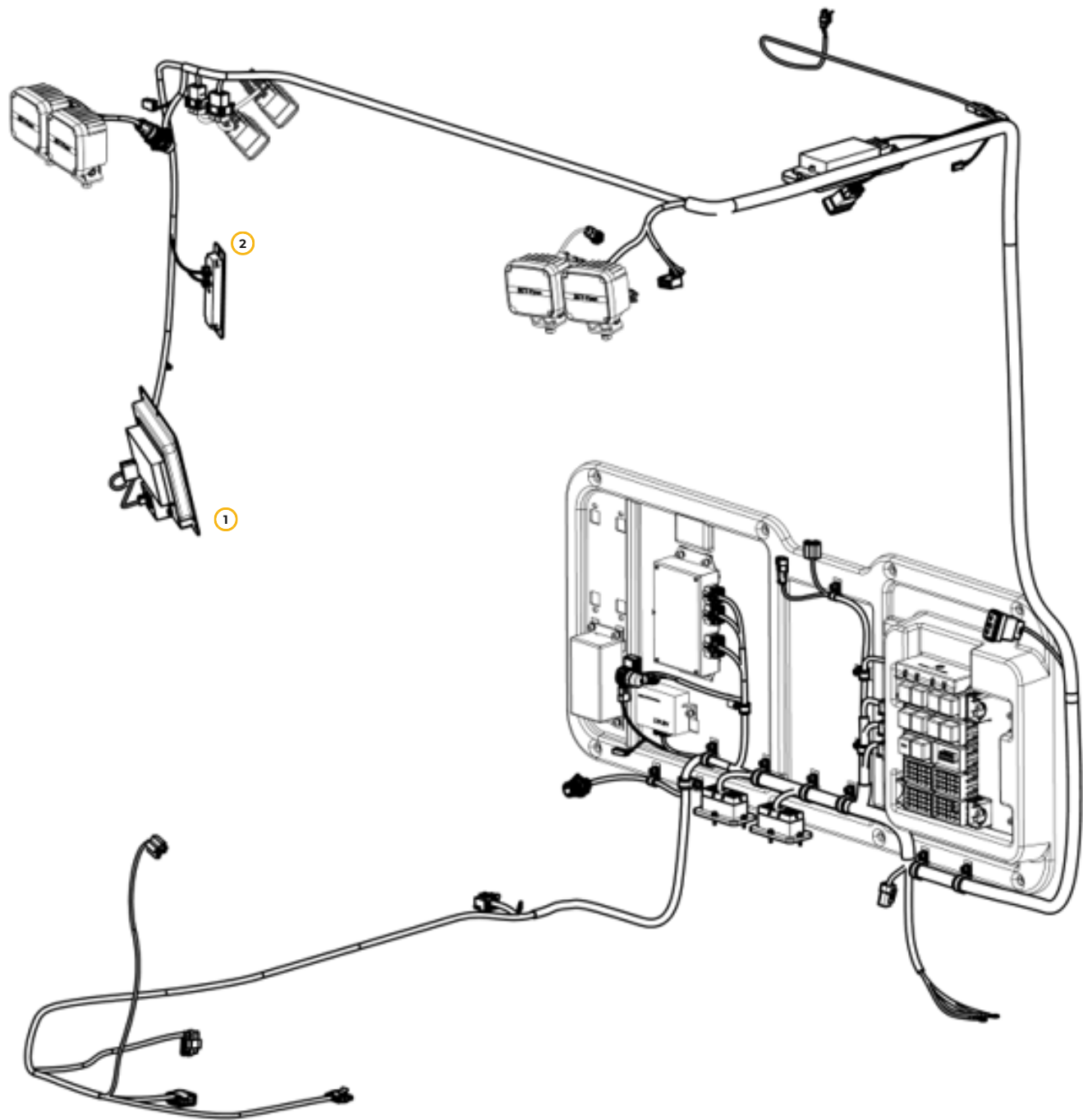
Рис. 58. Электрооборудование кабины
