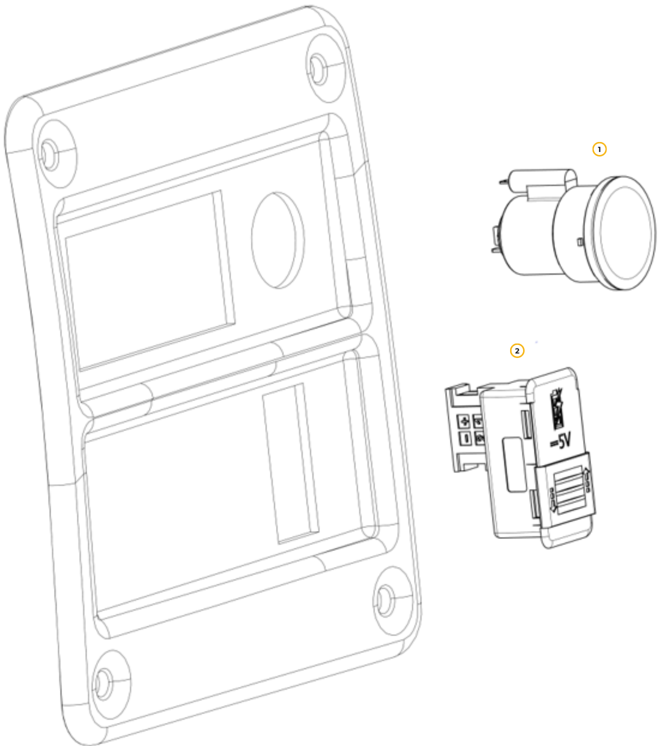
Рис. 64. Панель управления
