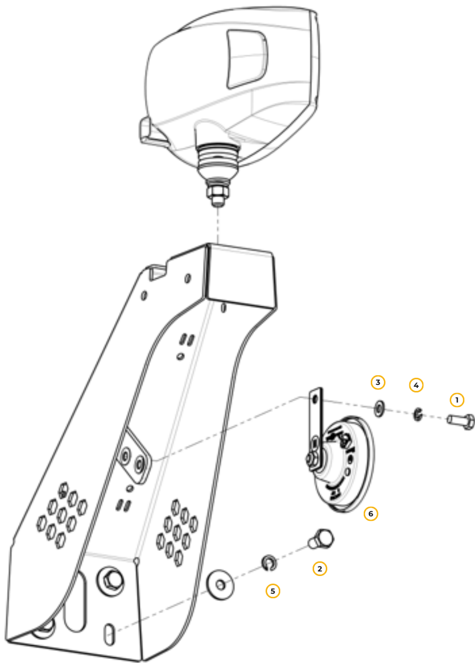
Рис. 75. Элементы освещения и звуковой сигнализации рамы
