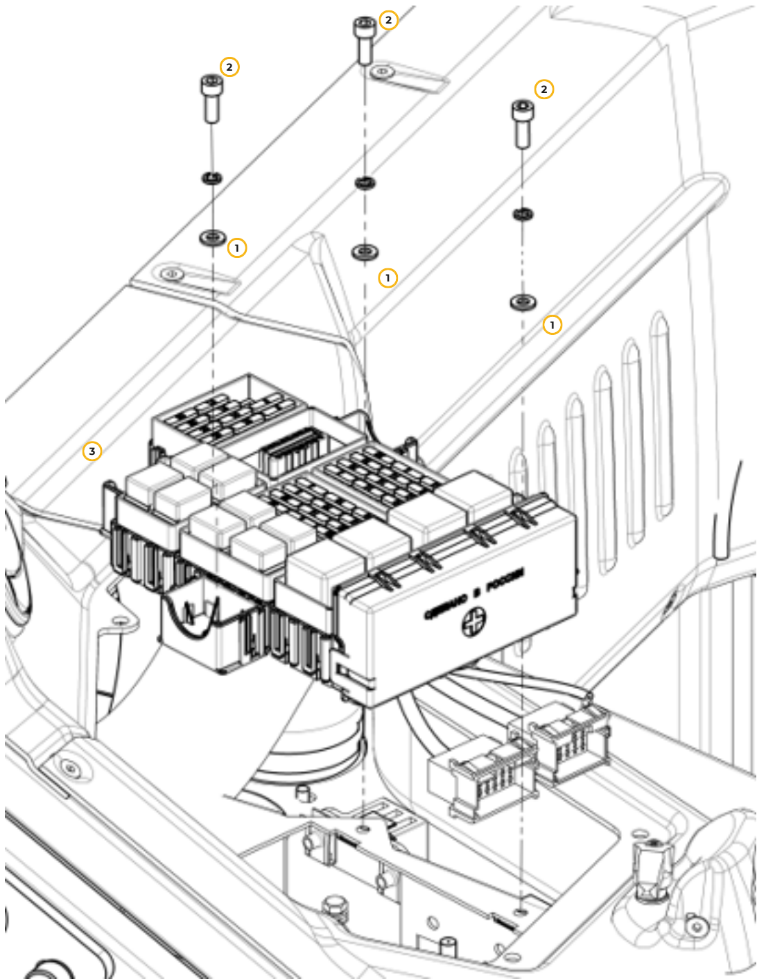
Рис. 69. Блок предохранителей и реле
