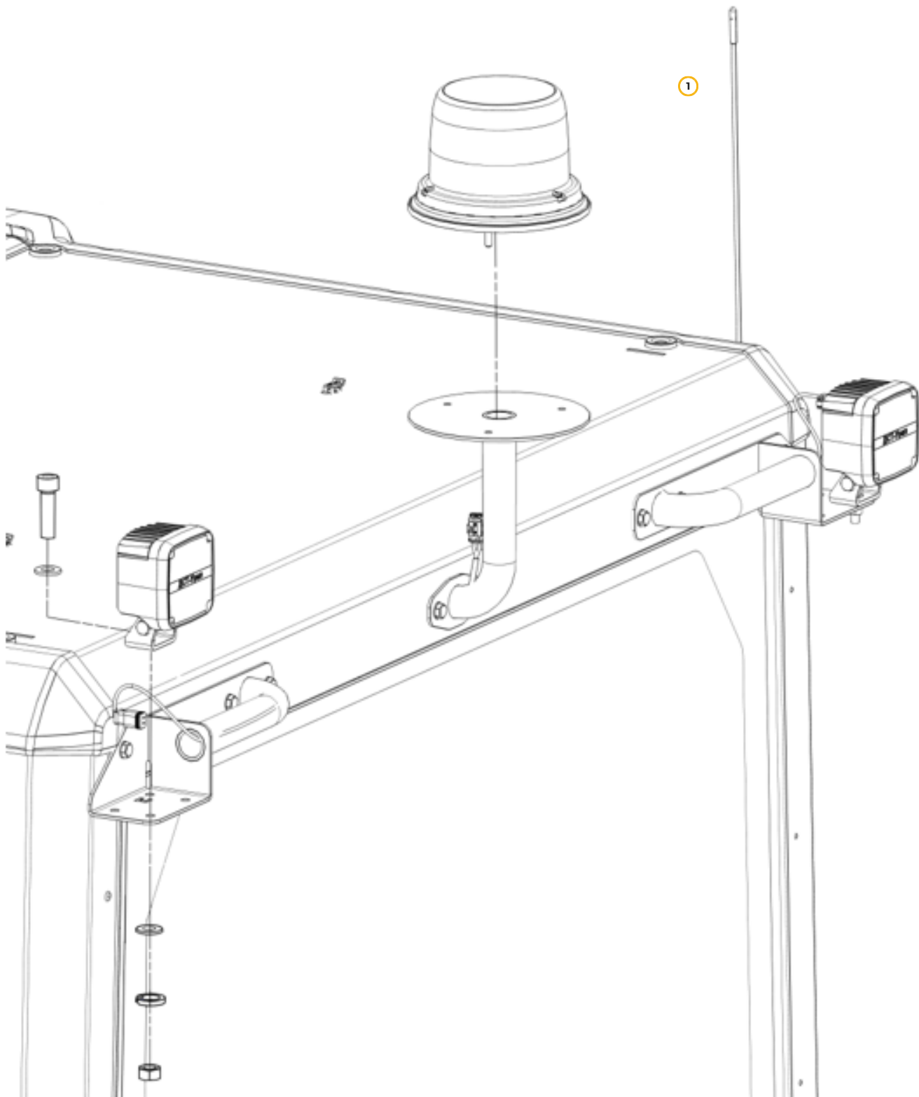
Рис. 61. Антенна радио
