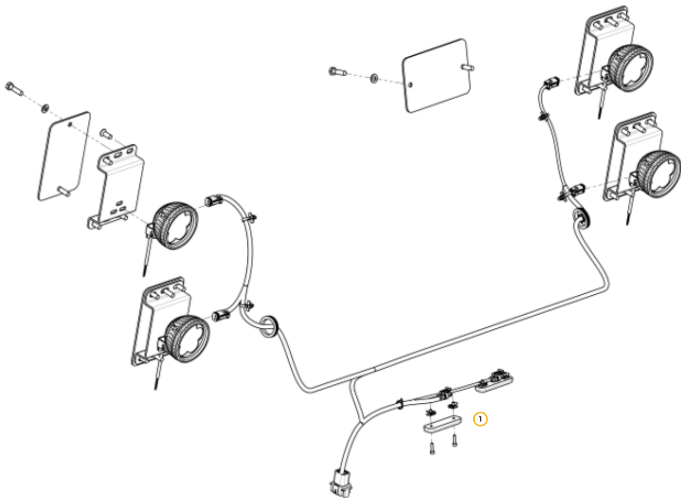
Рис. 77. Элементы освещения и звуковой сигнализации рамы
