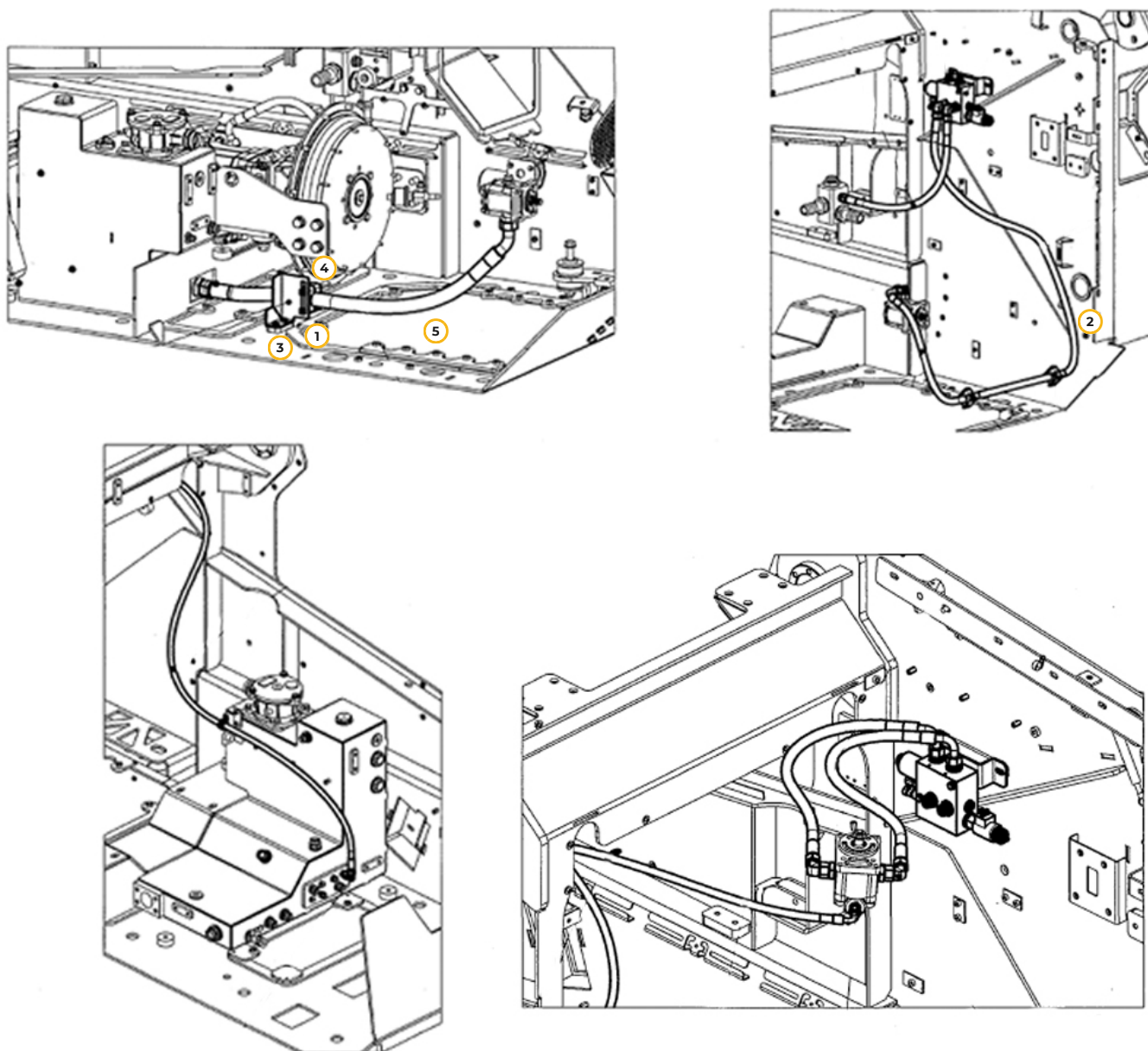
Рис. 11. Трубопроводы гидропривода вентилятора
