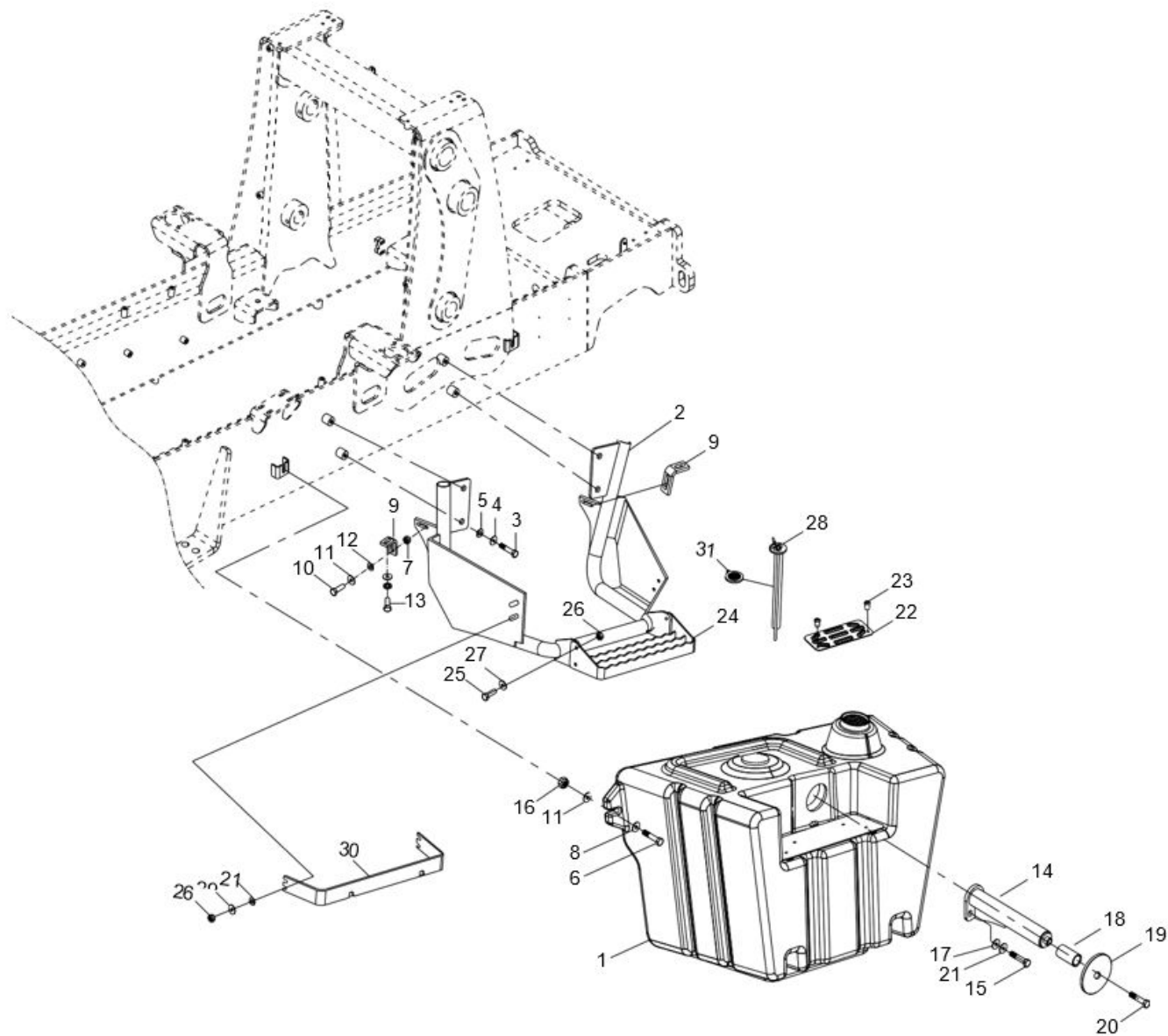
Рис. 15. Топливный бак в сборе
