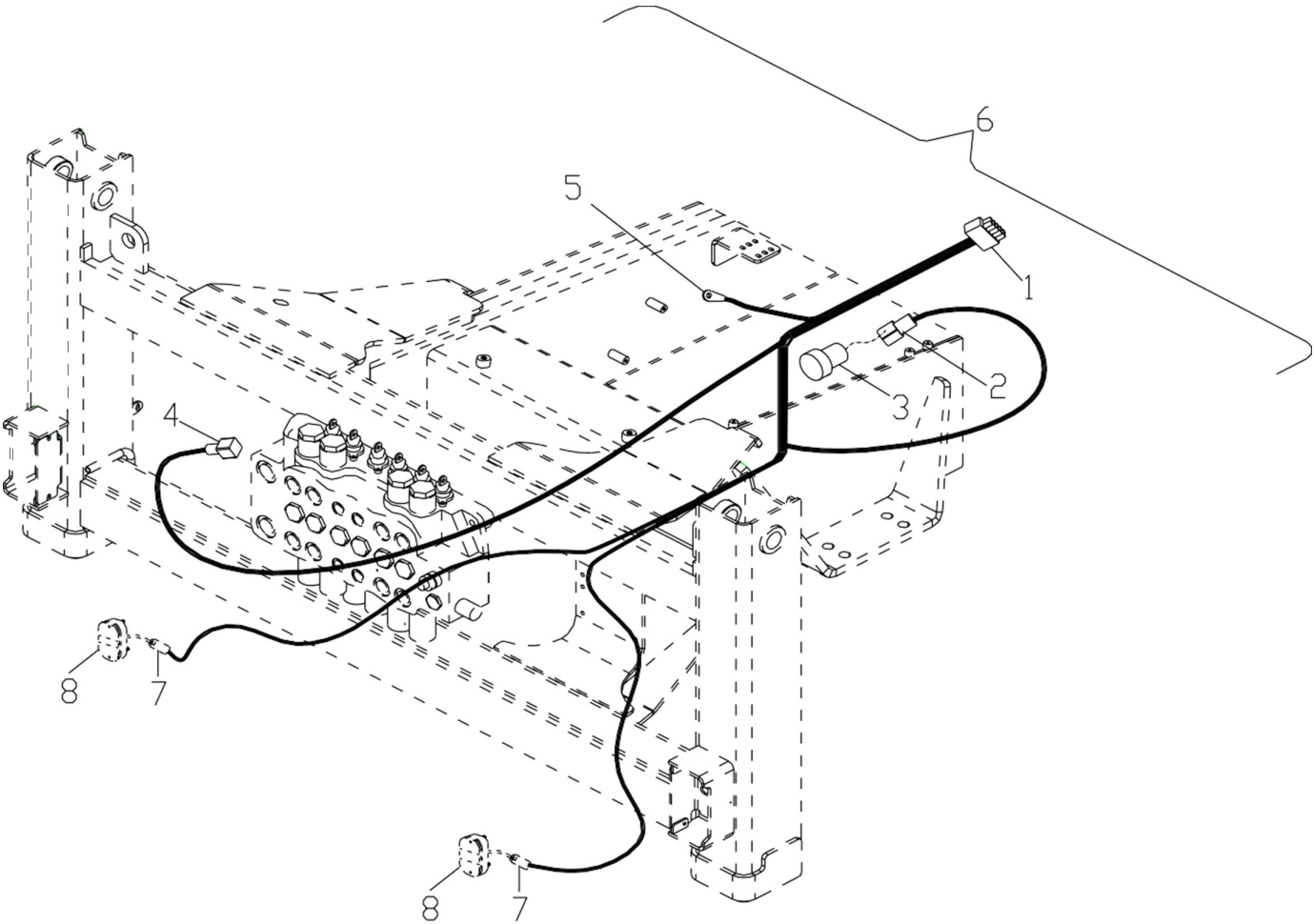
Рис. 42. Группа электропроводки рамы
