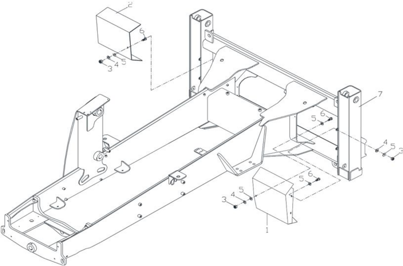
Рис. 19. Рама в сборе
