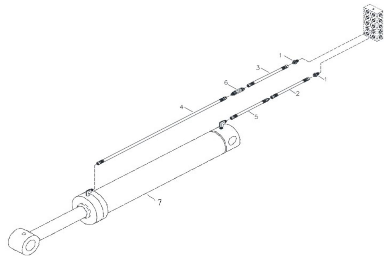
Рис. 79. Гидросистема рукояти экскаватора
