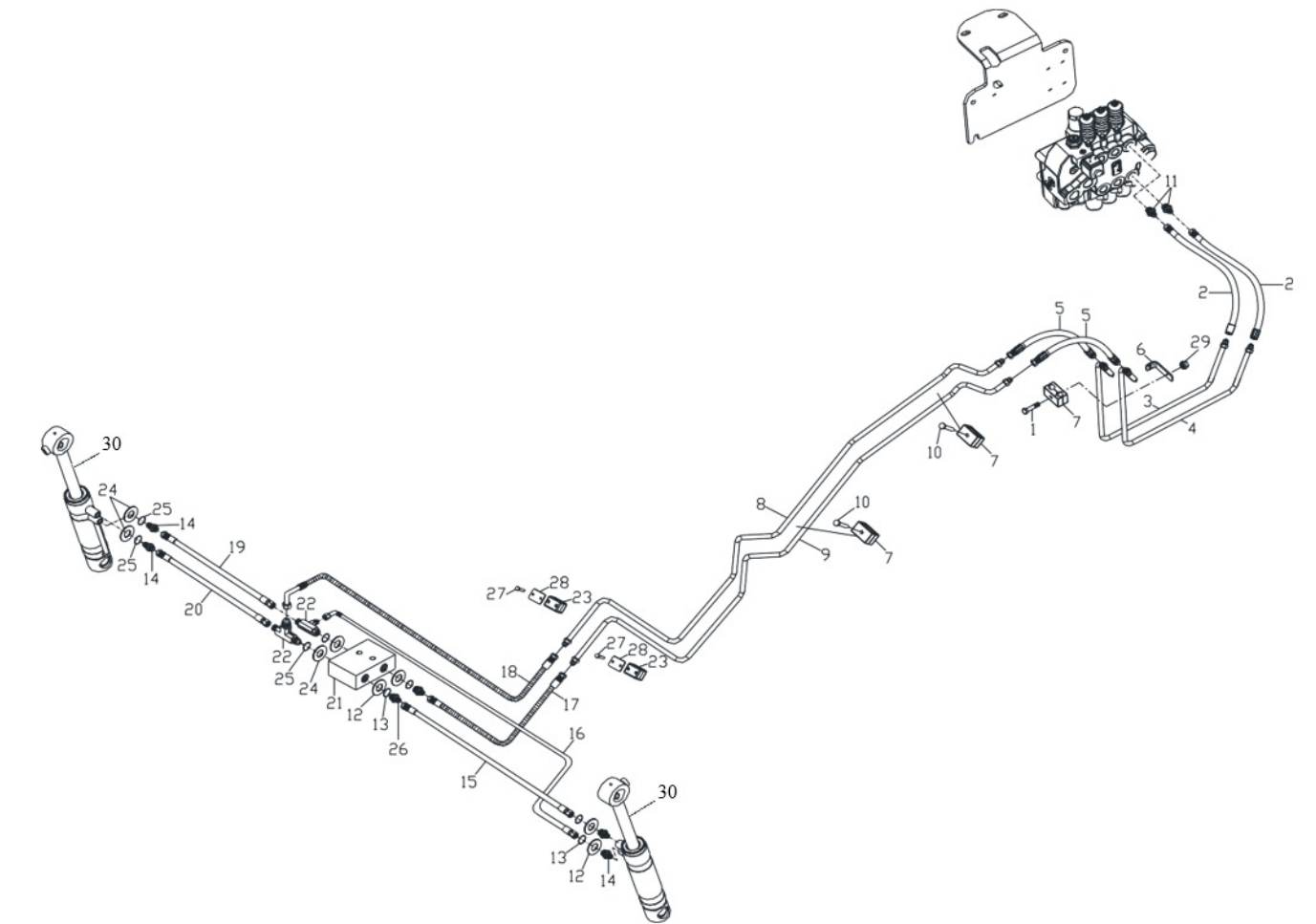
Рис. 65. Гидросистема открывания ковша погрузчика
