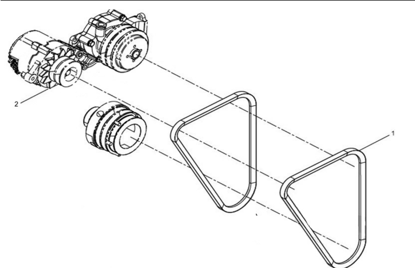
Рис. 1. Генератор и ремень
