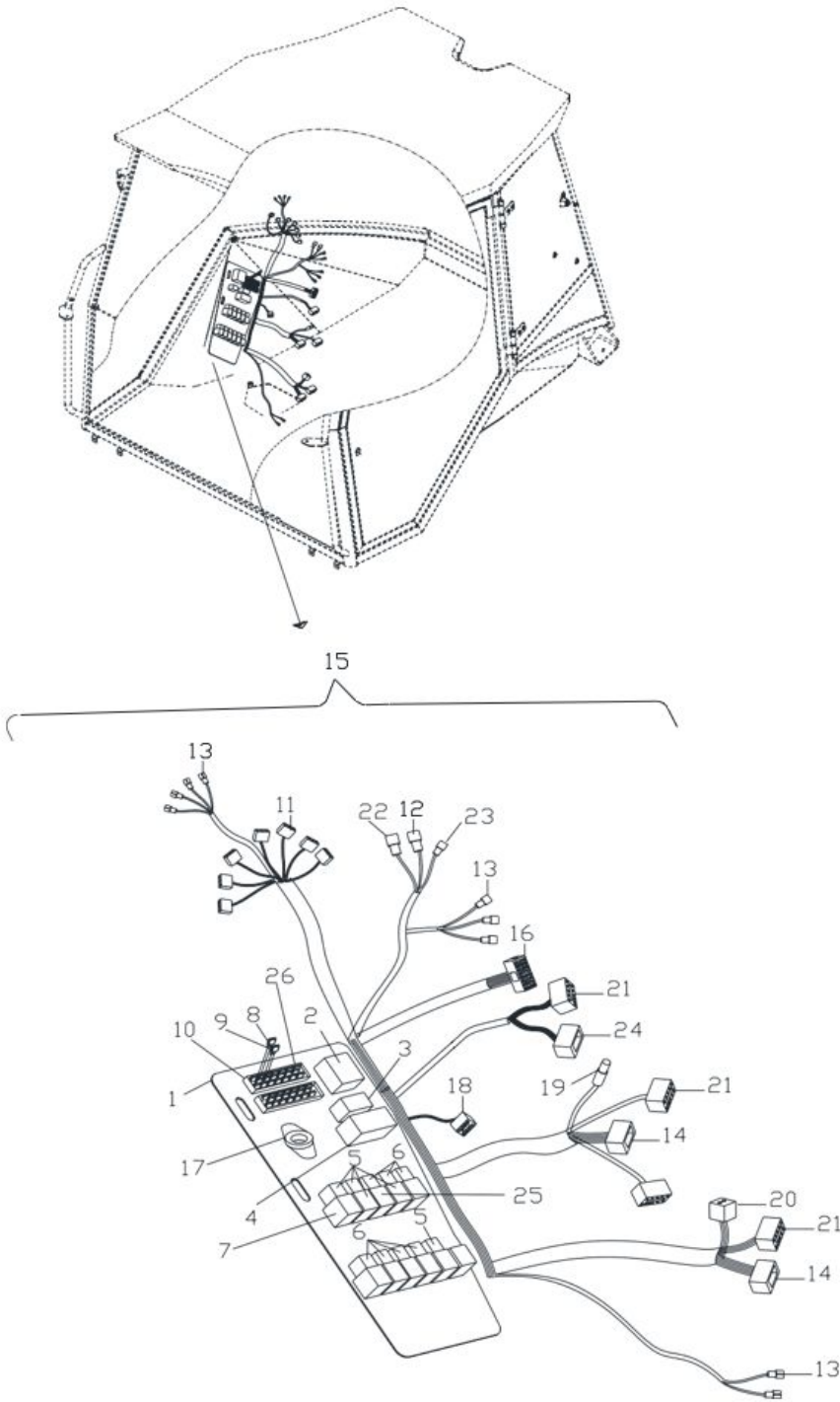
Рис. 36. Группа реле и предохранителей
