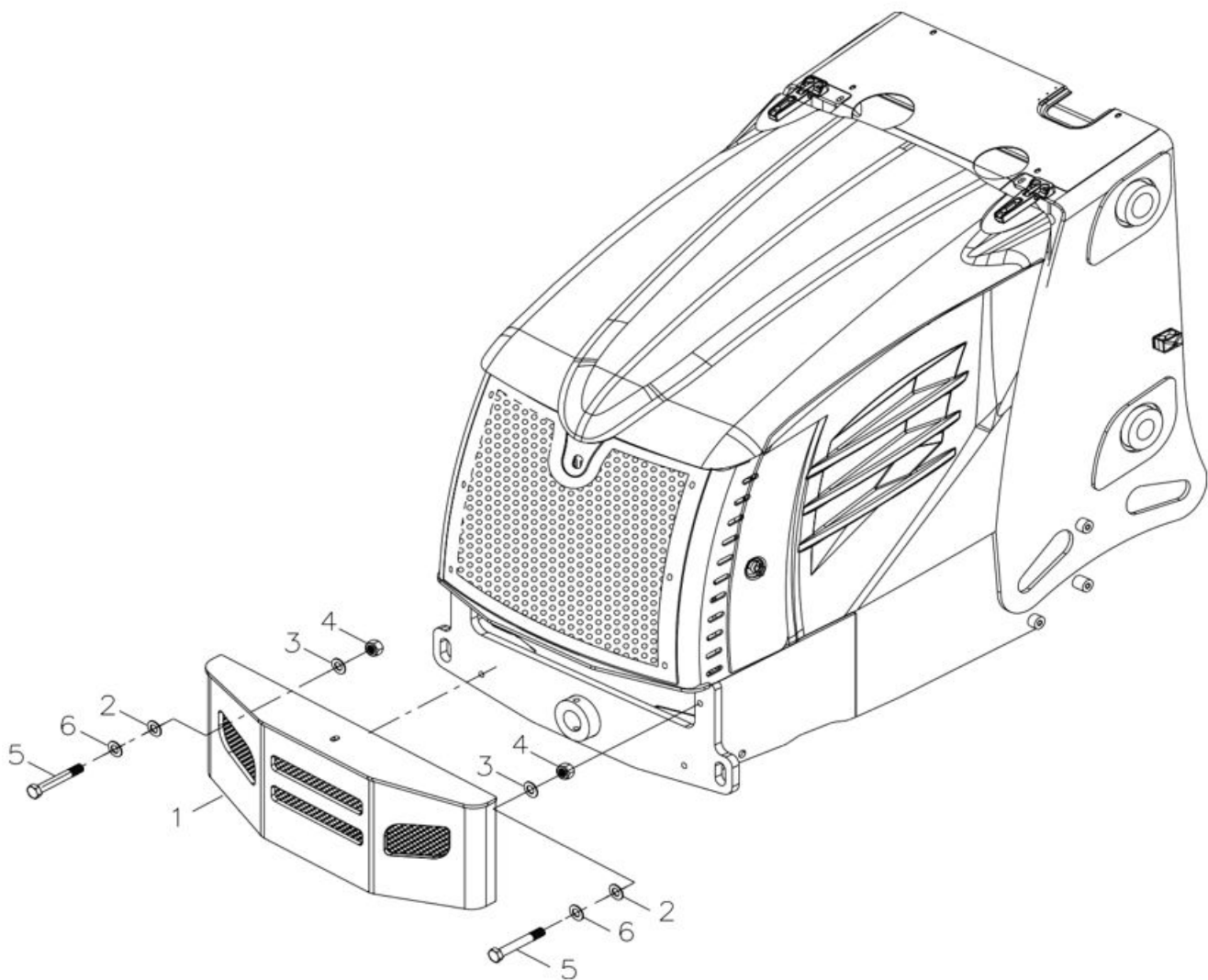
Рис. 64. Контргруз в сборе
