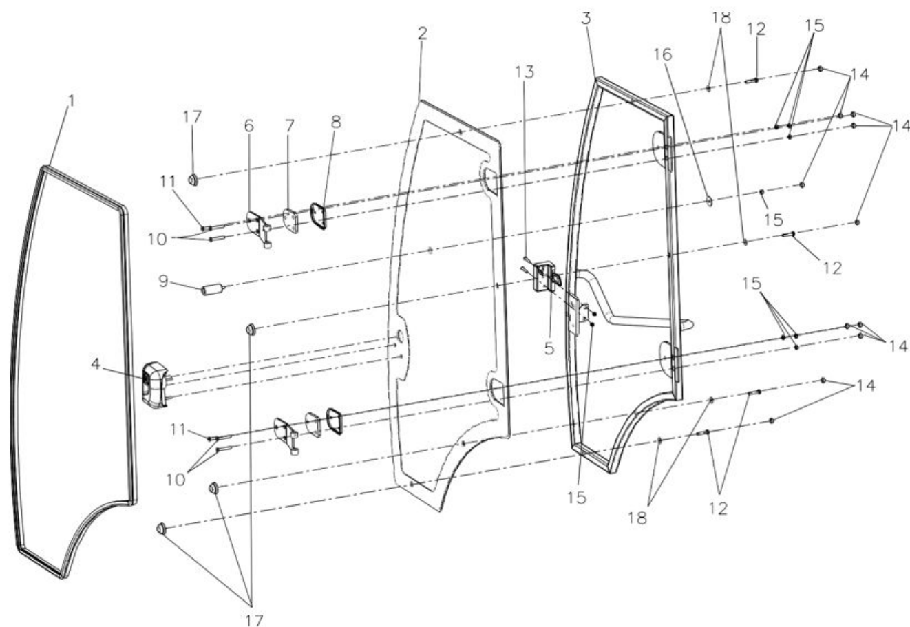
Рис. 48. Левая дверь в сборе
