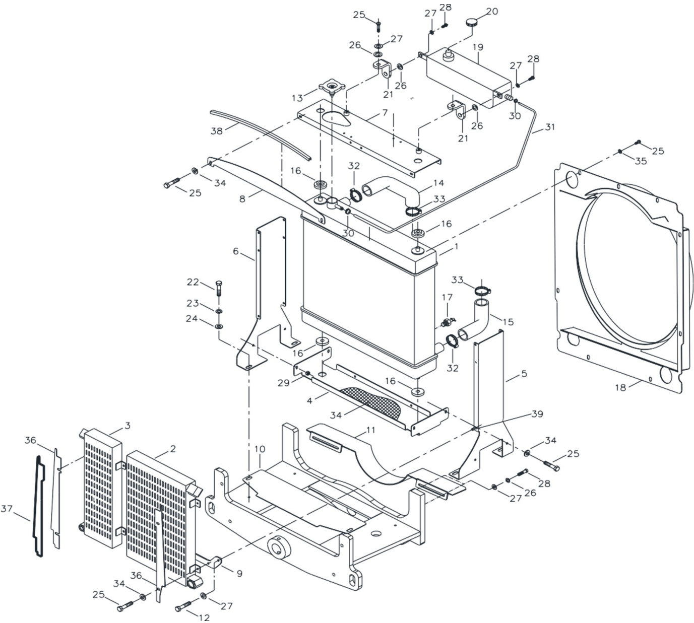
Рис. 10. Система охлаждения двигателя
