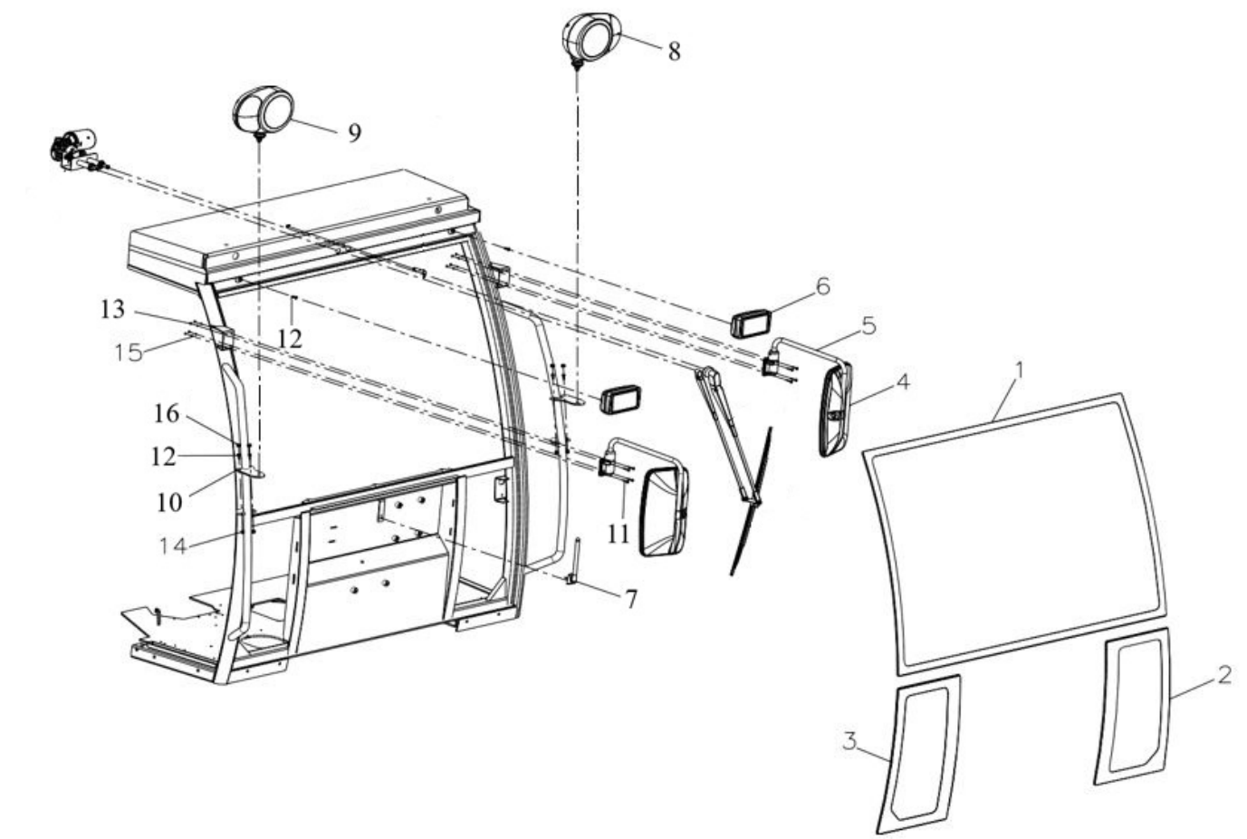
Рис. 50. Передние окна и внешние навесные элементы
