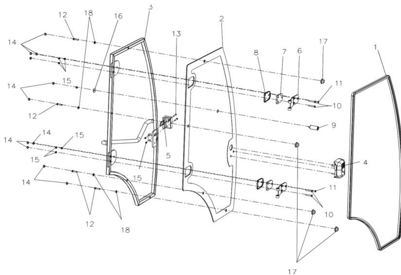
Рис. 51. Правая дверь в сборе
