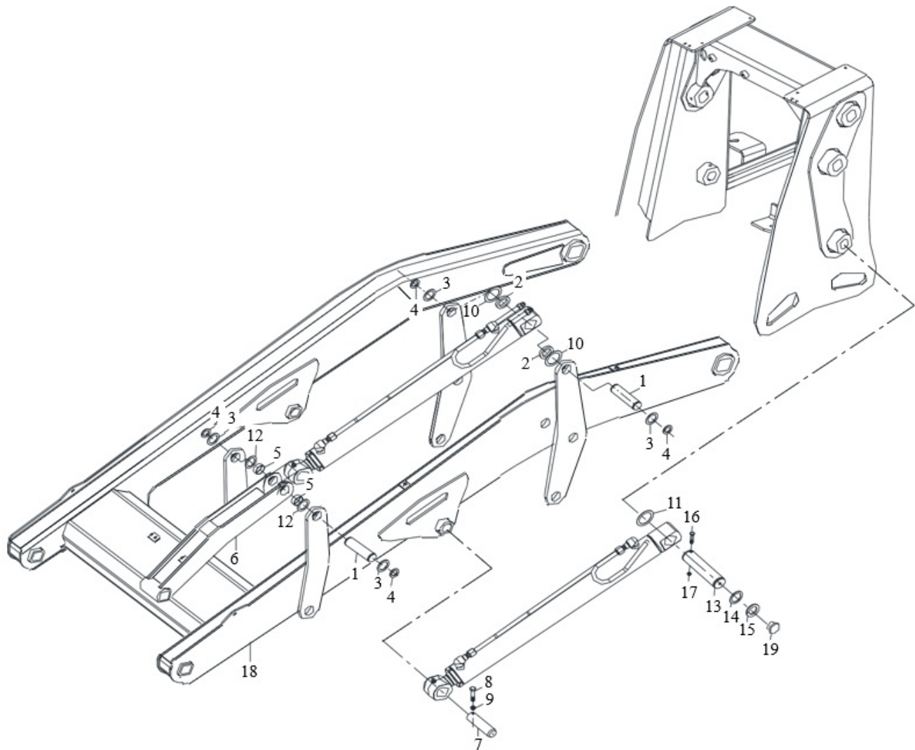
Рис. 69. Соединение стрелы и гидроцилиндра погрузчика
