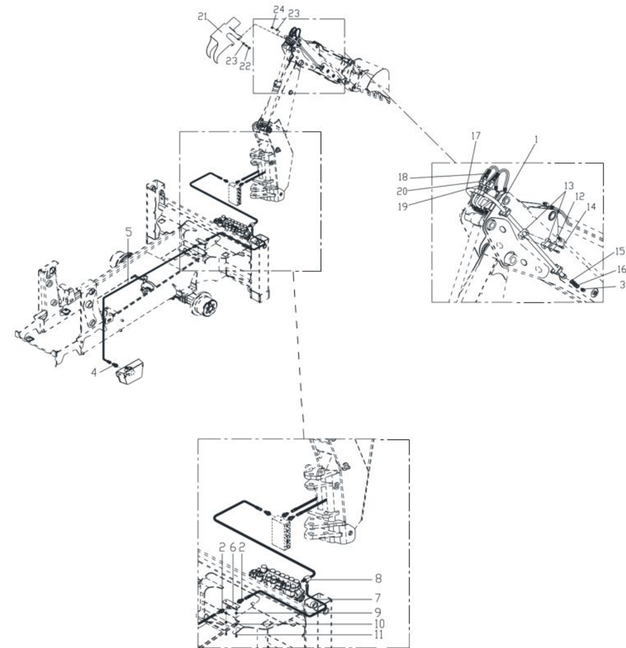
Рис. 74. Гидросистема универсального разъема высокого давления (модификация с телескопом)
