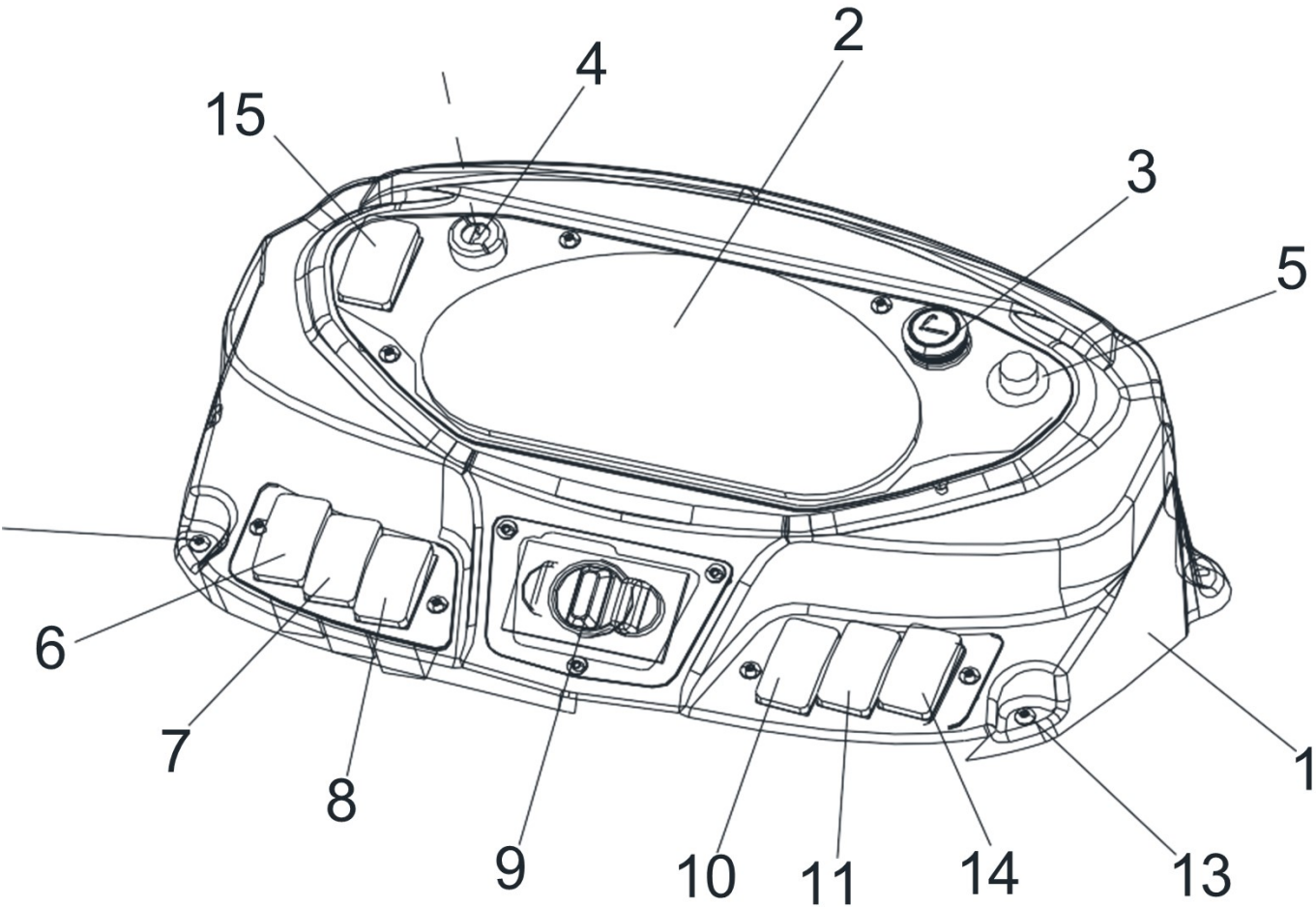
Рис. 35. Боковая консоль
