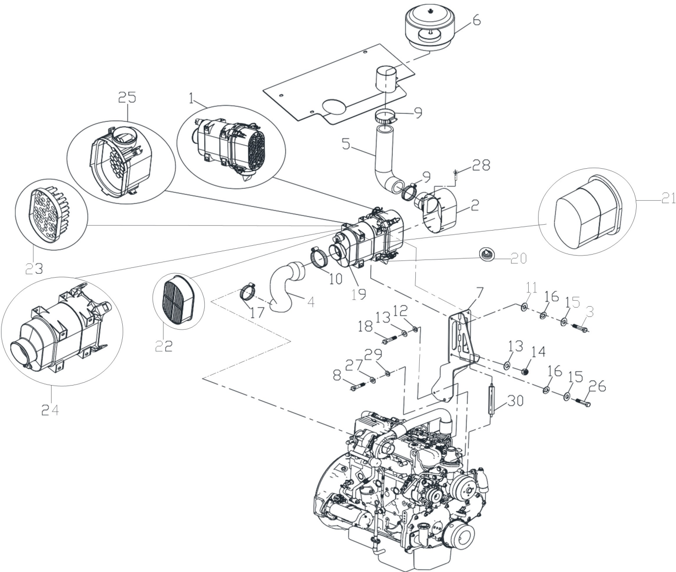
Рис. 12. Система впуска воздуха
