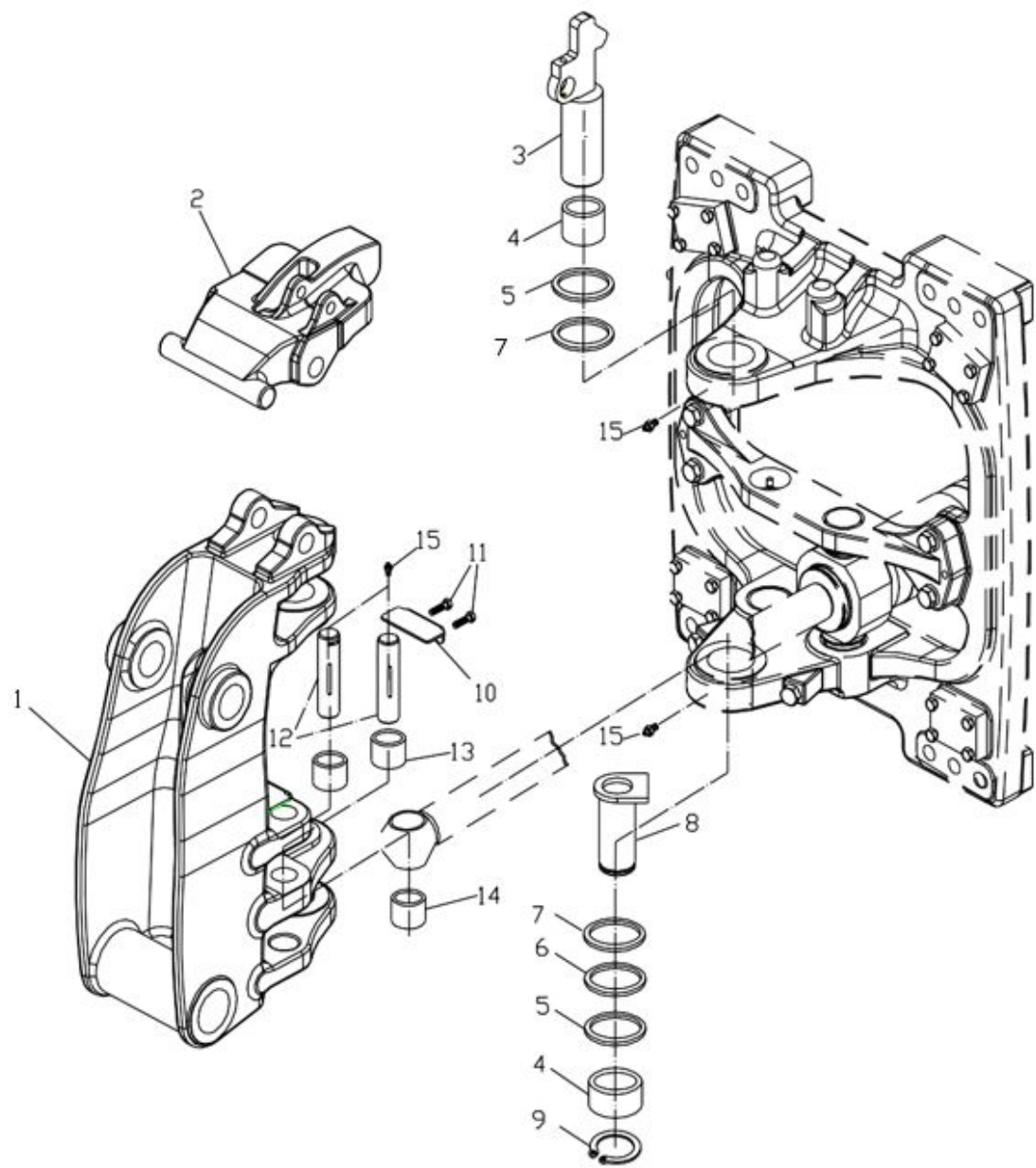
Рис. 86. Шарнир поворотного узла стрелы экскаватора
