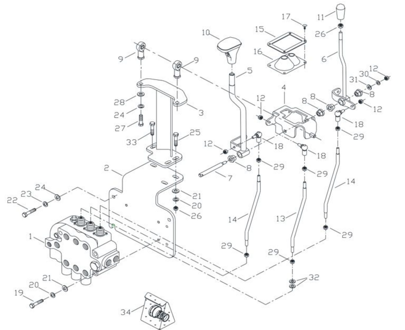
Рис. 23. Гидрораспределитель погрузчика с ковшом 6 в 1
