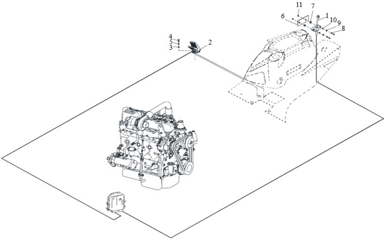
Рис. 3. Ручной дроссель и педаль акселератора
