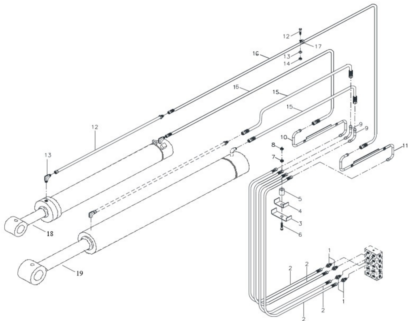
Рис. 77. Гидросистема ковша экскаватора (модификация с телескопом)
