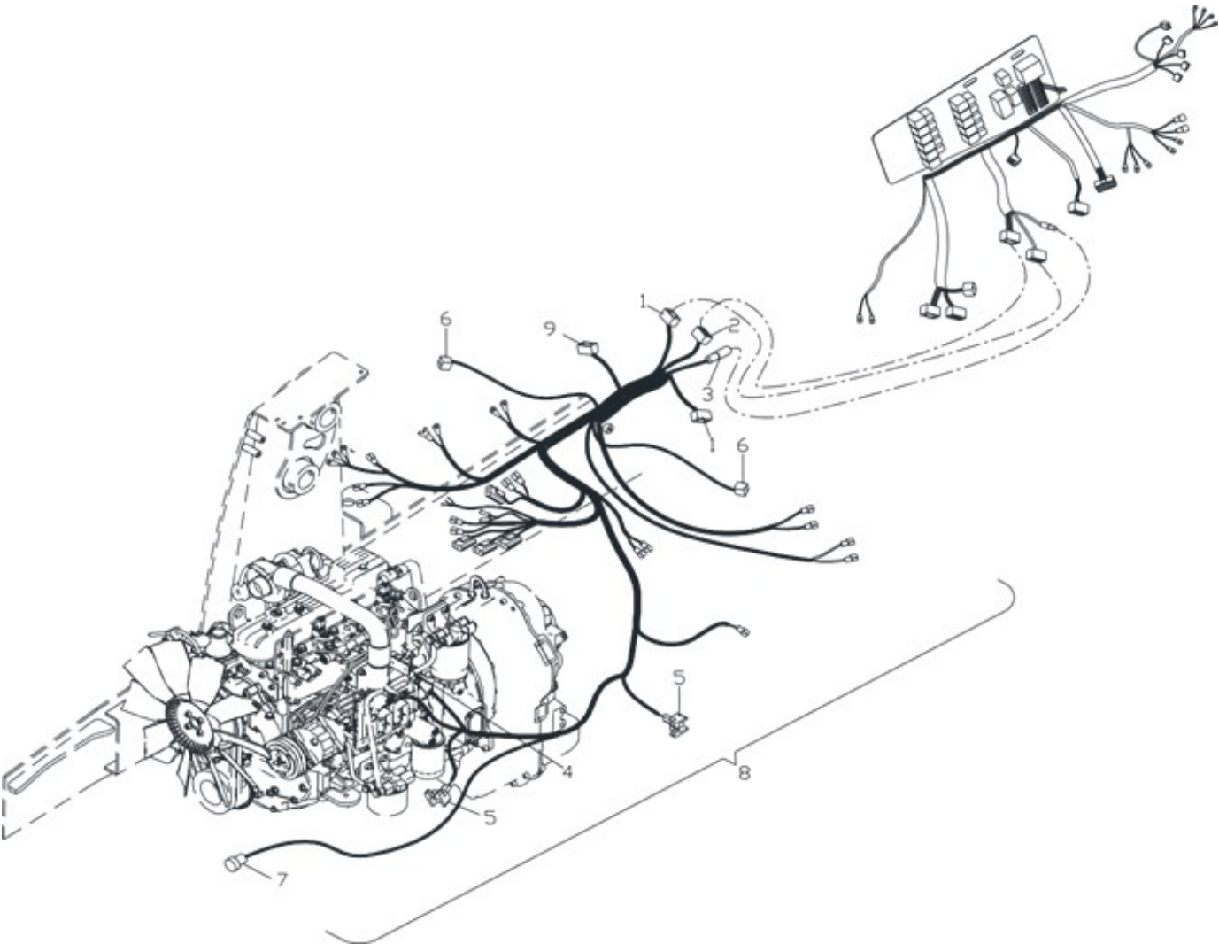
Рис. 39. Группа электропроводки двигателя (1)
