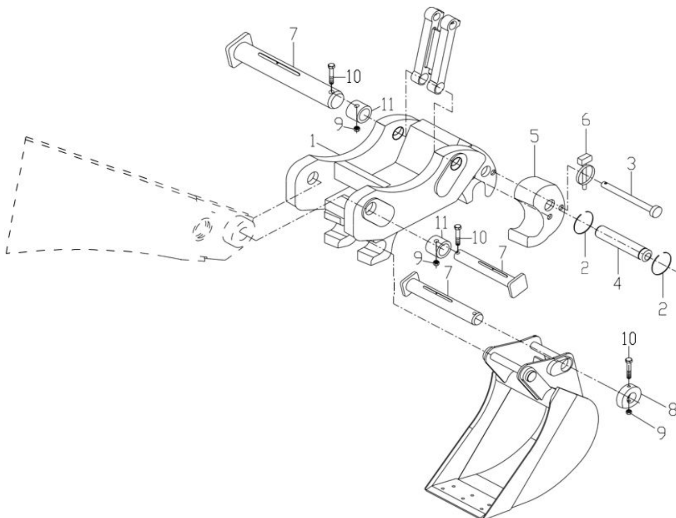
Рис. 75. Быстросъемное устройство ковша экскаватора
