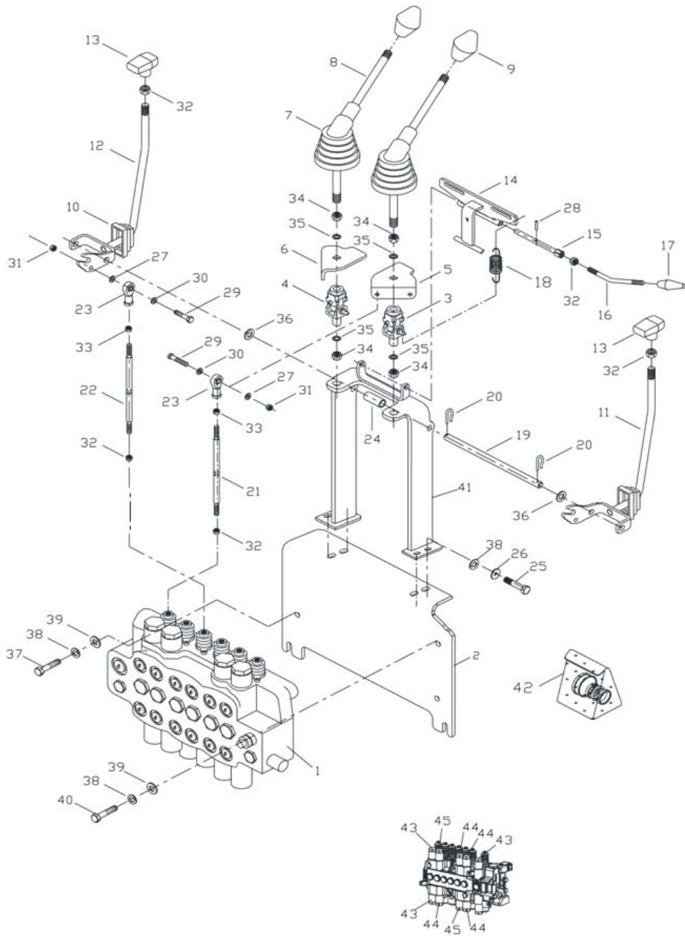
Рис. 24. Гидрораспределитель управления экскаваторным оборудованием
