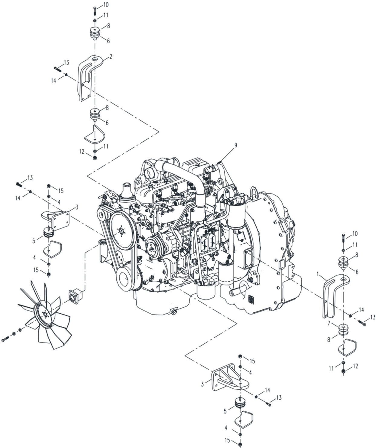
Рис. 2. Двигатель с креплением
