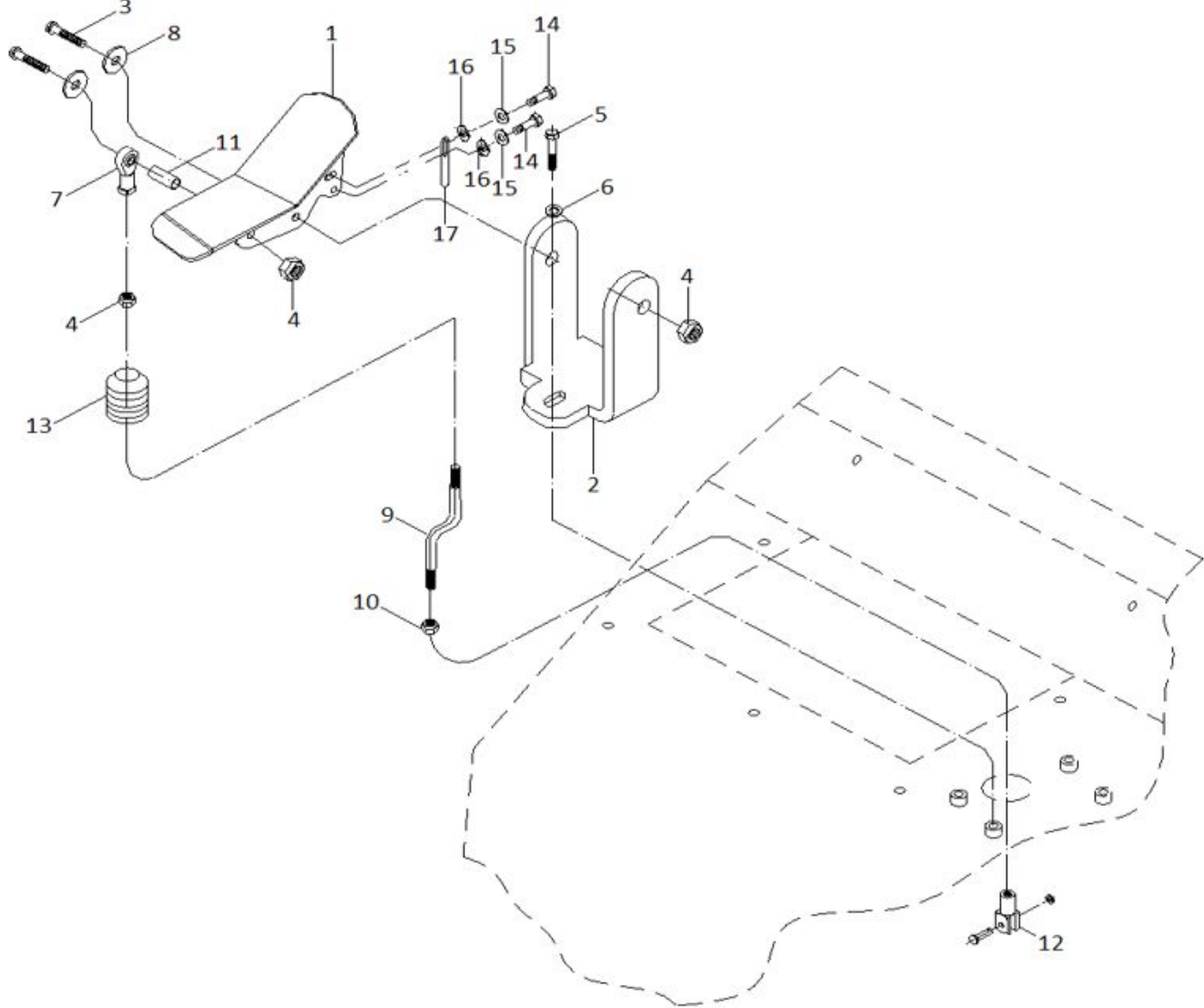
Рис. 59. Педаль телескопа в сборе
