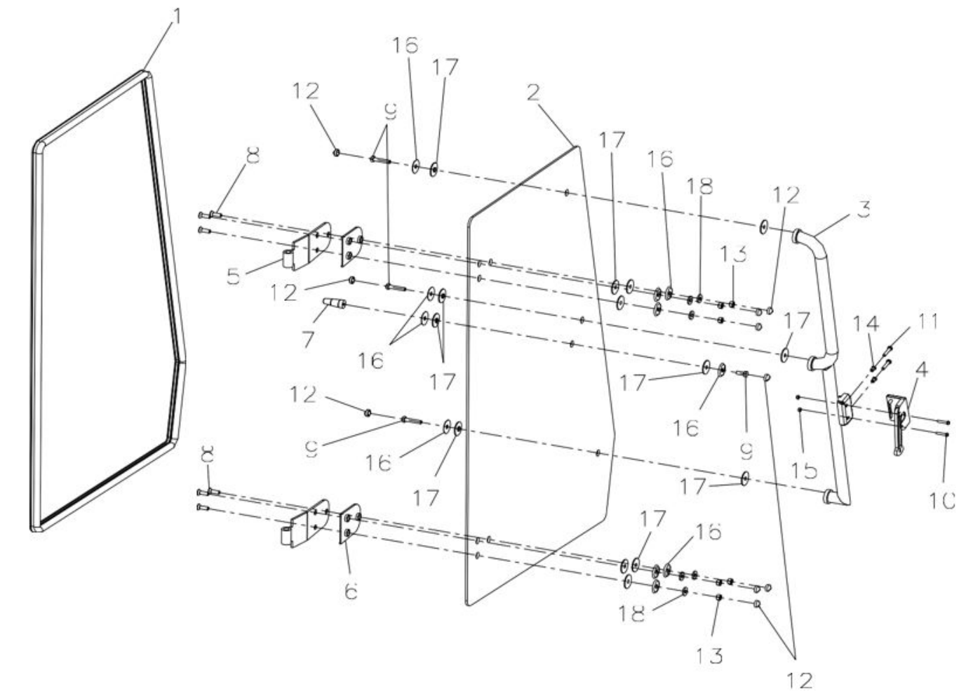
Рис. 52. Правое окно в сборе
