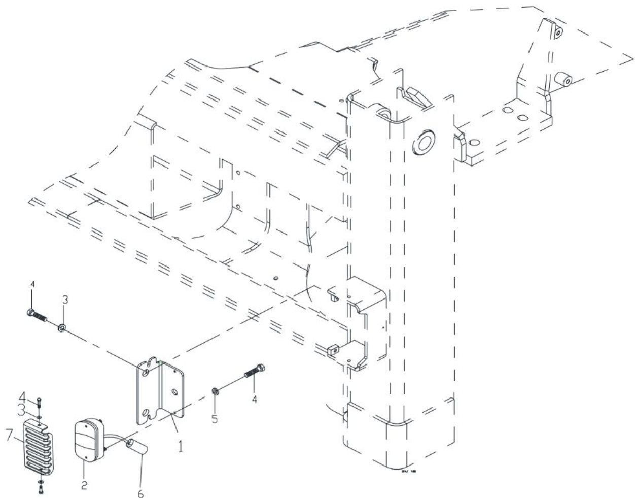
Рис. 43. Задний стоп-сигнал
