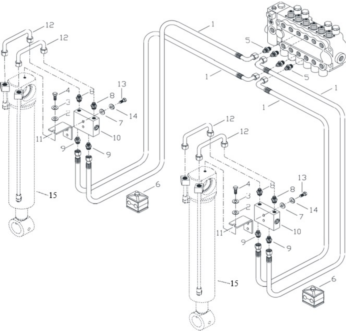
Рис. 72. Гидравлическая система аутригеров
