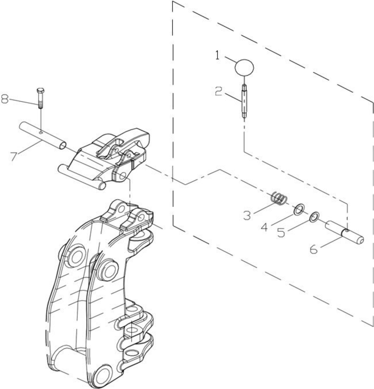
Рис. 81. Запирающий механизм поворотного узла стрелы экскаватора
