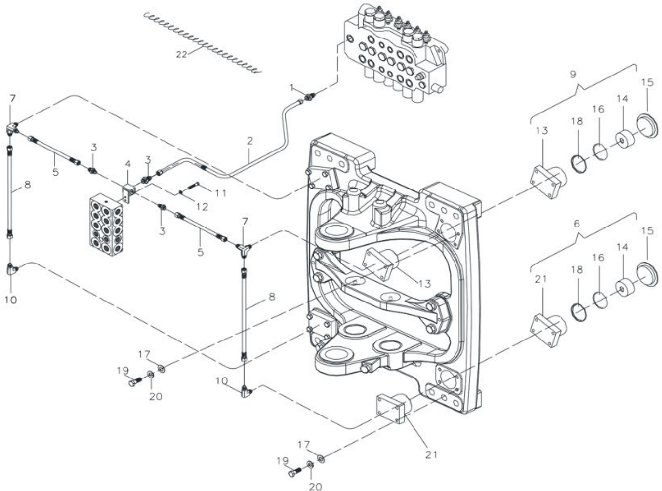
Рис. 76. Гидросистема блокировки каретки экскаватора
