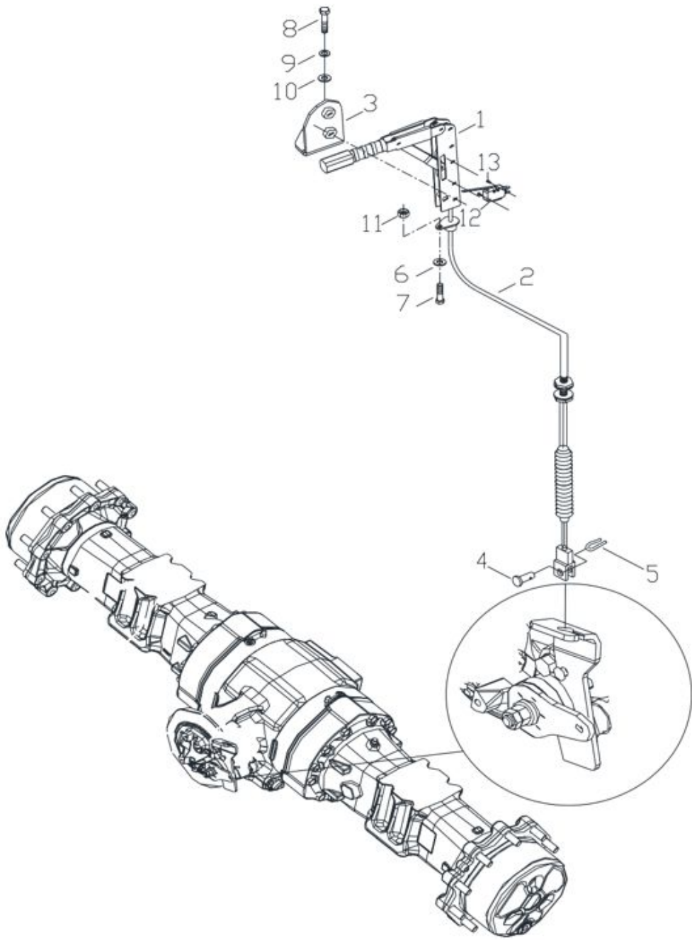
Рис. 33. Стояночная тормозная система
