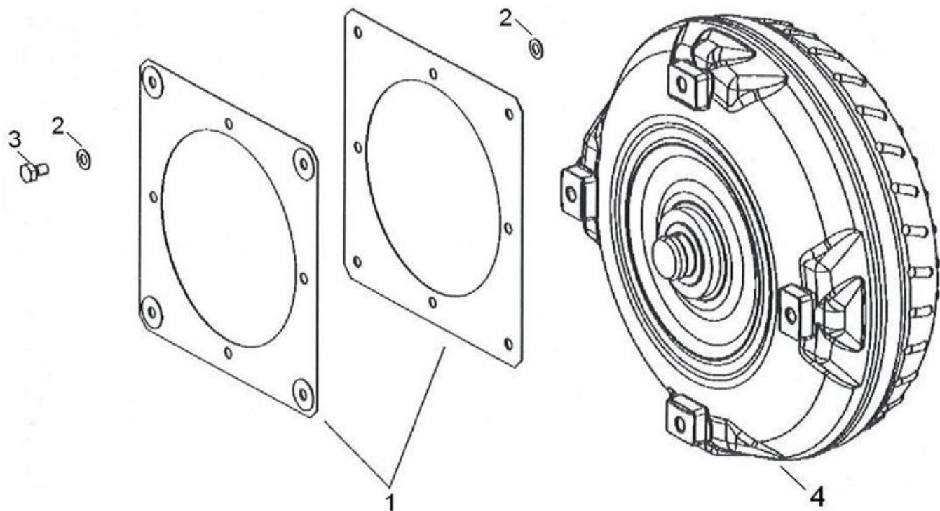
Рис. 6. Гидротрансформатор в сборе
