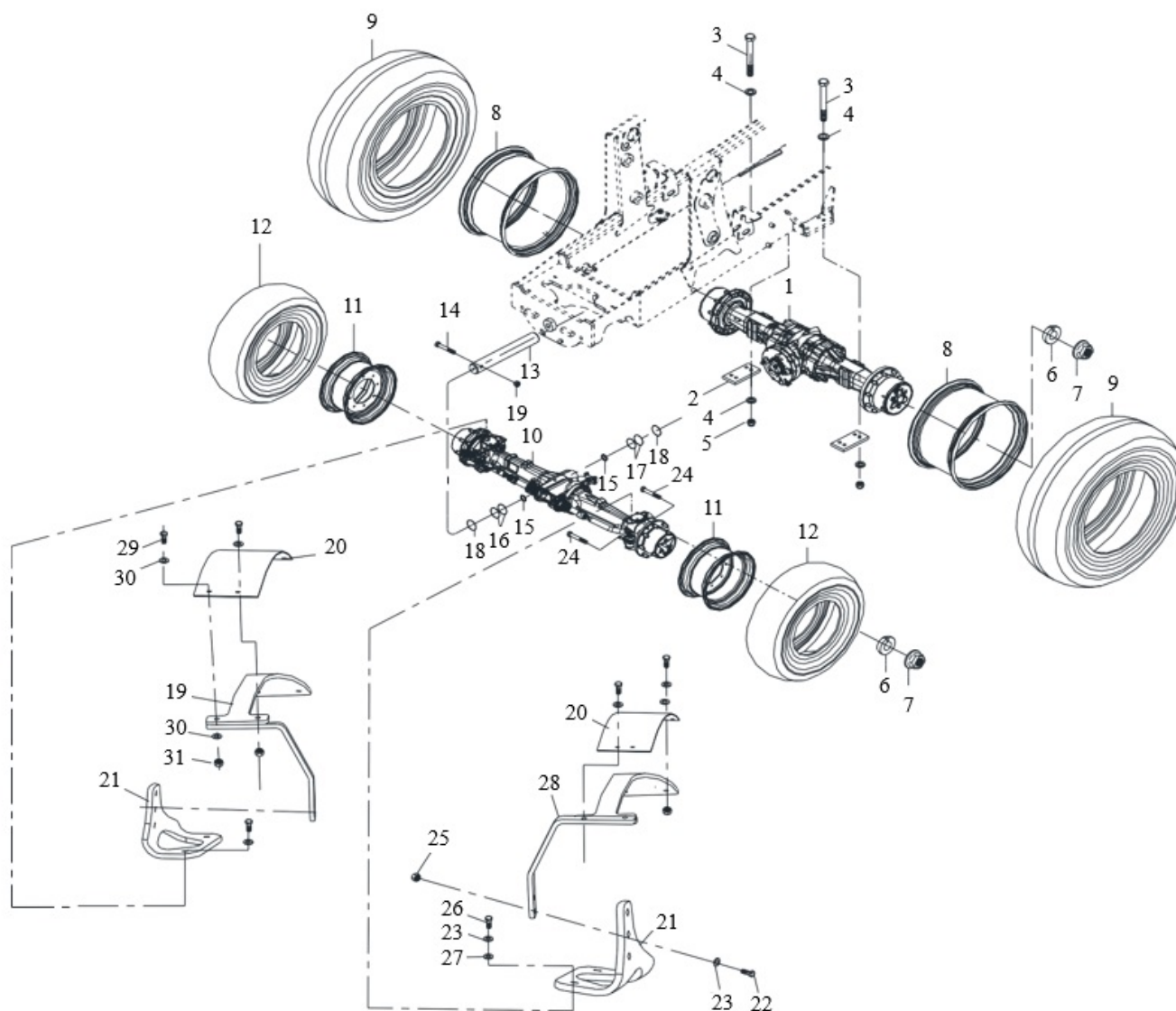
Рис. 21. Крепление колесных мостов и колес
