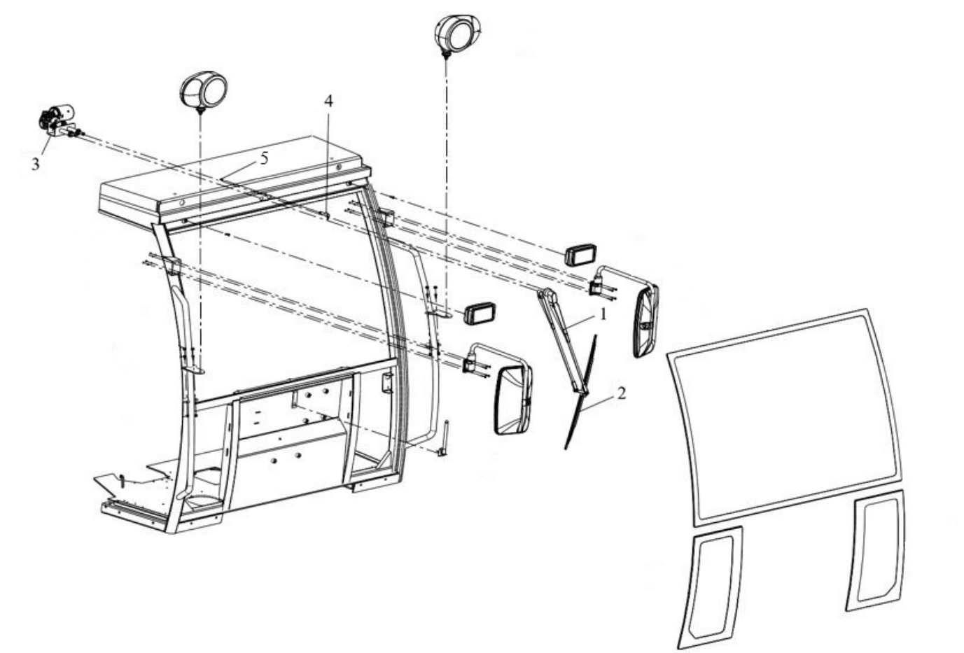
Рис. 54. Дворник лобового стекла в сборе
