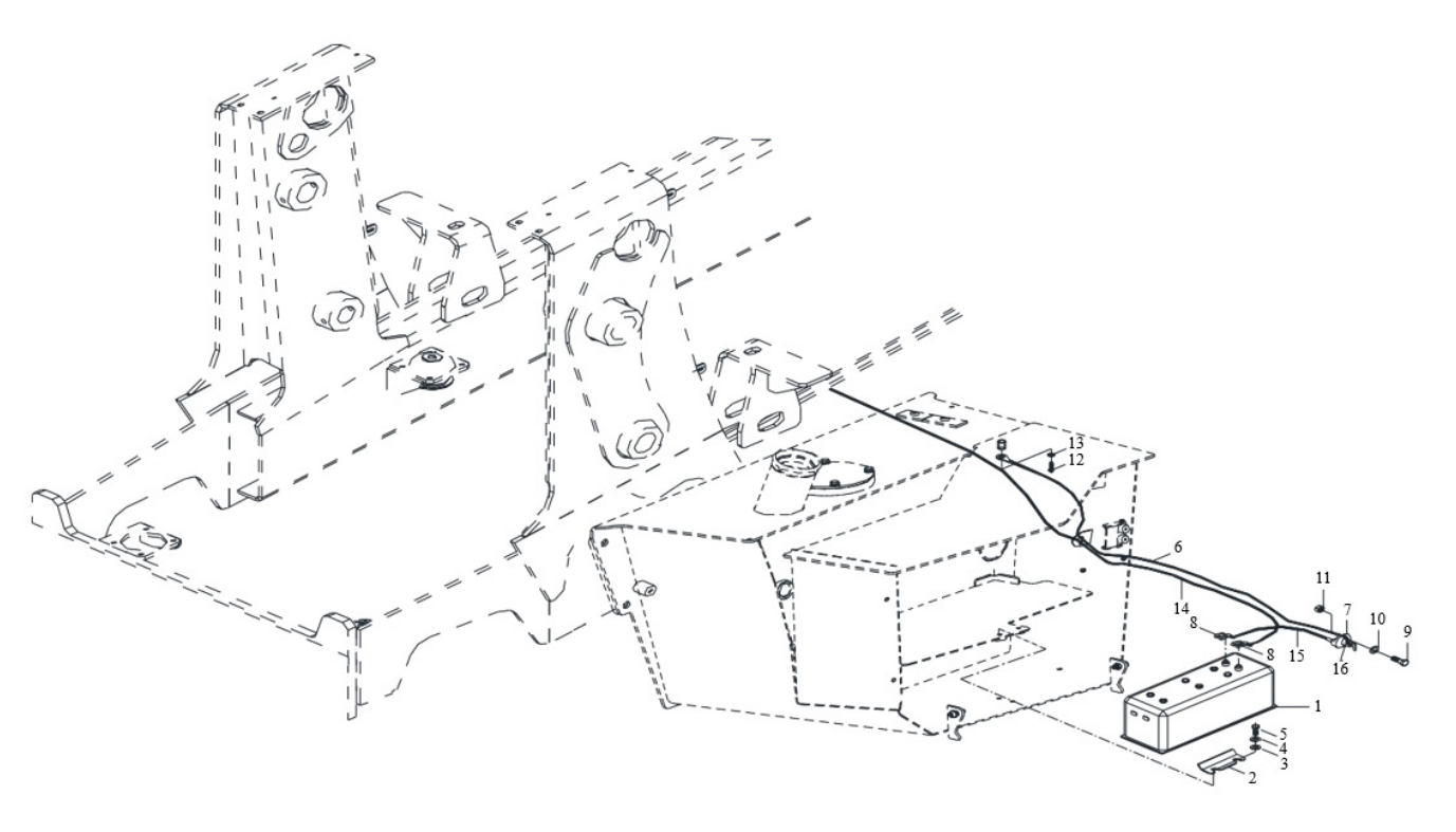
Рис. 41. Аккумулятор и его соединения
