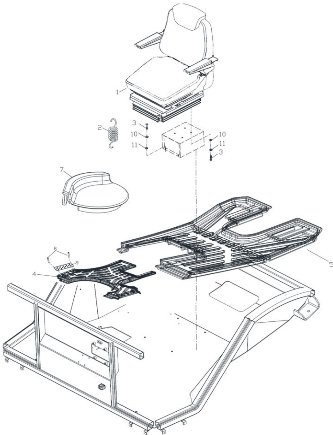
Рис. 46. Установка сиденья и элементов пола
