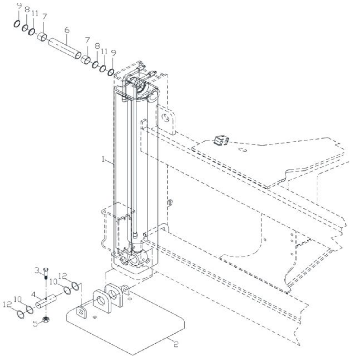
Рис. 73. Опора аутригера в сборе
