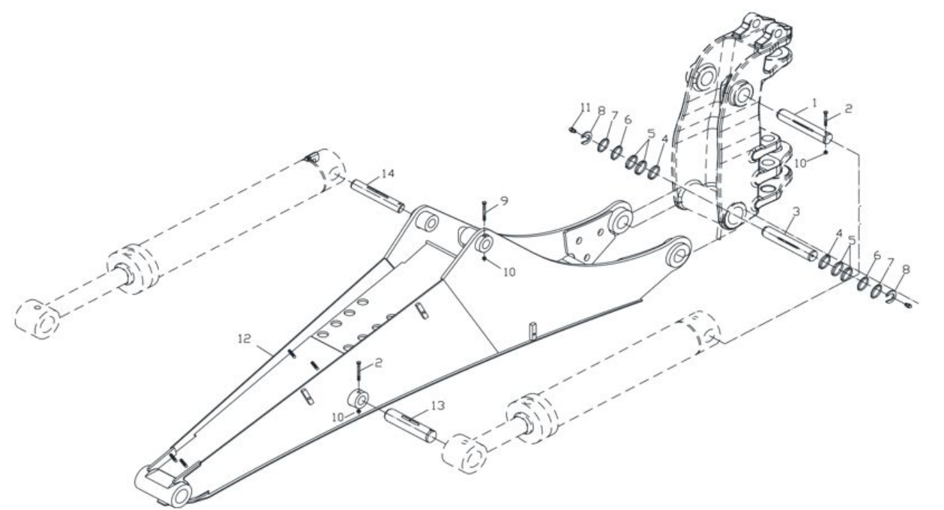
Рис. 84. Стрела экскаватора в сборе
