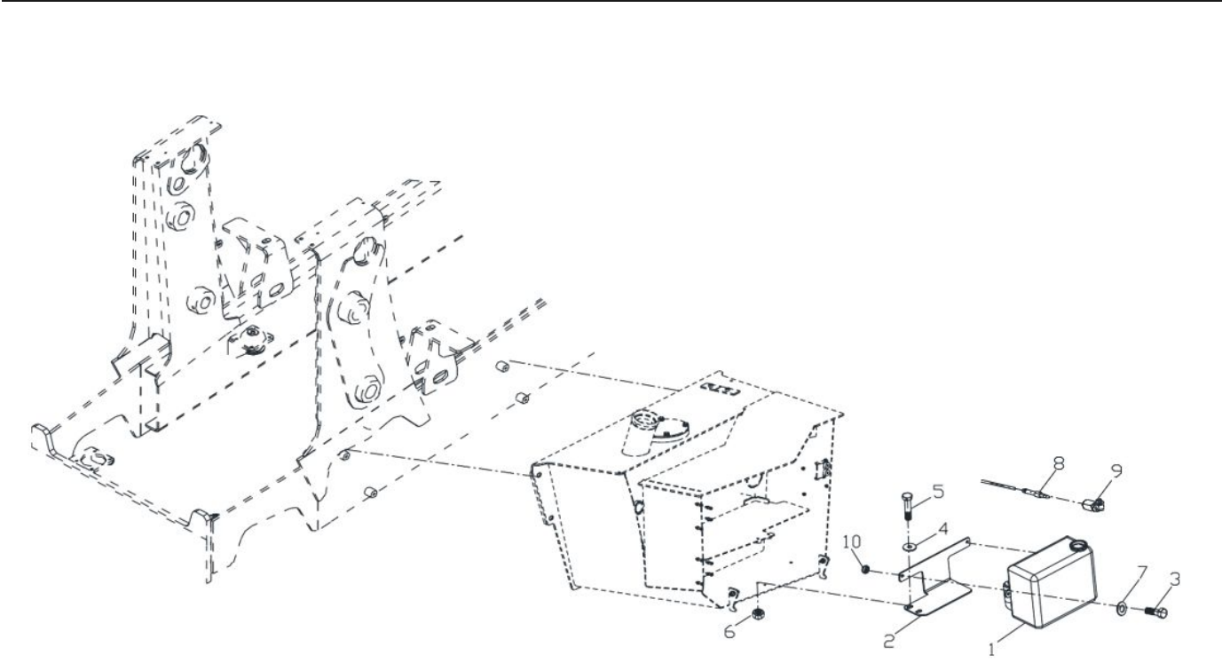
Рис. 53. Бачок омывателя лобового стекла
