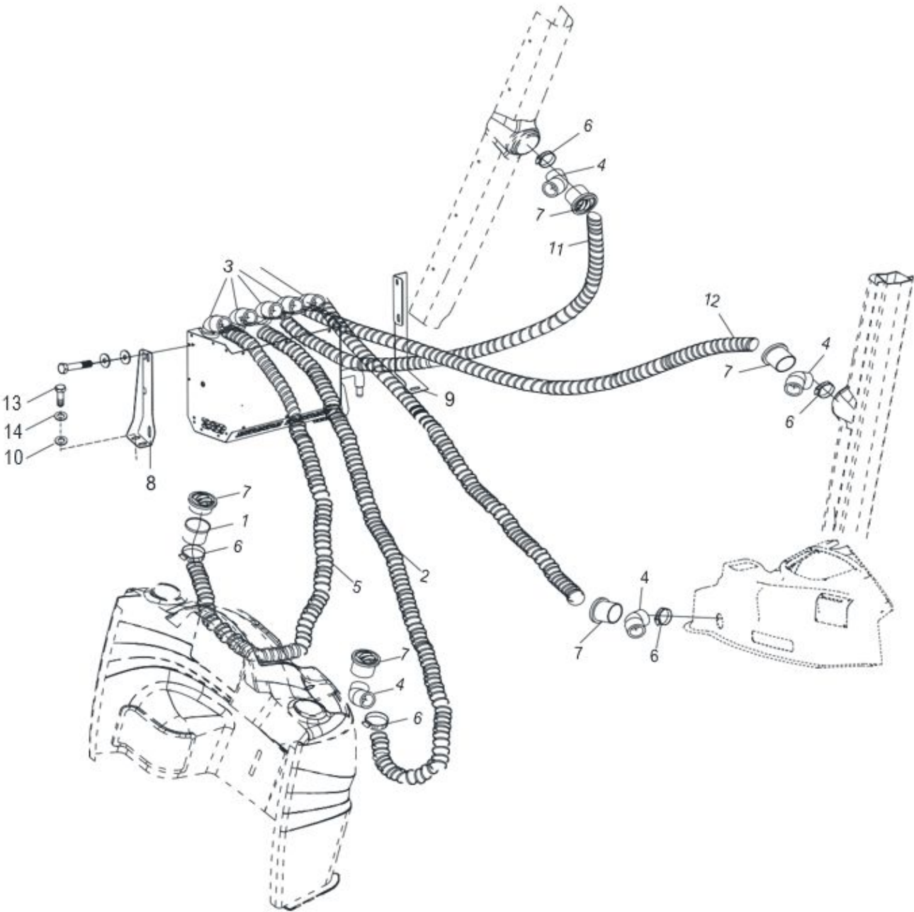
Рис. 55. Комплект воздухопроводов
