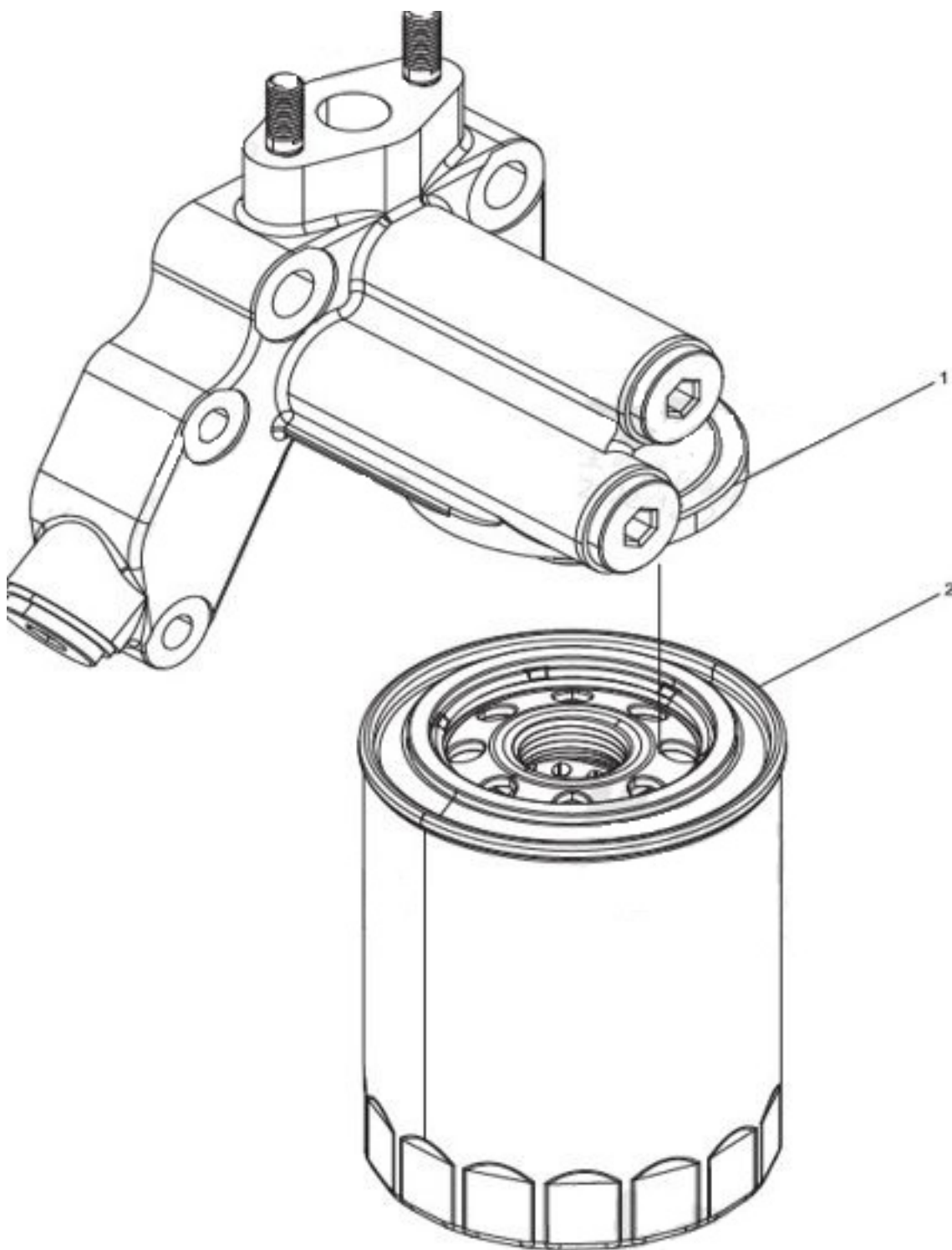
Рис. 4. Установка масляного фильтра
