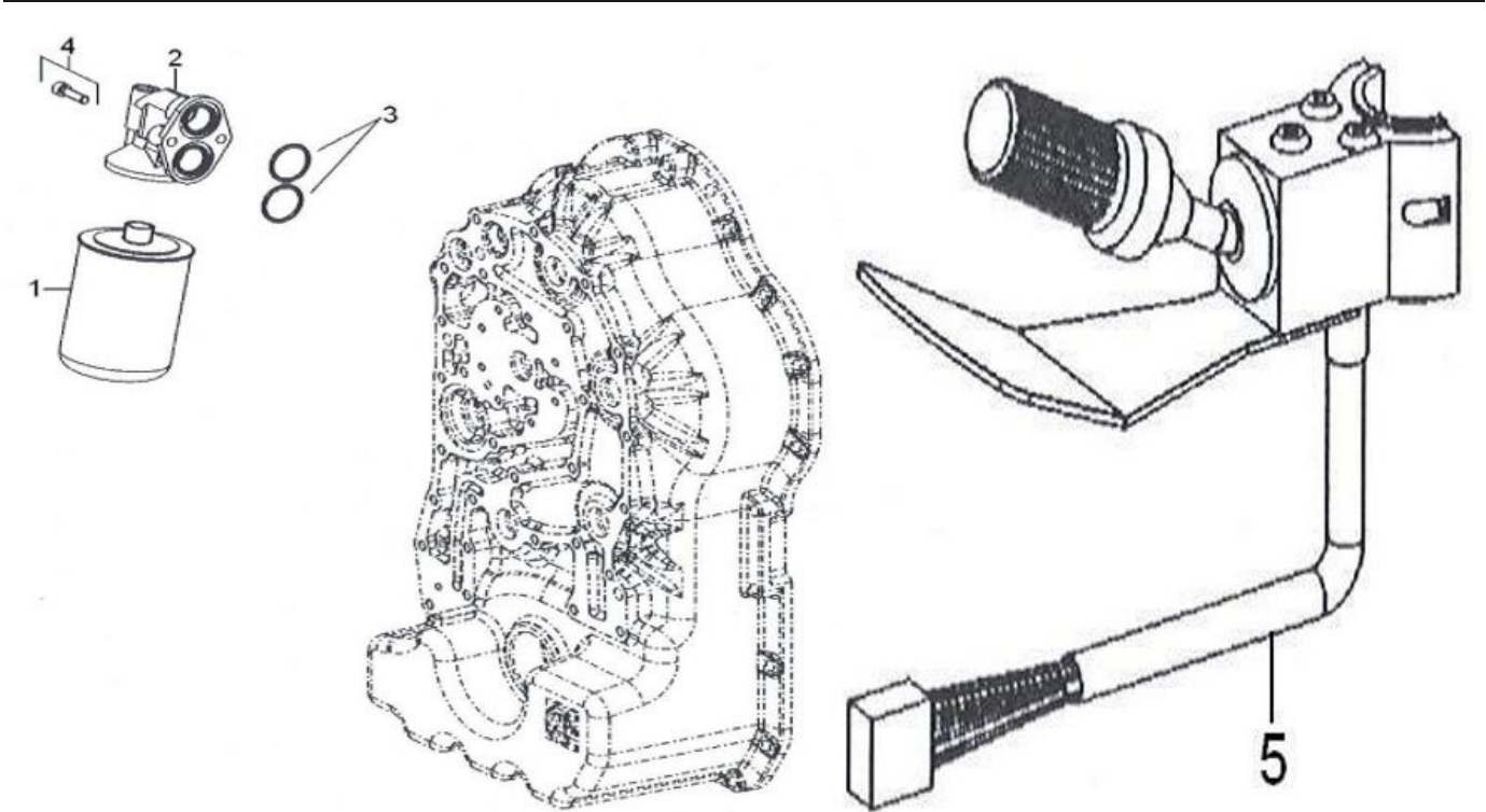
Рис. 8. Сборка масляного фильтра КПП
