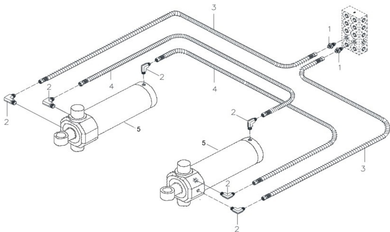
Рис. 78. Гидросистема поворота каретки экскаватора
