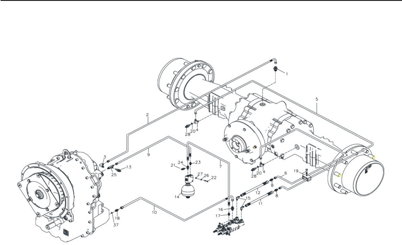
Рис. 34. Элементы тормозной системы
