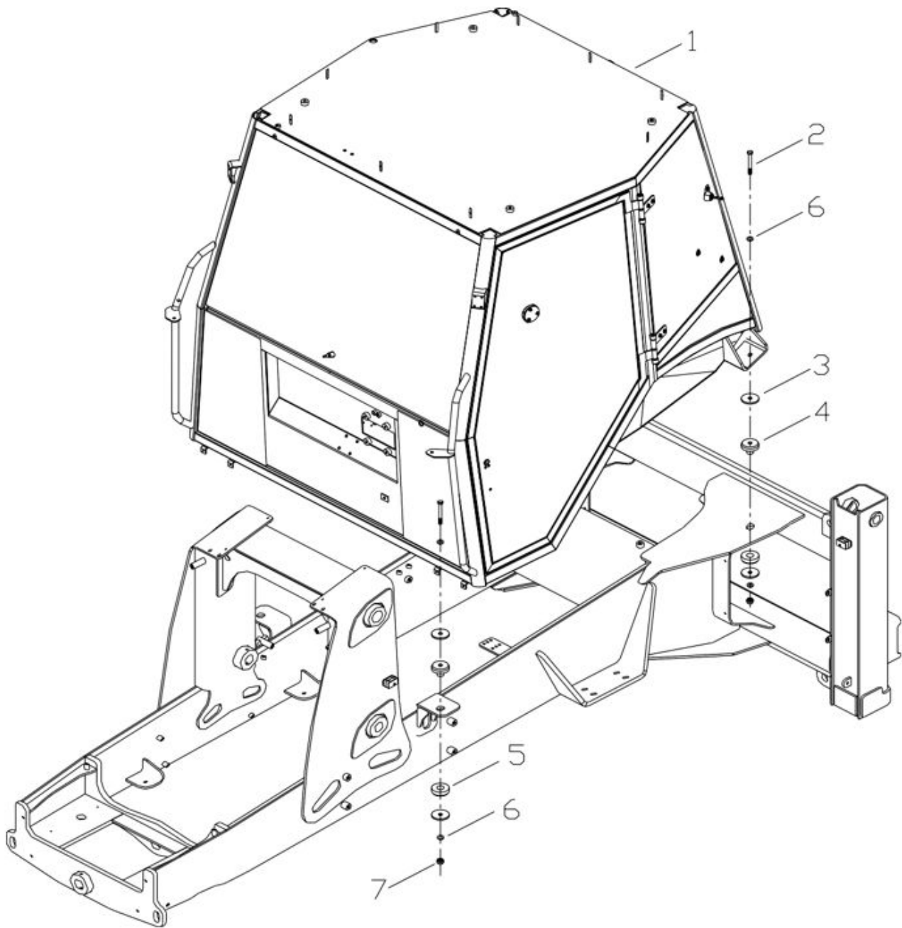
Рис. 45. Крепление кабины
