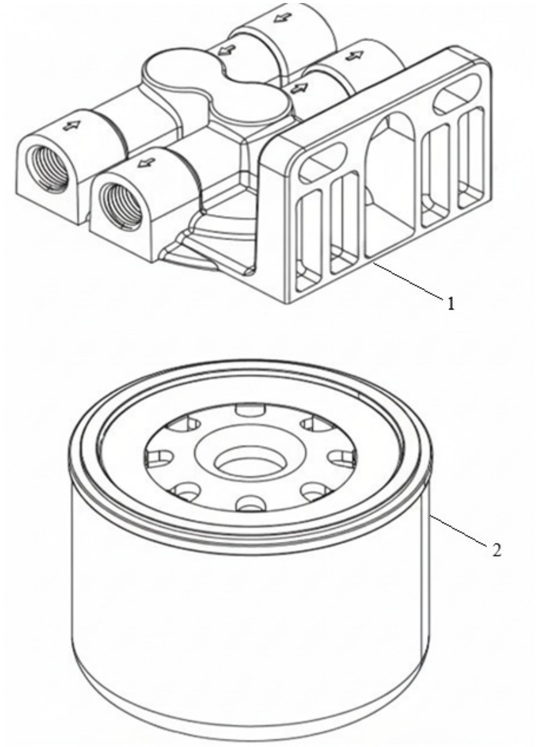
Рис. 18. Установка топливного фильтра тонкой очистки
