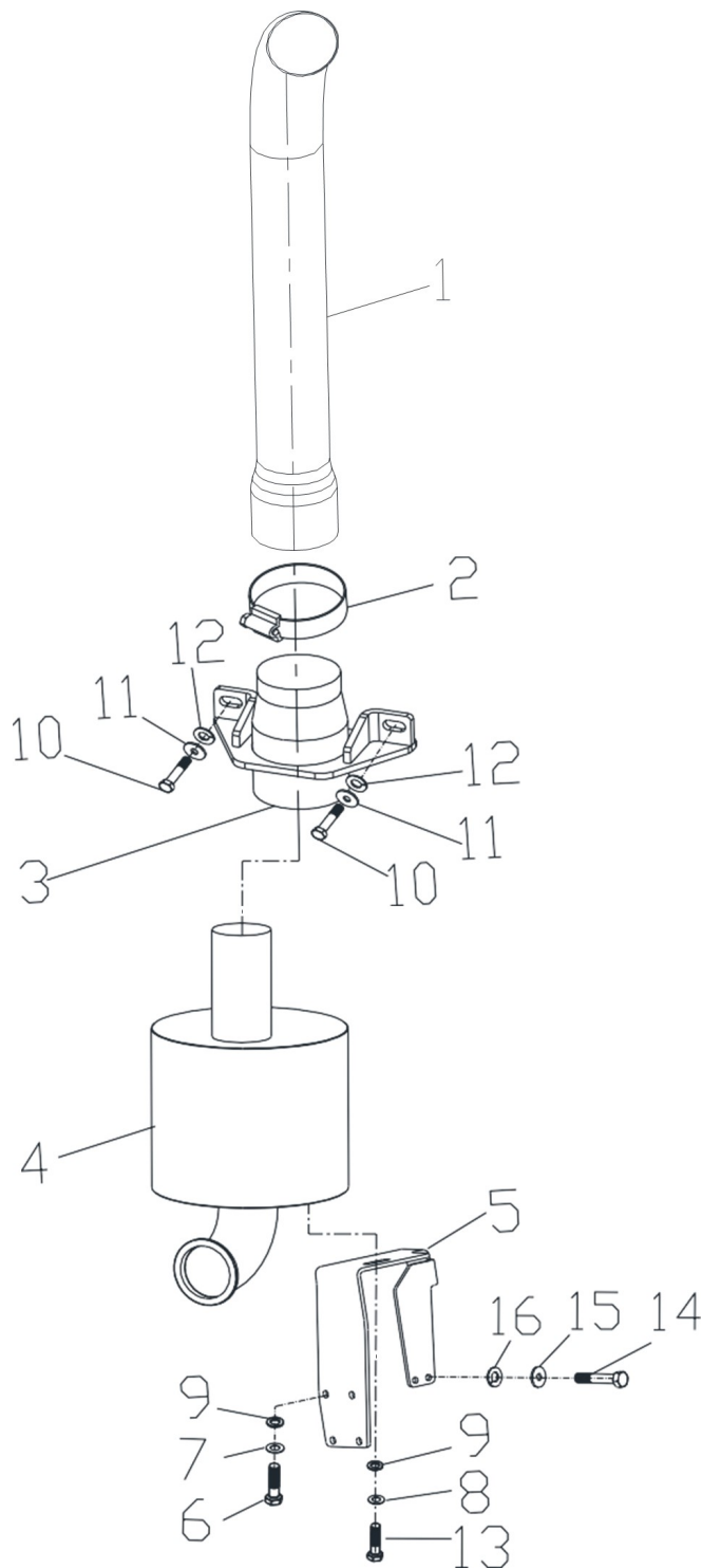
Рис. 13. Система выпуска воздуха
