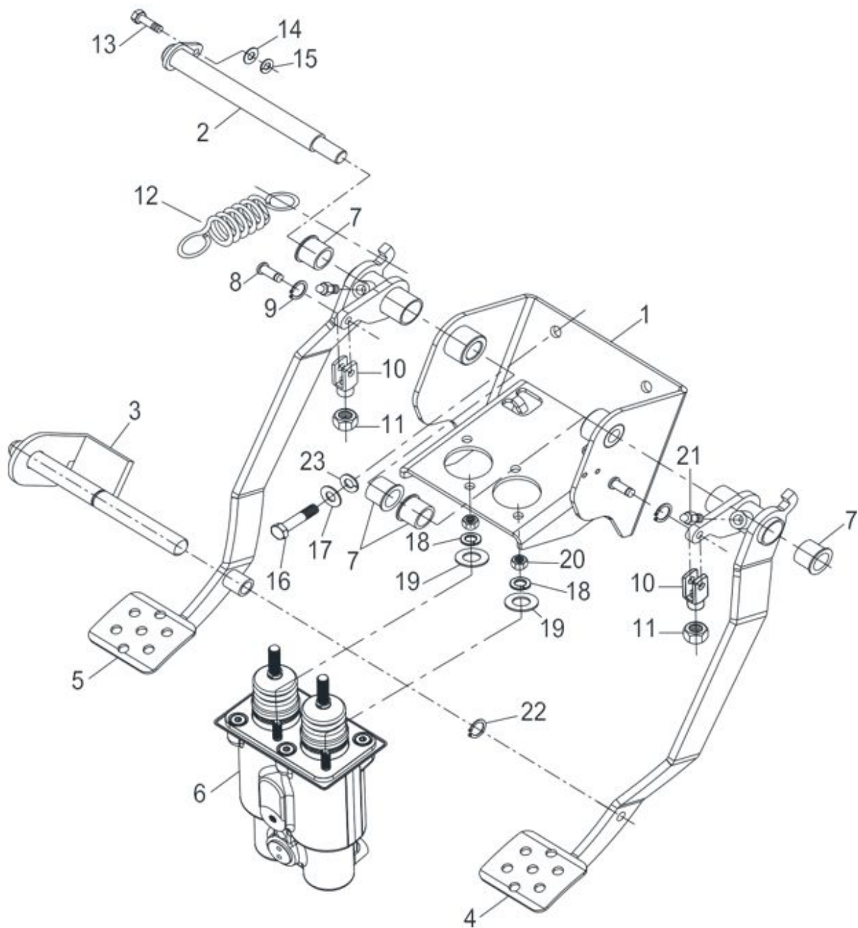
Рис. 32. Педаль тормоза в сборе
