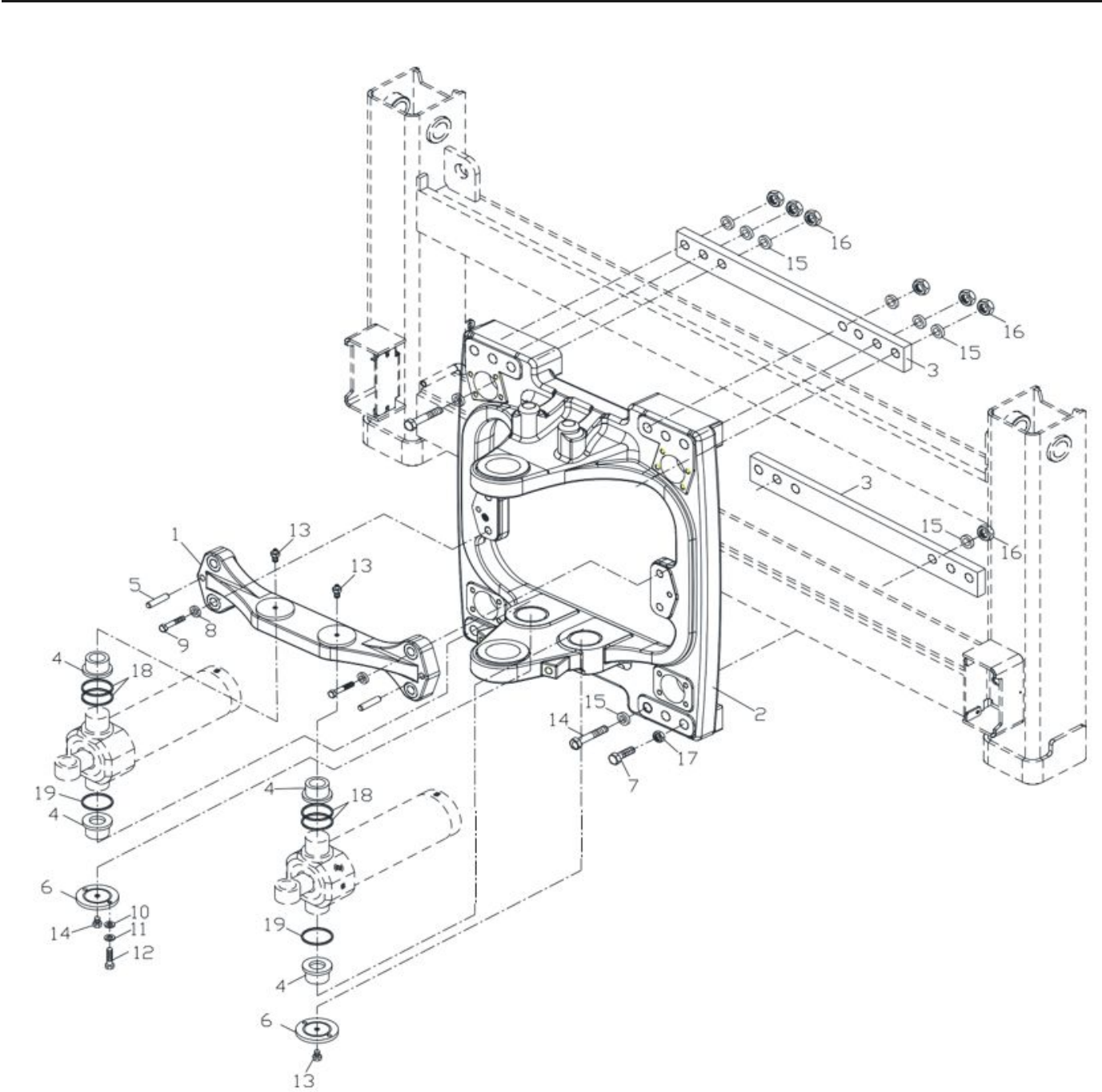
Рис. 82. Каретка бокового смещения поворотного механизма стрелы экскаватора в сборе
