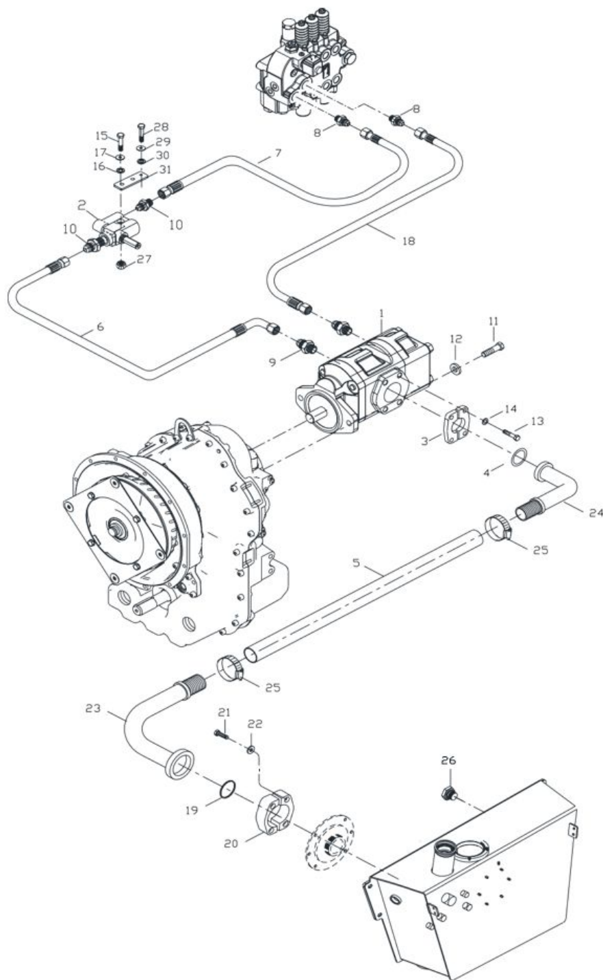
Рис. 26. Контур гидравлического насоса
