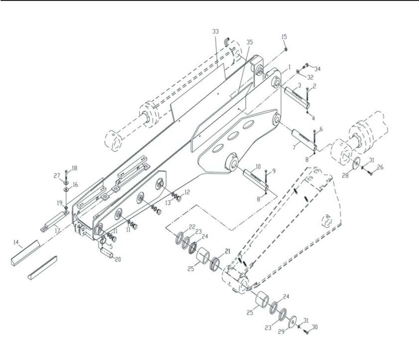
Рис. 83. Рукоять экскаватора в сборе (модификация с телескопом)
