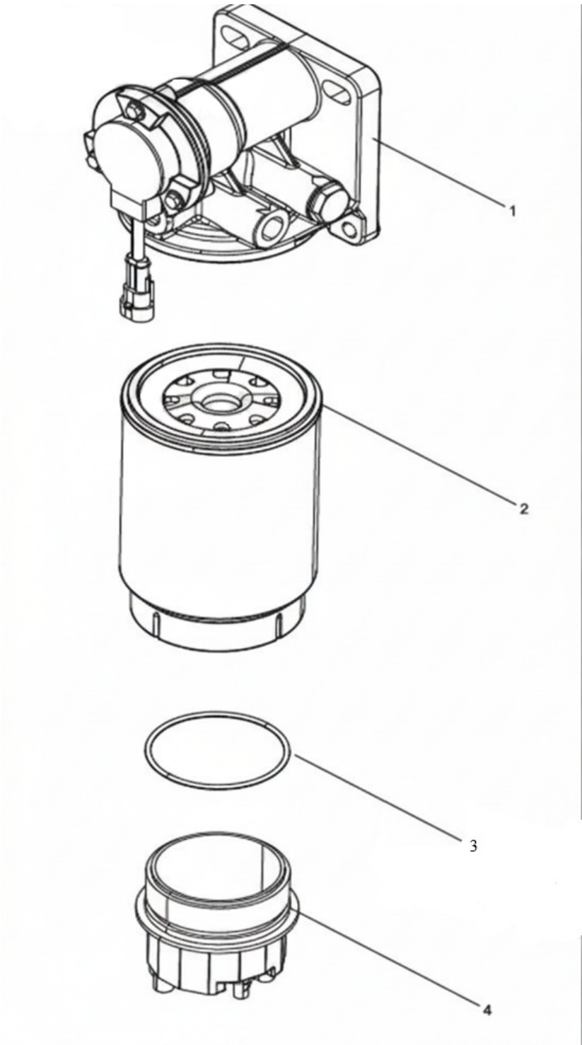
Рис. 16. Топливный насос в сборе
