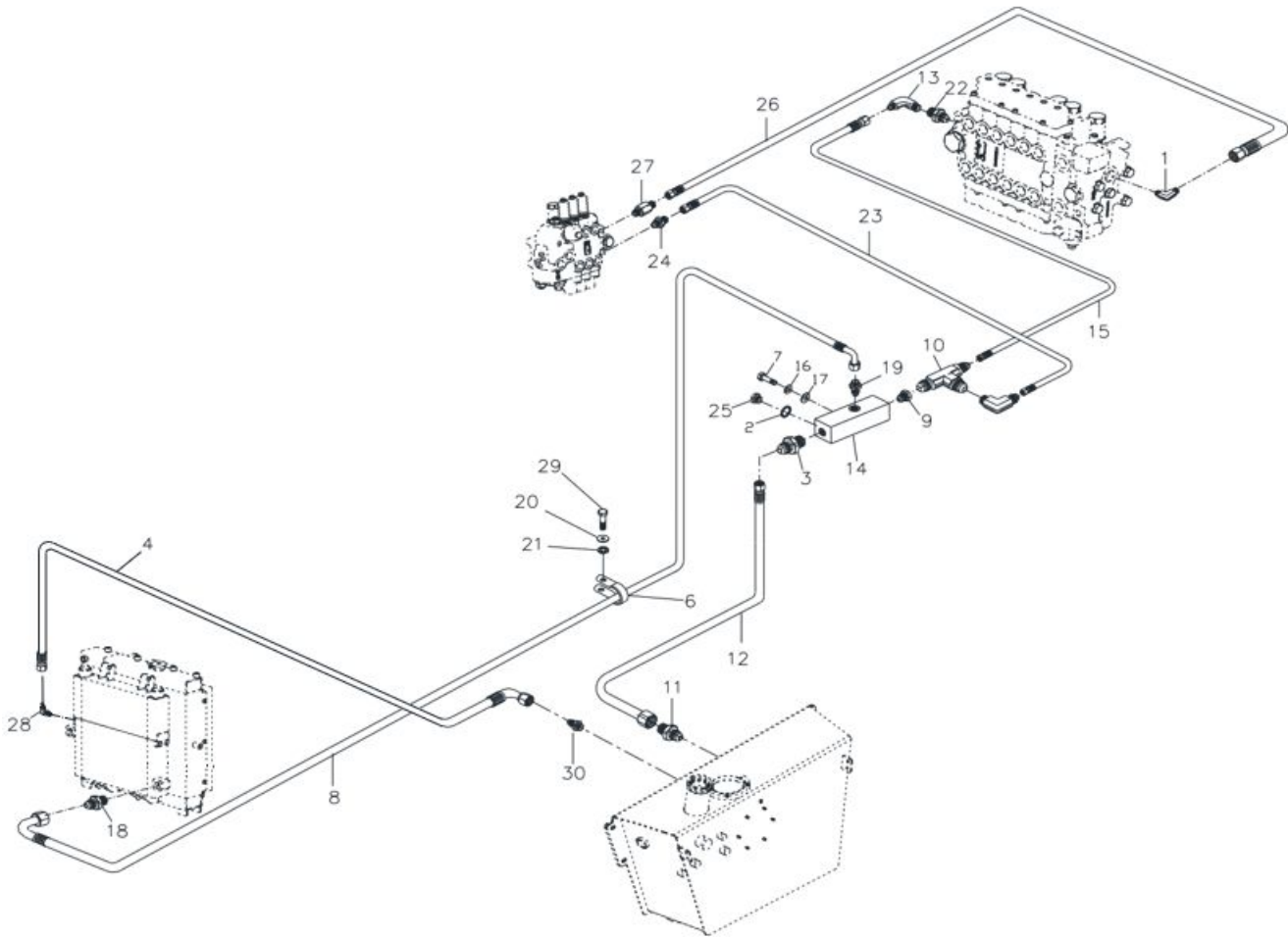
Рис. 25. Контур блока сбора утечек
