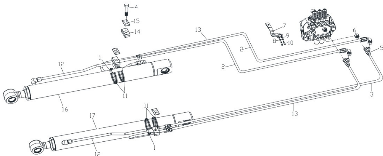
Рис. 67. Гидросистема подъема стрелы погрузчика
