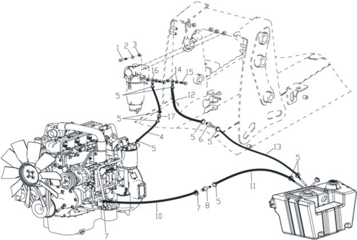
Рис. 14. Топливные шланги
