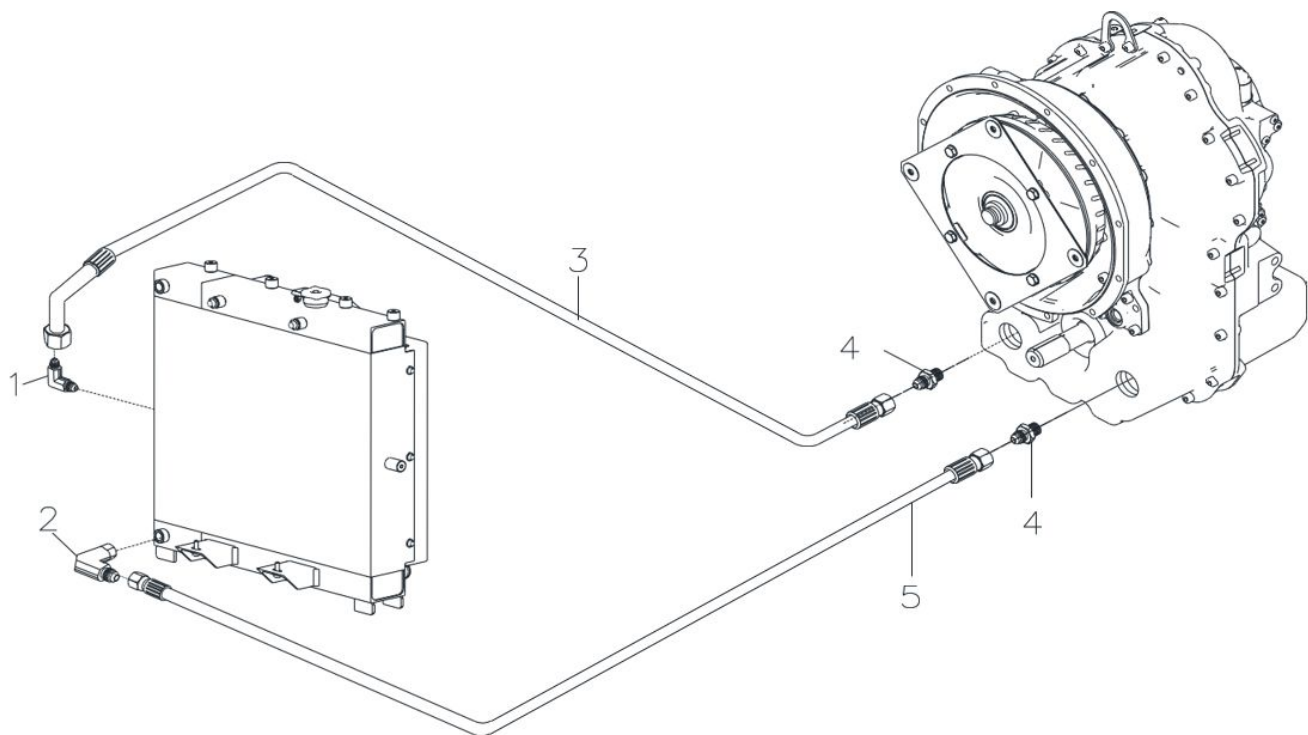
Рис. 11. Система охлаждения КПП
