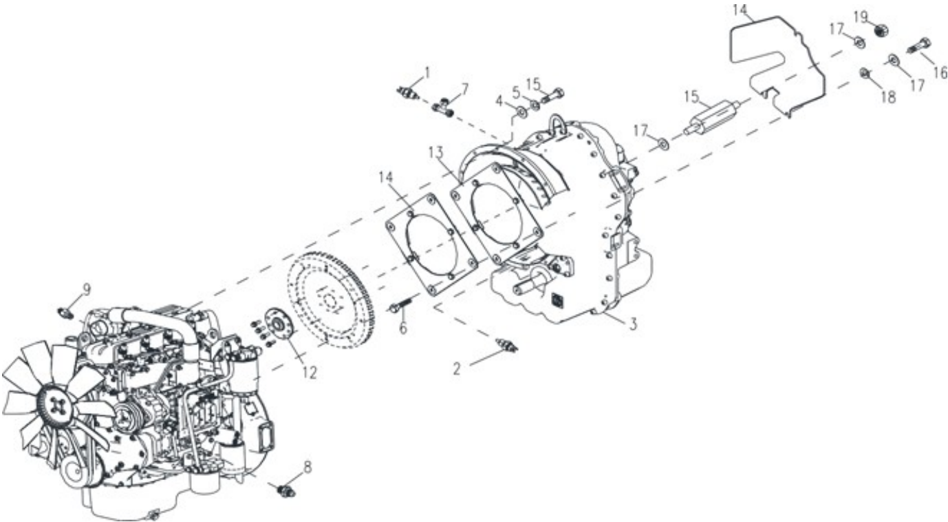
Рис. 7. КПП с креплением
