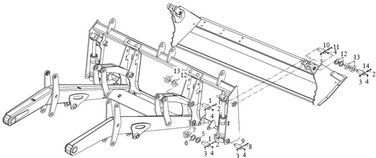
Рис. 68. Крепление откидного ковша погрузчика в сборе
