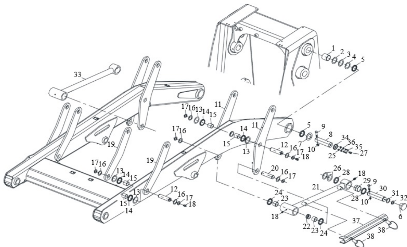
Рис. 70. Соединение стрелы и рычага погрузчика
