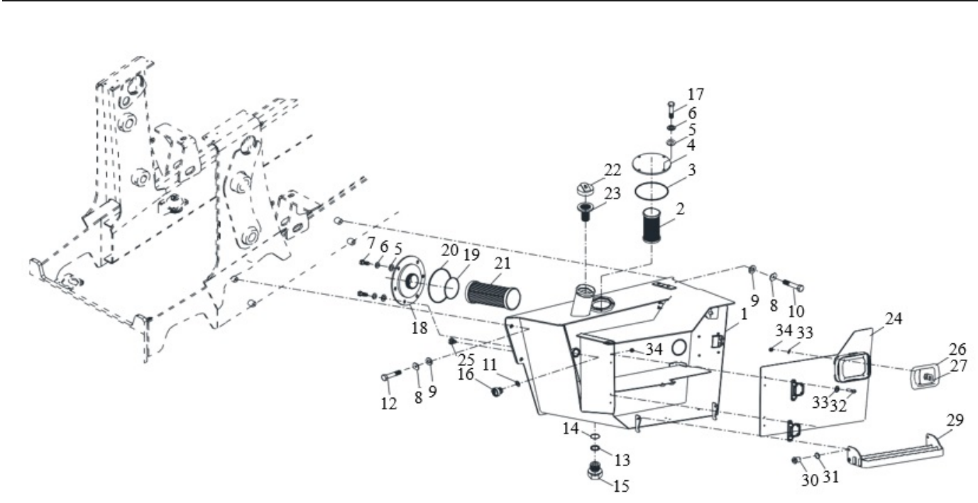
Рис. 30. Гидробак в сборе
