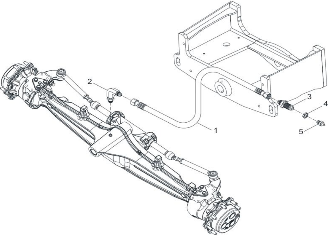
Рис. 22. Система смазки переднего моста
