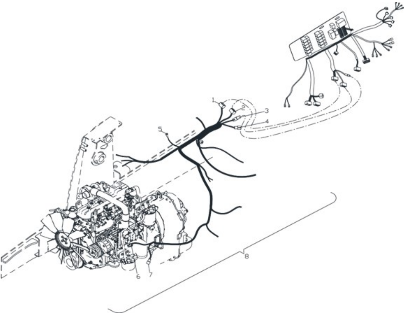
Рис. 40. Группа электропроводки двигателя (2)
