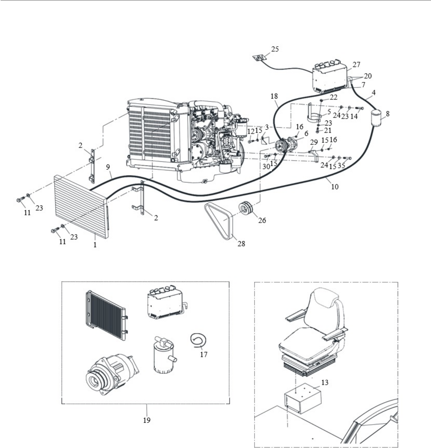
Рис. 56. Кондиционер, компрессор и радиатор в сборе
