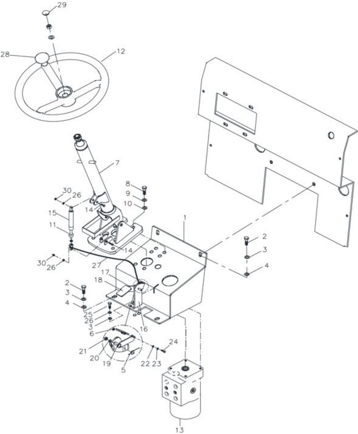
Рис. 60. Рулевая колонка в сборе
