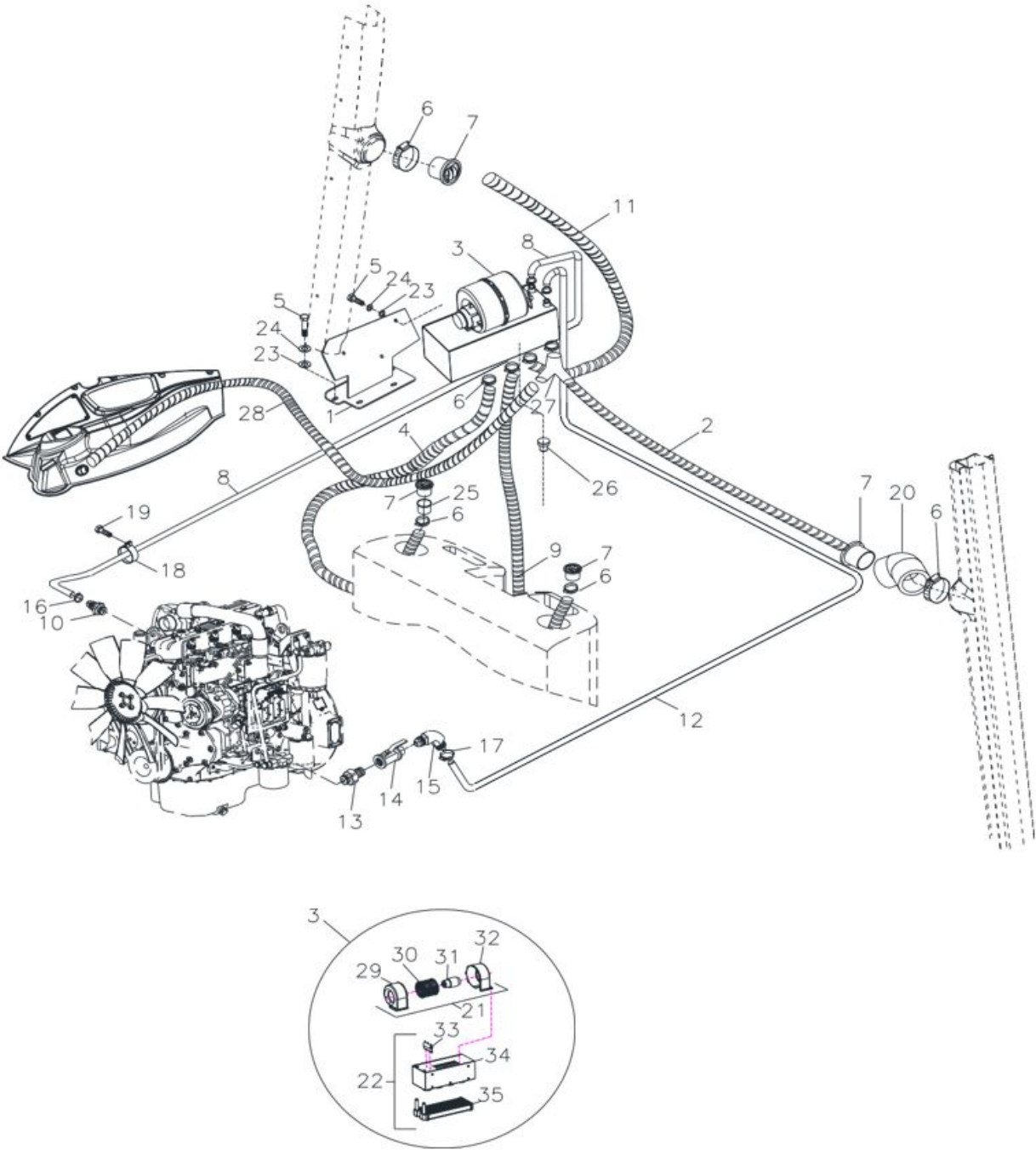
Рис. 57. Система обогрева воздуха и воздухопроводы (1)
