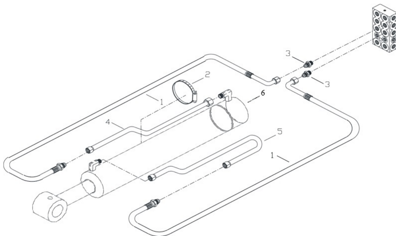
Рис. 80. Гидросистема стрелы экскаватора
