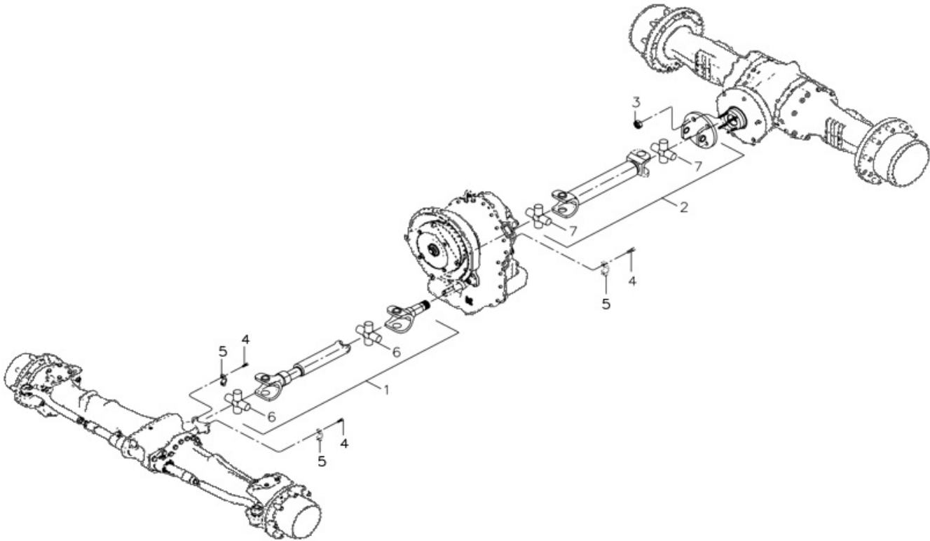
Рис. 9. Приводы мостов в сборе
