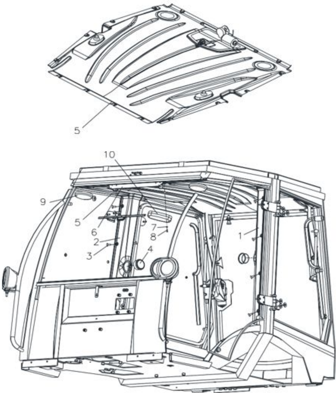
Рис. 63. Крыша и внутренние навесные элементы
