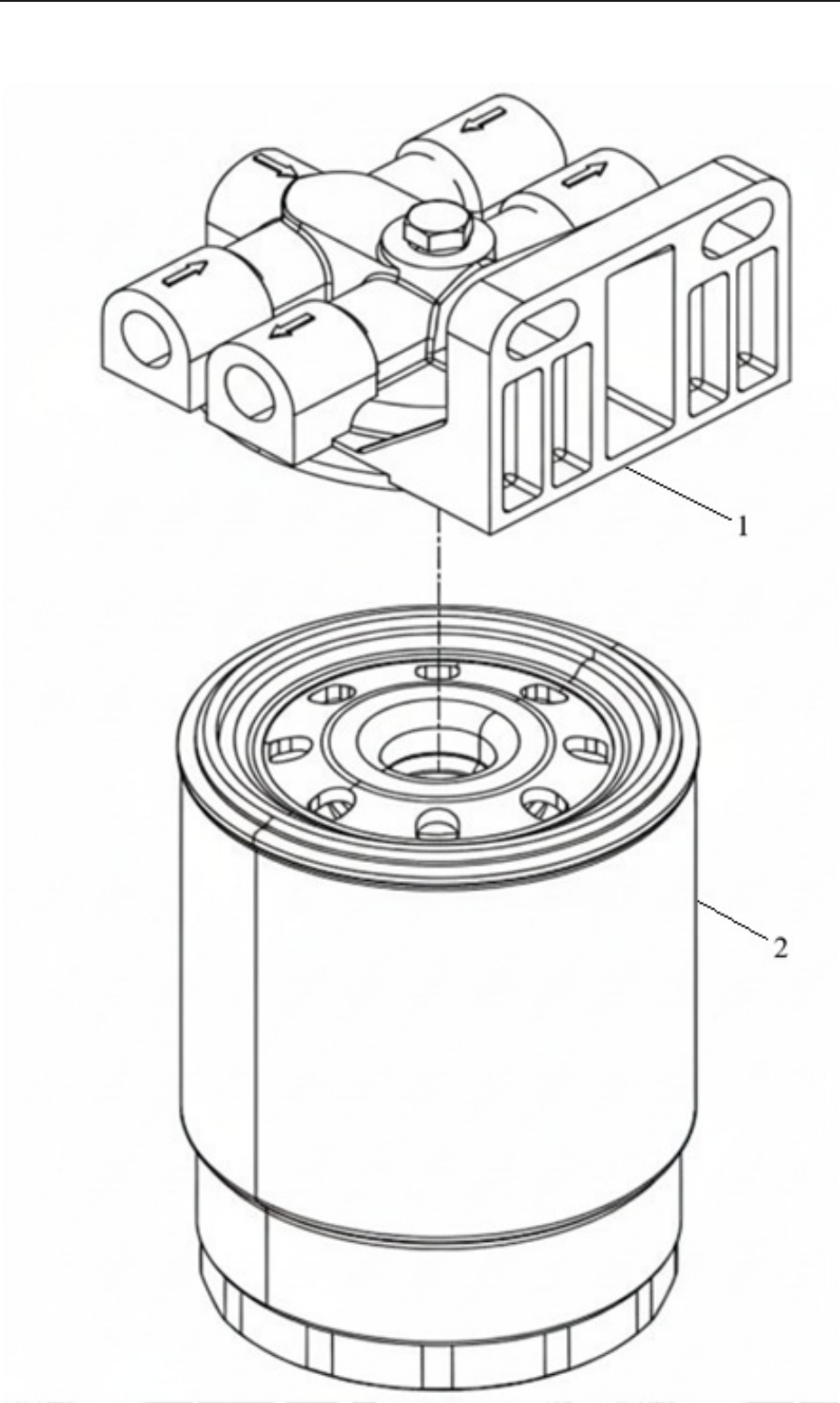
Рис. 17. Установка топливного фильтра грубой очистки
