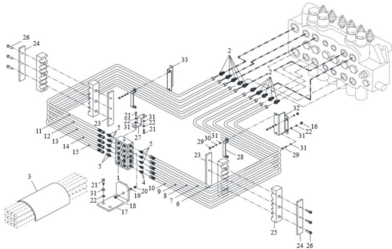
Рис. 27. Гидросистема заднего навесного оборудования
