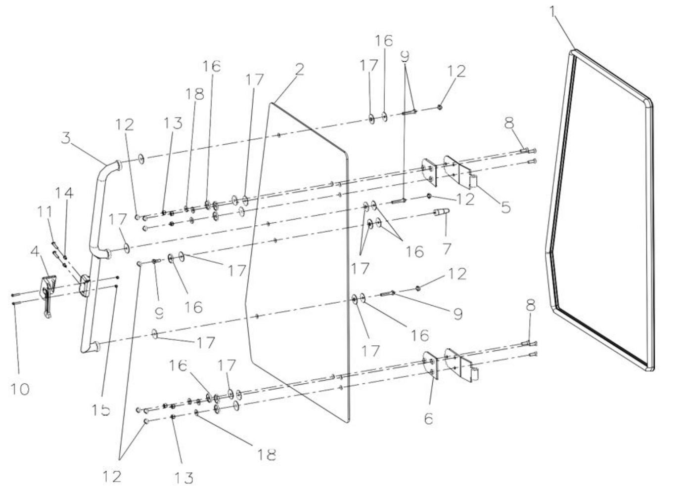
Рис. 49. Левое окно в сборе
