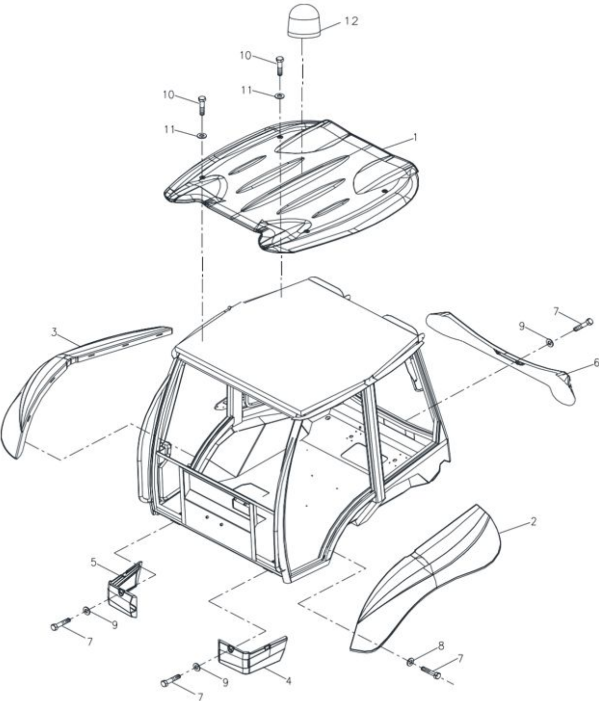
Рис. 61. Внешняя облицовка кабины
