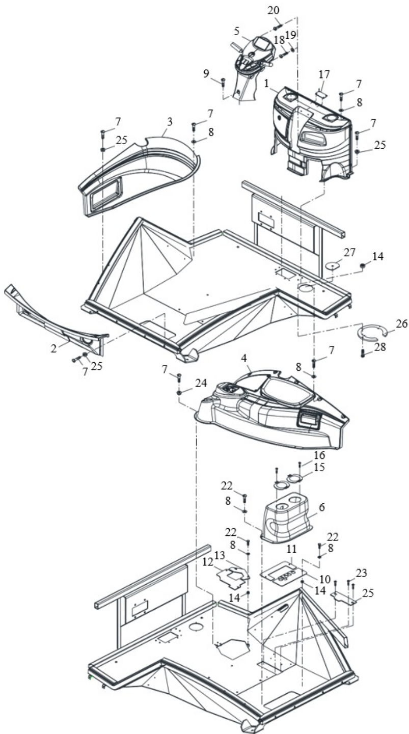
Рис. 62. Внутренняя облицовка кабины
