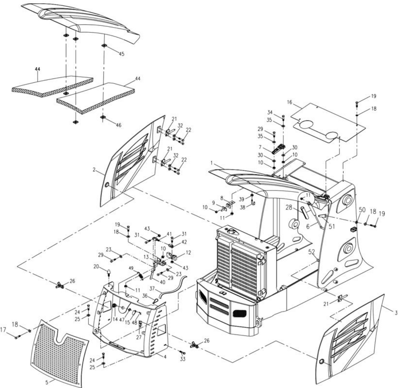
Рис. 20. Комплект облицовки капота
