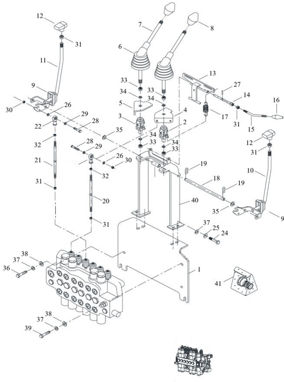
Рис. 29. Система управления экскаваторным оборудованием
