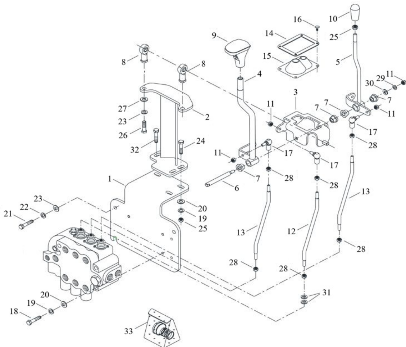
Рис. 28. Система управления погрузчиком с ковшом 6 в 1
