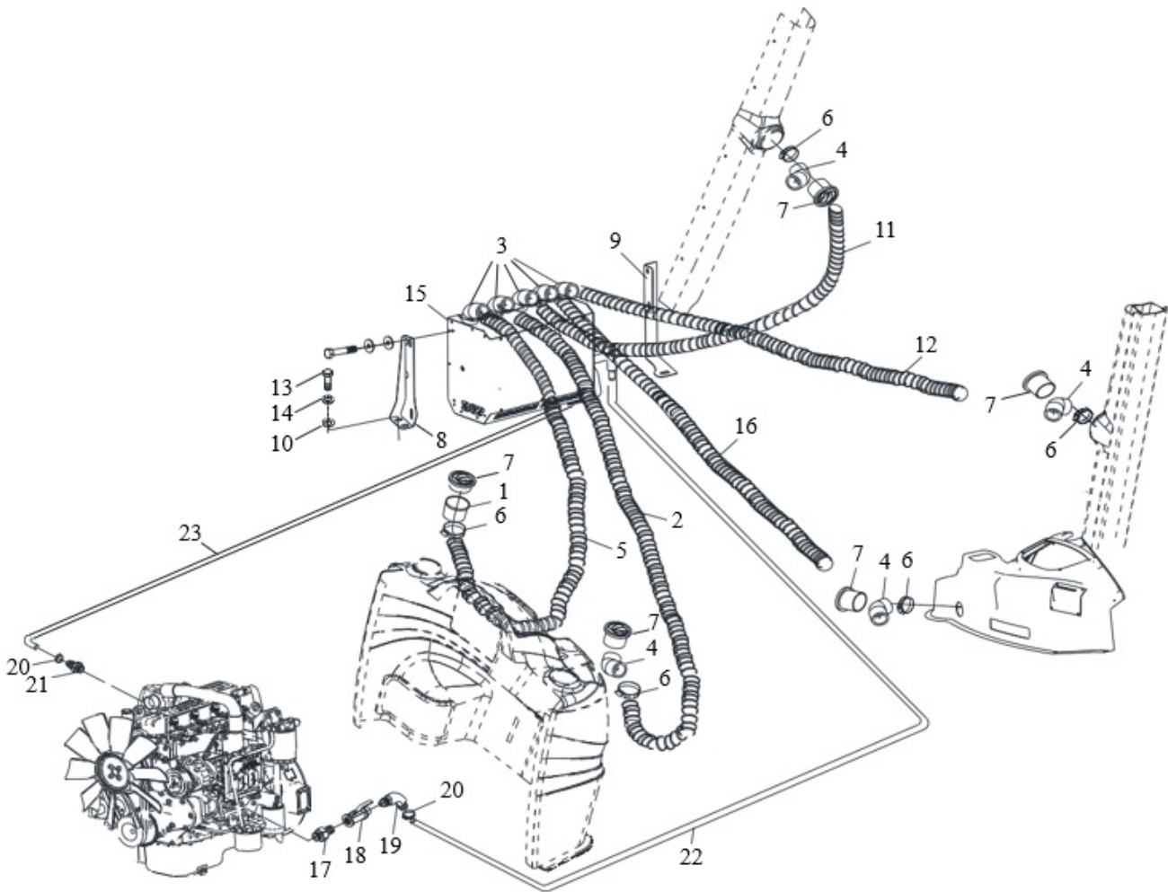
Рис. 58. Система обогрева воздуха и воздуховоды (2)
