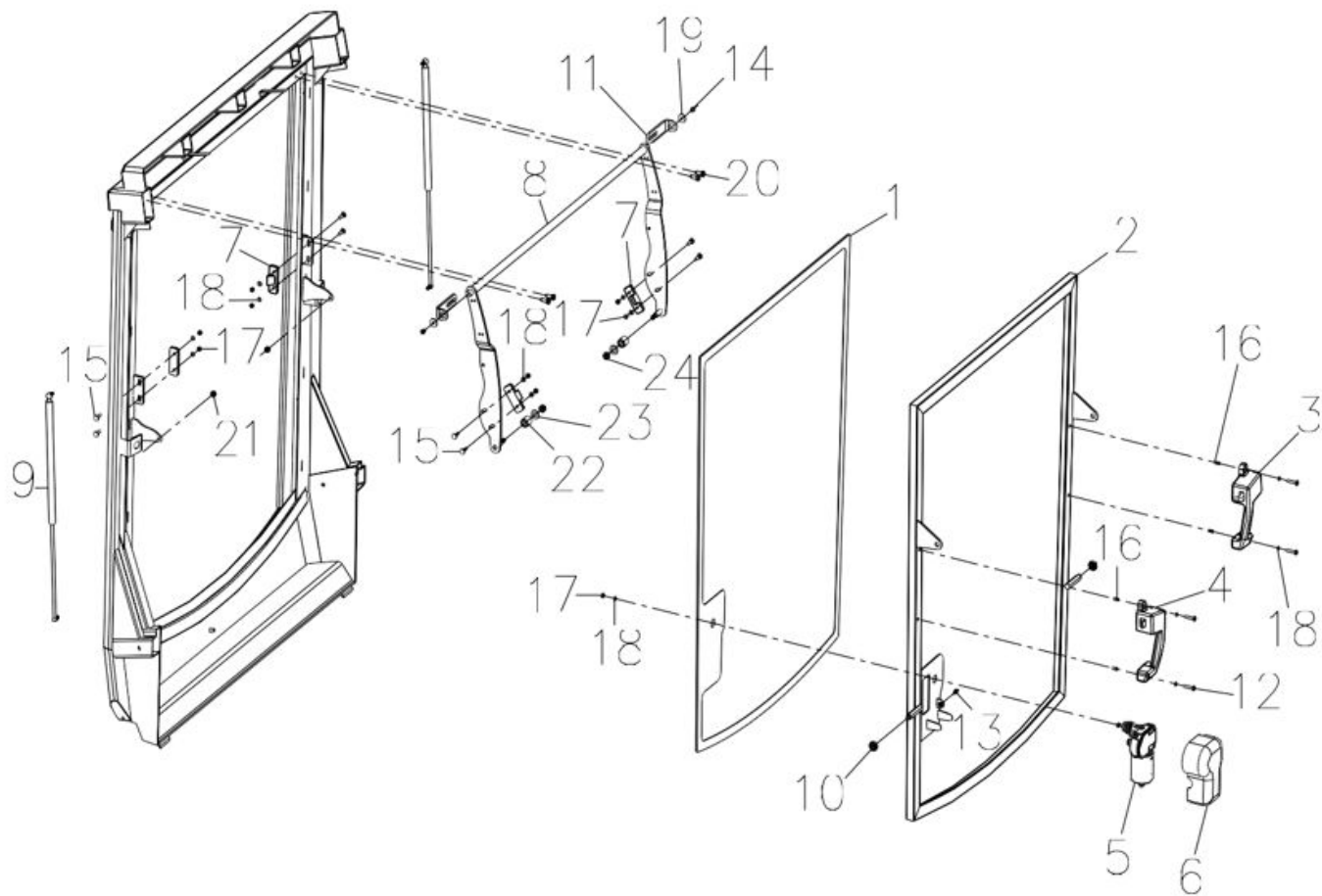
Рис. 47. Заднее окно в сборе
