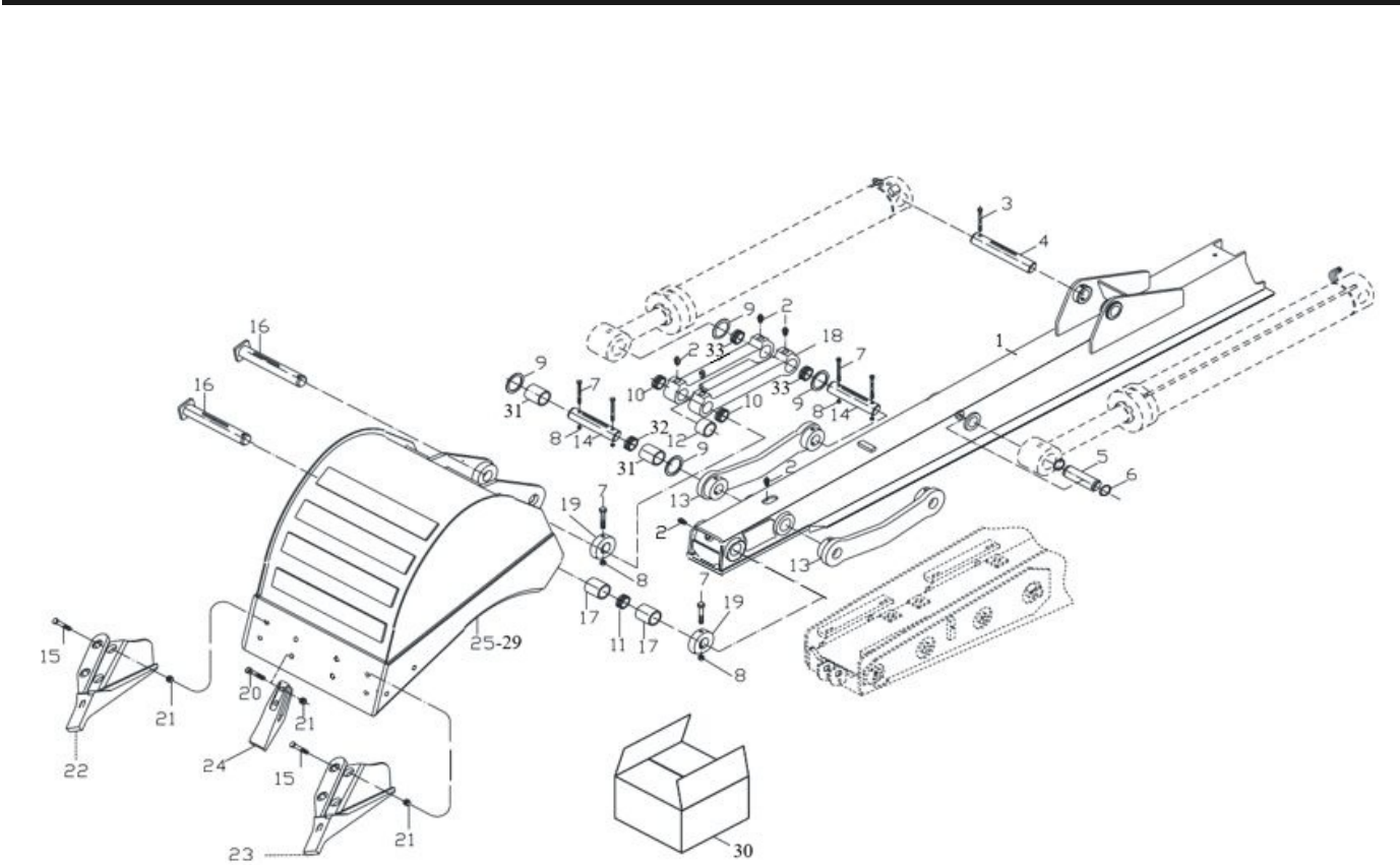
Рис. 85. Телескоп экскаватора и ковш в сборе (модификация с телескопом)
