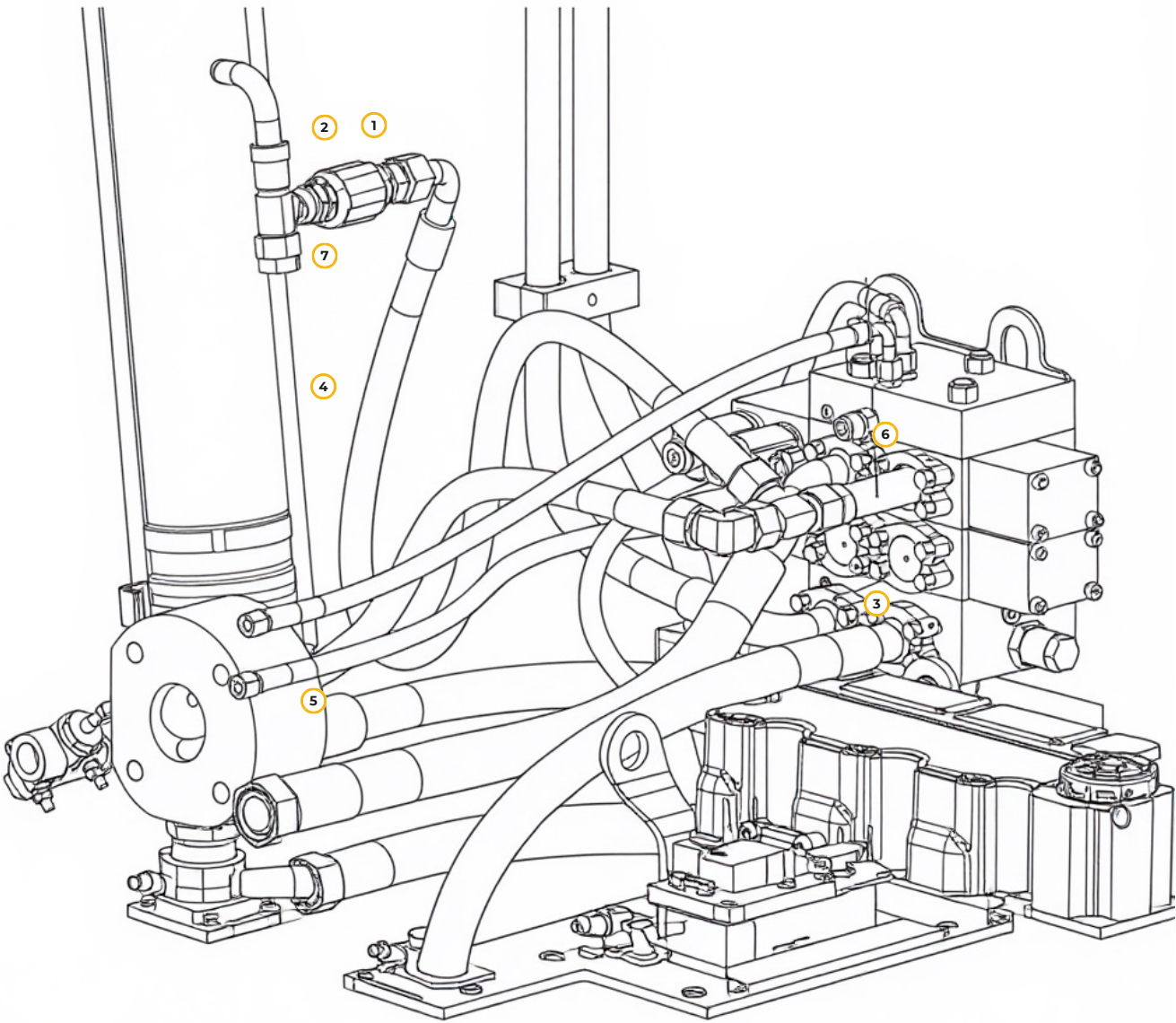
Рис. 31. РВД гидросистемы навесного оборудования
