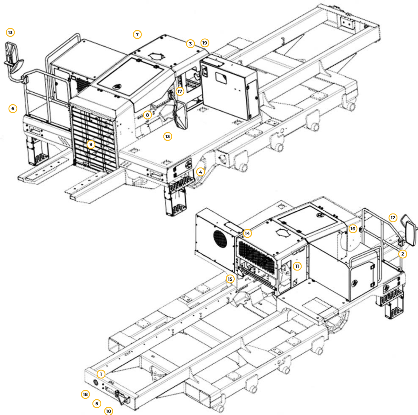
Рис. 19. Облицовка рамы
