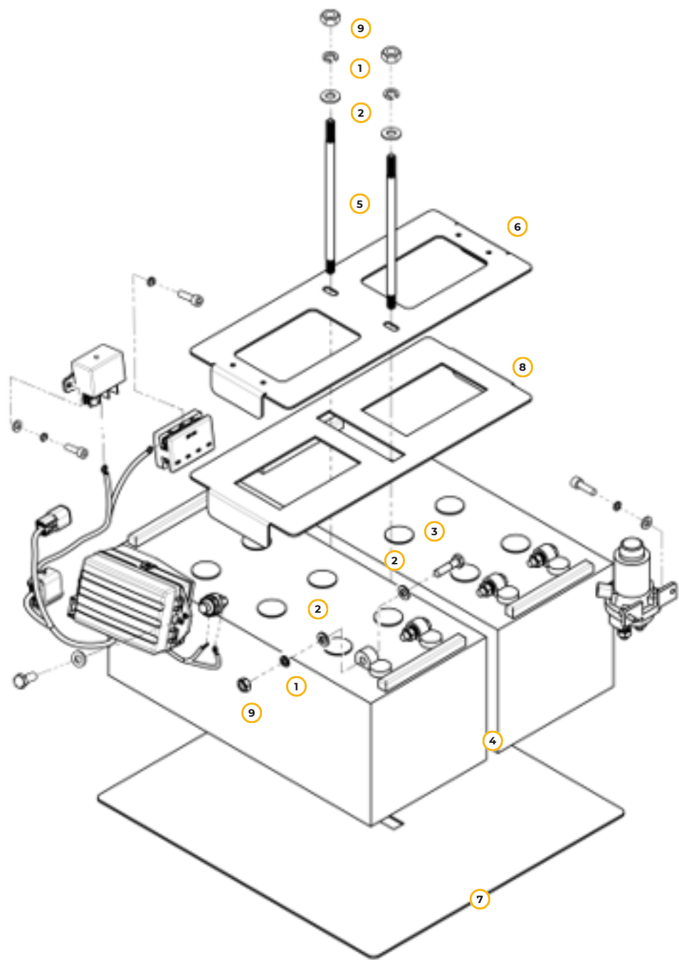
Рис. 59. Аккумуляторные батареи с элементами крепления
