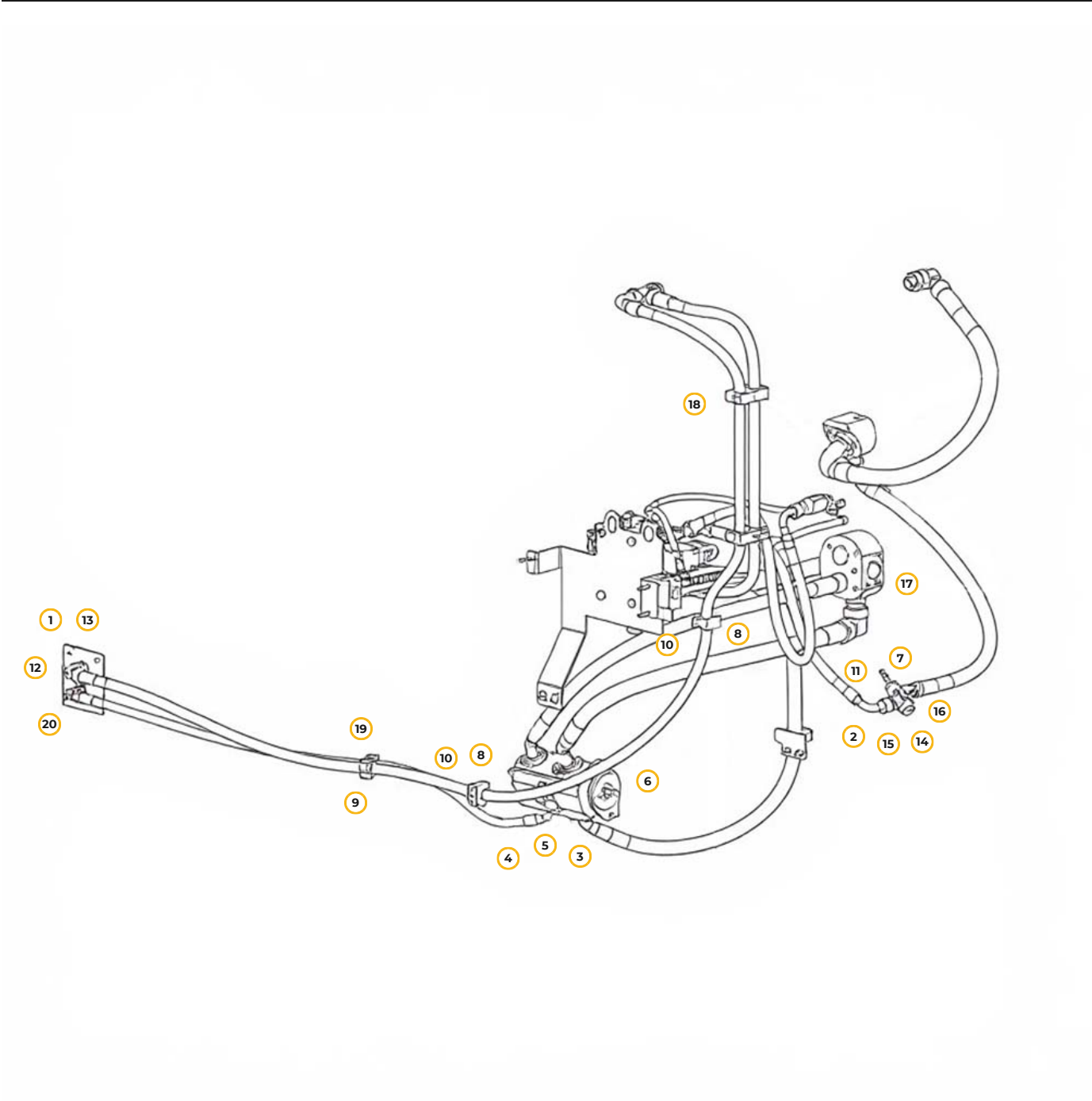
Рис. 30. РВД гидросистемы навесного оборудования
