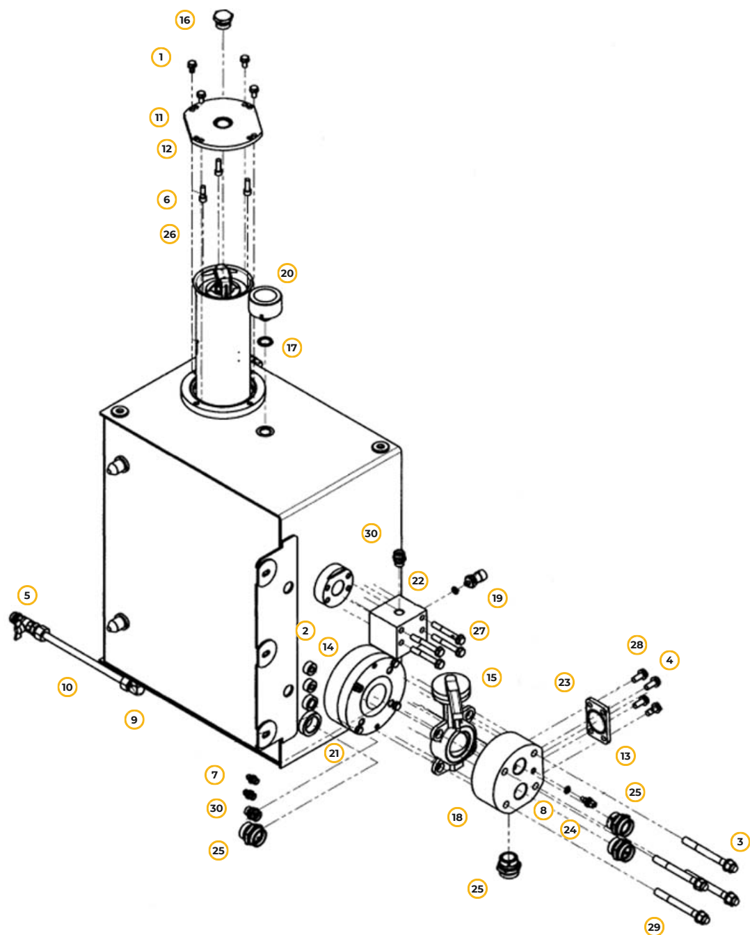
Рис. 38. Бак гидравлический в сборе
