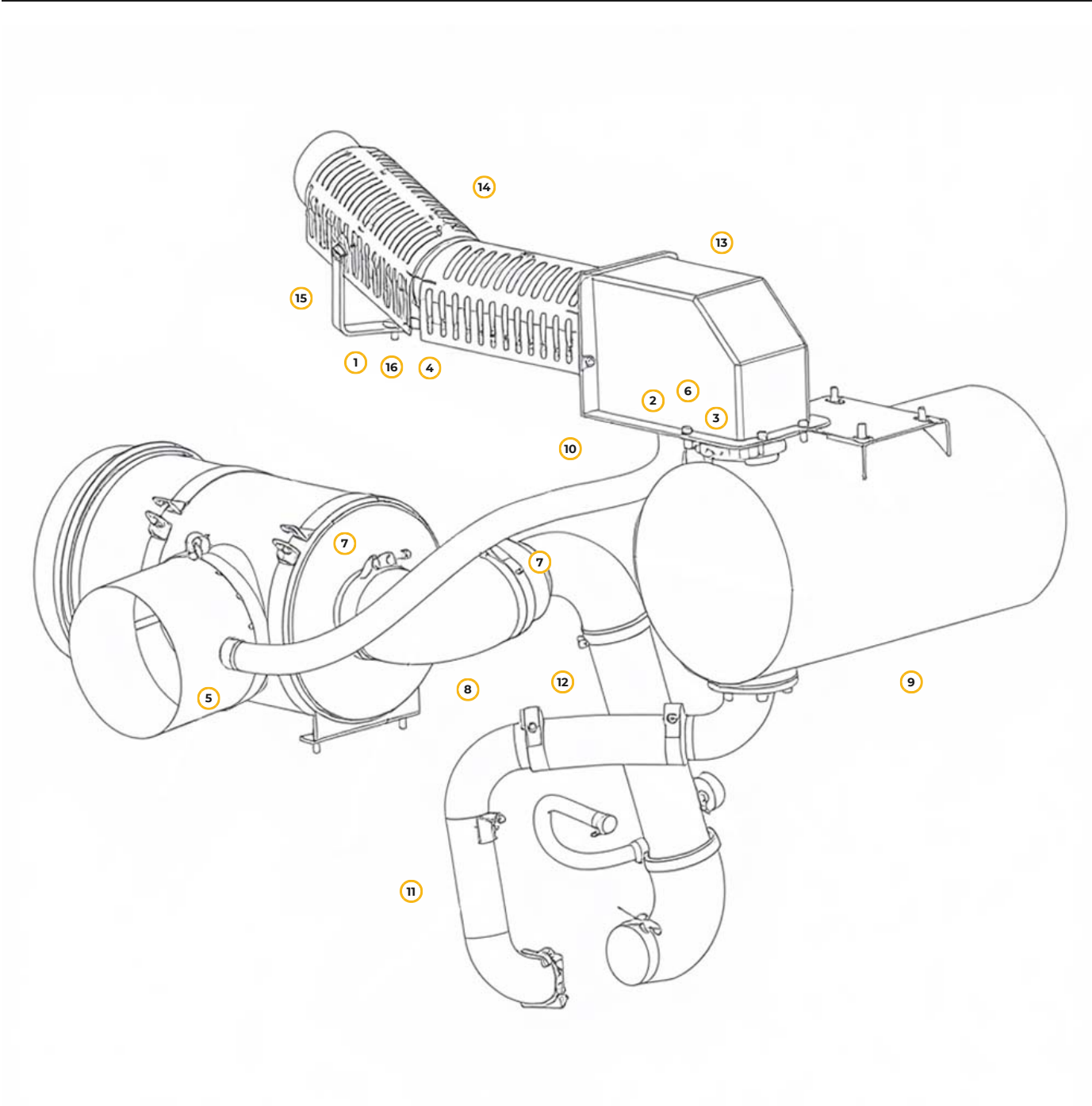
Рис. 11. Система впуска воздуха и выпуска ОГ
