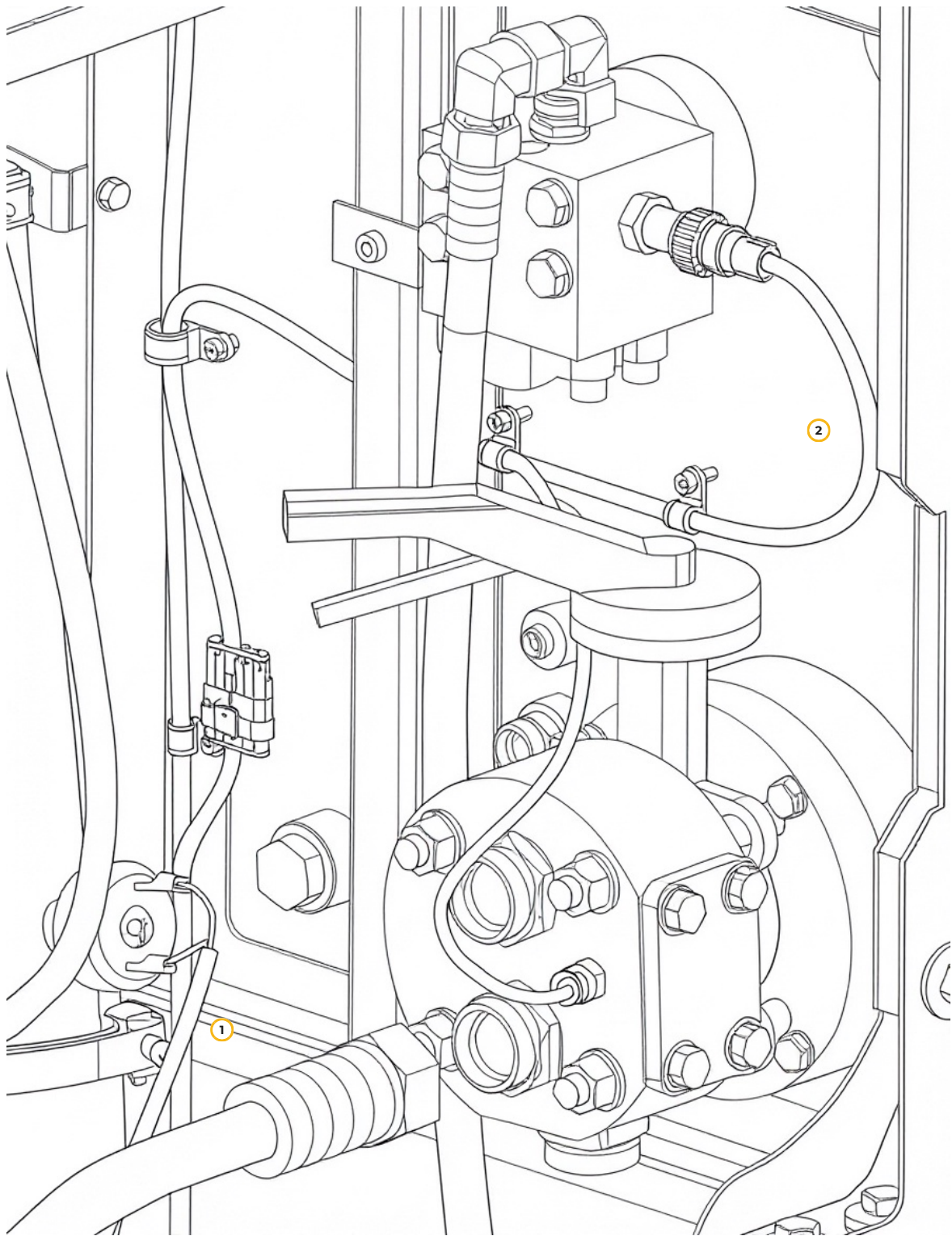
Рис. 56. Электрооборудования рамы
