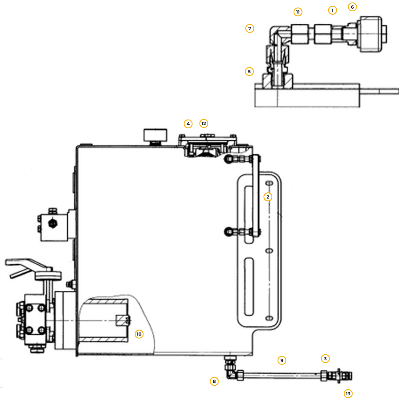
Рис. 37. Бак гидравлический в сборе
