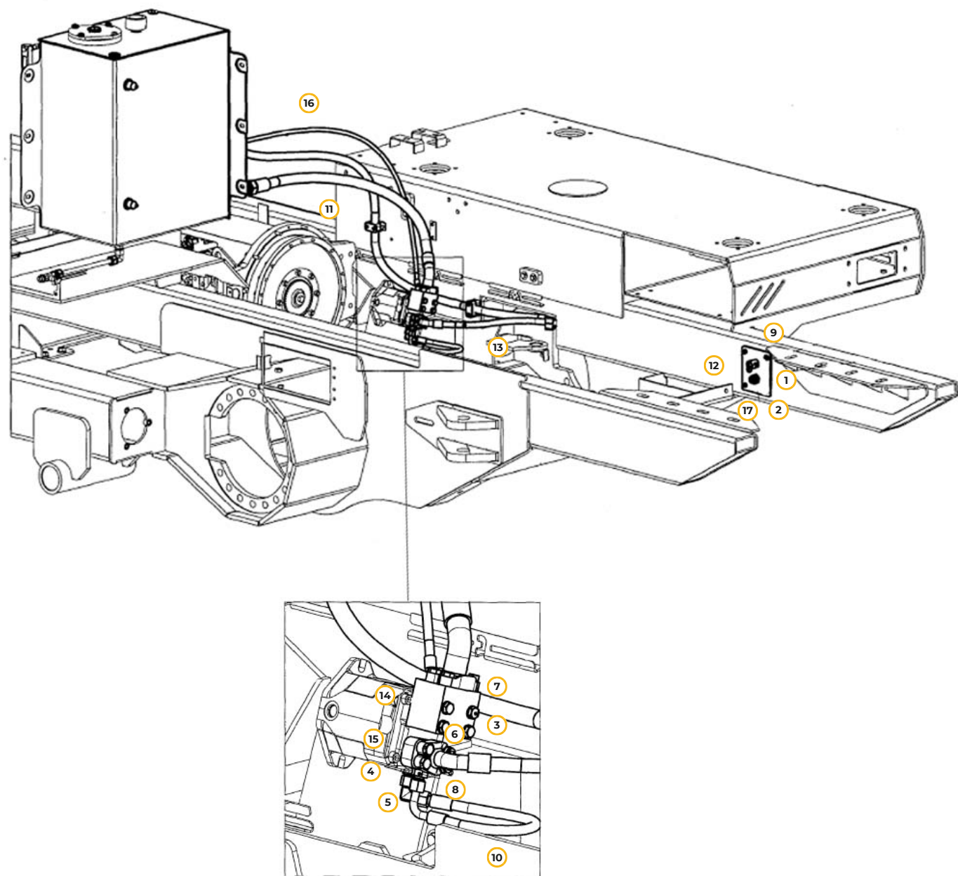
Рис. 36. РВД гидросистемы навесного оборудования
