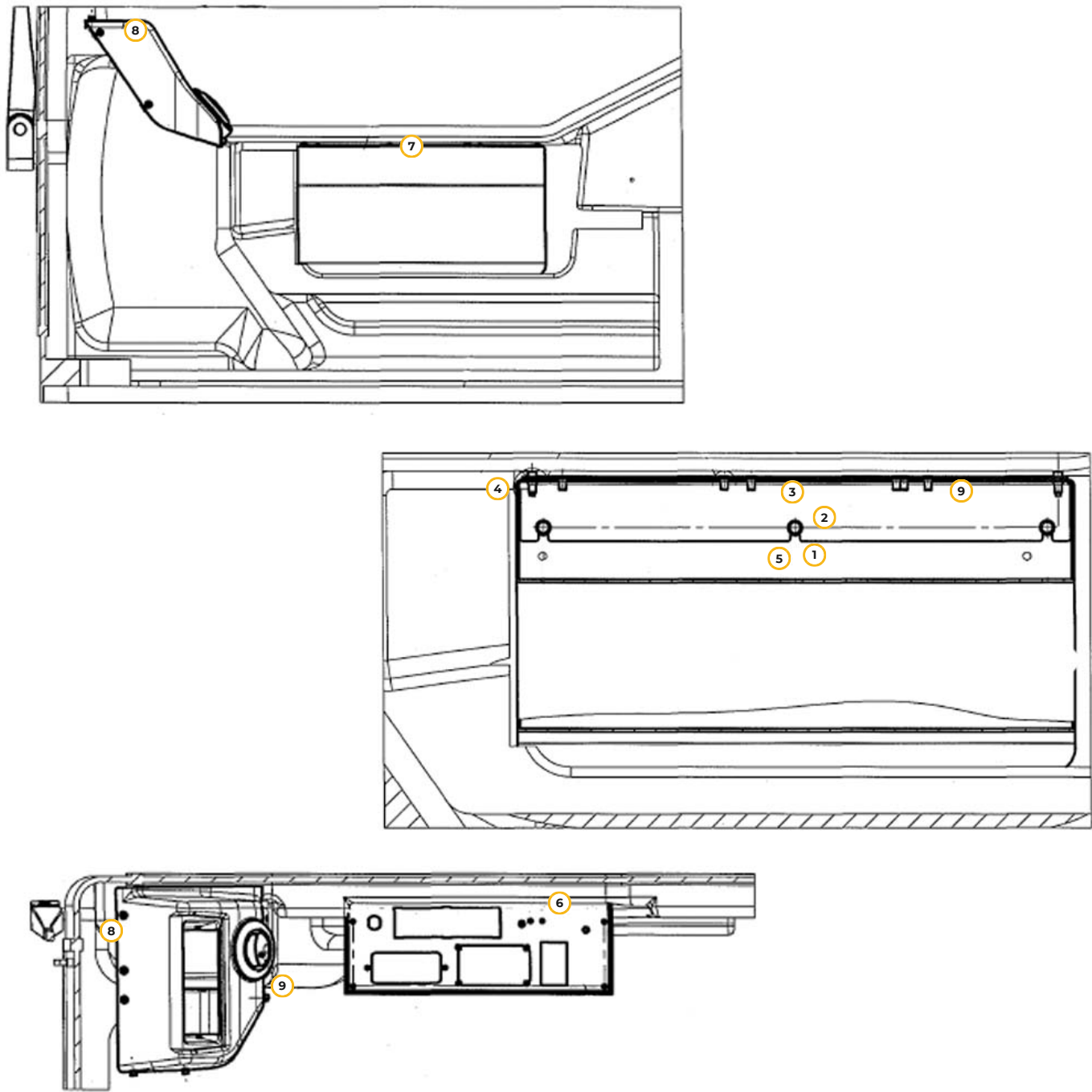
Рис. 65. Кронштейн в сборе
