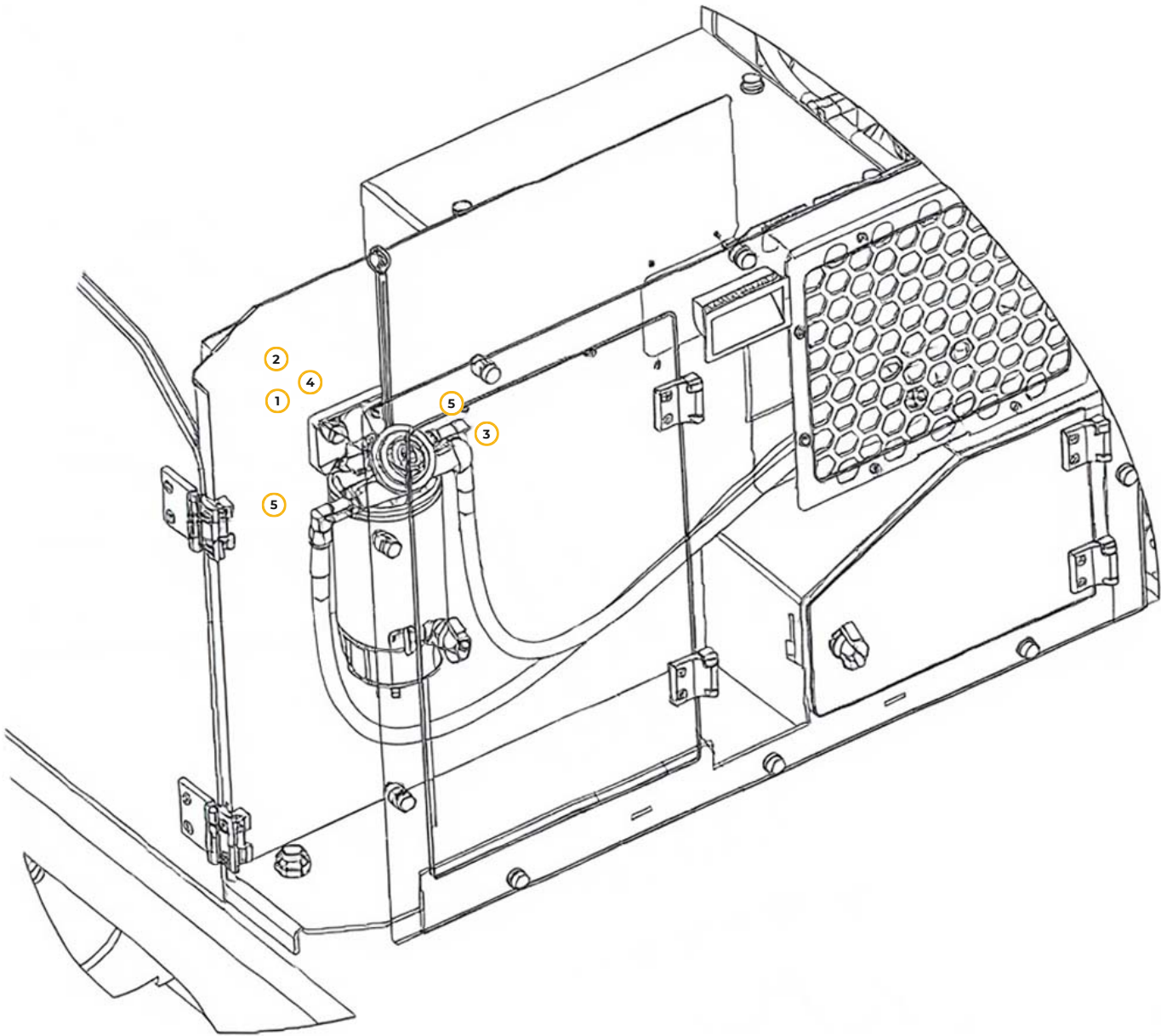
Рис. 14. Топливная система
