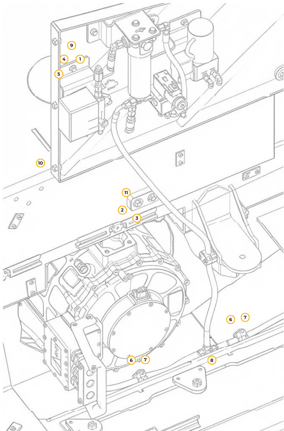
Рис. 43. Трубопроводы гидросистемы трансмиссии
