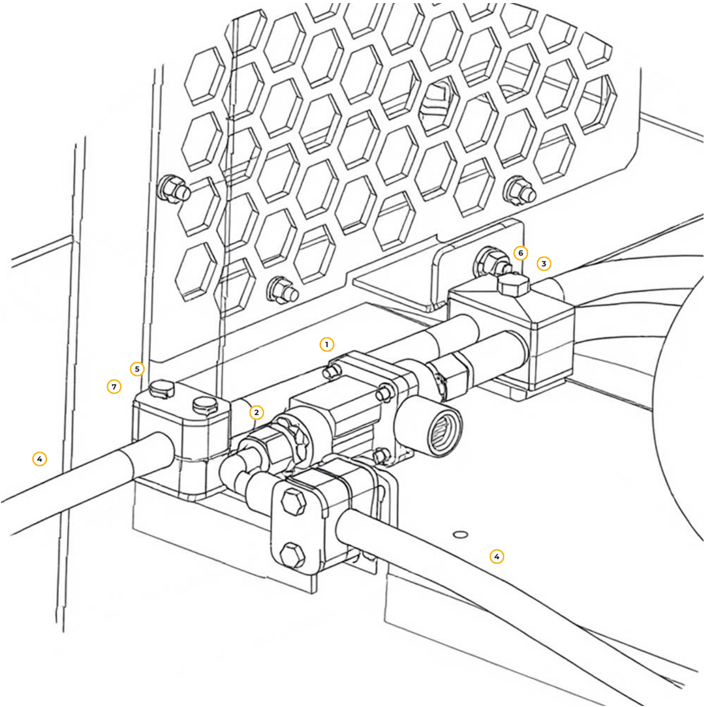
Рис. 13. Топливная система
