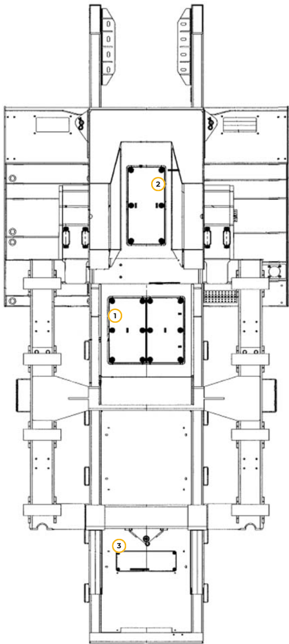
Рис. 24. Установка облицовки
