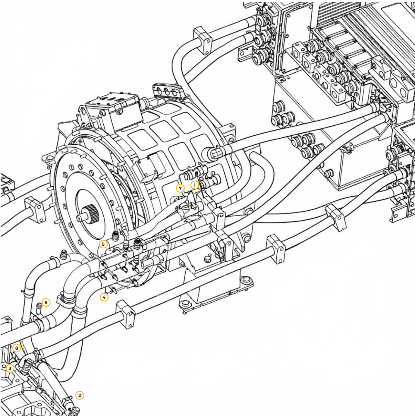
Рис. 4. Система охлаждения
