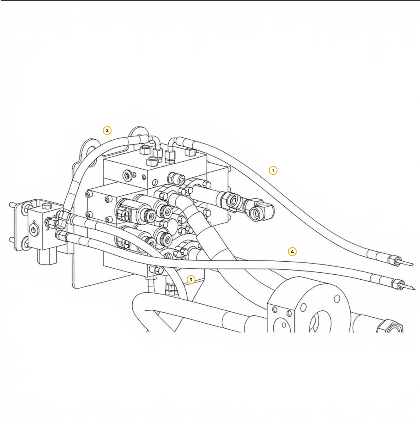
Рис. 32. РВД гидросистемы навесного оборудования
