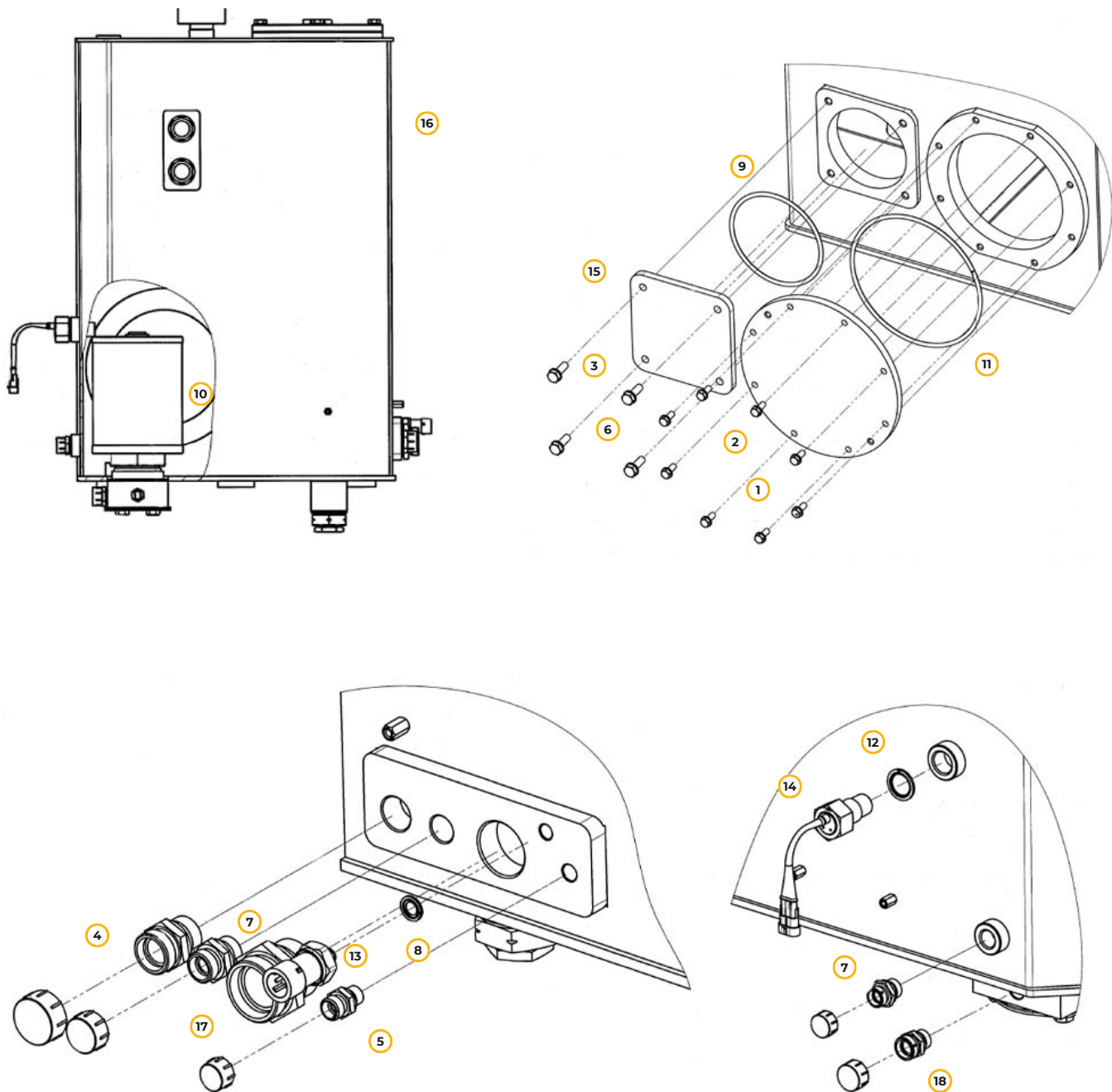
Рис. 43. Бак гидравлический в сборе
