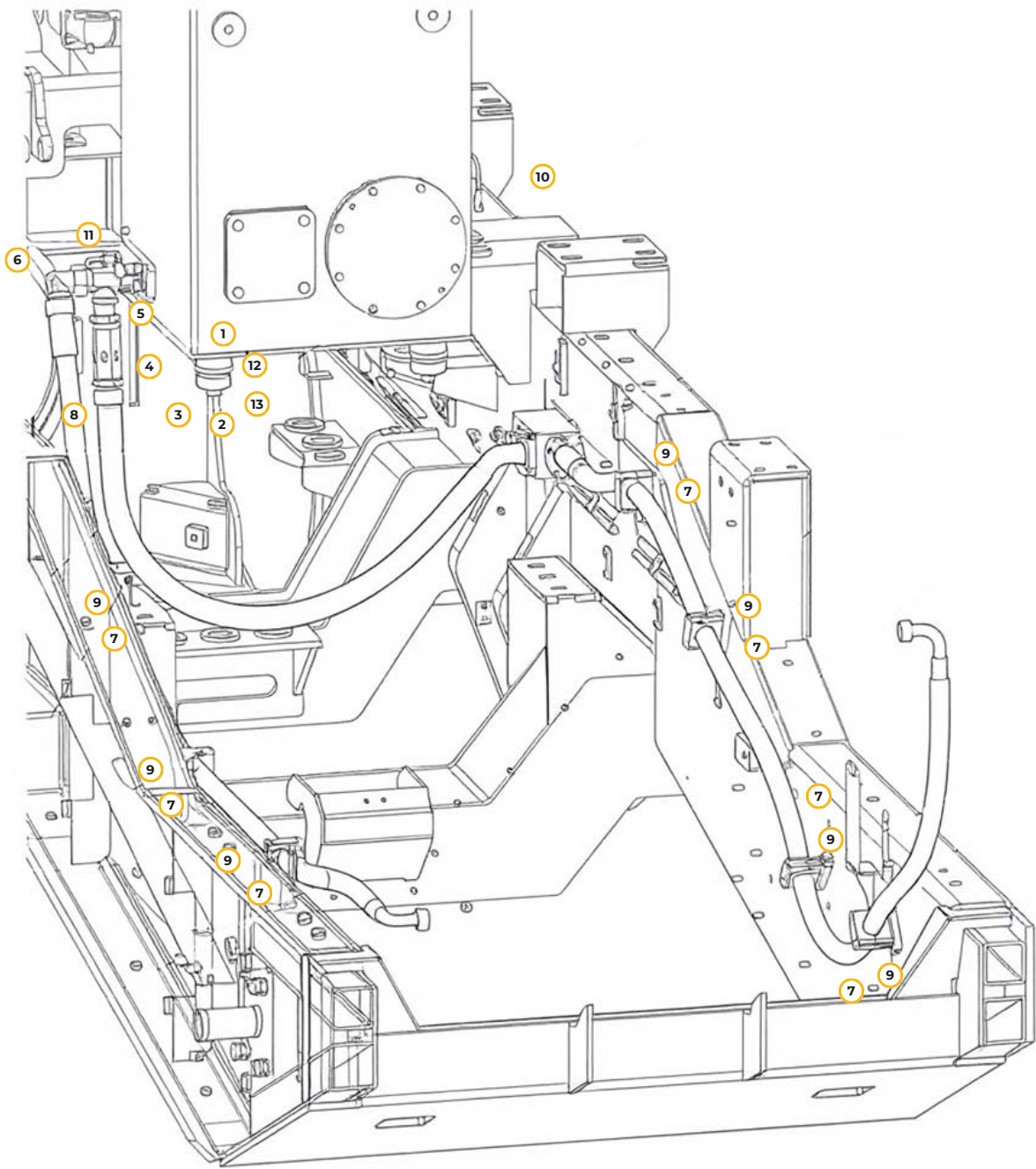
Рис. 40. РВД гидросистемы навесного оборудования
