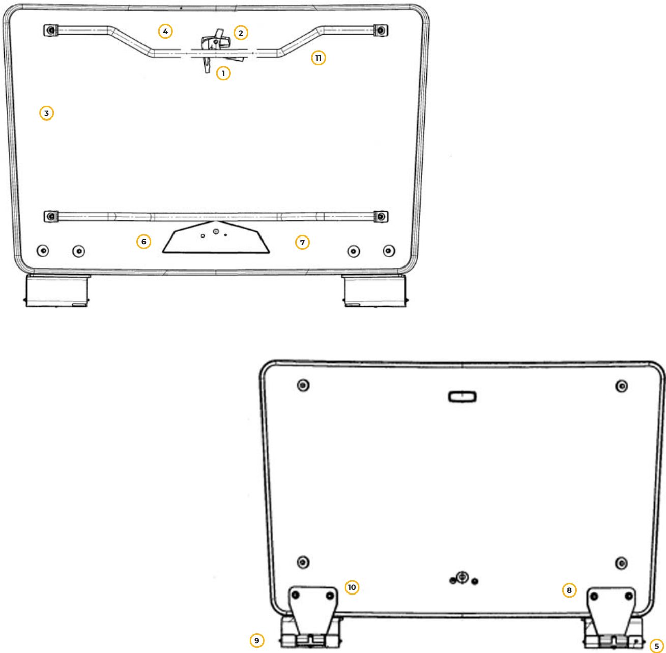
Рис. 87. Окно заднее в сборе
