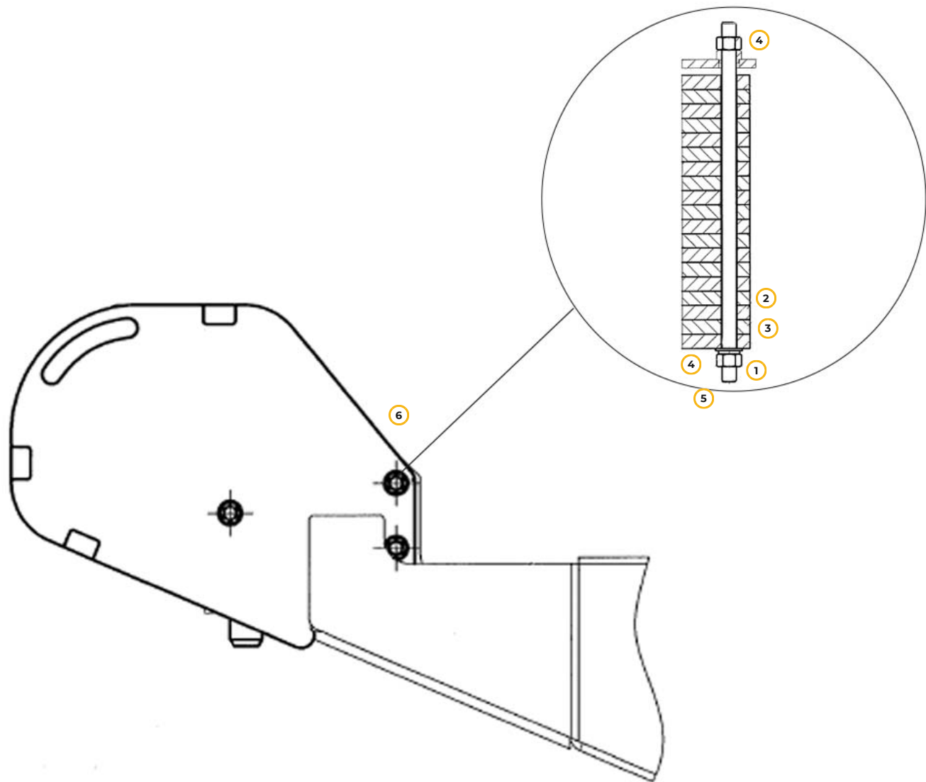
Рис. 19. Комплект балластировочных грузов
