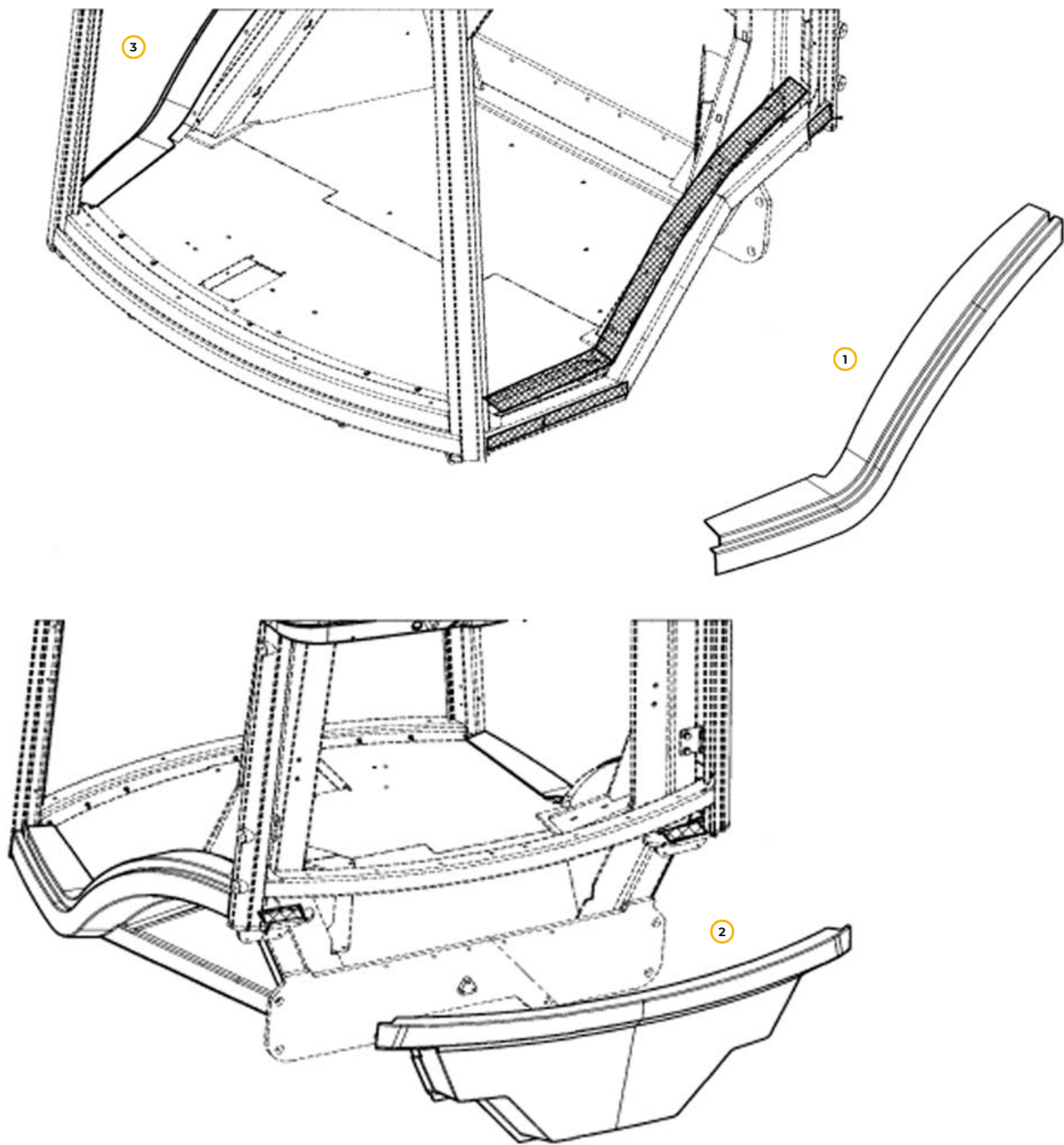
Рис. 96. Обшивка наружная
