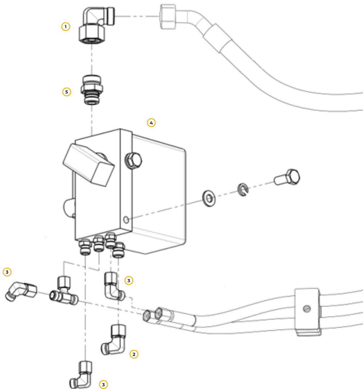
Рис. 45. Насос ручной в сборе
