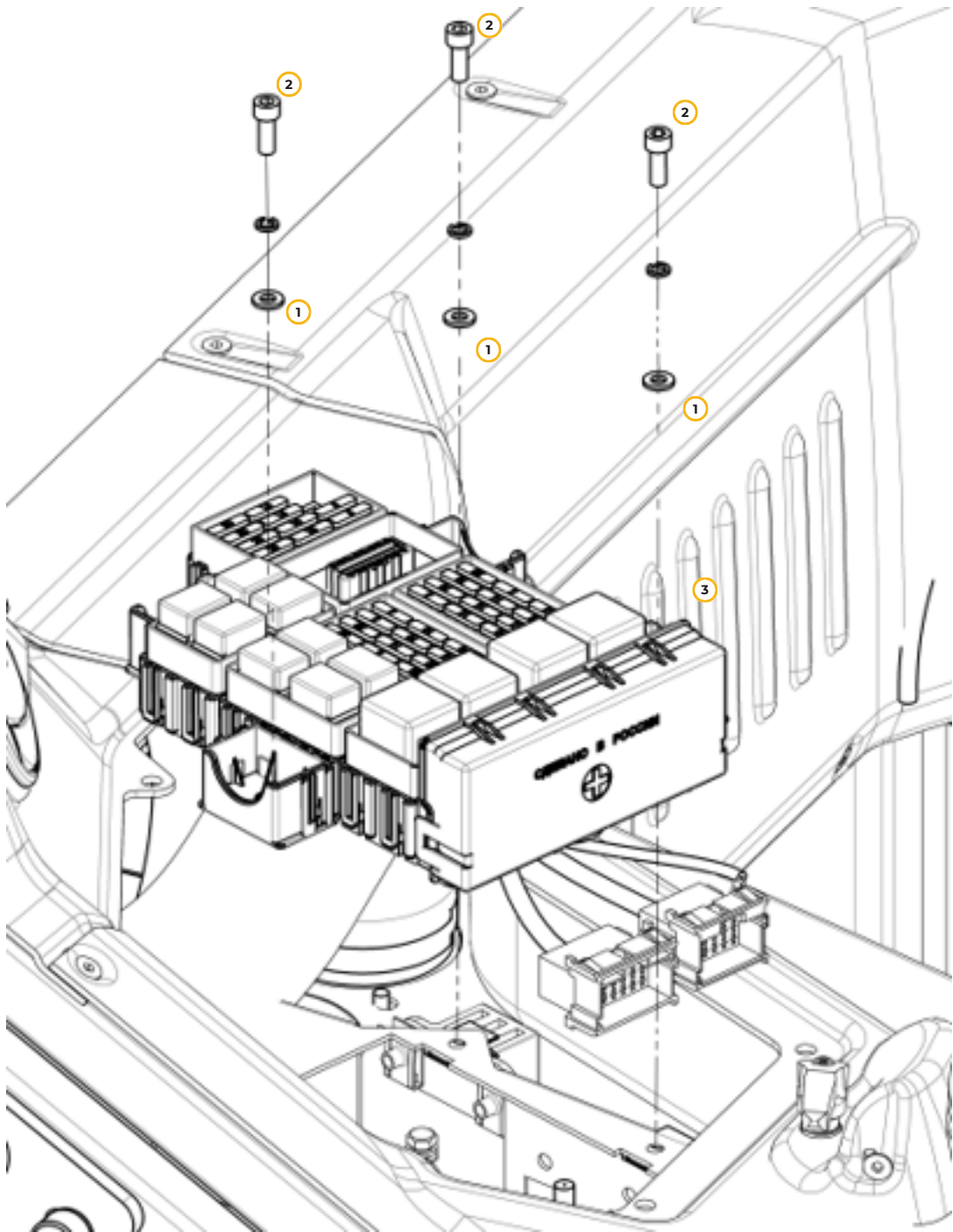
Рис. 64. Блок предохранителей и реле
