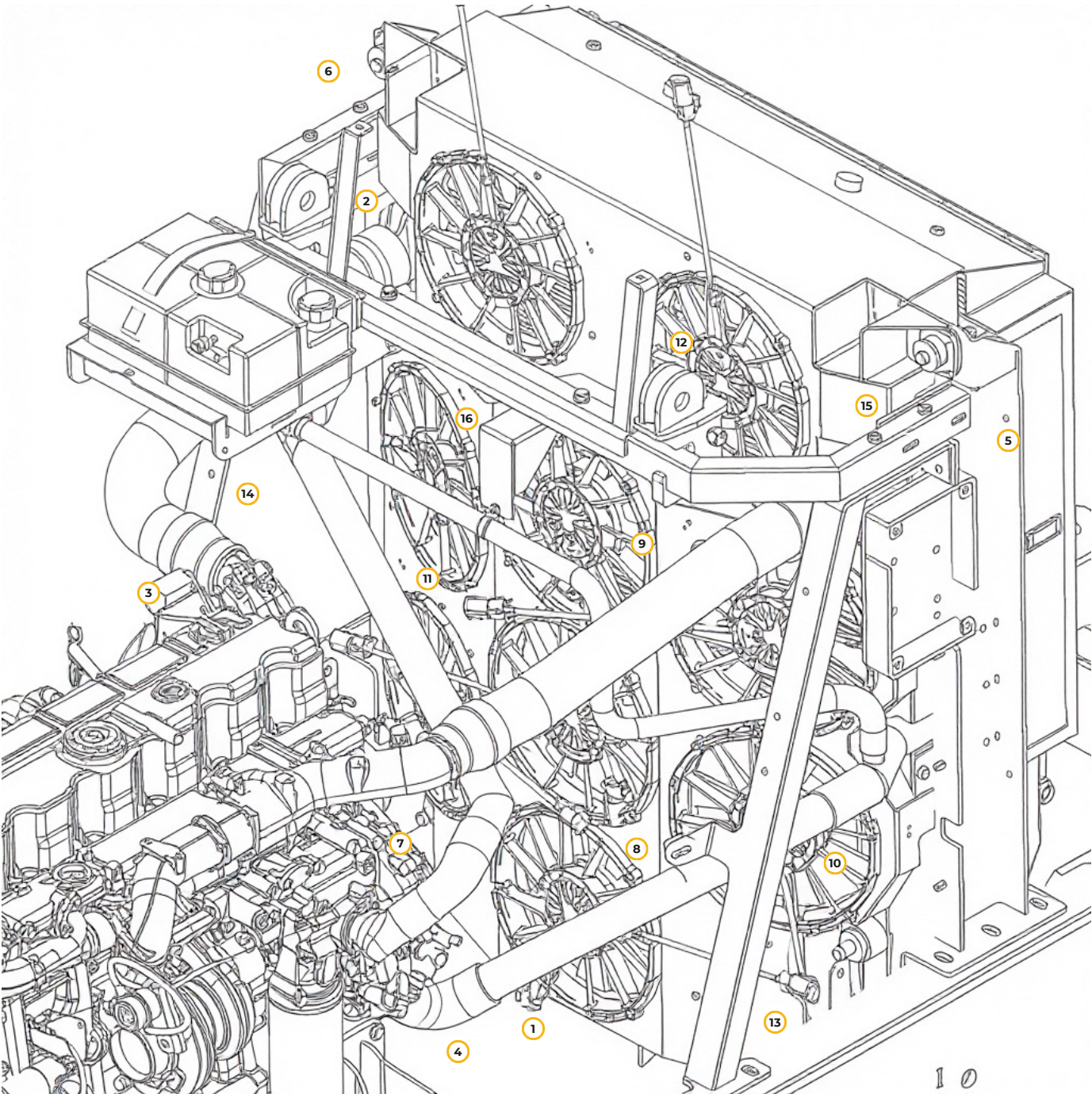
Рис. 5. Система охлаждения
