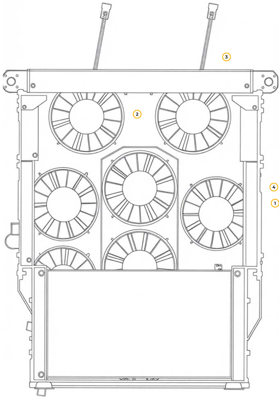
Рис. 8. Блок радиаторов в сборе
