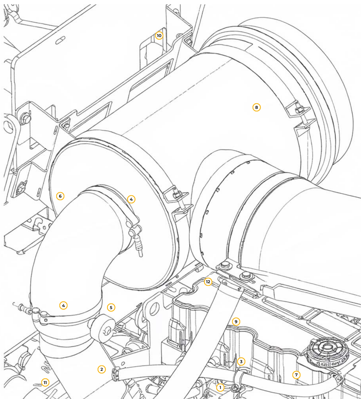
Рис. 14. Система впуска воздуха и выпуска ОГ
