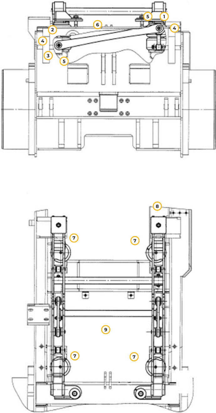
Рис. 79. Система подвески кабины
