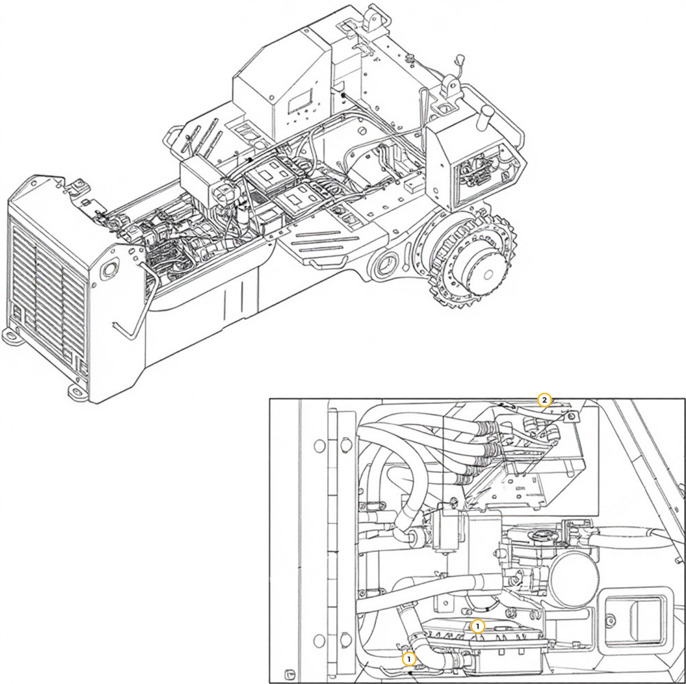
Рис. 54. Электромеханическая трансмиссия
