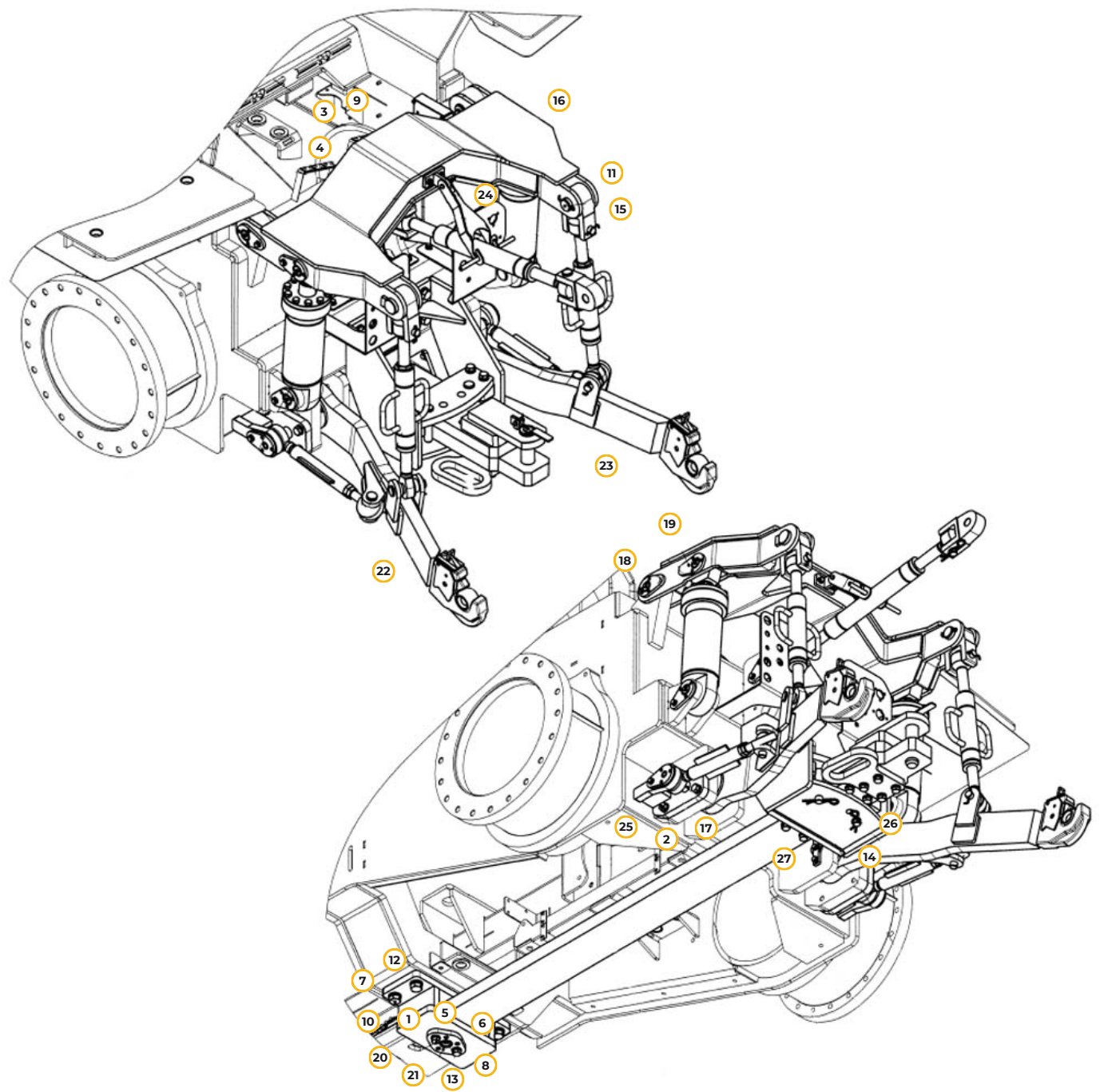
Рис. 97. Механизм навески
