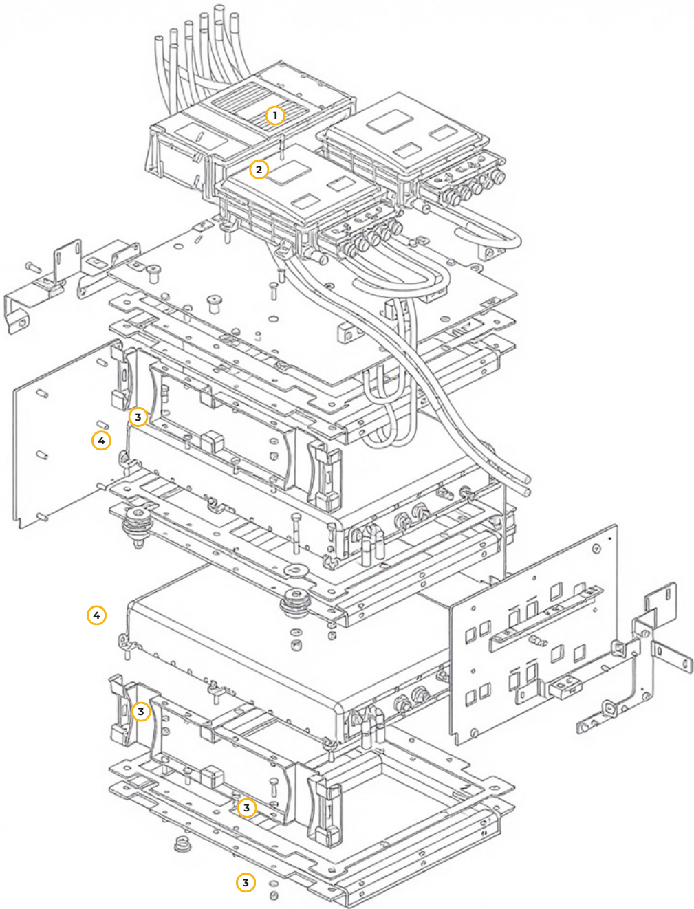
Рис. 57. Установка энергетическая
