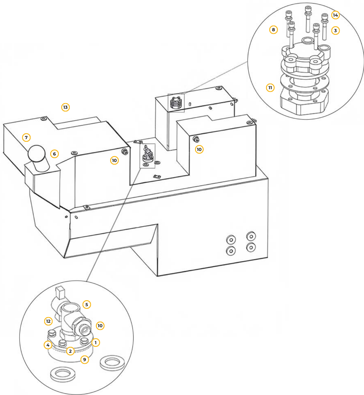
Рис. 18. Топливный бак
