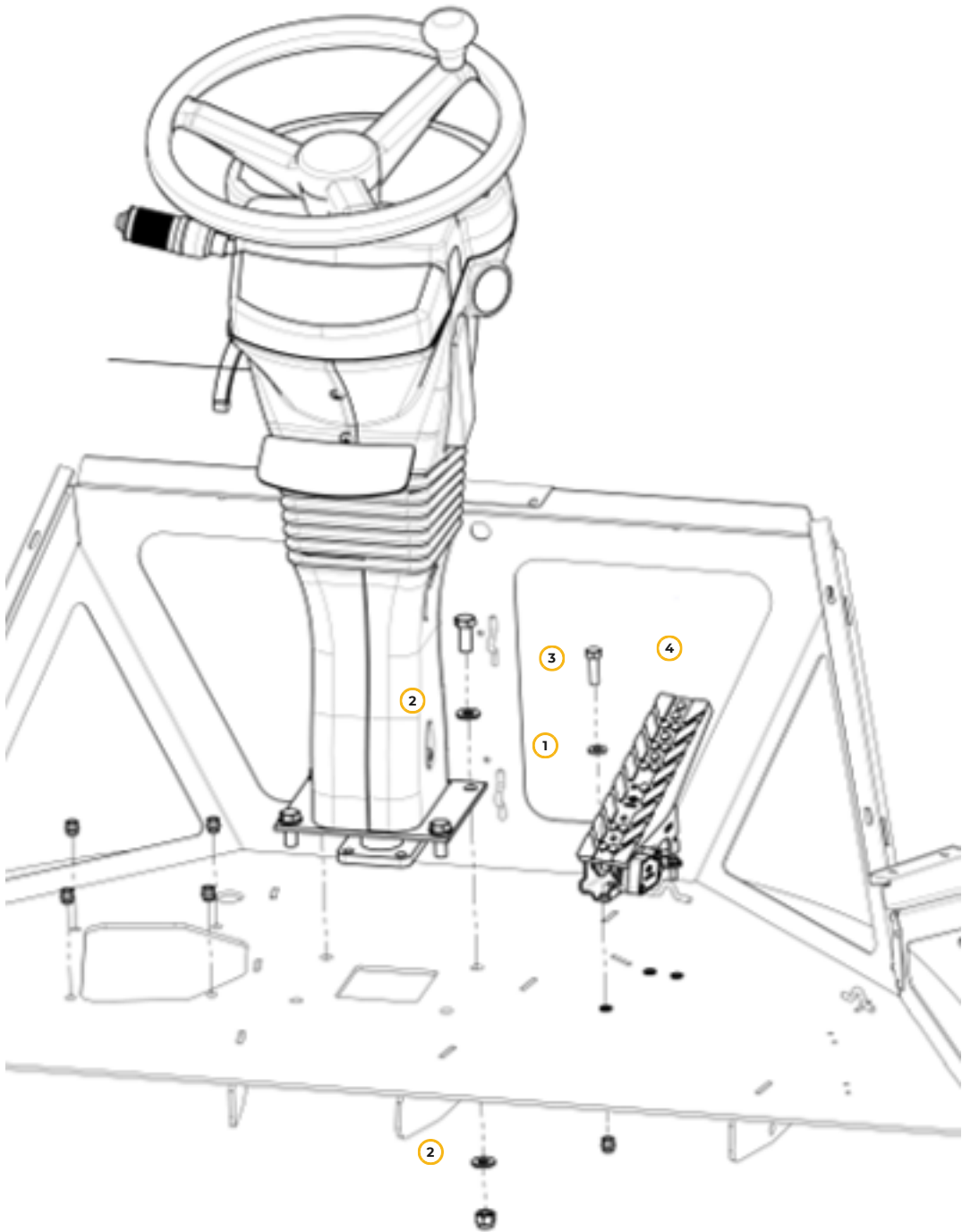
Рис. 91. Органы управления
