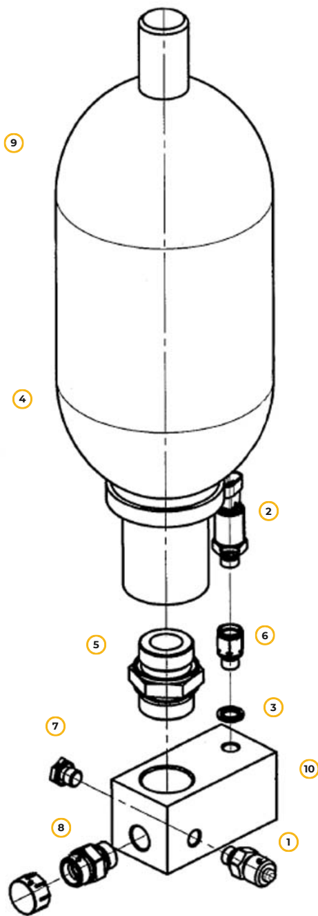
Рис. 51. Гидропневмоаккумулятор в сборе
