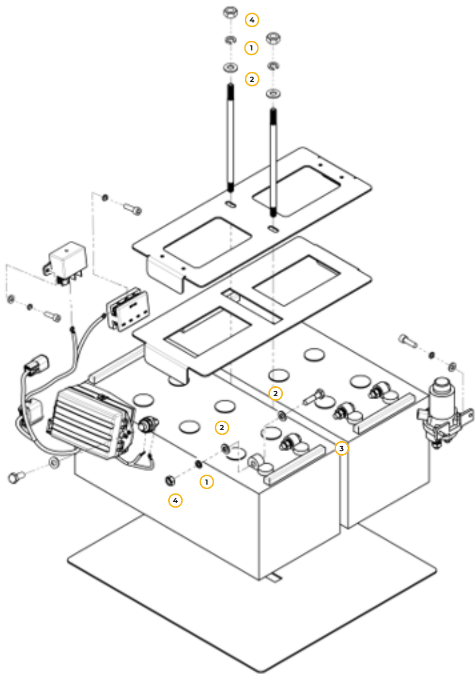
Рис. 74. Аккумуляторные батареи с элементами крепления
