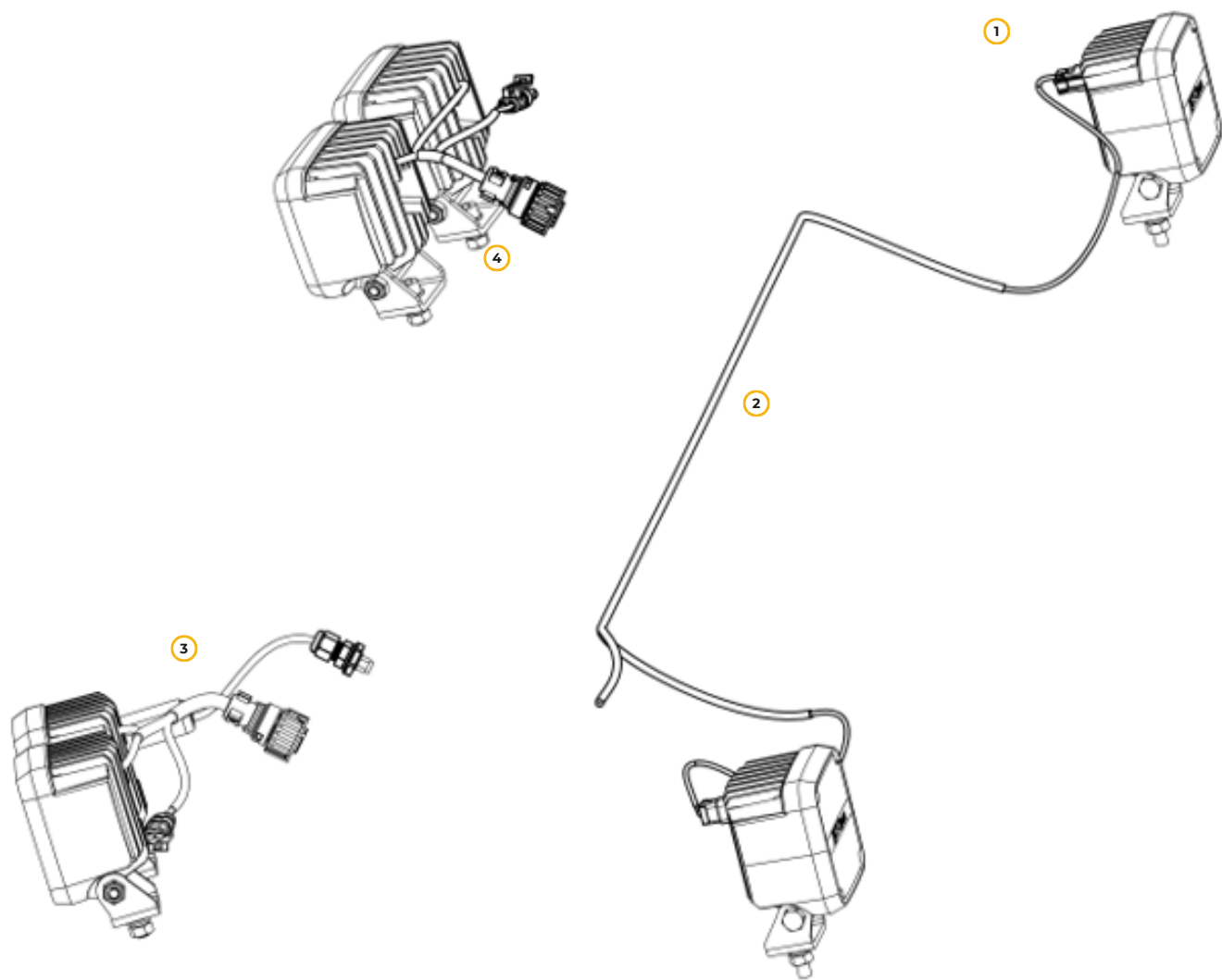
Рис. 63. Элементы освещения и звуковой сигнализации кабины
