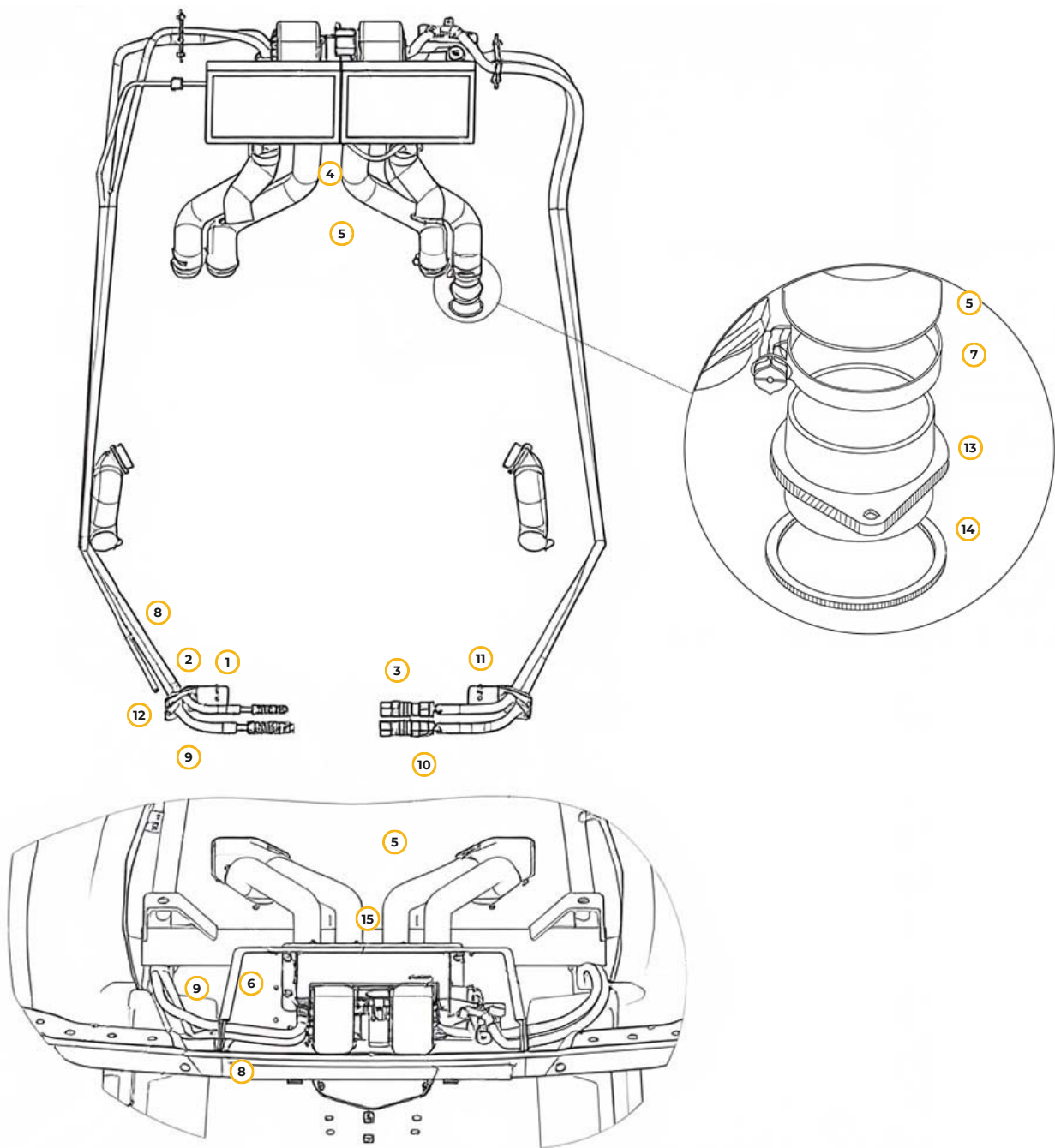
Рис. 90. Система климатическая
