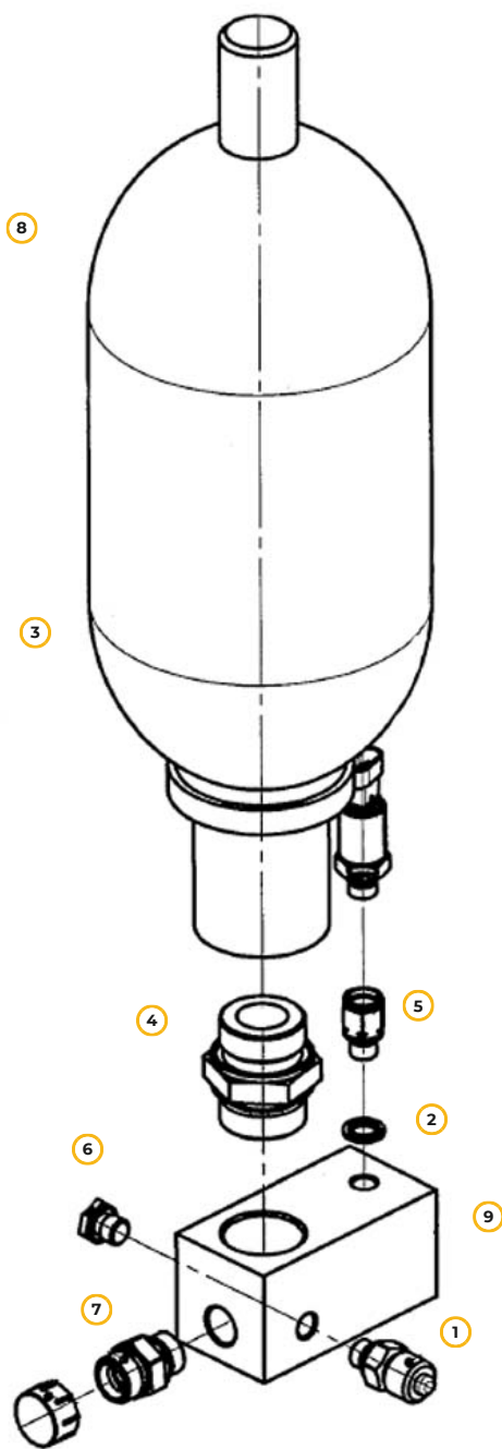
Рис. 50. Гидропневмоаккумулятор в сборе
