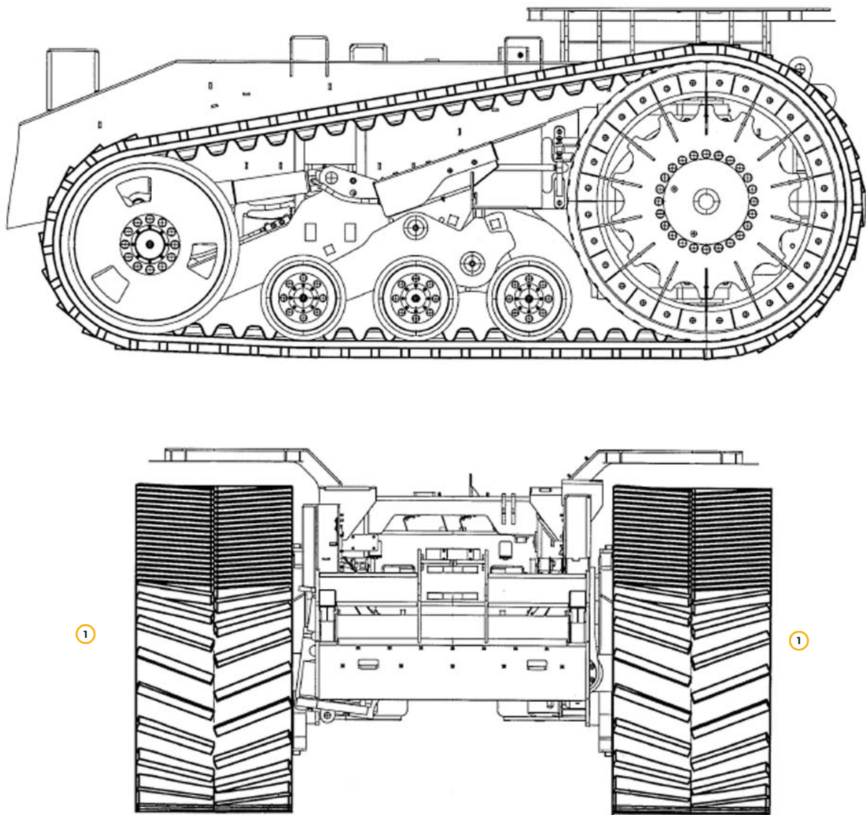
Рис. 22. Комплект установки гусениц
