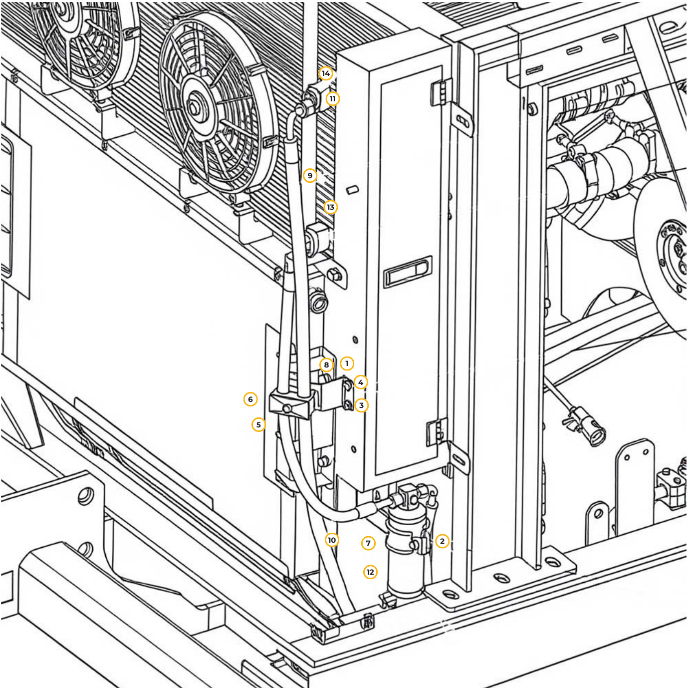
Рис. 12. Система климатическая
