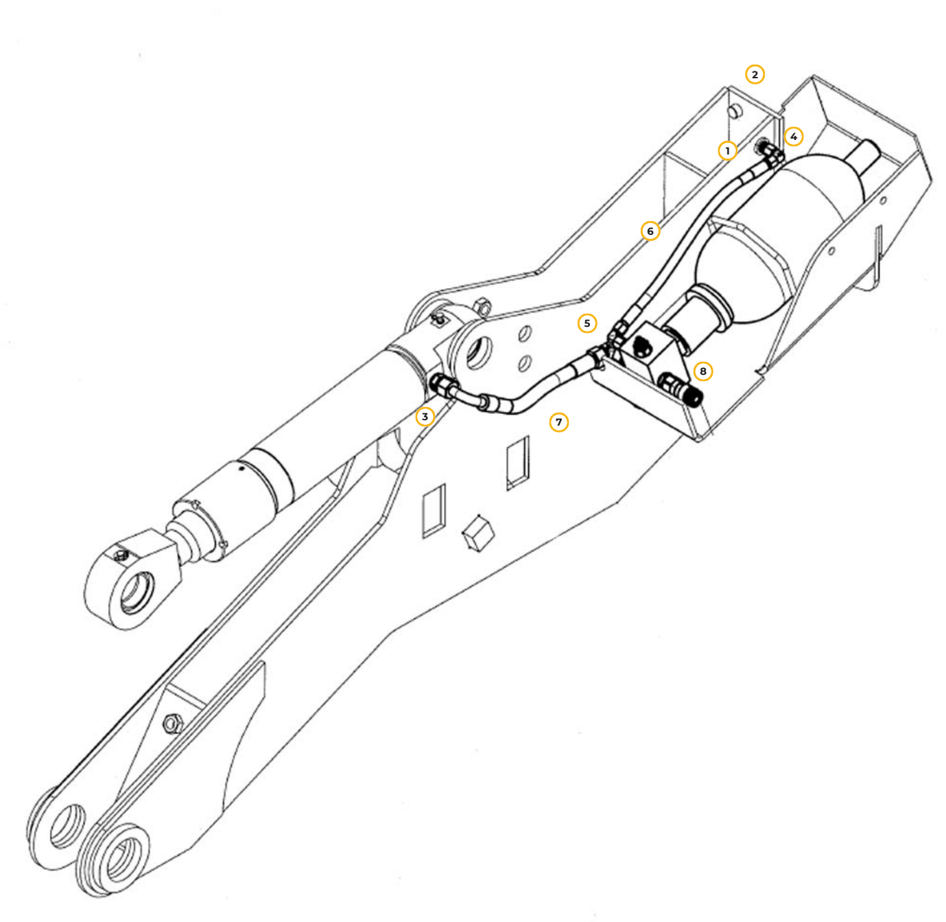
Рис. 28. Трубопроводы гидропривода механизма сдавания и натяжения гусениц
