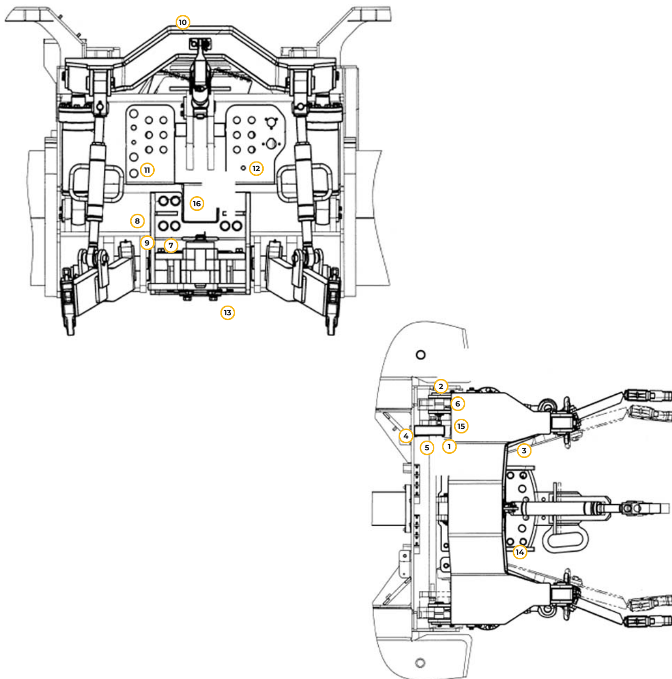
Рис. 98. Механизм навески
