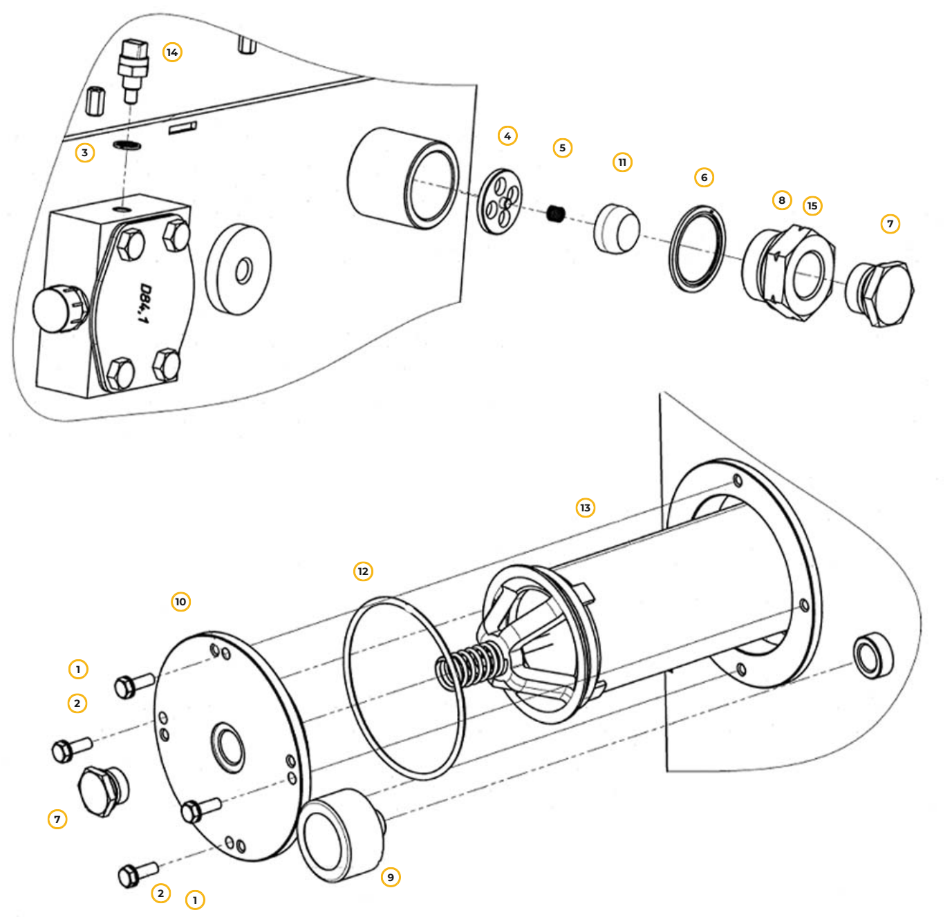
Рис. 42. Бак гидравлический в сборе
