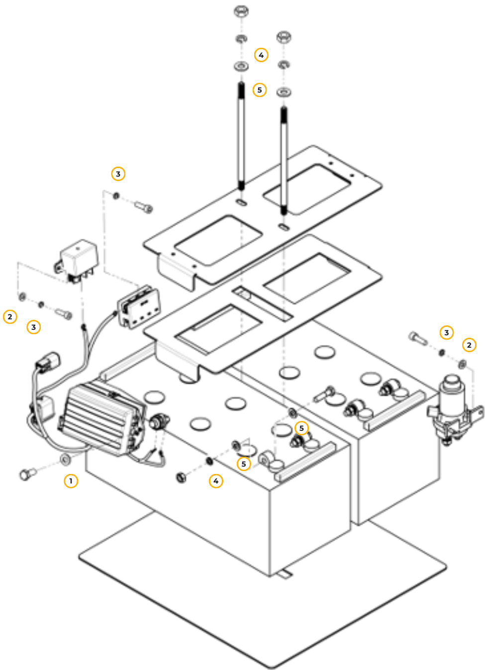
Рис. 68. Аккумуляторные батареи с элементами крепления
