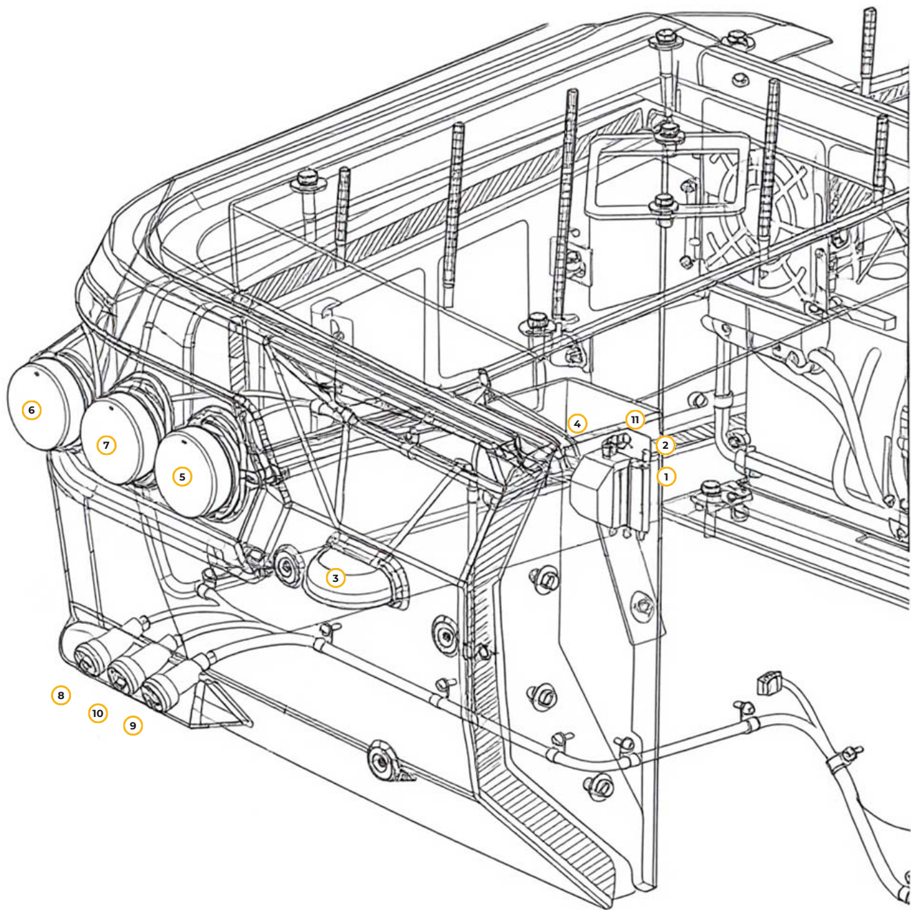
Рис. 72. Заднее электрооборудование рамы
