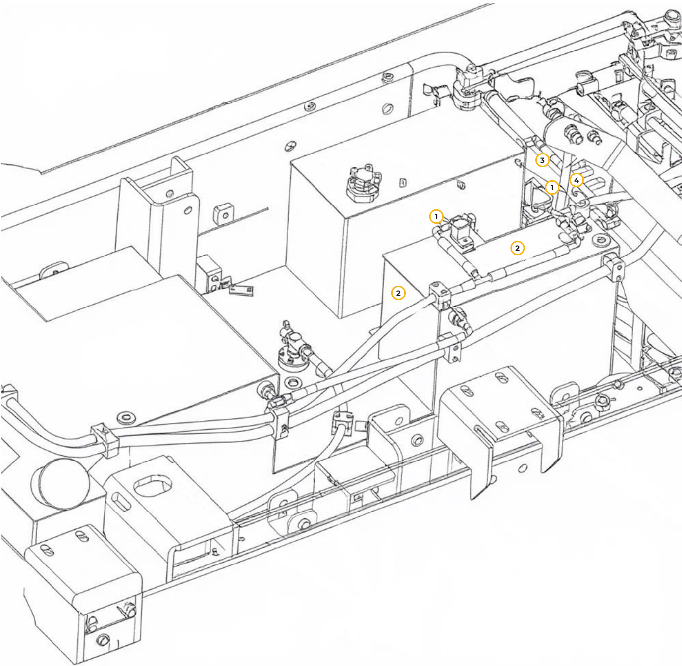
Рис. 11. Система климатическая
