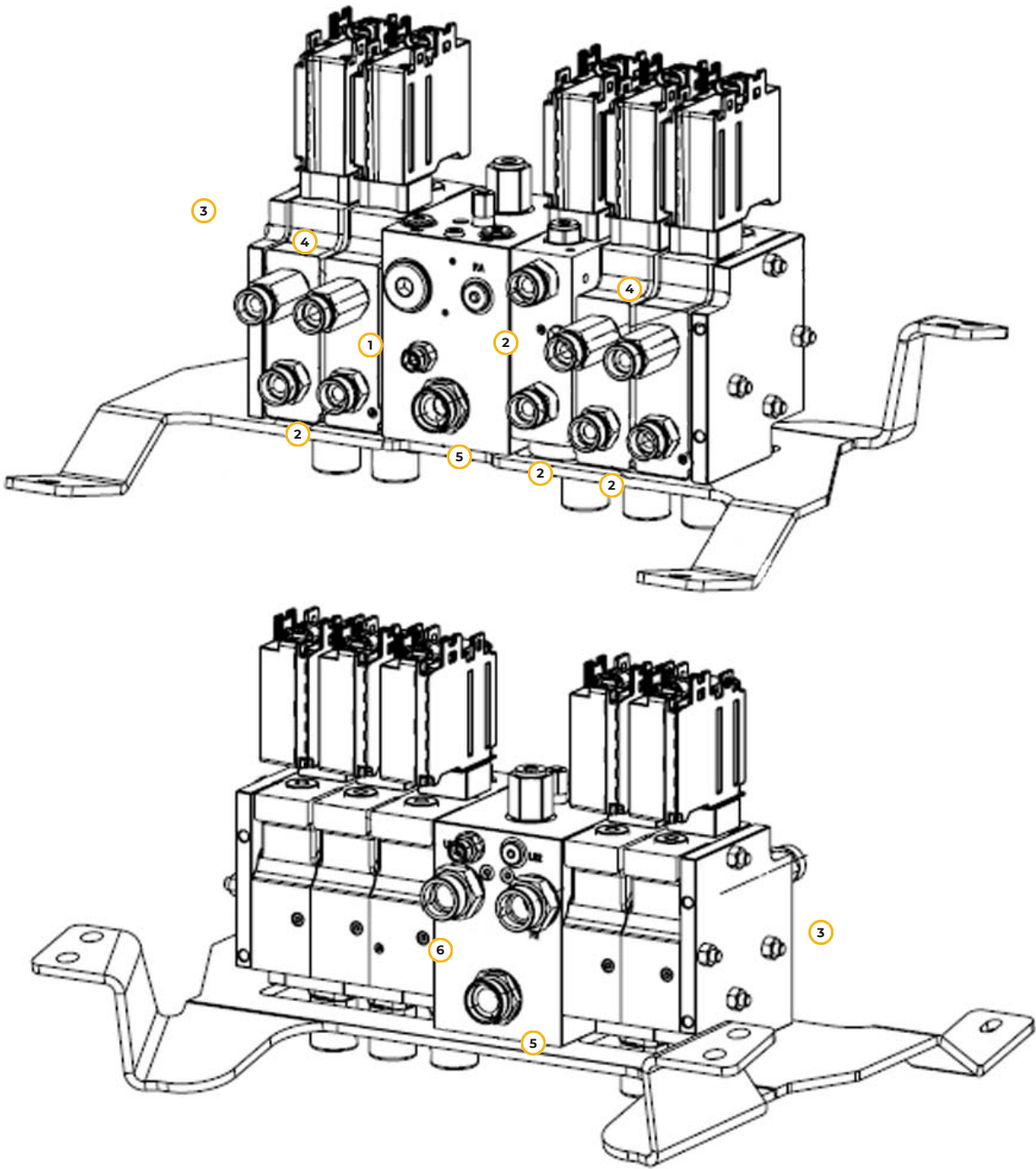
Рис. 37. Гидрораспределитель в сборе
