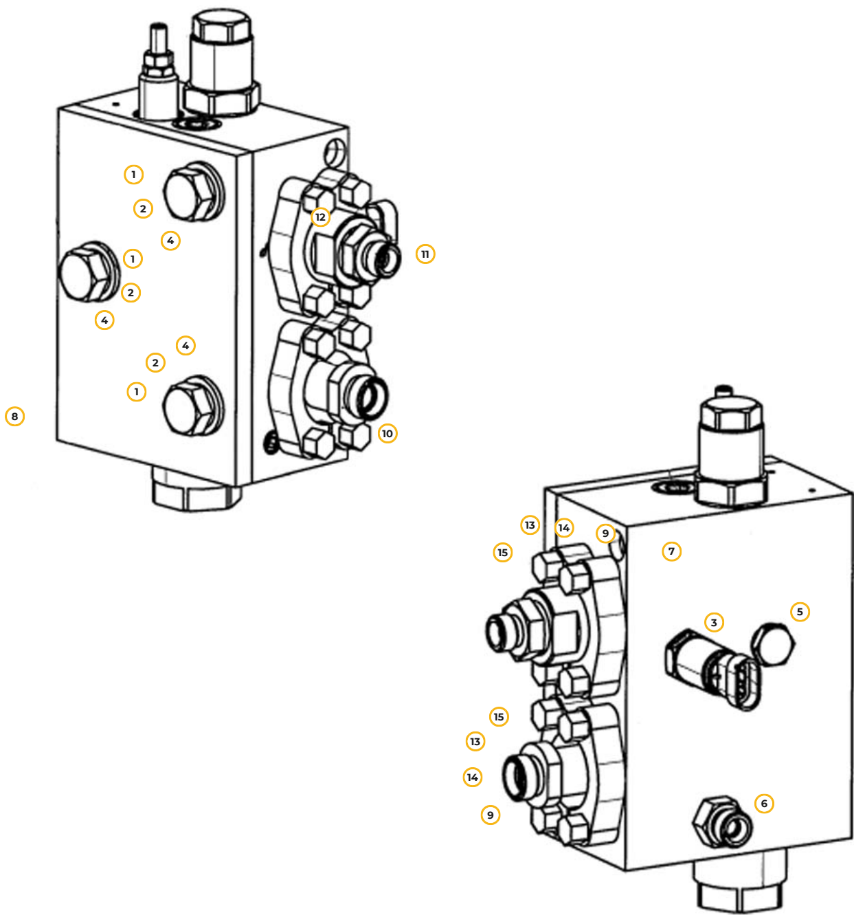
Рис. 38. Блок разгрузки в сборе
