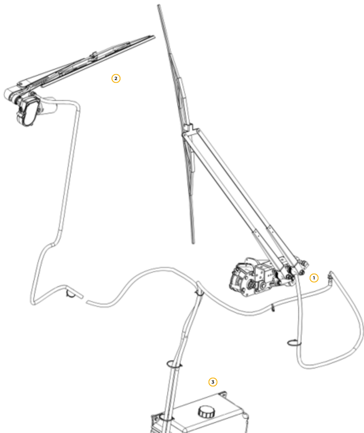
Рис. 85. Стеклоочистители кабины
